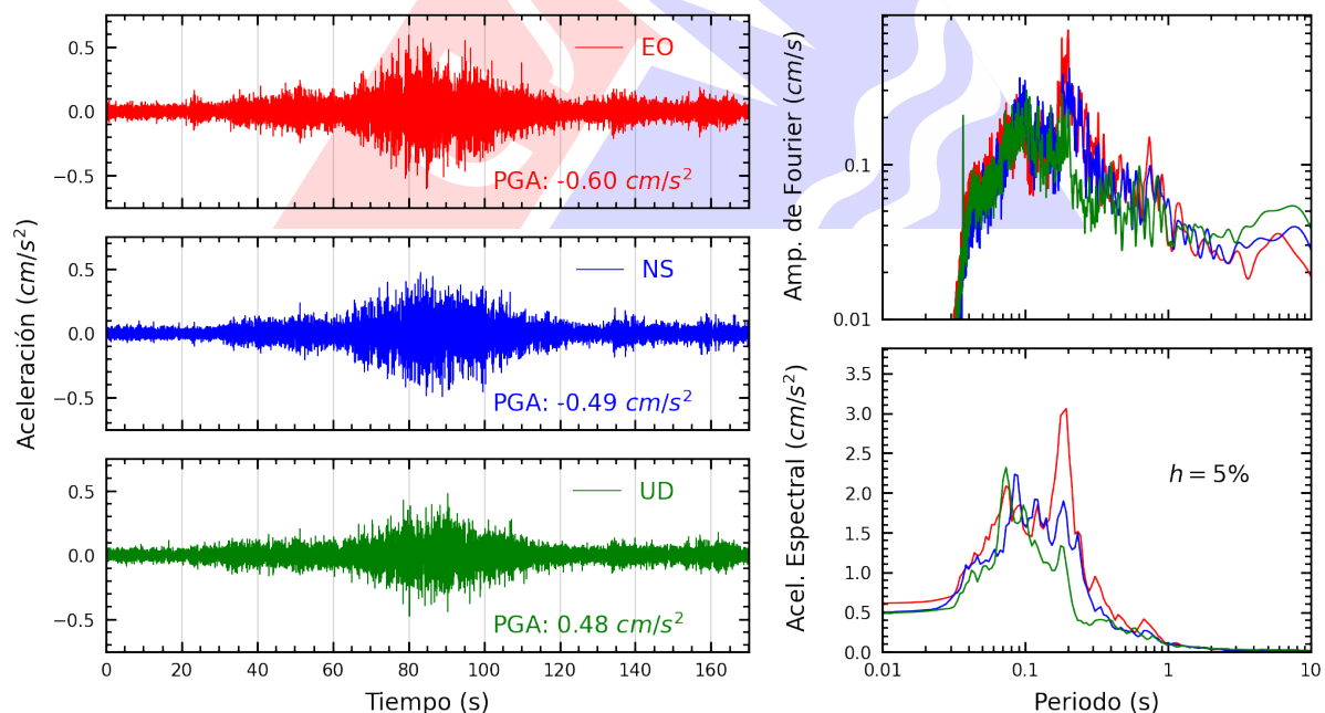
Figura A.16: Registros tiempo-historia, espectros de Fourier y de respuesta en las direcciones EO, NS y vertical de la estación INDEP. Sismo de Marcona, Nazca - Ica del 2025-05-28, 09:34:15 (Hora local)
