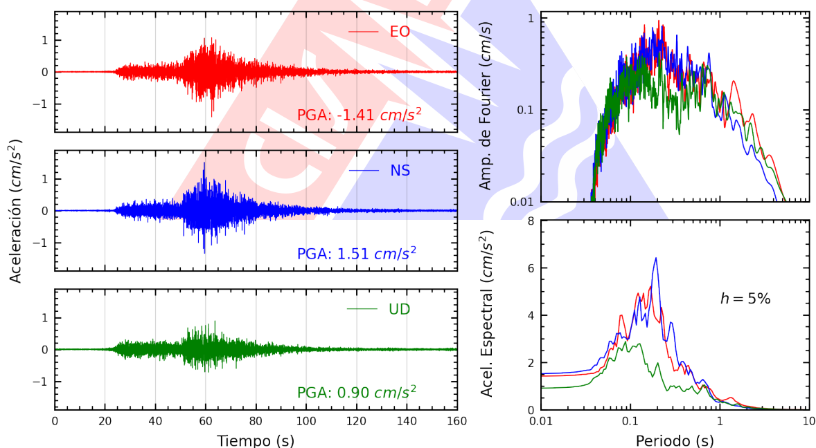
Figura A.2: Registros tiempo-historia, espectros de Fourier y de respuesta en las direcciones EO, NS y vertical de la estación ASIA. Sismo de Marcona, Nazca - Ica del 2025-05-28, 09:34:15 (Hora local)
