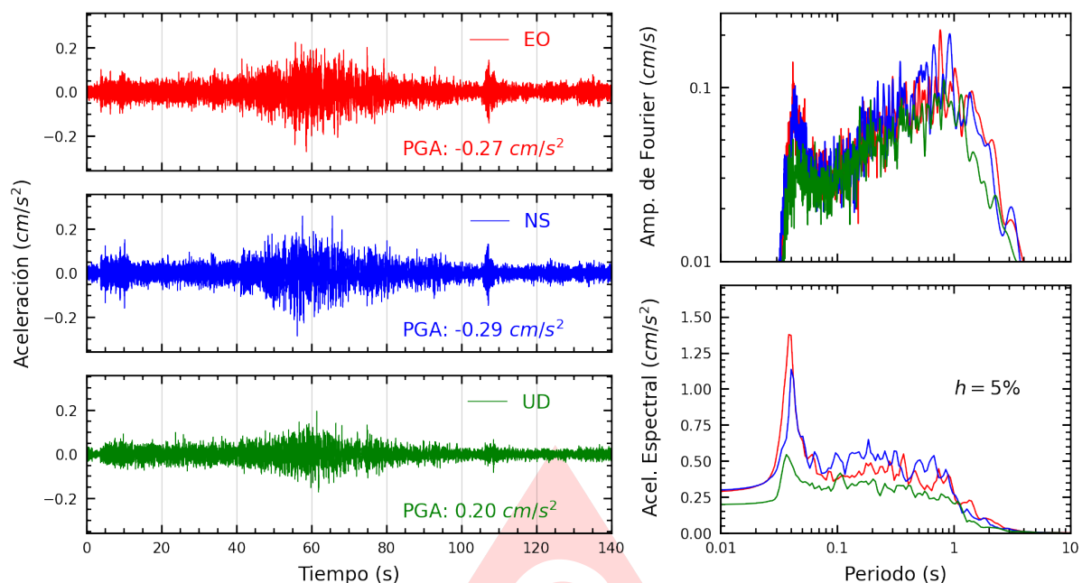
Figura A.35: Registros tiempo-historia, espectros de Fourier y de respuesta en las direcciones EO, NS y vertical de la estación BORJA. Sismo de Marcona, Nazca - Ica del 2025-05-28, 09:34:15 (Hora local)
