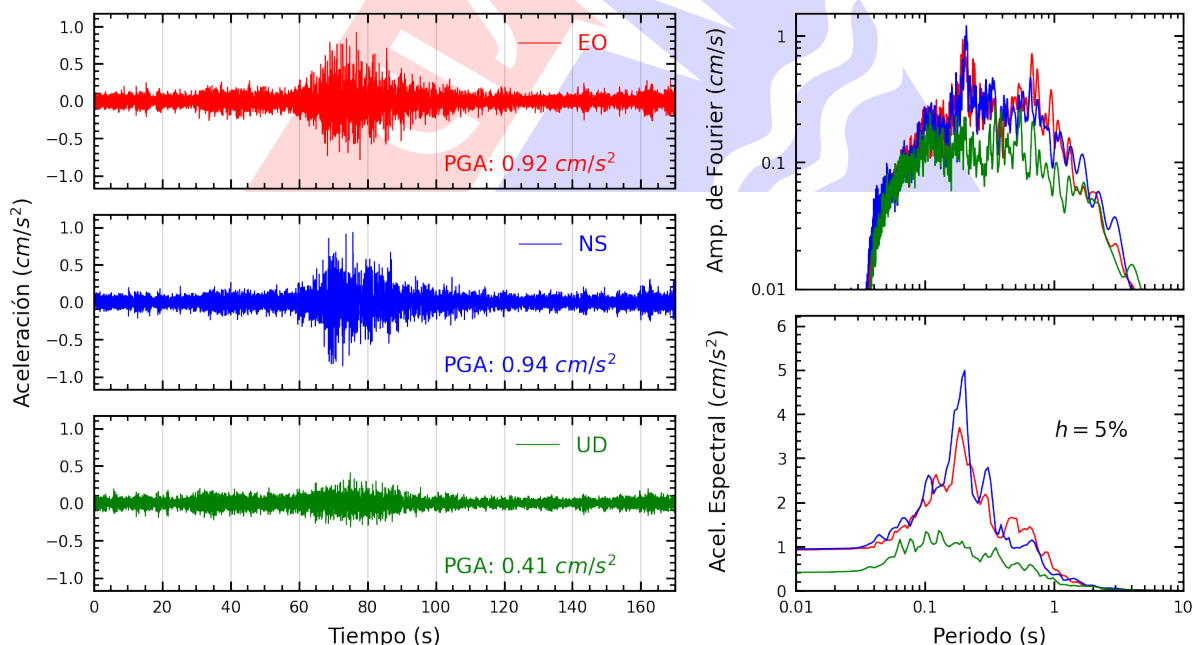
Figura A.6: Registros tiempo-historia, espectros de Fourier y de respuesta en las direcciones EO, NS y vertical de la estación SCCHO. Sismo de Marcona, Nazca - Ica del 2025-05-28, 09:34:15 (Hora local)
