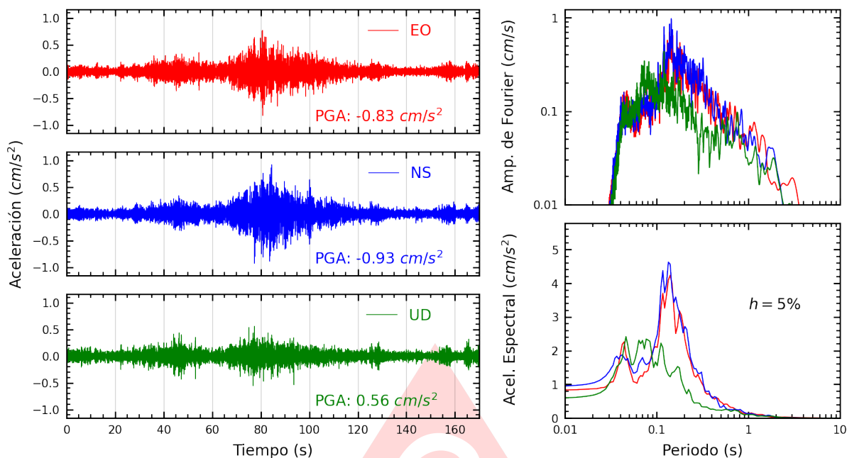
Figura A.9: Registros tiempo-historia, espectros de Fourier y de respuesta en las direcciones EO, NS y vertical de la estación CARA2. Sismo de Marcona, Nazca - Ica del 2025-05-28, 09:34:15 (Hora local)
