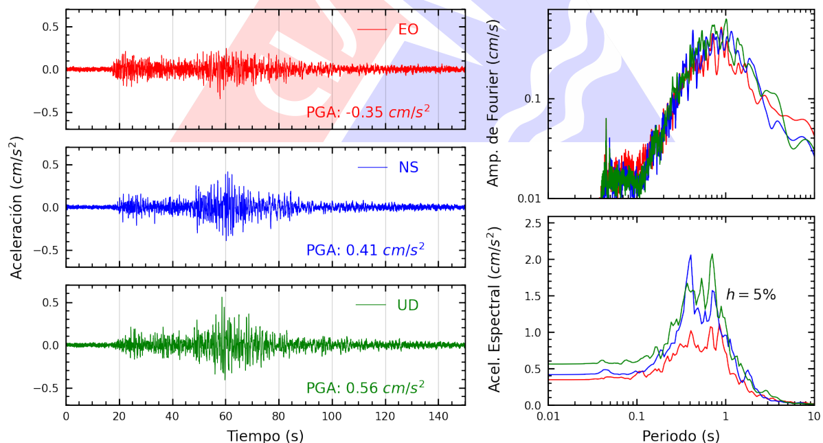
Figura A.22: Registros tiempo-historia, espectros de Fourier y de respuesta en las direcciones EO, NS y vertical de la estación UNSCH. Sismo de Marcona, Nazca - Ica del 2025-05-28, 09:34:15 (Hora local)
