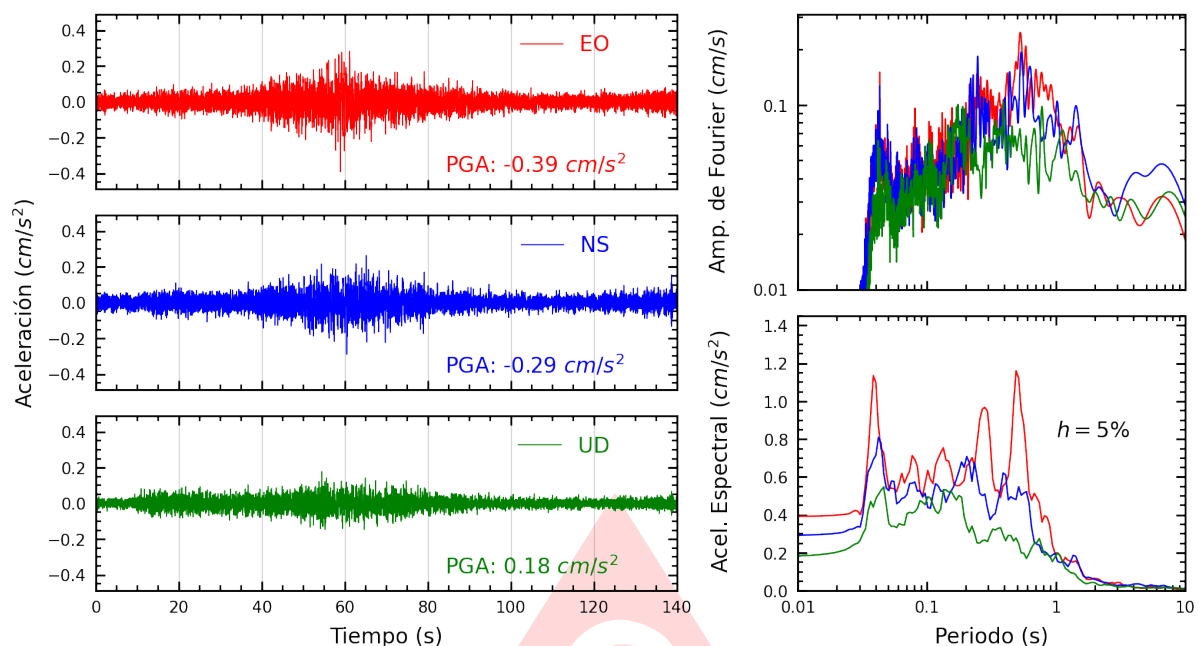
Figura A.27: Registros tiempo-historia, espectros de Fourier y de respuesta en las direcciones EO, NS y vertical de la estación CEPRE. Sismo de Marcona, Nazca - Ica del 2025-05-28, 09:34:15 (Hora local)
