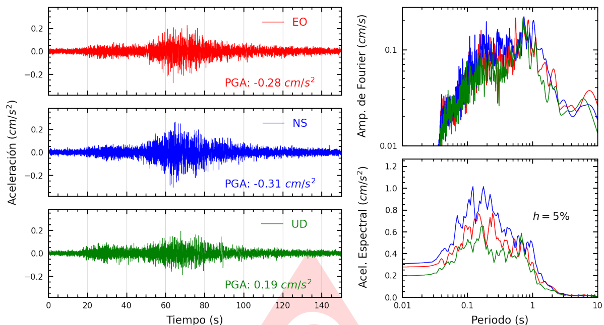
Figura A.33: Registros tiempo-historia, espectros de Fourier y de respuesta en las direcciones EO, NS y vertical de la estación SERVI. Sismo de Marcona, Nazca - Ica del 2025-05-28, 09:34:15 (Hora local)
