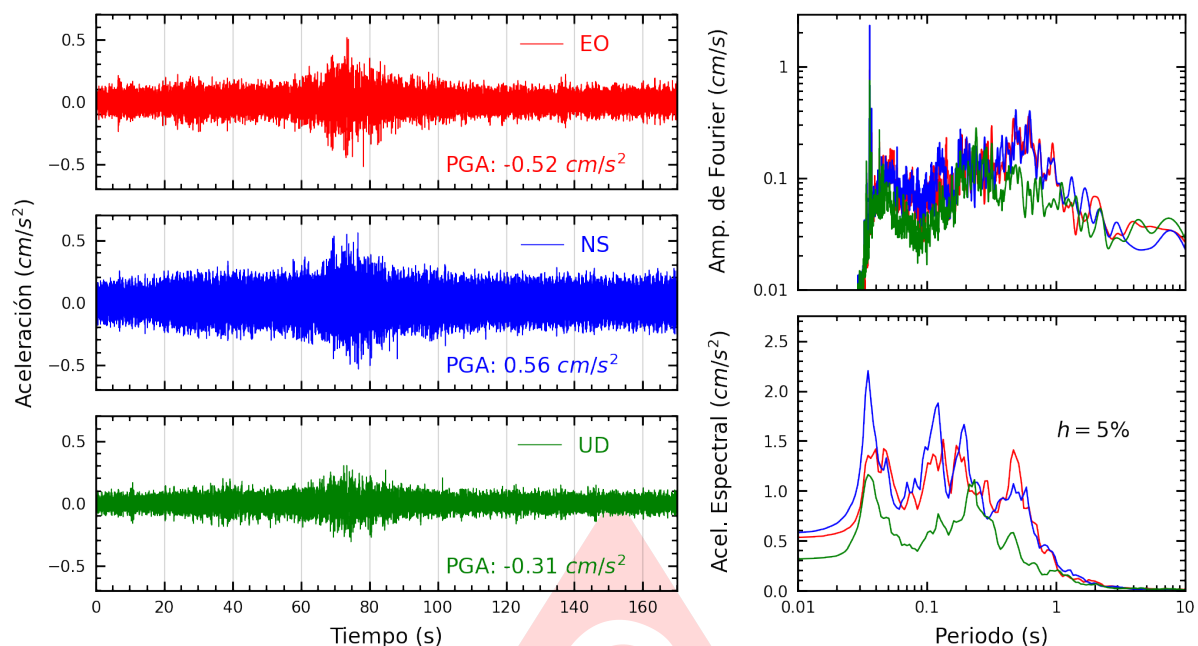
Figura A.21: Registros tiempo-historia, espectros de Fourier y de respuesta en las direcciones EO, NS y vertical de la estación UPCVI. Sismo de Marcona, Nazca - Ica del 2025-05-28, 09:34:15 (Hora local)
