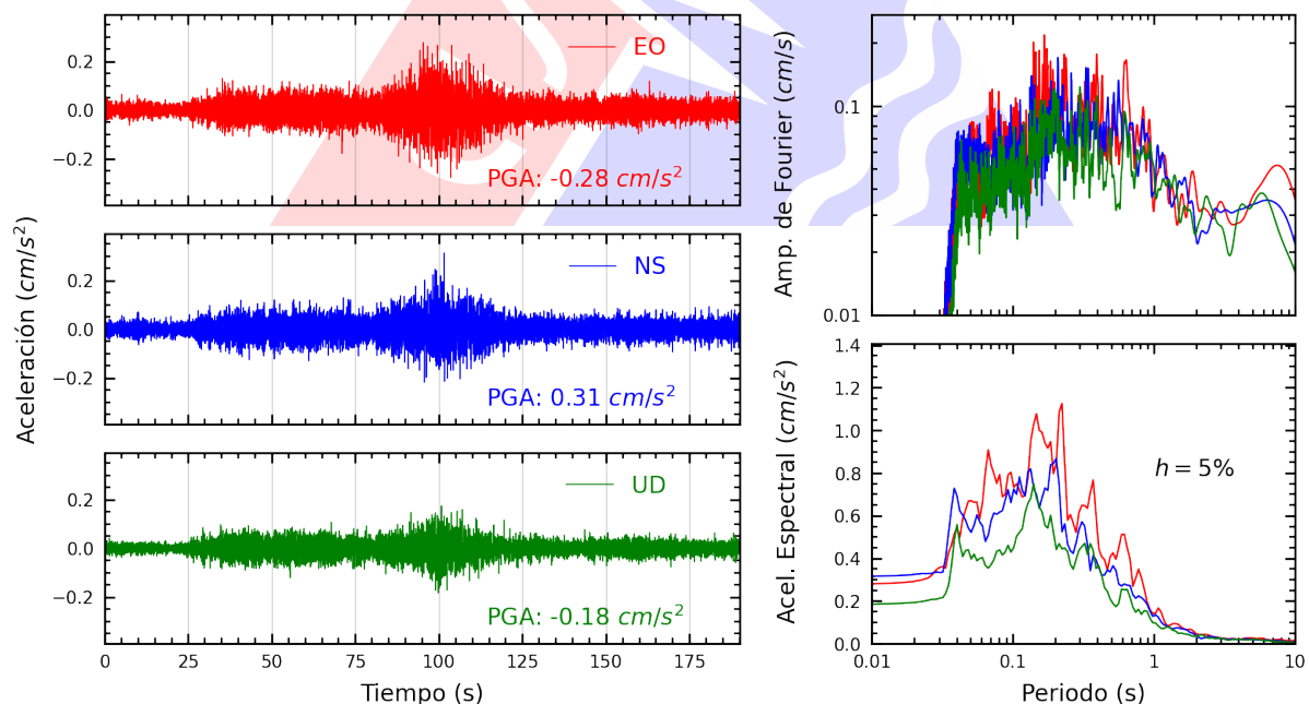
Figura A.32: Registros tiempo-historia, espectros de Fourier y de respuesta en las direcciones EO, NS y vertical de la estación FICPE. Sismo de Marcona, Nazca - Ica del 2025-05-28, 09:34:15 (Hora local)
