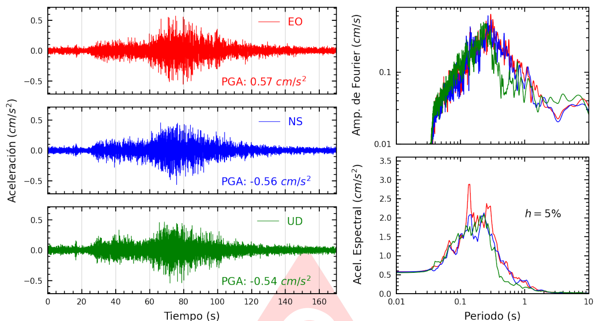
Figura A.19: Registros tiempo-historia, espectros de Fourier y de respuesta en las direcciones EO, NS y vertical de la estación SOVES. Sismo de Marcona, Nazca - Ica del 2025-05-28, 09:34:15 (Hora local)
