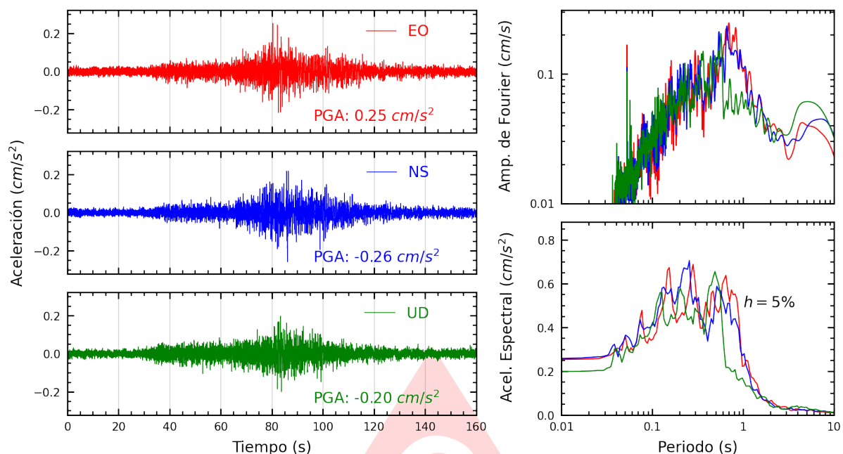
Figura A.39: Registros tiempo-historia, espectros de Fourier y de respuesta en las direcciones EO, NS y vertical de la estación UNMSM. Sismo de Marcona, Nazca - Ica del 2025-05-28, 09:34:15 (Hora local)
