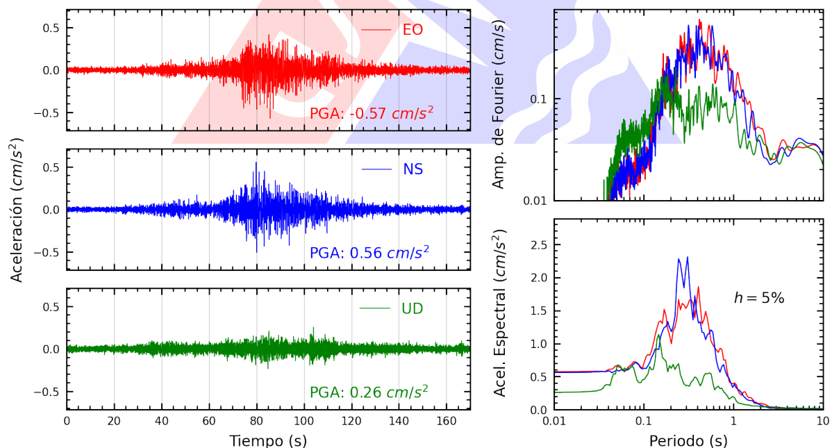
Figura A.20: Registros tiempo-historia, espectros de Fourier y de respuesta en las direcciones EO, NS y vertical de la estación ACAPU. Sismo de Marcona, Nazca - Ica del 2025-05-28, 09:34:15 (Hora local)
