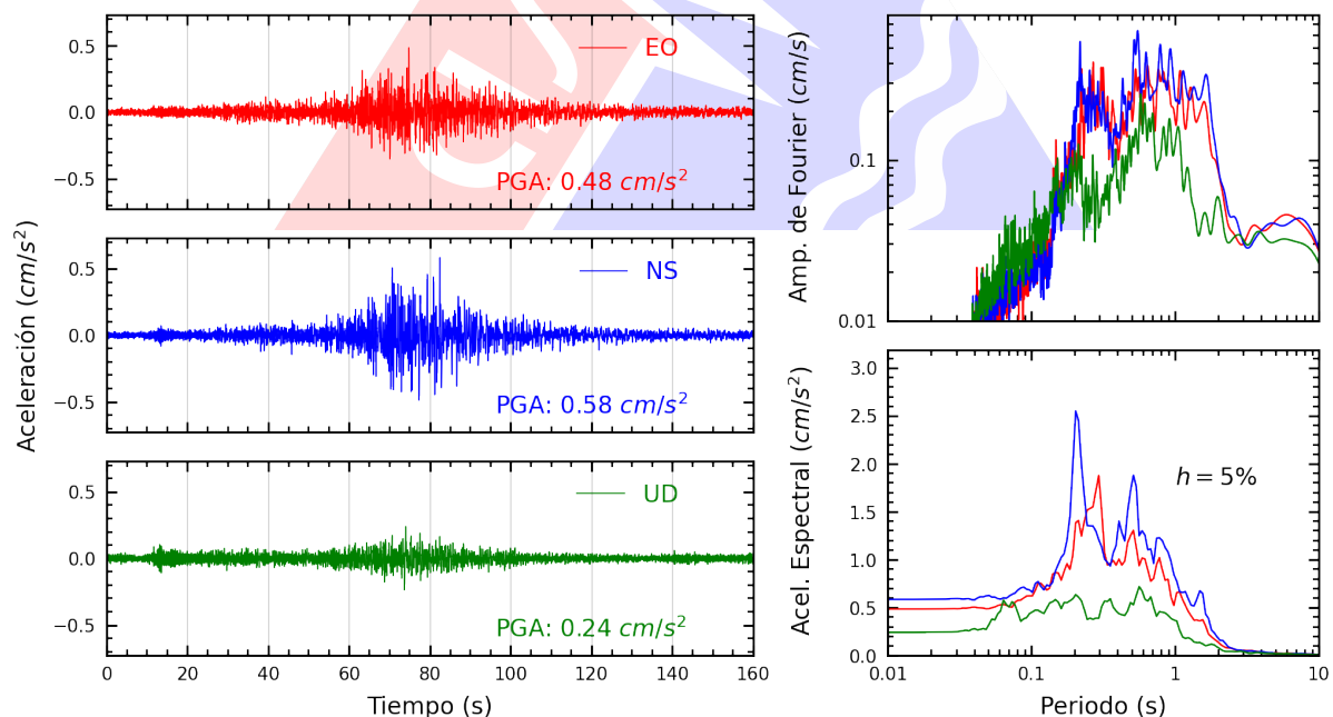
Figura A.18: Registros tiempo-historia, espectros de Fourier y de respuesta en las direcciones EO, NS y vertical de la estación DSMI. Sismo de Marcona, Nazca - Ica del 2025-05-28, 09:34:15 (Hora local)
