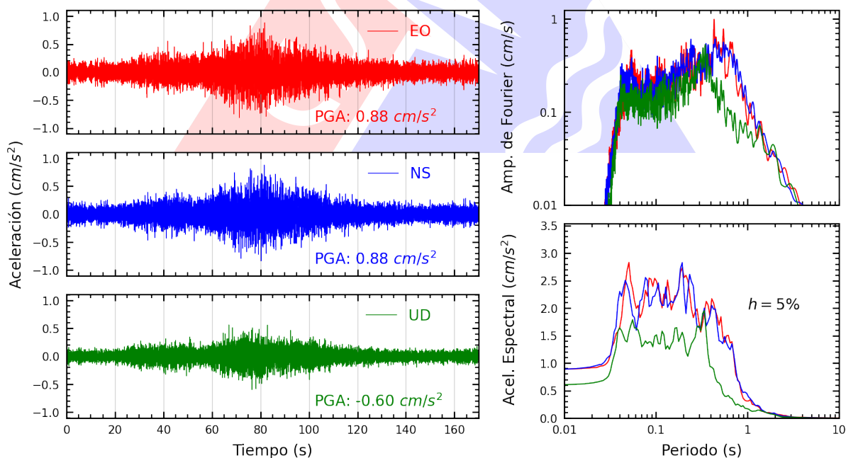
Figura A.10: Registros tiempo-historia, espectros de Fourier y de respuesta en las direcciones EO, NS y vertical de la estación UNTEL. Sismo de Marcona, Nazca - Ica del 2025-05-28, 09:34:15 (Hora local)
