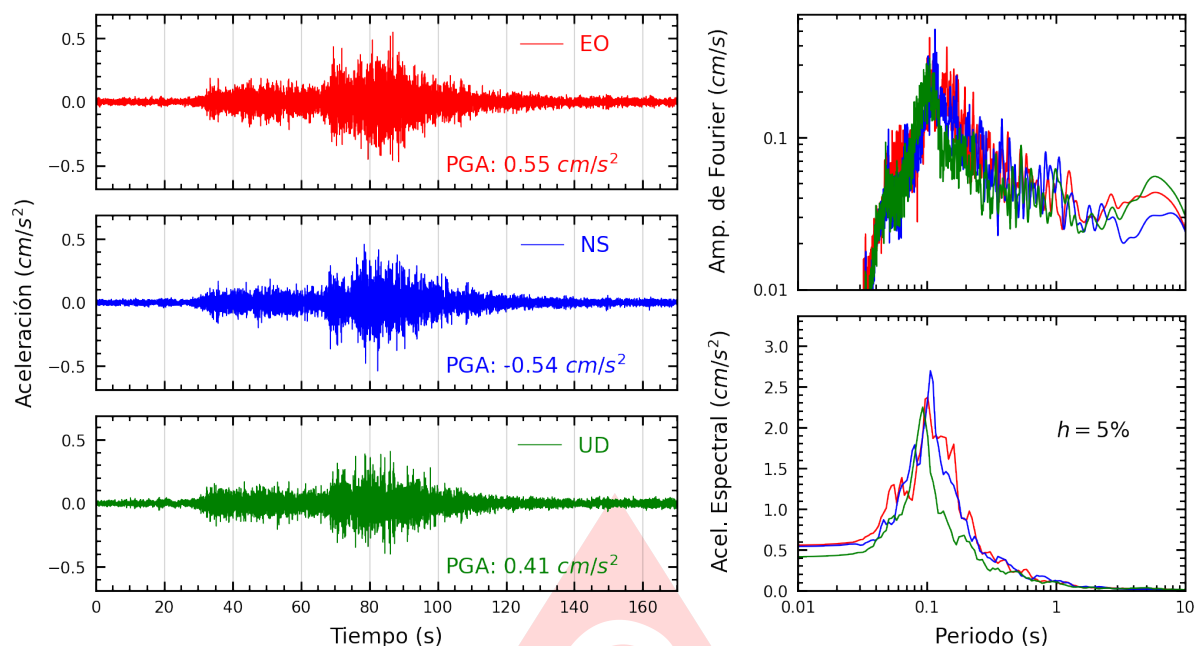
Figura A.23: Registros tiempo-historia, espectros de Fourier y de respuesta en las direcciones EO, NS y vertical de la estación AMORE. Sismo de Marcona, Nazca - Ica del 2025-05-28, 09:34:15 (Hora local)
