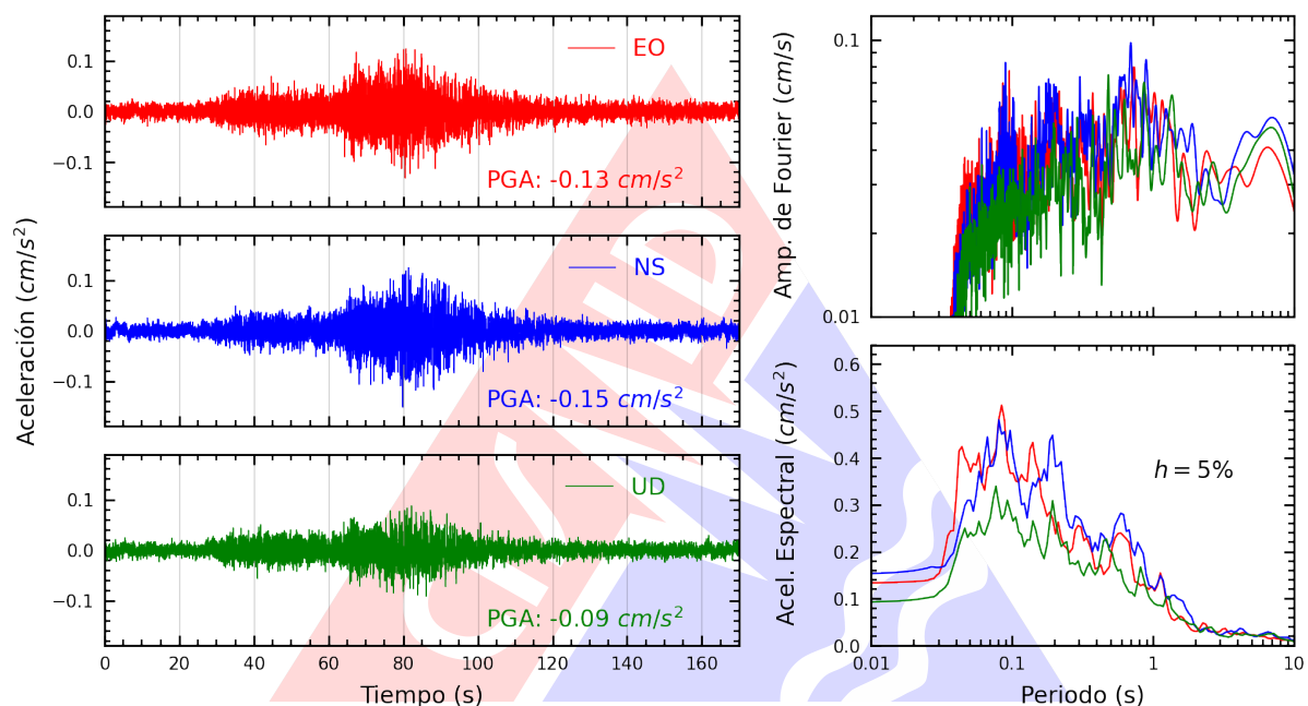
Figura A.41: Registros tiempo-historia, espectros de Fourier y de respuesta en las direcciones EO, NS y vertical de la estación UCSS. Sismo de Marcona, Nazca - Ica del 2025-05-28, 09:34:15 (Hora local)
