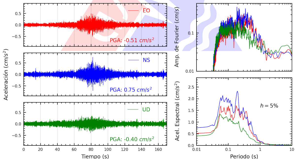
Figura A.14: Registros tiempo-historia, espectros de Fourier y de respuesta en las direcciones EO, NS y vertical de la estación SJLSC. Sismo de Marcona, Nazca - Ica del 2025-05-28, 09:34:15 (Hora local)
