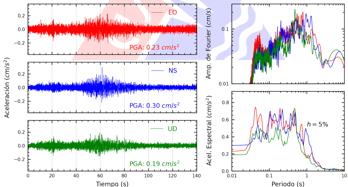
Figura A.34: Registros tiempo-historia, espectros de Fourier y de respuesta en las direcciones EO, NS y vertical de la estación INICT. Sismo de Marcona, Nazca - Ica del 2025-05-28, 09:34:15 (Hora local)
