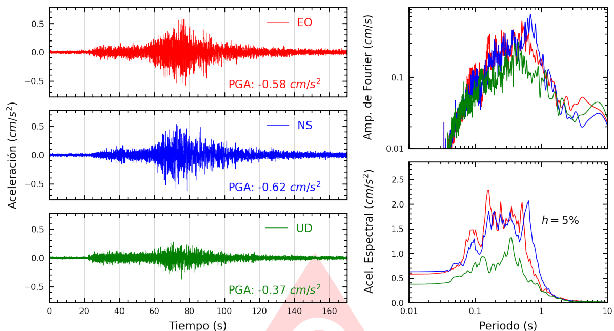
Figura A.15: Registros tiempo-historia, espectros de Fourier y de respuesta en las direcciones EO, NS y vertical de la estación USILP. Sismo de Marcona, Nazca - Ica del 2025-05-28, 09:34:15 (Hora local)
