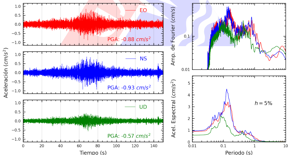
Figura A.8: Registros tiempo-historia, espectros de Fourier y de respuesta en las direcciones EO, NS y vertical de la estación USILM. Sismo de Marcona, Nazca - Ica del 2025-05-28, 09:34:15 (Hora local)
