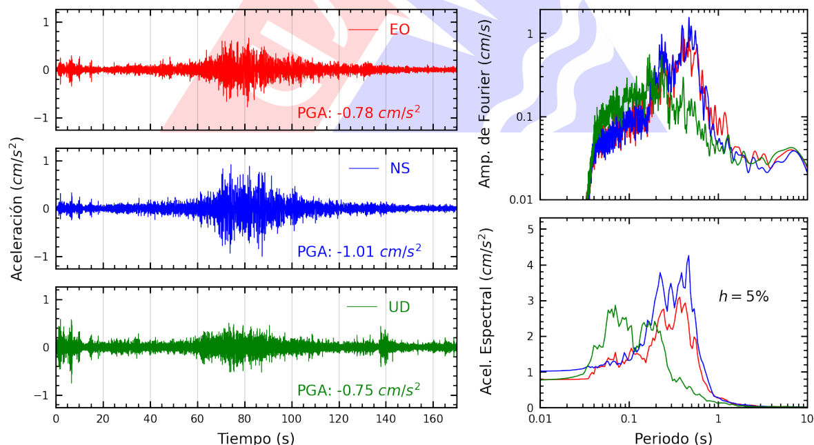
Figura A.4: Registros tiempo-historia, espectros de Fourier y de respuesta en las direcciones EO, NS y vertical de la estación MDPP. Sismo de Marcona, Nazca - Ica del 2025-05-28, 09:34:15 (Hora local)
