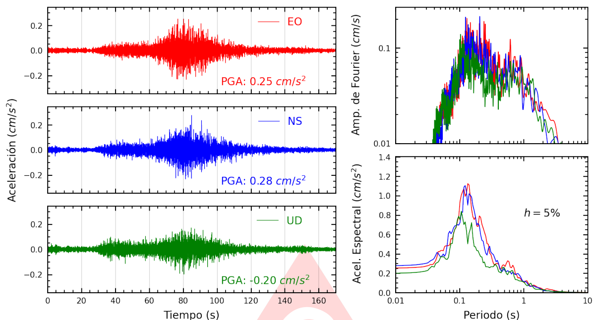
Figura A.37: Registros tiempo-historia, espectros de Fourier y de respuesta en las direcciones EO, NS y vertical de la estación JALV2. Sismo de Marcona, Nazca - Ica del 2025-05-28, 09:34:15 (Hora local)
