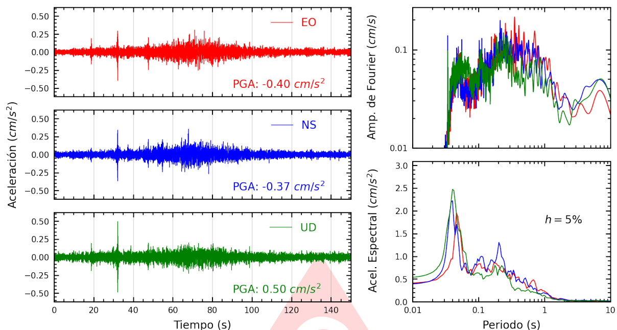
Figura A.25: Registros tiempo-historia, espectros de Fourier y de respuesta en las direcciones EO, NS y vertical de la estación USMP. Sismo de Marcona, Nazca - Ica del 2025-05-28, 09:34:15 (Hora local)
