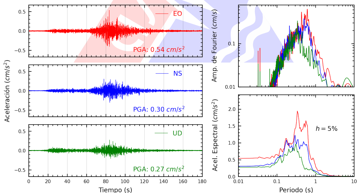
Figura A.24: Registros tiempo-historia, espectros de Fourier y de respuesta en las direcciones EO, NS y vertical de la estación CARAL. Sismo de Marcona, Nazca - Ica del 2025-05-28, 09:34:15 (Hora local)
