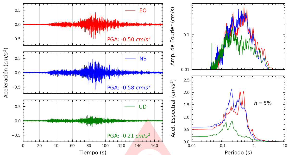
Figura A.17: Registros tiempo-historia, espectros de Fourier y de respuesta en las direcciones EO, NS y vertical de la estación VHAY2. Sismo de Marcona, Nazca - Ica del 2025-05-28, 09:34:15 (Hora local)
