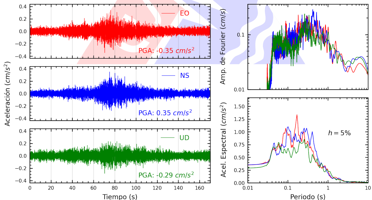
Figura A.30: Registros tiempo-historia, espectros de Fourier y de respuesta en las direcciones EO, NS y vertical de la estación URPPE. Sismo de Marcona, Nazca - Ica del 2025-05-28, 09:34:15 (Hora local)
