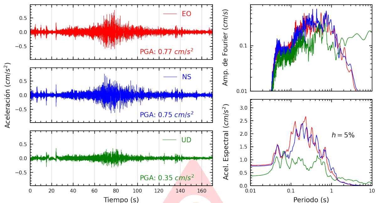
Figura A.13: Registros tiempo-historia, espectros de Fourier y de respuesta en las direcciones EO, NS y vertical de la estación BRISA. Sismo de Marcona, Nazca - Ica del 2025-05-28, 09:34:15 (Hora local)
