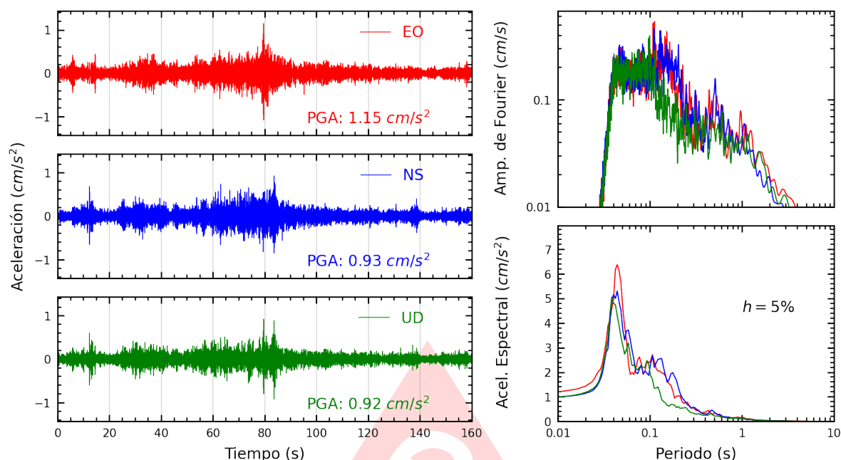
Figura A.3: Registros tiempo-historia, espectros de Fourier y de respuesta en las direcciones EO, NS y vertical de la estación SROS2. Sismo de Marcona, Nazca - Ica del 2025-05-28, 09:34:15 (Hora local)
