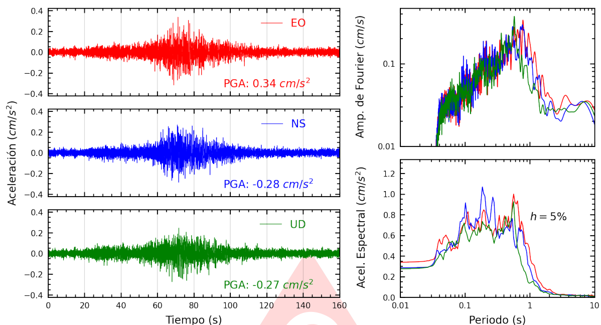
Figura A.31: Registros tiempo-historia, espectros de Fourier y de respuesta en las direcciones EO, NS y vertical de la estación IMCA. Sismo de Marcona, Nazca - Ica del 2025-05-28, 09:34:15 (Hora local)
