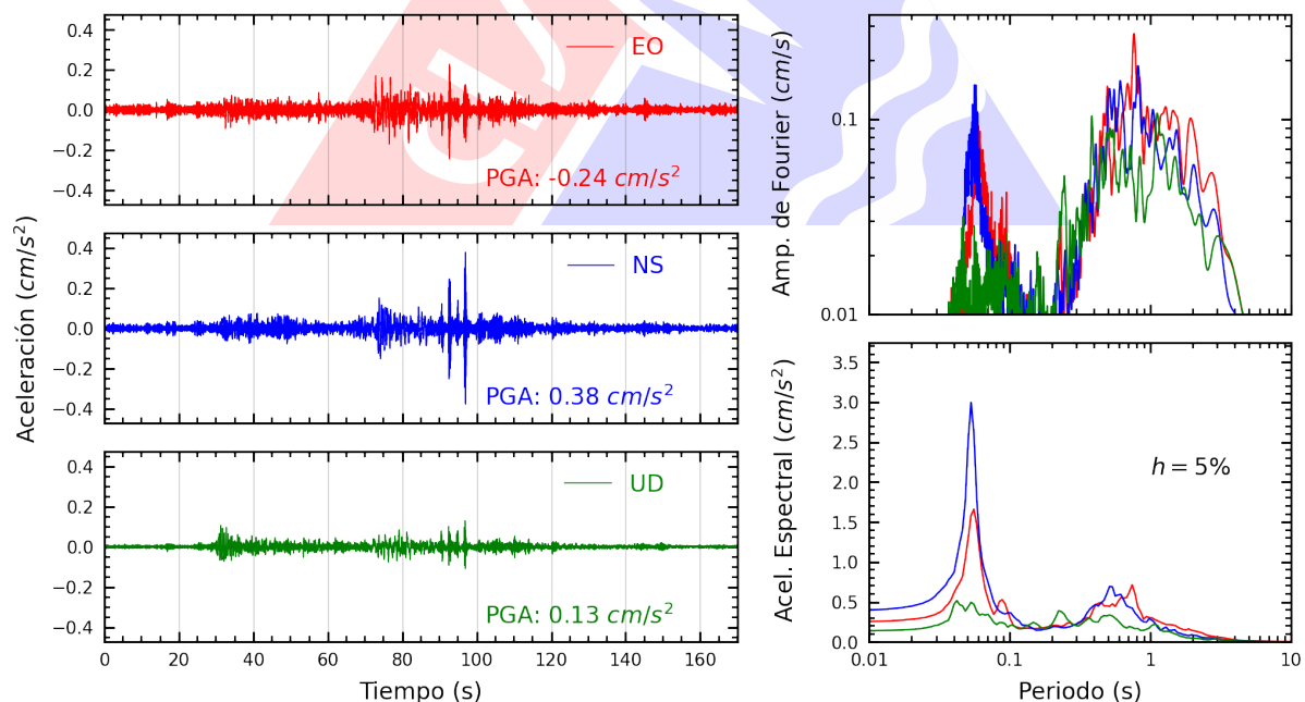
Figura A.28: Registros tiempo-historia, espectros de Fourier y de respuesta en las direcciones EO, NS y vertical de la estación UNMBA. Sismo de Marcona, Nazca - Ica del 2025-05-28, 09:34:15 (Hora local)
