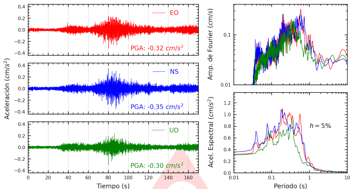
Figura A.29: Registros tiempo-historia, espectros de Fourier y de respuesta en las direcciones EO, NS y vertical de la estación COMAS. Sismo de Marcona, Nazca - Ica del 2025-05-28, 09:34:15 (Hora local)
