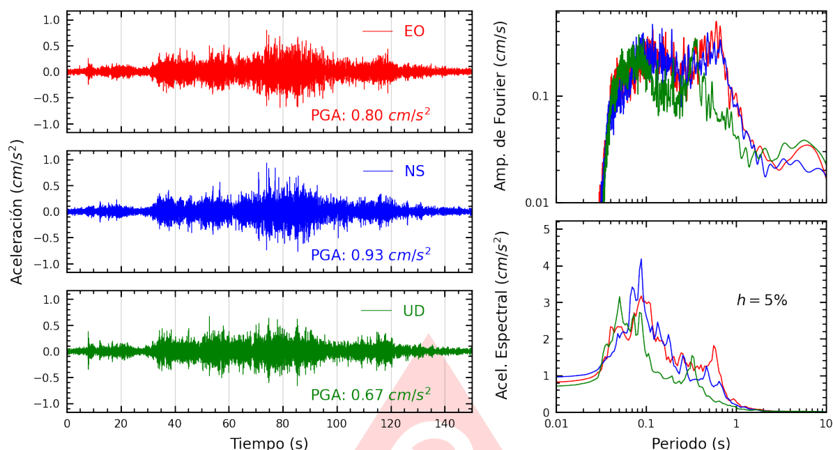
Figura A.7: Registros tiempo-historia, espectros de Fourier y de respuesta en las direcciones EO, NS y vertical de la estación SJLSV. Sismo de Marcona, Nazca - Ica del 2025-05-28, 09:34:15 (Hora local)
