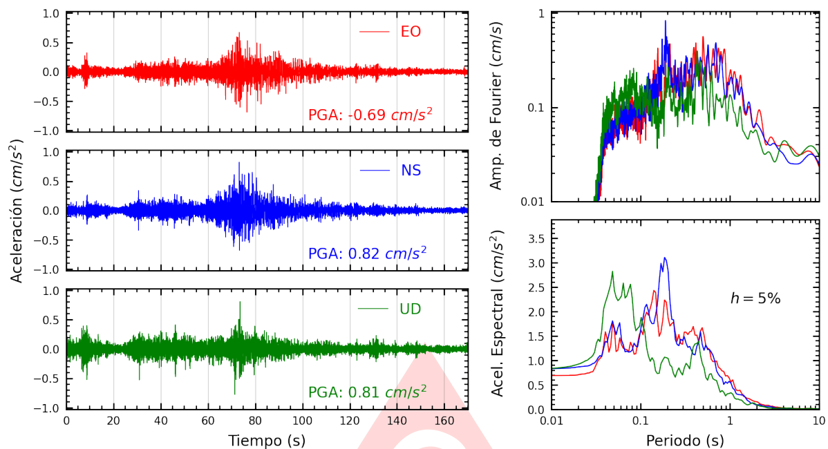
Figura A.11: Registros tiempo-historia, espectros de Fourier y de respuesta en las direcciones EO, NS y vertical de la estación SOCHO. Sismo de Marcona, Nazca - Ica del 2025-05-28, 09:34:15 (Hora local)
