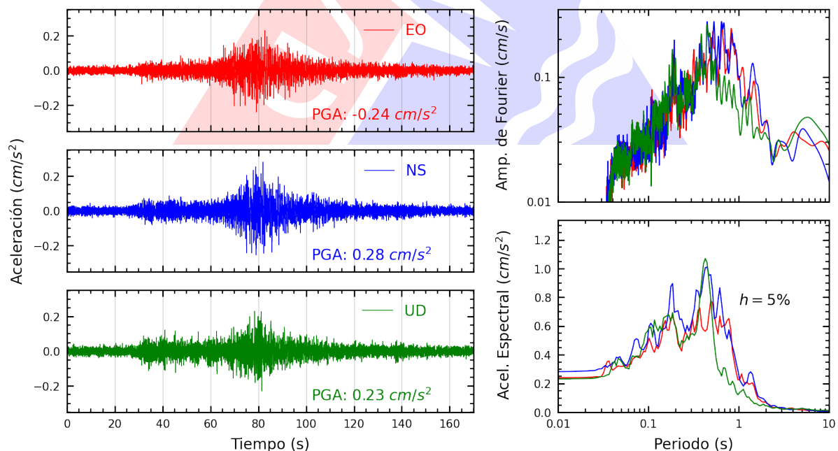
Figura A.36: Registros tiempo-historia, espectros de Fourier y de respuesta en las direcciones EO, NS y vertical de la estación UNFV. Sismo de Marcona, Nazca - Ica del 2025-05-28, 09:34:15 (Hora local)
