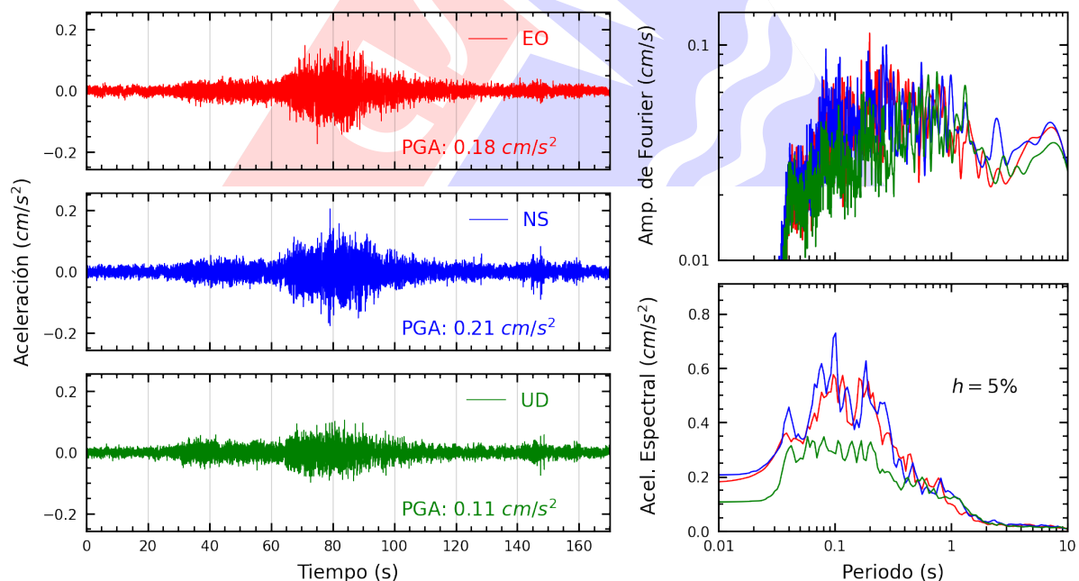
Figura A.40: Registros tiempo-historia, espectros de Fourier y de respuesta en las direcciones EO, NS y vertical de la estación SJLCE. Sismo de Marcona, Nazca - Ica del 2025-05-28, 09:34:15 (Hora local)
