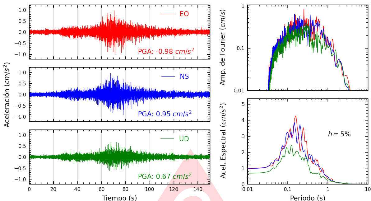
Figura A.5: Registros tiempo-historia, espectros de Fourier y de respuesta en las direcciones EO, NS y vertical de la estación PHER2. Sismo de Marcona, Nazca - Ica del 2025-05-28, 09:34:15 (Hora local)
