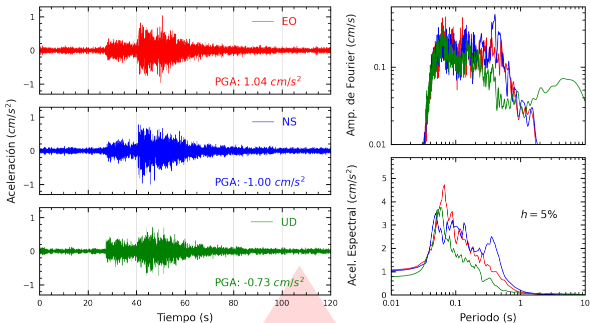
Figura A.1: Registros tiempo-historia, espectros de Fourier y de respuesta en las direcciones EO, NS y vertical de la estación SCARQ. Sismo de Vitor, Arequipa - Arequipa del 2025-05-28, 18:19:39 (Hora local)
