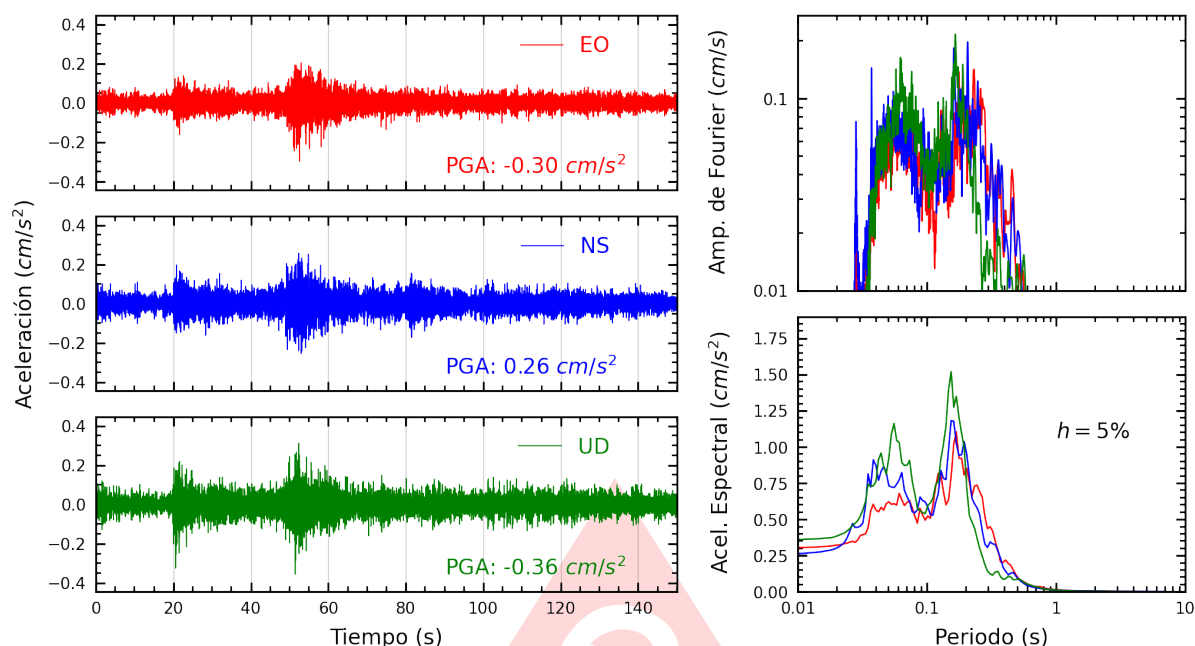
Figura A.5: Registros tiempo-historia, espectros de Fourier y de respuesta en las direcciones EO, NS y vertical de la estación UJBG4. Sismo de Vitor, Arequipa - Arequipa del 2025-05-28, 18:19:39 (Hora local)
