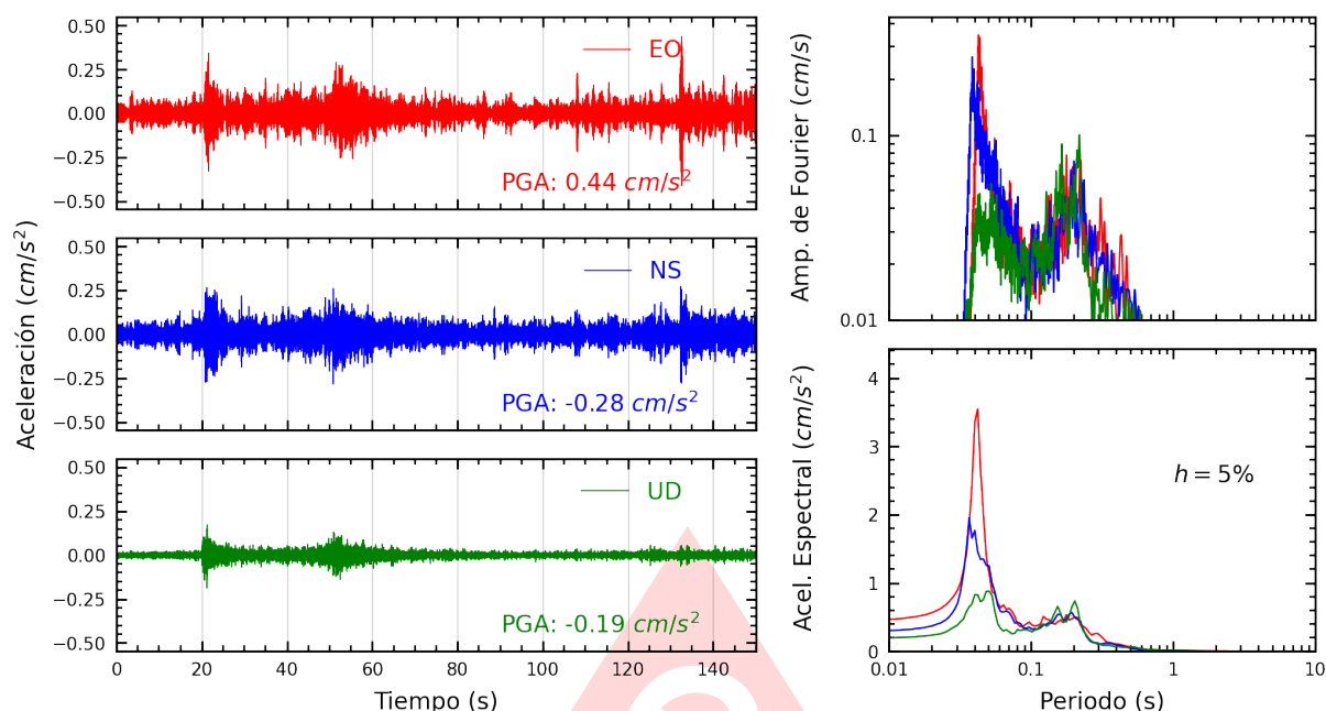
Figura A.3: Registros tiempo-historia, espectros de Fourier y de respuesta en las direcciones EO, NS y vertical de la estación UPTAC. Sismo de Vitor, Arequipa - Arequipa del 2025-05-28, 18:19:39 (Hora local)
