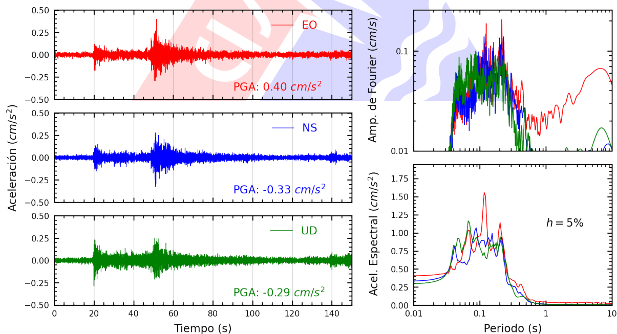
Figura A.4: Registros tiempo-historia, espectros de Fourier y de respuesta en las direcciones EO, NS y vertical de la estación UJBG3. Sismo de Vitor, Arequipa - Arequipa del 2025-05-28, 18:19:39 (Hora local)
