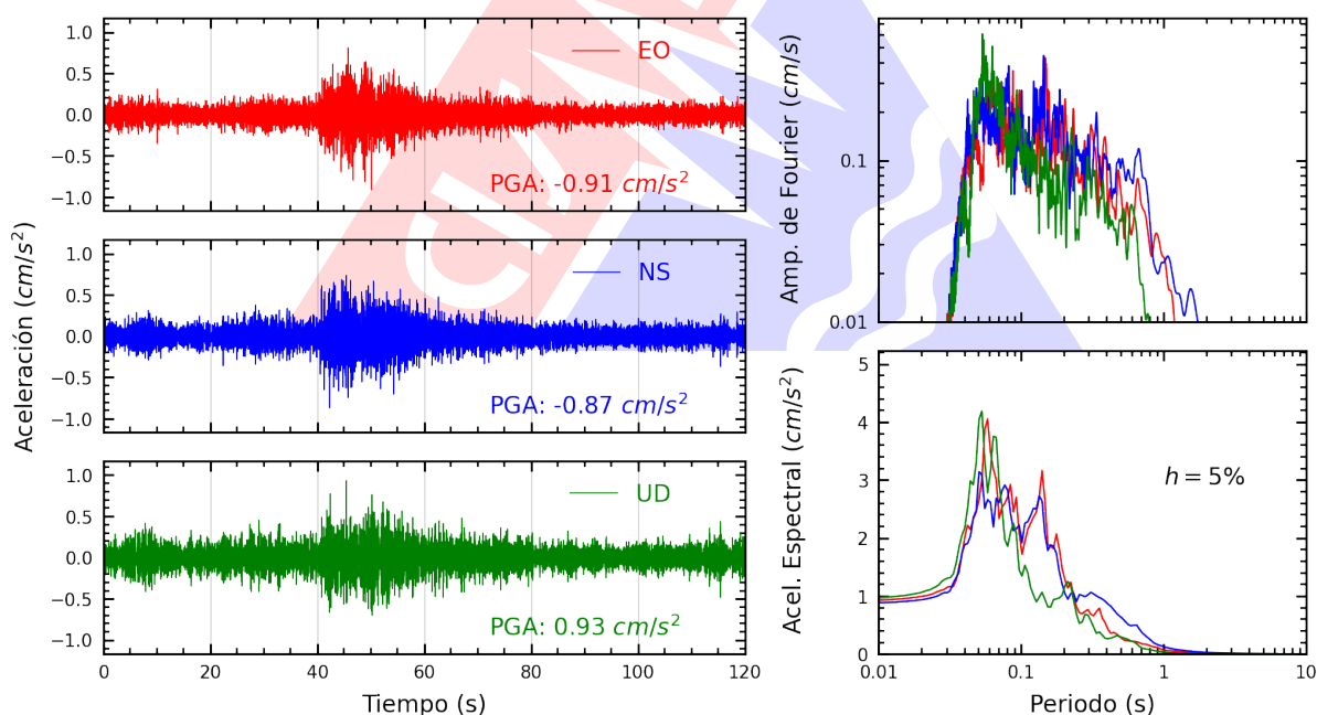
Figura A.2: Registros tiempo-historia, espectros de Fourier y de respuesta en las direcciones EO, NS y vertical de la estación SCAR2. Sismo de Vitor, Arequipa - Arequipa del 2025-05-28, 18:19:39 (Hora local)
