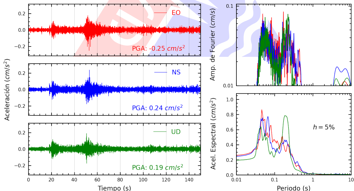
Figura A.6: Registros tiempo-historia, espectros de Fourier y de respuesta en las direcciones EO, NS y vertical de la estación CREY. Sismo de Vitor, Arequipa - Arequipa del 2025-05-28, 18:19:39 (Hora local)
