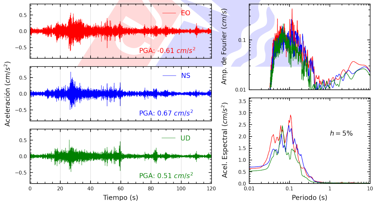
Figura A.36: Registros tiempo-historia, espectros de Fourier y de respuesta en las direcciones EO, NS y vertical de la estación SOBAR. Sismo de Lima, Lima - Lima del 2025-06-02, 00:34:43 (Hora local)
