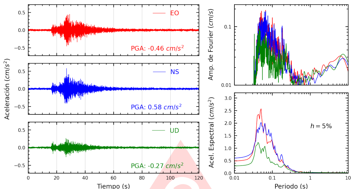
Figura A.41: Registros tiempo-historia, espectros de Fourier y de respuesta en las direcciones EO, NS y vertical de la estación UPCVI. Sismo de Lima, Lima - Lima del 2025-06-02, 00:34:43 (Hora local)
