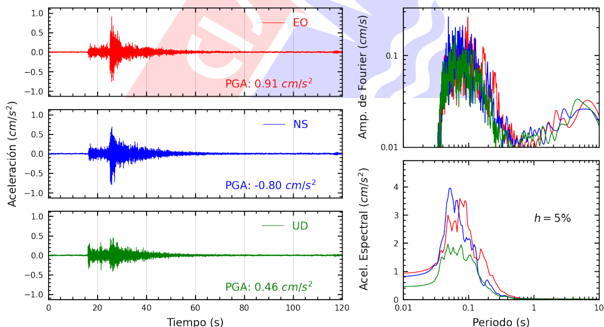
Figura A.26: Registros tiempo-historia, espectros de Fourier y de respuesta en las direcciones EO, NS y vertical de la estación SERVI. Sismo de Lima, Lima - Lima del 2025-06-02, 00:34:43 (Hora local)
