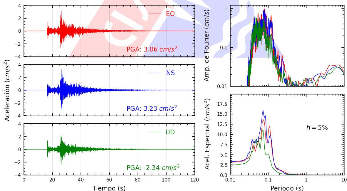
Figura A.4: Registros tiempo-historia, espectros de Fourier y de respuesta en las direcciones EO, NS y vertical de la estación JOSEO. Sismo de Lima, Lima - Lima del 2025-06-02, 00:34:43 (Hora local)
