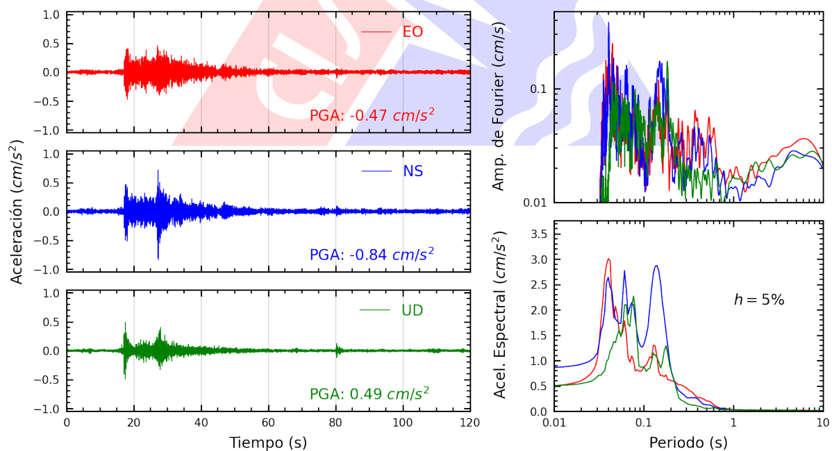
Figura A.28: Registros tiempo-historia, espectros de Fourier y de respuesta en las direcciones EO, NS y vertical de la estación DHNPE. Sismo de Lima, Lima - Lima del 2025-06-02, 00:34:43 (Hora local)
