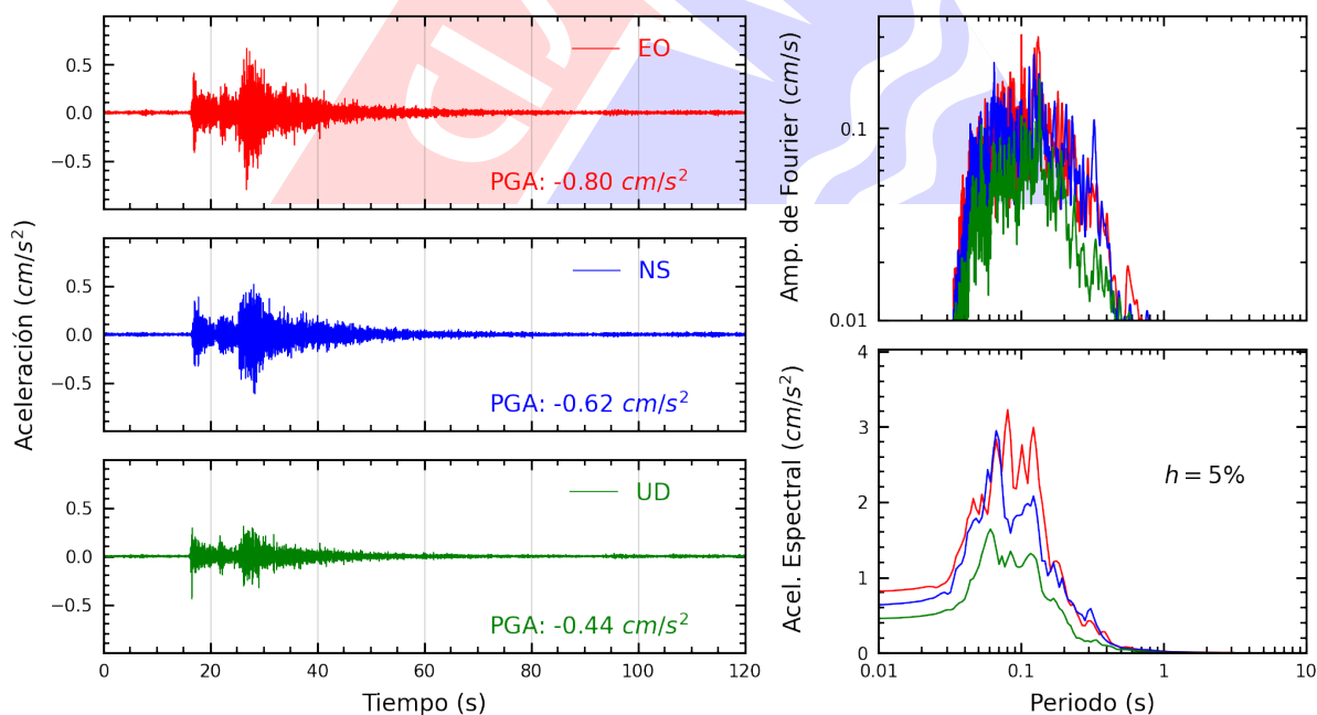
Figura A.30: Registros tiempo-historia, espectros de Fourier y de respuesta en las direcciones EO, NS y vertical de la estación BRIS2. Sismo de Lima, Lima - Lima del 2025-06-02, 00:34:43 (Hora local)
