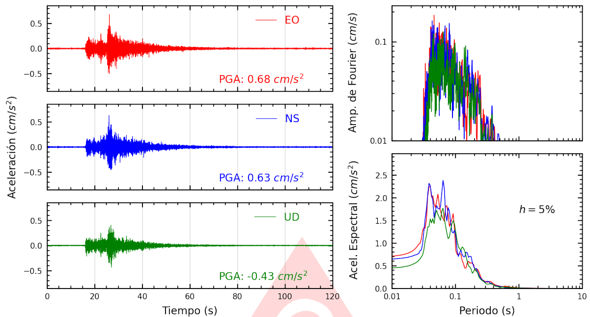
Figura A.35: Registros tiempo-historia, espectros de Fourier y de respuesta en las direcciones EO, NS y vertical de la estación BORJA. Sismo de Lima, Lima - Lima del 2025-06-02, 00:34:43 (Hora local)
