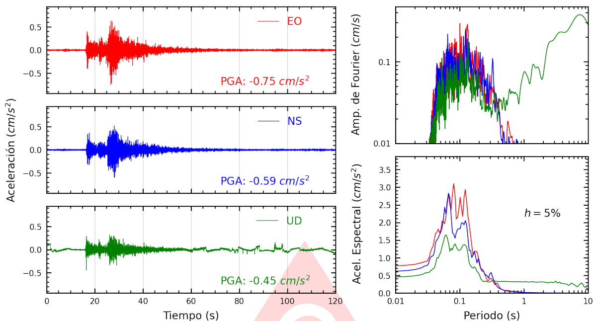
Figura A.33: Registros tiempo-historia, espectros de Fourier y de respuesta en las direcciones EO, NS y vertical de la estación BRISA. Sismo de Lima, Lima - Lima del 2025-06-02, 00:34:43 (Hora local)
