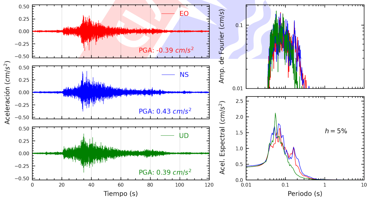
Figura A.44: Registros tiempo-historia, espectros de Fourier y de respuesta en las direcciones EO, NS y vertical de la estación ASIA. Sismo de Lima, Lima - Lima del 2025-06-02, 00:34:43 (Hora local)
