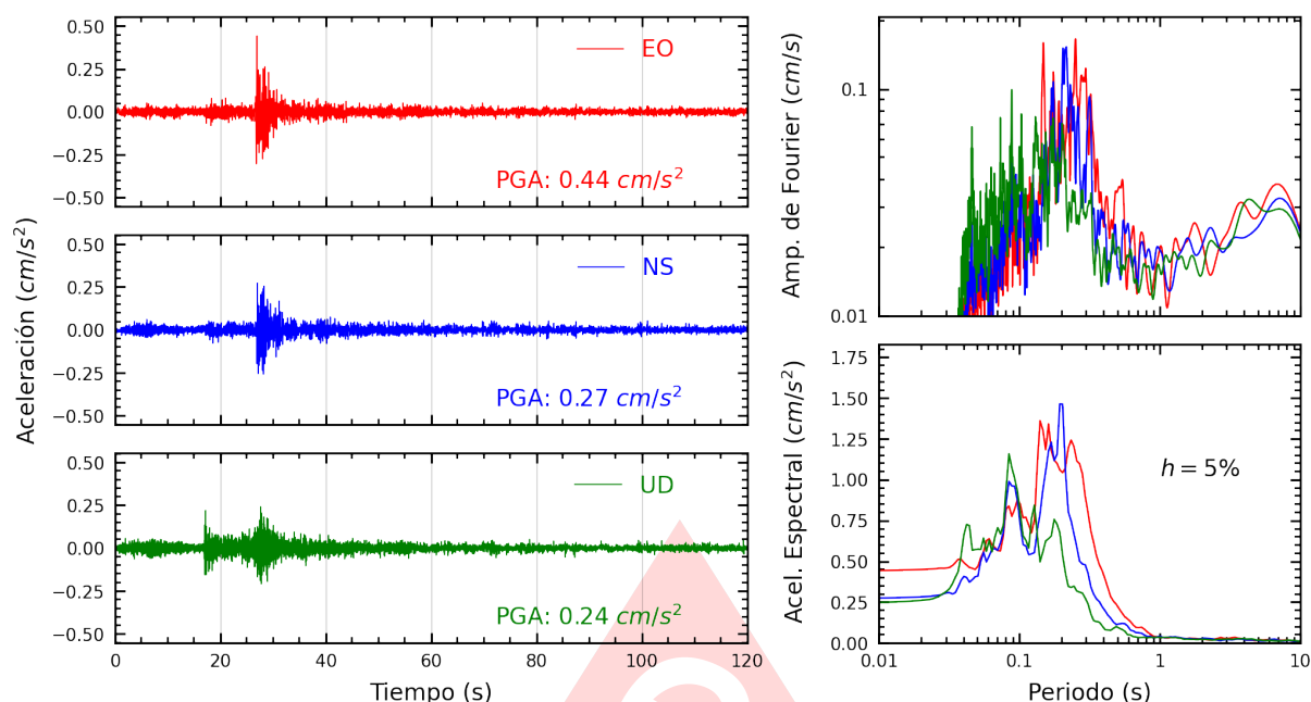
Figura A.43: Registros tiempo-historia, espectros de Fourier y de respuesta en las direcciones EO, NS y vertical de la estación DSML. Sismo de Lima, Lima - Lima del 2025-06-02, 00:34:43 (Hora local)
