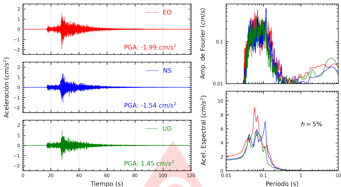
Figura A.11: Registros tiempo-historia, espectros de Fourier y de respuesta en las direcciones EO, NS y vertical de la estación AMORE. Sismo de Lima, Lima - Lima del 2025-06-02, 00:34:43 (Hora local)
