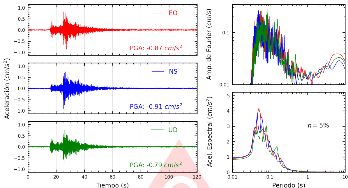
Figura A.25: Registros tiempo-historia, espectros de Fourier y de respuesta en las direcciones EO, NS y vertical de la estación IMCA. Sismo de Lima, Lima - Lima del 2025-06-02, 00:34:43 (Hora local)
