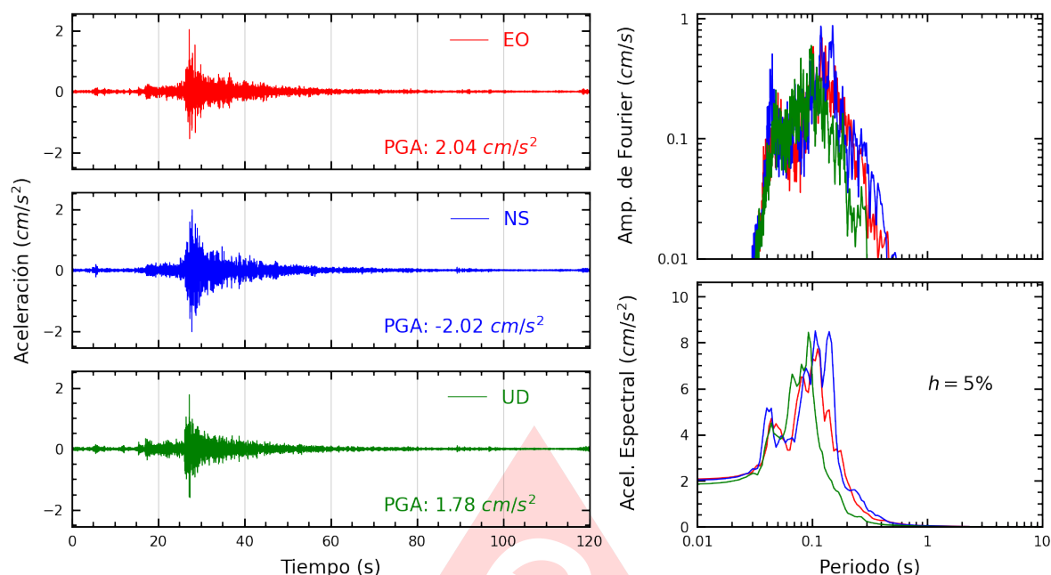
Figura A.9: Registros tiempo-historia, espectros de Fourier y de respuesta en las direcciones EO, NS y vertical de la estación CARA2. Sismo de Lima, Lima - Lima del 2025-06-02, 00:34:43 (Hora local)
