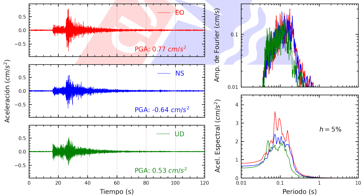
Figura A.32: Registros tiempo-historia, espectros de Fourier y de respuesta en las direcciones EO, NS y vertical de la estación SCCHO. Sismo de Lima, Lima - Lima del 2025-06-02, 00:34:43 (Hora local)
