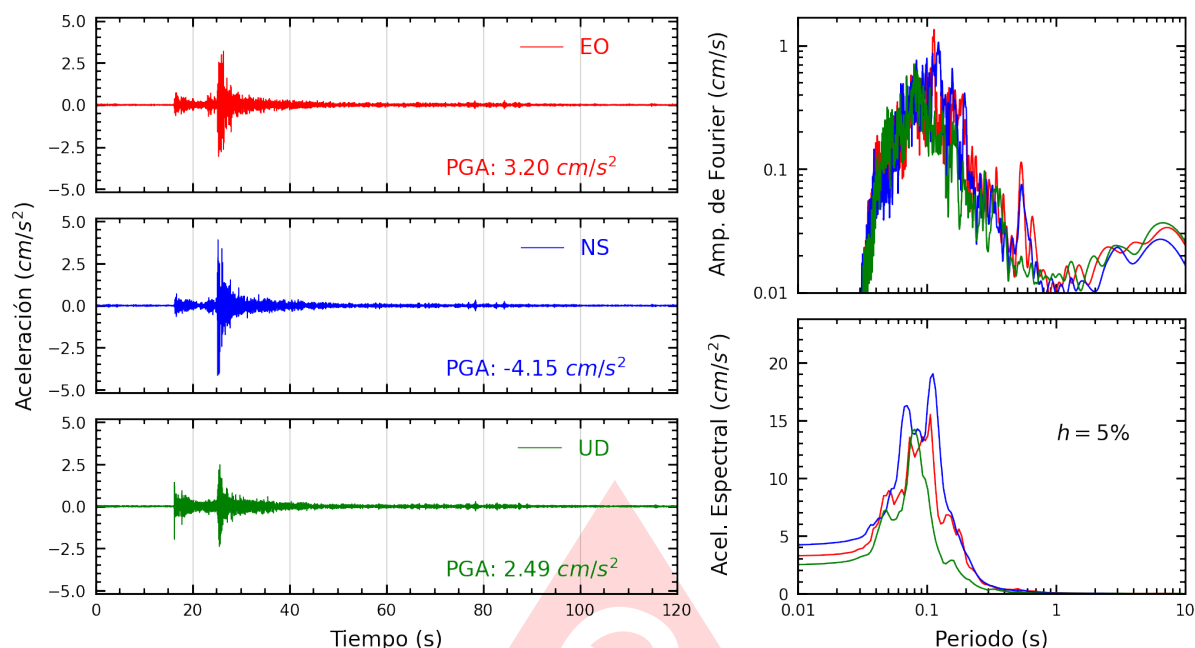
Figura A.3: Registros tiempo-historia, espectros de Fourier y de respuesta en las direcciones EO, NS y vertical de la estación SJLSV. Sismo de Lima, Lima - Lima del 2025-06-02, 00:34:43 (Hora local)
