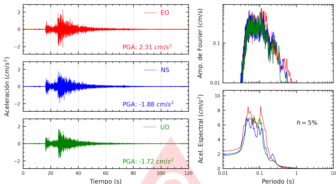
Figura A.7: Registros tiempo-historia, espectros de Fourier y de respuesta en las direcciones EO, NS y vertical de la estación PHER2. Sismo de Lima, Lima - Lima del 2025-06-02, 00:34:43 (Hora local)
