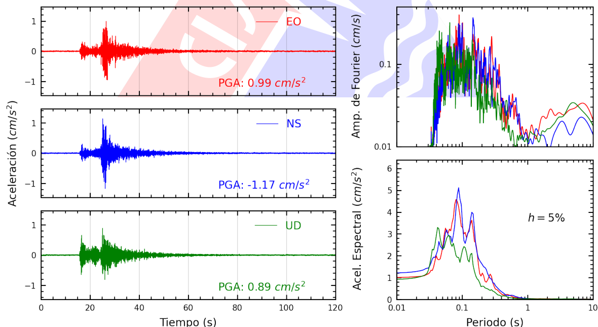
Figura A.20: Registros tiempo-historia, espectros de Fourier y de respuesta en las direcciones EO, NS y vertical de la estación USILP. Sismo de Lima, Lima - Lima del 2025-06-02, 00:34:43 (Hora local)
