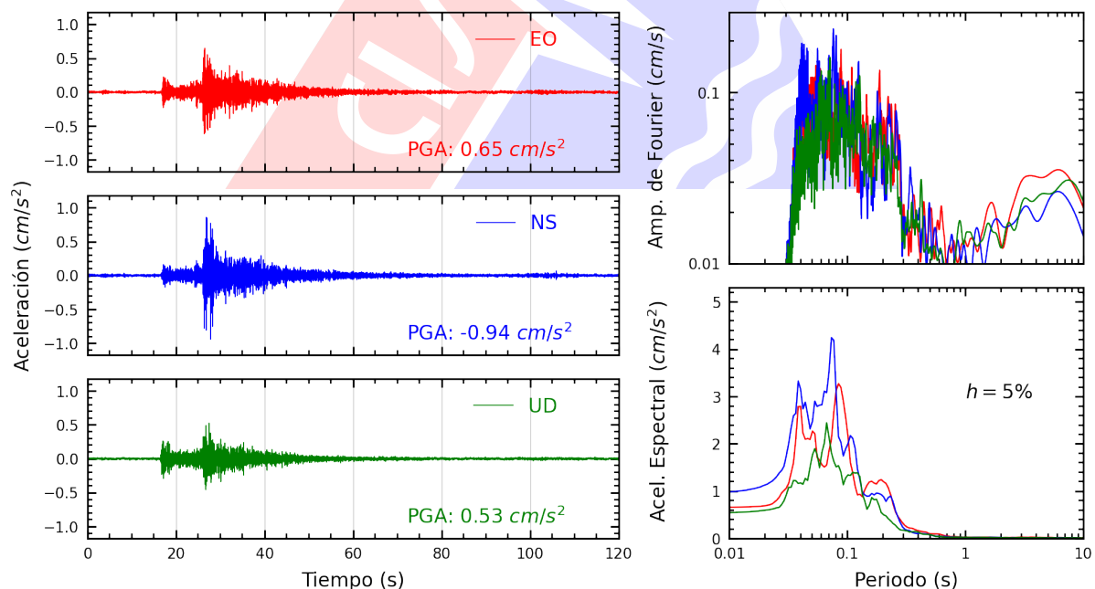
Figura A.22: Registros tiempo-historia, espectros de Fourier y de respuesta en las direcciones EO, NS y vertical de la estación COMAS. Sismo de Lima, Lima - Lima del 2025-06-02, 00:34:43 (Hora local)
