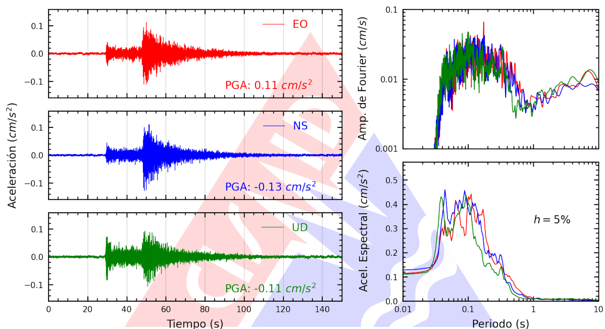
Figura A.45: Registros tiempo-historia, espectros de Fourier y de respuesta en las direcciones EO, NS y vertical de la estación CARAL. Sismo de Lima, Lima - Lima del 2025-06-02, 00:34:43 (Hora local)
