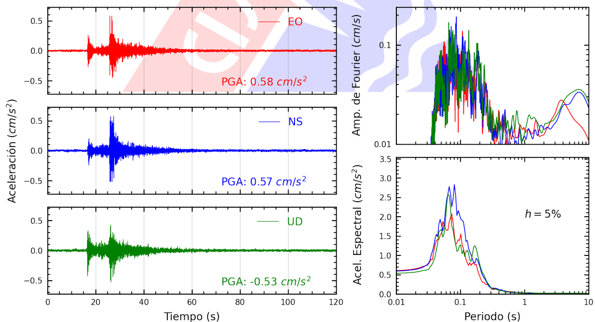
Figura A.40: Registros tiempo-historia, espectros de Fourier y de respuesta en las direcciones EO, NS y vertical de la estación UNFV. Sismo de Lima, Lima - Lima del 2025-06-02, 00:34:43 (Hora local)
