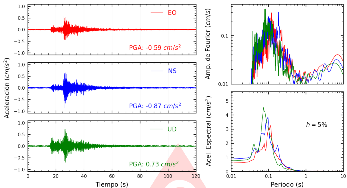
Figura A.27: Registros tiempo-historia, espectros de Fourier y de respuesta en las direcciones EO, NS y vertical de la estación SOCHO. Sismo de Lima, Lima - Lima del 2025-06-02, 00:34:43 (Hora local)
