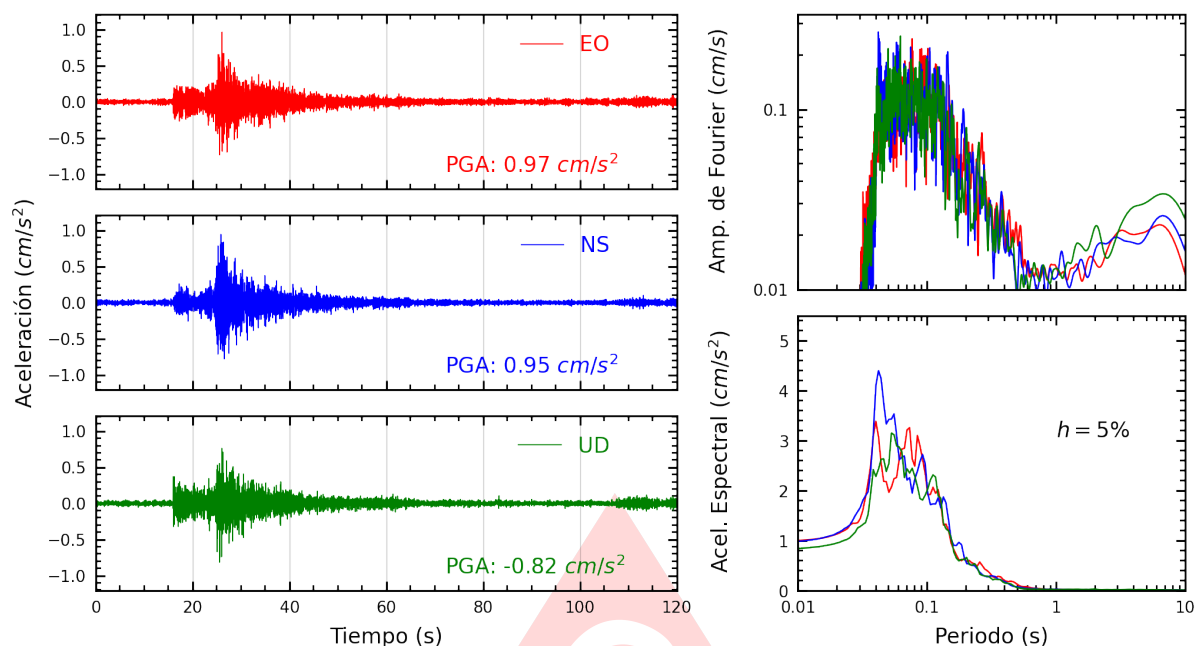
Figura A.21: Registros tiempo-historia, espectros de Fourier y de respuesta en las direcciones EO, NS y vertical de la estación URPE. Sismo de Lima, Lima - Lima del 2025-06-02, 00:34:43 (Hora local)
