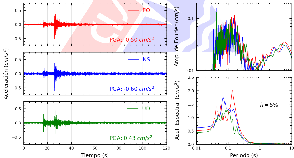
Figura A.38: Registros tiempo-historia, espectros de Fourier y de respuesta en las direcciones EO, NS y vertical de la estación BONDY. Sismo de Lima, Lima - Lima del 2025-06-02, 00:34:43 (Hora local)
