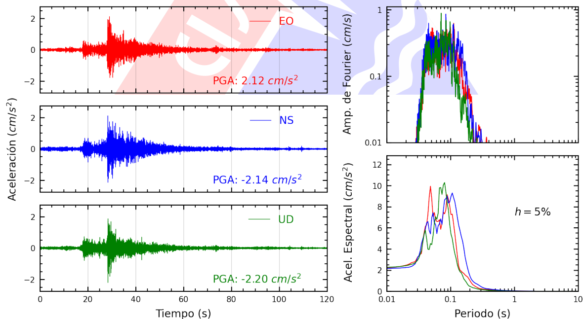
Figura A.8: Registros tiempo-historia, espectros de Fourier y de respuesta en las direcciones EO, NS y vertical de la estación SROS2. Sismo de Lima, Lima - Lima del 2025-06-02, 00:34:43 (Hora local)
