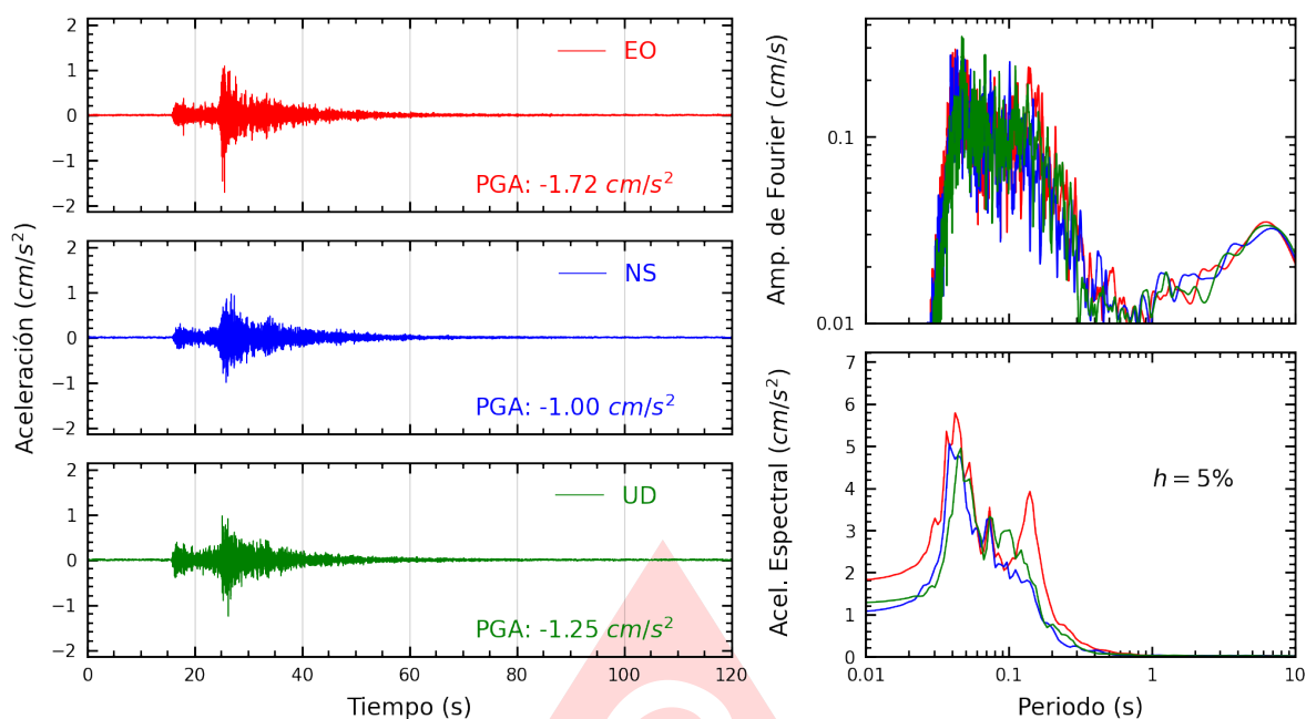
Figura A.13: Registros tiempo-historia, espectros de Fourier y de respuesta en las direcciones EO, NS y vertical de la estación USMP. Sismo de Lima, Lima - Lima del 2025-06-02, 00:34:43 (Hora local)
