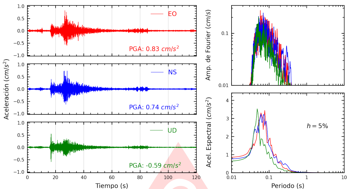
Figura A.29: Registros tiempo-historia, espectros de Fourier y de respuesta en las direcciones EO, NS y vertical de la estación PACHA. Sismo de Lima, Lima - Lima del 2025-06-02, 00:34:43 (Hora local)
