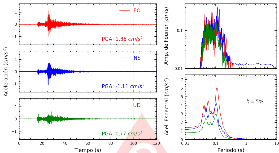
Figura A.15: Registros tiempo-historia, espectros de Fourier y de respuesta en las direcciones EO, NS y vertical de la estación ATARJ. Sismo de Lima, Lima - Lima del 2025-06-02, 00:34:43 (Hora local)
