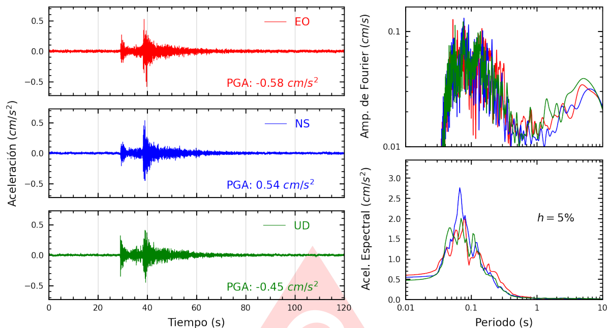
Figura A.39: Registros tiempo-historia, espectros de Fourier y de respuesta en las direcciones EO, NS y vertical de la estación UNMSM. Sismo de Lima, Lima - Lima del 2025-06-02, 00:34:43 (Hora local)
