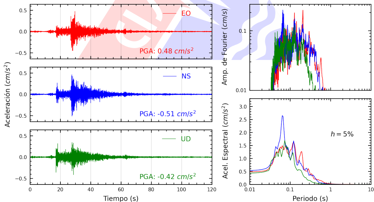
Figura A.42: Registros tiempo-historia, espectros de Fourier y de respuesta en las direcciones EO, NS y vertical de la estación VHAY2. Sismo de Lima, Lima - Lima del 2025-06-02, 00:34:43 (Hora local)
