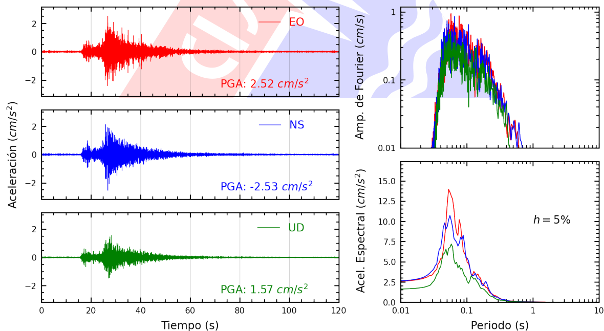
Figura A.6: Registros tiempo-historia, espectros de Fourier y de respuesta en las direcciones EO, NS y vertical de la estación UNTEL. Sismo de Lima, Lima - Lima del 2025-06-02, 00:34:43 (Hora local)
