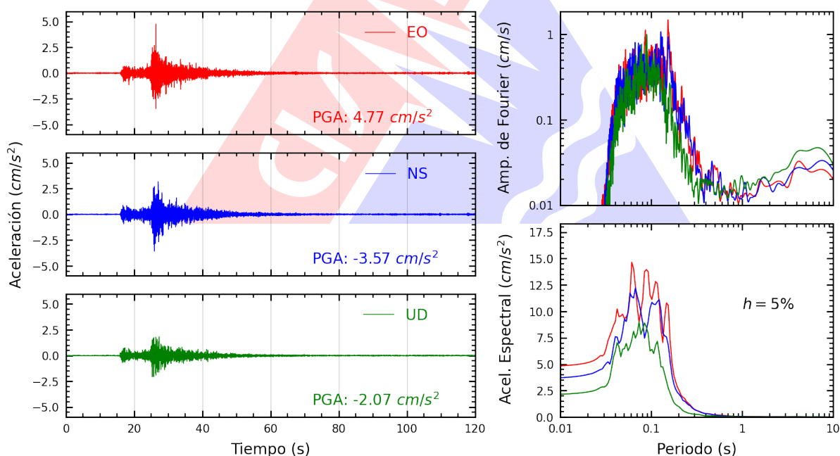
Figura A.2: Registros tiempo-historia, espectros de Fourier y de respuesta en las direcciones EO, NS y vertical de la estación USILM. Sismo de Lima, Lima - Lima del 2025-06-02, 00:34:43 (Hora local)
