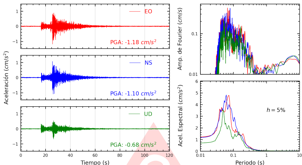
Figura A.19: Registros tiempo-historia, espectros de Fourier y de respuesta en las direcciones EO, NS y vertical de la estación FICPE. Sismo de Lima, Lima - Lima del 2025-06-02, 00:34:43 (Hora local)
