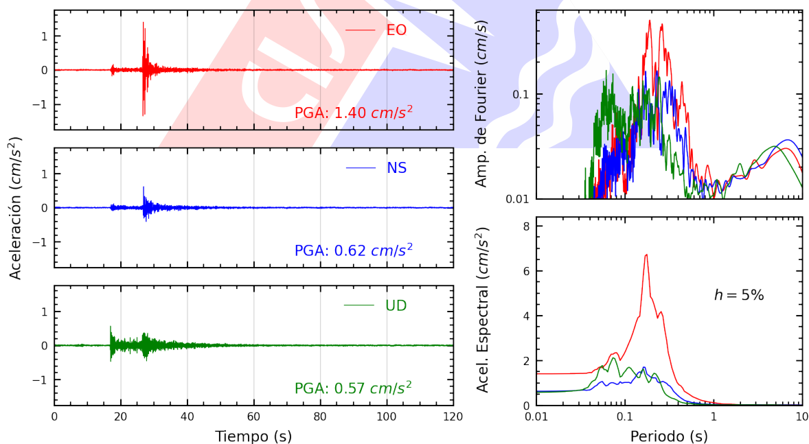
Figura A.14: Registros tiempo-historia, espectros de Fourier y de respuesta en las direcciones EO, NS y vertical de la estación ACAPU. Sismo de Lima, Lima - Lima del 2025-06-02, 00:34:43 (Hora local)
