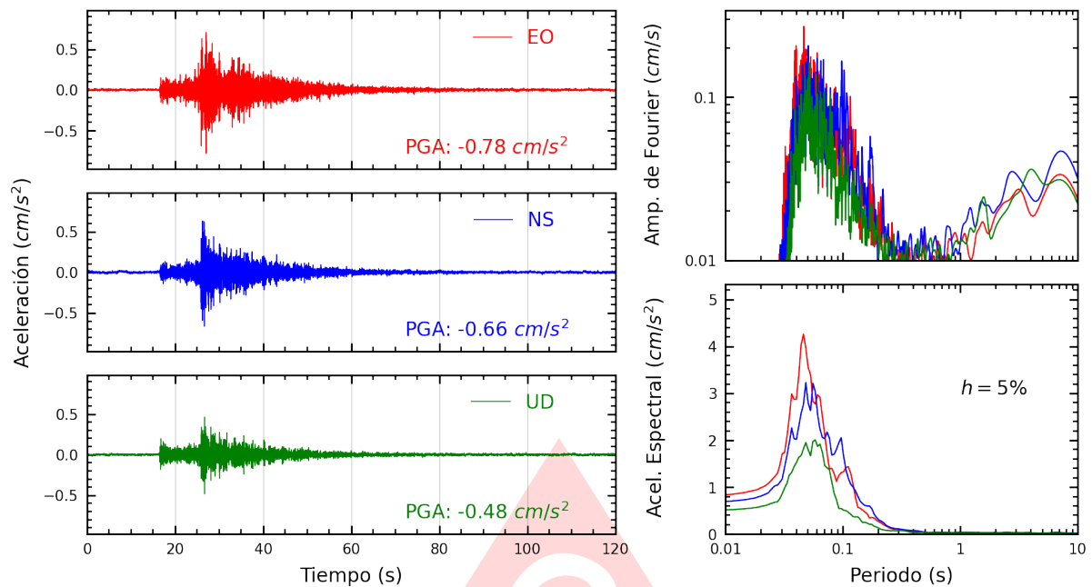
Figura A.31: Registros tiempo-historia, espectros de Fourier y de respuesta en las direcciones EO, NS y vertical de la estación UCSS. Sismo de Lima, Lima - Lima del 2025-06-02, 00:34:43 (Hora local)
