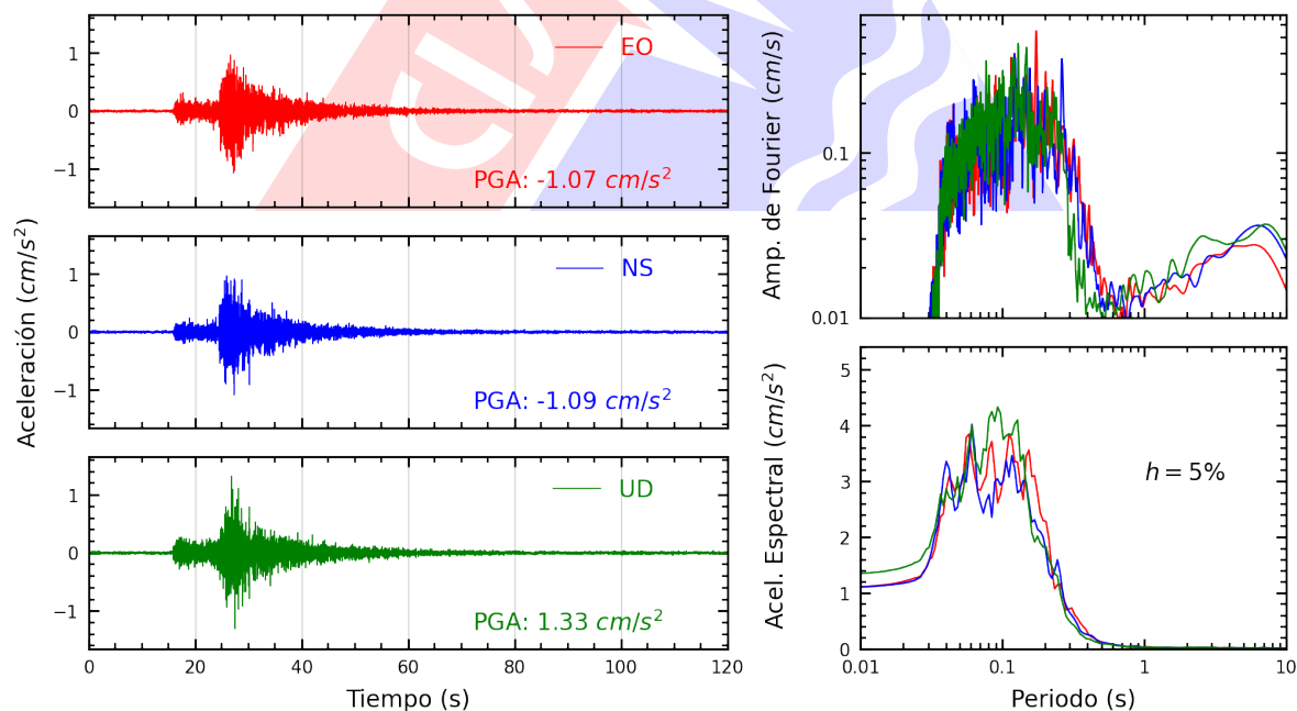
Figura A.16: Registros tiempo-historia, espectros de Fourier y de respuesta en las direcciones EO, NS y vertical de la estación SOVES. Sismo de Lima, Lima - Lima del 2025-06-02, 00:34:43 (Hora local)
