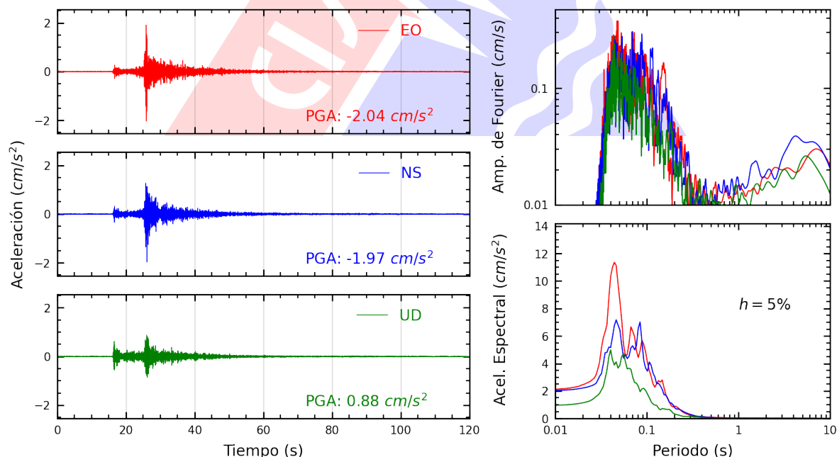
Figura A.10: Registros tiempo-historia, espectros de Fourier y de respuesta en las direcciones EO, NS y vertical de la estación SJLCE. Sismo de Lima, Lima - Lima del 2025-06-02, 00:34:43 (Hora local)
