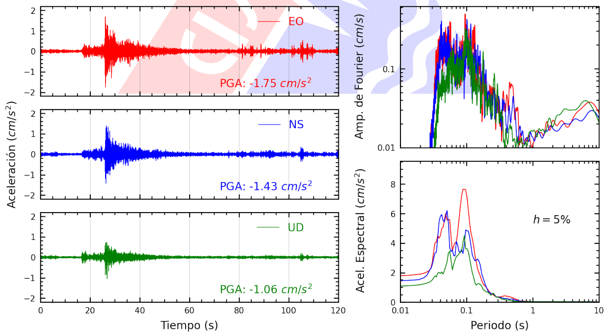
Figura A.12: Registros tiempo-historia, espectros de Fourier y de respuesta en las direcciones EO, NS y vertical de la estación OLIVO. Sismo de Lima, Lima - Lima del 2025-06-02, 00:34:43 (Hora local)
