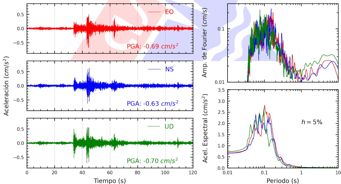
Figura A.34: Registros tiempo-historia, espectros de Fourier y de respuesta en las direcciones EO, NS y vertical de la estación PRADO. Sismo de Lima, Lima - Lima del 2025-06-02, 00:34:43 (Hora local)
