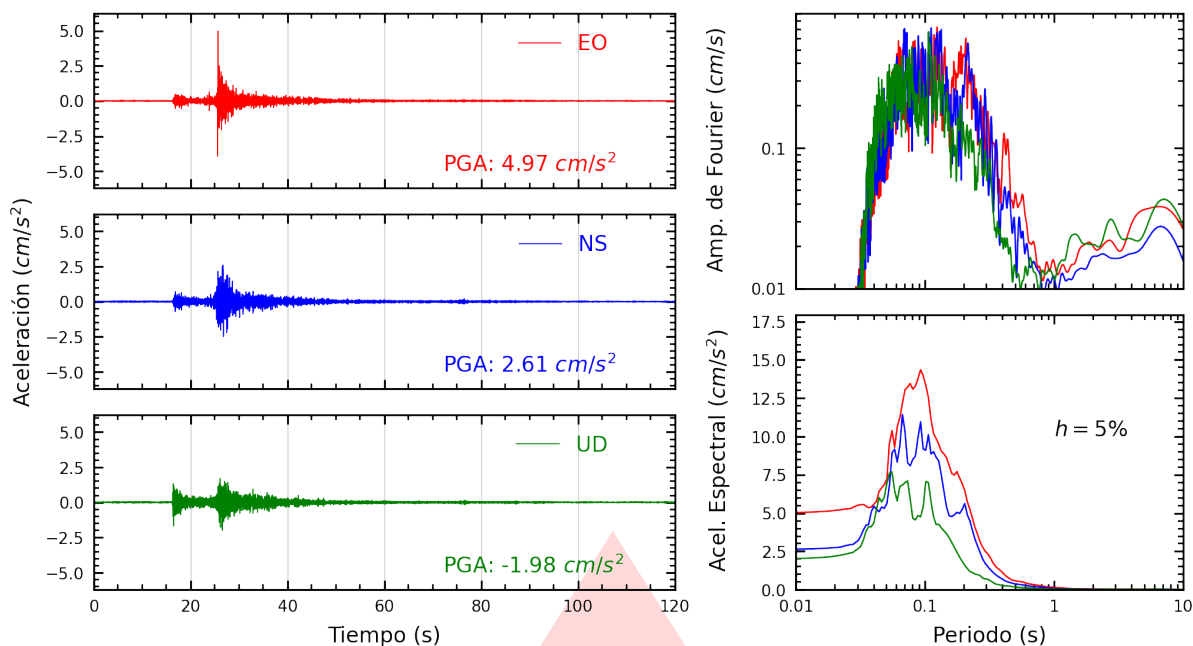
Figura A.1: Registros tiempo-historia, espectros de Fourier y de respuesta en las direcciones EO, NS y vertical de la estación SJLSC. Sismo de Lima, Lima - Lima del 2025-06-02, 00:34:43 (Hora local)
