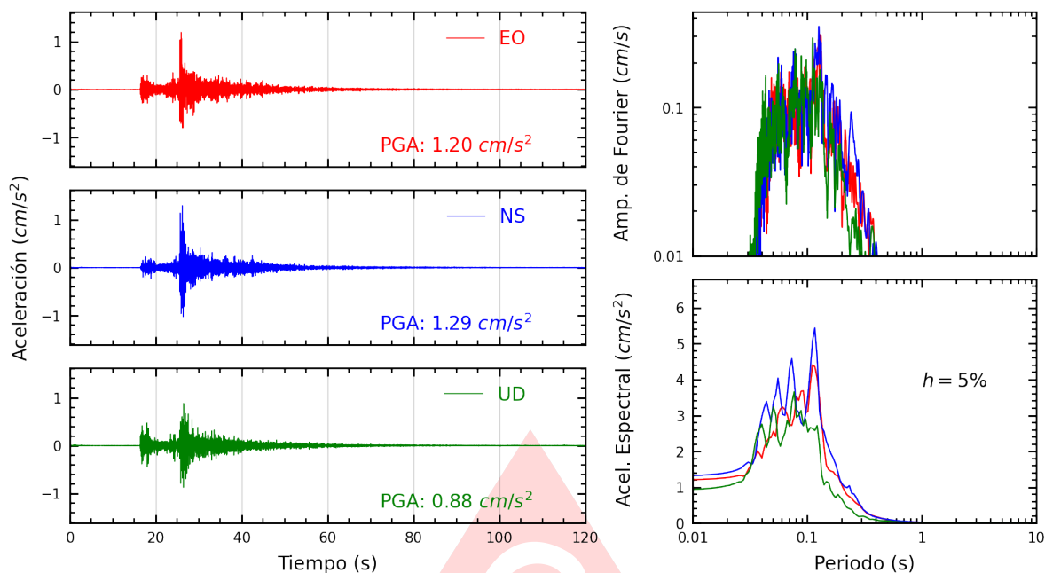
Figura A.17: Registros tiempo-historia, espectros de Fourier y de respuesta en las direcciones EO, NS y vertical de la estación JALV2. Sismo de Lima, Lima - Lima del 2025-06-02, 00:34:43 (Hora local)
