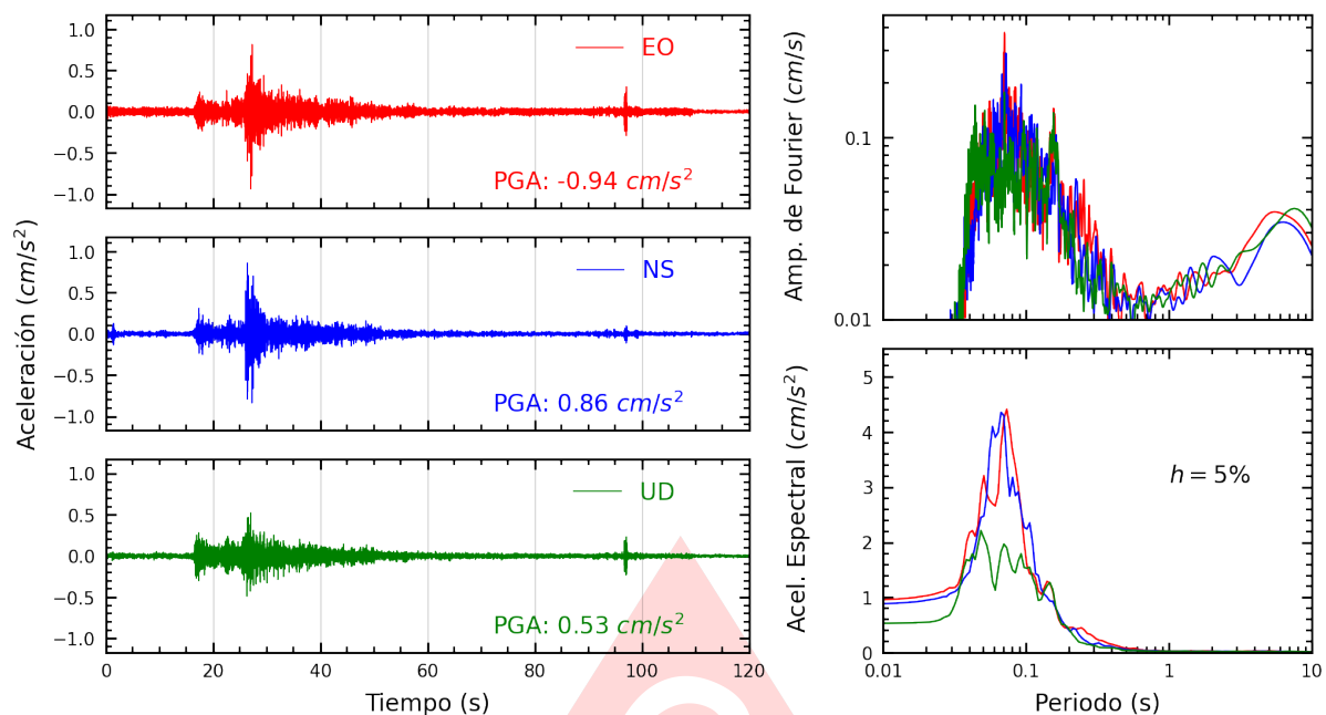
Figura A.23: Registros tiempo-historia, espectros de Fourier y de respuesta en las direcciones EO, NS y vertical de la estación UPCSM. Sismo de Lima, Lima - Lima del 2025-06-02, 00:34:43 (Hora local)
