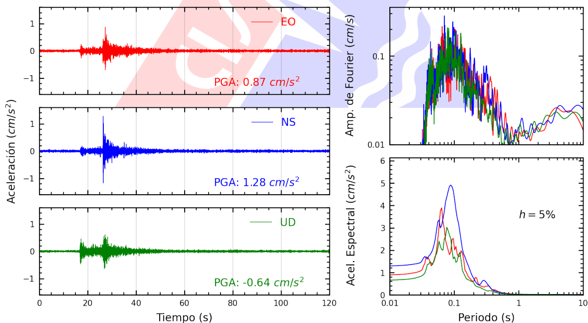
Figura A.18: Registros tiempo-historia, espectros de Fourier y de respuesta en las direcciones EO, NS y vertical de la estación MADRE. Sismo de Lima, Lima - Lima del 2025-06-02, 00:34:43 (Hora local)
