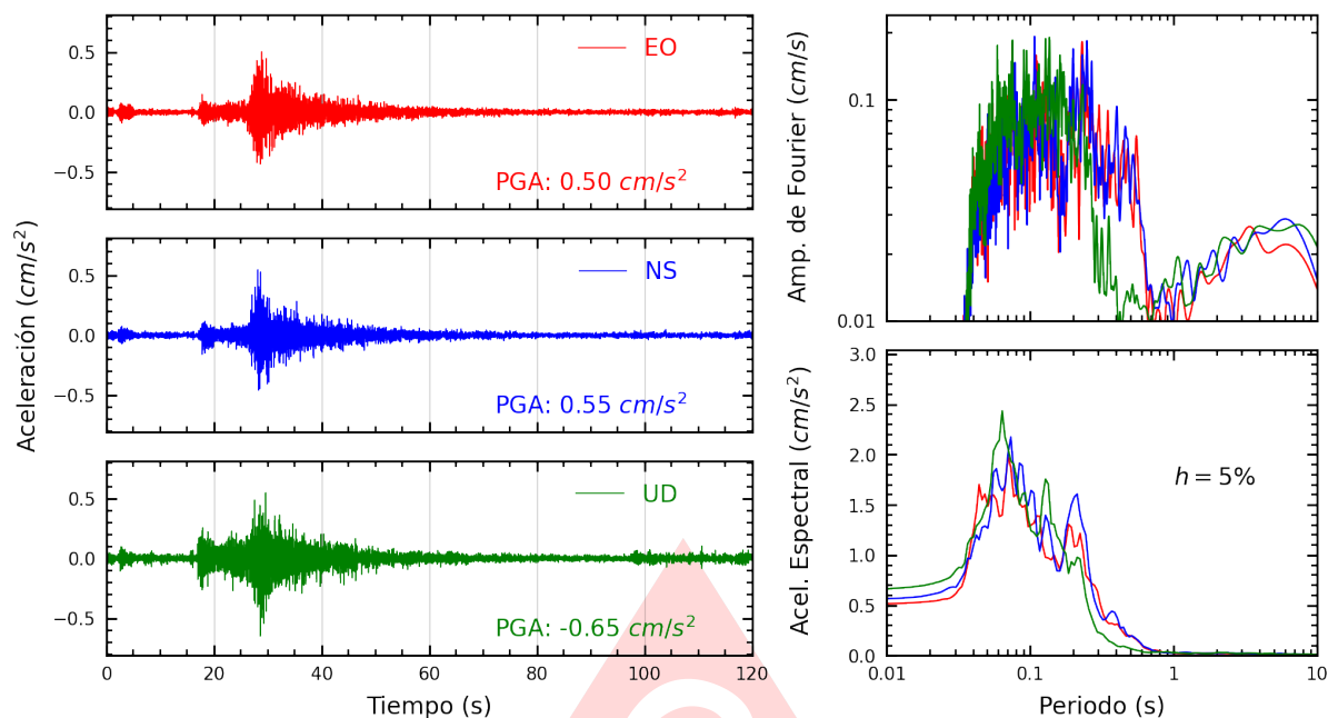
Figura A.37: Registros tiempo-historia, espectros de Fourier y de respuesta en las direcciones EO, NS y vertical de la estación MDPP. Sismo de Lima, Lima - Lima del 2025-06-02, 00:34:43 (Hora local)
