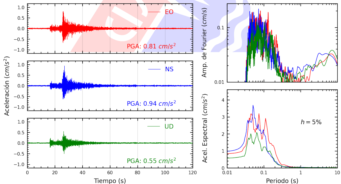
Figura A.24: Registros tiempo-historia, espectros de Fourier y de respuesta en las direcciones EO, NS y vertical de la estación CEPRE. Sismo de Lima, Lima - Lima del 2025-06-02, 00:34:43 (Hora local)
