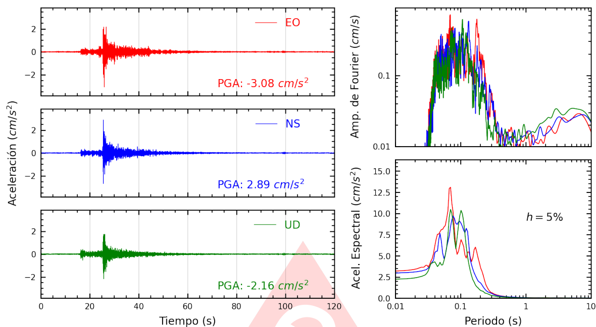
Figura A.5: Registros tiempo-historia, espectros de Fourier y de respuesta en las direcciones EO, NS y vertical de la estación INDEP. Sismo de Lima, Lima - Lima del 2025-06-02, 00:34:43 (Hora local)
