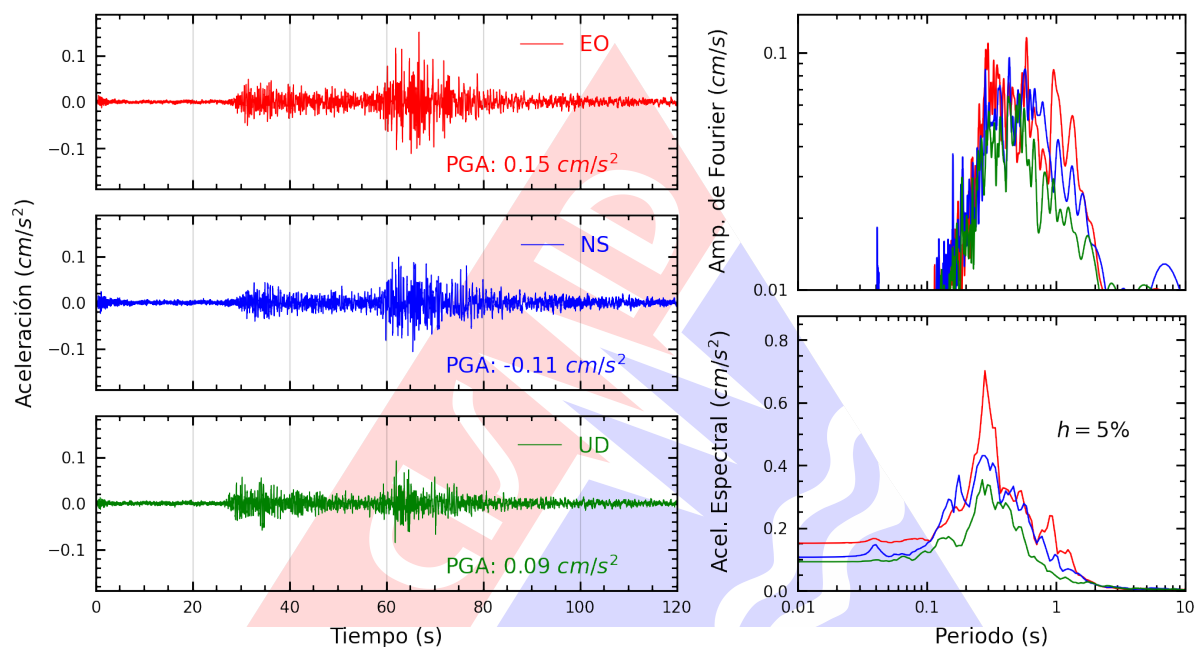
Figura A.5: Registros tiempo-historia, espectros de Fourier y de respuesta en las direcciones EO, NS y vertical de la estación UNJ. Sismo de Sechura, Sechura - Piura del 2025-06-02, 21:30:34 (Hora local)
