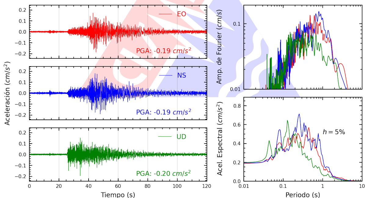
Figura A.2: Registros tiempo-historia, espectros de Fourier y de respuesta en las direcciones EO, NS y vertical de la estación UNF. Sismo de Sechura, Sechura - Piura del 2025-06-02, 21:30:34 (Hora local)
