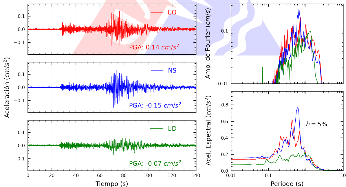
Figura A.4: Registros tiempo-historia, espectros de Fourier y de respuesta en las direcciones EO, NS y vertical de la estación UNC. Sismo de Sechura, Sechura - Piura del 2025-06-02, 21:30:34 (Hora local)
