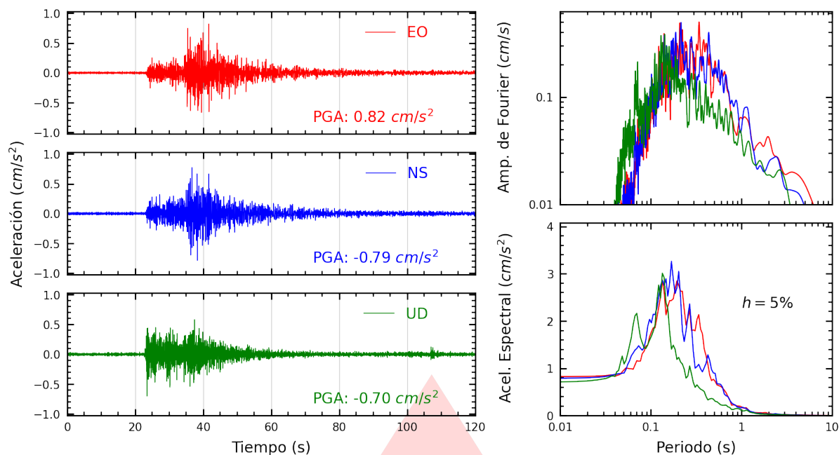
Figura A.1: Registros tiempo-historia, espectros de Fourier y de respuesta en las direcciones EO, NS y vertical de la estación UNP. Sismo de Sechura, Sechura - Piura del 2025-06-02, 21:30:34 (Hora local)
