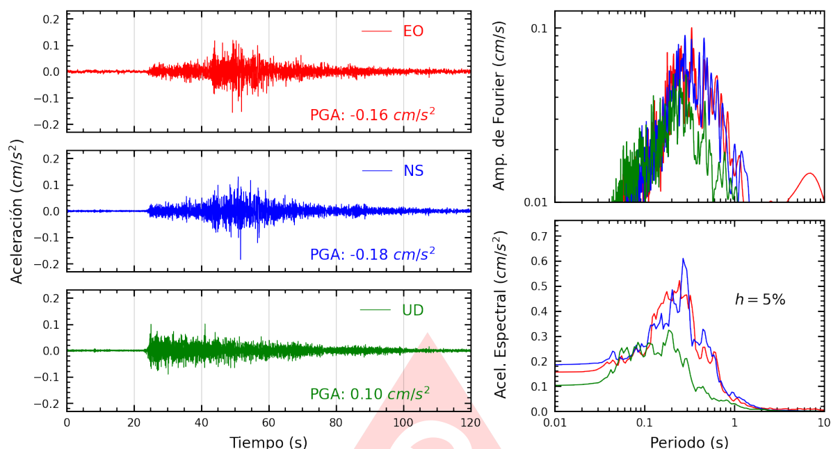
Figura A.3: Registros tiempo-historia, espectros de Fourier y de respuesta en las direcciones EO, NS y vertical de la estación SCCHI. Sismo de Sechura, Sechura - Piura del 2025-06-02, 21:30:34 (Hora local)
