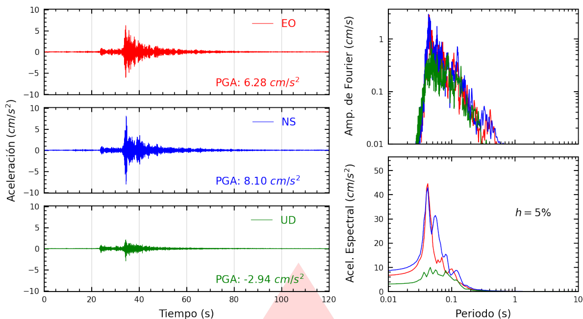
Figura A.1: Registros tiempo-historia, espectros de Fourier y de respuesta en las direcciones EO, NS y vertical de la estación SCTR. Sismo de San Pedro De Lloc, Pacasmayo - La Libertad del 2025-06-06, 22:59:17 (Hora local)
