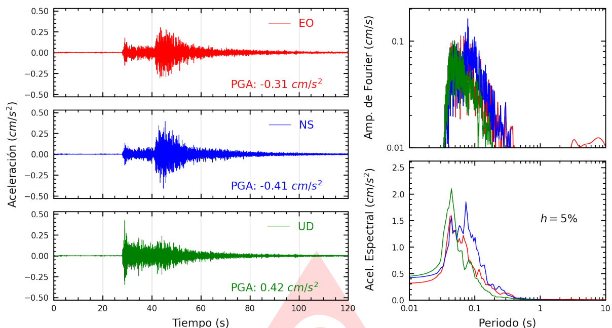
Figura A.3: Registros tiempo-historia, espectros de Fourier y de respuesta en las direcciones EO, NS y vertical de la estación SCCHI. Sismo de San Pedro De Lloc, Pacasmayo - La Libertad del 2025-06-06, 22:59:17 (Hora local)
