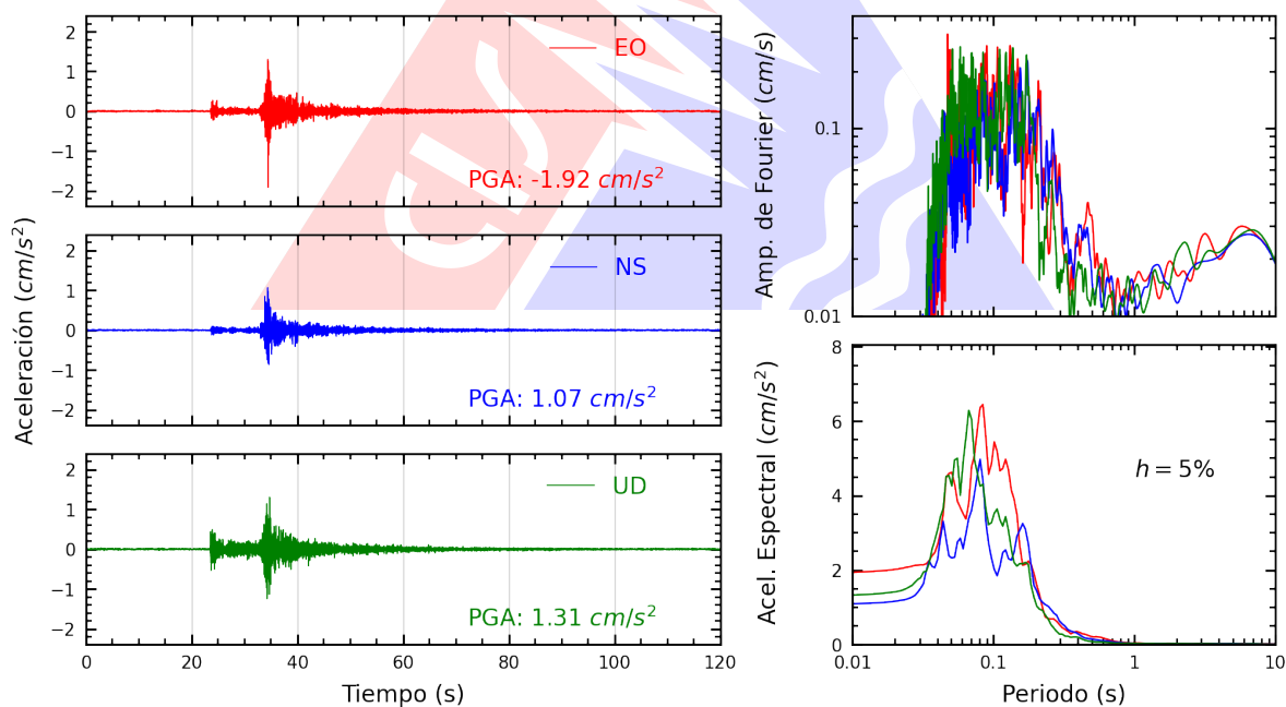
Figura A.2: Registros tiempo-historia, espectros de Fourier y de respuesta en las direcciones EO, NS y vertical de la estación UPAOT. Sismo de San Pedro De Lloc, Pacasmayo - La Libertad del 2025-06-06, 22:59:17 (Hora local)
