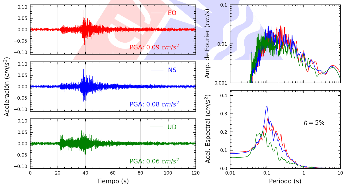
Figura A.4: Registros tiempo-historia, espectros de Fourier y de respuesta en las direcciones EO, NS y vertical de la estación UNC. Sismo de San Pedro De Lloc, Pacasmayo - La Libertad del 2025-06-06, 22:59:17 (Hora local)
