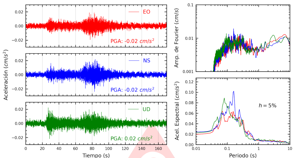
Figura A.5: Registros tiempo-historia, espectros de Fourier y de respuesta en las direcciones EO, NS y vertical de la estación CARAL. Sismo de San Pedro De Lloc, Pacasmayo - La Libertad del 2025-06-06, 22:59:17 (Hora local)
