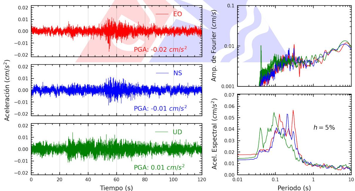
Figura A.6: Registros tiempo-historia, espectros de Fourier y de respuesta en las direcciones EO, NS y vertical de la estación UNJ. Sismo de San Pedro De Lloc, Pacasmayo - La Libertad del 2025-06-06, 22:59:17 (Hora local)
