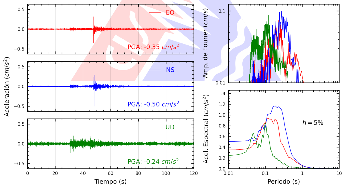
Figura A.2: Registros tiempo-historia, espectros de Fourier y de respuesta en las direcciones EO, NS y vertical de la estación SCPUC. Sismo de Pucallpa, Coronel Portillo - Ucayali del 2025-06-07, 08:02:28 (Hora local)
