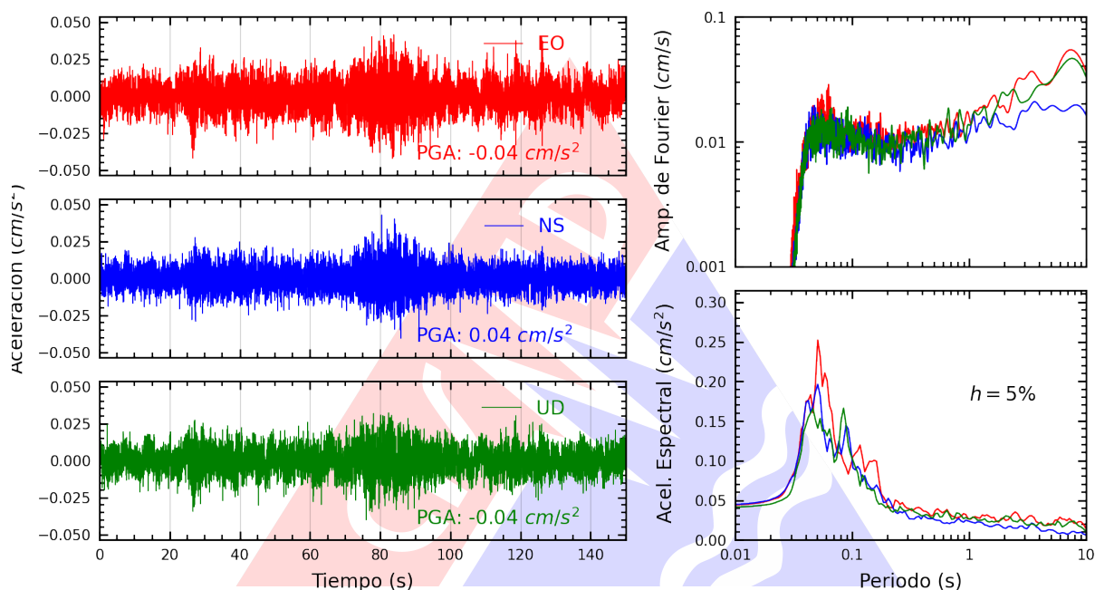
Figura A.5: Registros tiempo-historia, espectros de Fourier y de respuesta en las direcciones EO, NS y vertical de la estación AMORE. Sismo de Pucallpa, Coronel Portillo - Ucayali del 2025-06-07, 08:02:28 (Hora local)
