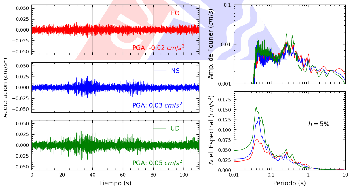
Figura A.4: Registros tiempo-historia, espectros de Fourier y de respuesta en las direcciones EO, NS y vertical de la estación UNC. Sismo de Pucallpa, Coronel Portillo - Ucayali del 2025-06-07, 08:02:28 (Hora local)
