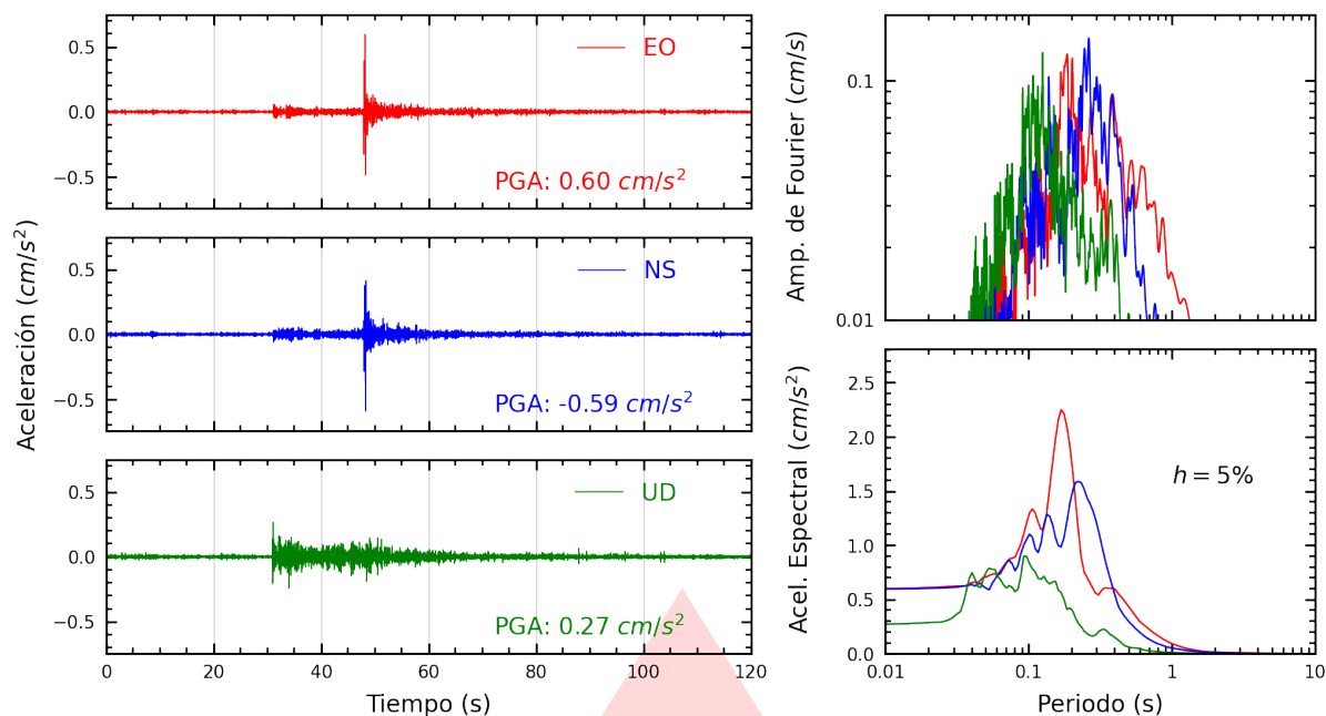
Figura A.1: Registros tiempo-historia, espectros de Fourier y de respuesta en las direcciones EO, NS y vertical de la estación UNIA. Sismo de Pucallpa, Coronel Portillo - Ucayali del 2025-06-07, 08:02:28 (Hora local)
