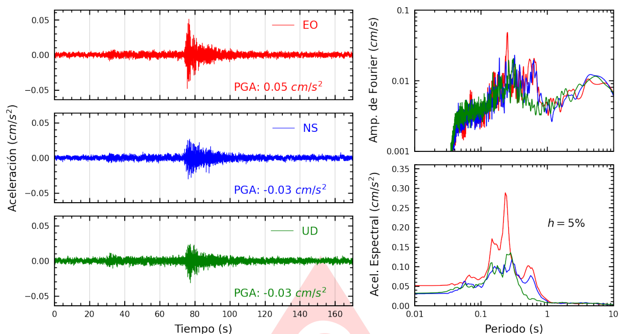
Figura A.3: Registros tiempo-historia, espectros de Fourier y de respuesta en las direcciones EO, NS y vertical de la estación CARAL. Sismo de Pucallpa, Coronel Portillo - Ucayali del 2025-06-07, 08:02:28 (Hora local)
