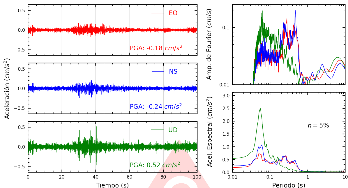
Figura A.5: Registros tiempo-historia, espectros de Fourier y de respuesta en las direcciones EO, NS y vertical de la estación MDPP. Sismo de Casma, Casma - Ancash del 2025-06-07, 18:45:31 (Hora local)
