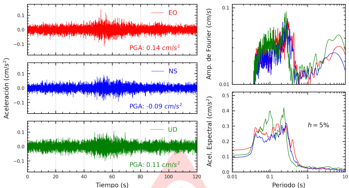
Figura A.17: Registros tiempo-historia, espectros de Fourier y de respuesta en las direcciones EO, NS y vertical de la estación SOVES. Sismo de Casma, Casma - Ancash del 2025-06-07, 18:45:31 (Hora local)
