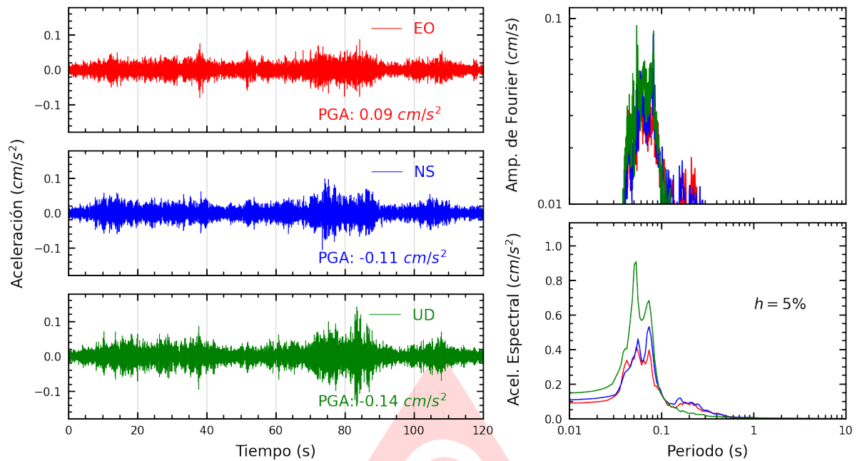
Figura A.15: Registros tiempo-historia, espectros de Fourier y de respuesta en las direcciones EO, NS y vertical de la estación ASIA. Sismo de Casma, Casma - Ancash del 2025-06-07, 18:45:31 (Hora local)
