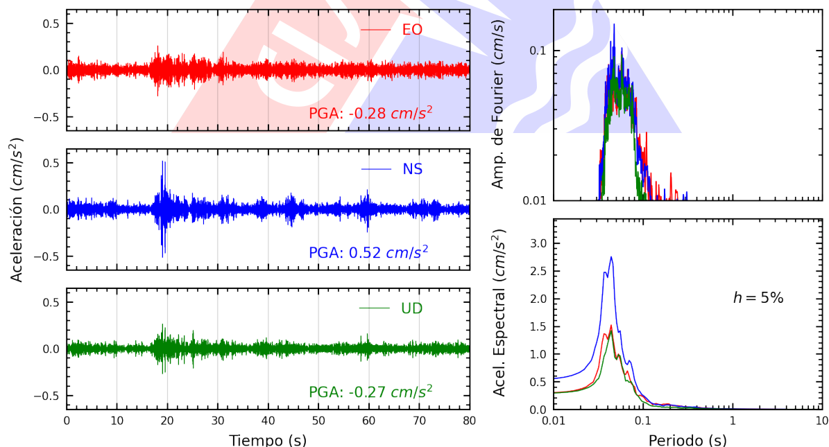
Figura A.4: Registros tiempo-historia, espectros de Fourier y de respuesta en las direcciones EO, NS y vertical de la estación PACHA. Sismo de Casma, Casma - Ancash del 2025-06-07, 18:45:31 (Hora local)
