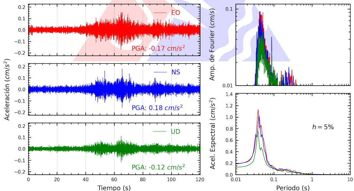
Figura A.12: Registros tiempo-historia, espectros de Fourier y de respuesta en las direcciones EO, NS y vertical de la estación BORJA. Sismo de Casma, Casma - Ancash del 2025-06-07, 18:45:31 (Hora local)
