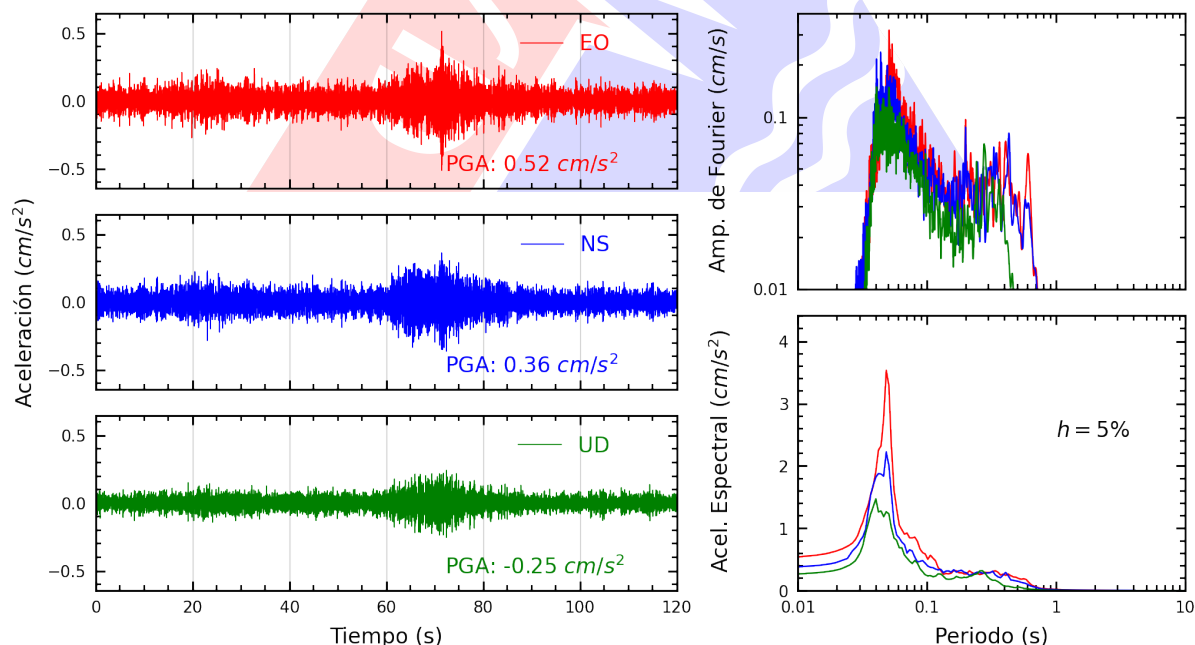
Figura A.6: Registros tiempo-historia, espectros de Fourier y de respuesta en las direcciones EO, NS y vertical de la estación UNTEL. Sismo de Casma, Casma - Ancash del 2025-06-07, 18:45:31 (Hora local)
