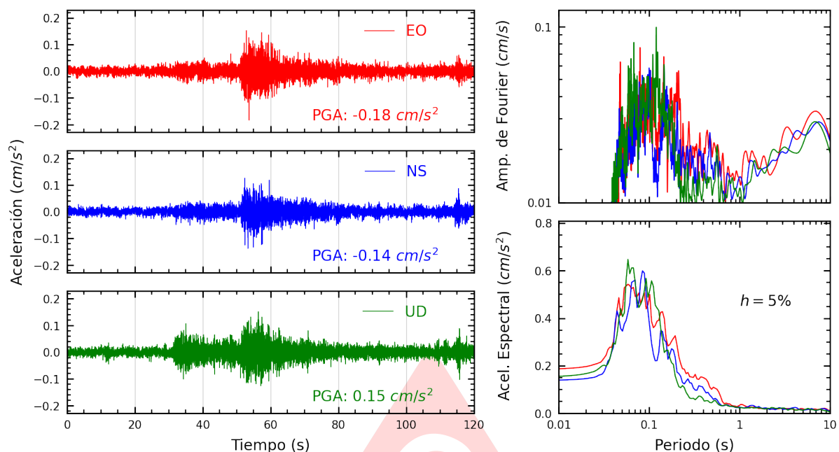
Figura A.11: Registros tiempo-historia, espectros de Fourier y de respuesta en las direcciones EO, NS y vertical de la estación UPAOT. Sismo de Casma, Casma - Ancash del 2025-06-07, 18:45:31 (Hora local)
