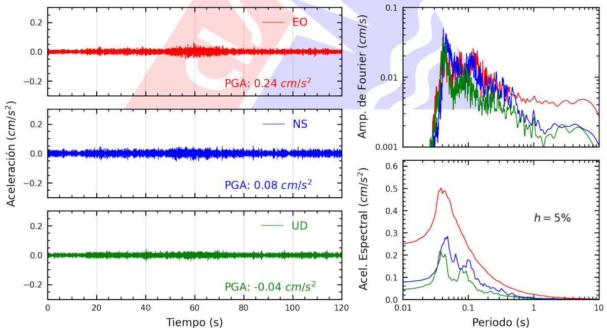
Figura A.10: Registros tiempo-historia, espectros de Fourier y de respuesta en las direcciones EO, NS y vertical de la estación ATARJ. Sismo de Casma, Casma - Ancash del 2025-06-07, 18:45:31 (Hora local)
