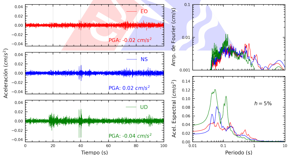
Figura A.24: Registros tiempo-historia, espectros de Fourier y de respuesta en las direcciones EO, NS y vertical de la estación UNIA. Sismo de Casma, Casma - Ancash del 2025-06-07, 18:45:31 (Hora local)
