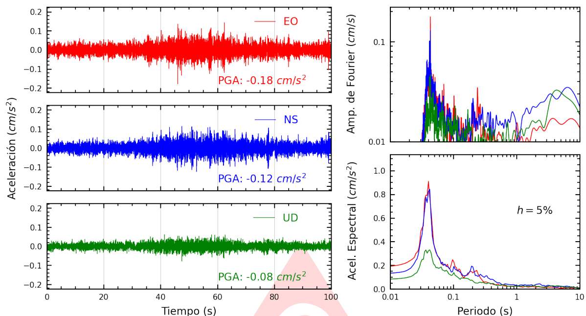
Figura A.13: Registros tiempo-historia, espectros de Fourier y de respuesta en las direcciones EO, NS y vertical de la estación CEPRE. Sismo de Casma, Casma - Ancash del 2025-06-07, 18:45:31 (Hora local)
