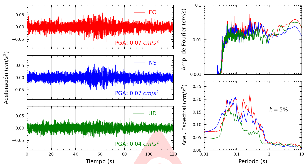
Figura A.21: Registros tiempo-historia, espectros de Fourier y de respuesta en las direcciones EO, NS y vertical de la estación USILP. Sismo de Casma, Casma - Ancash del 2025-06-07, 18:45:31 (Hora local)
