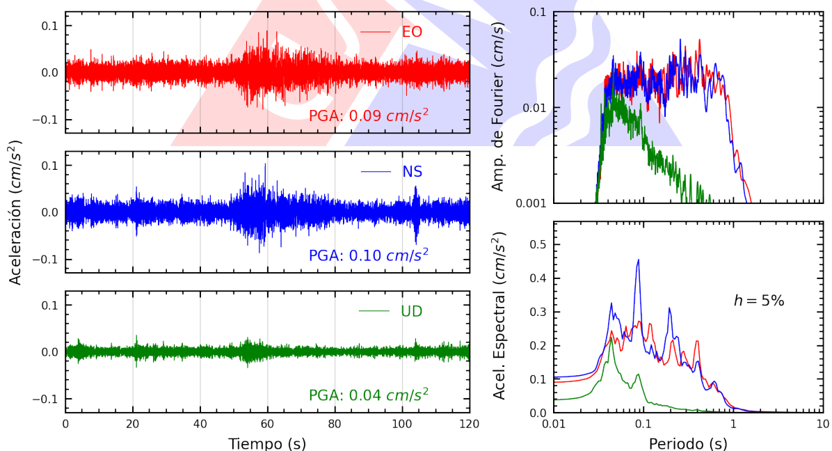
Figura A.20: Registros tiempo-historia, espectros de Fourier y de respuesta en las direcciones EO, NS y vertical de la estación UCVA2. Sismo de Casma, Casma - Ancash del 2025-06-07, 18:45:31 (Hora local)
