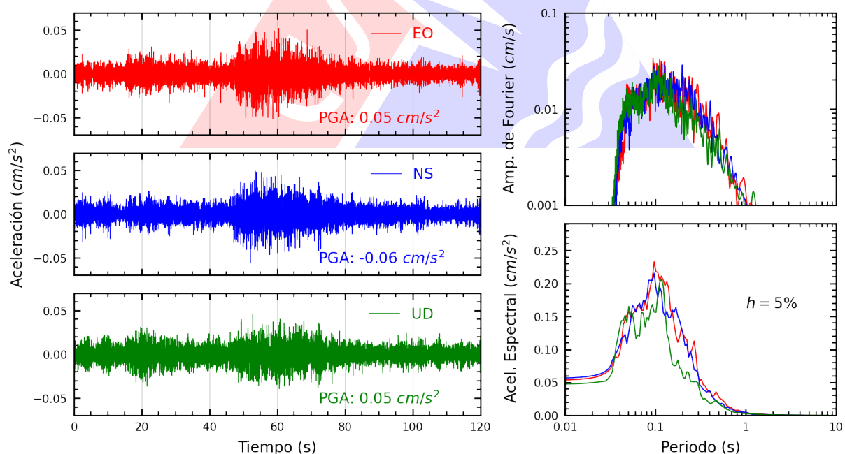
Figura A.22: Registros tiempo-historia, espectros de Fourier y de respuesta en las direcciones EO, NS y vertical de la estación JALV2. Sismo de Casma, Casma - Ancash del 2025-06-07, 18:45:31 (Hora local)
