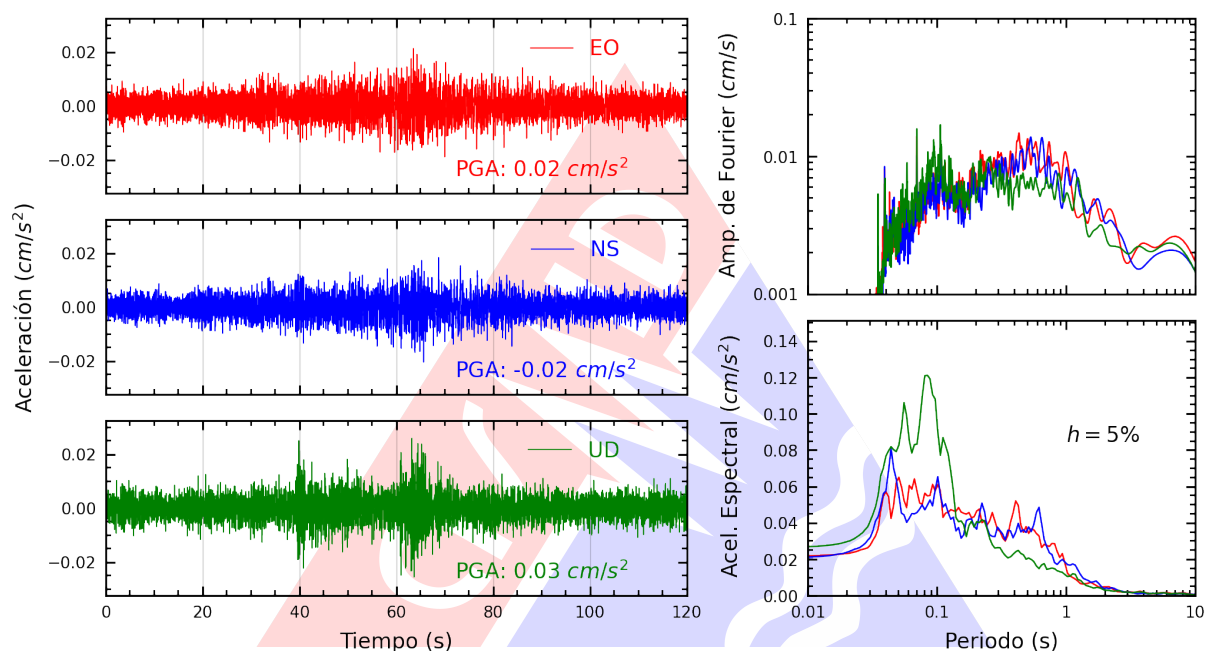
Figura A.25: Registros tiempo-historia, espectros de Fourier y de respuesta en las direcciones EO, NS y vertical de la estación UNC. Sismo de Casma, Casma - Ancash del 2025-06-07, 18:45:31 (Hora local)
