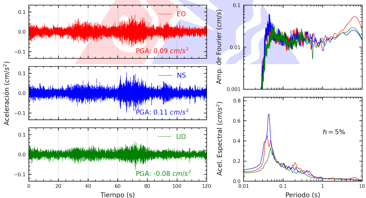
Figura A.18: Registros tiempo-historia, espectros de Fourier y de respuesta en las direcciones EO, NS y vertical de la estación COMAS. Sismo de Casma, Casma - Ancash del 2025-06-07, 18:45:31 (Hora local)
