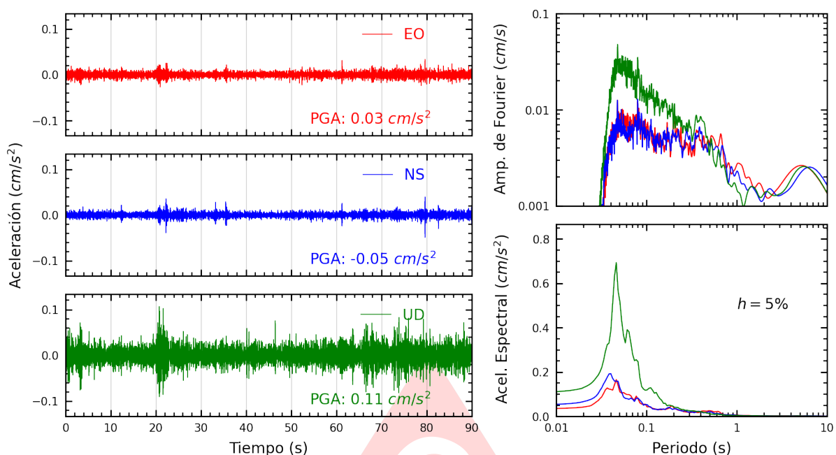
Figura A.19: Registros tiempo-historia, espectros de Fourier y de respuesta en las direcciones EO, NS y vertical de la estación SCPUC. Sismo de Casma, Casma - Ancash del 2025-06-07, 18:45:31 (Hora local)
