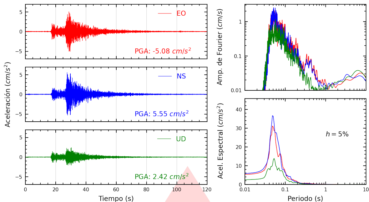
Figura A.1: Registros tiempo-historia, espectros de Fourier y de respuesta en las direcciones EO, NS y vertical de la estación USP. Sismo de Casma, Casma - Ancash del 2025-06-07, 18:45:31 (Hora local)
