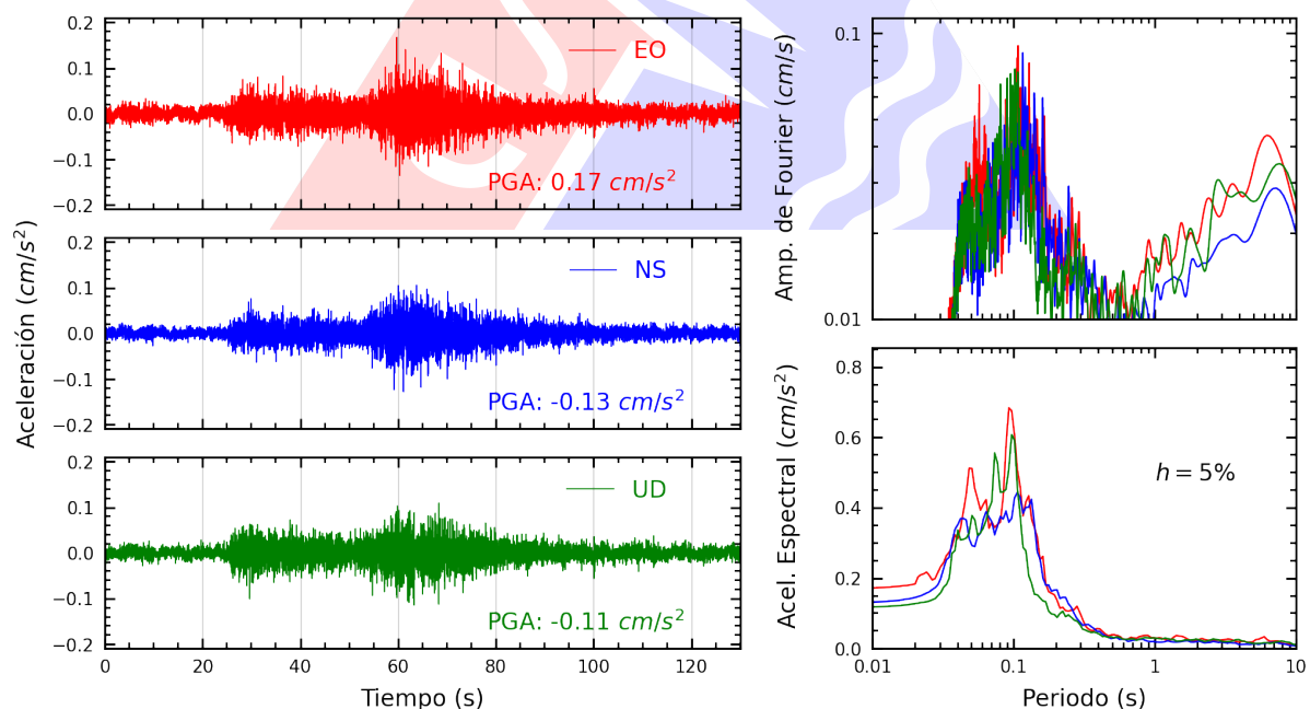
Figura A.14: Registros tiempo-historia, espectros de Fourier y de respuesta en las direcciones EO, NS y vertical de la estación AMORE. Sismo de Casma, Casma - Ancash del 2025-06-07, 18:45:31 (Hora local)
