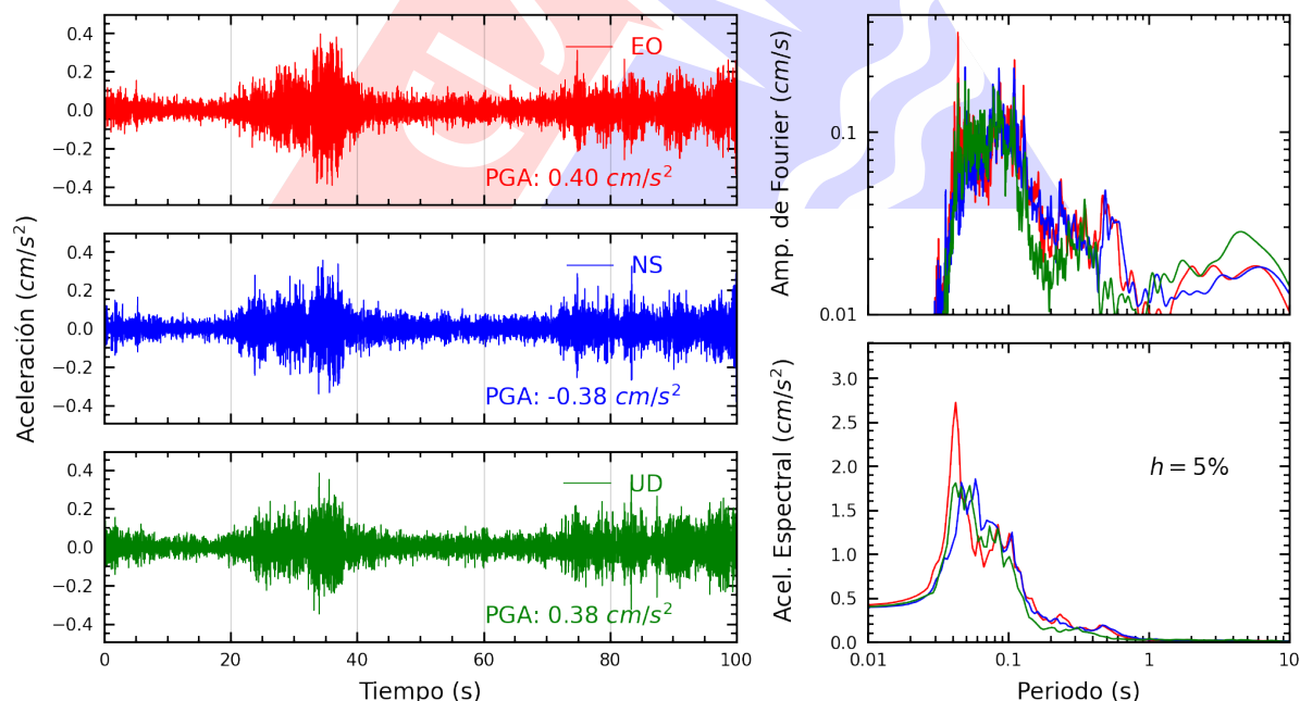
Figura A.8: Registros tiempo-historia, espectros de Fourier y de respuesta en las direcciones EO, NS y vertical de la estación SJLSV. Sismo de Casma, Casma - Ancash del 2025-06-07, 18:45:31 (Hora local)
