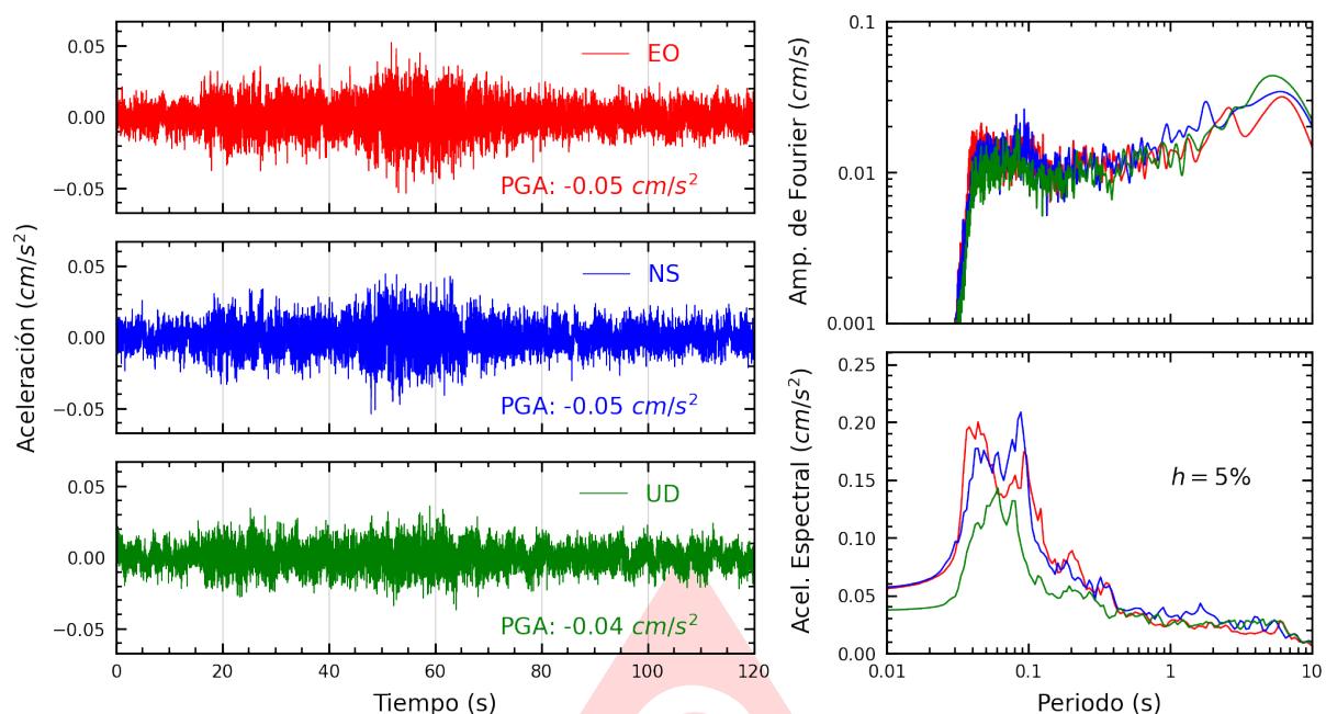
Figura A.23: Registros tiempo-historia, espectros de Fourier y de respuesta en las direcciones EO, NS y vertical de la estación UCSS. Sismo de Casma, Casma - Ancash del 2025-06-07, 18:45:31 (Hora local)
