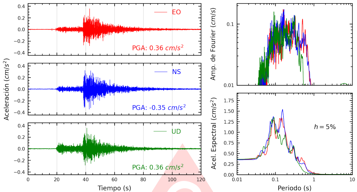
Figura A.9: Registros tiempo-historia, espectros de Fourier y de respuesta en las direcciones EO, NS y vertical de la estación CARAL. Sismo de Casma, Casma - Ancash del 2025-06-07, 18:45:31 (Hora local)
