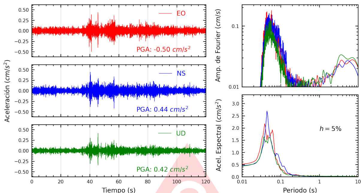
Figura A.7: Registros tiempo-historia, espectros de Fourier y de respuesta en las direcciones EO, NS y vertical de la estación JOSEO. Sismo de Casma, Casma - Ancash del 2025-06-07, 18:45:31 (Hora local)
