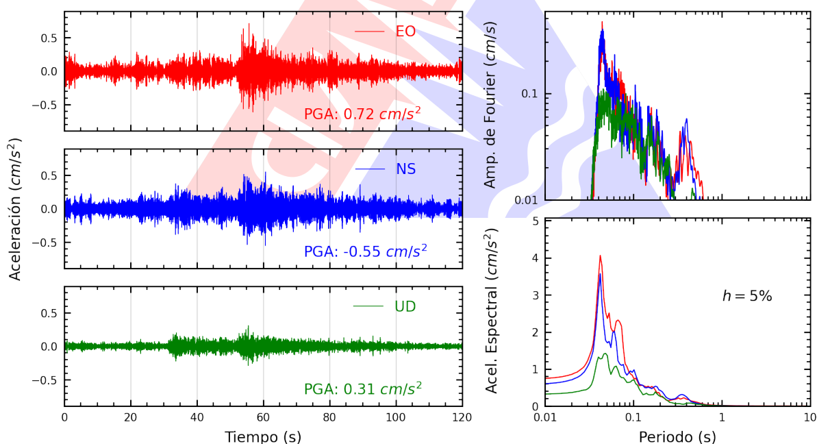
Figura A.2: Registros tiempo-historia, espectros de Fourier y de respuesta en las direcciones EO, NS y vertical de la estación SCTRU. Sismo de Casma, Casma - Ancash del 2025-06-07, 18:45:31 (Hora local)
