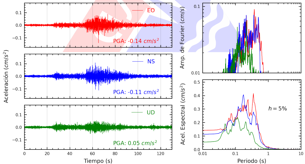
Figura A.16: Registros tiempo-historia, espectros de Fourier y de respuesta en las direcciones EO, NS y vertical de la estación VHAY2. Sismo de Casma, Casma - Ancash del 2025-06-07, 18:45:31 (Hora local)
