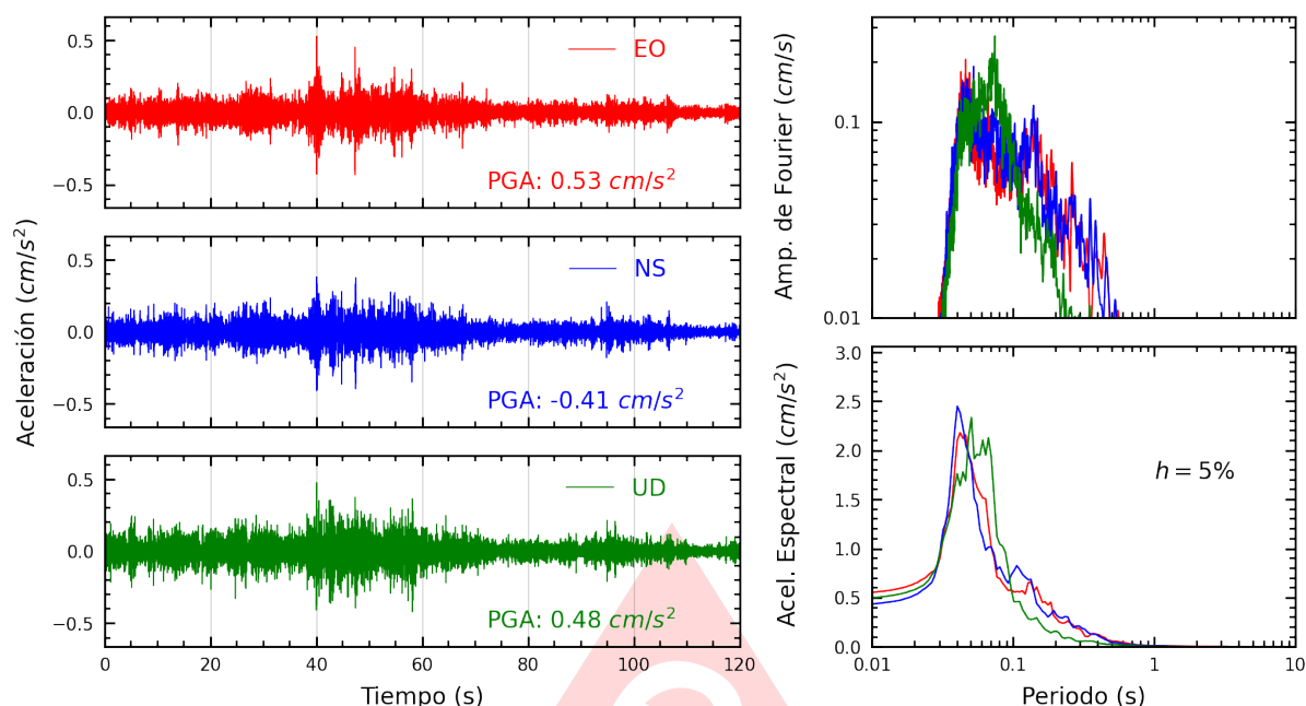
Figura A.3: Registros tiempo-historia, espectros de Fourier y de respuesta en las direcciones EO, NS y vertical de la estación CARA2. Sismo de Casma, Casma - Ancash del 2025-06-07, 18:45:31 (Hora local)
