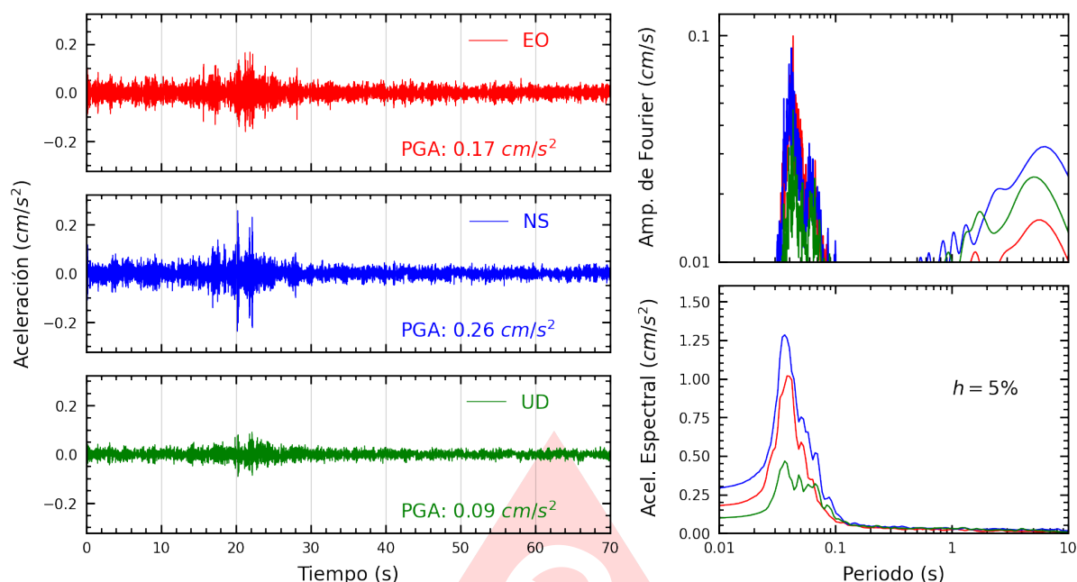
Figura A.5: Registros tiempo-historia, espectros de Fourier y de respuesta en las direcciones EO, NS y vertical de la estación CEPRE. Sismo de Satipo, Satipo - Junin del 2025-06-08, 12:12:33 (Hora local)
