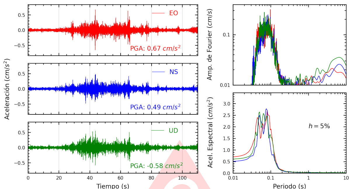
Figura A.3: Registros tiempo-historia, espectros de Fourier y de respuesta en las direcciones EO, NS y vertical de la estación SJLSV. Sismo de Satipo, Satipo - Junin del 2025-06-08, 12:12:33 (Hora local)
