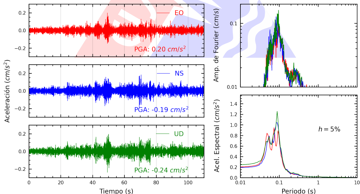
Figura A.6: Registros tiempo-historia, espectros de Fourier y de respuesta en las direcciones EO, NS y vertical de la estación UNICA. Sismo de Satipo, Satipo - Junin del 2025-06-08, 12:12:33 (Hora local)
