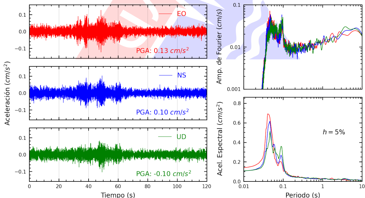
Figura A.8: Registros tiempo-historia, espectros de Fourier y de respuesta en las direcciones EO, NS y vertical de la estación IMCA. Sismo de Satipo, Satipo - Junin del 2025-06-08, 12:12:33 (Hora local)
