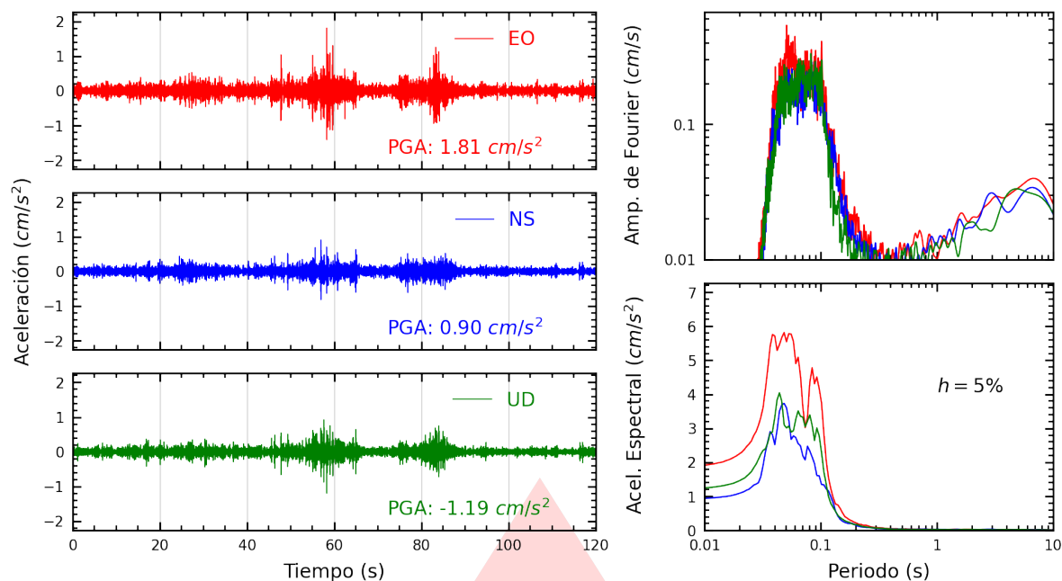
Figura A.1: Registros tiempo-historia, espectros de Fourier y de respuesta en las direcciones EO, NS y vertical de la estación SOBAR. Sismo de Satipo, Satipo - Junin del 2025-06-08, 12:12:33 (Hora local)
