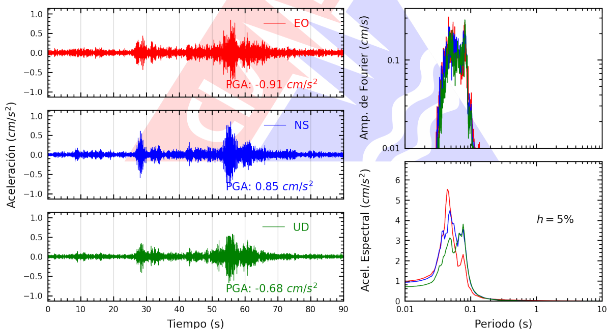
Figura A.2: Registros tiempo-historia, espectros de Fourier y de respuesta en las direcciones EO, NS y vertical de la estación PACHA. Sismo de Satipo, Satipo - Junin del 2025-06-08, 12:12:33 (Hora local)
