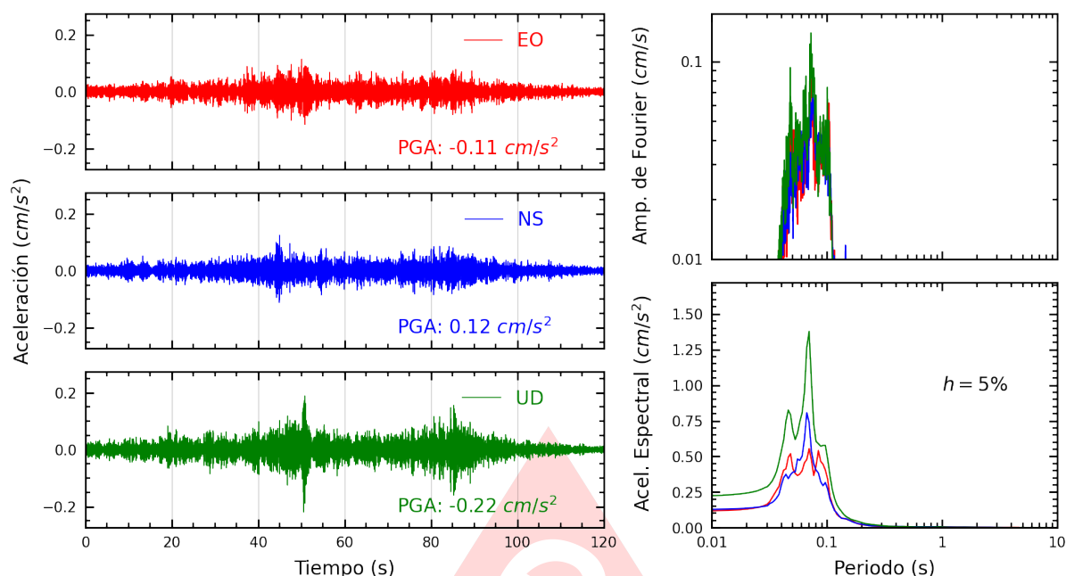
Figura A.7: Registros tiempo-historia, espectros de Fourier y de respuesta en las direcciones EO, NS y vertical de la estación ASIA. Sismo de Satipo, Satipo - Junin del 2025-06-08, 12:12:33 (Hora local)
