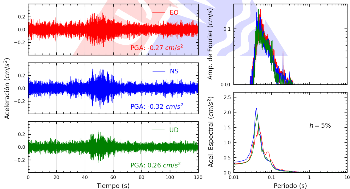
Figura A.4: Registros tiempo-historia, espectros de Fourier y de respuesta en las direcciones EO, NS y vertical de la estación UNTEL. Sismo de Satipo, Satipo - Junin del 2025-06-08, 12:12:33 (Hora local)
