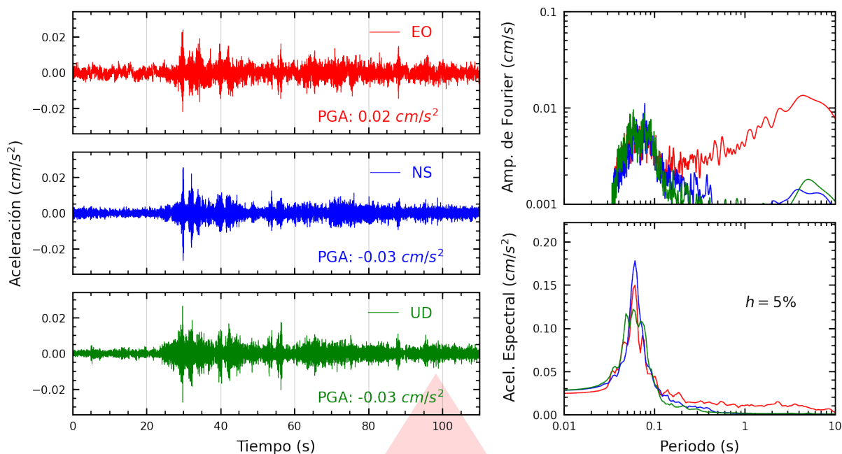
Figura A.1: Registros tiempo-historia, espectros de Fourier y de respuesta en las direcciones EO, NS y vertical de la estación SCCHI. Sismo de Barranca, Datem del Maraón - Loreto del 2025-06-08, 20:47:54 (Hora local)
