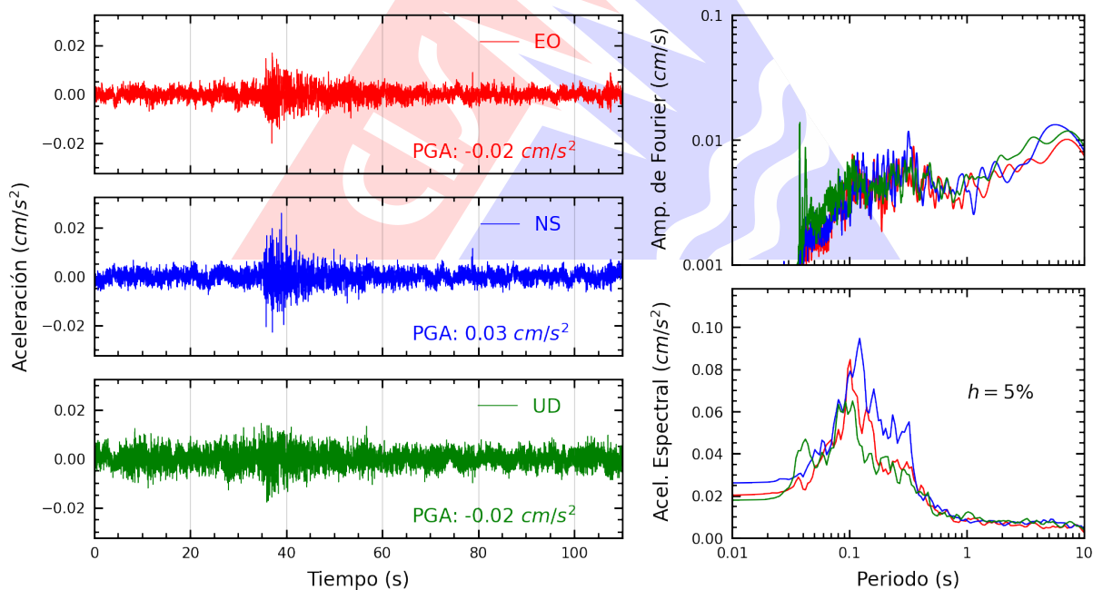
Figura A.2: Registros tiempo-historia, espectros de Fourier y de respuesta en las direcciones EO, NS y vertical de la estación UNJ. Sismo de Barranca, Datem del Maraón - Loreto del 2025-06-08, 20:47:54 (Hora local)
