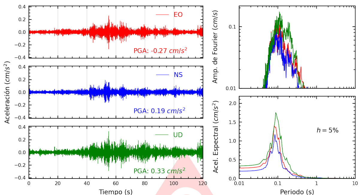
Figura A.3: Registros tiempo-historia, espectros de Fourier y de respuesta en las direcciones EO, NS y vertical de la estación UANCV. Sismo de Camana, Camana - Arequipa del 2025-06-10, 22:04:21 (Hora local)
