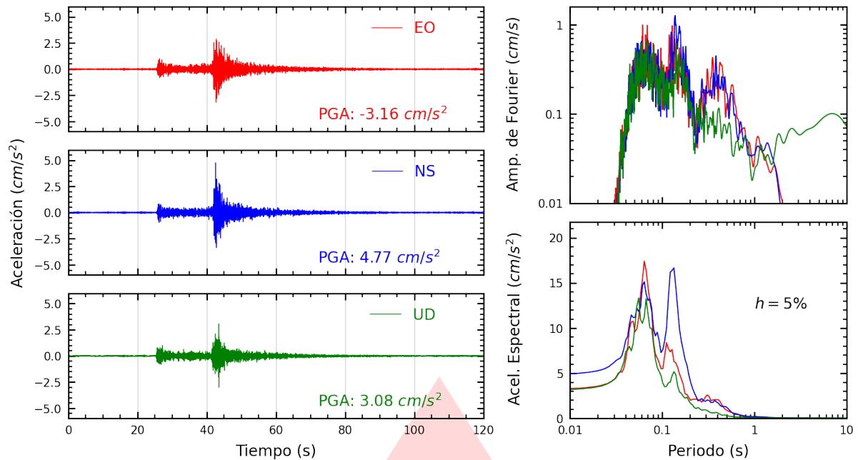
Figura A.1: Registros tiempo-historia, espectros de Fourier y de respuesta en las direcciones EO, NS y vertical de la estación SCARQ. Sismo de Camana, Camana - Arequipa del 2025-06-10, 22:04:21 (Hora local)
