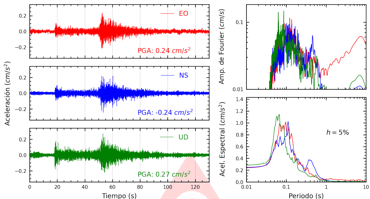
Figura A.5: Registros tiempo-historia, espectros de Fourier y de respuesta en las direcciones EO, NS y vertical de la estación UJBG3. Sismo de Camana, Camana - Arequipa del 2025-06-10, 22:04:21 (Hora local)
