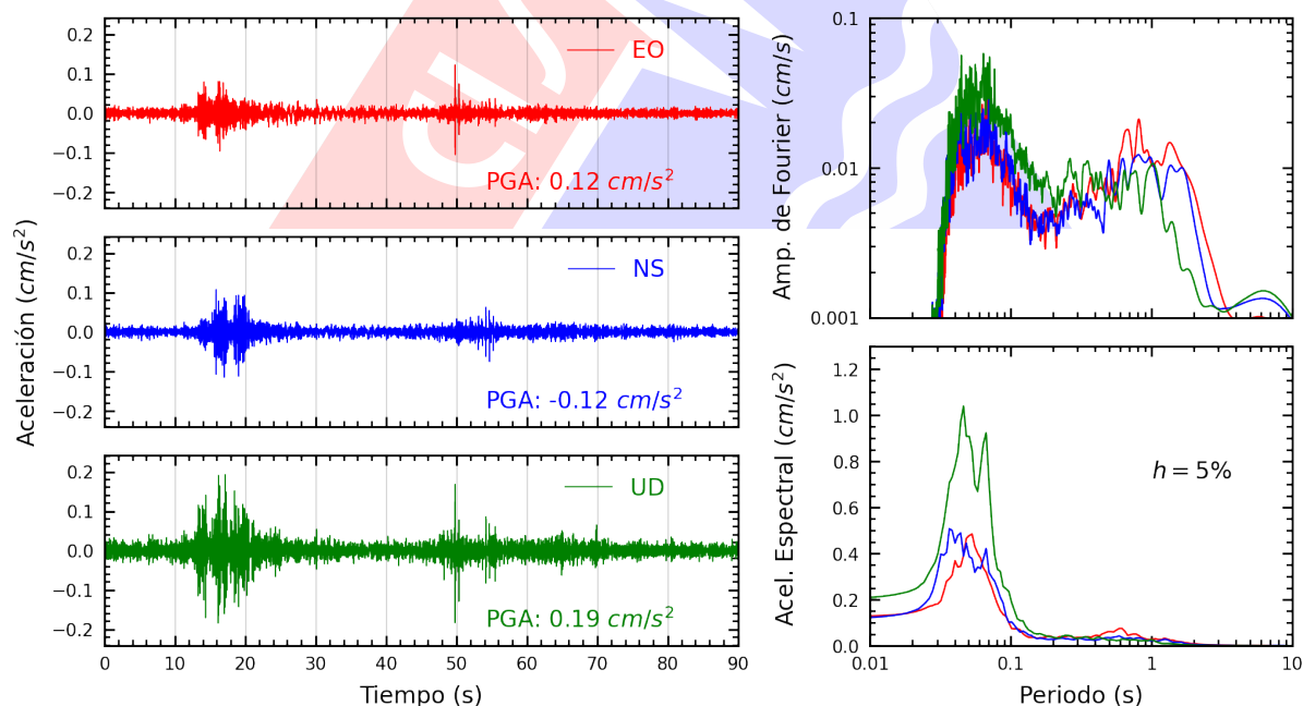
Figura A.8: Registros tiempo-historia, espectros de Fourier y de respuesta en las direcciones EO, NS y vertical de la estación SCCUS. Sismo de Camana, Camana - Arequipa del 2025-06-10, 22:04:21 (Hora local)
