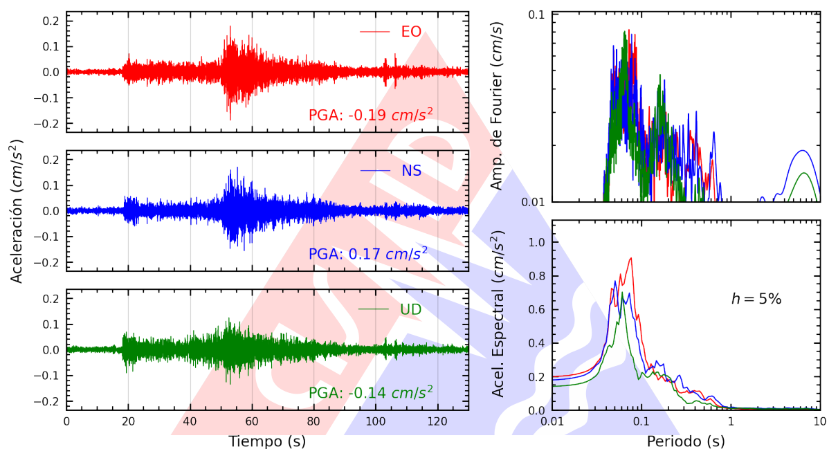
Figura A.9: Registros tiempo-historia, espectros de Fourier y de respuesta en las direcciones EO, NS y vertical de la estación CREY. Sismo de Camana, Camana - Arequipa del 2025-06-10, 22:04:21 (Hora local)
