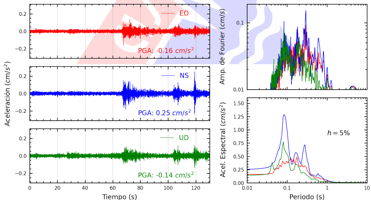
Figura A.6: Registros tiempo-historia, espectros de Fourier y de respuesta en las direcciones EO, NS y vertical de la estación UNICA. Sismo de Camana, Camana - Arequipa del 2025-06-10, 22:04:21 (Hora local)
