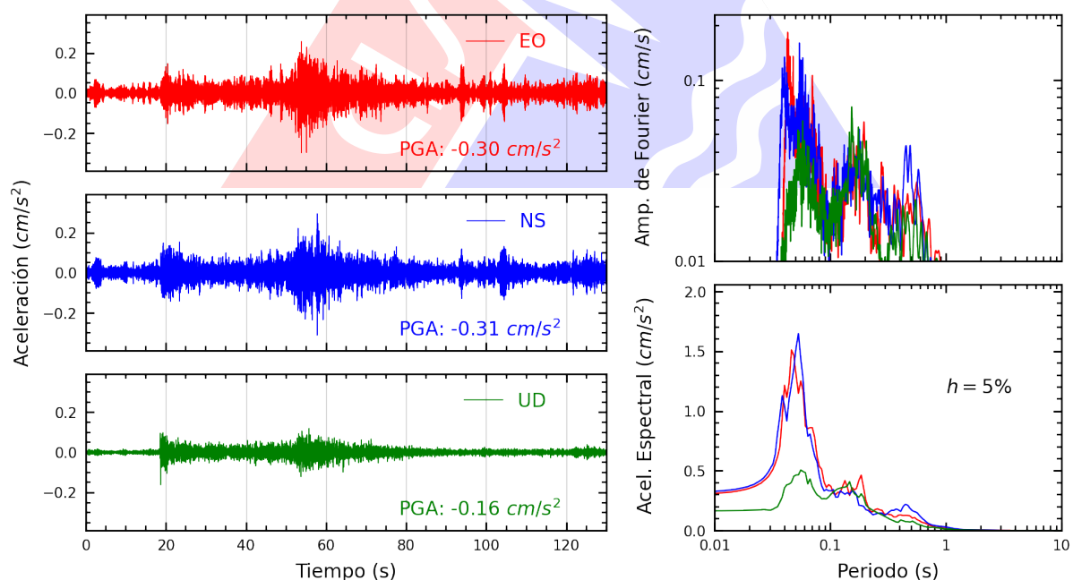
Figura A.4: Registros tiempo-historia, espectros de Fourier y de respuesta en las direcciones EO, NS y vertical de la estación UPTAC. Sismo de Camana, Camana - Arequipa del 2025-06-10, 22:04:21 (Hora local)
