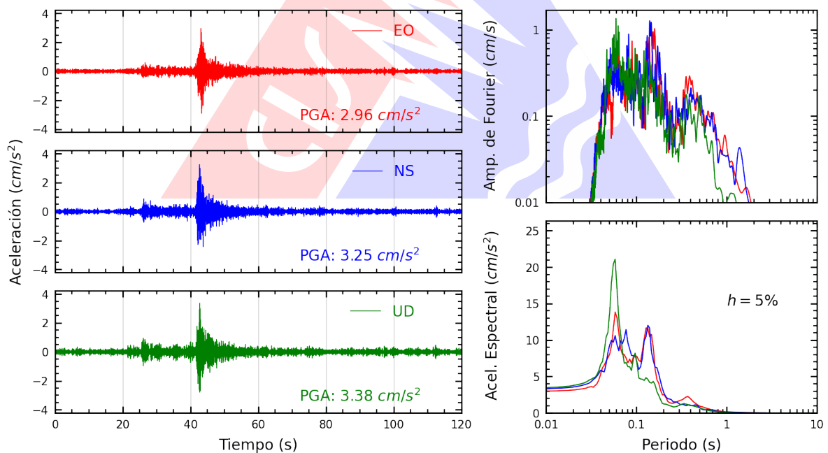
Figura A.2: Registros tiempo-historia, espectros de Fourier y de respuesta en las direcciones EO, NS y vertical de la estación SCAR2. Sismo de Camana, Camana - Arequipa del 2025-06-10, 22:04:21 (Hora local)
