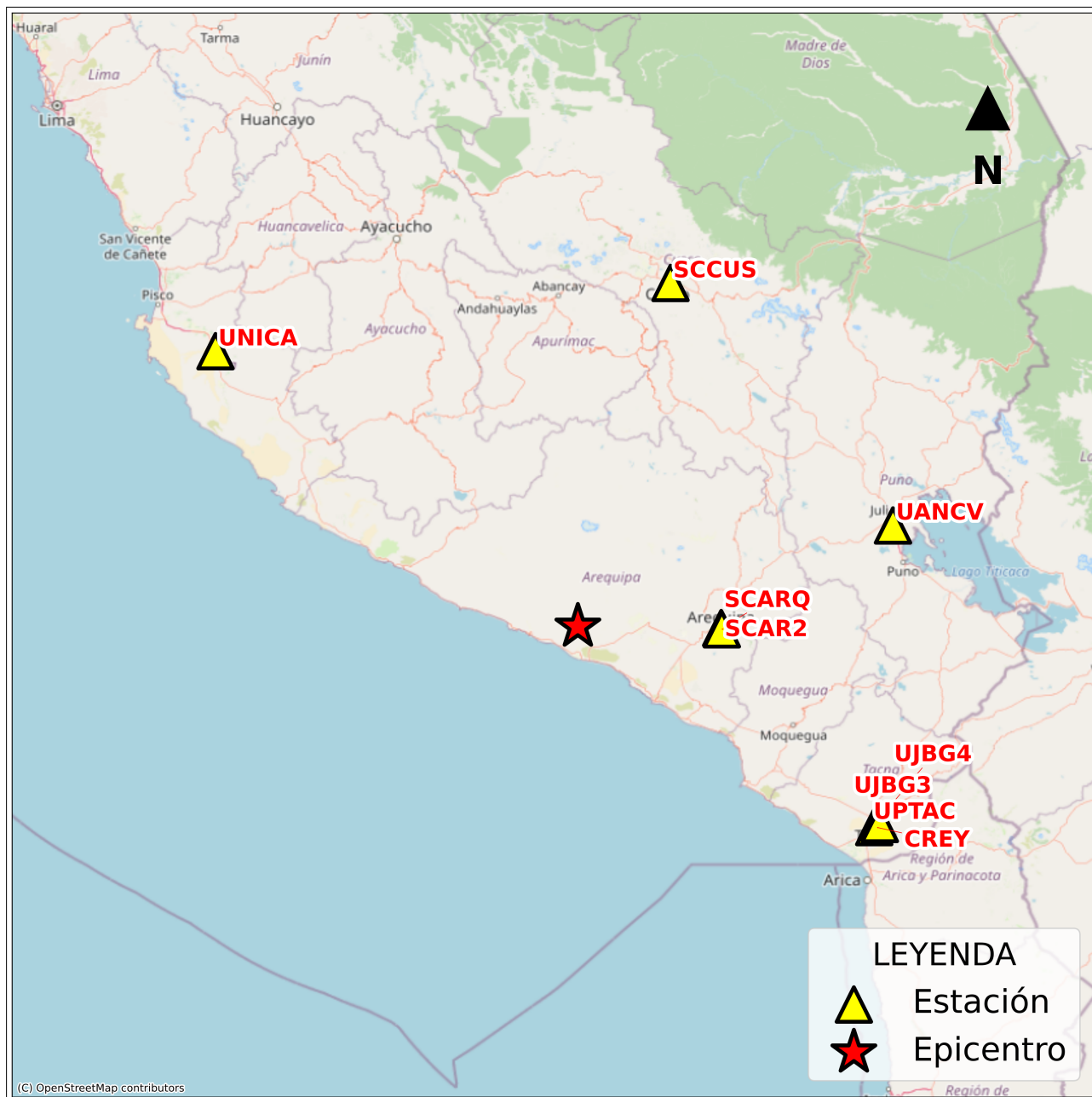
Figura 2: Mapa de ubicación de la(s) estación(es) acelerográfica(s) correspondiente(s) al Sismo de Camana, Camana - Arequipa del 10 de junio de 2025 a las 22:04:21 (hora local)
