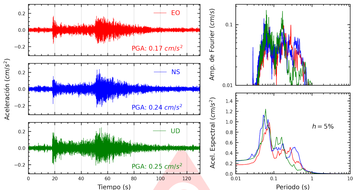
Figura A.7: Registros tiempo-historia, espectros de Fourier y de respuesta en las direcciones EO, NS y vertical de la estación UJBG4. Sismo de Camana, Camana - Arequipa del 2025-06-10, 22:04:21 (Hora local)
