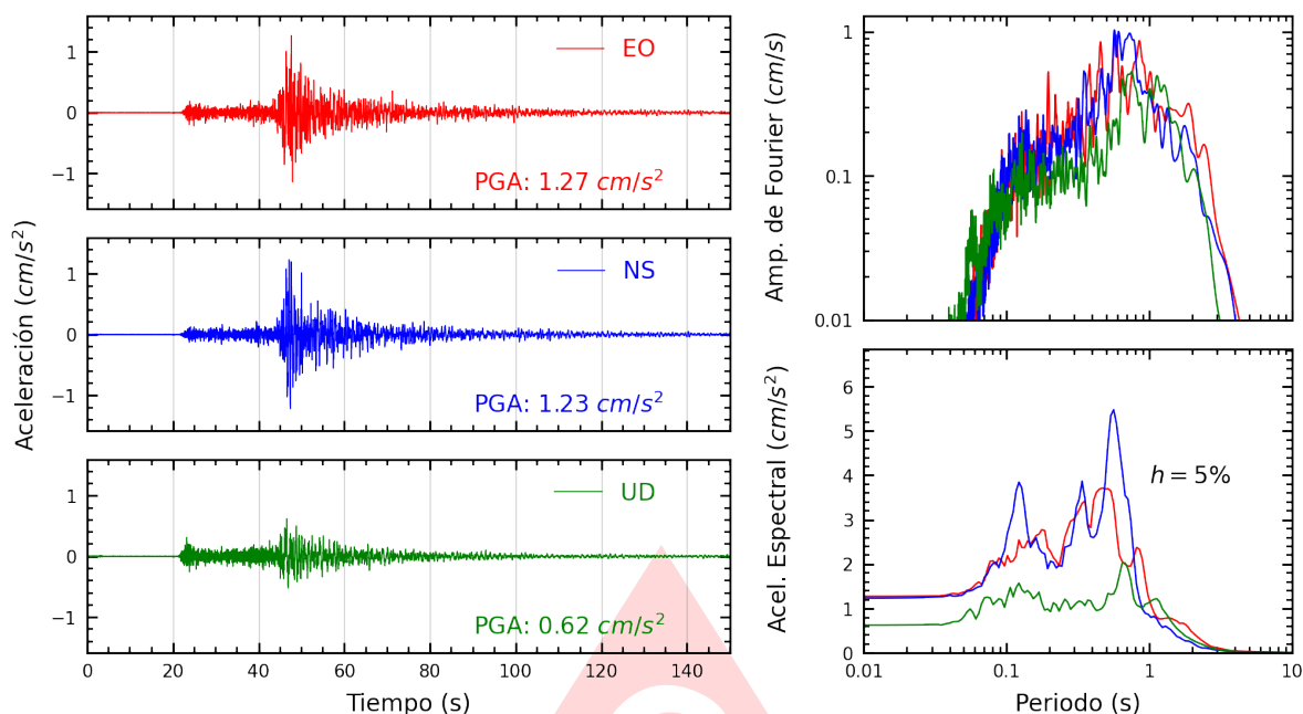
Figura A.5: Registros tiempo-historia, espectros de Fourier y de respuesta en las direcciones EO, NS y vertical de la estación UNC. Sismo de Lambayeque, Lambayeque - Lambayeque del 2025-06-11, 22:36:10 (Hora local)
