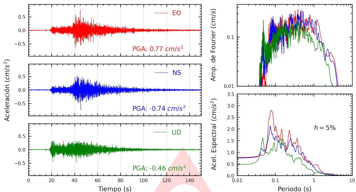
Figura A.9: Registros tiempo-historia, espectros de Fourier y de respuesta en las direcciones EO, NS y vertical de la estación UNF. Sismo de Lambayeque, Lambayeque - Lambayeque del 2025-06-11, 22:36:10 (Hora local)
