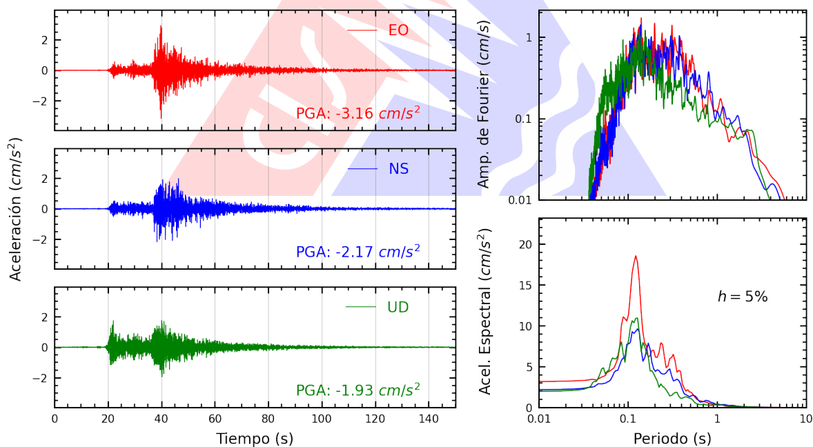
Figura A.2: Registros tiempo-historia, espectros de Fourier y de respuesta en las direcciones EO, NS y vertical de la estación UNP. Sismo de Lambayeque, Lambayeque - Lambayeque del 2025-06-11, 22:36:10 (Hora local)
