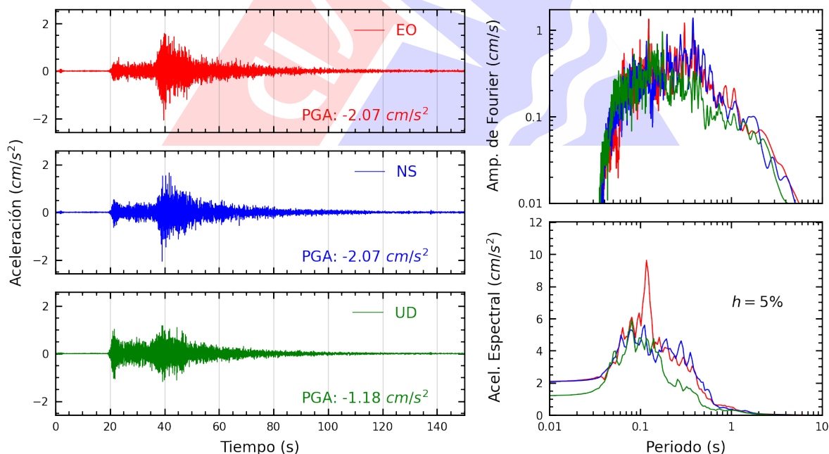
Figura A.4: Registros tiempo-historia, espectros de Fourier y de respuesta en las direcciones EO, NS y vertical de la estación UPAOP. Sismo de Lambayeque, Lambayeque - Lambayeque del 2025-06-11, 22:36:10 (Hora local)
