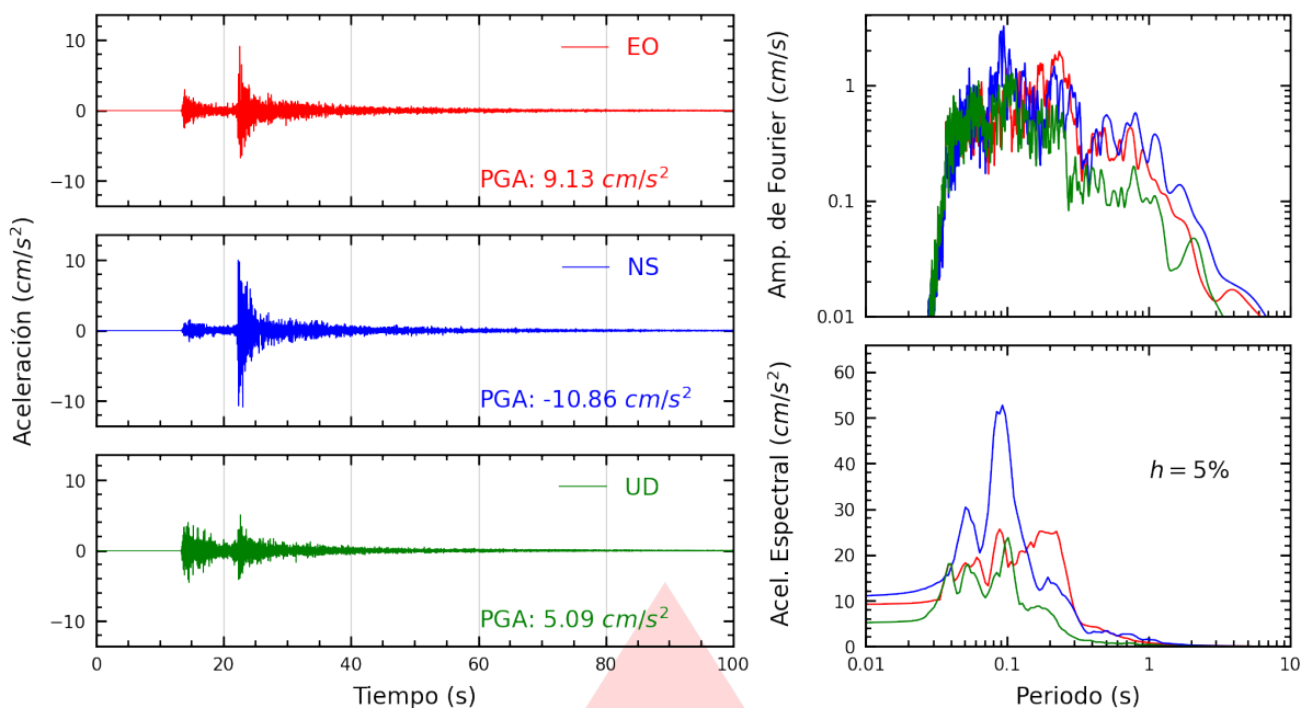
Figura A.1: Registros tiempo-historia, espectros de Fourier y de respuesta en las direcciones EO, NS y vertical de la estación SCCHI. Sismo de Lambayeque, Lambayeque - Lambayeque del 2025-06-11, 22:36:10 (Hora local)
