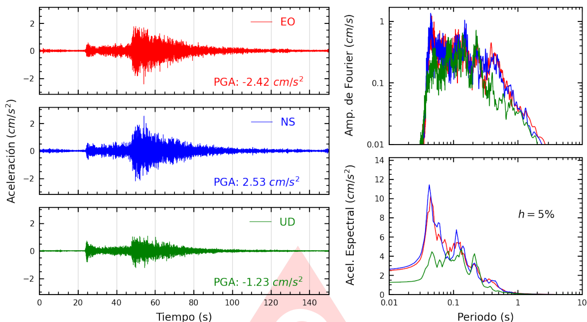
Figura A.3: Registros tiempo-historia, espectros de Fourier y de respuesta en las direcciones EO, NS y vertical de la estación SCTRU. Sismo de Lambayeque, Lambayeque - Lambayeque del 2025-06-11, 22:36:10 (Hora local)
