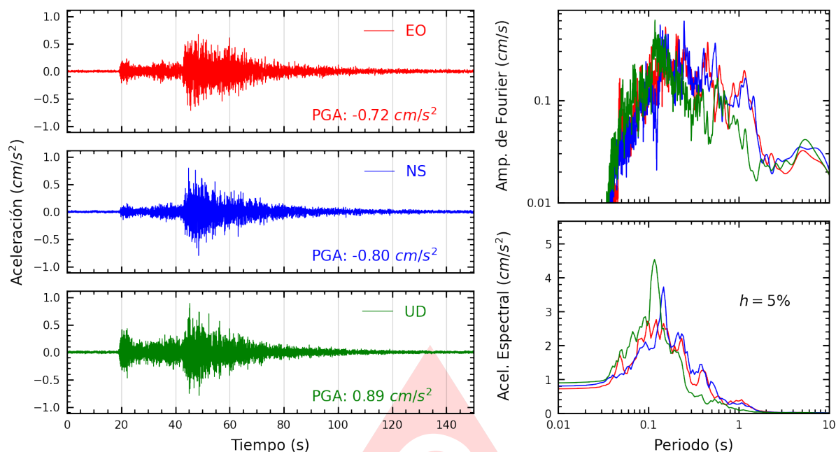
Figura A.7: Registros tiempo-historia, espectros de Fourier y de respuesta en las direcciones EO, NS y vertical de la estación UPAOT. Sismo de Lambayeque, Lambayeque - Lambayeque del 2025-06-11, 22:36:10 (Hora local)
