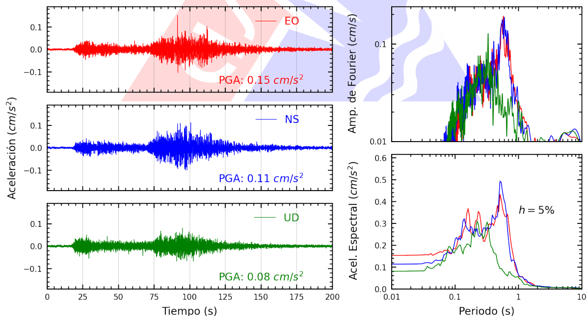
Figura A.10: Registros tiempo-historia, espectros de Fourier y de respuesta en las direcciones EO, NS y vertical de la estación CARAL. Sismo de Lambayeque, Lambayeque - Lambayeque del 2025-06-11, 22:36:10 (Hora local)
