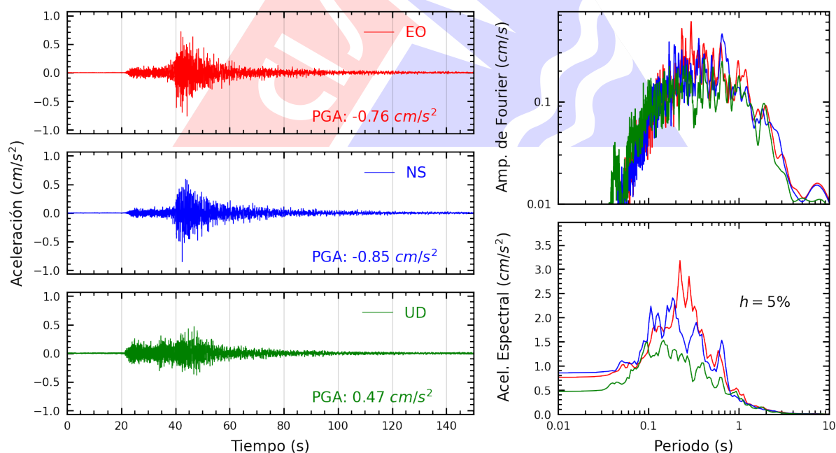
Figura A.8: Registros tiempo-historia, espectros de Fourier y de respuesta en las direcciones EO, NS y vertical de la estación UNJ. Sismo de Lambayeque, Lambayeque - Lambayeque del 2025-06-11, 22:36:10 (Hora local)
