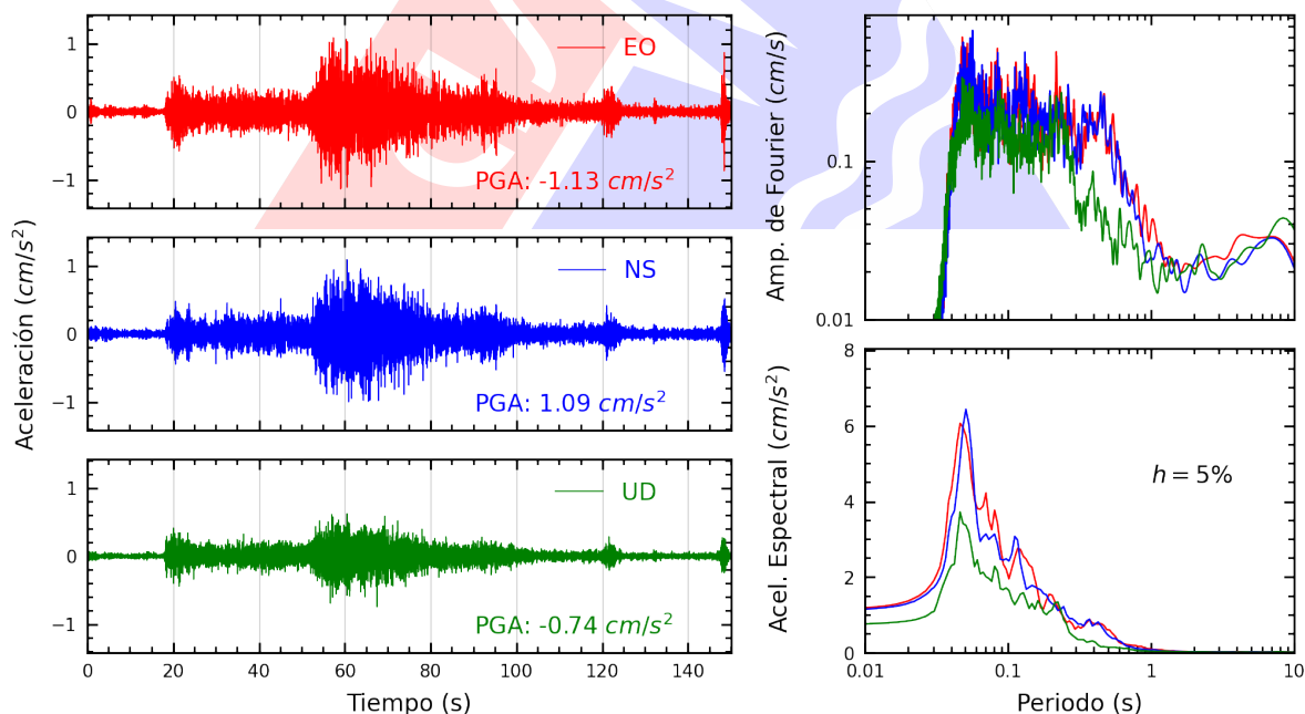
Figura A.6: Registros tiempo-historia, espectros de Fourier y de respuesta en las direcciones EO, NS y vertical de la estación USP. Sismo de Lambayeque, Lambayeque - Lambayeque del 2025-06-11, 22:36:10 (Hora local)
