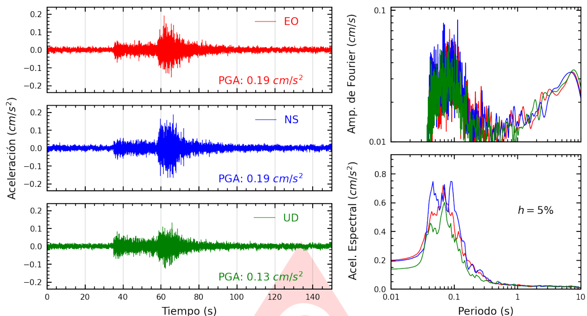
Figura A.31: Registros tiempo-historia, espectros de Fourier y de respuesta en las direcciones EO, NS y vertical de la estación SERVI. Sismo de Copa, Cajatambo - Lima del 2025-06-15, 00:52:12 (Hora local)
