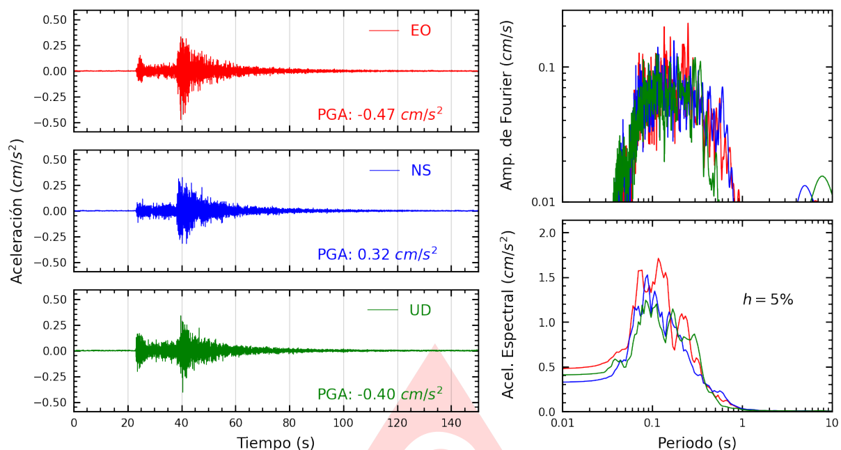
Figura A.11: Registros tiempo-historia, espectros de Fourier y de respuesta en las direcciones EO, NS y vertical de la estación CARAL. Sismo de Copa, Cajatambo - Lima del 2025-06-15, 00:52:12 (Hora local)
