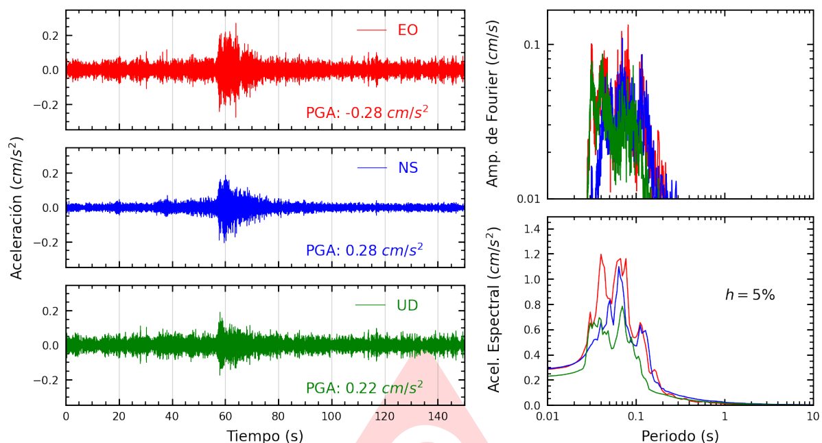
Figura A.19: Registros tiempo-historia, espectros de Fourier y de respuesta en las direcciones EO, NS y vertical de la estación ATARJ. Sismo de Copa, Cajatambo - Lima del 2025-06-15, 00:52:12 (Hora local)
