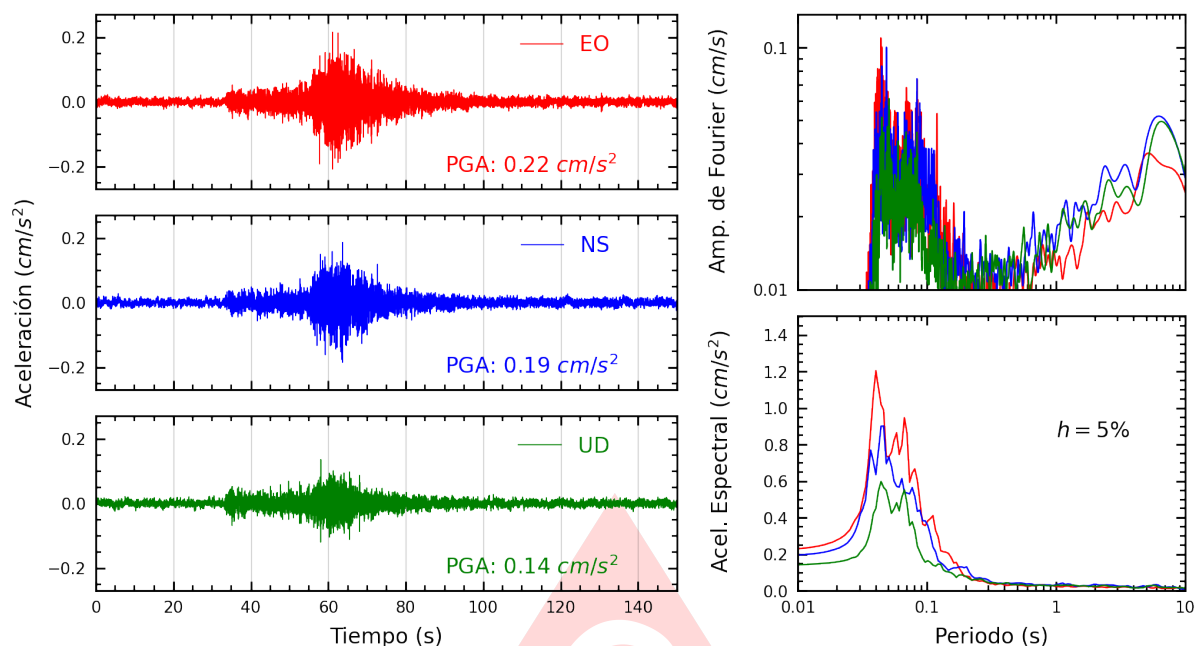
Figura A.29: Registros tiempo-historia, espectros de Fourier y de respuesta en las direcciones EO, NS y vertical de la estación UCSS. Sismo de Copa, Cajatambo - Lima del 2025-06-15, 00:52:12 (Hora local)
