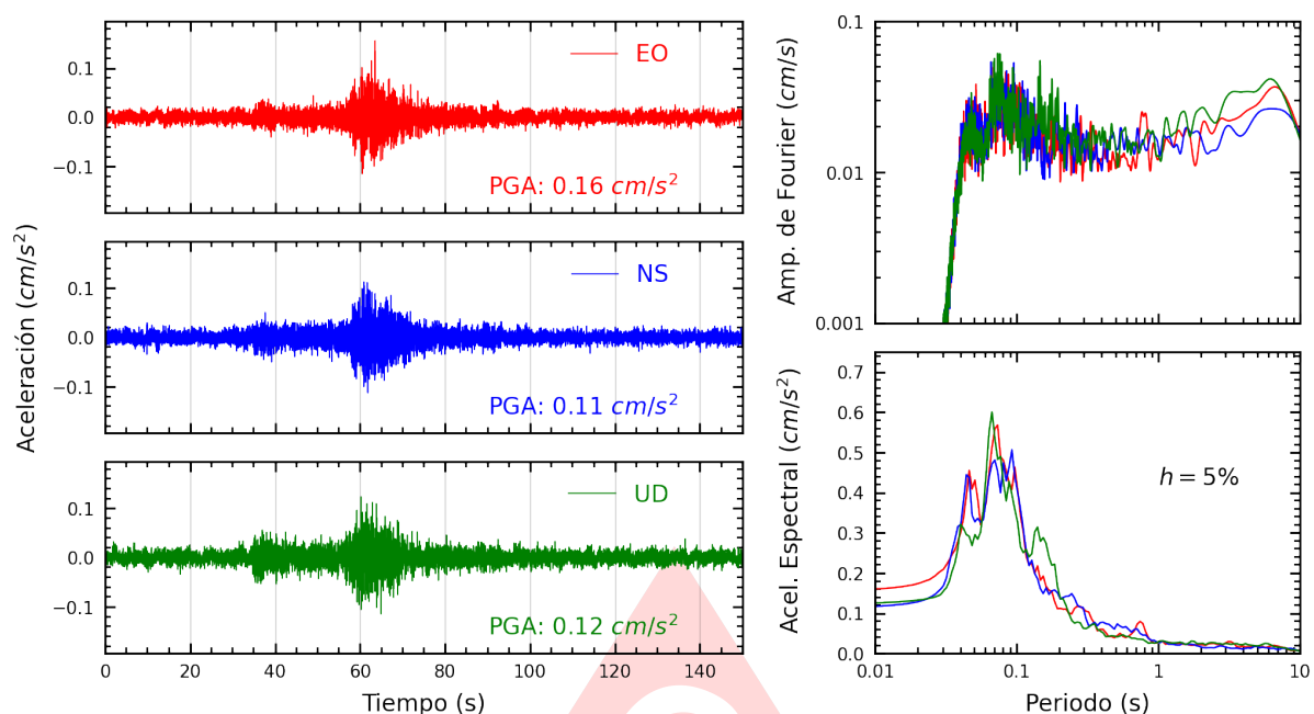
Figura A.33: Registros tiempo-historia, espectros de Fourier y de respuesta en las direcciones EO, NS y vertical de la estación UNFV. Sismo de Copa, Cajatambo - Lima del 2025-06-15, 00:52:12 (Hora local)
