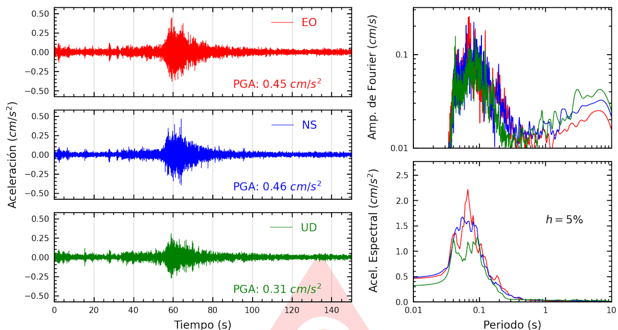
Figura A.13: Registros tiempo-historia, espectros de Fourier y de respuesta en las direcciones EO, NS y vertical de la estación INDEP. Sismo de Copa, Cajatambo - Lima del 2025-06-15, 00:52:12 (Hora local)
