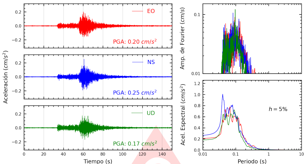
Figura A.23: Registros tiempo-historia, espectros de Fourier y de respuesta en las direcciones EO, NS y vertical de la estación JALV2. Sismo de Copa, Cajatambo - Lima del 2025-06-15, 00:52:12 (Hora local)
