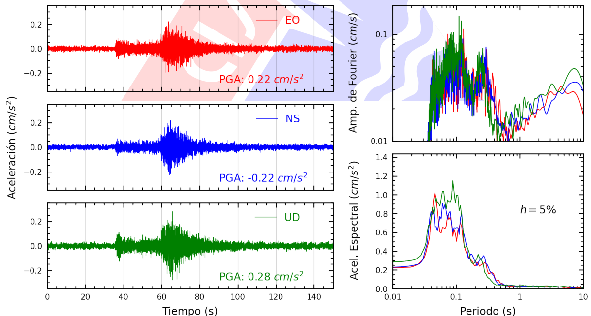
Figura A.18: Registros tiempo-historia, espectros de Fourier y de respuesta en las direcciones EO, NS y vertical de la estación SOVES. Sismo de Copa, Cajatambo - Lima del 2025-06-15, 00:52:12 (Hora local)
