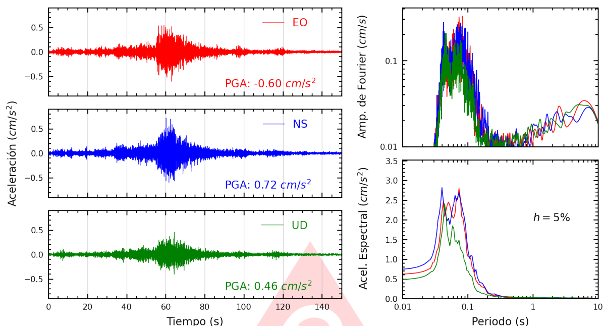
Figura A.5: Registros tiempo-historia, espectros de Fourier y de respuesta en las direcciones EO, NS y vertical de la estación JOSEO. Sismo de Copa, Cajatambo - Lima del 2025-06-15, 00:52:12 (Hora local)
