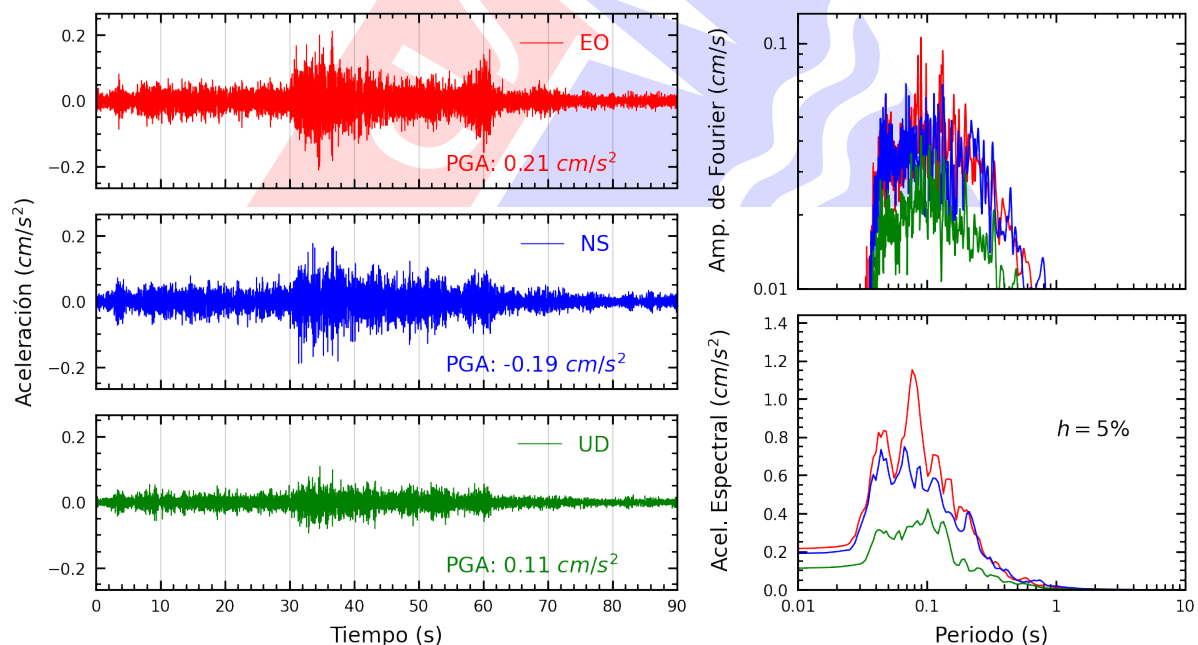
Figura A.30: Registros tiempo-historia, espectros de Fourier y de respuesta en las direcciones EO, NS y vertical de la estación BRIS2. Sismo de Copa, Cajatambo - Lima del 2025-06-15, 00:52:12 (Hora local)
