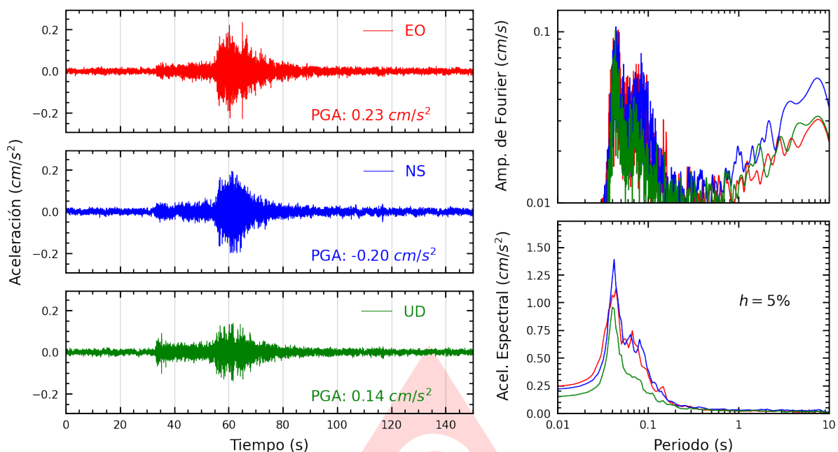
Figura A.27: Registros tiempo-historia, espectros de Fourier y de respuesta en las direcciones EO, NS y vertical de la estación SJLCE. Sismo de Copa, Cajatambo - Lima del 2025-06-15, 00:52:12 (Hora local)
