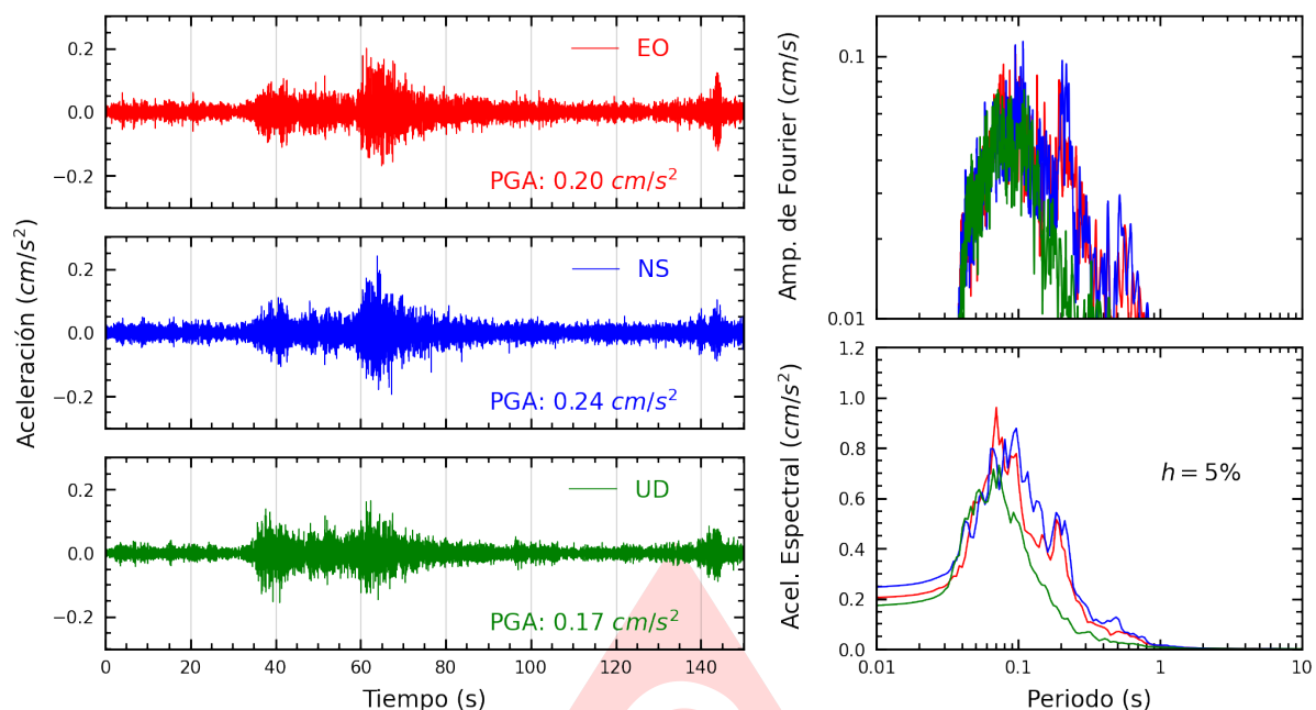
Figura A.25: Registros tiempo-historia, espectros de Fourier y de respuesta en las direcciones EO, NS y vertical de la estación SCCHO. Sismo de Copa, Cajatambo - Lima del 2025-06-15, 00:52:12 (Hora local)
