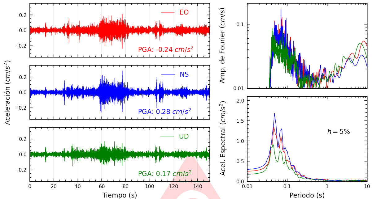
Figura A.17: Registros tiempo-historia, espectros de Fourier y de respuesta en las direcciones EO, NS y vertical de la estación UPCSM. Sismo de Copa, Cajatambo - Lima del 2025-06-15, 00:52:12 (Hora local)
