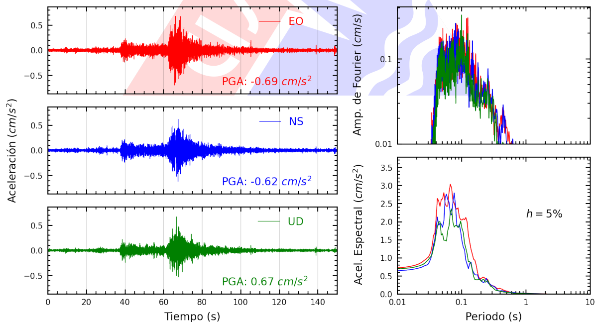
Figura A.6: Registros tiempo-historia, espectros de Fourier y de respuesta en las direcciones EO, NS y vertical de la estación PHER2. Sismo de Copa, Cajatambo - Lima del 2025-06-15, 00:52:12 (Hora local)
