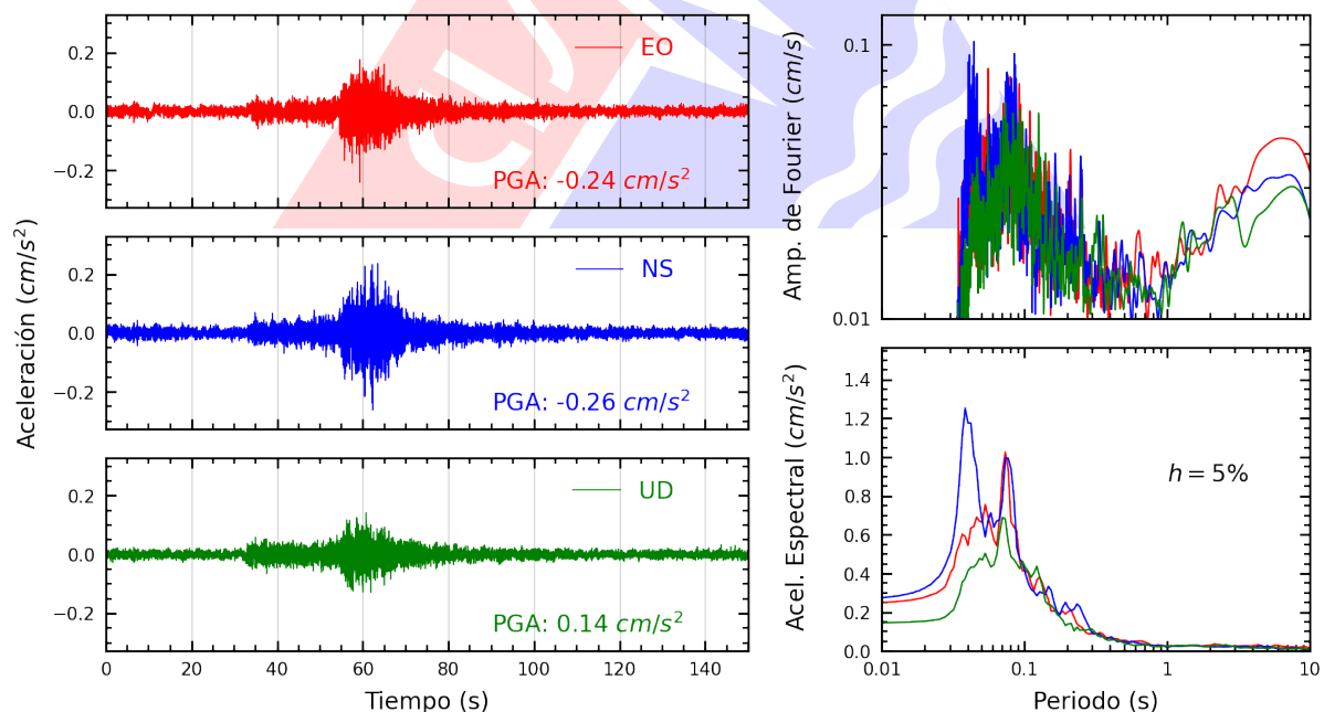
Figura A.22: Registros tiempo-historia, espectros de Fourier y de respuesta en las direcciones EO, NS y vertical de la estación COMAS. Sismo de Copa, Cajatambo - Lima del 2025-06-15, 00:52:12 (Hora local)
