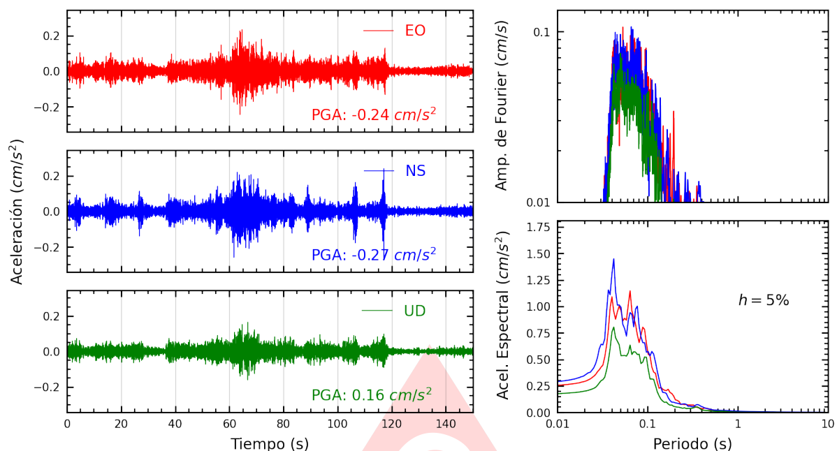
Figura A.21: Registros tiempo-historia, espectros de Fourier y de respuesta en las direcciones EO, NS y vertical de la estación PACHA. Sismo de Copa, Cajatambo - Lima del 2025-06-15, 00:52:12 (Hora local)
