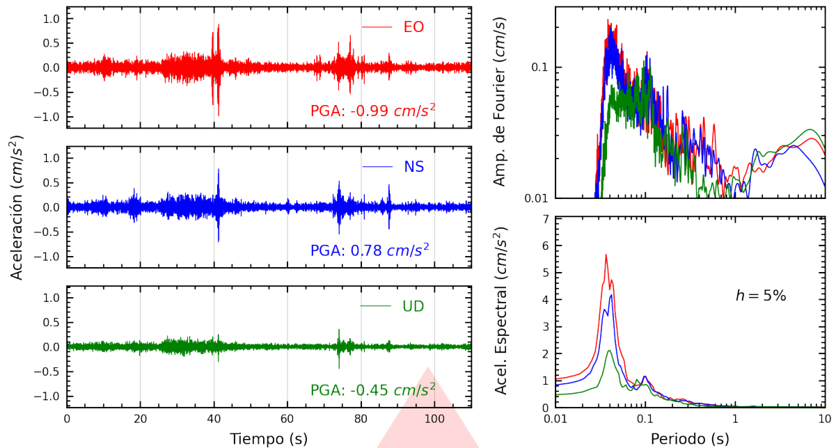
Figura A.1: Registros tiempo-historia, espectros de Fourier y de respuesta en las direcciones EO, NS y vertical de la estación OLIVO. Sismo de Copa, Cajatambo - Lima del 2025-06-15, 00:52:12 (Hora local)
