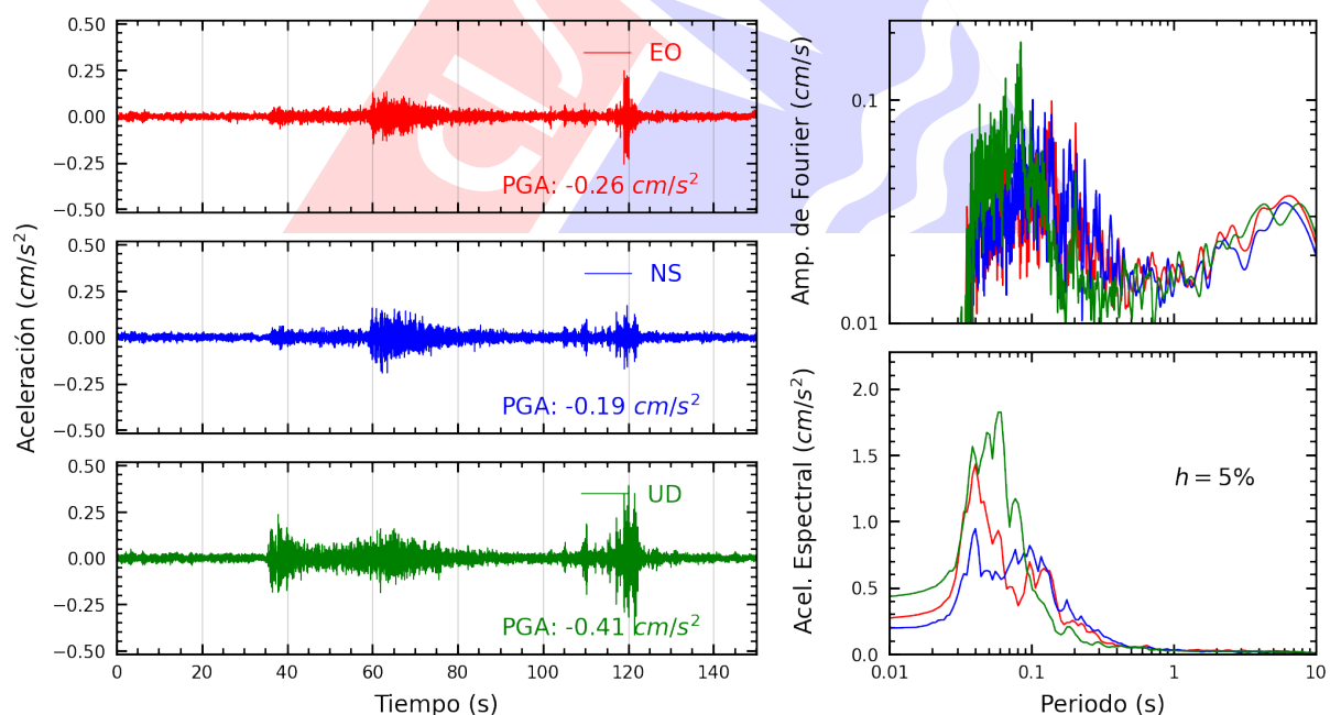
Figura A.14: Registros tiempo-historia, espectros de Fourier y de respuesta en las direcciones EO, NS y vertical de la estación SOCHO. Sismo de Copa, Cajatambo - Lima del 2025-06-15, 00:52:12 (Hora local)
