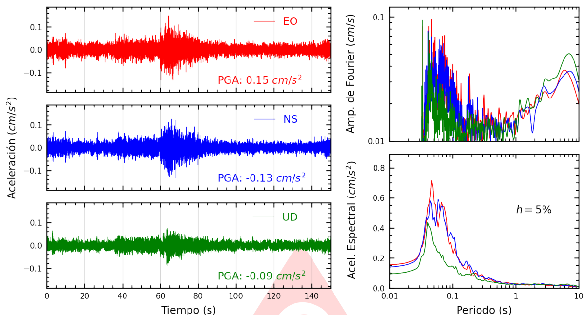
Figura A.35: Registros tiempo-historia, espectros de Fourier y de respuesta en las direcciones EO, NS y vertical de la estación UPCVI. Sismo de Copa, Cajatambo - Lima del 2025-06-15, 00:52:12 (Hora local)
