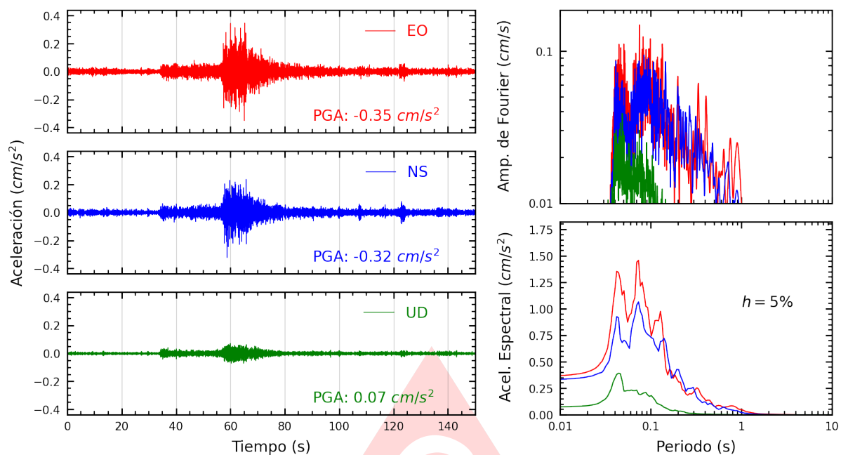
Figura A.15: Registros tiempo-historia, espectros de Fourier y de respuesta en las direcciones EO, NS y vertical de la estación UCVA2. Sismo de Copa, Cajatambo - Lima del 2025-06-15, 00:52:12 (Hora local)
