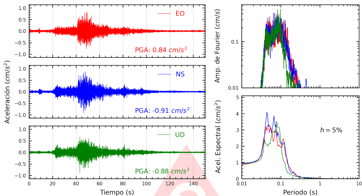
Figura A.3: Registros tiempo-historia, espectros de Fourier y de respuesta en las direcciones EO, NS y vertical de la estación SROS2. Sismo de Copa, Cajatambo - Lima del 2025-06-15, 00:52:12 (Hora local)
