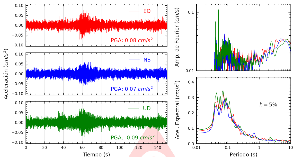
Figura A.39: Registros tiempo-historia, espectros de Fourier y de respuesta en las direcciones EO, NS y vertical de la estación BONDY. Sismo de Copa, Cajatambo - Lima del 2025-06-15, 00:52:12 (Hora local)
