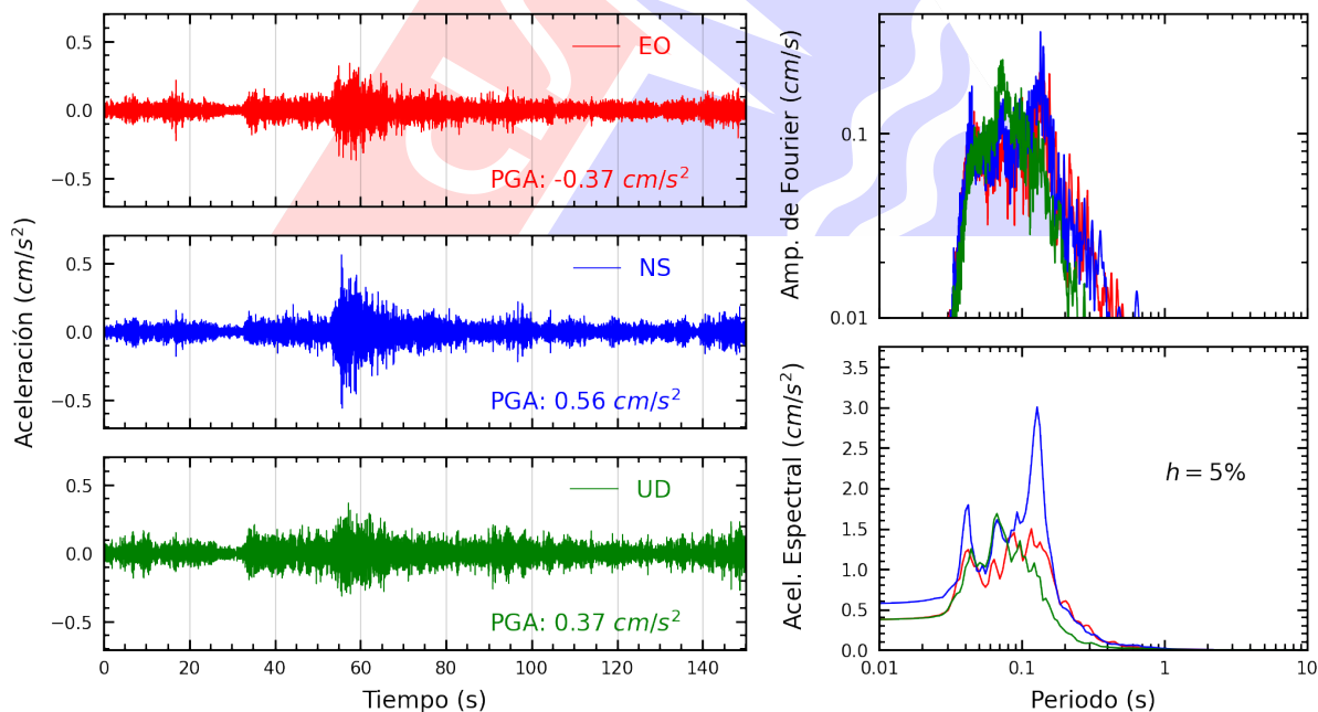
Figura A.10: Registros tiempo-historia, espectros de Fourier y de respuesta en las direcciones EO, NS y vertical de la estación CARA2. Sismo de Copa, Cajatambo - Lima del 2025-06-15, 00:52:12 (Hora local)
