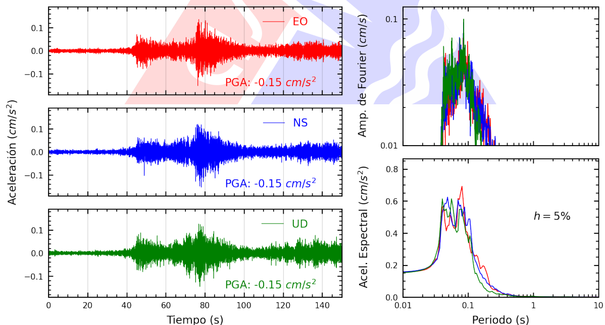
Figura A.34: Registros tiempo-historia, espectros de Fourier y de respuesta en las direcciones EO, NS y vertical de la estación ASIA. Sismo de Copa, Cajatambo - Lima del 2025-06-15, 00:52:12 (Hora local)
