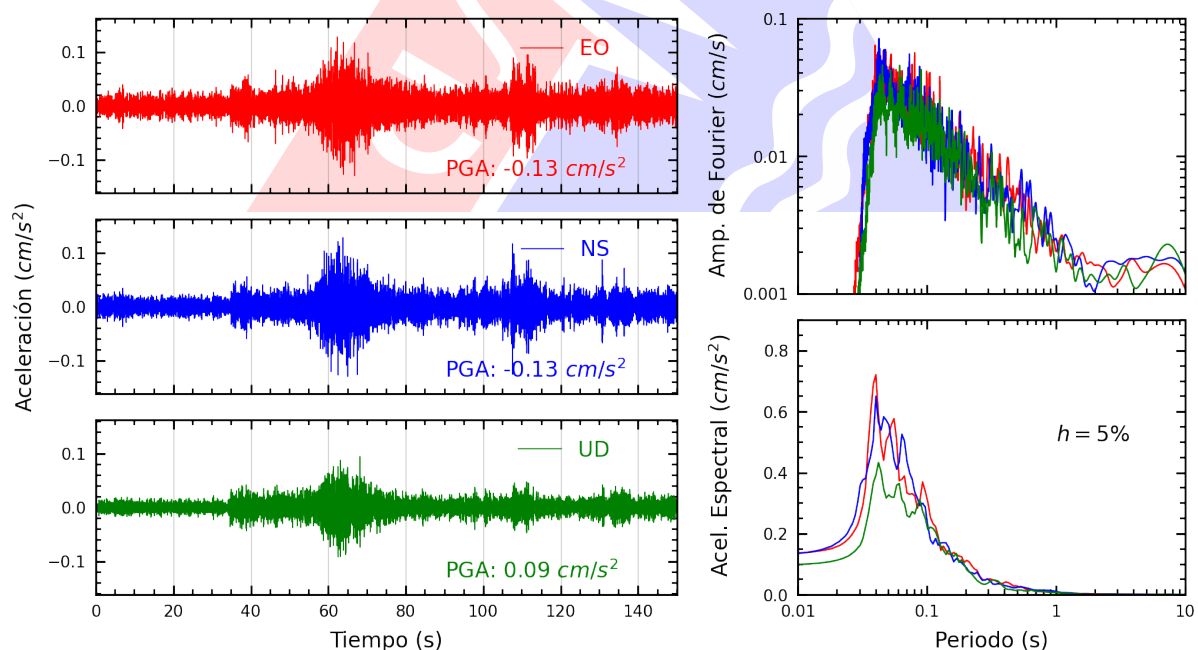
Figura A.36: Registros tiempo-historia, espectros de Fourier y de respuesta en las direcciones EO, NS y vertical de la estación BORJA. Sismo de Copa, Cajatambo - Lima del 2025-06-15, 00:52:12 (Hora local)
