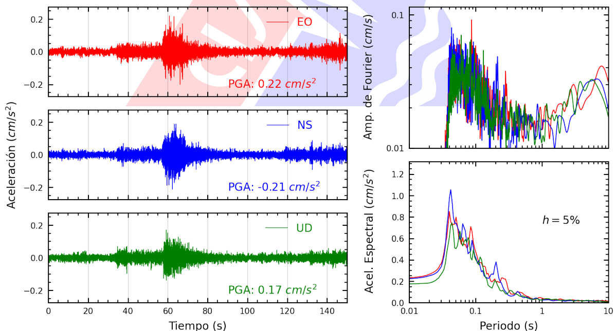
Figura A.28: Registros tiempo-historia, espectros de Fourier y de respuesta en las direcciones EO, NS y vertical de la estación IMCA. Sismo de Copa, Cajatambo - Lima del 2025-06-15, 00:52:12 (Hora local)
