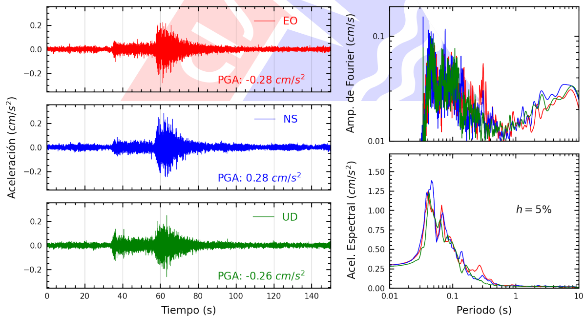
Figura A.16: Registros tiempo-historia, espectros de Fourier y de respuesta en las direcciones EO, NS y vertical de la estación USMP. Sismo de Copa, Cajatambo - Lima del 2025-06-15, 00:52:12 (Hora local)
