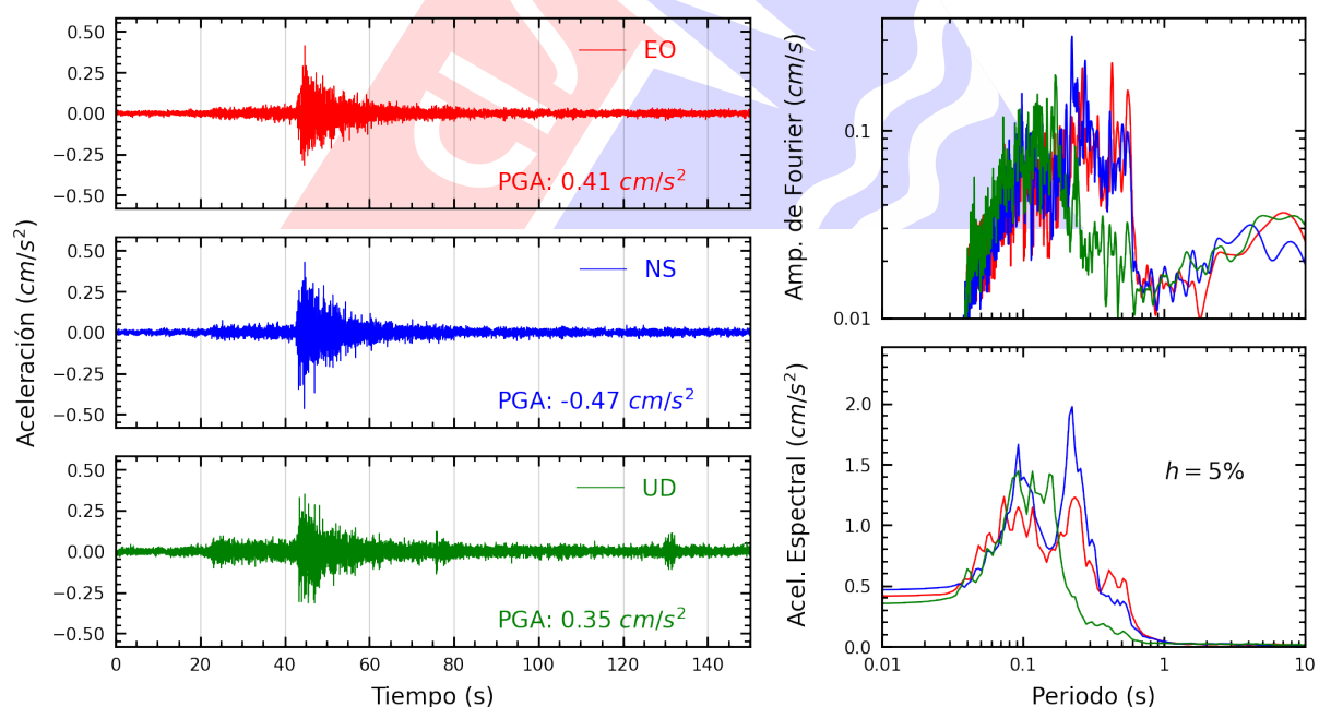
Figura A.12: Registros tiempo-historia, espectros de Fourier y de respuesta en las direcciones EO, NS y vertical de la estación MDPP. Sismo de Copa, Cajatambo - Lima del 2025-06-15, 00:52:12 (Hora local)
