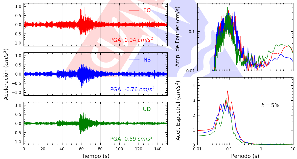
Figura A.2: Registros tiempo-historia, espectros de Fourier y de respuesta en las direcciones EO, NS y vertical de la estación USILM. Sismo de Copa, Cajatambo - Lima del 2025-06-15, 00:52:12 (Hora local)
