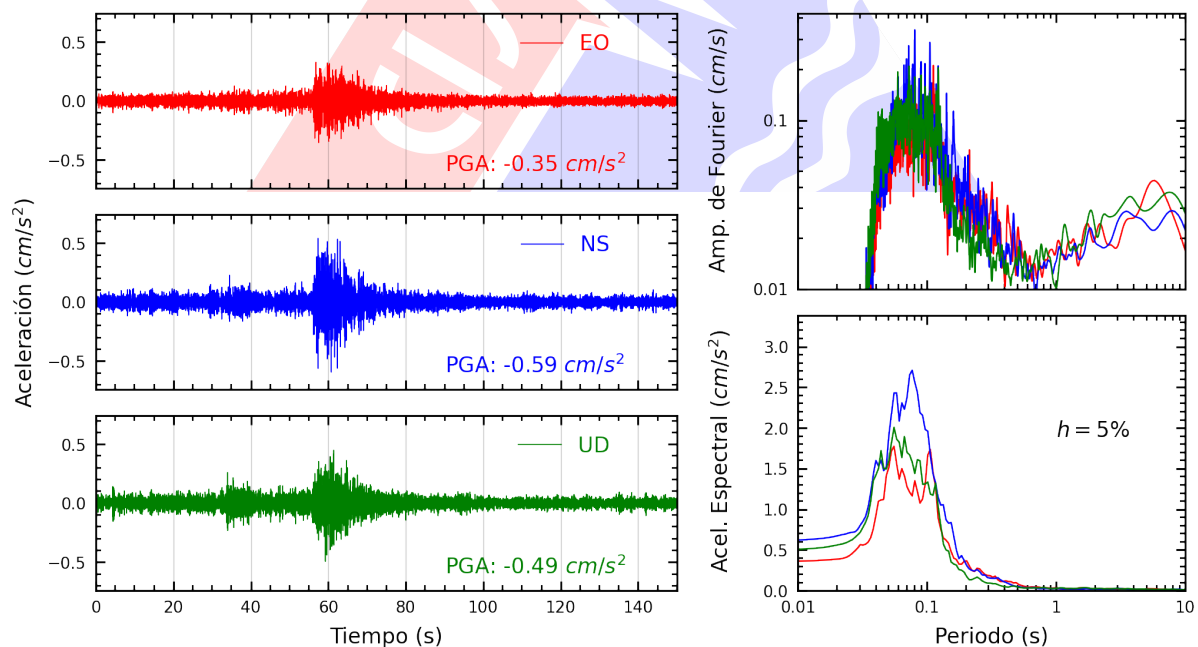
Figura A.8: Registros tiempo-historia, espectros de Fourier y de respuesta en las direcciones EO, NS y vertical de la estación SJLSC. Sismo de Copa, Cajatambo - Lima del 2025-06-15, 00:52:12 (Hora local)
