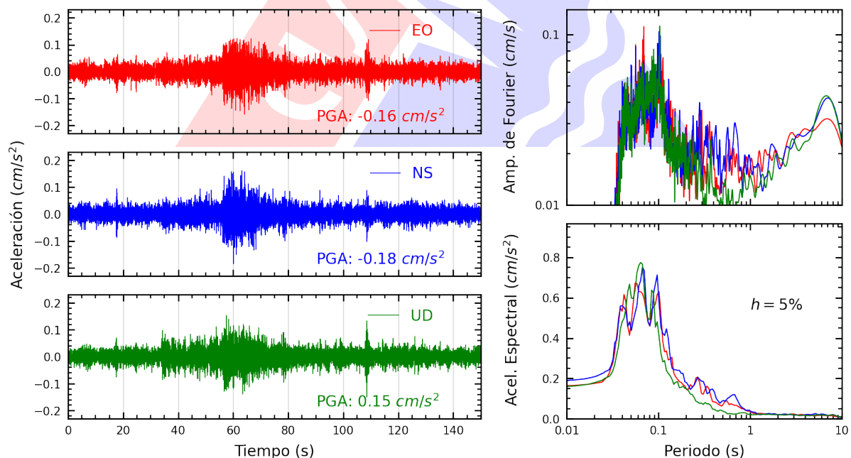
Figura A.32: Registros tiempo-historia, espectros de Fourier y de respuesta en las direcciones EO, NS y vertical de la estación MADRE. Sismo de Copa, Cajatambo - Lima del 2025-06-15, 00:52:12 (Hora local)
