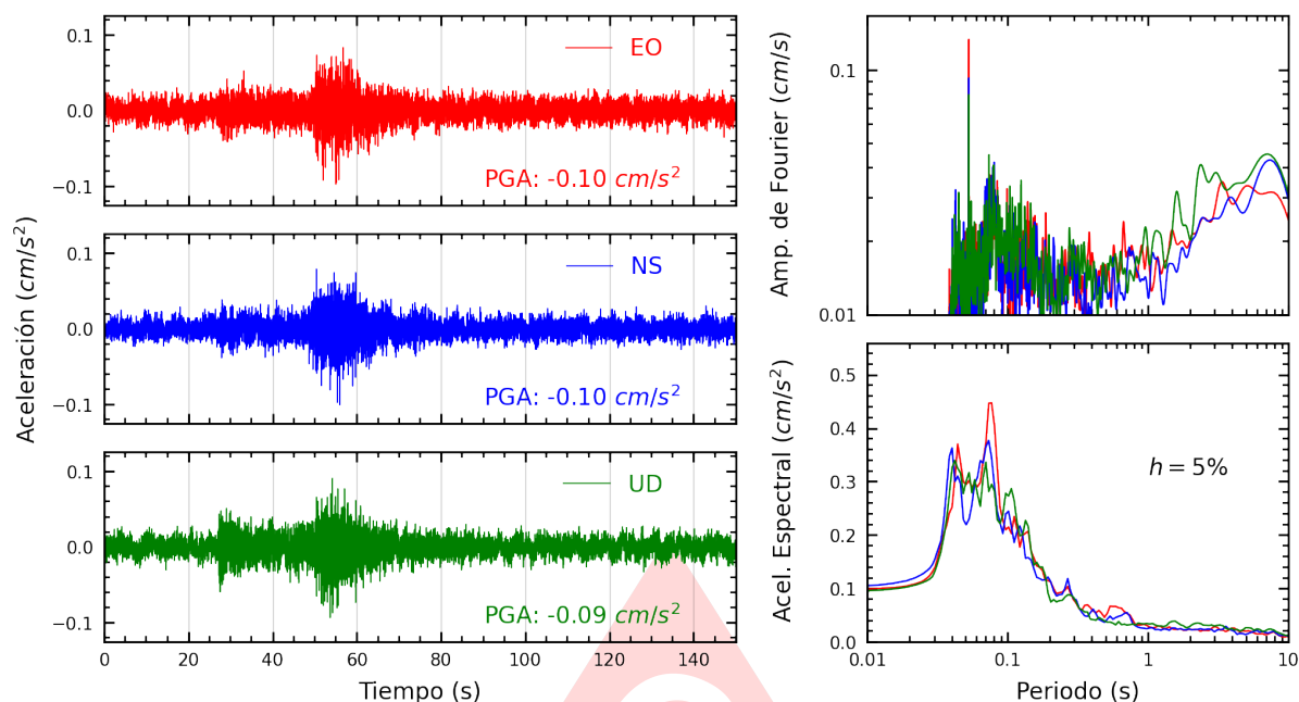
Figura A.37: Registros tiempo-historia, espectros de Fourier y de respuesta en las direcciones EO, NS y vertical de la estación UNMSM. Sismo de Copa, Cajatambo - Lima del 2025-06-15, 00:52:12 (Hora local)
