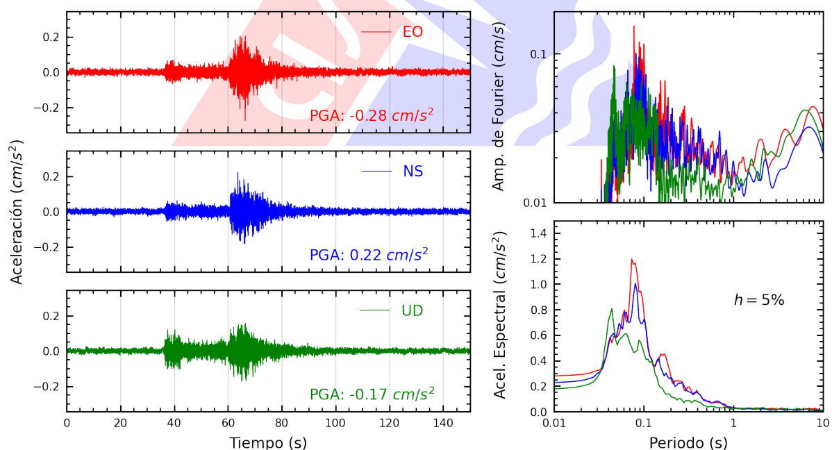
Figura A.20: Registros tiempo-historia, espectros de Fourier y de respuesta en las direcciones EO, NS y vertical de la estación USILP. Sismo de Copa, Cajatambo - Lima del 2025-06-15, 00:52:12 (Hora local)
