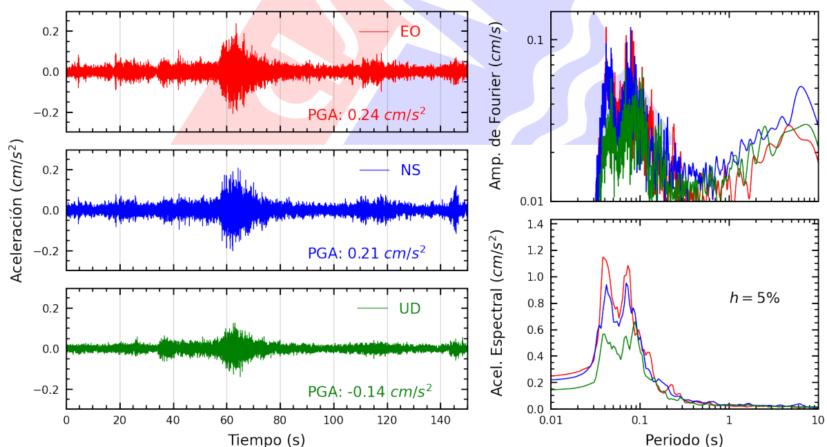
Figura A.26: Registros tiempo-historia, espectros de Fourier y de respuesta en las direcciones EO, NS y vertical de la estación CEPRE. Sismo de Copa, Cajatambo - Lima del 2025-06-15, 00:52:12 (Hora local)
