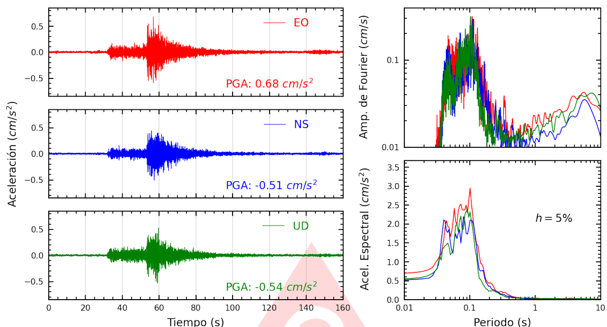
Figura A.7: Registros tiempo-historia, espectros de Fourier y de respuesta en las direcciones EO, NS y vertical de la estación AMORE. Sismo de Copa, Cajatambo - Lima del 2025-06-15, 00:52:12 (Hora local)
