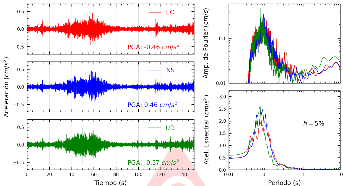
Figura A.9: Registros tiempo-historia, espectros de Fourier y de respuesta en las direcciones EO, NS y vertical de la estación SJLSV. Sismo de Copa, Cajatambo - Lima del 2025-06-15, 00:52:12 (Hora local)
