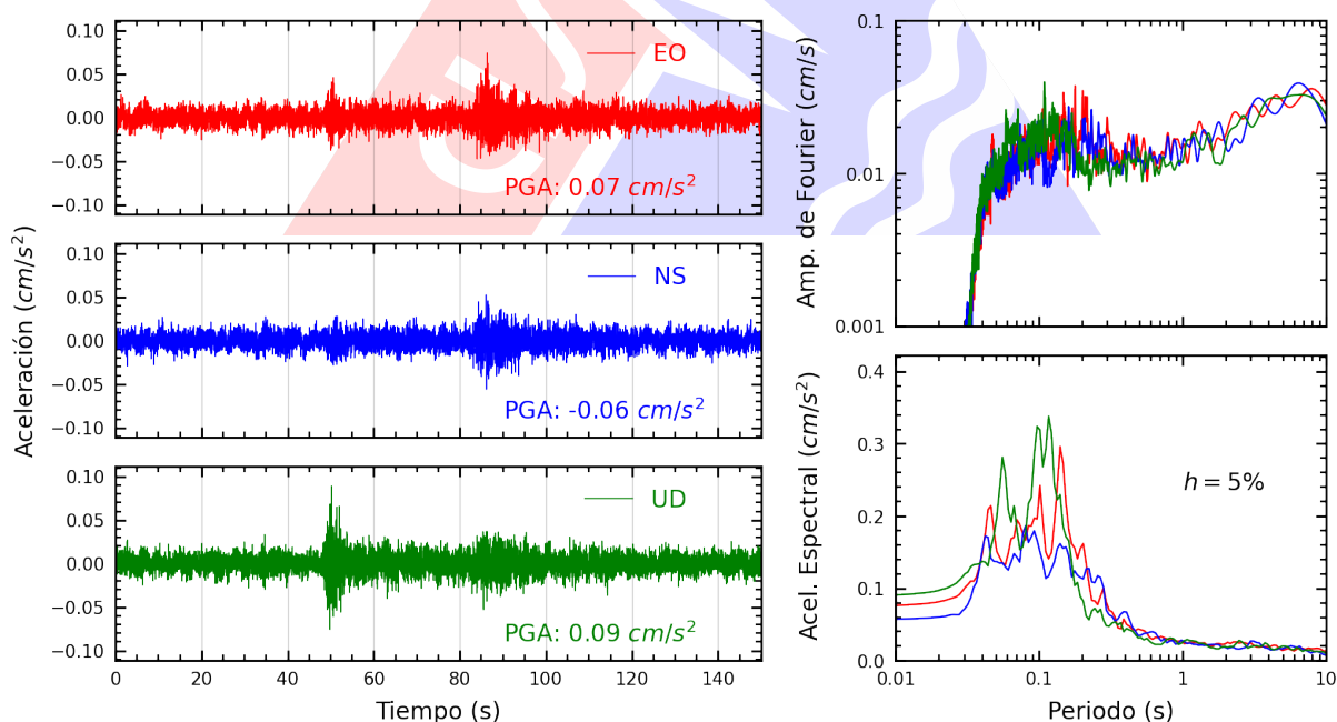
Figura A.38: Registros tiempo-historia, espectros de Fourier y de respuesta en las direcciones EO, NS y vertical de la estación UPAOT. Sismo de Copa, Cajatambo - Lima del 2025-06-15, 00:52:12 (Hora local)
