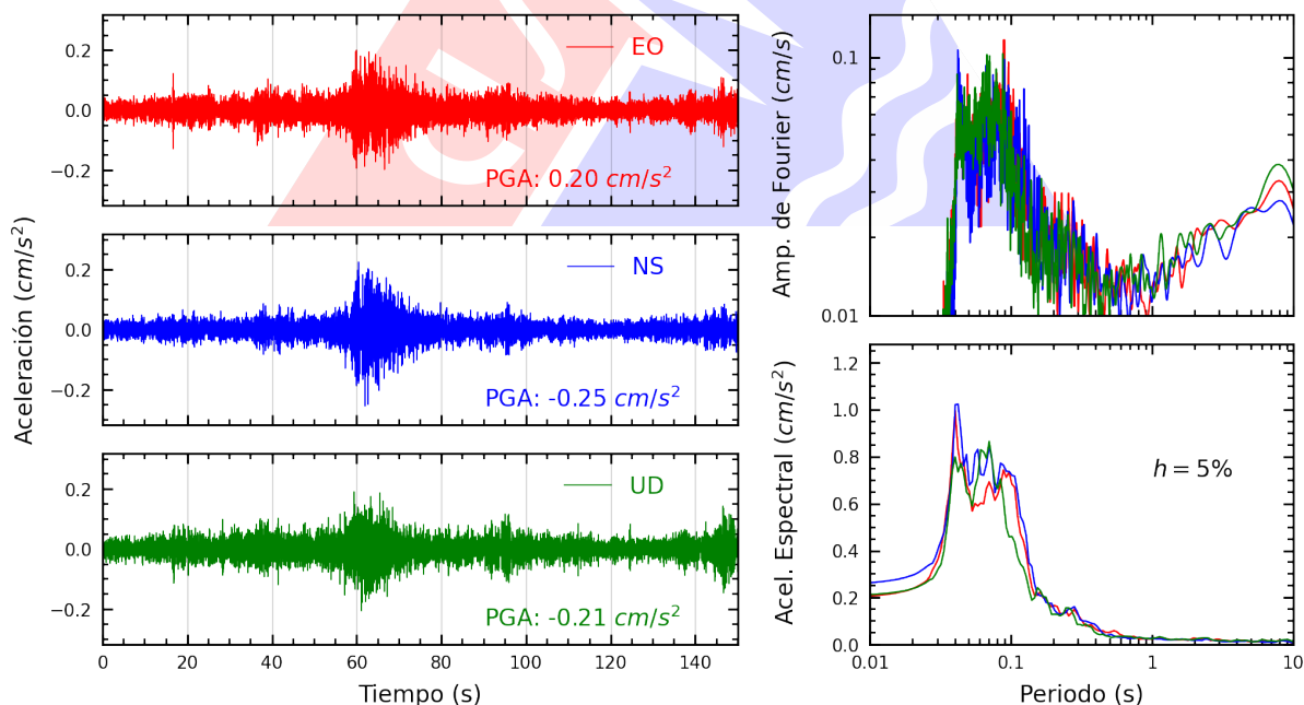
Figura A.24: Registros tiempo-historia, espectros de Fourier y de respuesta en las direcciones EO, NS y vertical de la estación URPPE. Sismo de Copa, Cajatambo - Lima del 2025-06-15, 00:52:12 (Hora local)
