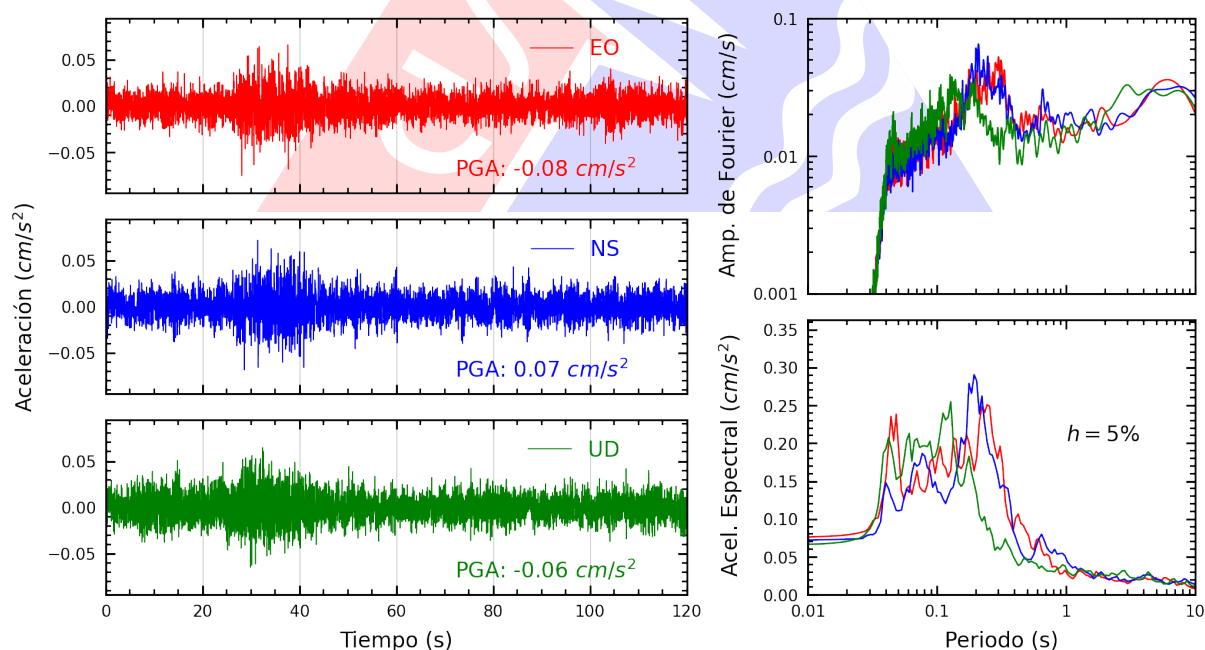
Figura A.40: Registros tiempo-historia, espectros de Fourier y de respuesta en las direcciones EO, NS y vertical de la estación DSMI. Sismo de Copa, Cajatambo - Lima del 2025-06-15, 00:52:12 (Hora local)
