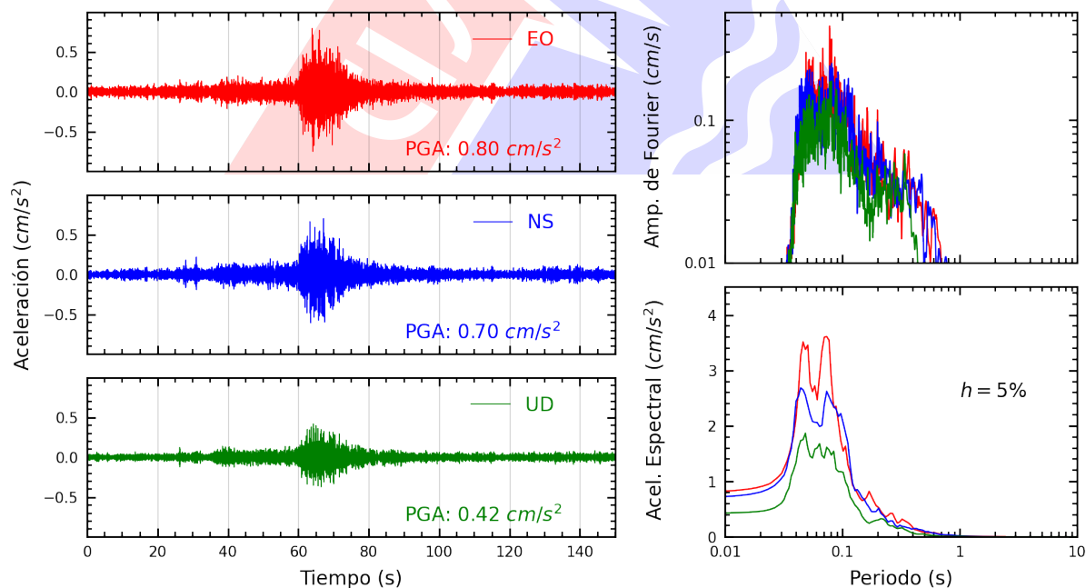
Figura A.4: Registros tiempo-historia, espectros de Fourier y de respuesta en las direcciones EO, NS y vertical de la estación UNTEL. Sismo de Copa, Cajatambo - Lima del 2025-06-15, 00:52:12 (Hora local)
