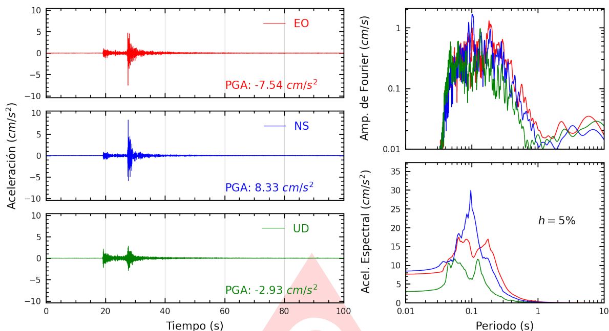
Figura A.3: Registros tiempo-historia, espectros de Fourier y de respuesta en las direcciones EO, NS y vertical de la estación USILP. Sismo de Provincia Constitucional del Callao , Callao - Lima del 2025-06-15, 12:03:46 (Hora local)
