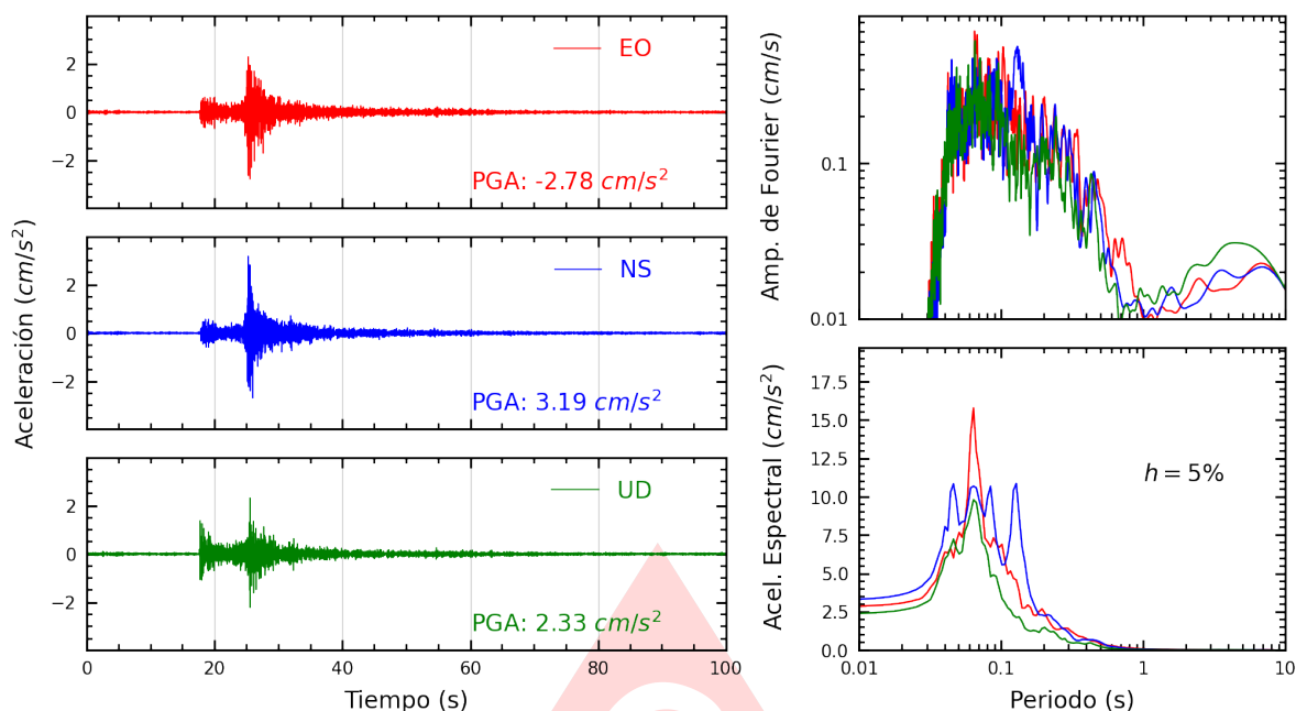
Figura A.25: Registros tiempo-historia, espectros de Fourier y de respuesta en las direcciones EO, NS y vertical de la estación URPE. Sismo de Provincia Constitucional del Callao, Callao - Lima del 2025-06-15, 12:03:46 (Hora local)
