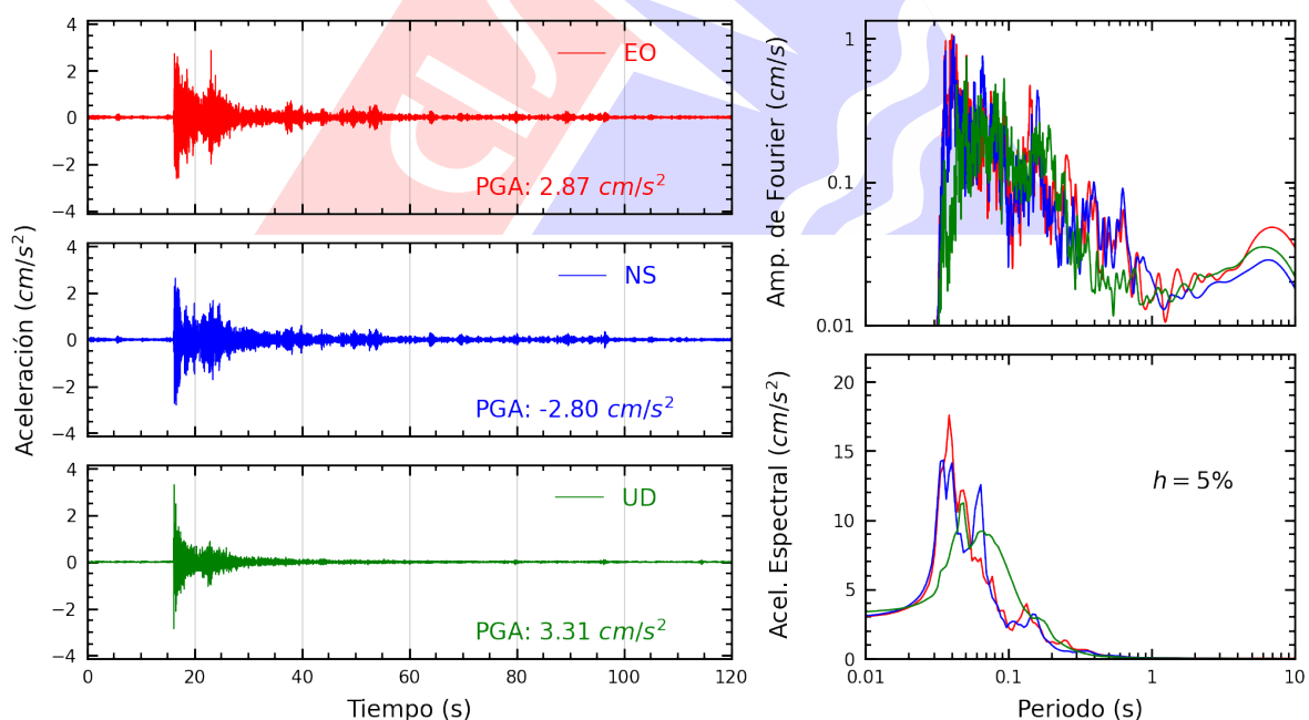
Figura A.24: Registros tiempo-historia, espectros de Fourier y de respuesta en las direcciones EO, NS y vertical de la estación DHNPE. Sismo de Provincia Constitucional del Callao , Callao - Lima del 2025-06-15, 12:03:46 (Hora local)
