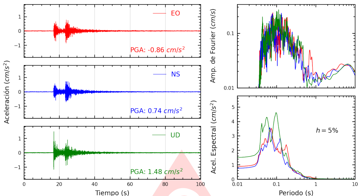
Figura A.41: Registros tiempo-historia, espectros de Fourier y de respuesta en las direcciones EO, NS y vertical de la estación BONDY. Sismo de Provincia Constitucional del Callao , Callao - Lima del 2025-06-15, 12:03:46 (Hora local)
