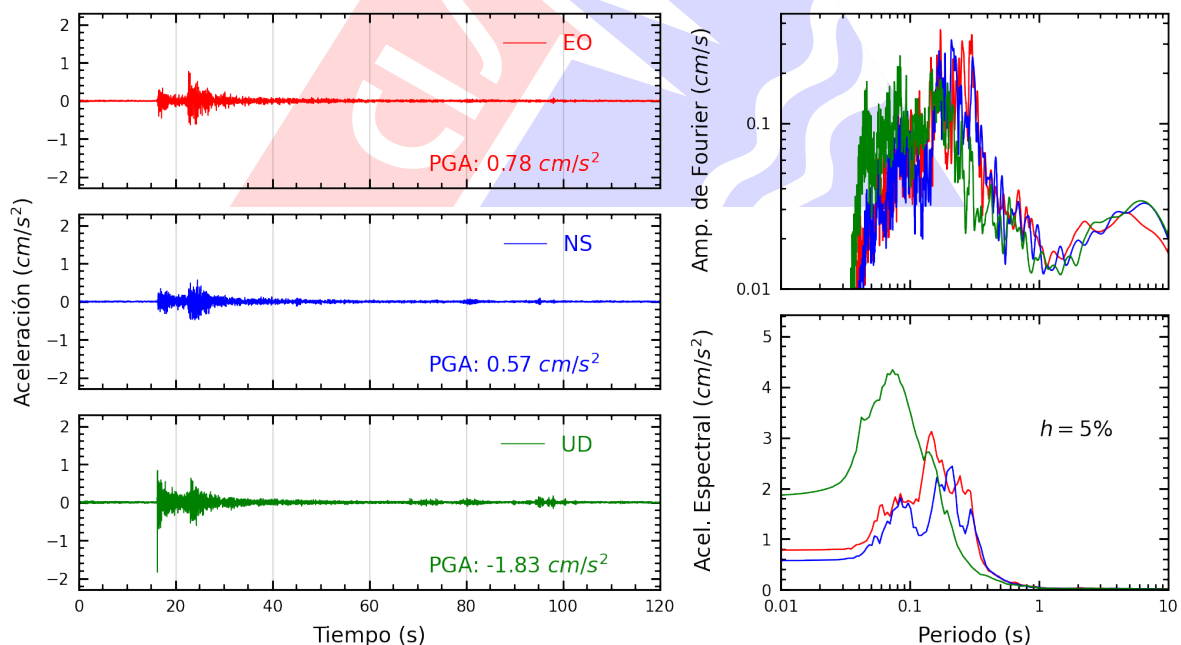
Figura A.40: Registros tiempo-historia, espectros de Fourier y de respuesta en las direcciones EO, NS y vertical de la estación DSMI. Sismo de Provincia Constitucional del Callao , Callao - Lima del 2025-06-15, 12:03:46 (Hora local)
