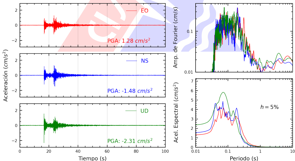
Figura A.36: Registros tiempo-historia, espectros de Fourier y de respuesta en las direcciones EO, NS y vertical de la estación UNFV. Sismo de Provincia Constitucional del Callao , Callao - Lima del 2025-06-15, 12:03:46 (Hora local)
