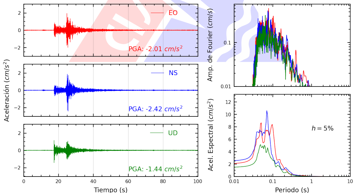
Figura A.34: Registros tiempo-historia, espectros de Fourier y de respuesta en las direcciones EO, NS y vertical de la estación BORJA. Sismo de Provincia Constitucional del Callao , Callao - Lima del 2025-06-15, 12:03:46 (Hora local)
