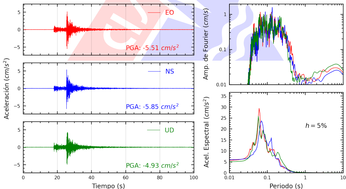
Figura A.12: Registros tiempo-historia, espectros de Fourier y de respuesta en las direcciones EO, NS y vertical de la estación SOVES. Sismo de Provincia Constitucional del Callao , Callao - Lima del 2025-06-15, 12:03:46 (Hora local)
