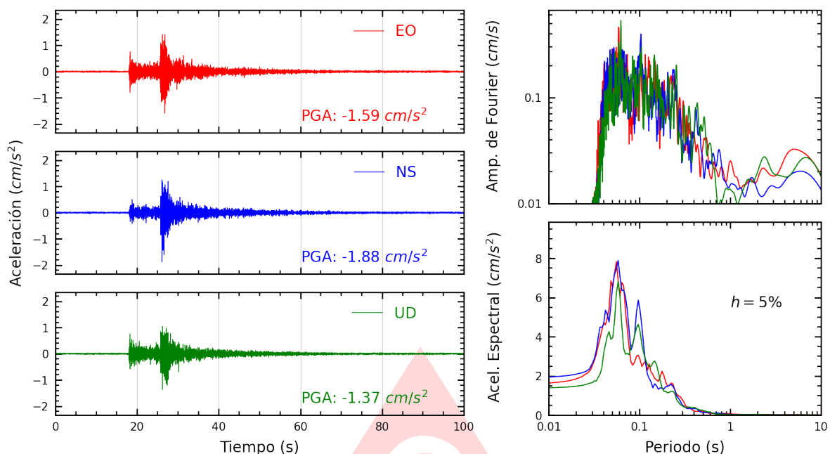
Figura A.39: Registros tiempo-historia, espectros de Fourier y de respuesta en las direcciones EO, NS y vertical de la estación IMCA. Sismo de Provincia Constitucional del Callao , Callao - Lima del 2025-06-15, 12:03:46 (Hora local)
