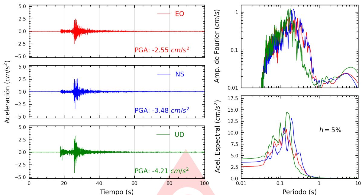
Figura A.19: Registros tiempo-historia, espectros de Fourier y de respuesta en las direcciones EO, NS y vertical de la estación MDPP. Sismo de Provincia Constitucional del Callao , Callao - Lima del 2025-06-15, 12:03:46 (Hora local)
