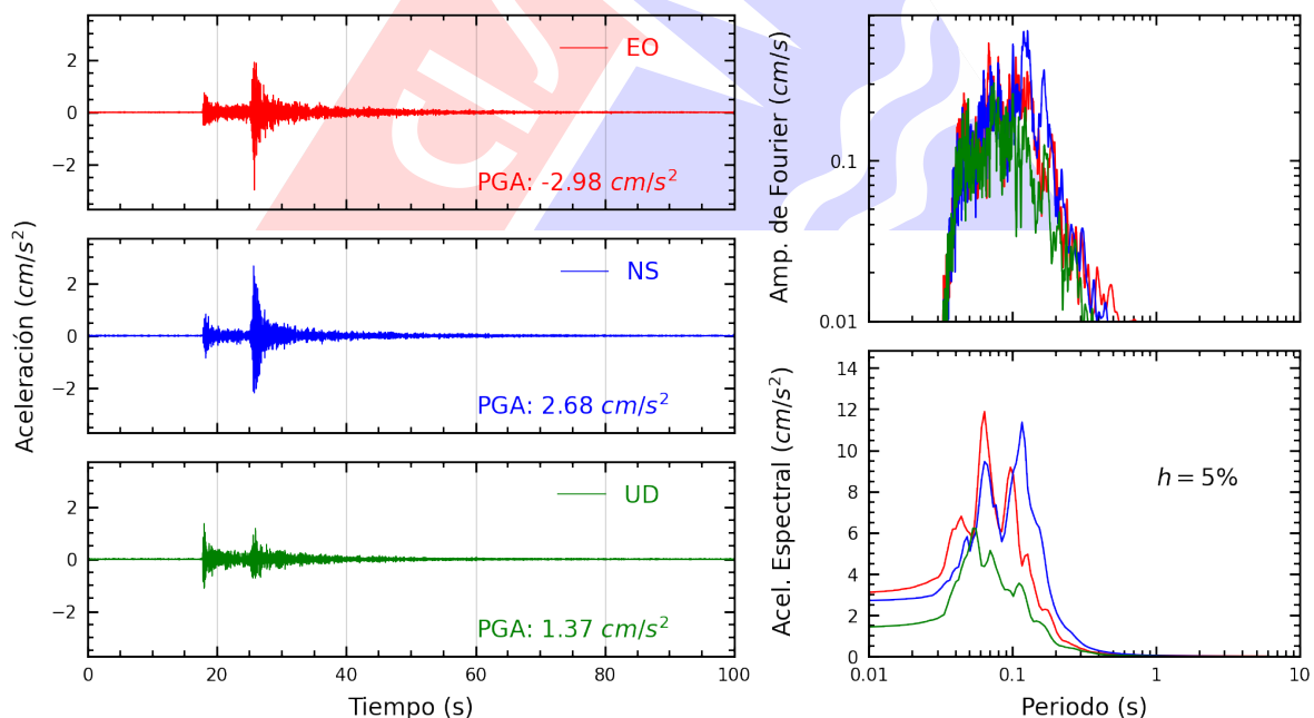
Figura A.30: Registros tiempo-historia, espectros de Fourier y de respuesta en las direcciones EO, NS y vertical de la estación ATARJ. Sismo de Provincia Constitucional del Callao , Callao - Lima del 2025-06-15, 12:03:46 (Hora local)
