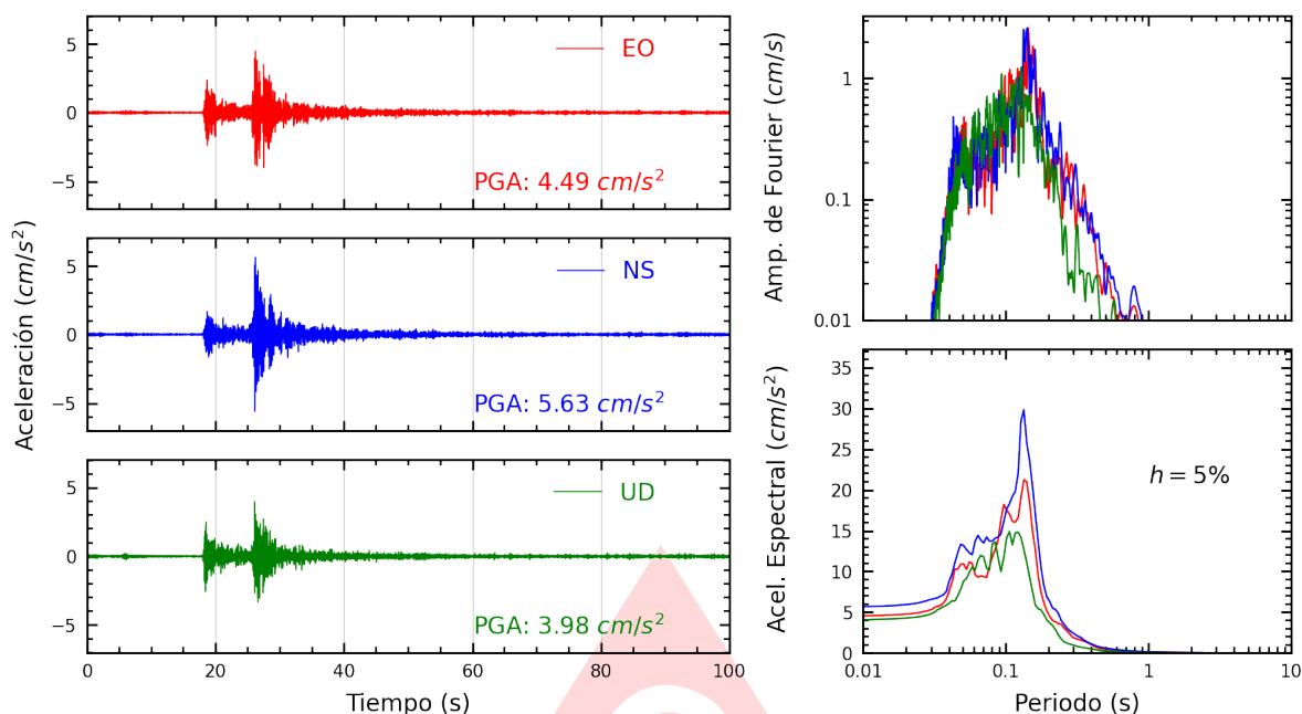
Figura A.13: Registros tiempo-historia, espectros de Fourier y de respuesta en las direcciones EO, NS y vertical de la estación CARA2. Sismo de Provincia Constitucional del Callao , Callao - Lima del 2025-06-15, 12:03:46 (Hora local)
