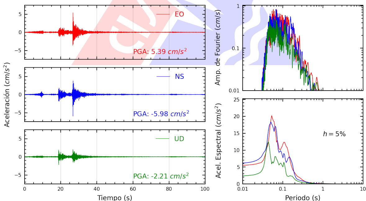
Figura A.10: Registros tiempo-historia, espectros de Fourier y de respuesta en las direcciones EO, NS y vertical de la estación PACHA. Sismo de Provincia Constitucional del Callao , Callao - Lima del 2025-06-15, 12:03:46 (Hora local)
