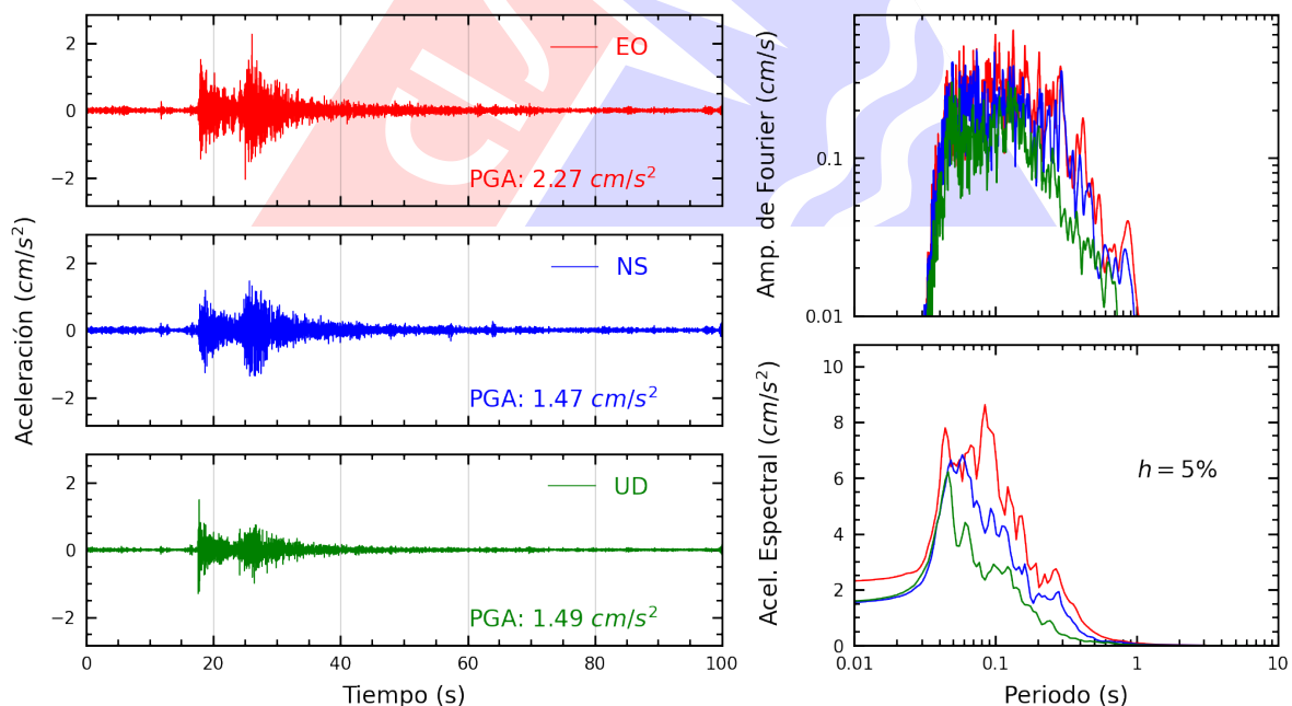
Figura A.38: Registros tiempo-historia, espectros de Fourier y de respuesta en las direcciones EO, NS y vertical de la estación BRIS2. Sismo de Provincia Constitucional del Callao , Callao - Lima del 2025-06-15, 12:03:46 (Hora local)
