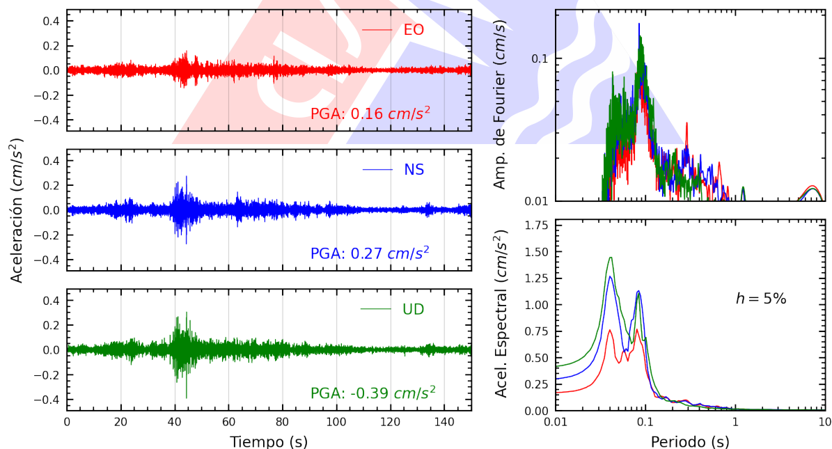
Figura A.44: Registros tiempo-historia, espectros de Fourier y de respuesta en las direcciones EO, NS y vertical de la estación UNICA. Sismo de Provincia Constitucional del Callao , Callao - Lima del 2025-06-15, 12:03:46 (Hora local)
