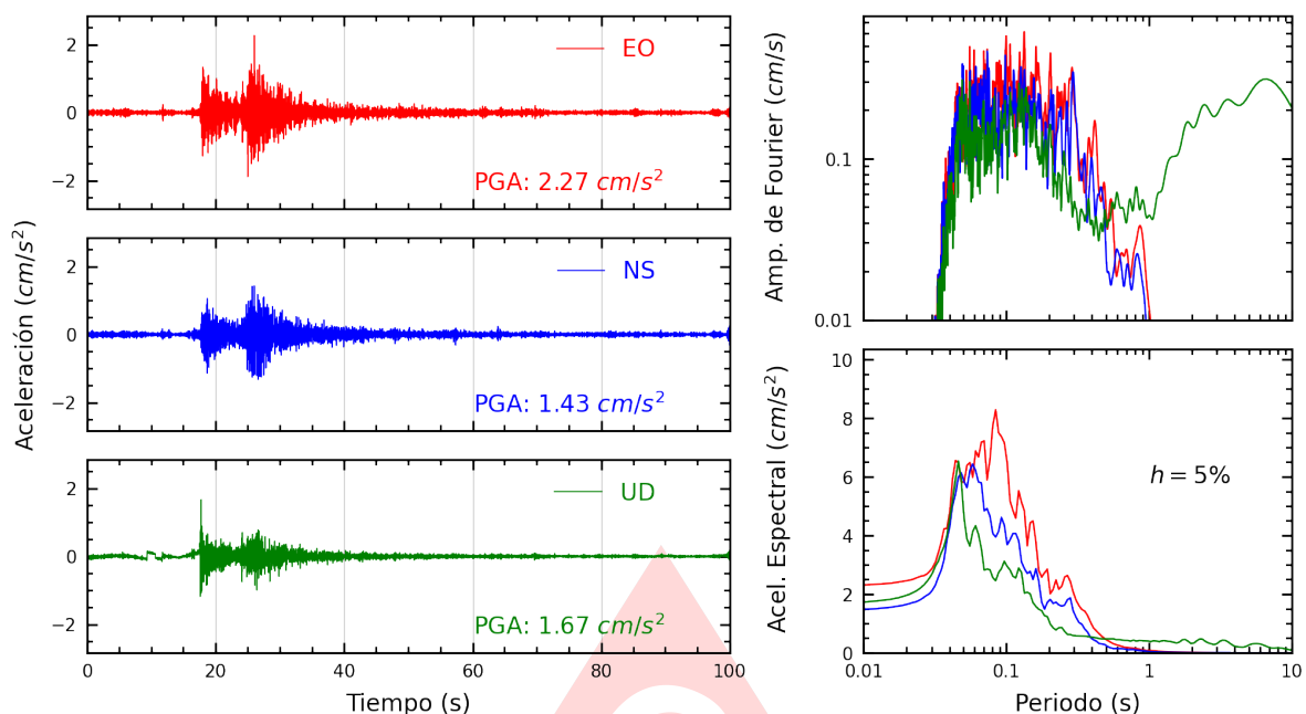
Figura A.37: Registros tiempo-historia, espectros de Fourier y de respuesta en las direcciones EO, NS y vertical de la estación BRISA. Sismo de Provincia Constitucional del Callao , Callao - Lima del 2025-06-15, 12:03:46 (Hora local)
