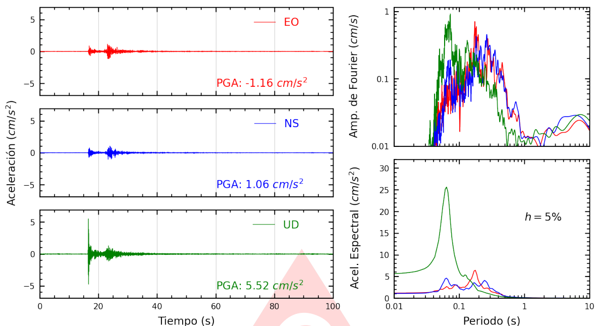
Figura A.15: Registros tiempo-historia, espectros de Fourier y de respuesta en las direcciones EO, NS y vertical de la estación ACAPU. Sismo de Provincia Constitucional del Callao , Callao - Lima del 2025-06-15, 12:03:46 (Hora local)
