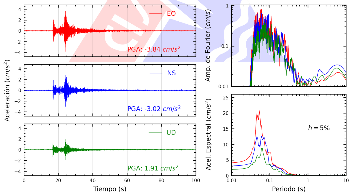
Figura A.22: Registros tiempo-historia, espectros de Fourier y de respuesta en las direcciones EO, NS y vertical de la estación CEPRE. Sismo de Provincia Constitucional del Callao , Callao - Lima del 2025-06-15, 12:03:46 (Hora local)
