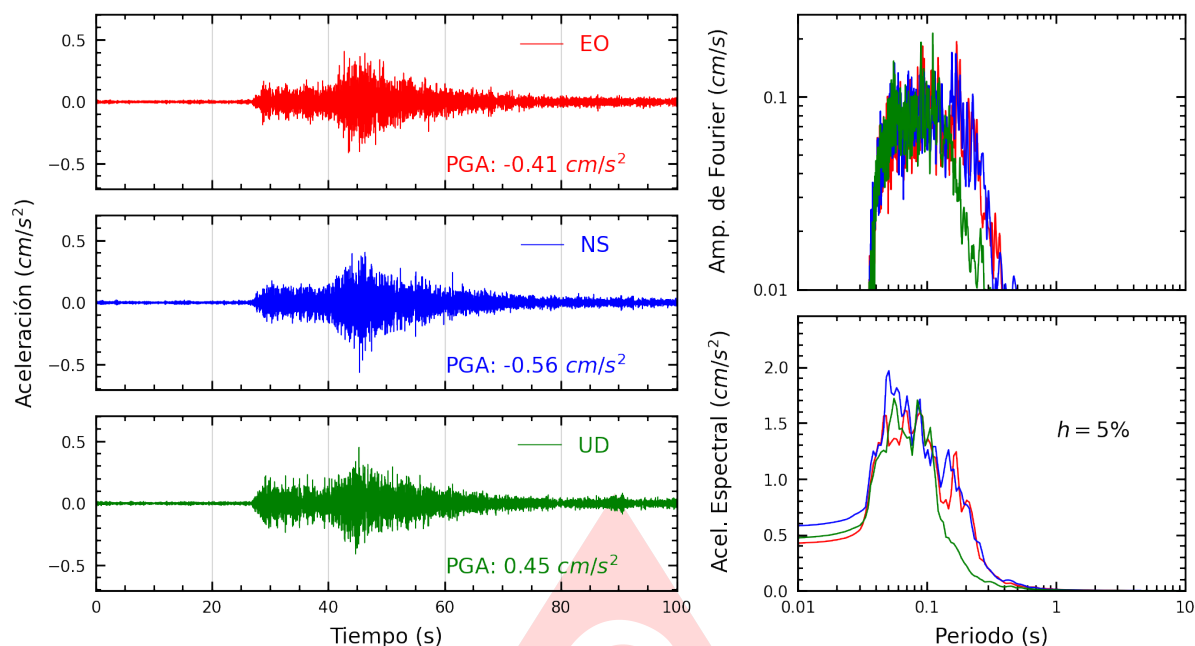
Figura A.43: Registros tiempo-historia, espectros de Fourier y de respuesta en las direcciones EO, NS y vertical de la estación ASIA. Sismo de Provincia Constitucional del Callao , Callao - Lima del 2025-06-15, 12:03:46 (Hora local)
