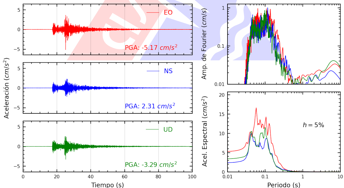
Figura A.16: Registros tiempo-historia, espectros de Fourier y de respuesta en las direcciones EO, NS y vertical de la estación AMORE. Sismo de Provincia Constitucional del Callao , Callao - Lima del 2025-06-15, 12:03:46 (Hora local)
