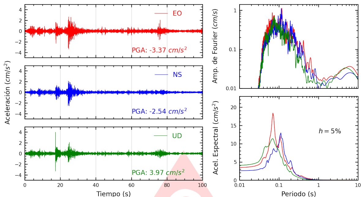
Figura A.21: Registros tiempo-historia, espectros de Fourier y de respuesta en las direcciones EO, NS y vertical de la estación SOBAR. Sismo de Provincia Constitucional del Callao , Callao - Lima del 2025-06-15, 12:03:46 (Hora local)
