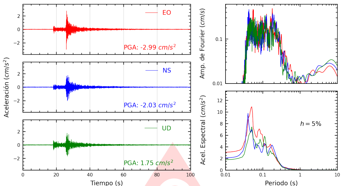
Figura A.29: Registros tiempo-historia, espectros de Fourier y de respuesta en las direcciones EO, NS y vertical de la estación USMP. Sismo de Provincia Constitucional del Callao , Callao - Lima del 2025-06-15, 12:03:46 (Hora local)
