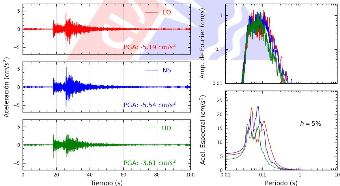
Figura A.14: Registros tiempo-historia, espectros de Fourier y de respuesta en las direcciones EO, NS y vertical de la estación SROS2. Sismo de Provincia Constitucional del Callao , Callao - Lima del 2025-06-15, 12:03:46 (Hora local)
