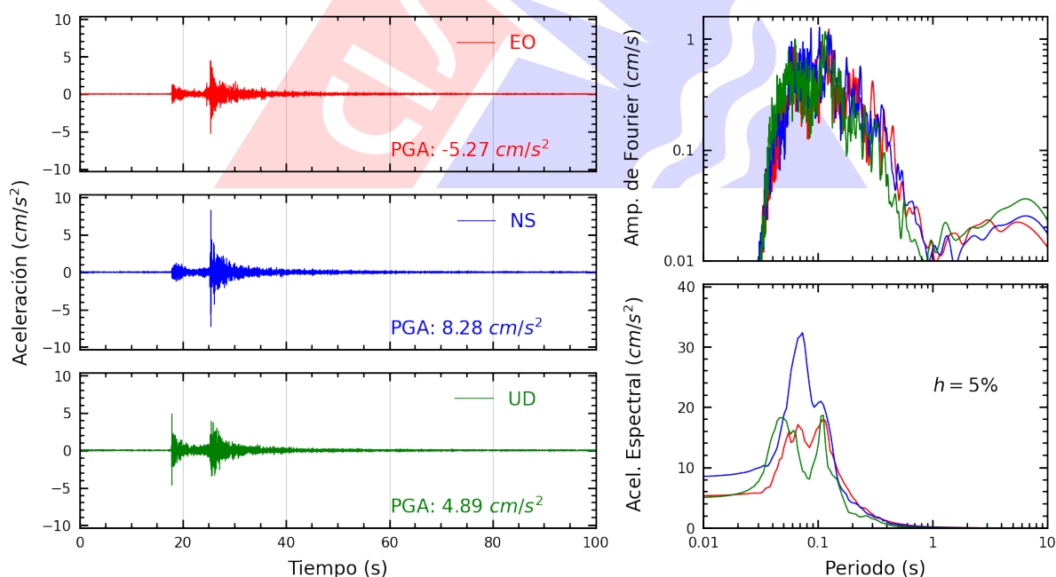
Figura A.4: Registros tiempo-historia, espectros de Fourier y de respuesta en las direcciones EO, NS y vertical de la estación SJLSC. Sismo de Provincia Constitucional del Callao , Callao - Lima del 2025-06-15, 12:03:46 (Hora local)
