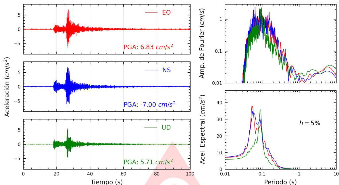
Figura A.7: Registros tiempo-historia, espectros de Fourier y de respuesta en las direcciones EO, NS y vertical de la estación USILM. Sismo de Provincia Constitucional del Callao , Callao - Lima del 2025-06-15, 12:03:46 (Hora local)
