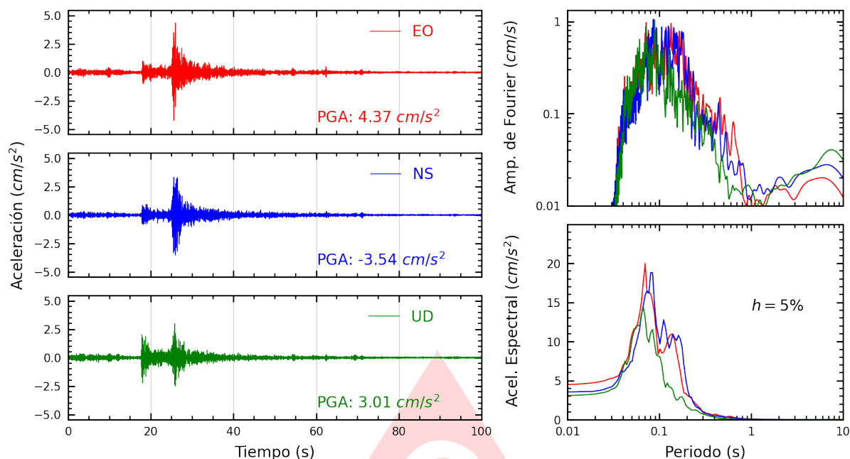
Figura A.17: Registros tiempo-historia, espectros de Fourier y de respuesta en las direcciones EO, NS y vertical de la estación SJLSV. Sismo de Provincia Constitucional del Callao , Callao - Lima del 2025-06-15, 12:03:46 (Hora local)
