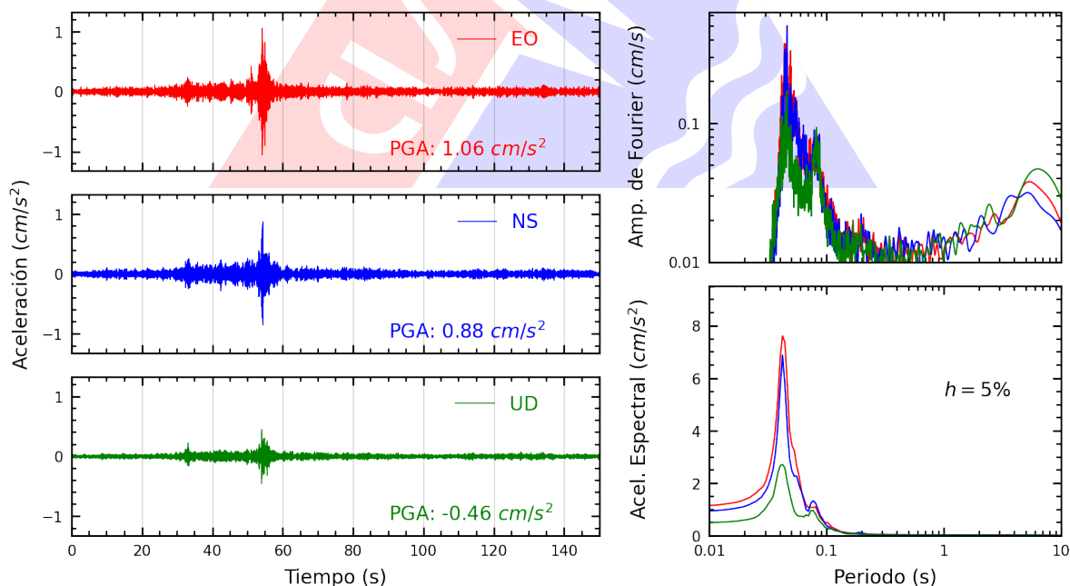
Figura A.42: Registros tiempo-historia, espectros de Fourier y de respuesta en las direcciones EO, NS y vertical de la estación USP. Sismo de Provincia Constitucional del Callao , Callao - Lima del 2025-06-15, 12:03:46 (Hora local)
