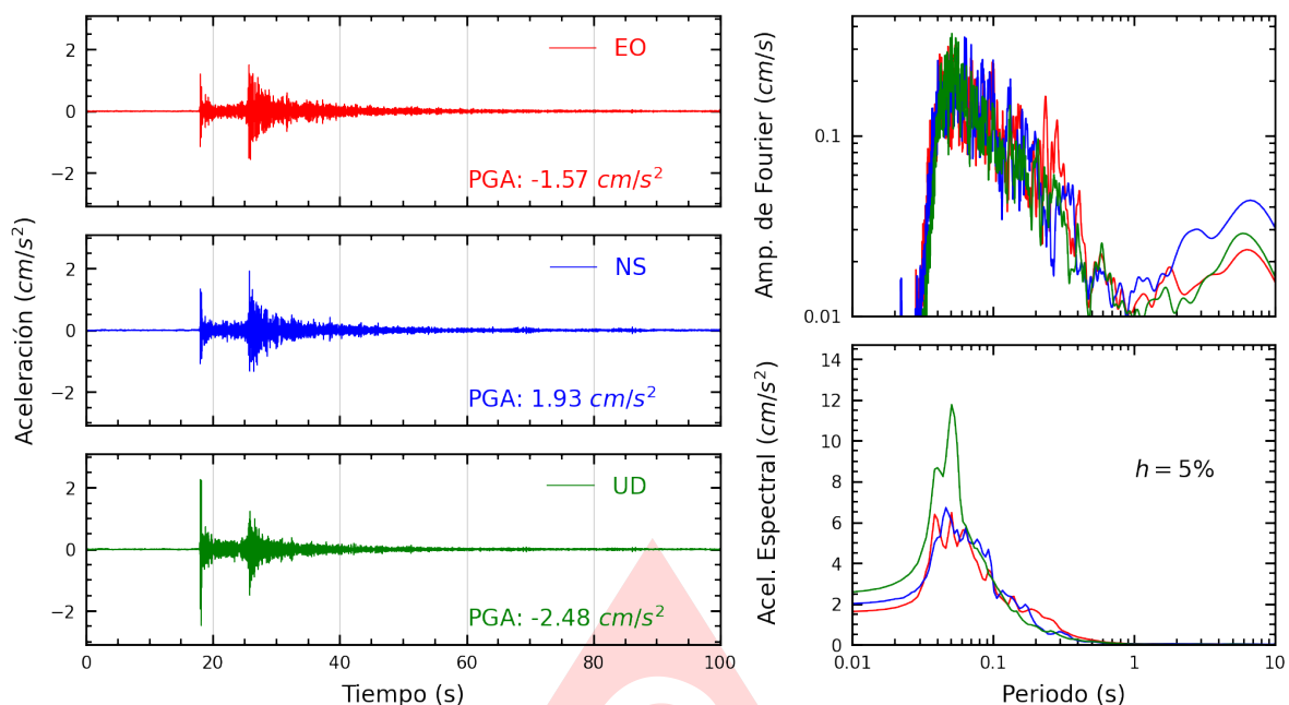
Figura A.33: Registros tiempo-historia, espectros de Fourier y de respuesta en las direcciones EO, NS y vertical de la estación SJLCE. Sismo de Provincia Constitucional del Callao , Callao - Lima del 2025-06-15, 12:03:46 (Hora local)
