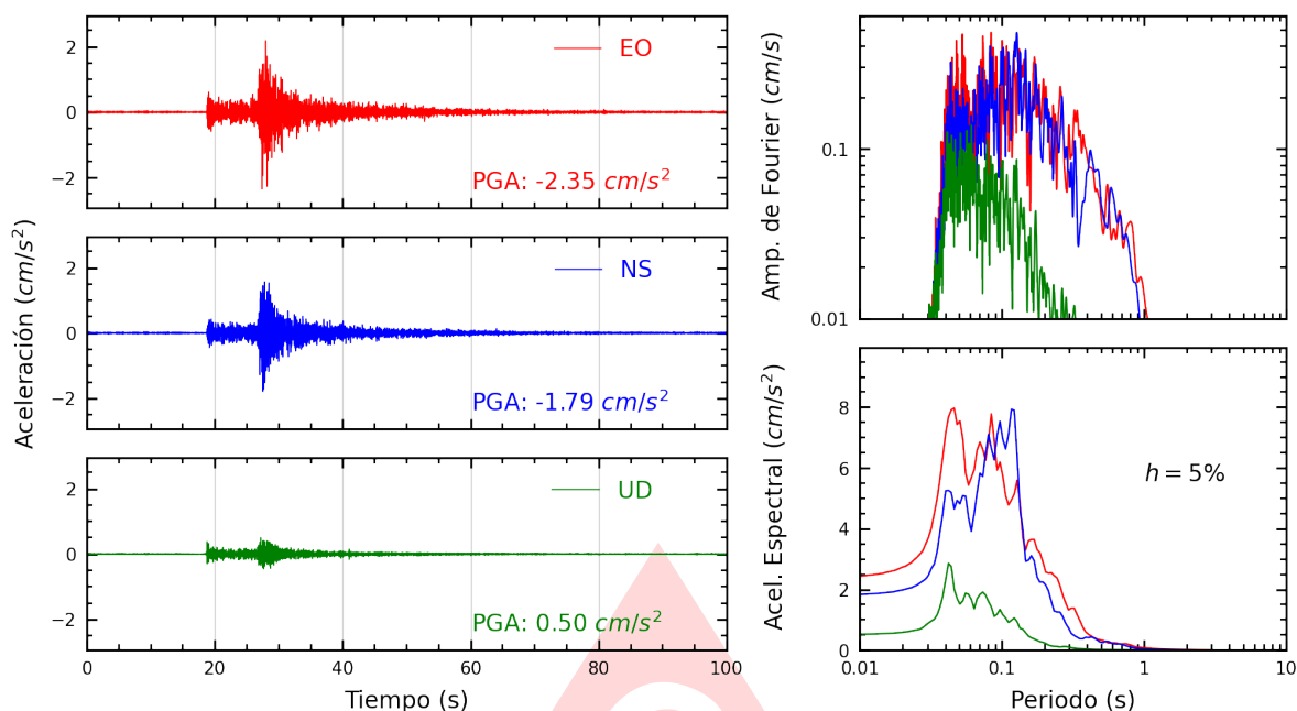
Figura A.35: Registros tiempo-historia, espectros de Fourier y de respuesta en las direcciones EO, NS y vertical de la estación UCVA2. Sismo de Provincia Constitucional del Callao , Callao - Lima del 2025-06-15, 12:03:46 (Hora local)
