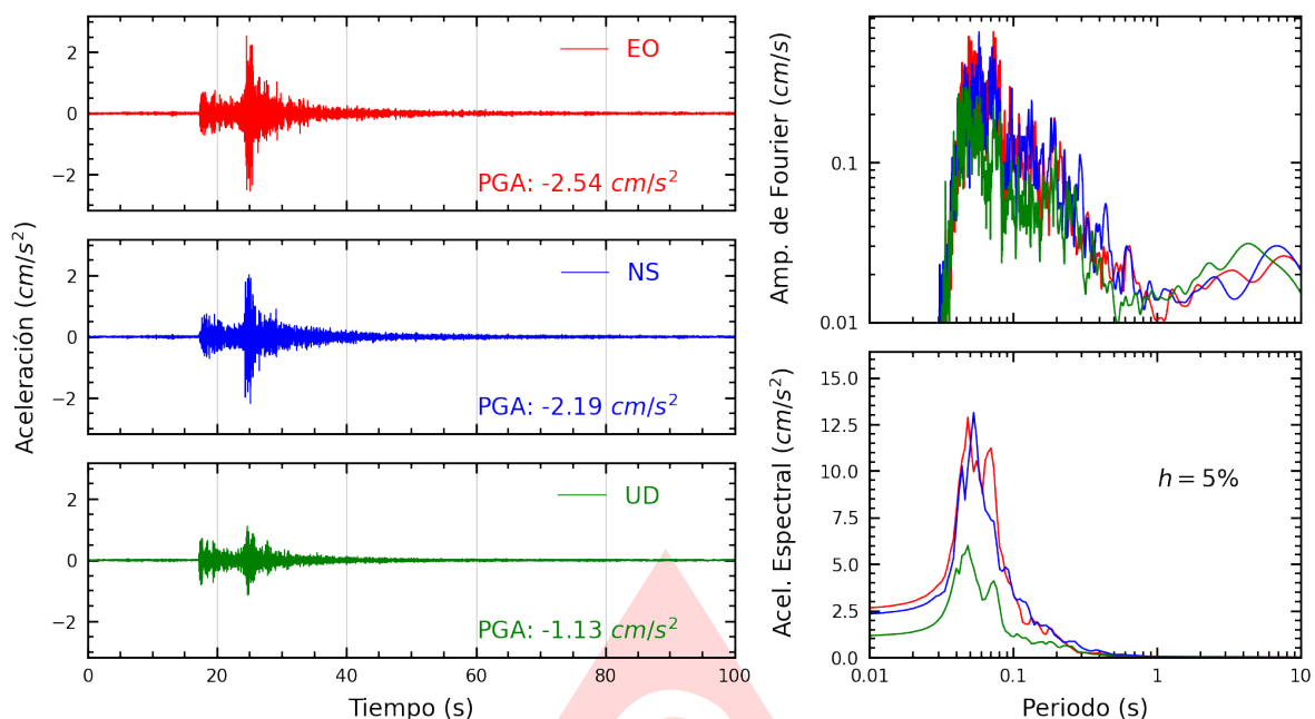
Figura A.31: Registros tiempo-historia, espectros de Fourier y de respuesta en las direcciones EO, NS y vertical de la estación UPCVI. Sismo de Provincia Constitucional del Callao, Callao - Lima del 2025-06-15, 12:03:46 (Hora local)
