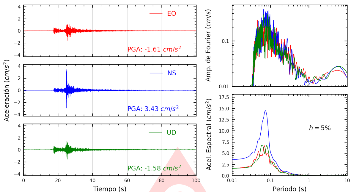
Figura A.23: Registros tiempo-historia, espectros de Fourier y de respuesta en las direcciones EO, NS y vertical de la estación SERVI. Sismo de Provincia Constitucional del Callao , Callao - Lima del 2025-06-15, 12:03:46 (Hora local)
