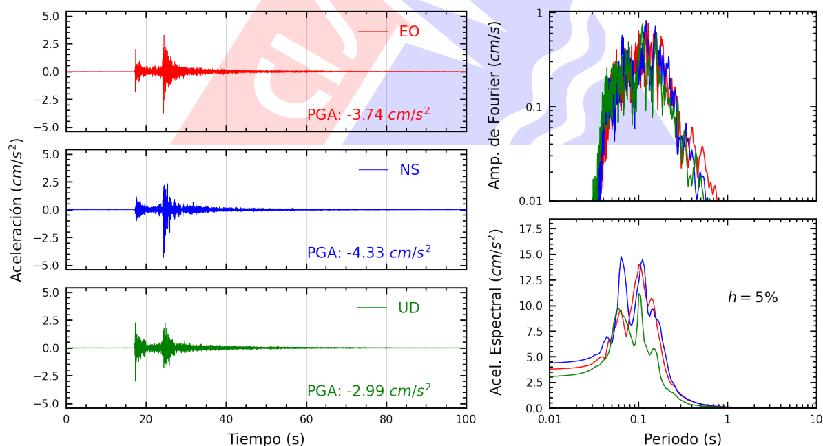
Figura A.18: Registros tiempo-historia, espectros de Fourier y de respuesta en las direcciones EO, NS y vertical de la estación JALV2. Sismo de Provincia Constitucional del Callao , Callao - Lima del 2025-06-15, 12:03:46 (Hora local)
