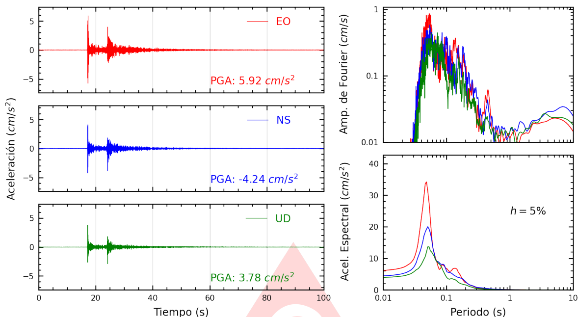
Figura A.11: Registros tiempo-historia, espectros de Fourier y de respuesta en las direcciones EO, NS y vertical de la estación UCSS. Sismo de Provincia Constitucional del Callao , Callao - Lima del 2025-06-15, 12:03:46 (Hora local)
