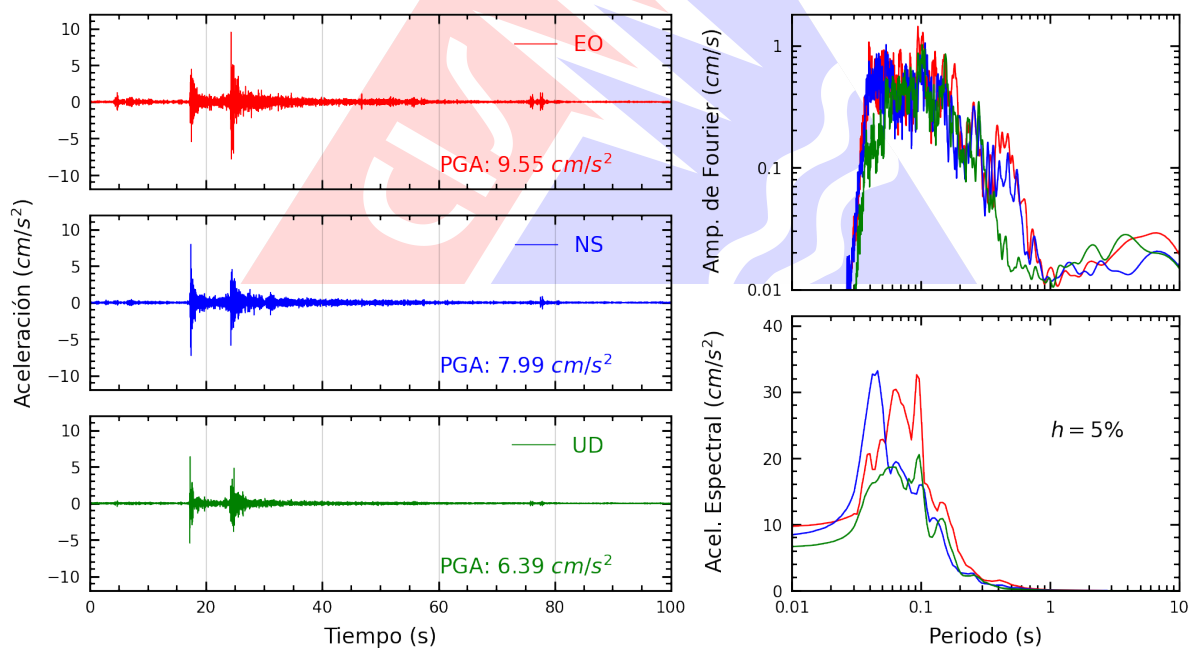
Figura A.2: Registros tiempo-historia, espectros de Fourier y de respuesta en las direcciones EO, NS y vertical de la estación OLIVO. Sismo de Provincia Constitucional del Callao , Callao - Lima del 2025-06-15, 12:03:46 (Hora local)
