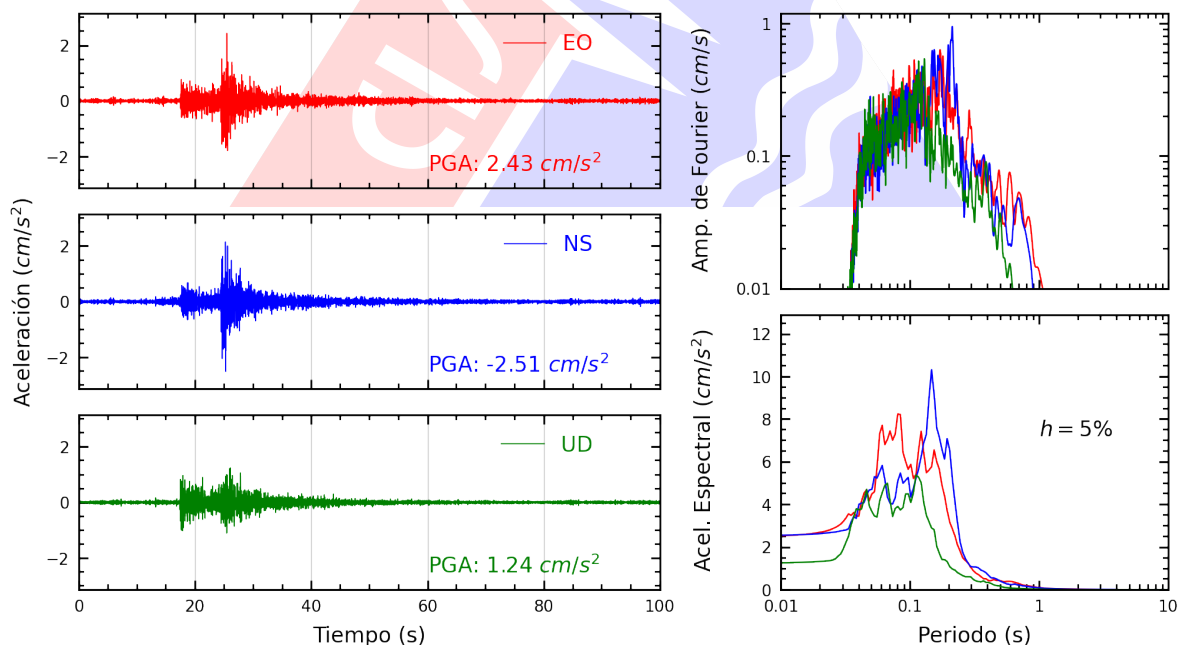
Figura A.32: Registros tiempo-historia, espectros de Fourier y de respuesta en las direcciones EO, NS y vertical de la estación SCCHO. Sismo de Provincia Constitucional del Callao, Callao - Lima del 2025-06-15, 12:03:46 (Hora local)
