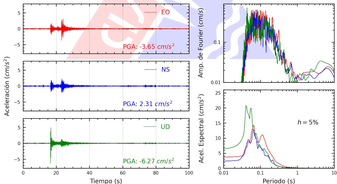
Figura A.8: Registros tiempo-historia, espectros de Fourier y de respuesta en las direcciones EO, NS y vertical de la estación UPCSM. Sismo de Provincia Constitucional del Callao , Callao - Lima del 2025-06-15, 12:03:46 (Hora local)
