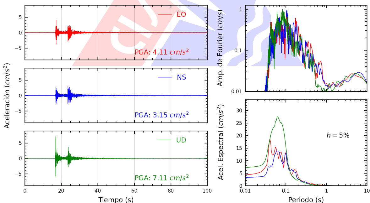
Figura A.6: Registros tiempo-historia, espectros de Fourier y de respuesta en las direcciones EO, NS y vertical de la estación MADRE. Sismo de Provincia Constitucional del Callao , Callao - Lima del 2025-06-15, 12:03:46 (Hora local)
