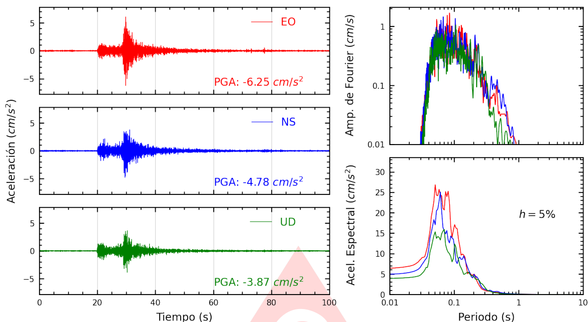
Figura A.9: Registros tiempo-historia, espectros de Fourier y de respuesta en las direcciones EO, NS y vertical de la estación PHER2. Sismo de Provincia Constitucional del Callao , Callao - Lima del 2025-06-15, 12:03:46 (Hora local)
