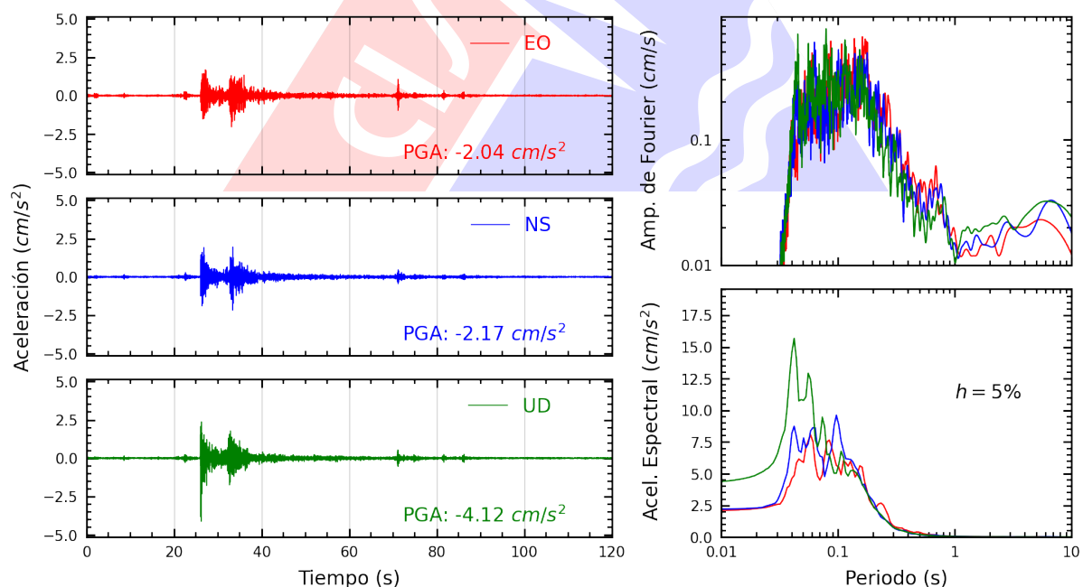
Figura A.20: Registros tiempo-historia, espectros de Fourier y de respuesta en las direcciones EO, NS y vertical de la estación PRADO. Sismo de Provincia Constitucional del Callao , Callao - Lima del 2025-06-15, 12:03:46 (Hora local)
