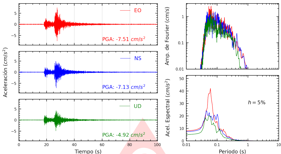
Figura A.5: Registros tiempo-historia, espectros de Fourier y de respuesta en las direcciones EO, NS y vertical de la estación UNTEL. Sismo de Provincia Constitucional del Callao , Callao - Lima del 2025-06-15, 12:03:46 (Hora local)
