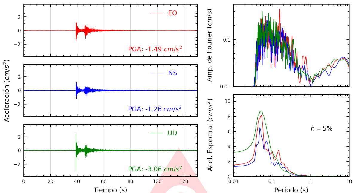
Figura A.27: Registros tiempo-historia, espectros de Fourier y de respuesta en las direcciones EO, NS y vertical de la estación UNMSM. Sismo de Provincia Constitucional del Callao , Callao - Lima del 2025-06-15, 12:03:46 (Hora local)
