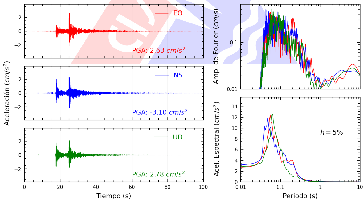
Figura A.26: Registros tiempo-historia, espectros de Fourier y de respuesta en las direcciones EO, NS y vertical de la estación COMAS. Sismo de Provincia Constitucional del Callao, Callao - Lima del 2025-06-15, 12:03:46 (Hora local)
