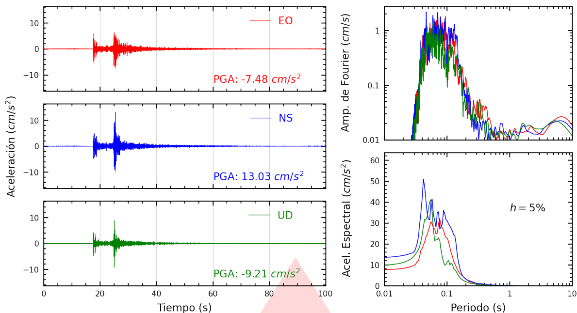
Figura A.1: Registros tiempo-historia, espectros de Fourier y de respuesta en las direcciones EO, NS y vertical de la estación JOSEO. Sismo de Provincia Constitucional del Callao , Callao - Lima del 2025-06-15, 12:03:46 (Hora local)
