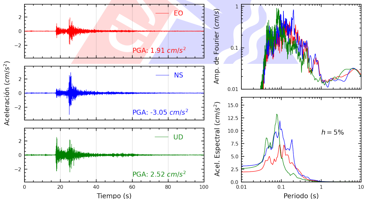
Figura A.28: Registros tiempo-historia, espectros de Fourier y de respuesta en las direcciones EO, NS y vertical de la estación SOCHO. Sismo de Provincia Constitucional del Callao , Callao - Lima del 2025-06-15, 12:03:46 (Hora local)
