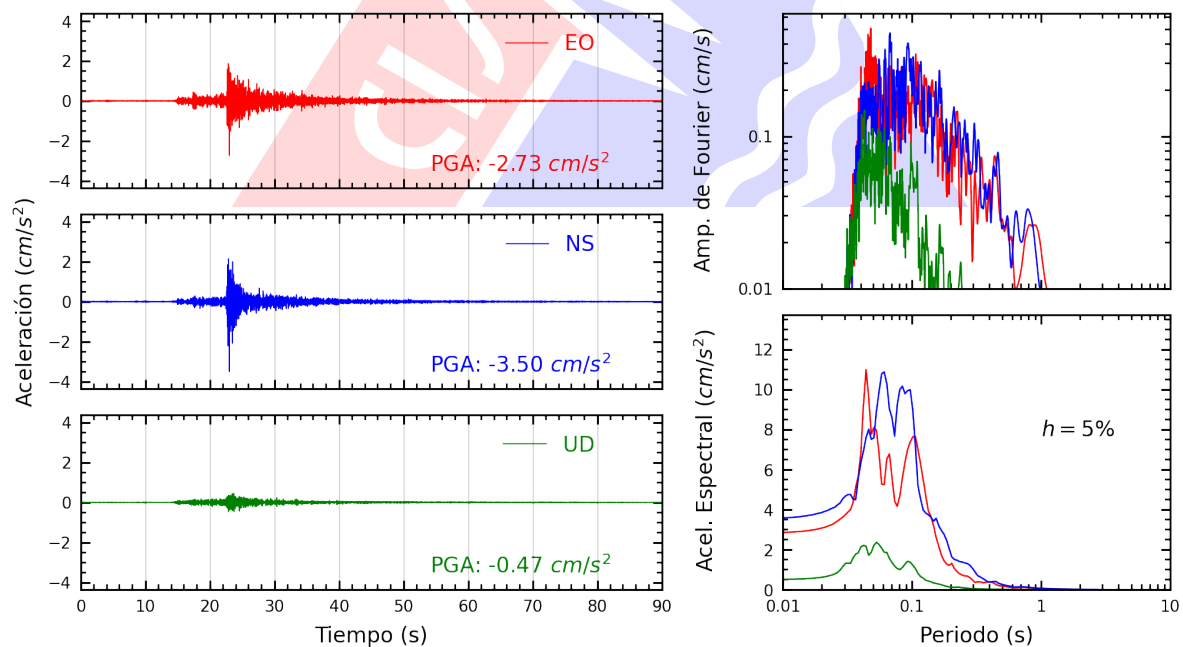
Figura A.16: Registros tiempo-historia, espectros de Fourier y de respuesta en las direcciones EO, NS y vertical de la estación UCVA2. Sismo de Ancon, Lima - Lima del 2025-06-17, 00:31:31 (Hora local)
