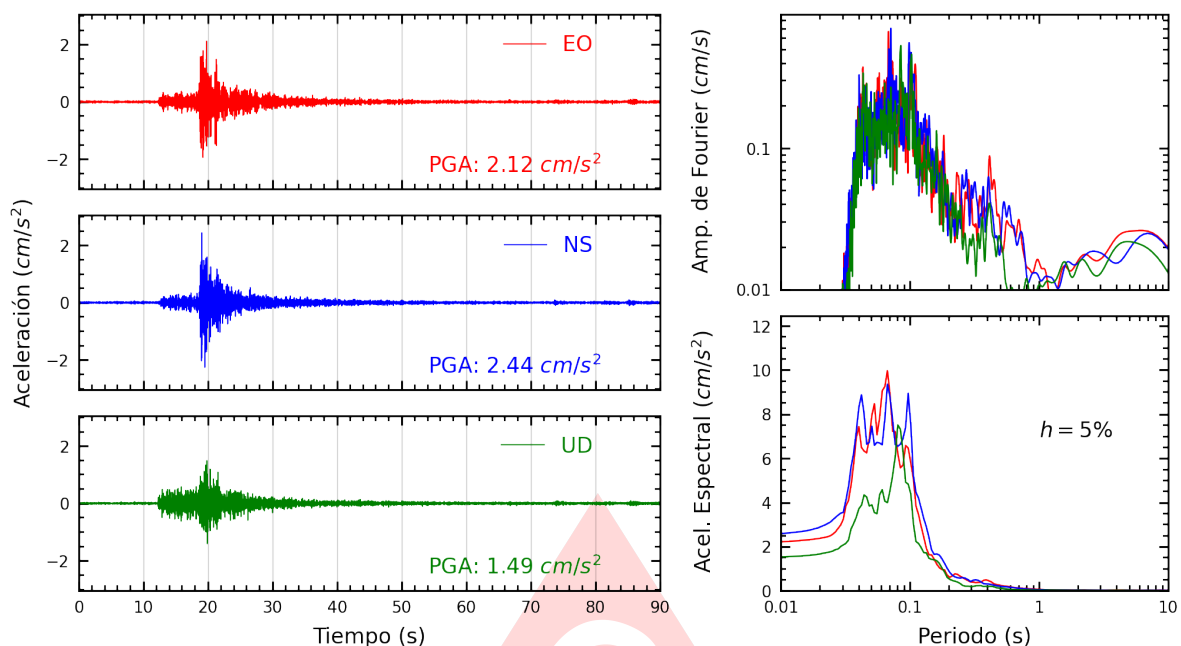
Figura A.25: Registros tiempo-historia, espectros de Fourier y de respuesta en las direcciones EO, NS y vertical de la estación MADRE. Sismo de Ancon, Lima - Lima del 2025-06-17, 00:31:31 (Hora local)
