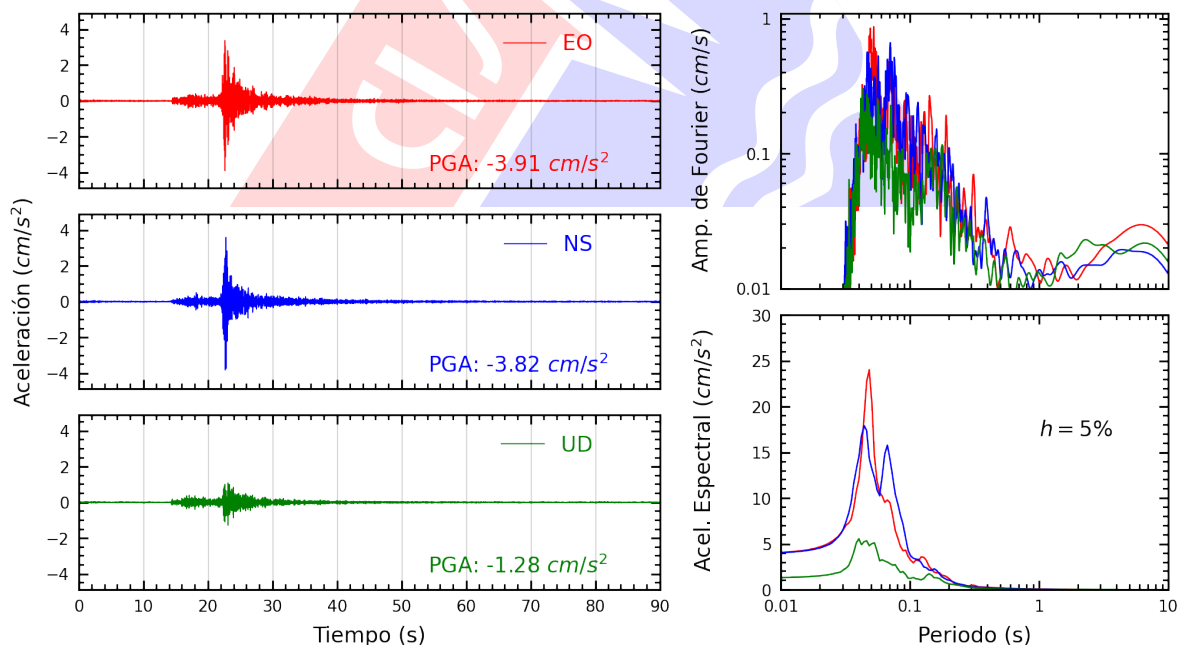
Figura A.12: Registros tiempo-historia, espectros de Fourier y de respuesta en las direcciones EO, NS y vertical de la estación UPCVI. Sismo de Ancon, Lima - Lima del 2025-06-17, 00:31:31 (Hora local)
