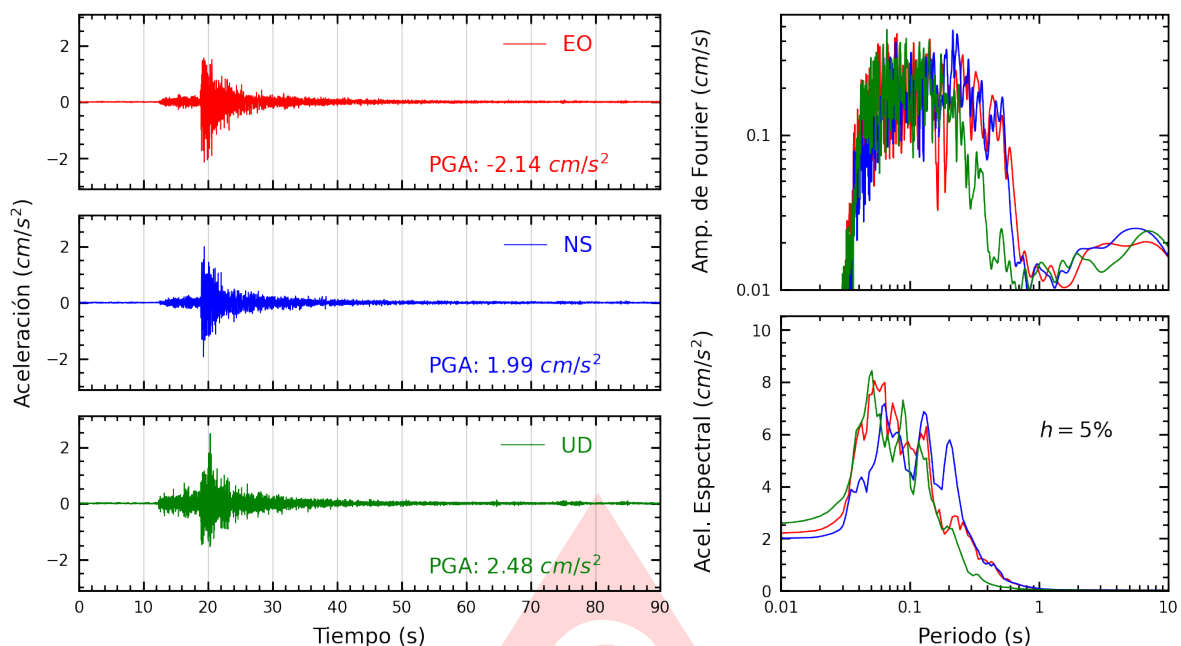
Figura A.23: Registros tiempo-historia, espectros de Fourier y de respuesta en las direcciones EO, NS y vertical de la estación MDP. Sismo de Ancon, Lima - Lima del 2025-06-17, 00:31:31 (Hora local)
