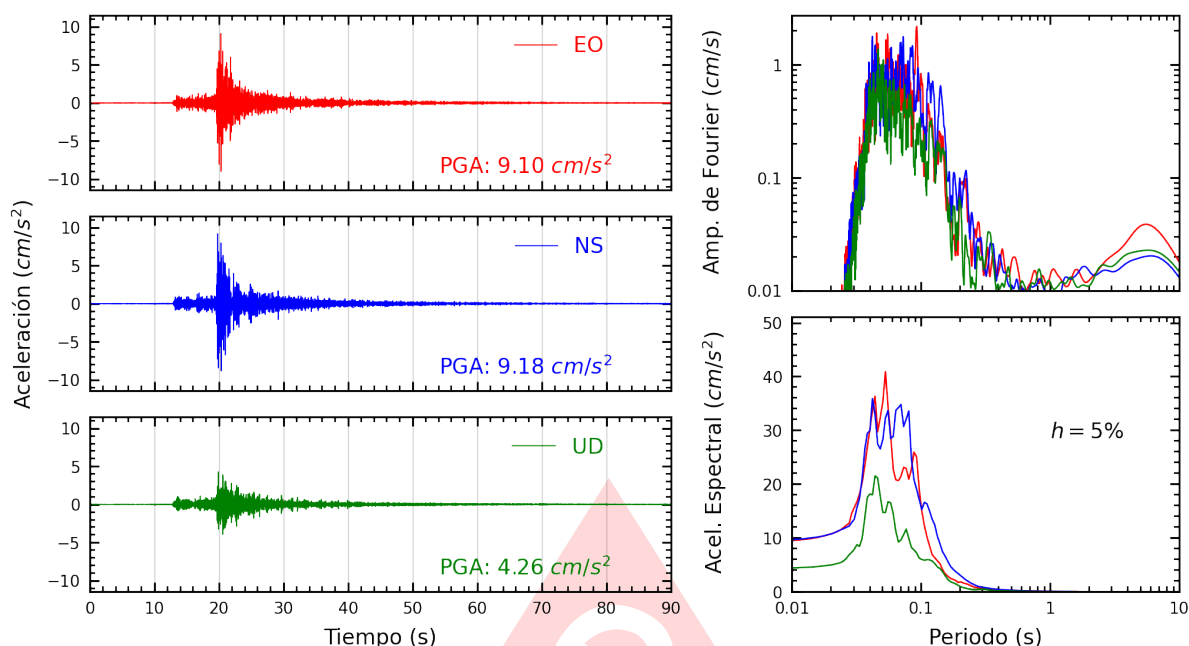
Figura A.3: Registros tiempo-historia, espectros de Fourier y de respuesta en las direcciones EO, NS y vertical de la estación JOSEO. Sismo de Ancon, Lima - Lima del 2025-06-17, 00:31:31 (Hora local)
