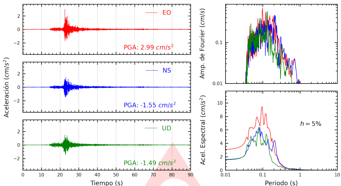
Figura A.19: Registros tiempo-historia, espectros de Fourier y de respuesta en las direcciones EO, NS y vertical de la estación SCCHO. Sismo de Ancon, Lima - Lima del 2025-06-17, 00:31:31 (Hora local)
