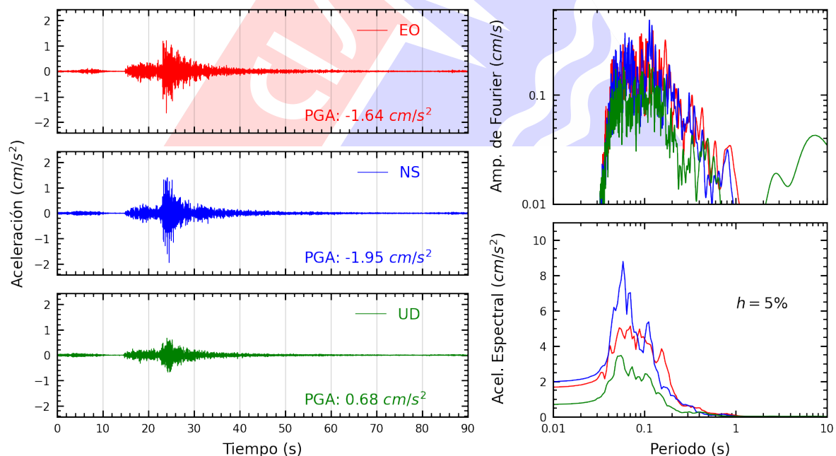
Figura A.32: Registros tiempo-historia, espectros de Fourier y de respuesta en las direcciones EO, NS y vertical de la estación BRISA. Sismo de Ancon, Lima - Lima del 2025-06-17, 00:31:31 (Hora local)
