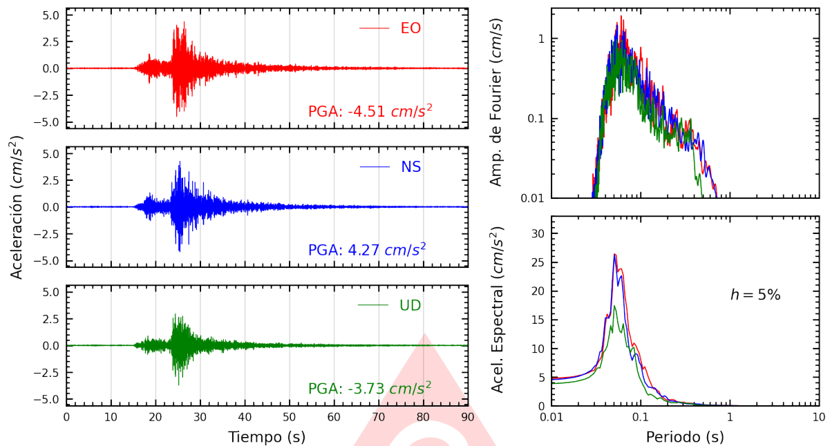
Figura A.9: Registros tiempo-historia, espectros de Fourier y de respuesta en las direcciones EO, NS y vertical de la estación UNTEL. Sismo de Ancon, Lima - Lima del 2025-06-17, 00:31:31 (Hora local)
