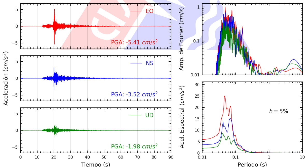
Figura A.6: Registros tiempo-historia, espectros de Fourier y de respuesta en las direcciones EO, NS y vertical de la estación FICPE. Sismo de Ancon, Lima - Lima del 2025-06-17, 00:31:31 (Hora local)
