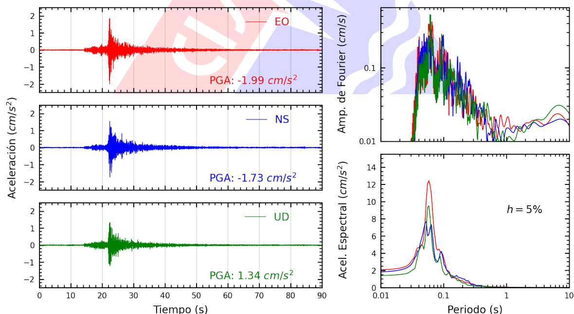
Figura A.30: Registros tiempo-historia, espectros de Fourier y de respuesta en las direcciones EO, NS y vertical de la estación IMCA. Sismo de Ancon, Lima - Lima del 2025-06-17, 00:31:31 (Hora local)
