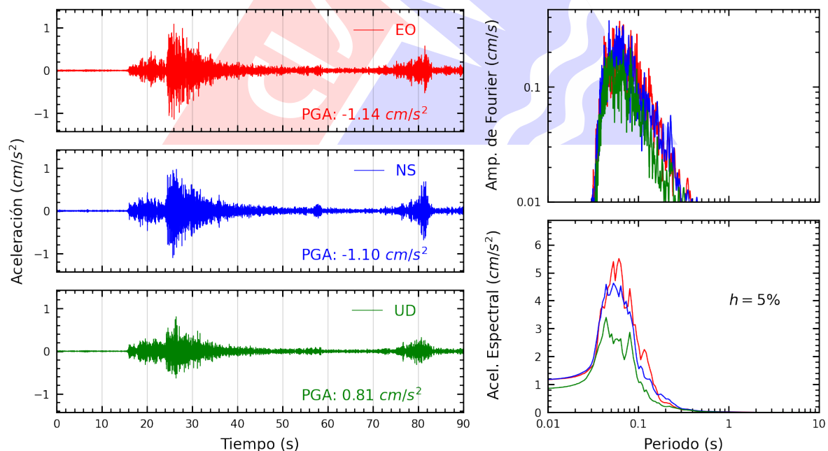
Figura A.40: Registros tiempo-historia, espectros de Fourier y de respuesta en las direcciones EO, NS y vertical de la estación PACHA. Sismo de Ancon, Lima - Lima del 2025-06-17, 00:31:31 (Hora local)
