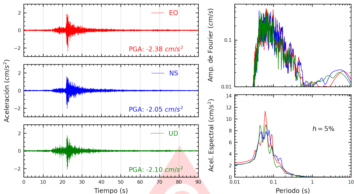
Figura A.27: Registros tiempo-historia, espectros de Fourier y de respuesta en las direcciones EO, NS y vertical de la estación URPPE. Sismo de Ancon, Lima - Lima del 2025-06-17, 00:31:31 (Hora local)
