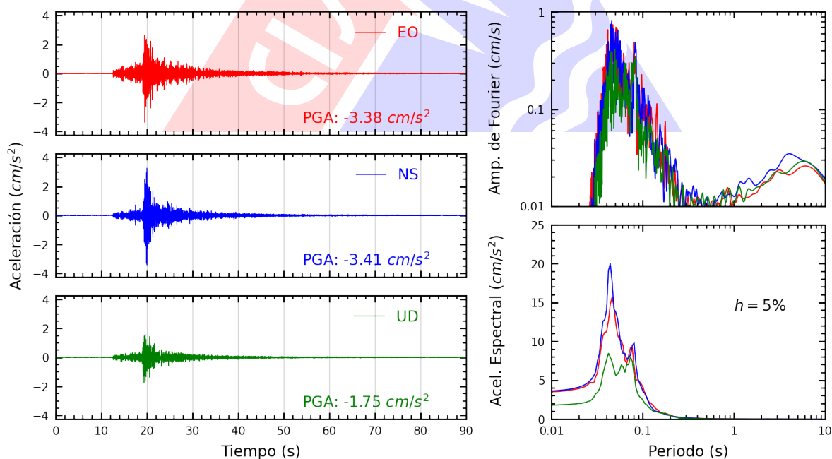
Figura A.18: Registros tiempo-historia, espectros de Fourier y de respuesta en las direcciones EO, NS y vertical de la estación UCSS. Sismo de Ancon, Lima - Lima del 2025-06-17, 00:31:31 (Hora local)
