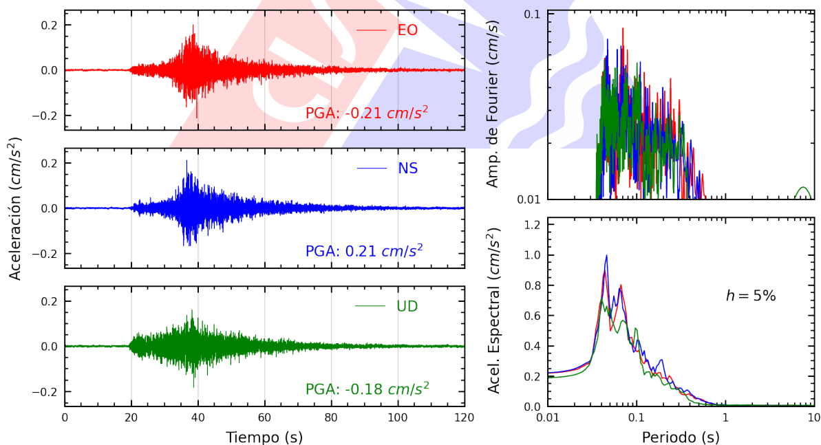
Figura A.44: Registros tiempo-historia, espectros de Fourier y de respuesta en las direcciones EO, NS y vertical de la estación CARAL. Sismo de Ancon, Lima - Lima del 2025-06-17, 00:31:31 (Hora local)
