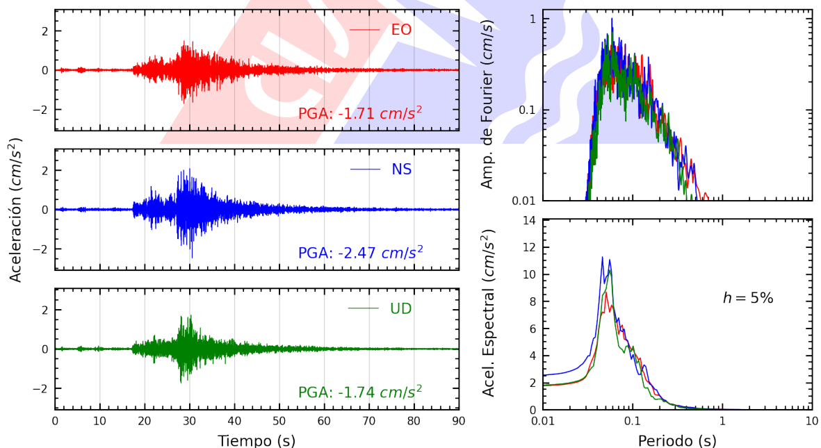
Figura A.24: Registros tiempo-historia, espectros de Fourier y de respuesta en las direcciones EO, NS y vertical de la estación PHER2. Sismo de Ancon, Lima - Lima del 2025-06-17, 00:31:31 (Hora local)
