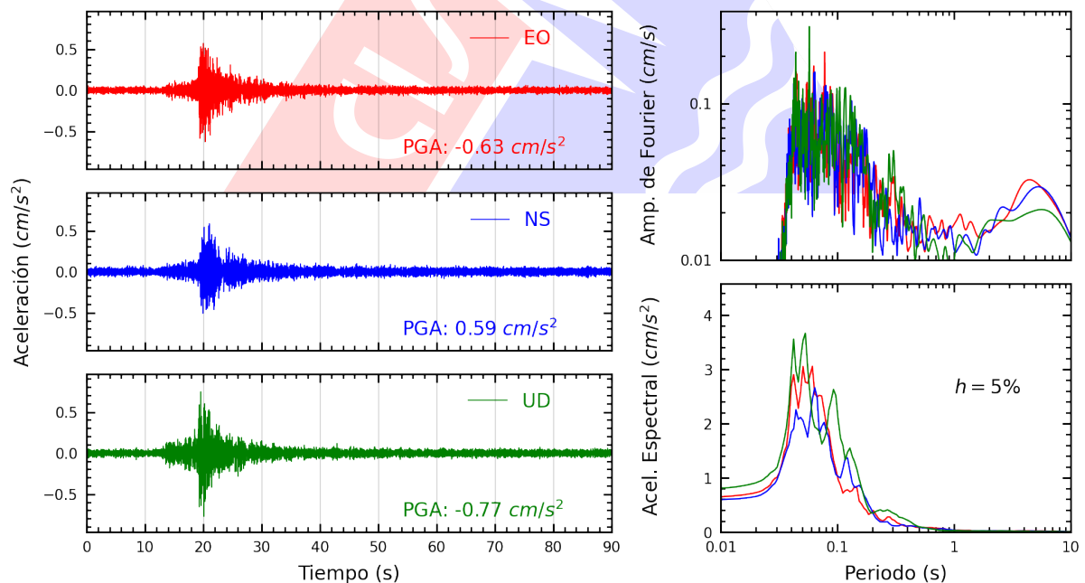
Figura A.42: Registros tiempo-historia, espectros de Fourier y de respuesta en las direcciones EO, NS y vertical de la estación BONDY. Sismo de Ancon, Lima - Lima del 2025-06-17, 00:31:31 (Hora local)
