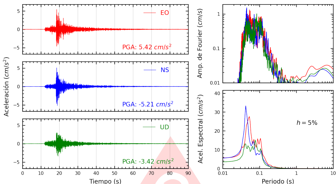
Figura A.5: Registros tiempo-historia, espectros de Fourier y de respuesta en las direcciones EO, NS y vertical de la estación AMORE. Sismo de Ancon, Lima - Lima del 2025-06-17, 00:31:31 (Hora local)
