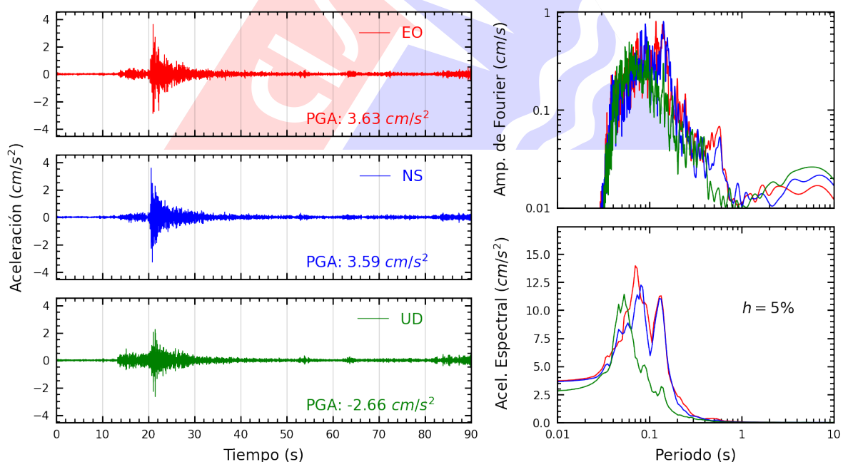
Figura A.14: Registros tiempo-historia, espectros de Fourier y de respuesta en las direcciones EO, NS y vertical de la estación SJLSV. Sismo de Ancon, Lima - Lima del 2025-06-17, 00:31:31 (Hora local)
