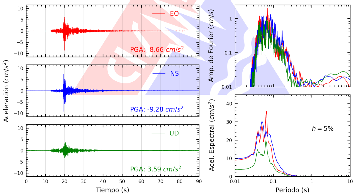
Figura A.2: Registros tiempo-historia, espectros de Fourier y de respuesta en las direcciones EO, NS y vertical de la estación INDEP. Sismo de Ancon, Lima - Lima del 2025-06-17, 00:31:31 (Hora local)
