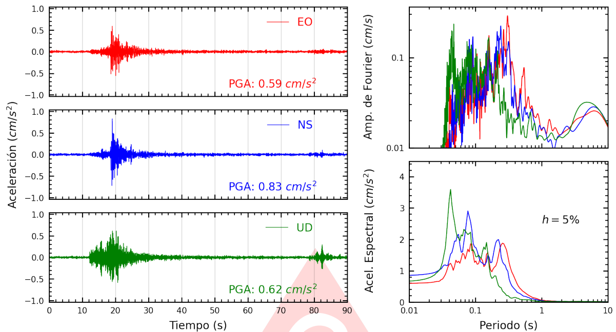
Figura A.41: Registros tiempo-historia, espectros de Fourier y de respuesta en las direcciones EO, NS y vertical de la estación DSML. Sismo de Ancon, Lima - Lima del 2025-06-17, 00:31:31 (Hora local)
