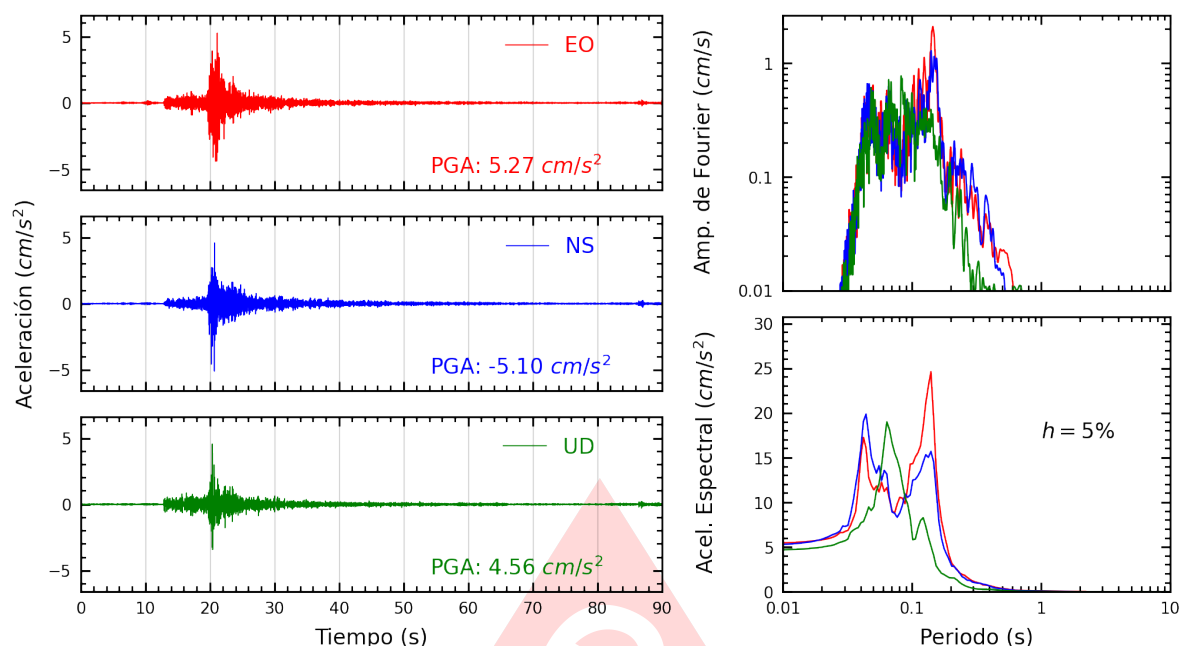
Figura A.7: Registros tiempo-historia, espectros de Fourier y de respuesta en las direcciones EO, NS y vertical de la estación CARA2. Sismo de Ancon, Lima - Lima del 2025-06-17, 00:31:31 (Hora local)
