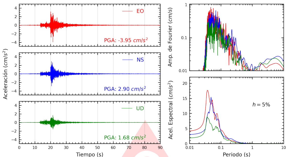
Figura A.11: Registros tiempo-historia, espectros de Fourier y de respuesta en las direcciones EO, NS y vertical de la estación CEPRE. Sismo de Ancon, Lima - Lima del 2025-06-17, 00:31:31 (Hora local)
