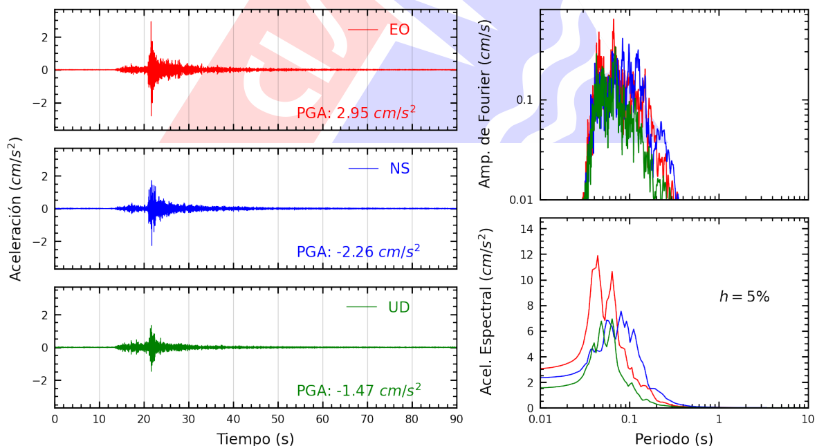
Figura A.20: Registros tiempo-historia, espectros de Fourier y de respuesta en las direcciones EO, NS y vertical de la estación ATARJ. Sismo de Ancon, Lima - Lima del 2025-06-17, 00:31:31 (Hora local)
