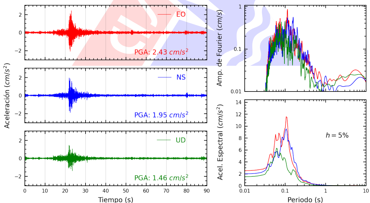
Figura A.26: Registros tiempo-historia, espectros de Fourier y de respuesta en las direcciones EO, NS y vertical de la estación SOBAR. Sismo de Ancon, Lima - Lima del 2025-06-17, 00:31:31 (Hora local)
