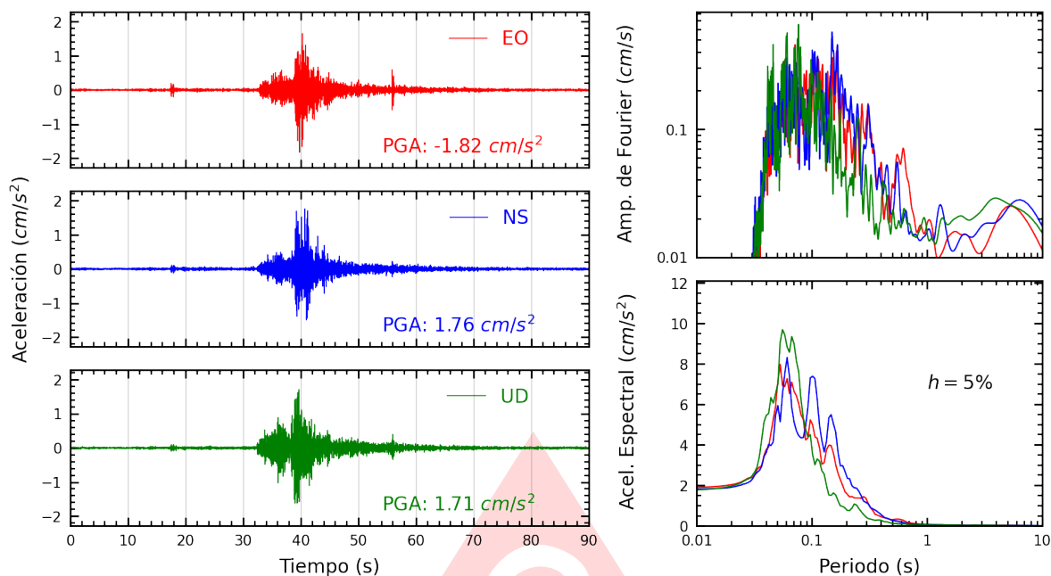
Figura A.35: Registros tiempo-historia, espectros de Fourier y de respuesta en las direcciones EO, NS y vertical de la estación PRADO. Sismo de Ancon, Lima - Lima del 2025-06-17, 00:31:31 (Hora local)
