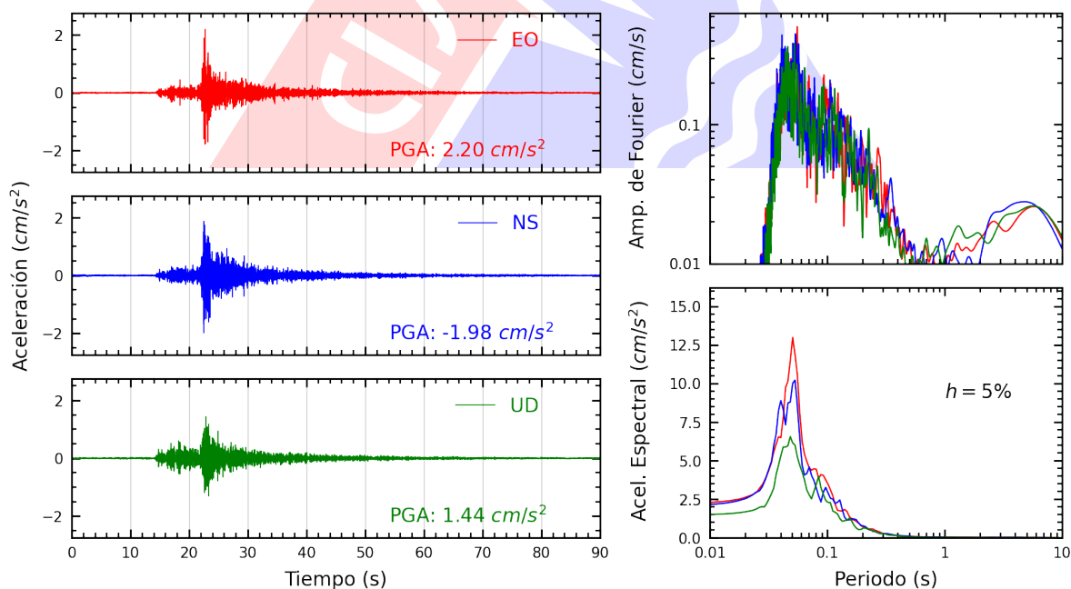
Figura A.28: Registros tiempo-historia, espectros de Fourier y de respuesta en las direcciones EO, NS y vertical de la estación USMP. Sismo de Ancon, Lima - Lima del 2025-06-17, 00:31:31 (Hora local)
