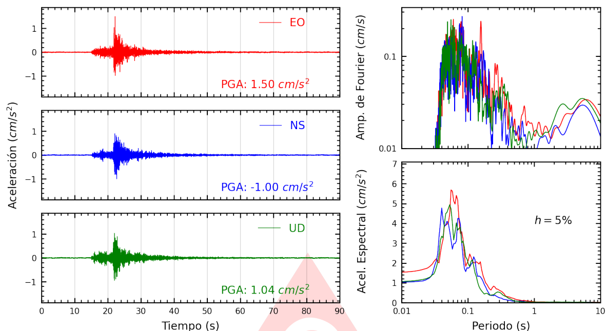
Figura A.37: Registros tiempo-historia, espectros de Fourier y de respuesta en las direcciones EO, NS y vertical de la estación UNMSM. Sismo de Ancon, Lima - Lima del 2025-06-17, 00:31:31 (Hora local)
