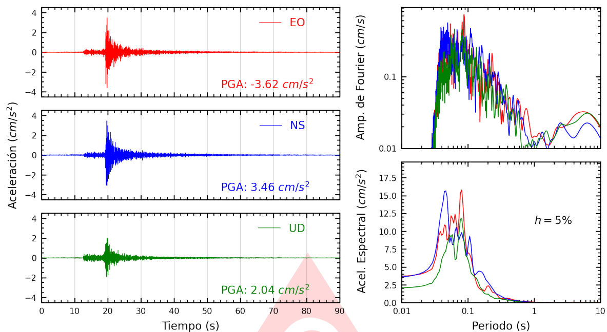
Figura A.15: Registros tiempo-historia, espectros de Fourier y de respuesta en las direcciones EO, NS y vertical de la estación COMAS. Sismo de Ancon, Lima - Lima del 2025-06-17, 00:31:31 (Hora local)
