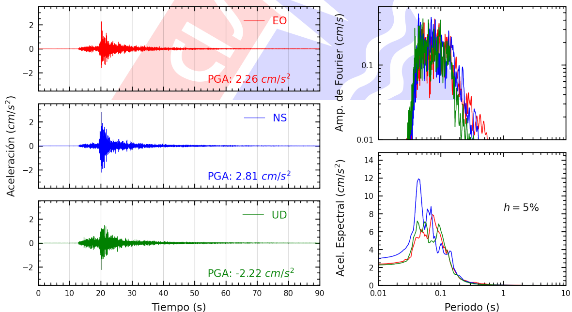
Figura A.22: Registros tiempo-historia, espectros de Fourier y de respuesta en las direcciones EO, NS y vertical de la estación JALV2. Sismo de Ancon, Lima - Lima del 2025-06-17, 00:31:31 (Hora local)
