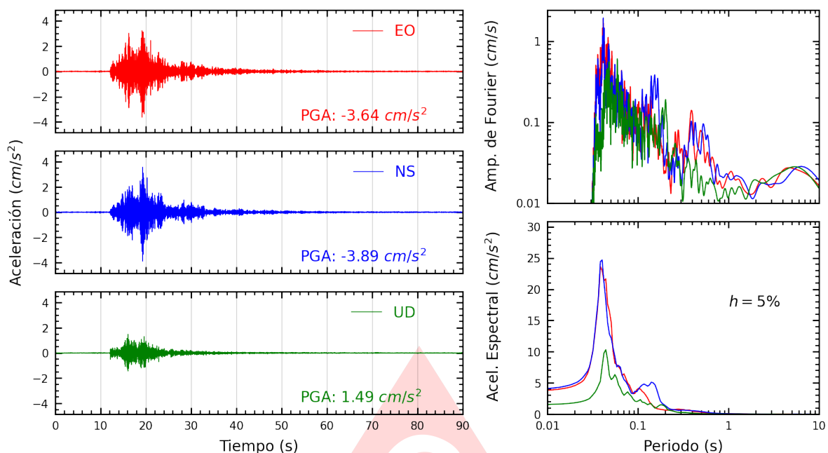
Figura A.13: Registros tiempo-historia, espectros de Fourier y de respuesta en las direcciones EO, NS y vertical de la estación DHNPE. Sismo de Ancon, Lima - Lima del 2025-06-17, 00:31:31 (Hora local)
