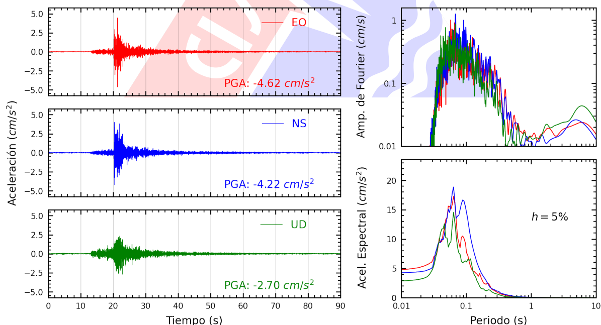
Figura A.8: Registros tiempo-historia, espectros de Fourier y de respuesta en las direcciones EO, NS y vertical de la estación SJLSC. Sismo de Ancon, Lima - Lima del 2025-06-17, 00:31:31 (Hora local)
