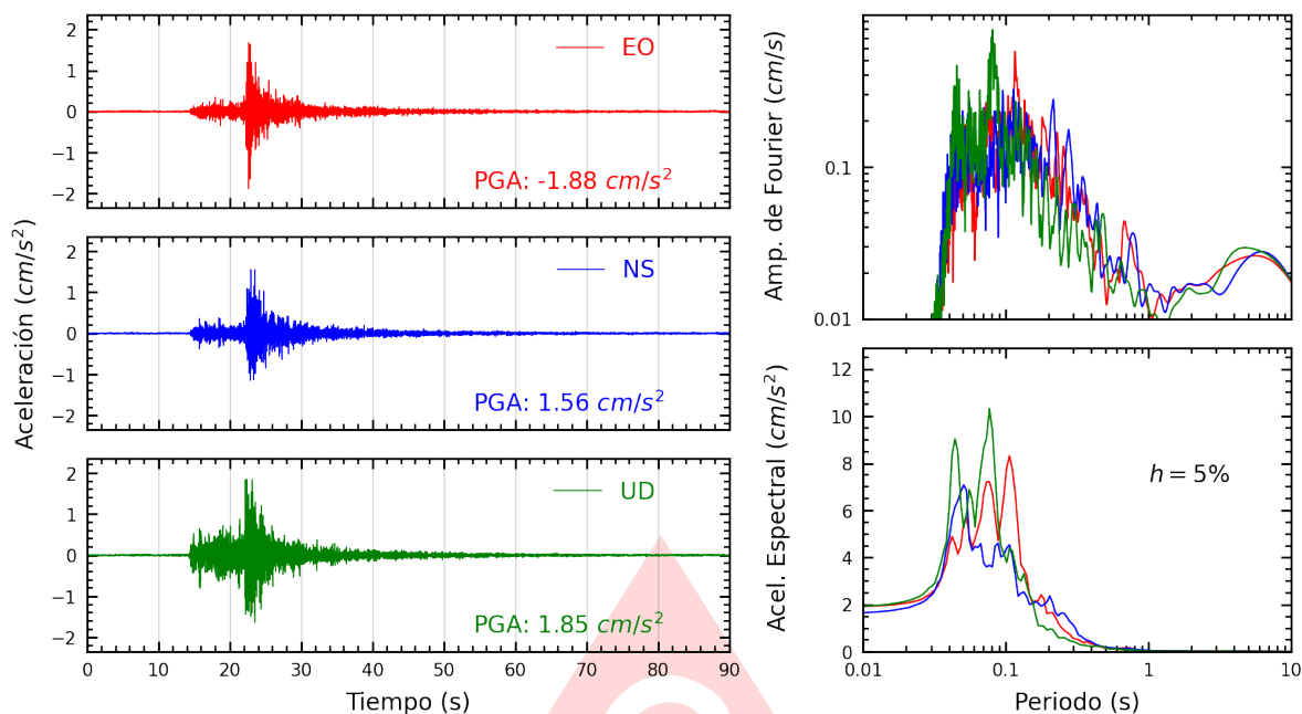
Figura A.33: Registros tiempo-historia, espectros de Fourier y de respuesta en las direcciones EO, NS y vertical de la estación SOCHO. Sismo de Ancon, Lima - Lima del 2025-06-17, 00:31:31 (Hora local)
