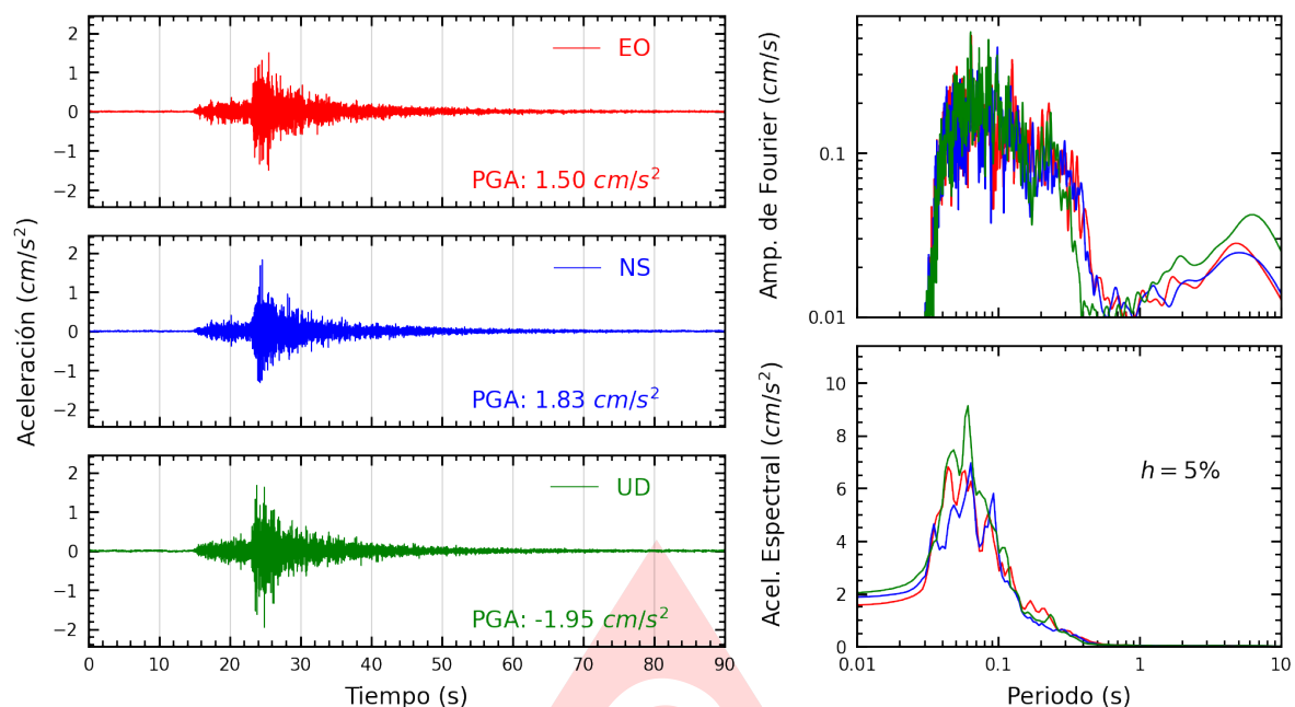
Figura A.31: Registros tiempo-historia, espectros de Fourier y de respuesta en las direcciones EO, NS y vertical de la estación SOVES. Sismo de Ancon, Lima - Lima del 2025-06-17, 00:31:31 (Hora local)
