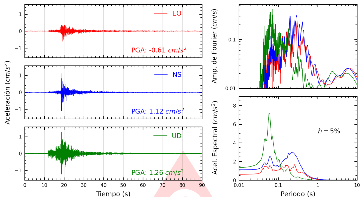
Figura A.39: Registros tiempo-historia, espectros de Fourier y de respuesta en las direcciones EO, NS y vertical de la estación ACAPU. Sismo de Ancon, Lima - Lima del 2025-06-17, 00:31:31 (Hora local)
