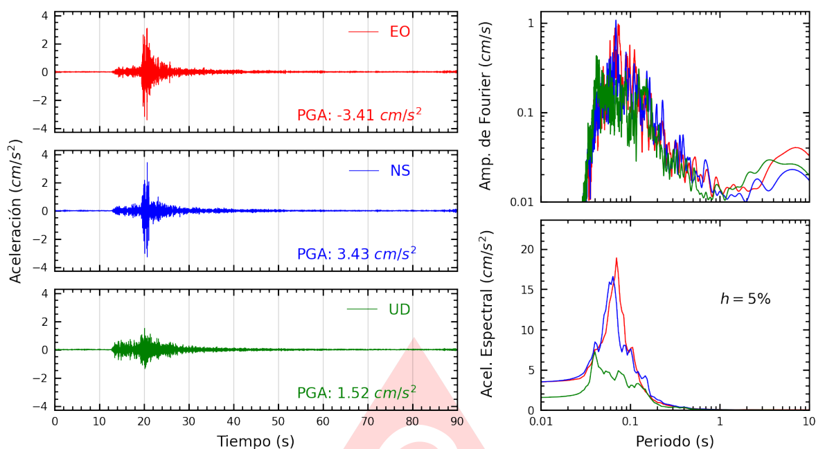
Figura A.17: Registros tiempo-historia, espectros de Fourier y de respuesta en las direcciones EO, NS y vertical de la estación UPCSM. Sismo de Ancon, Lima - Lima del 2025-06-17, 00:31:31 (Hora local)
