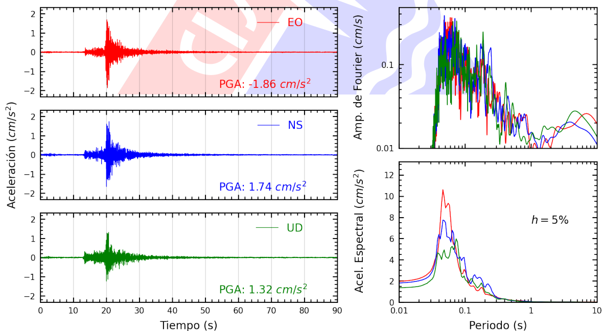
Figura A.34: Registros tiempo-historia, espectros de Fourier y de respuesta en las direcciones EO, NS y vertical de la estación UNFV. Sismo de Ancon, Lima - Lima del 2025-06-17, 00:31:31 (Hora local)
