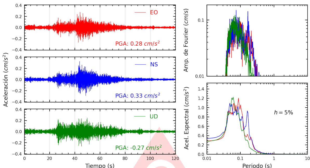
Figura A.43: Registros tiempo-historia, espectros de Fourier y de respuesta en las direcciones EO, NS y vertical de la estación ASIA. Sismo de Ancon, Lima - Lima del 2025-06-17, 00:31:31 (Hora local)
