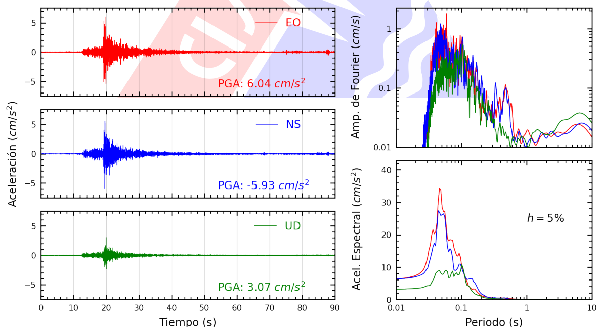
Figura A.4: Registros tiempo-historia, espectros de Fourier y de respuesta en las direcciones EO, NS y vertical de la estación OLIVO. Sismo de Ancon, Lima - Lima del 2025-06-17, 00:31:31 (Hora local)
