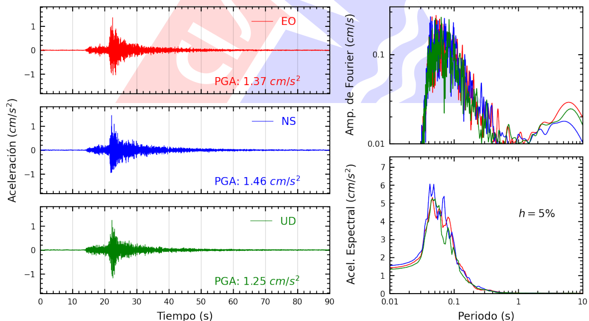
Figura A.38: Registros tiempo-historia, espectros de Fourier y de respuesta en las direcciones EO, NS y vertical de la estación SERVI. Sismo de Ancon, Lima - Lima del 2025-06-17, 00:31:31 (Hora local)
