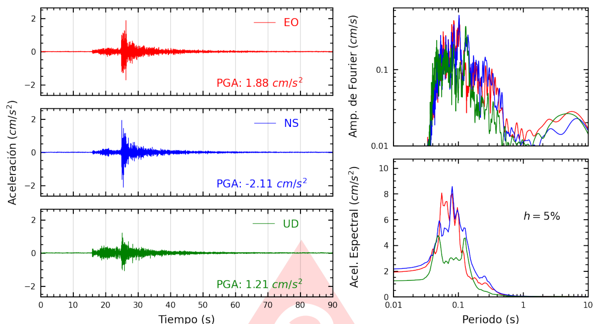
Figura A.29: Registros tiempo-historia, espectros de Fourier y de respuesta en las direcciones EO, NS y vertical de la estación USILP. Sismo de Ancon, Lima - Lima del 2025-06-17, 00:31:31 (Hora local)
