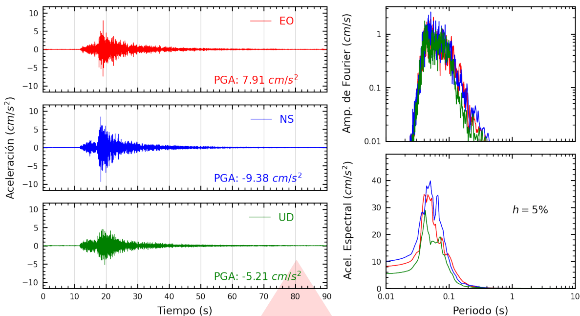
Figura A.1: Registros tiempo-historia, espectros de Fourier y de respuesta en las direcciones EO, NS y vertical de la estación SROS2. Sismo de Ancon, Lima - Lima del 2025-06-17, 00:31:31 (Hora local)
