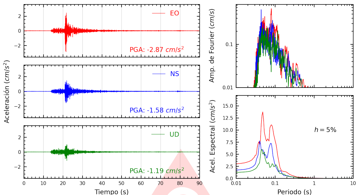
Figura A.21: Registros tiempo-historia, espectros de Fourier y de respuesta en las direcciones EO, NS y vertical de la estación BORJA. Sismo de Ancon, Lima - Lima del 2025-06-17, 00:31:31 (Hora local)
