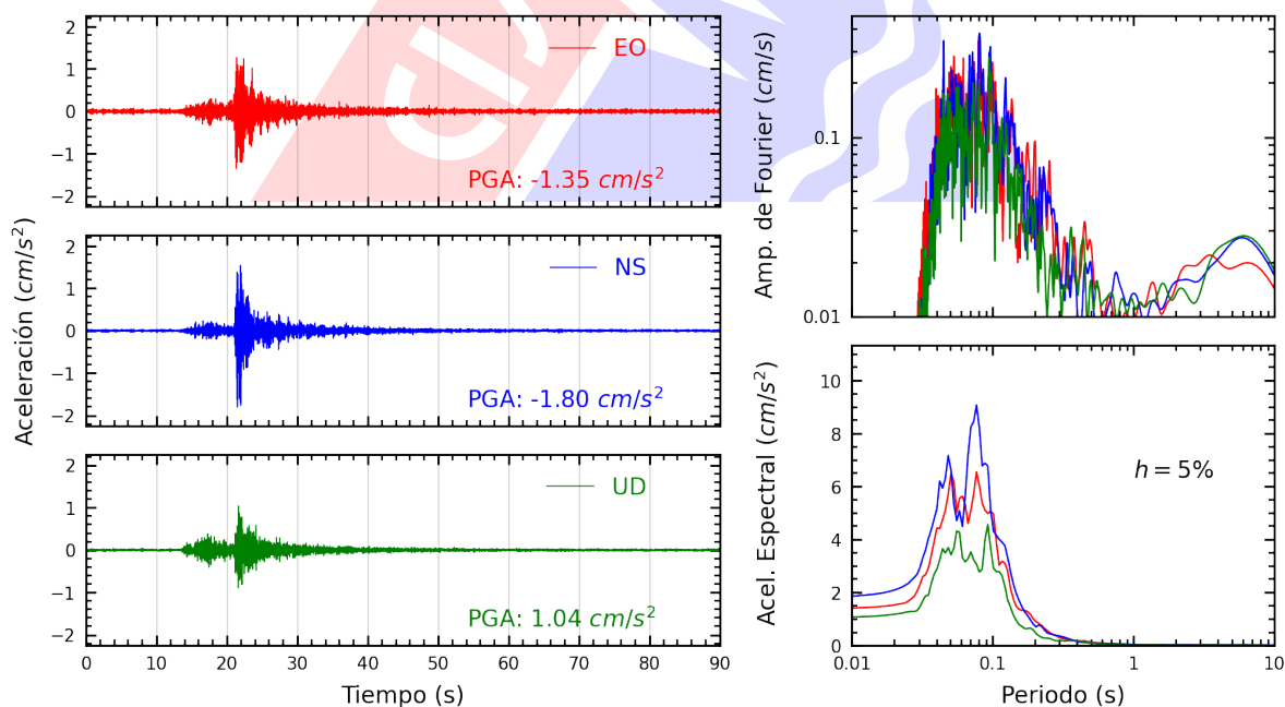
Figura A.36: Registros tiempo-historia, espectros de Fourier y de respuesta en las direcciones EO, NS y vertical de la estación INICT. Sismo de Ancon, Lima - Lima del 2025-06-17, 00:31:31 (Hora local)
