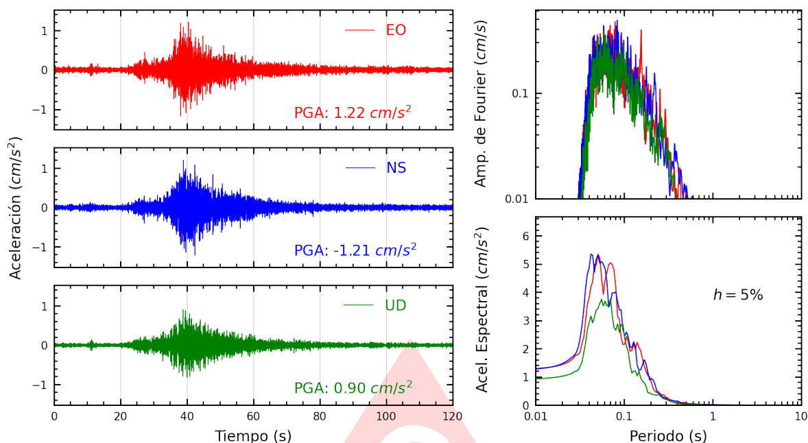
Figura A.3: Registros tiempo-historia, espectros de Fourier y de respuesta en las direcciones EO, NS y vertical de la estación PHERM. Sismo de San Vicente De Cañete, Cañete - Lima del 2025-06-24, 20:48:53 (Hora local)
