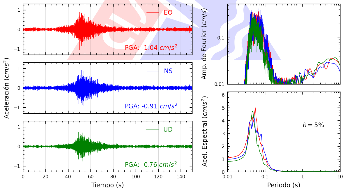
Figura A.6: Registros tiempo-historia, espectros de Fourier y de respuesta en las direcciones EO, NS y vertical de la estación JOSEO. Sismo de San Vicente De Cañete, Cañete - Lima del 2025-06-24, 20:48:53 (Hora local)
