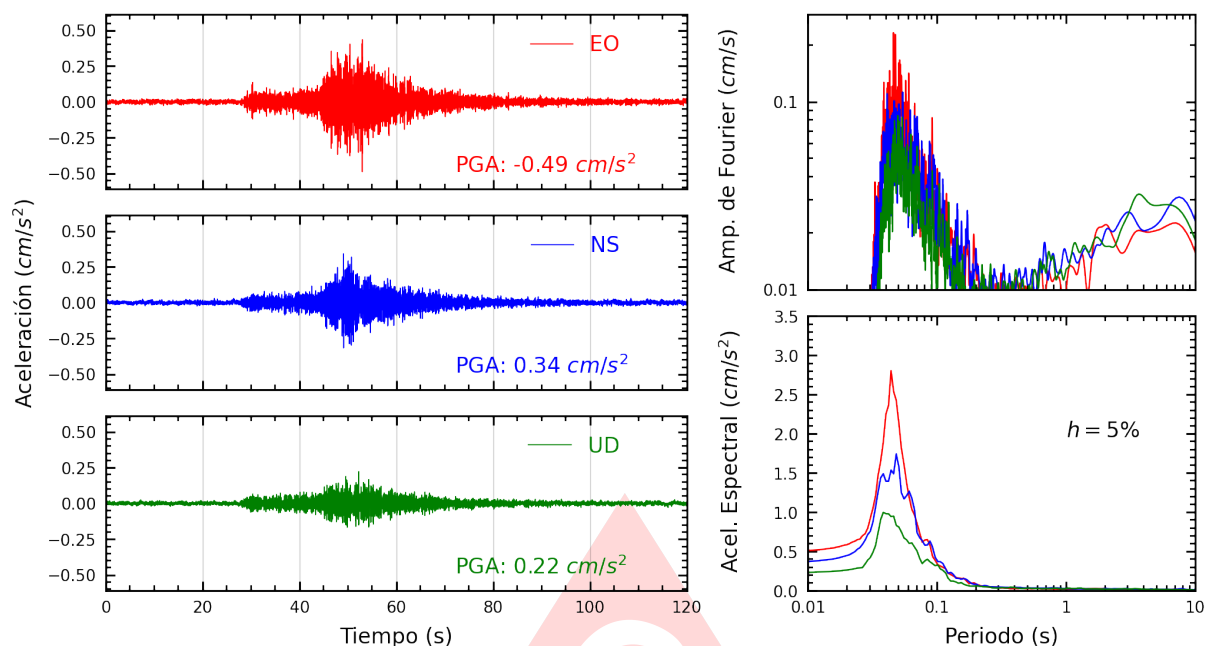
Figura A.23: Registros tiempo-historia, espectros de Fourier y de respuesta en las direcciones EO, NS y vertical de la estación UCSS. Sismo de San Vicente De Cañete, Cañete - Lima del 2025-06-24, 20:48:53 (Hora local)
