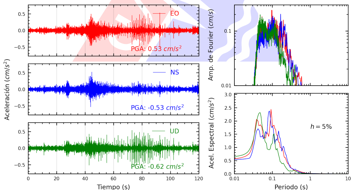
Figura A.16: Registros tiempo-historia, espectros de Fourier y de respuesta en las direcciones EO, NS y vertical de la estación SCCHO. Sismo de San Vicente De Cañete, Cañete - Lima del 2025-06-24, 20:48:53 (Hora local)
