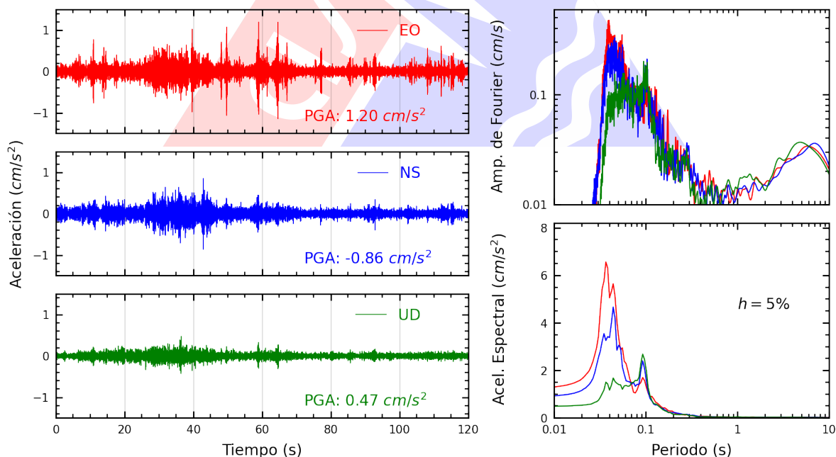
Figura A.4: Registros tiempo-historia, espectros de Fourier y de respuesta en las direcciones EO, NS y vertical de la estación OLIVO. Sismo de San Vicente De Cañete, Cañete - Lima del 2025-06-24, 20:48:53 (Hora local)
