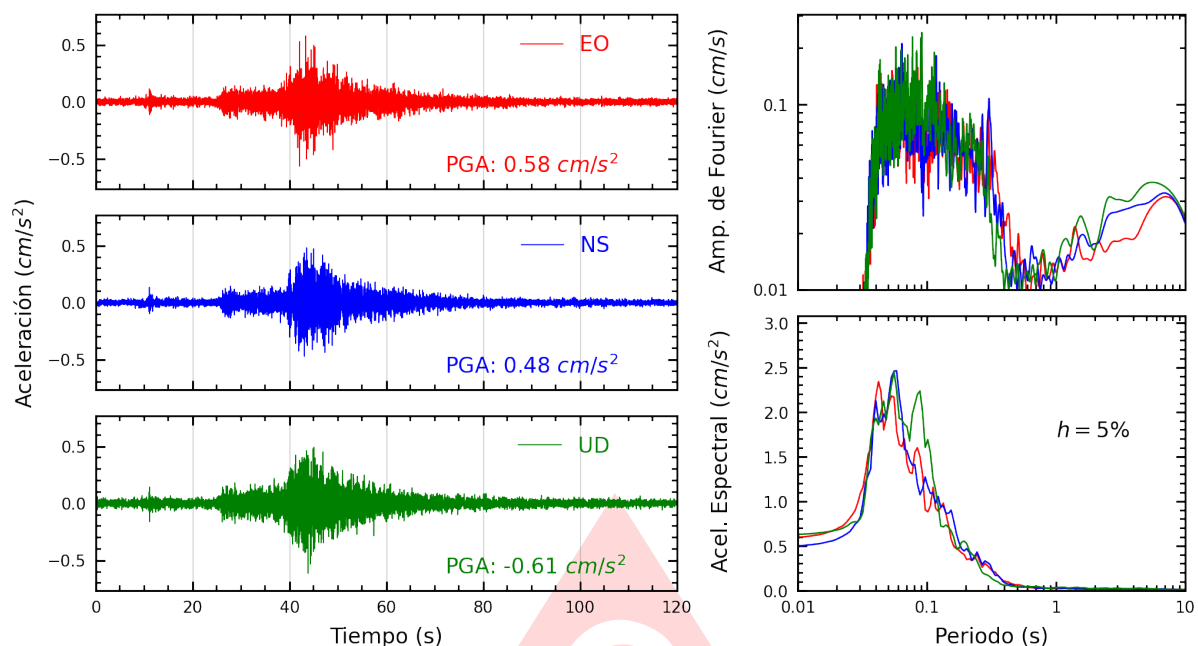
Figura A.17: Registros tiempo-historia, espectros de Fourier y de respuesta en las direcciones EO, NS y vertical de la estación SOVES. Sismo de San Vicente De Cañete, Cañete - Lima del 2025-06-24, 20:48:53 (Hora local)
