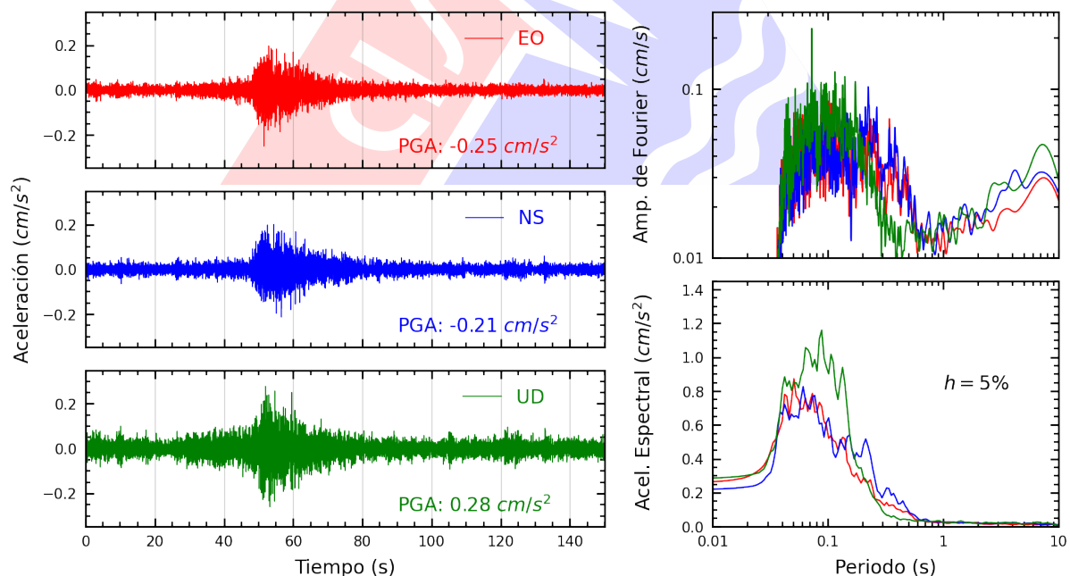
Figura A.36: Registros tiempo-historia, espectros de Fourier y de respuesta en las direcciones EO, NS y vertical de la estación MDPP. Sismo de San Vicente De Cañete, Cañete - Lima del 2025-06-24, 20:48:53 (Hora local)
