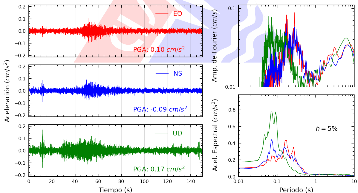
Figura A.40: Registros tiempo-historia, espectros de Fourier y de respuesta en las direcciones EO, NS y vertical de la estación ACAPU. Sismo de San Vicente De Cañete, Cañete - Lima del 2025-06-24, 20:48:53 (Hora local)
