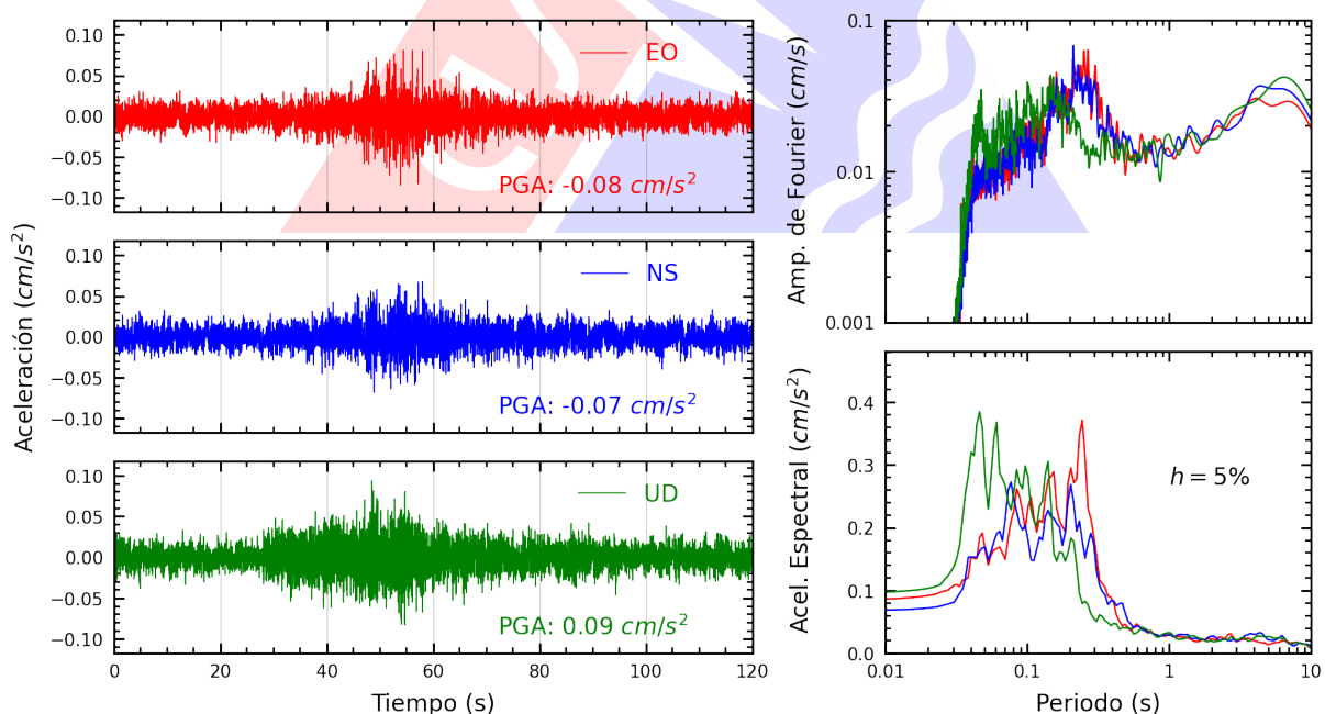
Figura A.44: Registros tiempo-historia, espectros de Fourier y de respuesta en las direcciones EO, NS y vertical de la estación DSMI. Sismo de San Vicente De Cañete, Cañete - Lima del 2025-06-24, 20:48:53 (Hora local)
