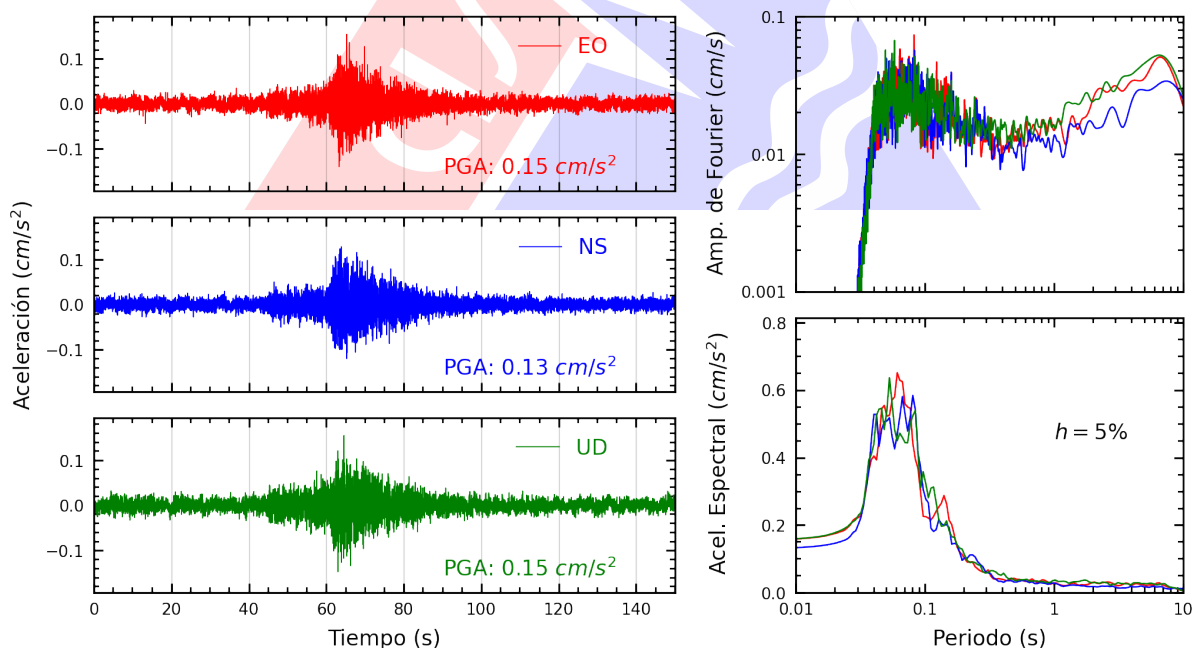
Figura A.42: Registros tiempo-historia, espectros de Fourier y de respuesta en las direcciones EO, NS y vertical de la estación UNMSM. Sismo de San Vicente De Cañete, Cañete - Lima del 2025-06-24, 20:48:53 (Hora local)
