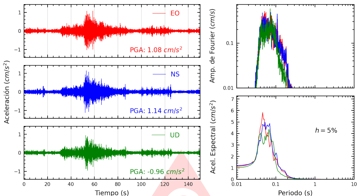
Figura A.5: Registros tiempo-historia, espectros de Fourier y de respuesta en las direcciones EO, NS y vertical de la estación SROSA. Sismo de San Vicente De Cañete, Cañete - Lima del 2025-06-24, 20:48:53 (Hora local)
