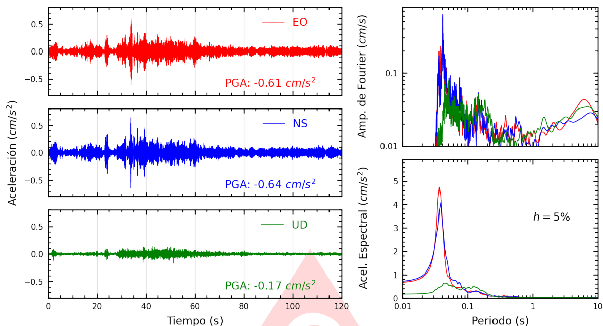
Figura A.15: Registros tiempo-historia, espectros de Fourier y de respuesta en las direcciones EO, NS y vertical de la estación DHNPE. Sismo de San Vicente De Cañete, Cañete - Lima del 2025-06-24, 20:48:53 (Hora local)
