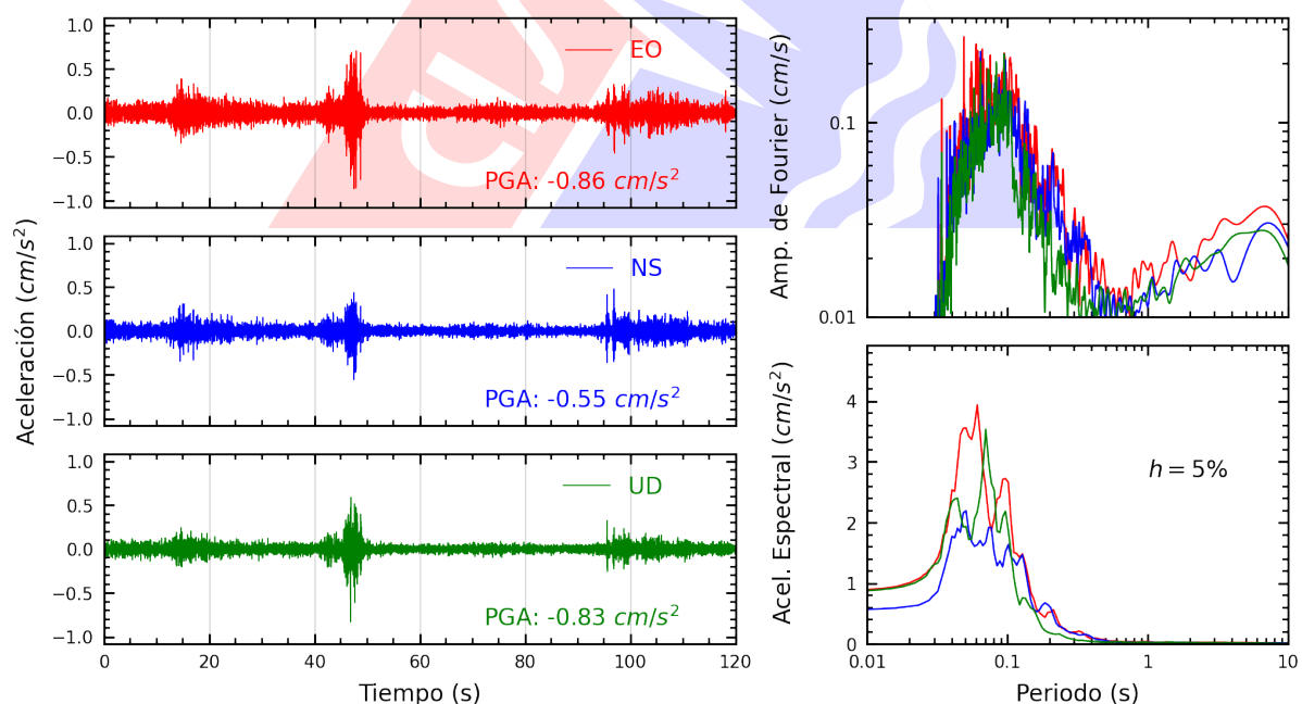
Figura A.8: Registros tiempo-historia, espectros de Fourier y de respuesta en las direcciones EO, NS y vertical de la estación SOBAR. Sismo de San Vicente De Cañete, Cañete - Lima del 2025-06-24, 20:48:53 (Hora local)
