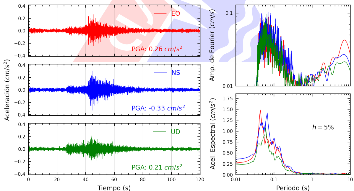
Figura A.30: Registros tiempo-historia, espectros de Fourier y de respuesta en las direcciones EO, NS y vertical de la estación SERVI. Sismo de San Vicente De Cañete, Cañete - Lima del 2025-06-24, 20:48:53 (Hora local)
