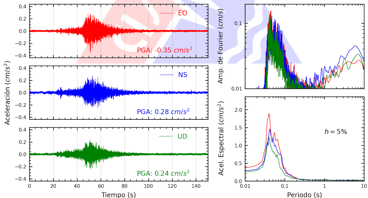
Figura A.28: Registros tiempo-historia, espectros de Fourier y de respuesta en las direcciones EO, NS y vertical de la estación SJLCE. Sismo de San Vicente De Cañete, Cañete - Lima del 2025-06-24, 20:48:53 (Hora local)
