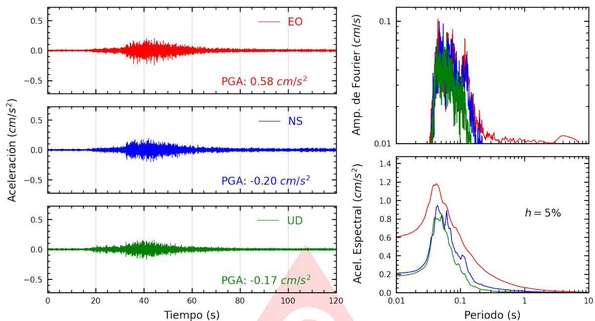
Figura A.19: Registros tiempo-historia, espectros de Fourier y de respuesta en las direcciones EO, NS y vertical de la estación ATARJ. Sismo de San Vicente De Cañete, Cañete - Lima del 2025-06-24, 20:48:53 (Hora local)
