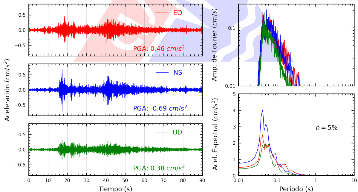
Figura A.14: Registros tiempo-historia, espectros de Fourier y de respuesta en las direcciones EO, NS y vertical de la estación PACHA. Sismo de San Vicente De Cañete, Cañete - Lima del 2025-06-24, 20:48:53 (Hora local)
