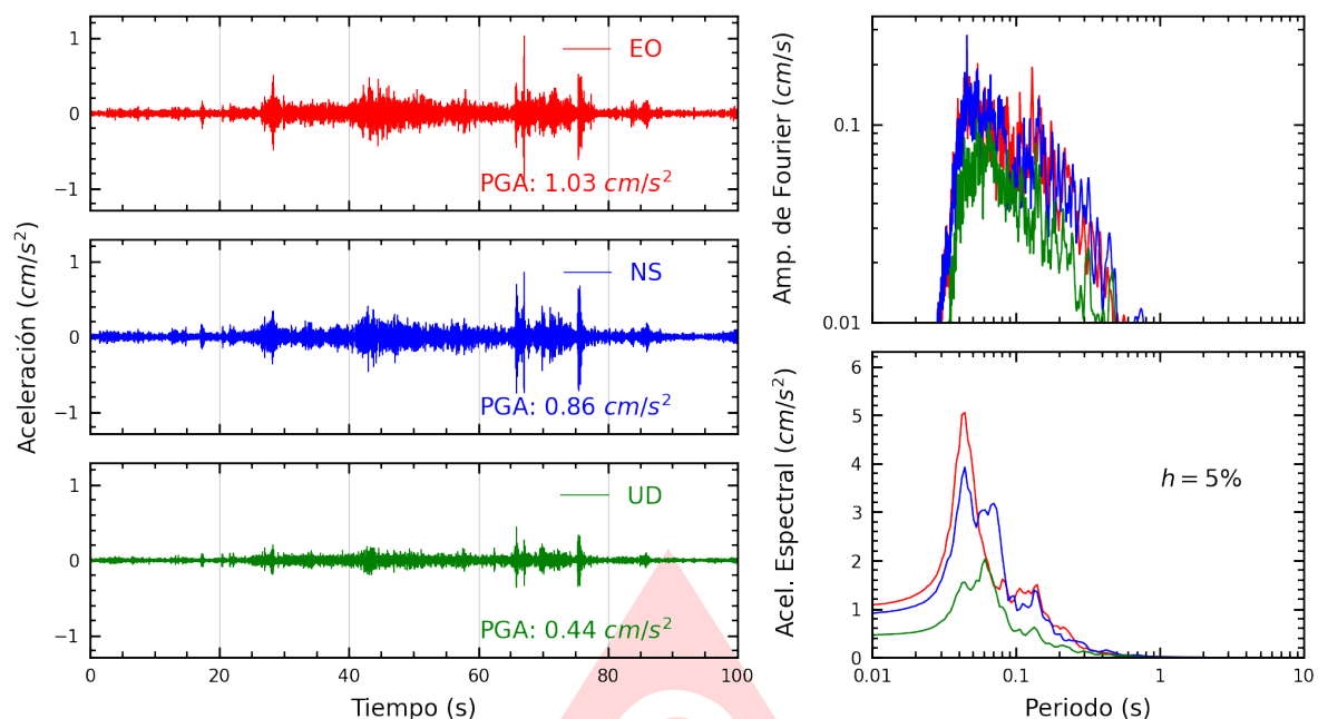
Figura A.7: Registros tiempo-historia, espectros de Fourier y de respuesta en las direcciones EO, NS y vertical de la estación BRIS2. Sismo de San Vicente De Cañete, Cañete - Lima del 2025-06-24, 20:48:53 (Hora local)
