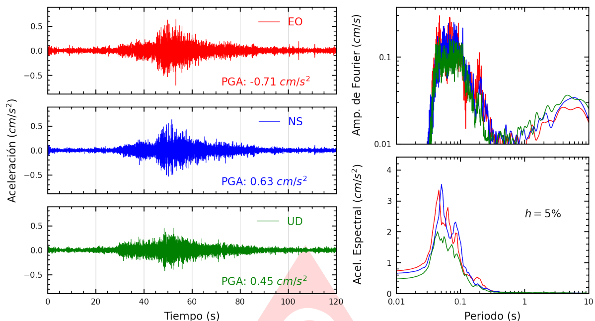
Figura A.13: Registros tiempo-historia, espectros de Fourier y de respuesta en las direcciones EO, NS y vertical de la estación INDEP. Sismo de San Vicente De Cañete, Cañete - Lima del 2025-06-24, 20:48:53 (Hora local)
