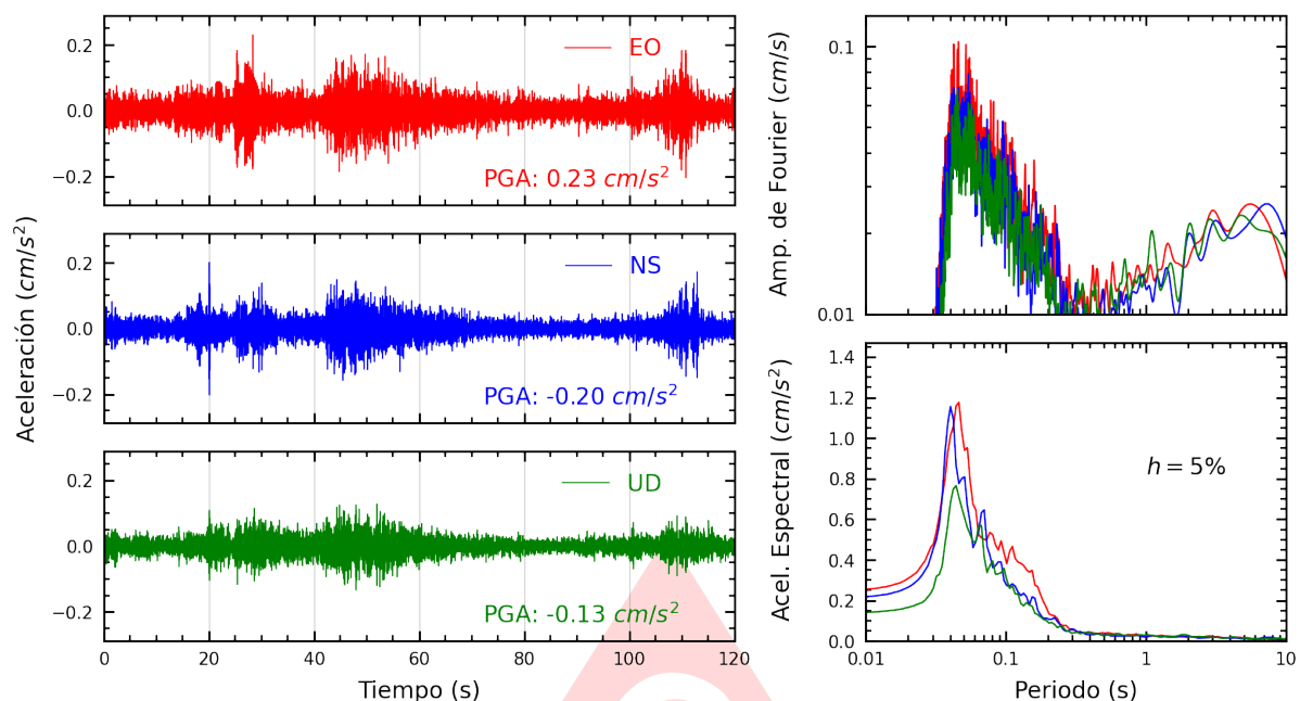
Figura A.37: Registros tiempo-historia, espectros de Fourier y de respuesta en las direcciones EO, NS y vertical de la estación INICT. Sismo de San Vicente De Cañete, Cañete - Lima del 2025-06-24, 20:48:53 (Hora local)
