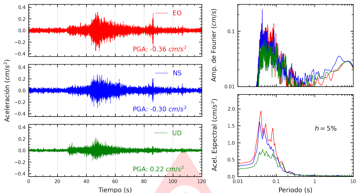
Figura A.27: Registros tiempo-historia, espectros de Fourier y de respuesta en las direcciones EO, NS y vertical de la estación CEPRE. Sismo de San Vicente De Cañete, Cañete - Lima del 2025-06-24, 20:48:53 (Hora local)
