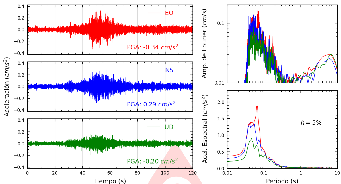
Figura A.29: Registros tiempo-historia, espectros de Fourier y de respuesta en las direcciones EO, NS y vertical de la estación FICPE. Sismo de San Vicente De Cañete, Cañete - Lima del 2025-06-24, 20:48:53 (Hora local)
