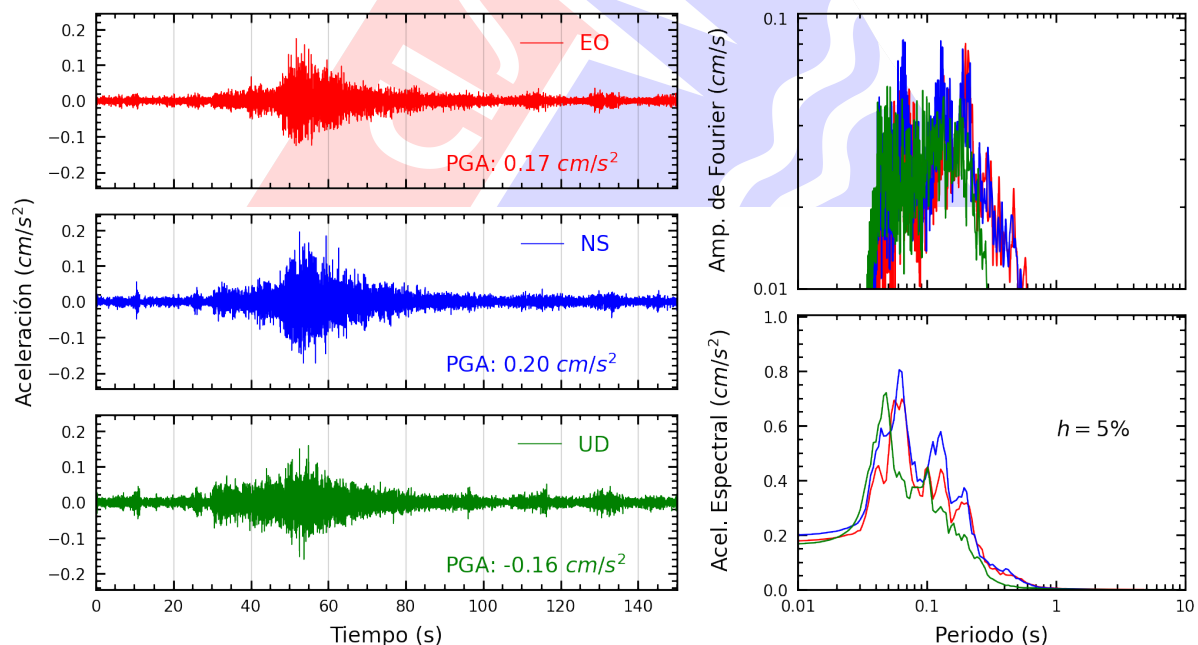
Figura A.38: Registros tiempo-historia, espectros de Fourier y de respuesta en las direcciones EO, NS y vertical de la estación VHAYA. Sismo de San Vicente De Cañete, Cañete - Lima del 2025-06-24, 20:48:53 (Hora local)
