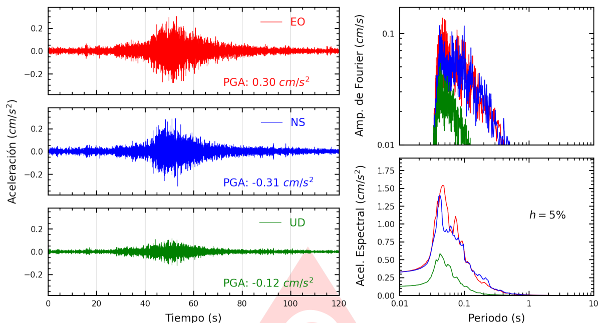
Figura A.33: Registros tiempo-historia, espectros de Fourier y de respuesta en las direcciones EO, NS y vertical de la estación UCVAT. Sismo de San Vicente De Cañete, Cañete - Lima del 2025-06-24, 20:48:53 (Hora local)
