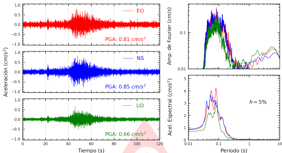
Figura A.9: Registros tiempo-historia, espectros de Fourier y de respuesta en las direcciones EO, NS y vertical de la estación USILM. Sismo de San Vicente De Cañete, Cañete - Lima del 2025-06-24, 20:48:53 (Hora local)
