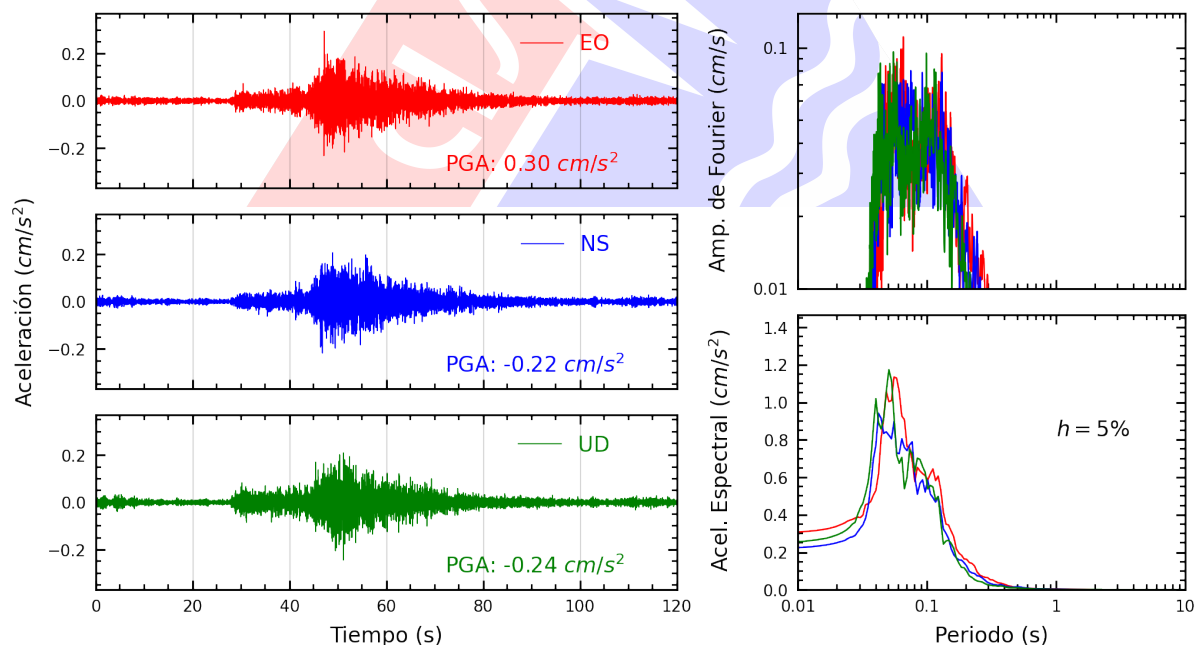
Figura A.34: Registros tiempo-historia, espectros de Fourier y de respuesta en las direcciones EO, NS y vertical de la estación JALV2. Sismo de San Vicente De Cañete, Cañete - Lima del 2025-06-24, 20:48:53 (Hora local)
