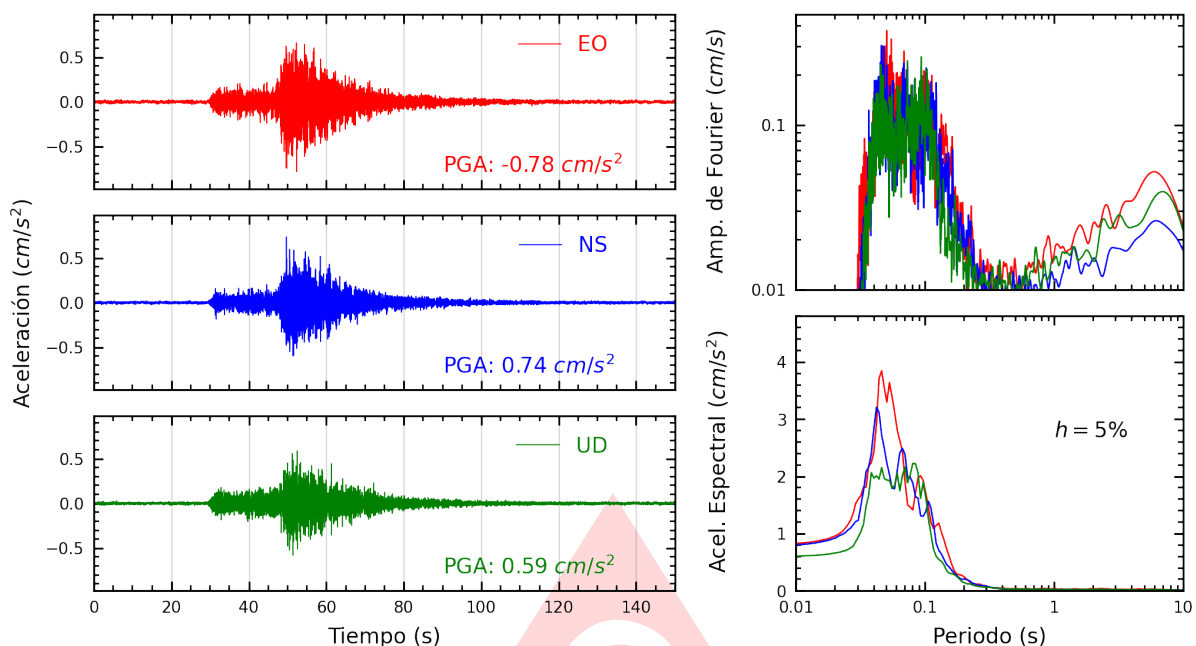
Figura A.11: Registros tiempo-historia, espectros de Fourier y de respuesta en las direcciones EO, NS y vertical de la estación AMORE. Sismo de San Vicente De Cañete, Cañete - Lima del 2025-06-24, 20:48:53 (Hora local)
