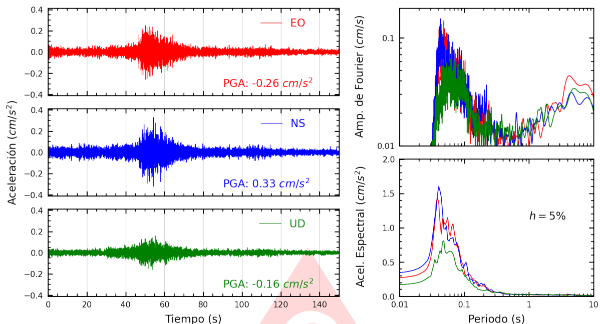
Figura A.31: Registros tiempo-historia, espectros de Fourier y de respuesta en las direcciones EO, NS y vertical de la estación COMAS. Sismo de San Vicente De Cañete, Cañete - Lima del 2025-06-24, 20:48:53 (Hora local)
