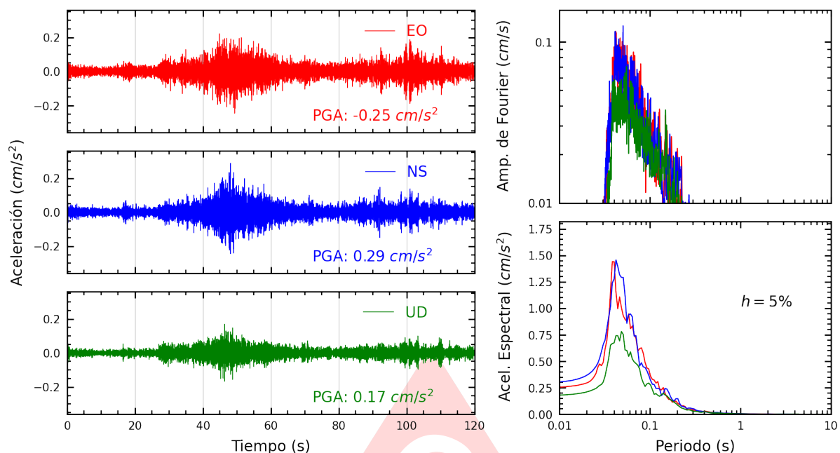
Figura A.35: Registros tiempo-historia, espectros de Fourier y de respuesta en las direcciones EO, NS y vertical de la estación BORJA. Sismo de San Vicente De Cañete, Cañete - Lima del 2025-06-24, 20:48:53 (Hora local)
