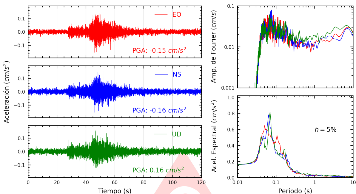
Figura A.41: Registros tiempo-historia, espectros de Fourier y de respuesta en las direcciones EO, NS y vertical de la estación UNFV. Sismo de San Vicente De Cañete, Cañete - Lima del 2025-06-24, 20:48:53 (Hora local)
