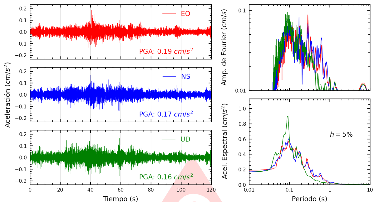
Figura A.39: Registros tiempo-historia, espectros de Fourier y de respuesta en las direcciones EO, NS y vertical de la estación UNICA. Sismo de San Vicente De Cañete, Cañete - Lima del 2025-06-24, 20:48:53 (Hora local)
