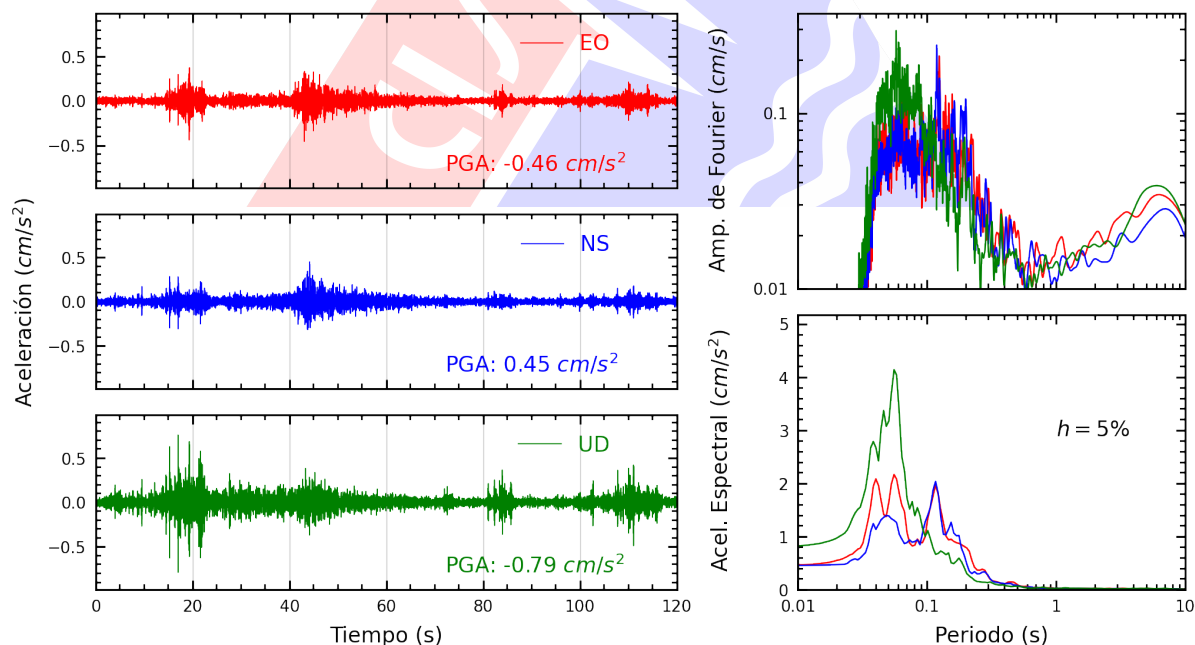
Figura A.10: Registros tiempo-historia, espectros de Fourier y de respuesta en las direcciones EO, NS y vertical de la estación SOCHO. Sismo de San Vicente De Cañete, Cañete - Lima del 2025-06-24, 20:48:53 (Hora local)
