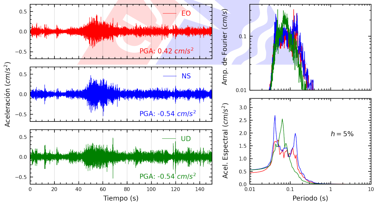
Figura A.20: Registros tiempo-historia, espectros de Fourier y de respuesta en las direcciones EO, NS y vertical de la estación CARAB. Sismo de San Vicente De Cañete, Cañete - Lima del 2025-06-24, 20:48:53 (Hora local)
