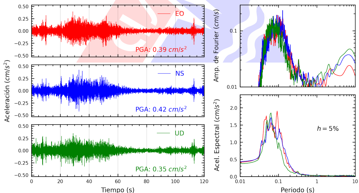
Figura A.24: Registros tiempo-historia, espectros de Fourier y de respuesta en las direcciones EO, NS y vertical de la estación SJLSV. Sismo de San Vicente De Cañete, Cañete - Lima del 2025-06-24, 20:48:53 (Hora local)
