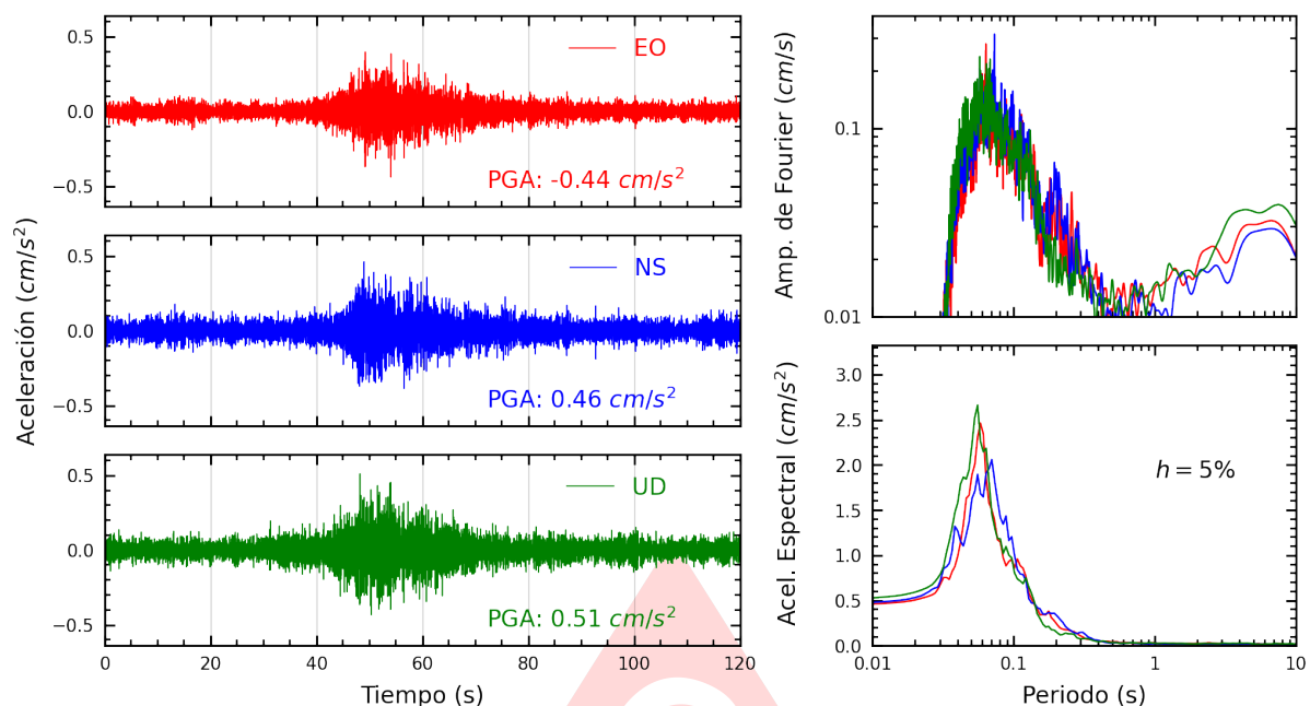
Figura A.21: Registros tiempo-historia, espectros de Fourier y de respuesta en las direcciones EO, NS y vertical de la estación SJLSC. Sismo de San Vicente De Cañete, Cañete - Lima del 2025-06-24, 20:48:53 (Hora local)
