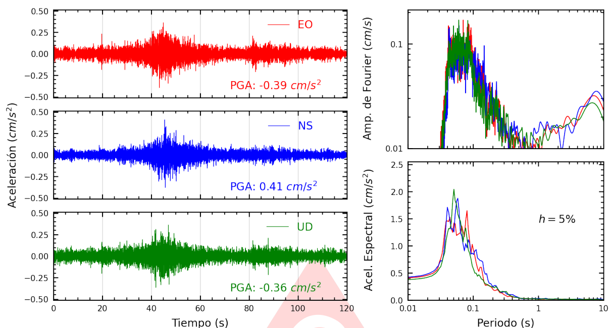
Figura A.25: Registros tiempo-historia, espectros de Fourier y de respuesta en las direcciones EO, NS y vertical de la estación URPE. Sismo de San Vicente De Cañete, Cañete - Lima del 2025-06-24, 20:48:53 (Hora local)
