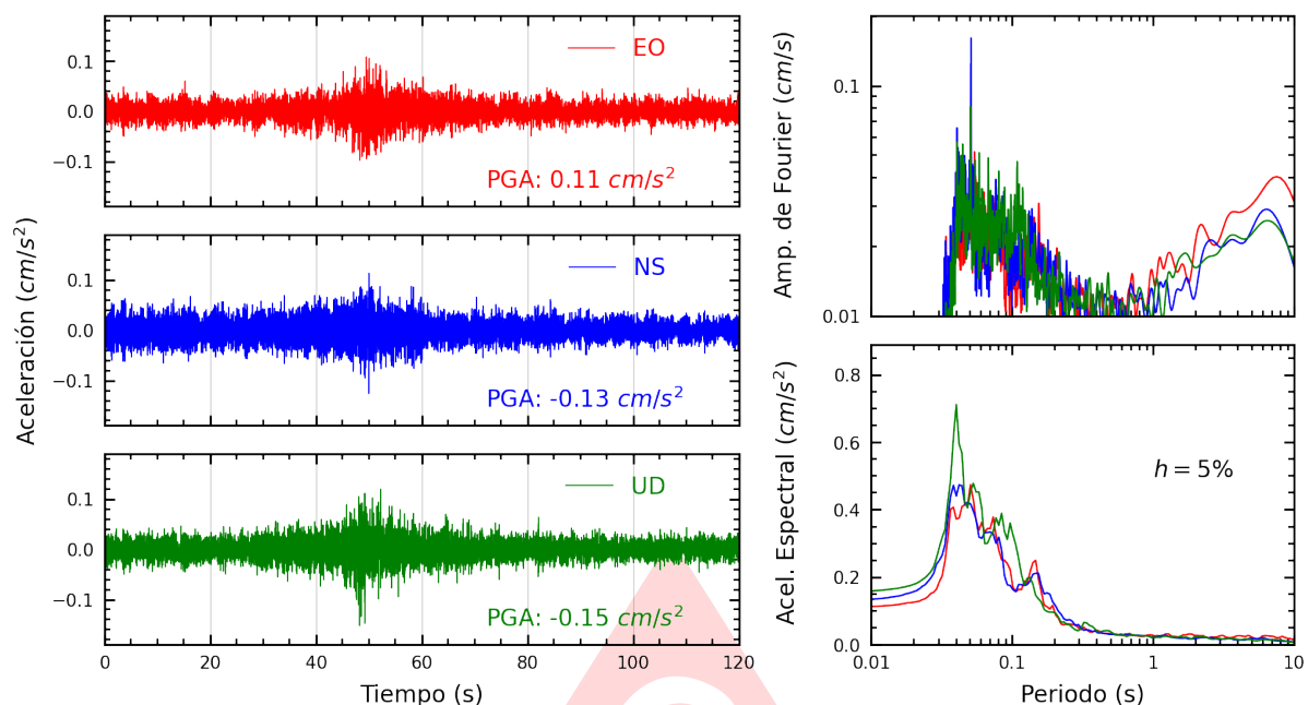
Figura A.43: Registros tiempo-historia, espectros de Fourier y de respuesta en las direcciones EO, NS y vertical de la estación BONDY. Sismo de San Vicente De Cañete, Cañete - Lima del 2025-06-24, 20:48:53 (Hora local)
