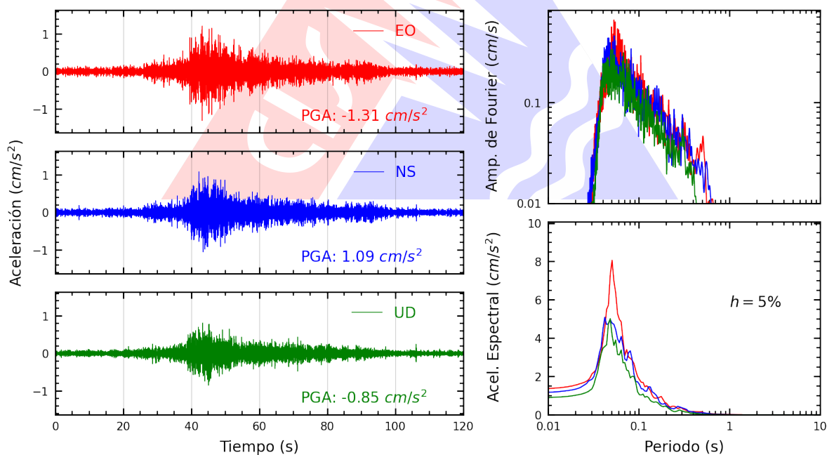
Figura A.2: Registros tiempo-historia, espectros de Fourier y de respuesta en las direcciones EO, NS y vertical de la estación UNTEL. Sismo de San Vicente De Cañete, Cañete - Lima del 2025-06-24, 20:48:53 (Hora local)
