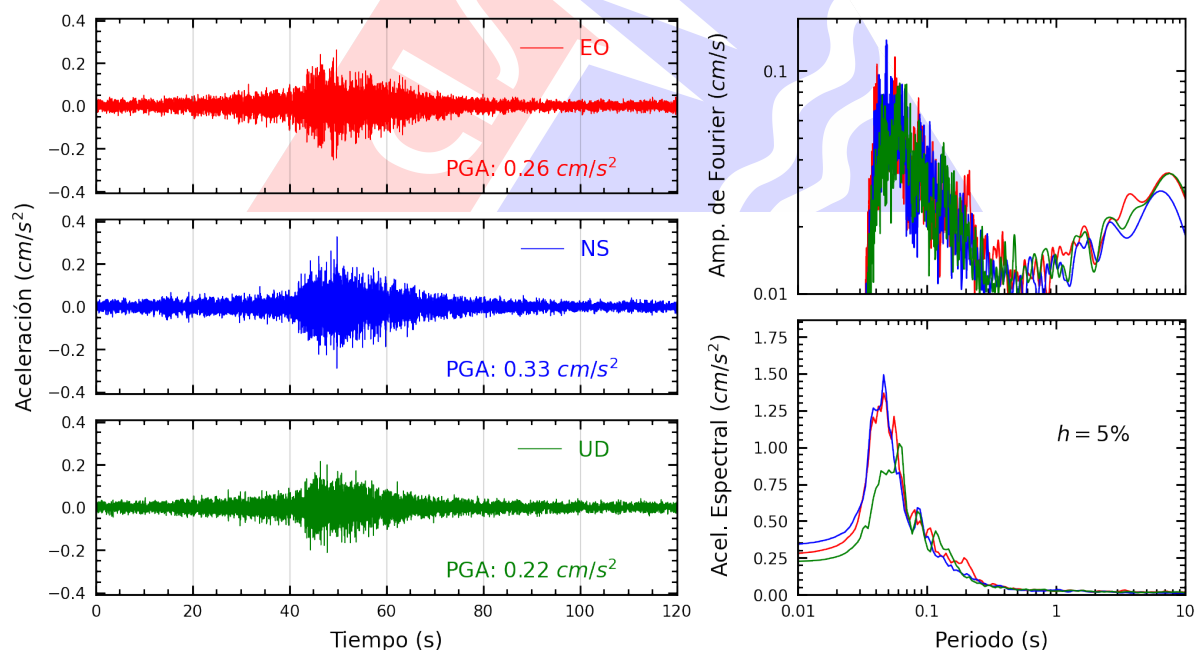
Figura A.32: Registros tiempo-historia, espectros de Fourier y de respuesta en las direcciones EO, NS y vertical de la estación IMCA. Sismo de San Vicente De Cañete, Cañete - Lima del 2025-06-24, 20:48:53 (Hora local)
