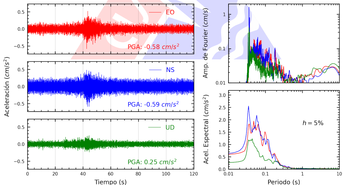
Figura A.18: Registros tiempo-historia, espectros de Fourier y de respuesta en las direcciones EO, NS y vertical de la estación UPCVI. Sismo de San Vicente De Cañete, Cañete - Lima del 2025-06-24, 20:48:53 (Hora local)
