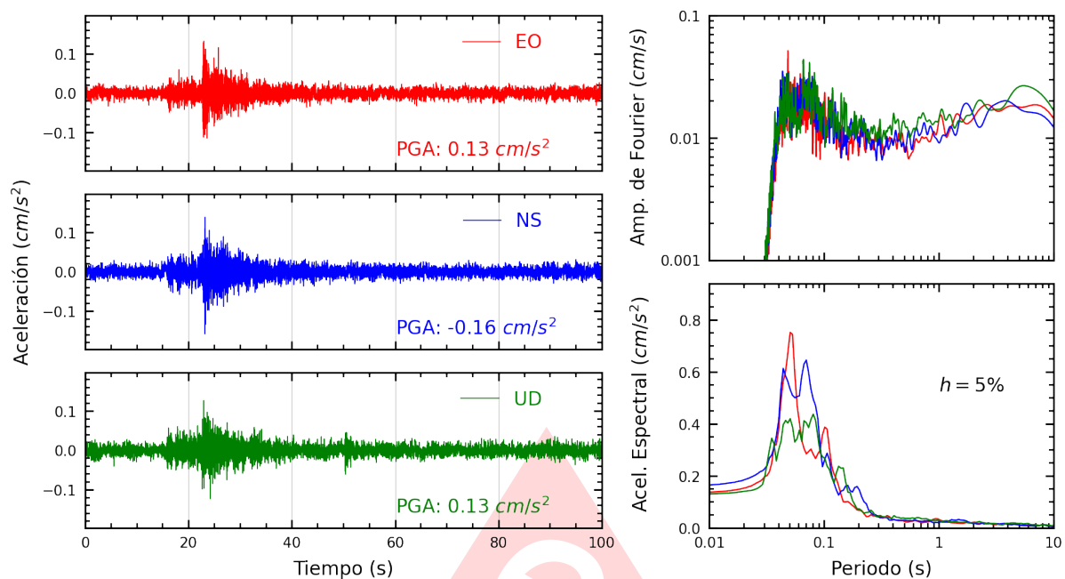
Figura A.25: Registros tiempo-historia, espectros de Fourier y de respuesta en las direcciones EO, NS y vertical de la estación UNFV. Sismo de Ancon, Lima - Lima del 2025-06-25, 20:16:54 (Hora local)
