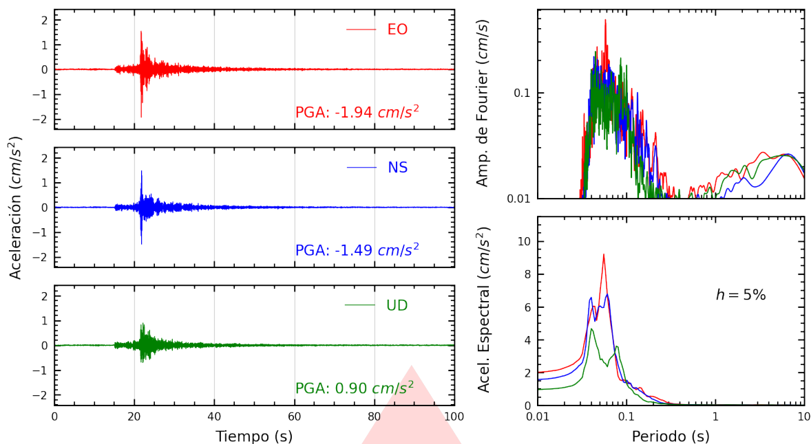
Figura A.1: Registros tiempo-historia, espectros de Fourier y de respuesta en las direcciones EO, NS y vertical de la estación AMORE. Sismo de Ancon, Lima - Lima del 2025-06-25, 20:16:54 (Hora local)
