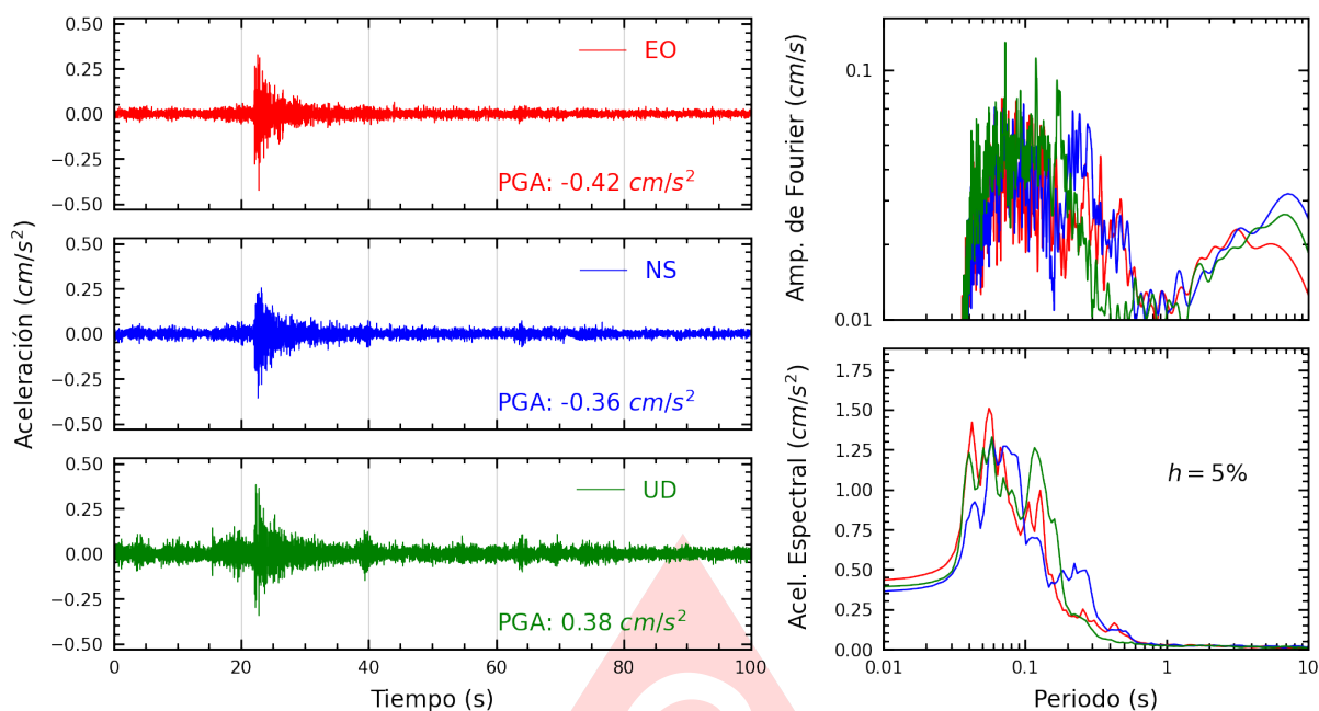
Figura A.13: Registros tiempo-historia, espectros de Fourier y de respuesta en las direcciones EO, NS y vertical de la estación MDPP. Sismo de Ancon, Lima - Lima del 2025-06-25, 20:16:54 (Hora local)
