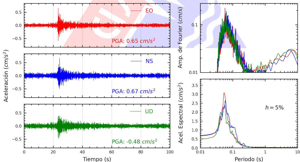
Figura A.8: Registros tiempo-historia, espectros de Fourier y de respuesta en las direcciones EO, NS y vertical de la estación SJLSC. Sismo de Ancon, Lima - Lima del 2025-06-25, 20:16:54 (Hora local)
