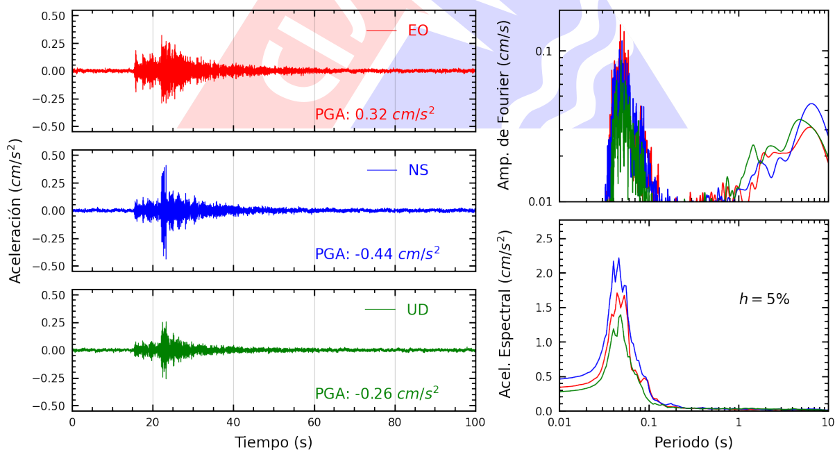
Figura A.12: Registros tiempo-historia, espectros de Fourier y de respuesta en las direcciones EO, NS y vertical de la estación UCSS. Sismo de Ancon, Lima - Lima del 2025-06-25, 20:16:54 (Hora local)
