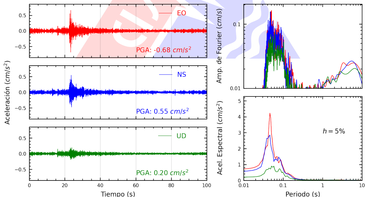
Figura A.6: Registros tiempo-historia, espectros de Fourier y de respuesta en las direcciones EO, NS y vertical de la estación FICPE. Sismo de Ancon, Lima - Lima del 2025-06-25, 20:16:54 (Hora local)
