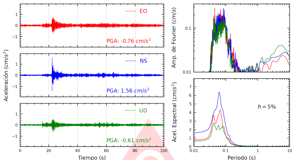
Figura A.3: Registros tiempo-historia, espectros de Fourier y de respuesta en las direcciones EO, NS y vertical de la estación INDEP. Sismo de Ancon, Lima - Lima del 2025-06-25, 20:16:54 (Hora local)
