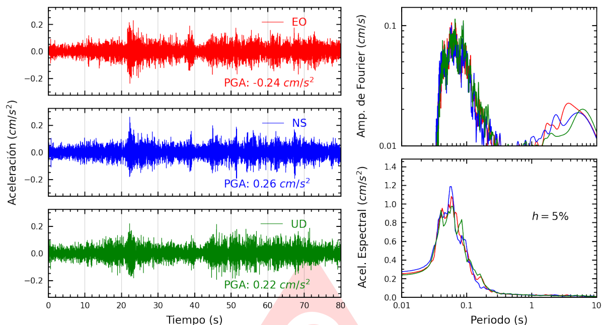
Figura A.19: Registros tiempo-historia, espectros de Fourier y de respuesta en las direcciones EO, NS y vertical de la estación MADRE. Sismo de Ancon, Lima - Lima del 2025-06-25, 20:16:54 (Hora local)
