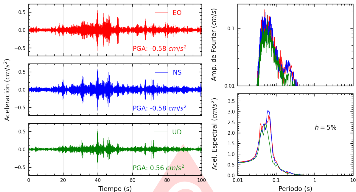
Figura A.9: Registros tiempo-historia, espectros de Fourier y de respuesta en las direcciones EO, NS y vertical de la estación BRISA. Sismo de Ancon, Lima - Lima del 2025-06-25, 20:16:54 (Hora local)
