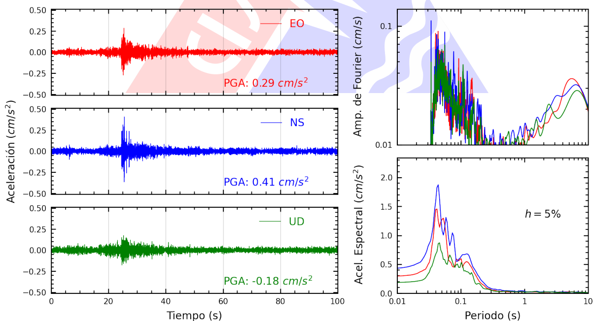
Figura A.14: Registros tiempo-historia, espectros de Fourier y de respuesta en las direcciones EO, NS y vertical de la estación USMP. Sismo de Ancon, Lima - Lima del 2025-06-25, 20:16:54 (Hora local)
