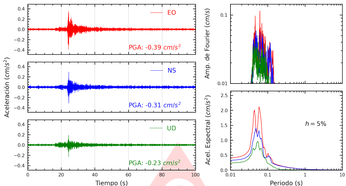
Figura A.17: Registros tiempo-historia, espectros de Fourier y de respuesta en las direcciones EO, NS y vertical de la estación ATARJ. Sismo de Ancon, Lima - Lima del 2025-06-25, 20:16:54 (Hora local)
