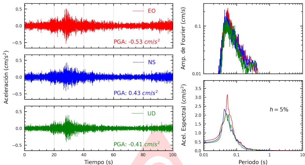
Figura A.11: Registros tiempo-historia, espectros de Fourier y de respuesta en las direcciones EO, NS y vertical de la estación UNTEL. Sismo de Ancon, Lima - Lima del 2025-06-25, 20:16:54 (Hora local)
