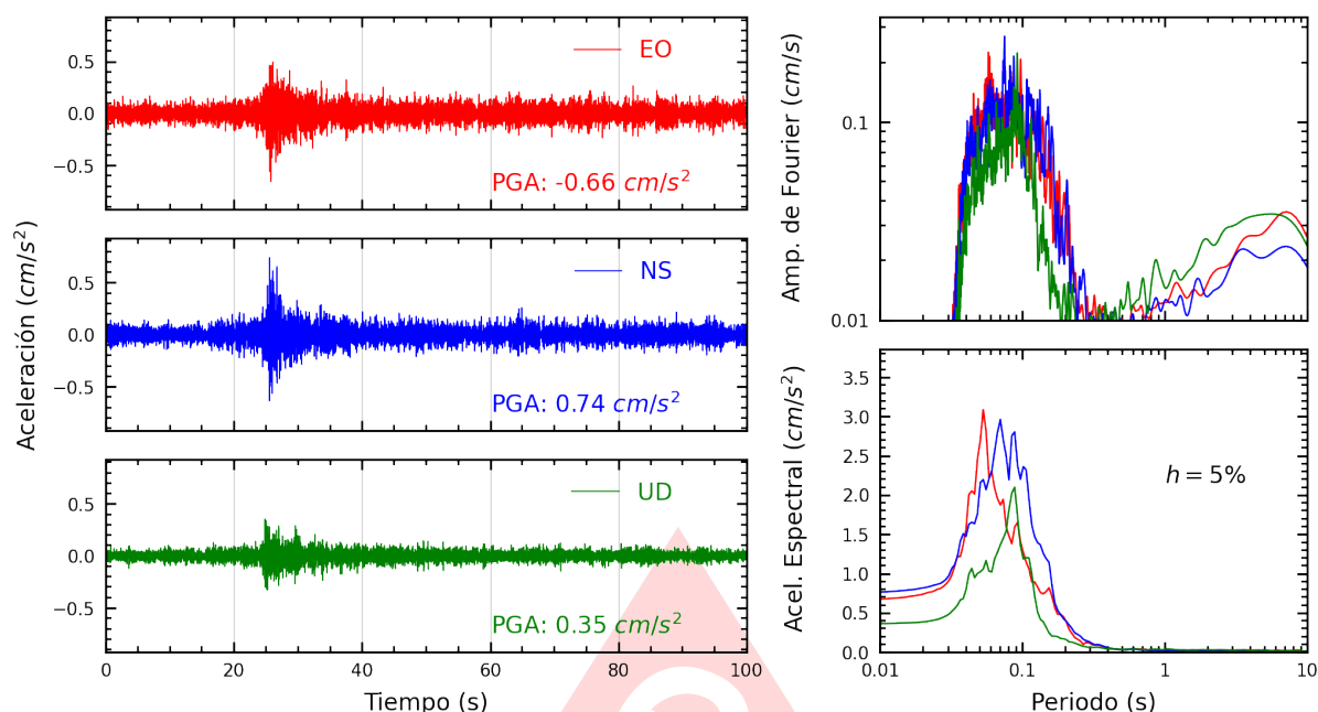
Figura A.5: Registros tiempo-historia, espectros de Fourier y de respuesta en las direcciones EO, NS y vertical de la estación USILM. Sismo de Ancon, Lima - Lima del 2025-06-25, 20:16:54 (Hora local)
