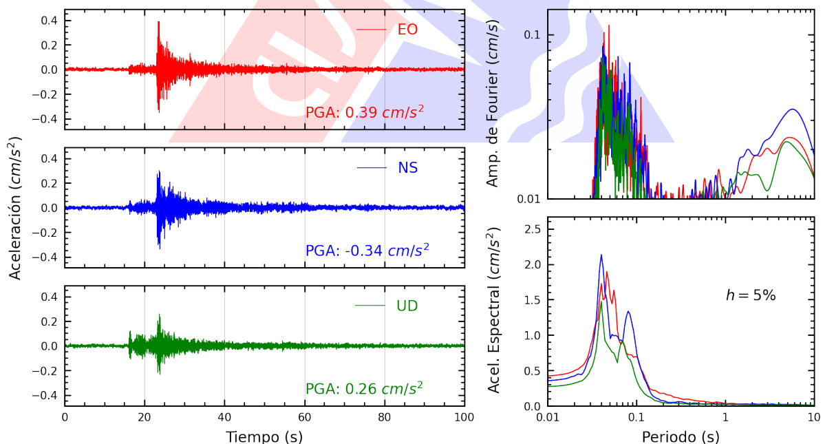
Figura A.16: Registros tiempo-historia, espectros de Fourier y de respuesta en las direcciones EO, NS y vertical de la estación SJLCE. Sismo de Ancon, Lima - Lima del 2025-06-25, 20:16:54 (Hora local)
