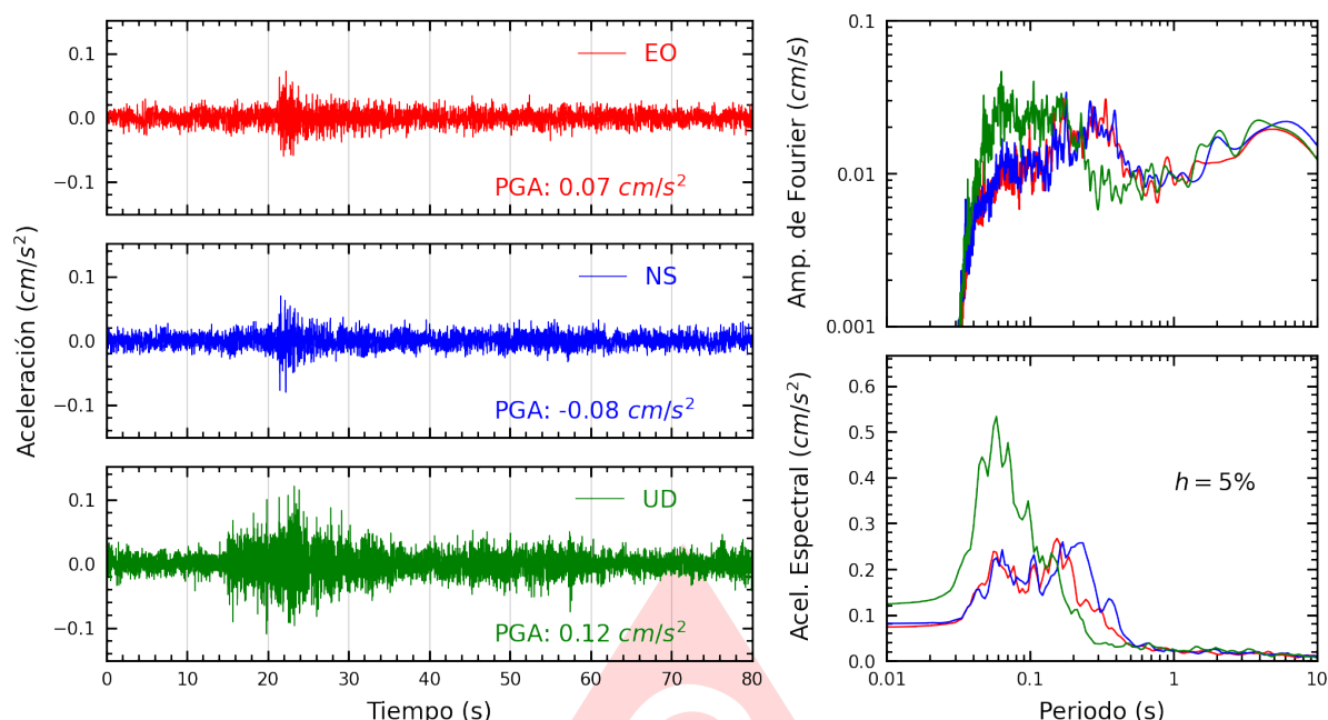
Figura A.29: Registros tiempo-historia, espectros de Fourier y de respuesta en las direcciones EO, NS y vertical de la estación ACAPU. Sismo de Ancon, Lima - Lima del 2025-06-25, 20:16:54 (Hora local)
