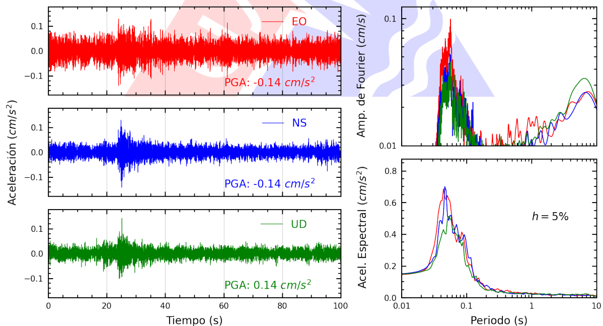
Figura A.26: Registros tiempo-historia, espectros de Fourier y de respuesta en las direcciones EO, NS y vertical de la estación INICT. Sismo de Ancon, Lima - Lima del 2025-06-25, 20:16:54 (Hora local)
