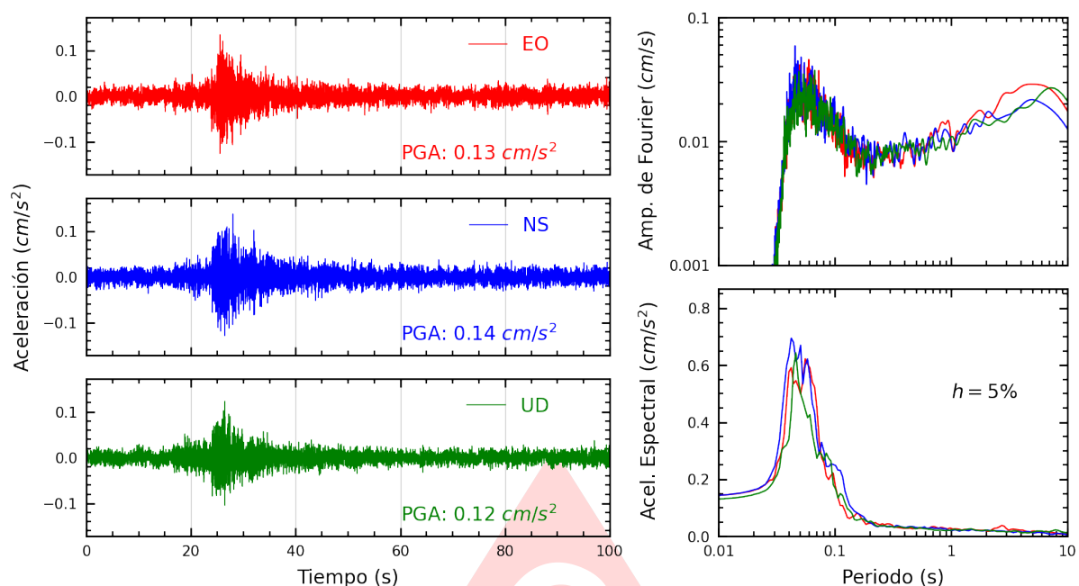
Figura A.27: Registros tiempo-historia, espectros de Fourier y de respuesta en las direcciones EO, NS y vertical de la estación SERVI. Sismo de Ancon, Lima - Lima del 2025-06-25, 20:16:54 (Hora local)
