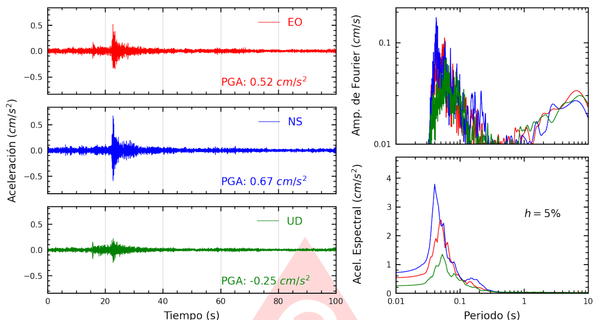
Figura A.7: Registros tiempo-historia, espectros de Fourier y de respuesta en las direcciones EO, NS y vertical de la estación COMAS. Sismo de Ancon, Lima - Lima del 2025-06-25, 20:16:54 (Hora local)
