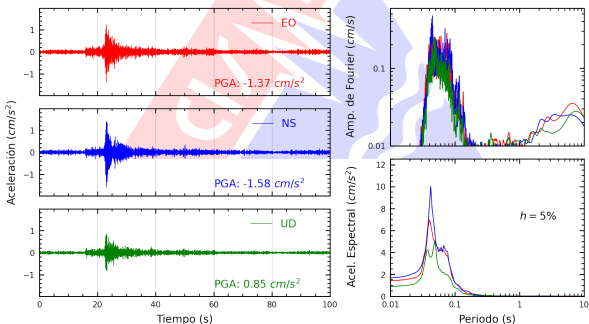
Figura A.2: Registros tiempo-historia, espectros de Fourier y de respuesta en las direcciones EO, NS y vertical de la estación JOSEO. Sismo de Ancon, Lima - Lima del 2025-06-25, 20:16:54 (Hora local)
