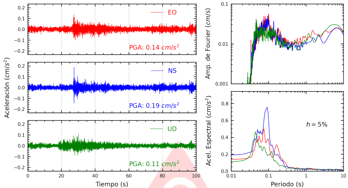
Figura A.23: Registros tiempo-historia, espectros de Fourier y de respuesta en las direcciones EO, NS y vertical de la estación USILP. Sismo de Ancon, Lima - Lima del 2025-06-25, 20:16:54 (Hora local)
