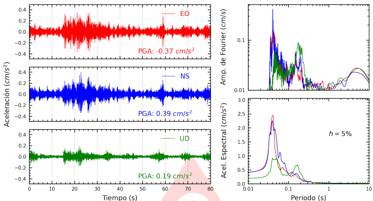
Figura A.15: Registros tiempo-historia, espectros de Fourier y de respuesta en las direcciones EO, NS y vertical de la estación DHNPE. Sismo de Ancon, Lima - Lima del 2025-06-25, 20:16:54 (Hora local)
