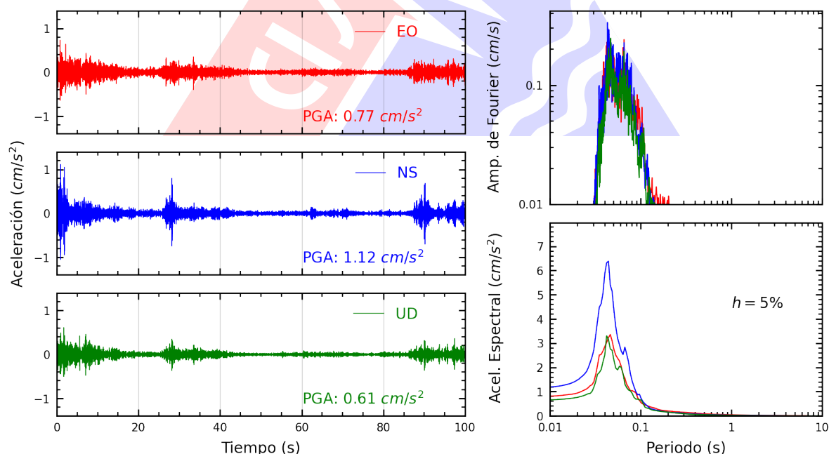
Figura A.4: Registros tiempo-historia, espectros de Fourier y de respuesta en las direcciones EO, NS y vertical de la estación PACHA. Sismo de Ancon, Lima - Lima del 2025-06-25, 20:16:54 (Hora local)
