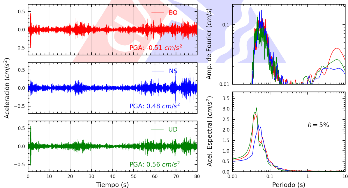
Figura A.10: Registros tiempo-historia, espectros de Fourier y de respuesta en las direcciones EO, NS y vertical de la estación UPCSM. Sismo de Ancon, Lima - Lima del 2025-06-25, 20:16:54 (Hora local)
