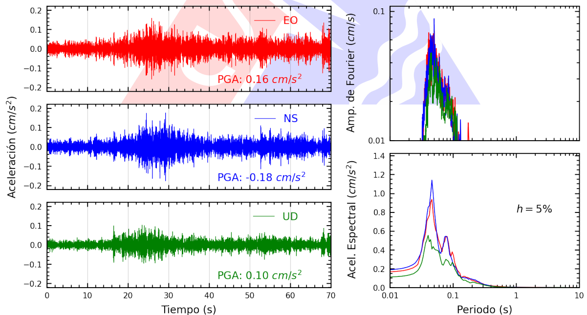
Figura A.24: Registros tiempo-historia, espectros de Fourier y de respuesta en las direcciones EO, NS y vertical de la estación BORJA. Sismo de Ancon, Lima - Lima del 2025-06-25, 20:16:54 (Hora local)
