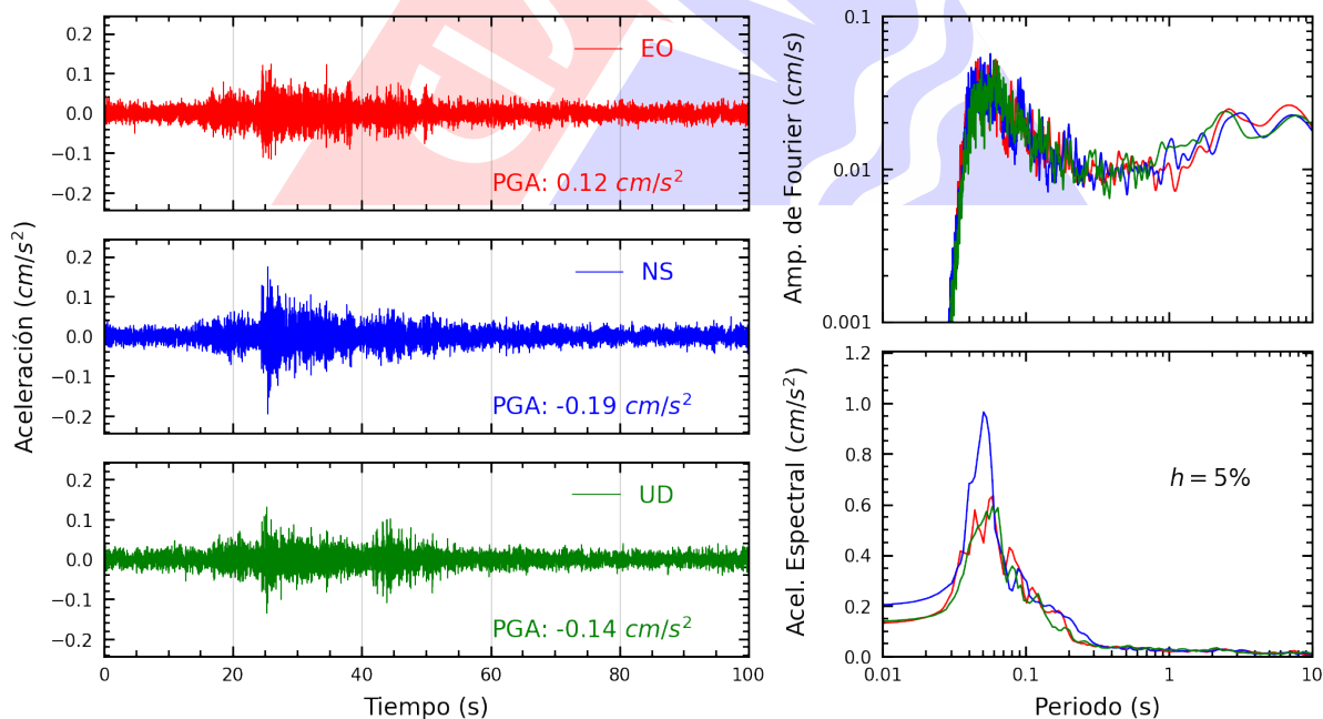
Figura A.22: Registros tiempo-historia, espectros de Fourier y de respuesta en las direcciones EO, NS y vertical de la estación IMCA. Sismo de Ancon, Lima - Lima del 2025-06-25, 20:16:54 (Hora local)
