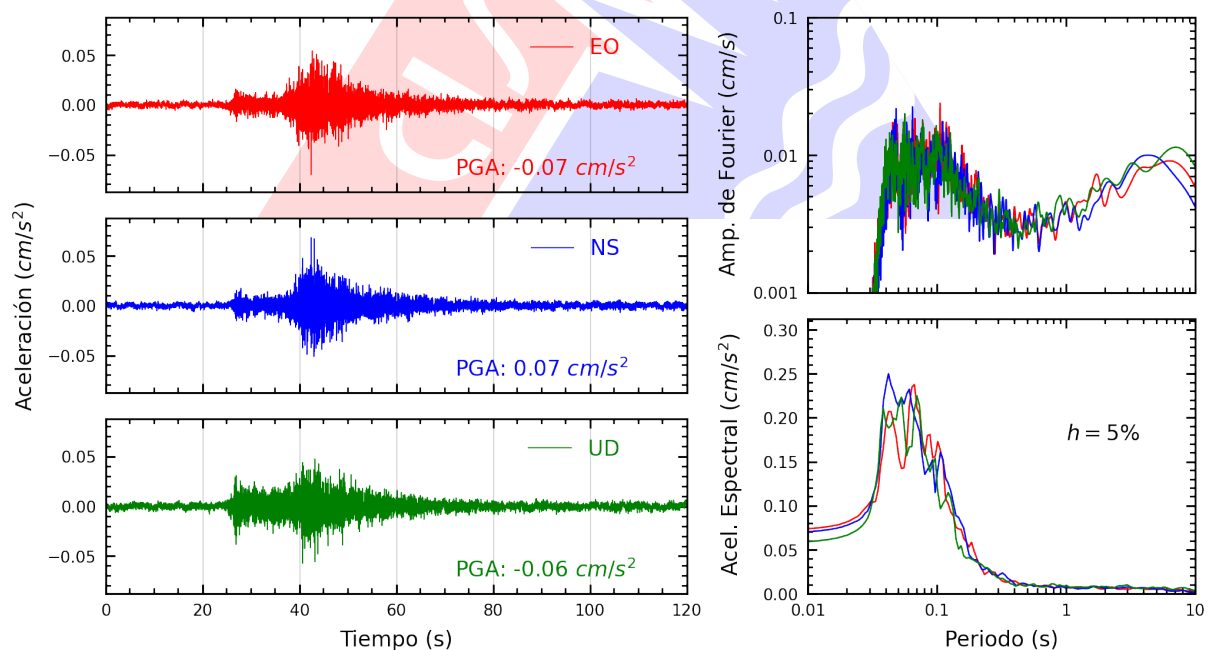
Figura A.32: Registros tiempo-historia, espectros de Fourier y de respuesta en las direcciones EO, NS y vertical de la estación CARAL. Sismo de Ancon, Lima - Lima del 2025-06-25, 20:16:54 (Hora local)
