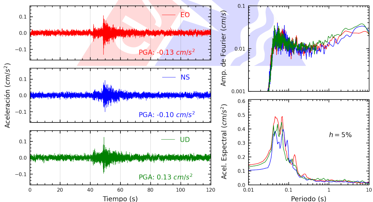
Figura A.28: Registros tiempo-historia, espectros de Fourier y de respuesta en las direcciones EO, NS y vertical de la estación UNMSM. Sismo de Ancon, Lima - Lima del 2025-06-25, 20:16:54 (Hora local)
