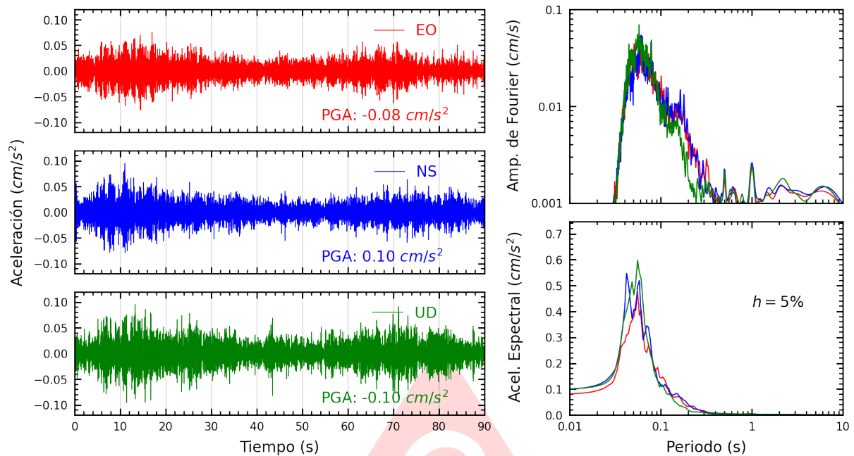
Figura A.31: Registros tiempo-historia, espectros de Fourier y de respuesta en las direcciones EO, NS y vertical de la estación ASIA. Sismo de Ancon, Lima - Lima del 2025-06-25, 20:16:54 (Hora local)
