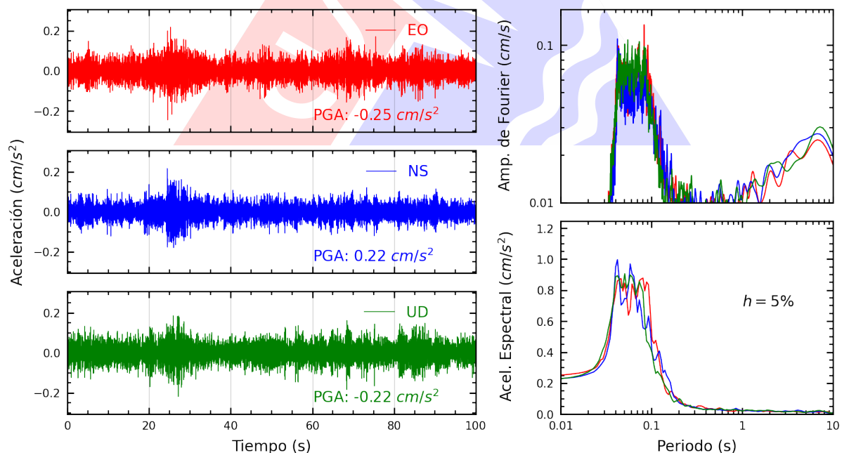
Figura A.20: Registros tiempo-historia, espectros de Fourier y de respuesta en las direcciones EO, NS y vertical de la estación URPPE. Sismo de Ancon, Lima - Lima del 2025-06-25, 20:16:54 (Hora local)
