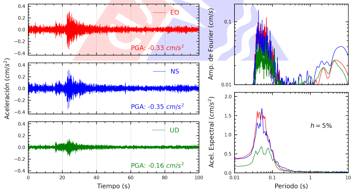
Figura A.18: Registros tiempo-historia, espectros de Fourier y de respuesta en las direcciones EO, NS y vertical de la estación CEPRE. Sismo de Ancon, Lima - Lima del 2025-06-25, 20:16:54 (Hora local)
