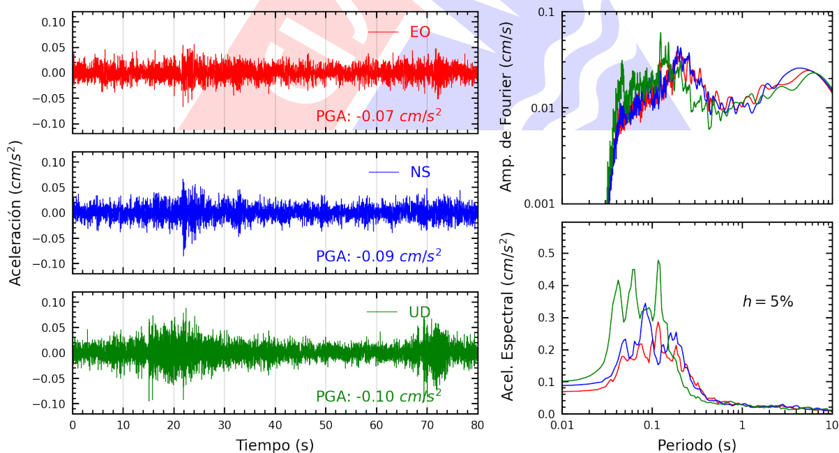
Figura A.30: Registros tiempo-historia, espectros de Fourier y de respuesta en las direcciones EO, NS y vertical de la estación DSMI. Sismo de Ancon, Lima - Lima del 2025-06-25, 20:16:54 (Hora local)
