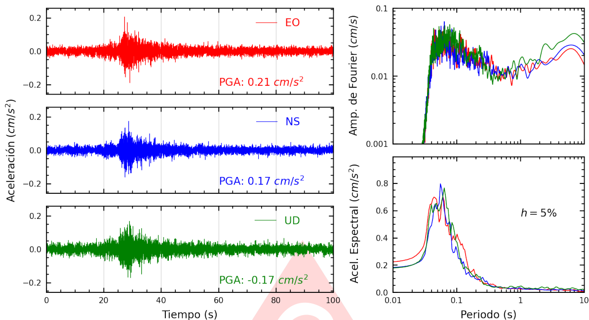
Figura A.21: Registros tiempo-historia, espectros de Fourier y de respuesta en las direcciones EO, NS y vertical de la estación SOVES. Sismo de Ancon, Lima - Lima del 2025-06-25, 20:16:54 (Hora local)
