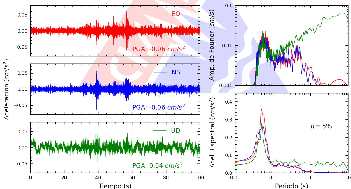
Figura A.2: Registros tiempo-historia, espectros de Fourier y de respuesta en las direcciones EO, NS y vertical de la estación SCARQ. Sismo de Chala, Caraveli - Arequipa del 2025-06-26, 03:33:32 (Hora local)
