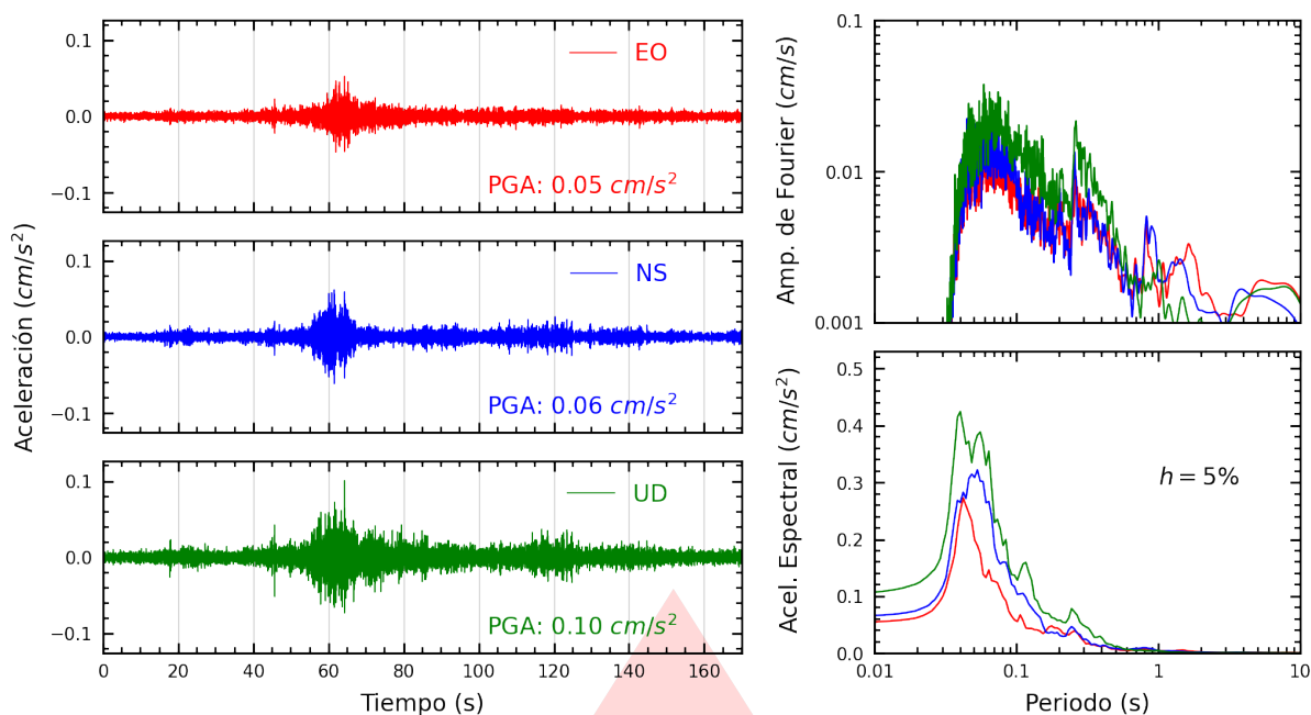
Figura A.1: Registros tiempo-historia, espectros de Fourier y de respuesta en las direcciones EO, NS y vertical de la estación SCCUS. Sismo de Chala, Caraveli - Arequipa del 2025-06-26, 03:33:32 (Hora local)
