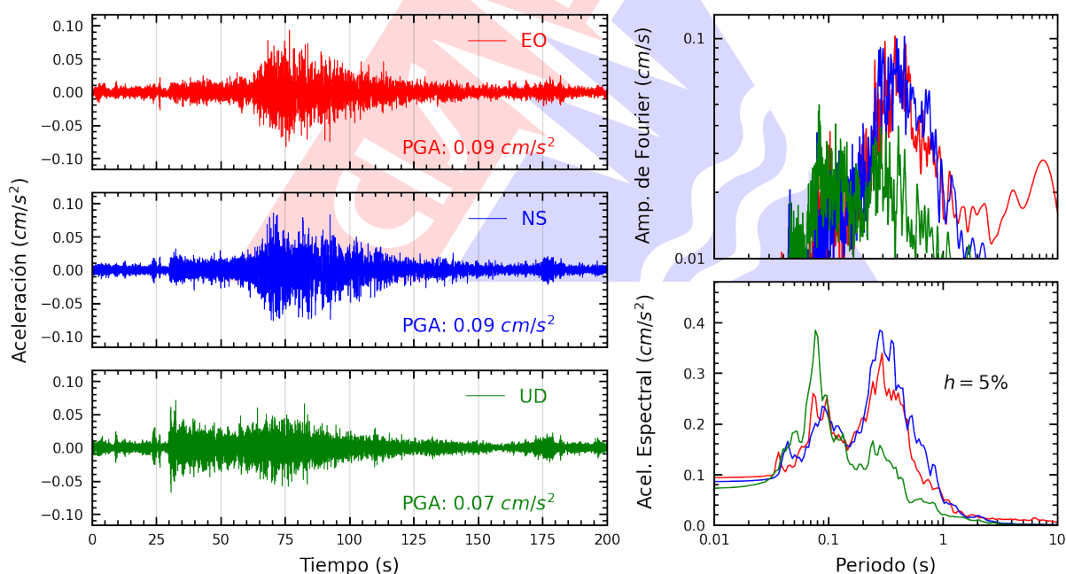
Figura A.2: Registros tiempo-historia, espectros de Fourier y de respuesta en las direcciones EO, NS y vertical de la estación SCPIU. Sismo de Zarumilla, Zarumilla - Tumbes del 2025-06-27, 01:31:53 (Hora local)
