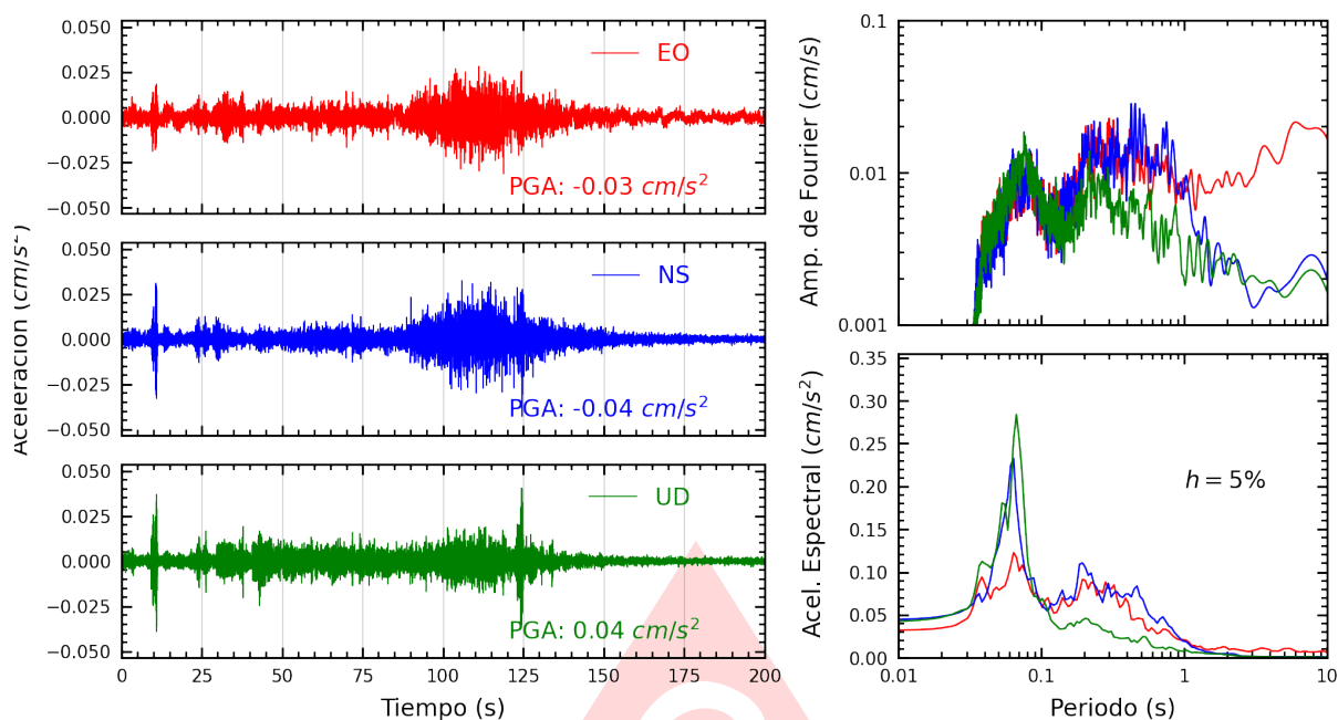
Figura A.5: Registros tiempo-historia, espectros de Fourier y de respuesta en las direcciones EO, NS y vertical de la estación SCCHI. Sismo de Zarumilla, Zarumilla - Tumbes del 2025-06-27, 01:31:53 (Hora local)
