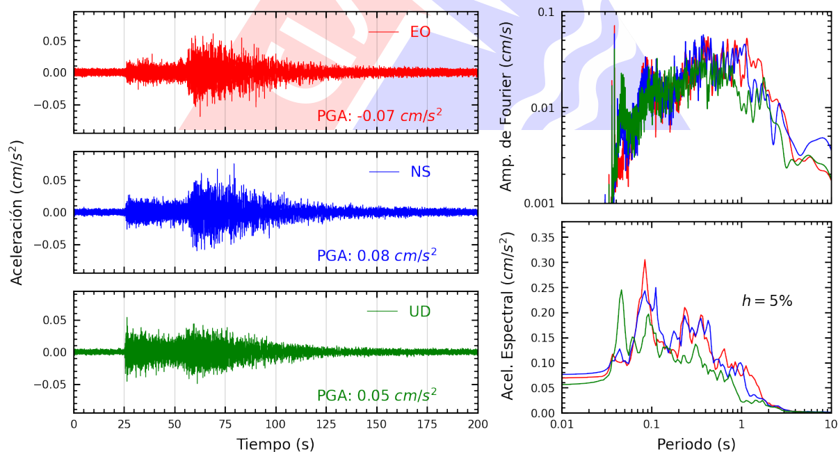
Figura A.4: Registros tiempo-historia, espectros de Fourier y de respuesta en las direcciones EO, NS y vertical de la estación UNF. Sismo de Zarumilla, Zarumilla - Tumbes del 2025-06-27, 01:31:53 (Hora local)
