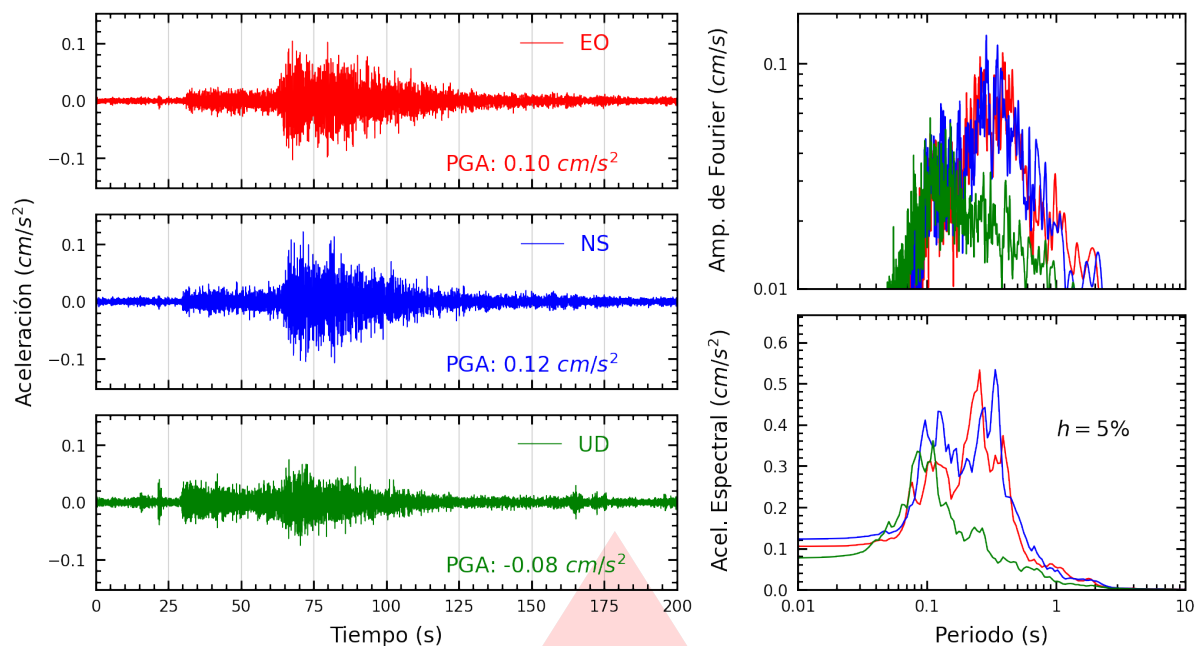
Figura A.1: Registros tiempo-historia, espectros de Fourier y de respuesta en las direcciones EO, NS y vertical de la estación UNP. Sismo de Zarumilla, Zarumilla - Tumbes del 2025-06-27, 01:31:53 (Hora local)
