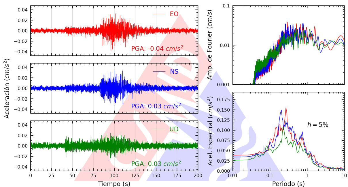
Figura A.7: Registros tiempo-historia, espectros de Fourier y de respuesta en las direcciones EO, NS y vertical de la estación UNJ. Sismo de Zarumilla, Zarumilla - Tumbes del 2025-06-27, 01:31:53 (Hora local)
