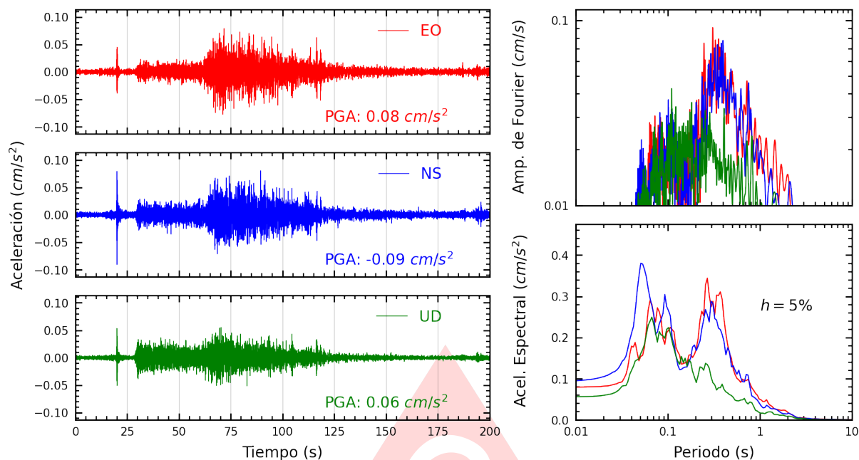
Figura A.3: Registros tiempo-historia, espectros de Fourier y de respuesta en las direcciones EO, NS y vertical de la estación UPAOP. Sismo de Zarumilla, Zarumilla - Tumbes del 2025-06-27, 01:31:53 (Hora local)
