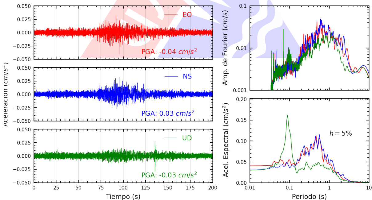
Figura A.6: Registros tiempo-historia, espectros de Fourier y de respuesta en las direcciones EO, NS y vertical de la estación UNC. Sismo de Zarumilla, Zarumilla - Tumbes del 2025-06-27, 01:31:53 (Hora local)
