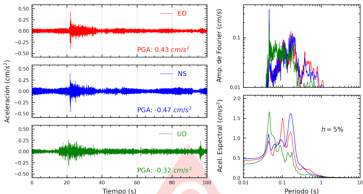
Figura A.3: Registros tiempo-historia, espectros de Fourier y de respuesta en las direcciones EO, NS y vertical de la estación UNP. Sismo de Sullana, Sullana - Piura del 2025-06-27, 12:11:26 (Hora local)
