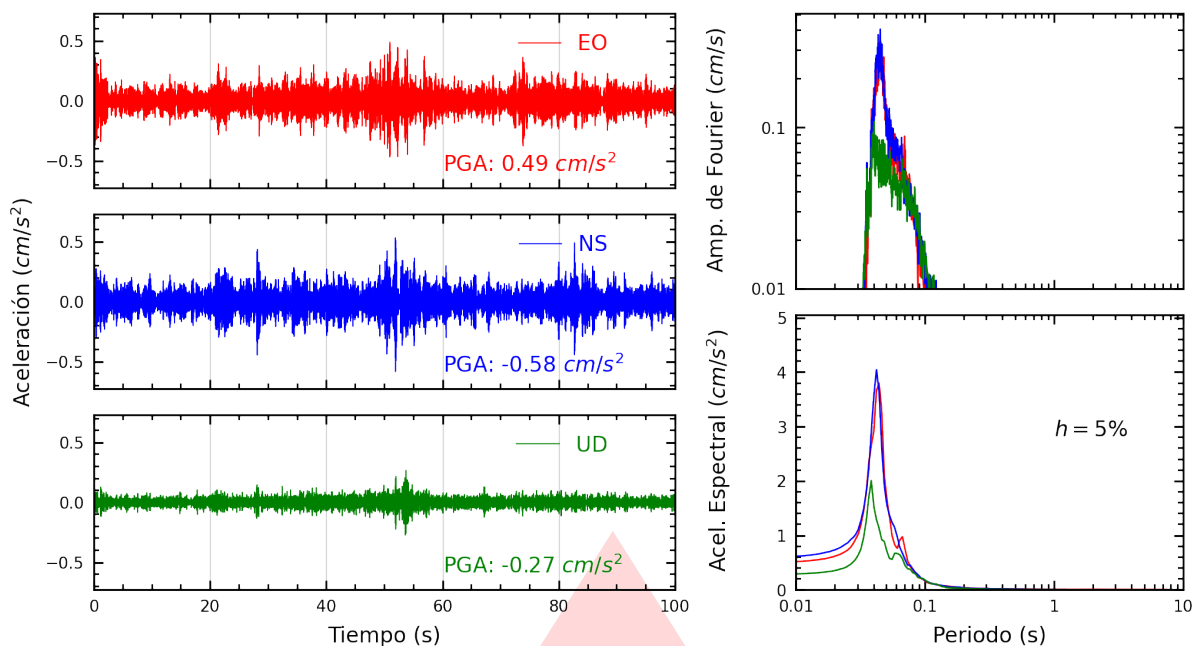
Figura A.1: Registros tiempo-historia, espectros de Fourier y de respuesta en las direcciones EO, NS y vertical de la estación SCTR. Sismo de Sullana, Sullana - Piura del 2025-06-27, 12:11:26 (Hora local)
