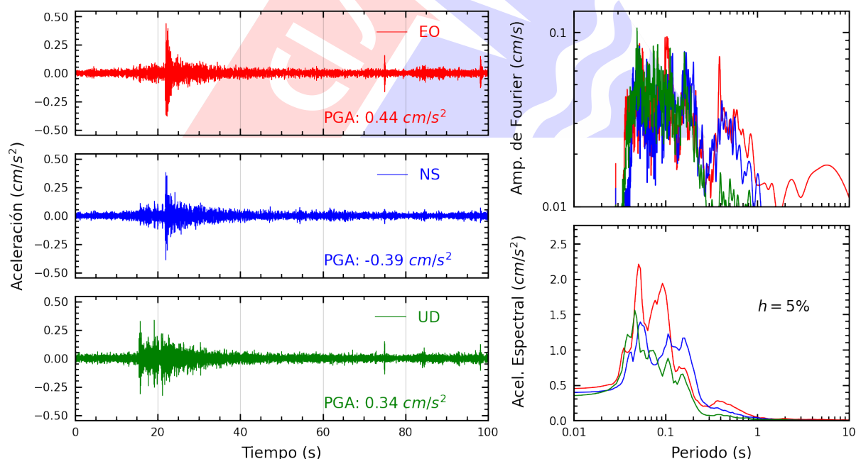
Figura A.4: Registros tiempo-historia, espectros de Fourier y de respuesta en las direcciones EO, NS y vertical de la estación SCPIU. Sismo de Sullana, Sullana - Piura del 2025-06-27, 12:11:26 (Hora local)
