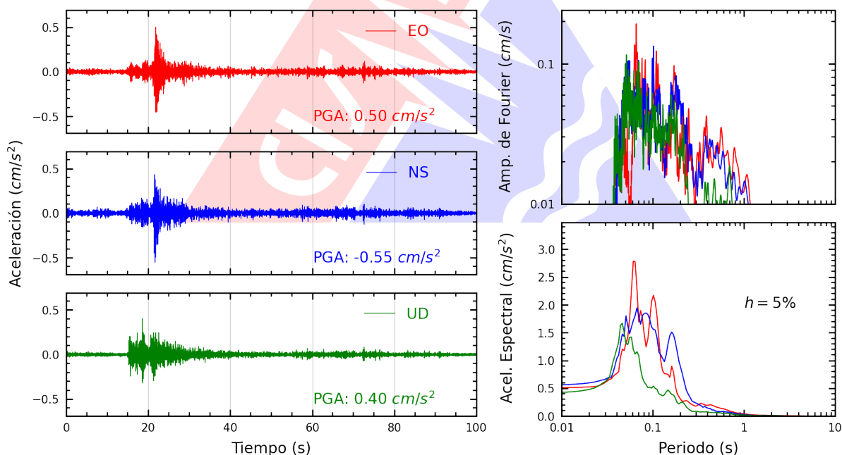
Figura A.2: Registros tiempo-historia, espectros de Fourier y de respuesta en las direcciones EO, NS y vertical de la estación UPAOP. Sismo de Sullana, Sullana - Piura del 2025-06-27, 12:11:26 (Hora local)
