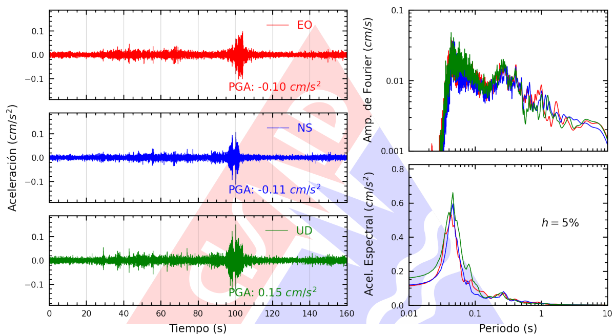
Figura A.5: Registros tiempo-historia, espectros de Fourier y de respuesta en las direcciones EO, NS y vertical de la estación UNC. Sismo de Sullana, Sullana - Piura del 2025-06-27, 12:11:26 (Hora local)
