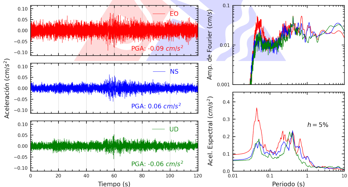
Figura A.26: Registros tiempo-historia, espectros de Fourier y de respuesta en las direcciones EO, NS y vertical de la estación INICT. Sismo de San Miguel, La Mar - Ayacucho del 2025-06-30, 03:44:06 (Hora local)
