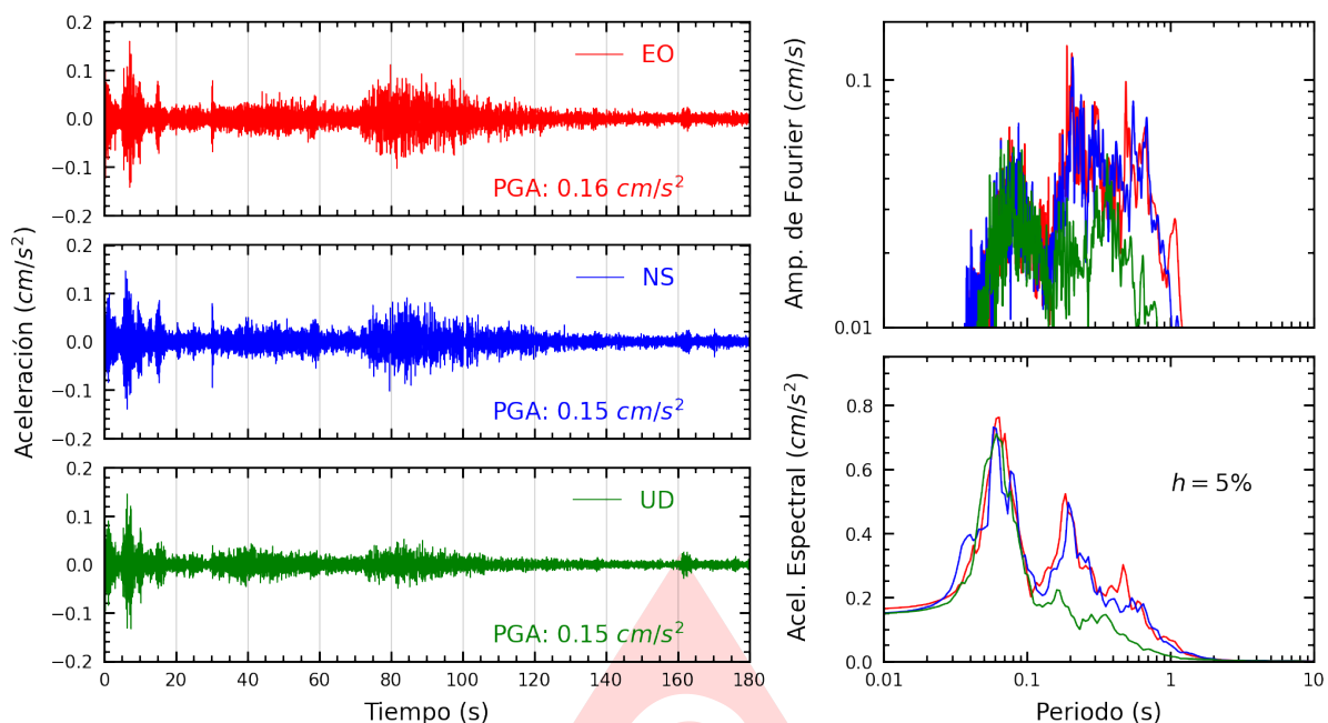
Figura A.15: Registros tiempo-historia, espectros de Fourier y de respuesta en las direcciones EO, NS y vertical de la estación SCCHO. Sismo de San Miguel, La Mar - Ayacucho del 2025-06-30, 03:44:06 (Hora local)
