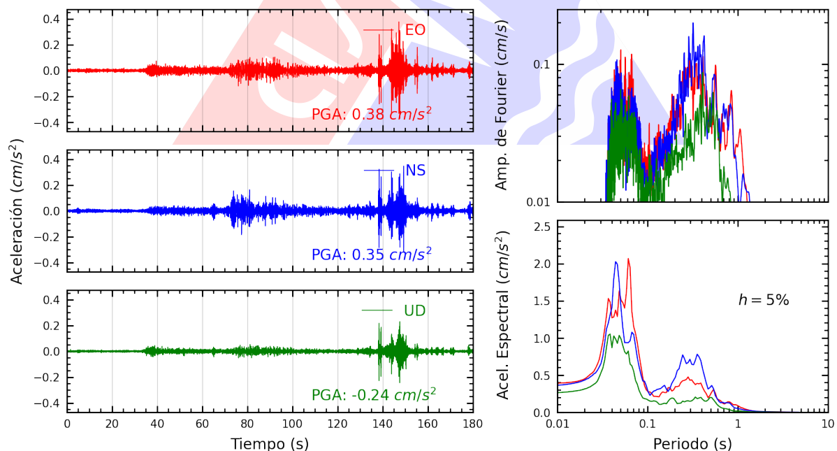
Figura A.4: Registros tiempo-historia, espectros de Fourier y de respuesta en las direcciones EO, NS y vertical de la estación BRIS2. Sismo de San Miguel, La Mar - Ayacucho del 2025-06-30, 03:44:06 (Hora local)
