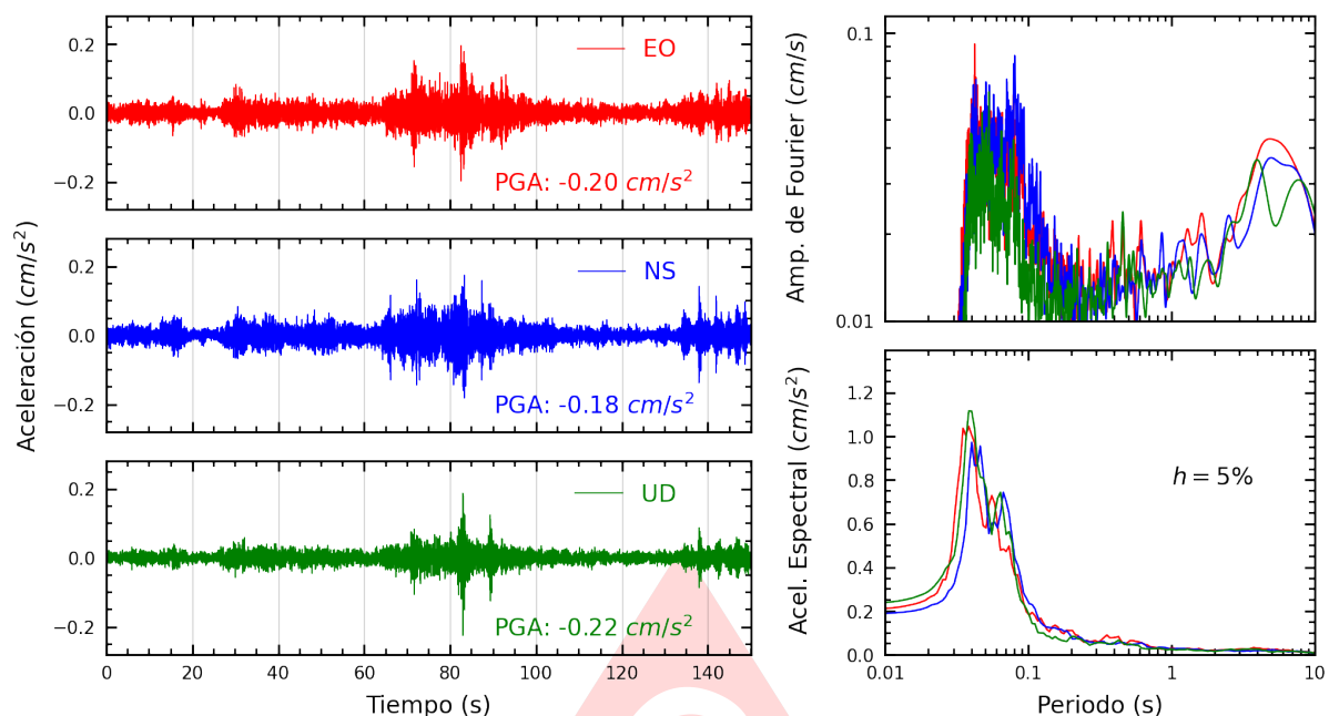
Figura A.9: Registros tiempo-historia, espectros de Fourier y de respuesta en las direcciones EO, NS y vertical de la estación JOSEO. Sismo de San Miguel, La Mar - Ayacucho del 2025-06-30, 03:44:06 (Hora local)
