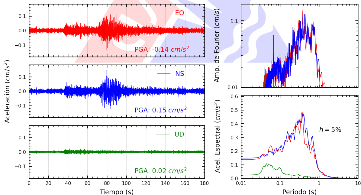
Figura A.18: Registros tiempo-historia, espectros de Fourier y de respuesta en las direcciones EO, NS y vertical de la estación UCVAT. Sismo de San Miguel, La Mar - Ayacucho del 2025-06-30, 03:44:06 (Hora local)
