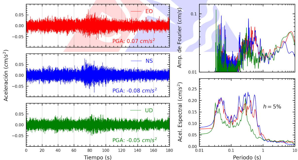
Figura A.28: Registros tiempo-historia, espectros de Fourier y de respuesta en las direcciones EO, NS y vertical de la estación UPCVI. Sismo de San Miguel, La Mar - Ayacucho del 2025-06-30, 03:44:06 (Hora local)
