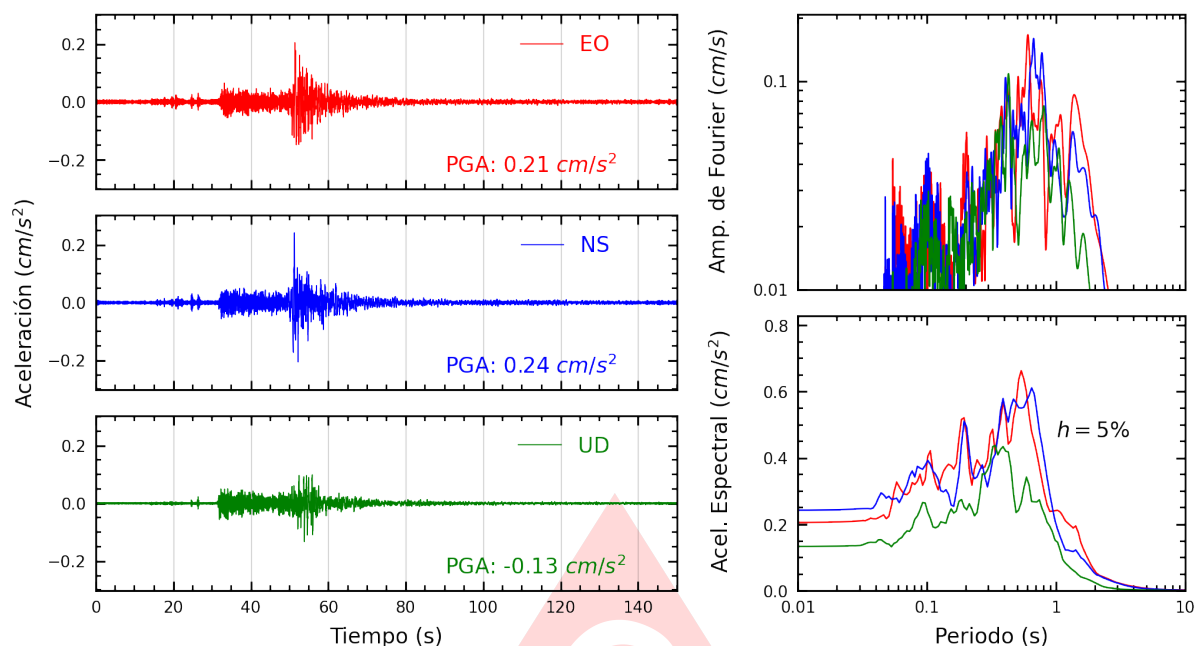
Figura A.7: Registros tiempo-historia, espectros de Fourier y de respuesta en las direcciones EO, NS y vertical de la estación UNMBA. Sismo de San Miguel, La Mar - Ayacucho del 2025-06-30, 03:44:06 (Hora local)
