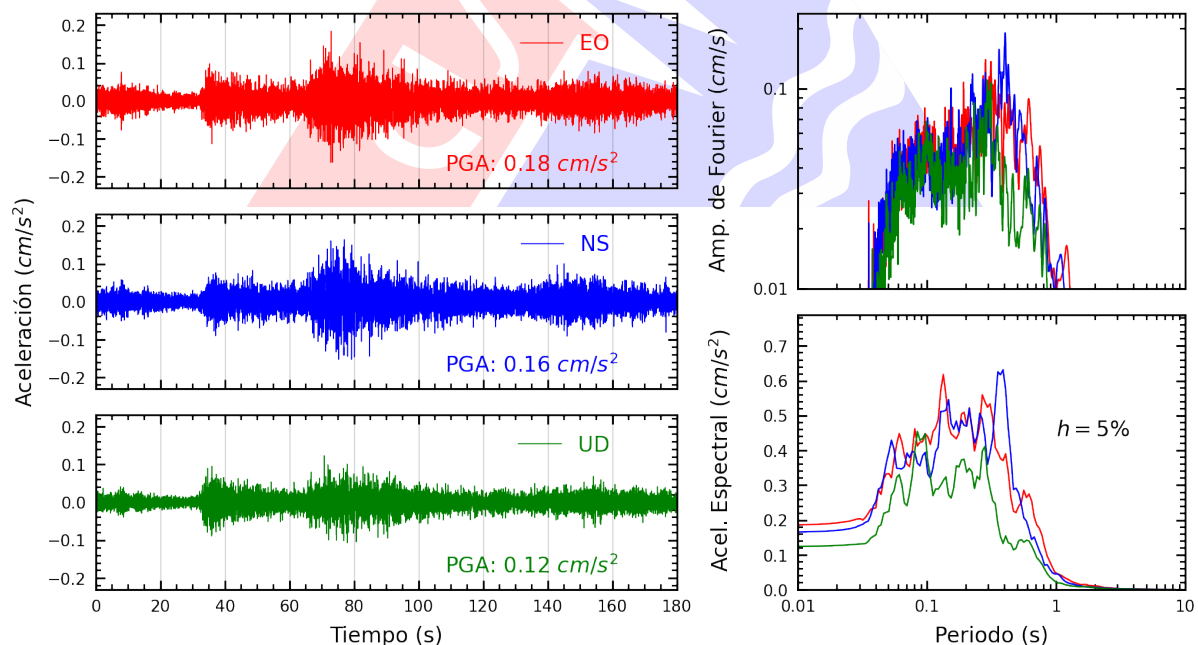
Figura A.12: Registros tiempo-historia, espectros de Fourier y de respuesta en las direcciones EO, NS y vertical de la estación PHERM. Sismo de San Miguel, La Mar - Ayacucho del 2025-06-30, 03:44:06 (Hora local)
