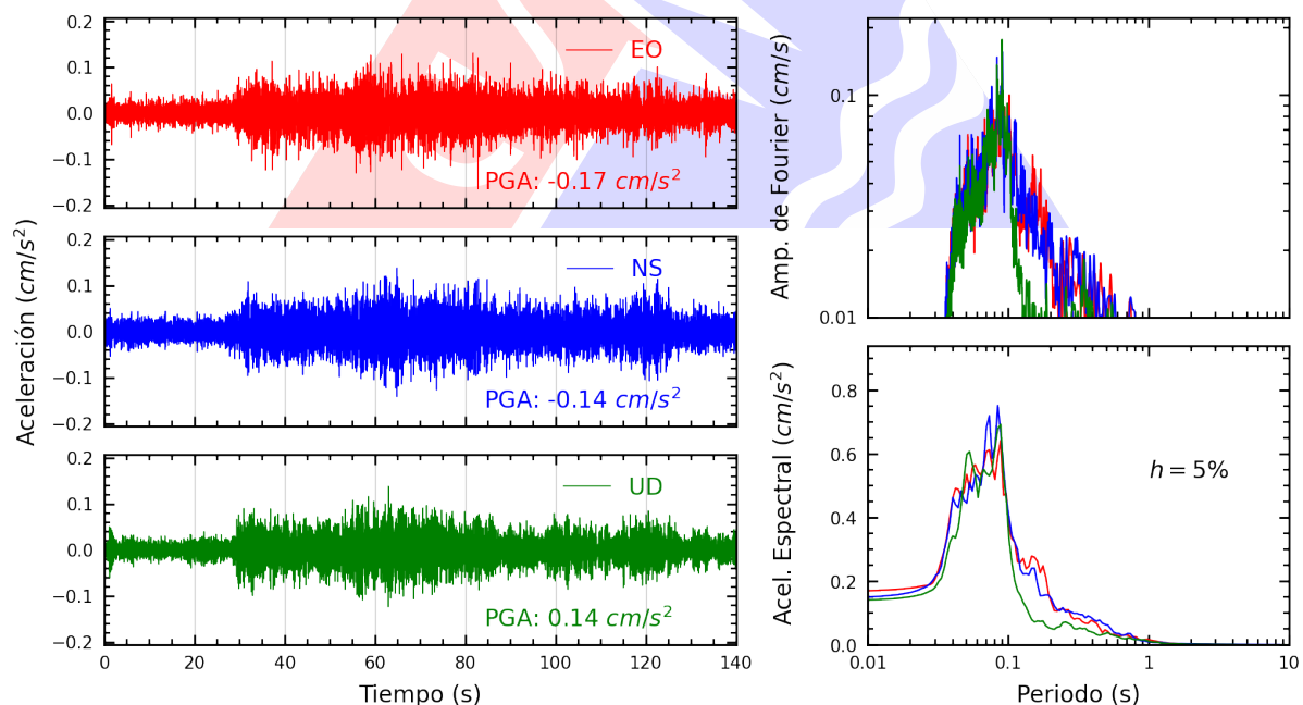
Figura A.14: Registros tiempo-historia, espectros de Fourier y de respuesta en las direcciones EO, NS y vertical de la estación SROSA. Sismo de San Miguel, La Mar - Ayacucho del 2025-06-30, 03:44:06 (Hora local)
