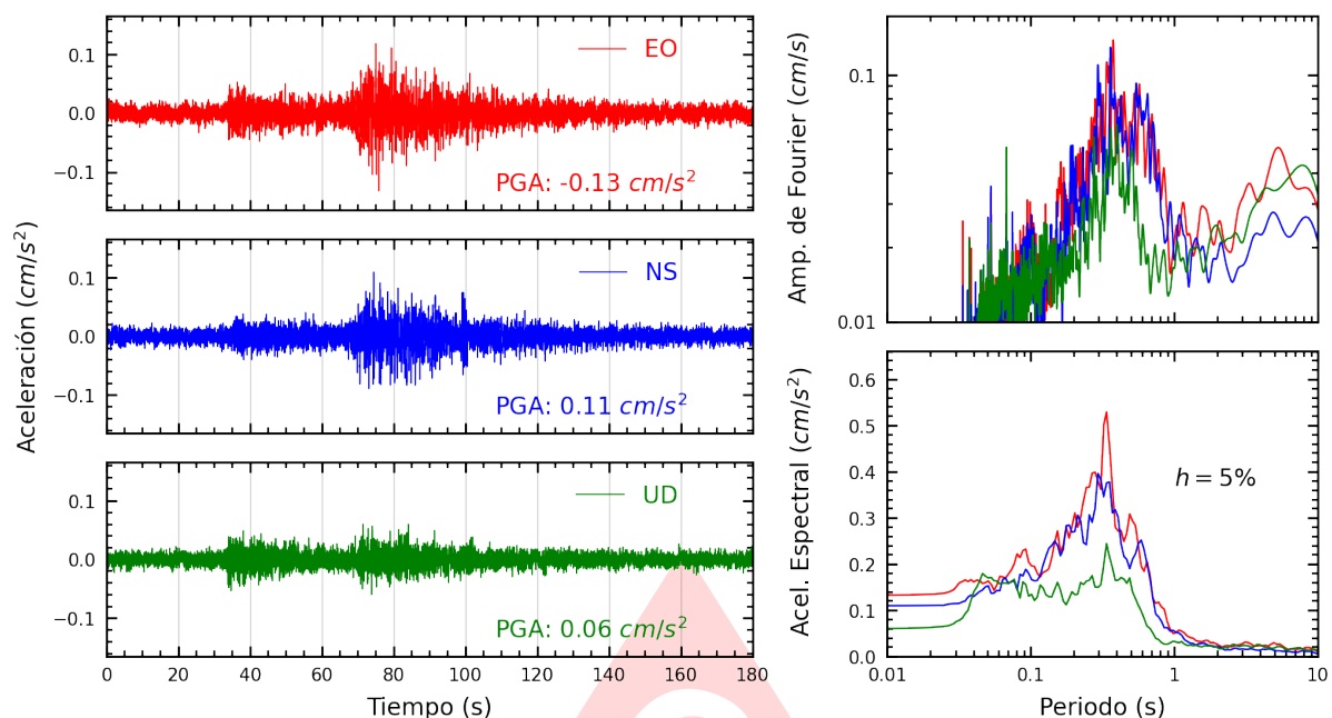
Figura A.19: Registros tiempo-historia, espectros de Fourier y de respuesta en las direcciones EO, NS y vertical de la estación USILP. Sismo de San Miguel, La Mar - Ayacucho del 2025-06-30, 03:44:06 (Hora local)
