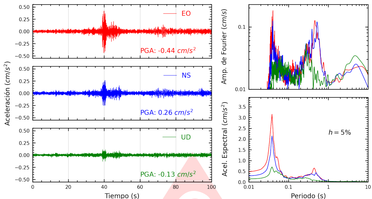
Figura A.3: Registros tiempo-historia, espectros de Fourier y de respuesta en las direcciones EO, NS y vertical de la estación OLIVO. Sismo de San Miguel, La Mar - Ayacucho del 2025-06-30, 03:44:06 (Hora local)
