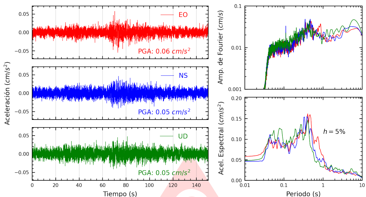
Figura A.39: Registros tiempo-historia, espectros de Fourier y de respuesta en las direcciones EO, NS y vertical de la estación UNFV. Sismo de San Miguel, La Mar - Ayacucho del 2025-06-30, 03:44:06 (Hora local)
