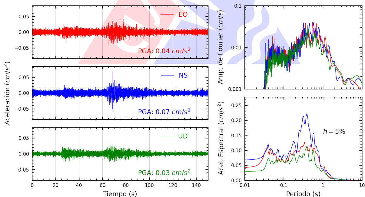
Figura A.34: Registros tiempo-historia, espectros de Fourier y de respuesta en las direcciones EO, NS y vertical de la estación BORJA. Sismo de San Miguel, La Mar - Ayacucho del 2025-06-30, 03:44:06 (Hora local)
