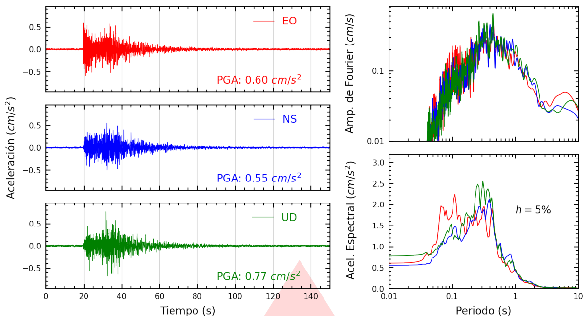
Figura A.1: Registros tiempo-historia, espectros de Fourier y de respuesta en las direcciones EO, NS y vertical de la estación UNSCH. Sismo de San Miguel, La Mar - Ayacucho del 2025-06-30, 03:44:06 (Hora local)
