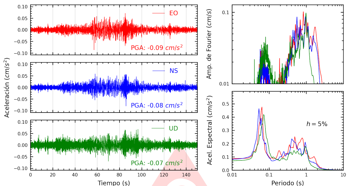
Figura A.27: Registros tiempo-historia, espectros de Fourier y de respuesta en las direcciones EO, NS y vertical de la estación SCCUS. Sismo de San Miguel, La Mar - Ayacucho del 2025-06-30, 03:44:06 (Hora local)
