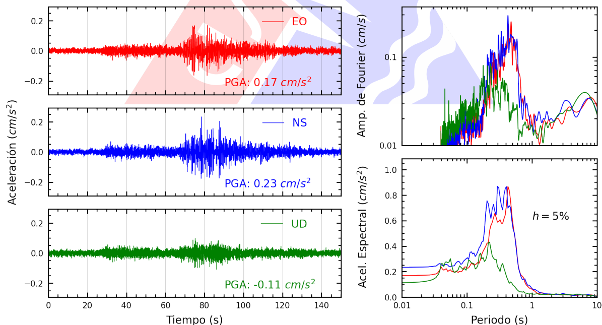
Figura A.8: Registros tiempo-historia, espectros de Fourier y de respuesta en las direcciones EO, NS y vertical de la estación MDPP. Sismo de San Miguel, La Mar - Ayacucho del 2025-06-30, 03:44:06 (Hora local)
