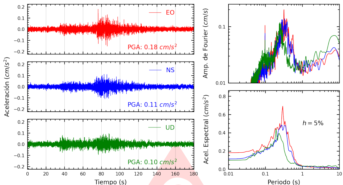
Figura A.13: Registros tiempo-historia, espectros de Fourier y de respuesta en las direcciones EO, NS y vertical de la estación SOVES. Sismo de San Miguel, La Mar - Ayacucho del 2025-06-30, 03:44:06 (Hora local)
