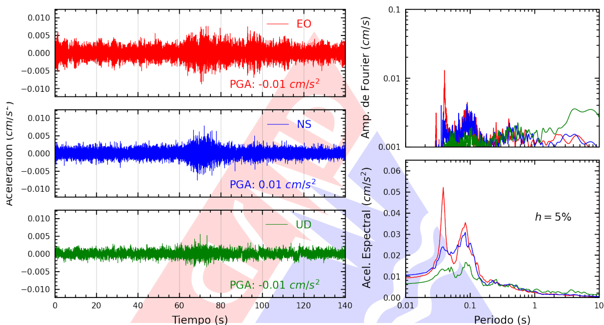
Figura A.41: Registros tiempo-historia, espectros de Fourier y de respuesta en las direcciones EO, NS y vertical de la estación UNAM. Sismo de San Miguel, La Mar - Ayacucho del 2025-06-30, 03:44:06 (Hora local)
