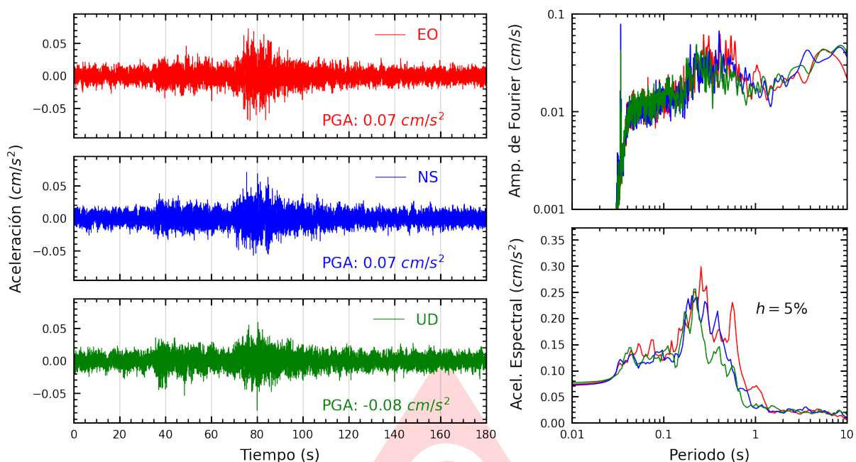
Figura A.29: Registros tiempo-historia, espectros de Fourier y de respuesta en las direcciones EO, NS y vertical de la estación USMP. Sismo de San Miguel, La Mar - Ayacucho del 2025-06-30, 03:44:06 (Hora local)
