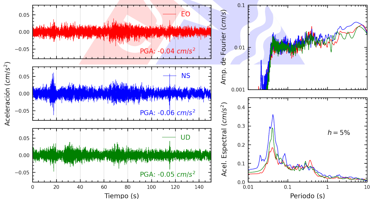
Figura A.36: Registros tiempo-historia, espectros de Fourier y de respuesta en las direcciones EO, NS y vertical de la estación SJLCE. Sismo de San Miguel, La Mar - Ayacucho del 2025-06-30, 03:44:06 (Hora local)
