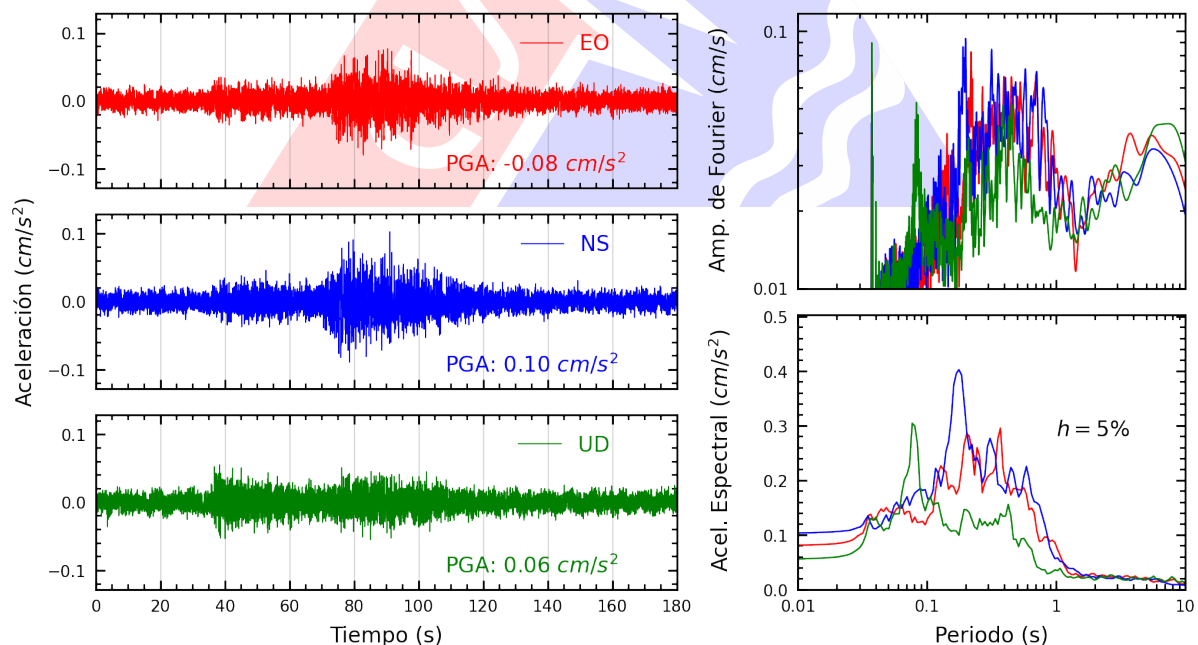
Figura A.22: Registros tiempo-historia, espectros de Fourier y de respuesta en las direcciones EO, NS y vertical de la estación SOCHO. Sismo de San Miguel, La Mar - Ayacucho del 2025-06-30, 03:44:06 (Hora local)
