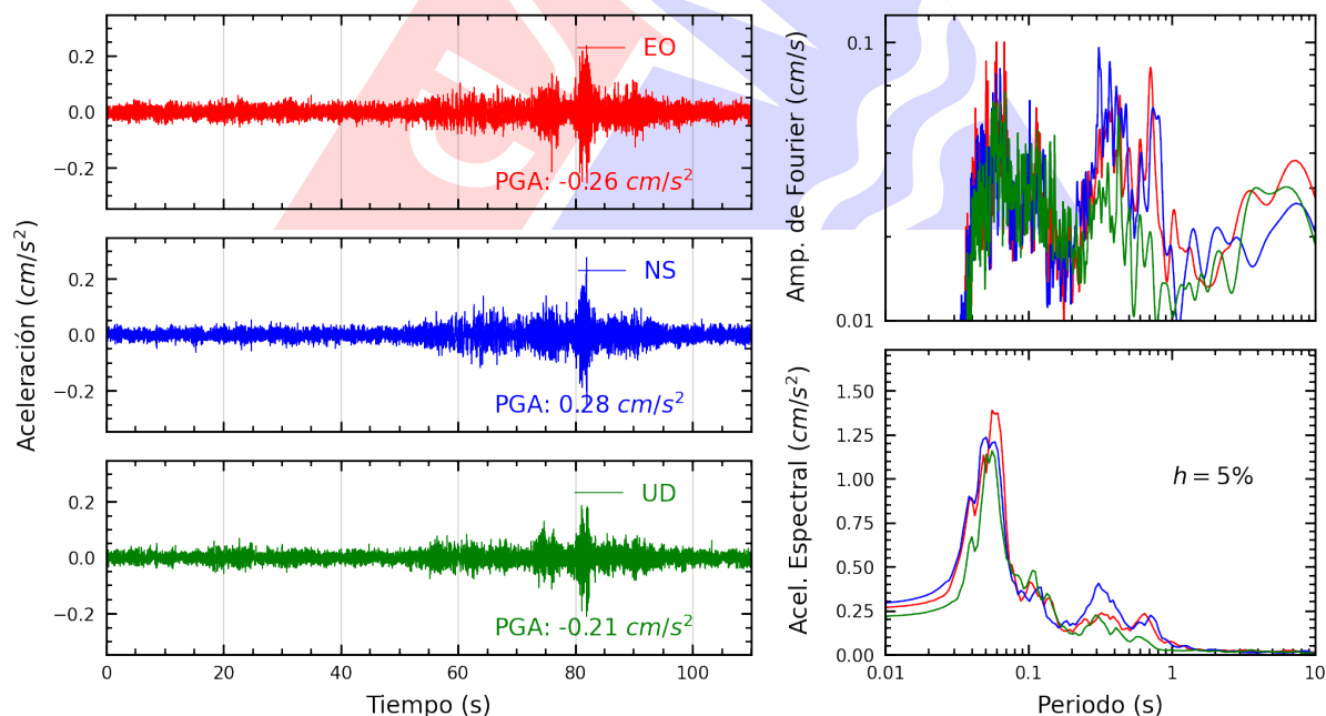
Figura A.6: Registros tiempo-historia, espectros de Fourier y de respuesta en las direcciones EO, NS y vertical de la estación MADRE. Sismo de San Miguel, La Mar - Ayacucho del 2025-06-30, 03:44:06 (Hora local)
