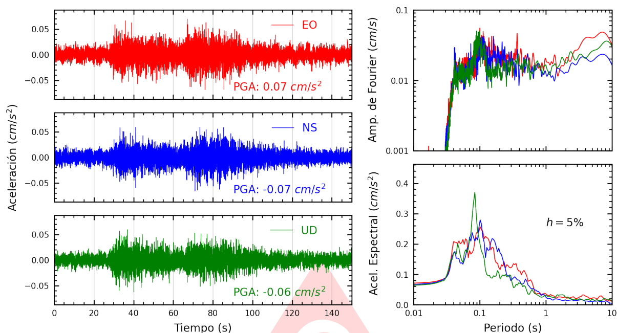
Figura A.33: Registros tiempo-historia, espectros de Fourier y de respuesta en las direcciones EO, NS y vertical de la estación AMORE. Sismo de San Miguel, La Mar - Ayacucho del 2025-06-30, 03:44:06 (Hora local)
