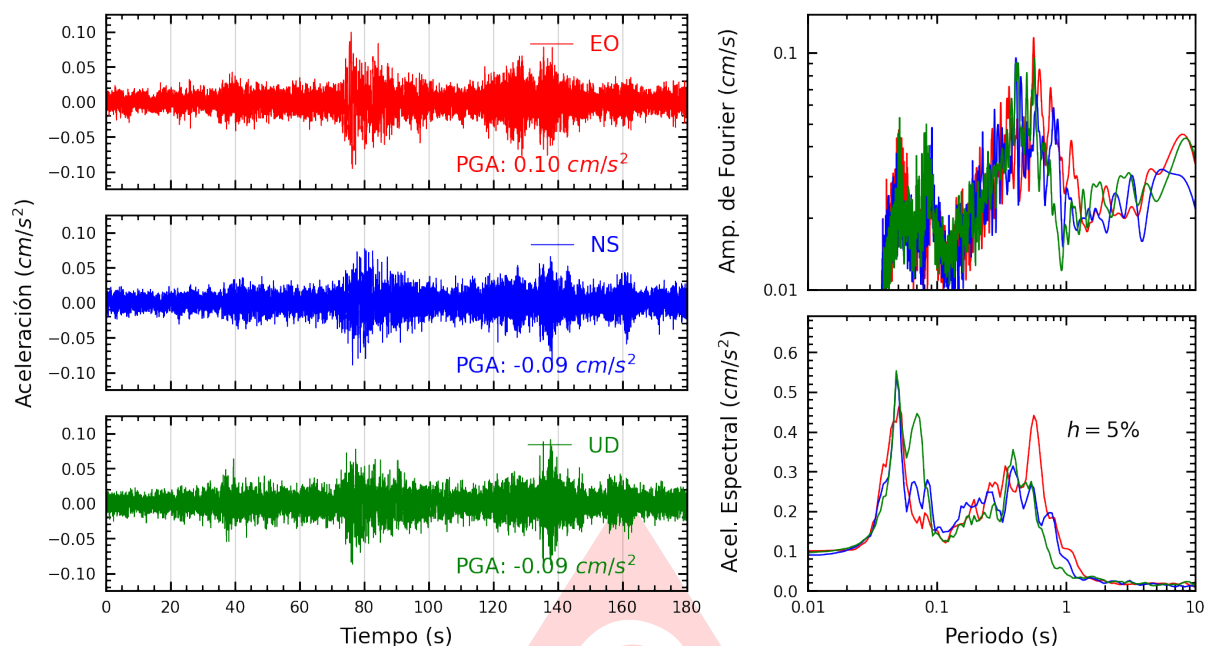
Figura A.25: Registros tiempo-historia, espectros de Fourier y de respuesta en las direcciones EO, NS y vertical de la estación IMCA. Sismo de San Miguel, La Mar - Ayacucho del 2025-06-30, 03:44:06 (Hora local)
