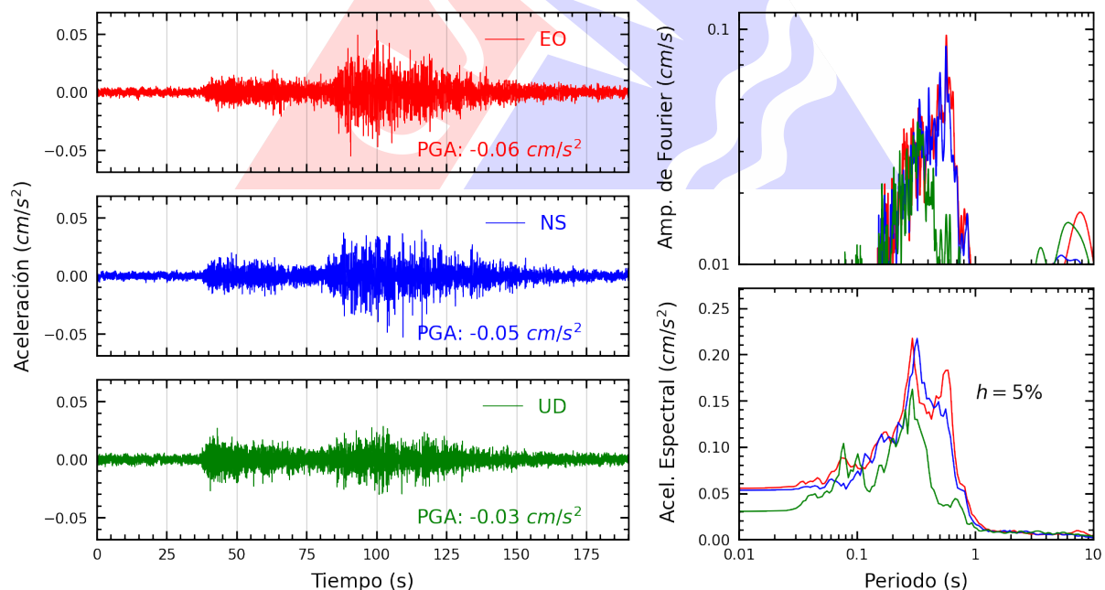
Figura A.40: Registros tiempo-historia, espectros de Fourier y de respuesta en las direcciones EO, NS y vertical de la estación CARAL. Sismo de San Miguel, La Mar - Ayacucho del 2025-06-30, 03:44:06 (Hora local)
