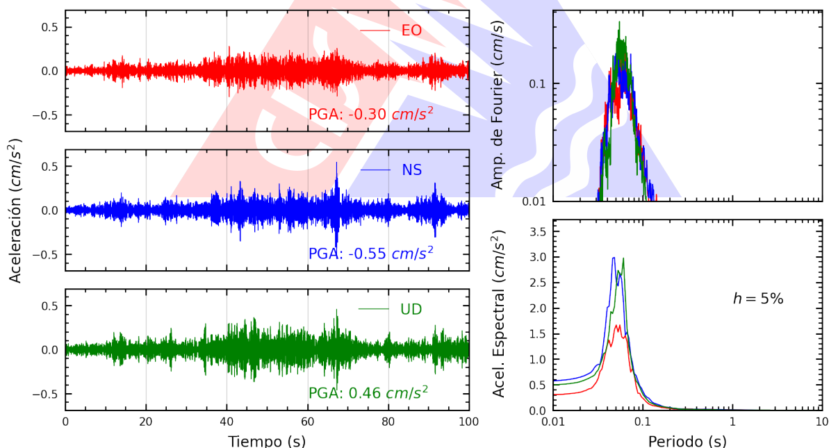
Figura A.2: Registros tiempo-historia, espectros de Fourier y de respuesta en las direcciones EO, NS y vertical de la estación SCAR2. Sismo de San Miguel, La Mar - Ayacucho del 2025-06-30, 03:44:06 (Hora local)
