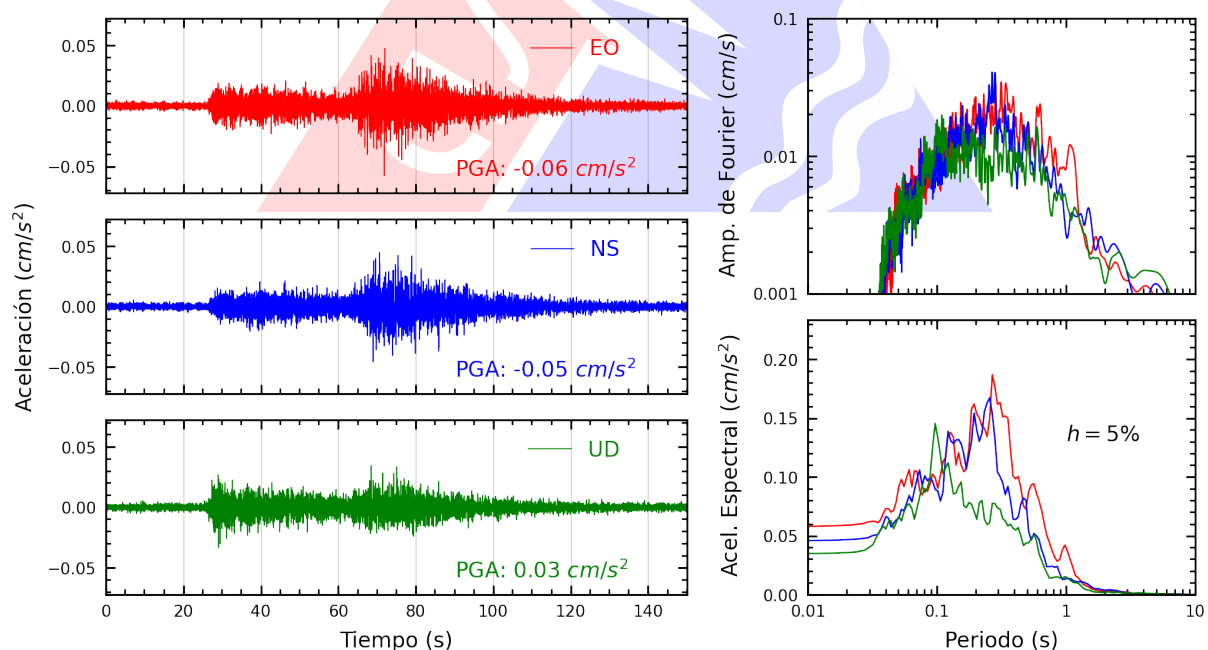
Figura A.38: Registros tiempo-historia, espectros de Fourier y de respuesta en las direcciones EO, NS y vertical de la estación JALV2. Sismo de San Miguel, La Mar - Ayacucho del 2025-06-30, 03:44:06 (Hora local)
