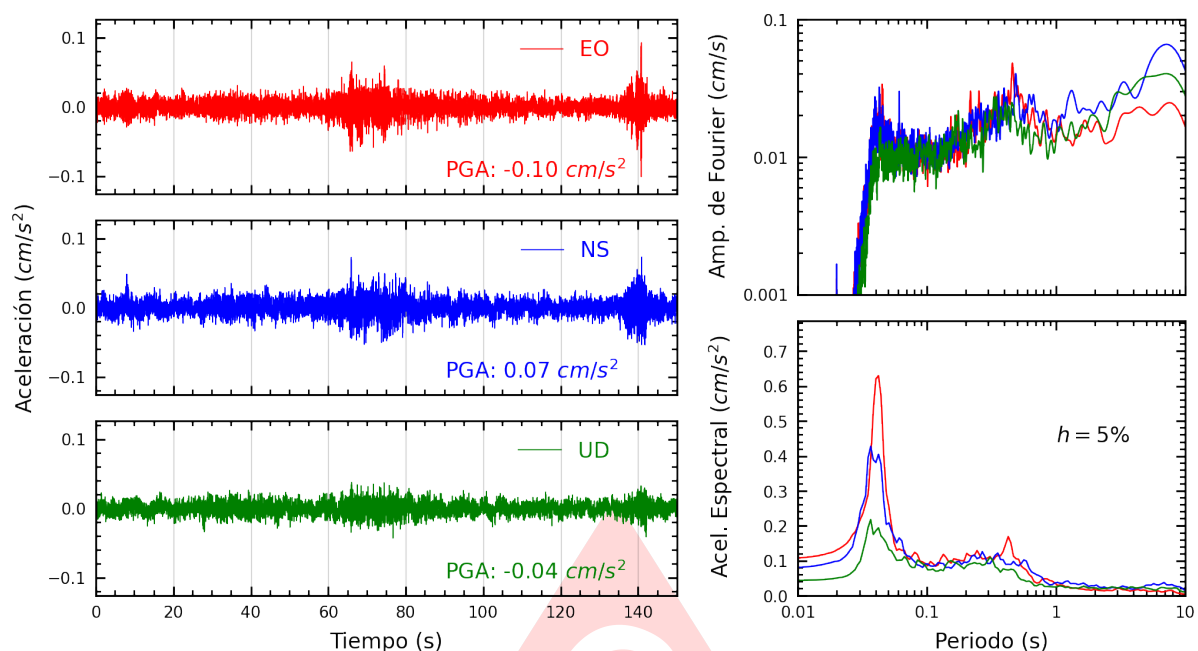
Figura A.23: Registros tiempo-historia, espectros de Fourier y de respuesta en las direcciones EO, NS y vertical de la estación CEPRE. Sismo de San Miguel, La Mar - Ayacucho del 2025-06-30, 03:44:06 (Hora local)
