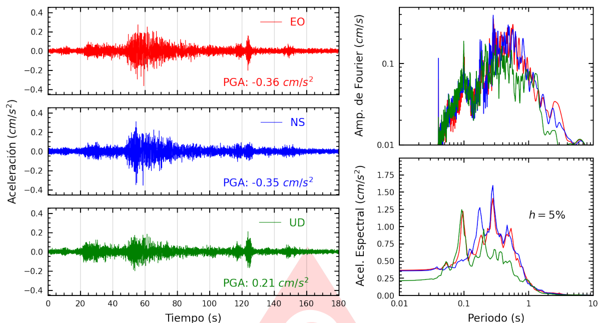
Figura A.5: Registros tiempo-historia, espectros de Fourier y de respuesta en las direcciones EO, NS y vertical de la estación UNICA. Sismo de San Miguel, La Mar - Ayacucho del 2025-06-30, 03:44:06 (Hora local)
