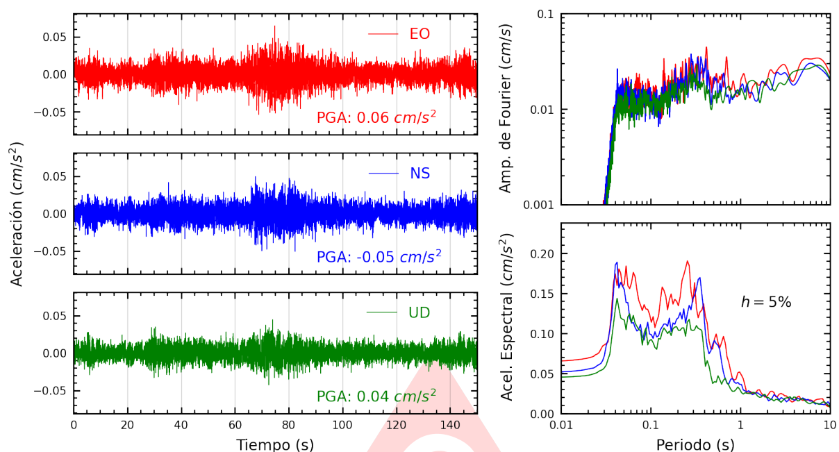
Figura A.35: Registros tiempo-historia, espectros de Fourier y de respuesta en las direcciones EO, NS y vertical de la estación FICPE. Sismo de San Miguel, La Mar - Ayacucho del 2025-06-30, 03:44:06 (Hora local)
