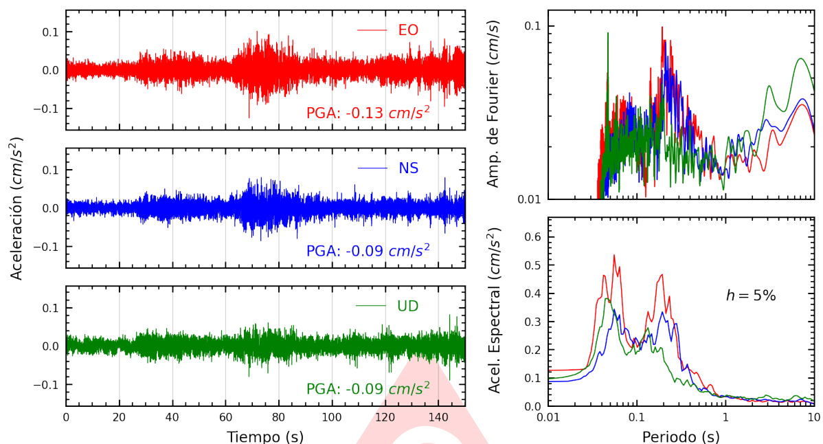
Figura A.21: Registros tiempo-historia, espectros de Fourier y de respuesta en las direcciones EO, NS y vertical de la estación INDEP. Sismo de San Miguel, La Mar - Ayacucho del 2025-06-30, 03:44:06 (Hora local)
