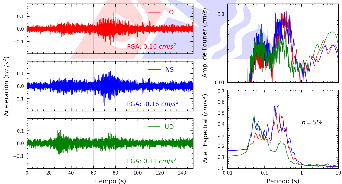
Figura A.16: Registros tiempo-historia, espectros de Fourier y de respuesta en las direcciones EO, NS y vertical de la estación SJLSC. Sismo de San Miguel, La Mar - Ayacucho del 2025-06-30, 03:44:06 (Hora local)
