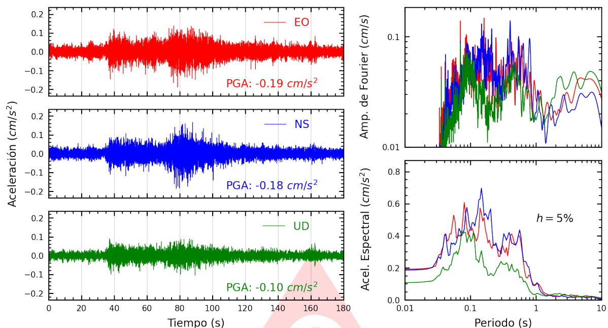
Figura A.11: Registros tiempo-historia, espectros de Fourier y de respuesta en las direcciones EO, NS y vertical de la estación USILM. Sismo de San Miguel, La Mar - Ayacucho del 2025-06-30, 03:44:06 (Hora local)
