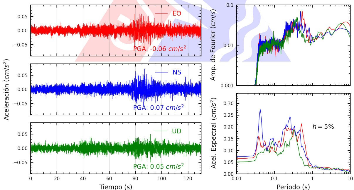
Figura A.30: Registros tiempo-historia, espectros de Fourier y de respuesta en las direcciones EO, NS y vertical de la estación COMAS. Sismo de San Miguel, La Mar - Ayacucho del 2025-06-30, 03:44:06 (Hora local)
