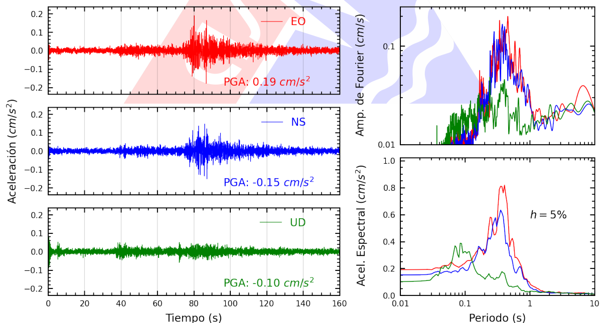
Figura A.10: Registros tiempo-historia, espectros de Fourier y de respuesta en las direcciones EO, NS y vertical de la estación ACAPU. Sismo de San Miguel, La Mar - Ayacucho del 2025-06-30, 03:44:06 (Hora local)
