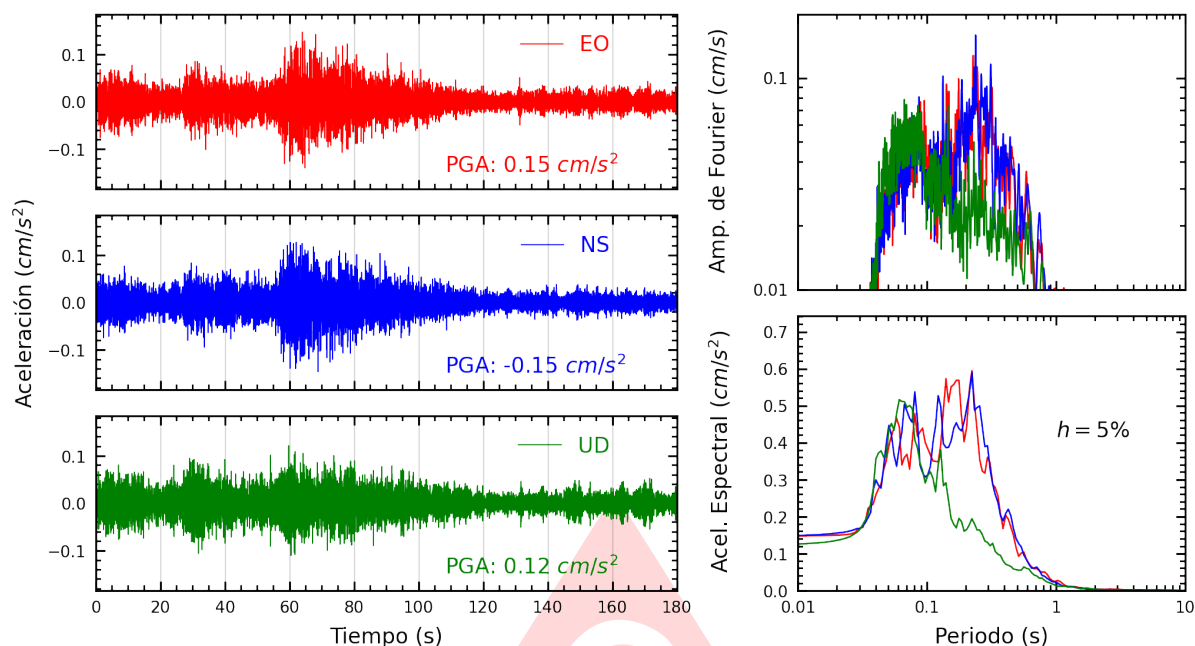
Figura A.17: Registros tiempo-historia, espectros de Fourier y de respuesta en las direcciones EO, NS y vertical de la estación ASIA. Sismo de San Miguel, La Mar - Ayacucho del 2025-06-30, 03:44:06 (Hora local)
