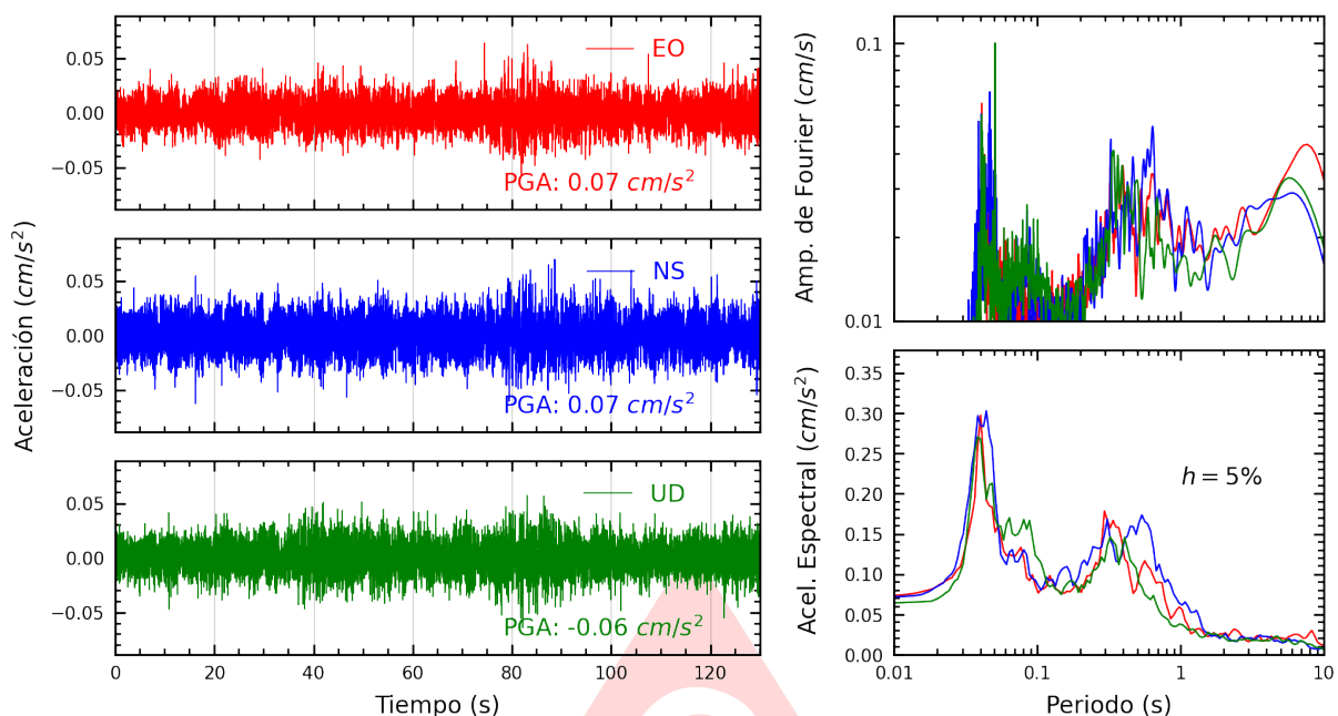
Figura A.31: Registros tiempo-historia, espectros de Fourier y de respuesta en las direcciones EO, NS y vertical de la estación BONDY. Sismo de San Miguel, La Mar - Ayacucho del 2025-06-30, 03:44:06 (Hora local)
