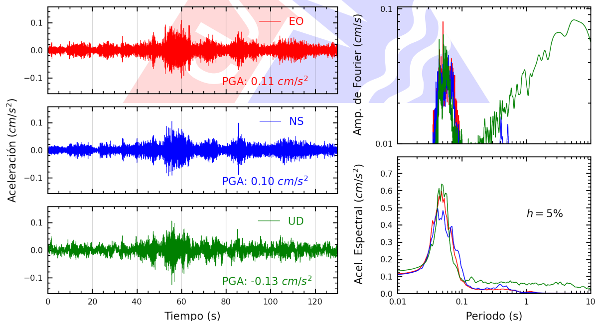
Figura A.20: Registros tiempo-historia, espectros de Fourier y de respuesta en las direcciones EO, NS y vertical de la estación SCARQ. Sismo de San Miguel, La Mar - Ayacucho del 2025-06-30, 03:44:06 (Hora local)
