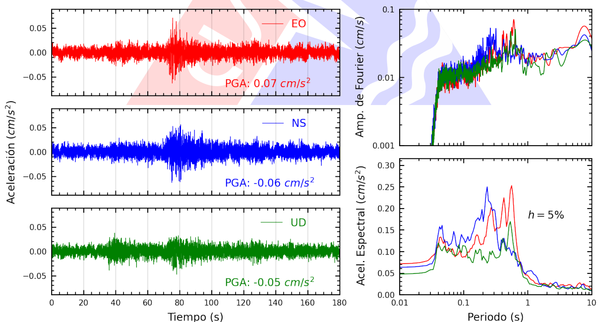
Figura A.32: Registros tiempo-historia, espectros de Fourier y de respuesta en las direcciones EO, NS y vertical de la estación SERVI. Sismo de San Miguel, La Mar - Ayacucho del 2025-06-30, 03:44:06 (Hora local)
