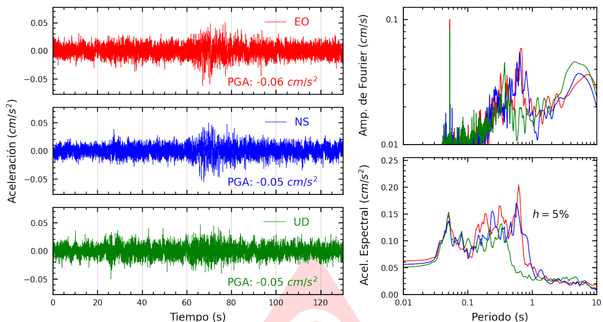
Figura A.37: Registros tiempo-historia, espectros de Fourier y de respuesta en las direcciones EO, NS y vertical de la estación UNMSM. Sismo de San Miguel, La Mar - Ayacucho del 2025-06-30, 03:44:06 (Hora local)
