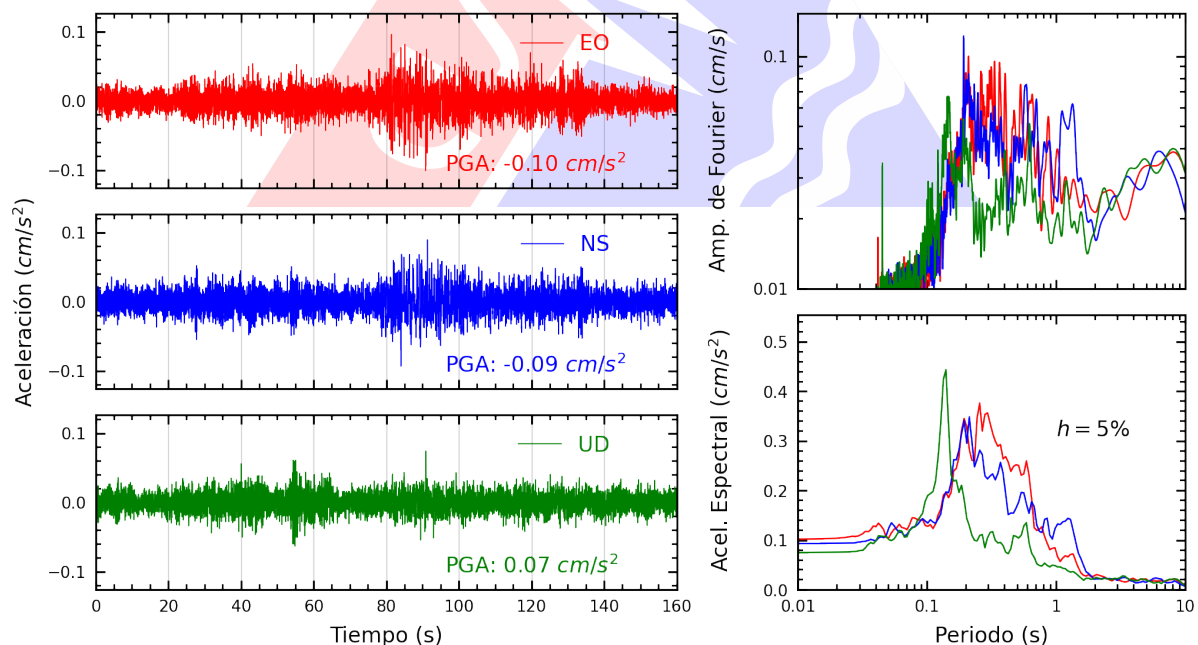
Figura A.24: Registros tiempo-historia, espectros de Fourier y de respuesta en las direcciones EO, NS y vertical de la estación DSMI. Sismo de San Miguel, La Mar - Ayacucho del 2025-06-30, 03:44:06 (Hora local)
