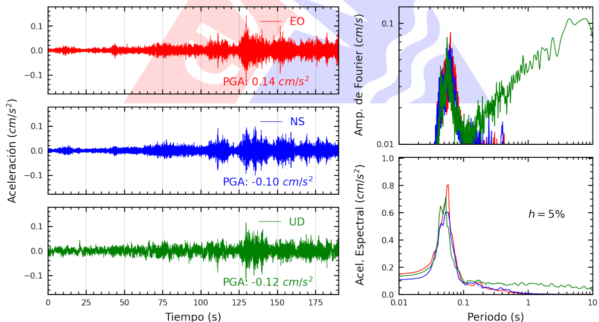
Figura A.14: Registros tiempo-historia, espectros de Fourier y de respuesta en las direcciones EO, NS y vertical de la estación SCARQ. Sismo de Antabamba, Antabamba - Apurímac del 2025-07-01, 04:09:30 (Hora local)
