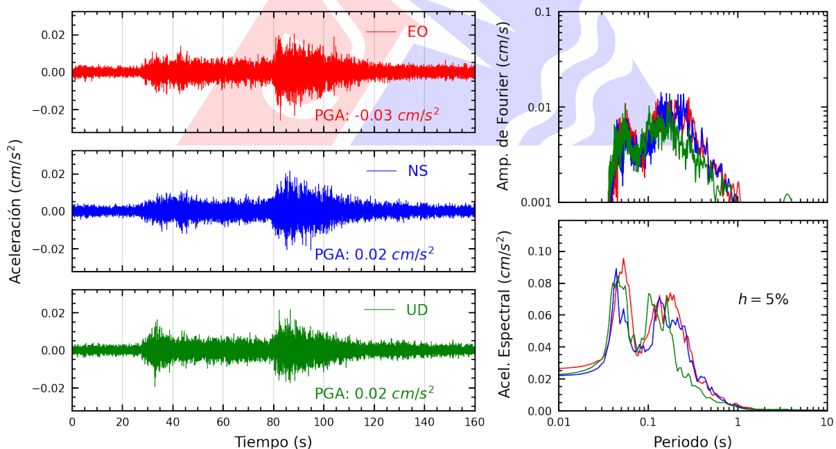
Figura A.32: Registros tiempo-historia, espectros de Fourier y de respuesta en las direcciones EO, NS y vertical de la estación JALV2. Sismo de Antabamba, Antabamba - Apurimac del 2025-07-01, 04:09:30 (Hora local)
