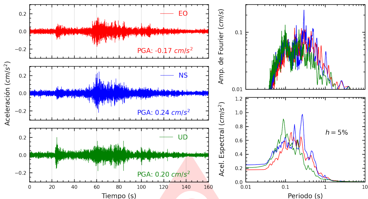
Figura A.5: Registros tiempo-historia, espectros de Fourier y de respuesta en las direcciones EO, NS y vertical de la estación UNICA. Sismo de Antabamba, Antabamba - Apurímac del 2025-07-01, 04:09:30 (Hora local)
