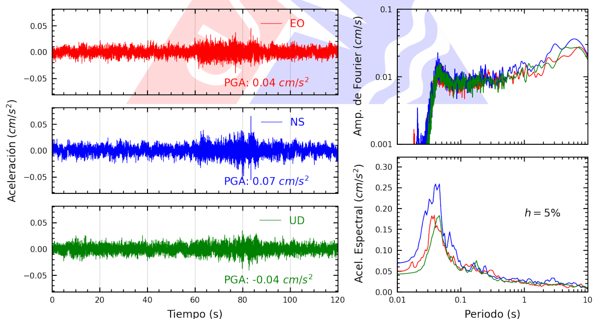
Figura A.26: Registros tiempo-historia, espectros de Fourier y de respuesta en las direcciones EO, NS y vertical de la estación SJLCE. Sismo de Antabamba, Antabamba - Apurímac del 2025-07-01, 04:09:30 (Hora local)
