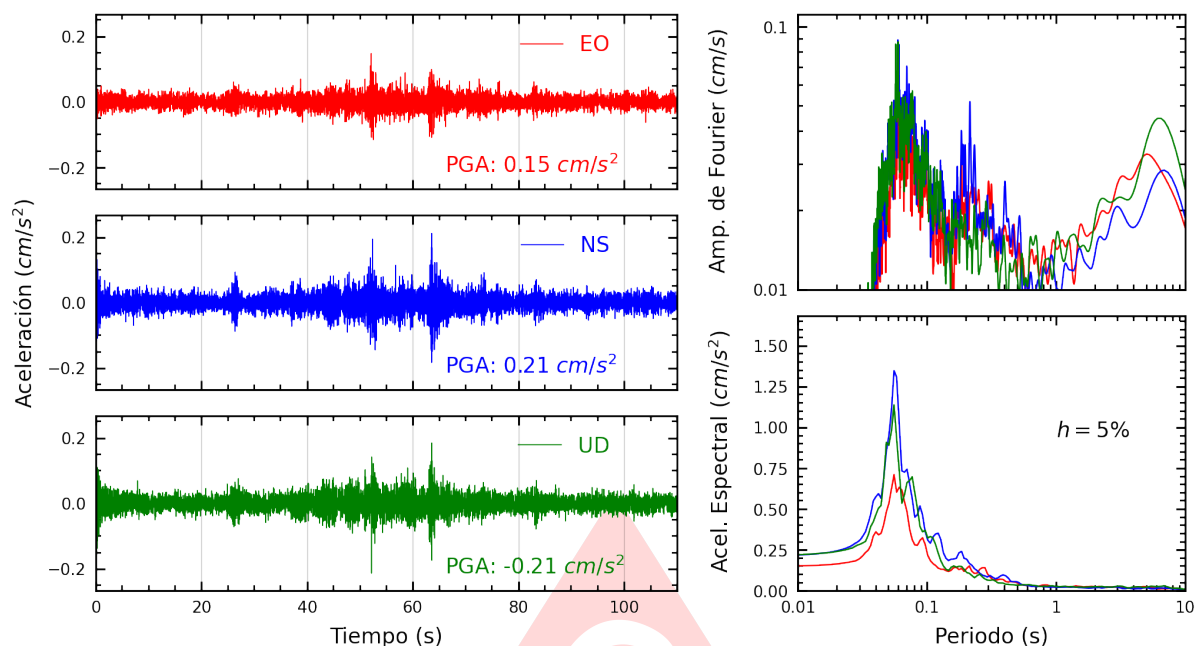
Figura A.7: Registros tiempo-historia, espectros de Fourier y de respuesta en las direcciones EO, NS y vertical de la estación SJLSC. Sismo de Antabamba, Antabamba - Apurímac del 2025-07-01, 04:09:30 (Hora local)
