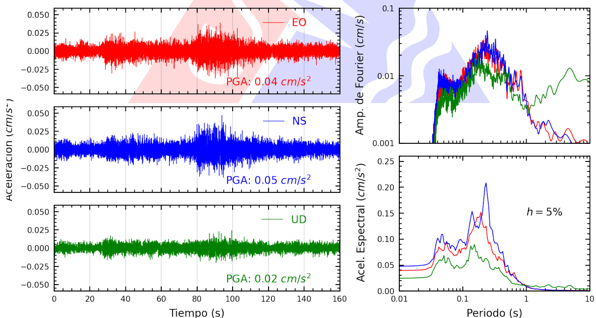
Figura A.30: Registros tiempo-historia, espectros de Fourier y de respuesta en las direcciones EO, NS y vertical de la estación BRISA. Sismo de Antabamba, Antabamba - Apurímac del 2025-07-01, 04:09:30 (Hora local)
