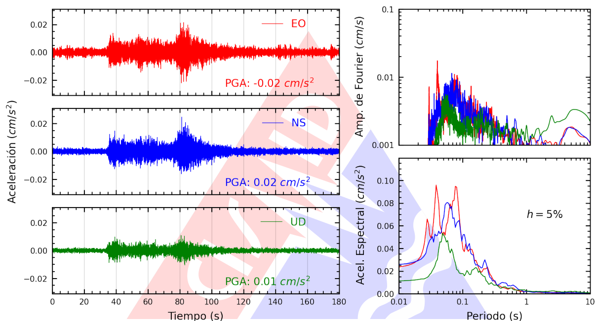
Figura A.33: Registros tiempo-historia, espectros de Fourier y de respuesta en las direcciones EO, NS y vertical de la estación UNAM. Sismo de Antabamba, Antabamba - Apurímac del 2025-07-01, 04:09:30 (Hora local)
