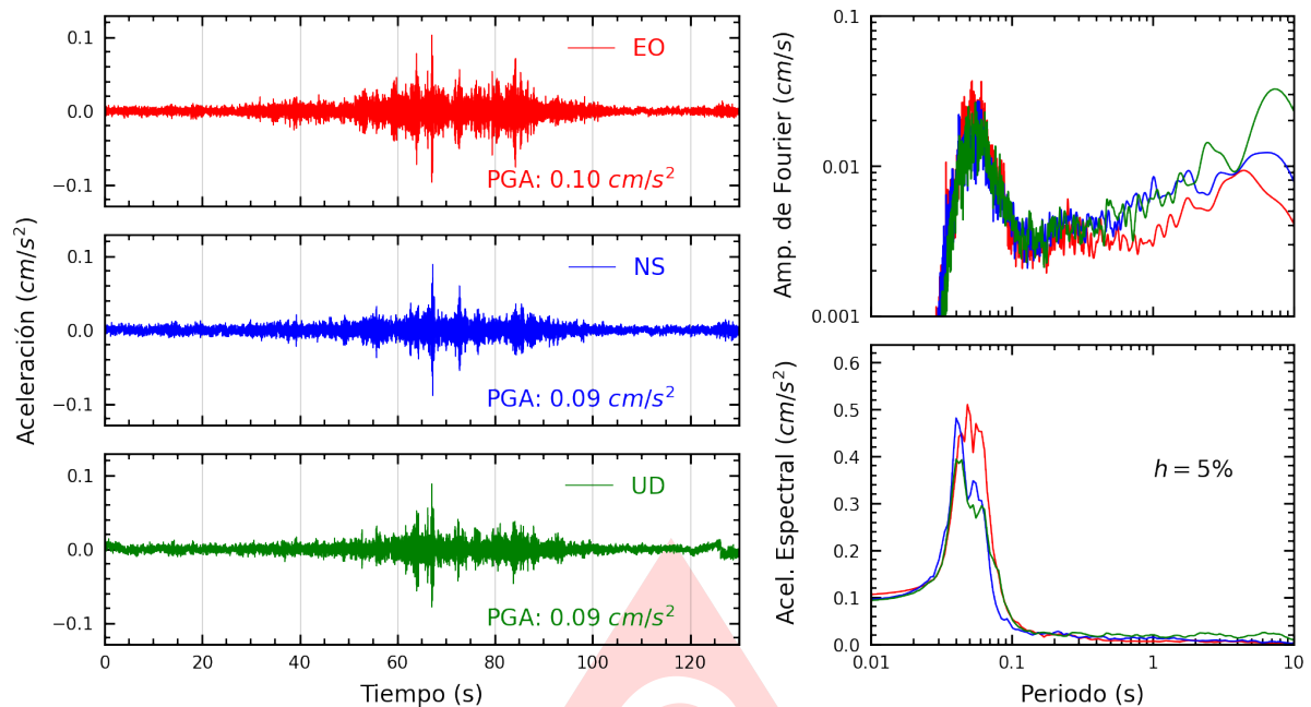
Figura A.19: Registros tiempo-historia, espectros de Fourier y de respuesta en las direcciones EO, NS y vertical de la estación CREY. Sismo de Antabamba, Antabamba - Apurimac del 2025-07-01, 04:09:30 (Hora local)
