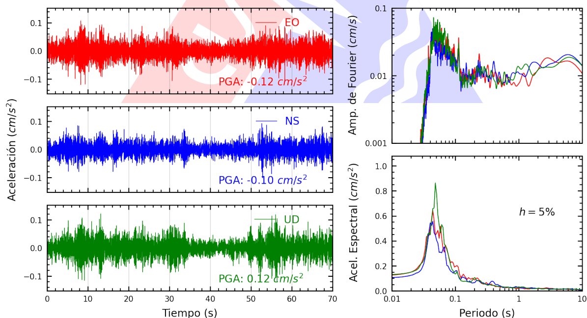
Figura A.16: Registros tiempo-historia, espectros de Fourier y de respuesta en las direcciones EO, NS y vertical de la estación URPPE. Sismo de Antabamba, Antabamba - Apurímac del 2025-07-01, 04:09:30 (Hora local)
