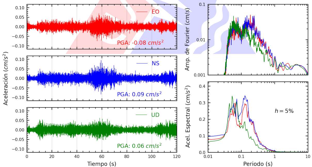
Figura A.20: Registros tiempo-historia, espectros de Fourier y de respuesta en las direcciones EO, NS y vertical de la estación ASIA. Sismo de Antabamba, Antabamba - Apurimac del 2025-07-01, 04:09:30 (Hora local)
