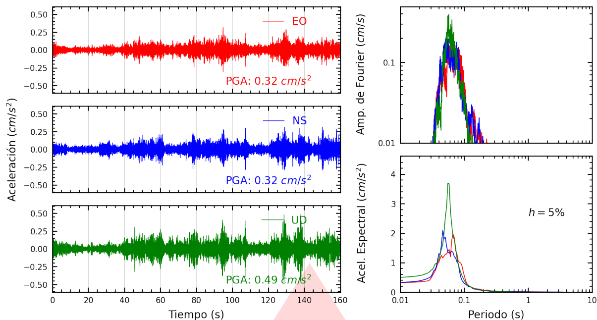
Figura A.1: Registros tiempo-historia, espectros de Fourier y de respuesta en las direcciones EO, NS y vertical de la estación SCAR2. Sismo de Antabamba, Antabamba - Apurímac del 2025-07-01, 04:09:30 (Hora local)
