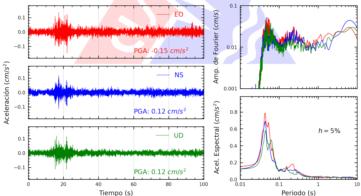
Figura A.12: Registros tiempo-historia, espectros de Fourier y de respuesta en las direcciones EO, NS y vertical de la estación SOBAR. Sismo de Antabamba, Antabamba - Apurímac del 2025-07-01, 04:09:30 (Hora local)
