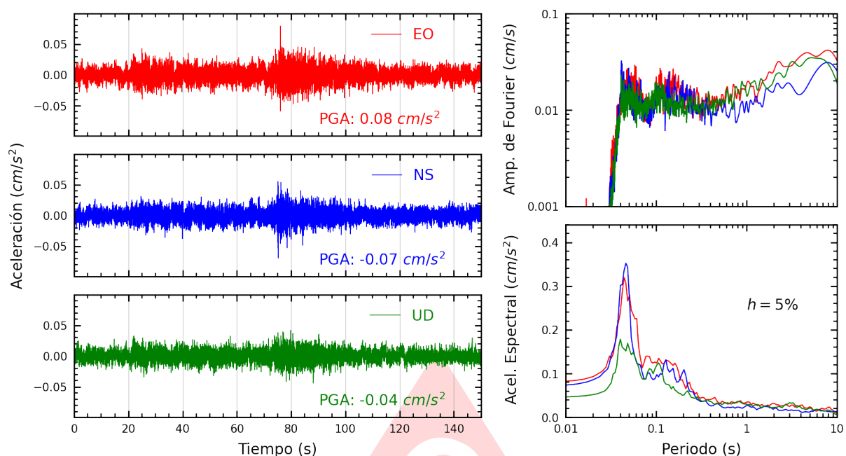
Figura A.21: Registros tiempo-historia, espectros de Fourier y de respuesta en las direcciones EO, NS y vertical de la estación AMORE. Sismo de Antabamba, Antabamba - Apurímac del 2025-07-01, 04:09:30 (Hora local)
