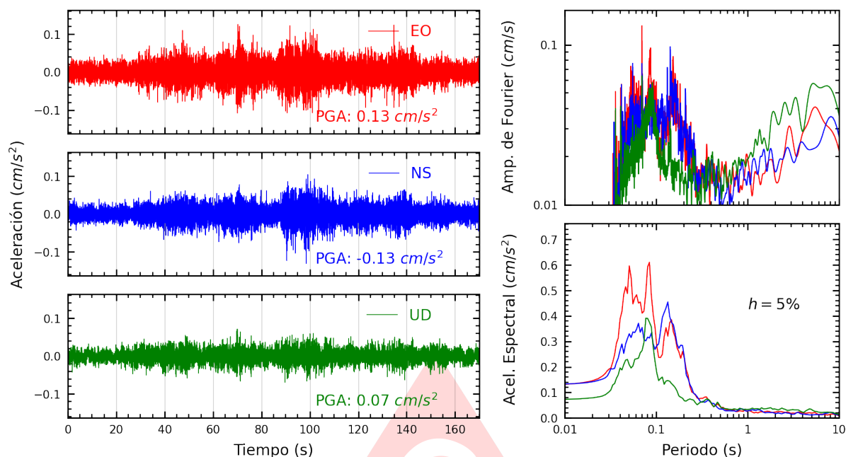
Figura A.15: Registros tiempo-historia, espectros de Fourier y de respuesta en las direcciones EO, NS y vertical de la estación USILM. Sismo de Antabamba, Antabamba - Apurímac del 2025-07-01, 04:09:30 (Hora local)
