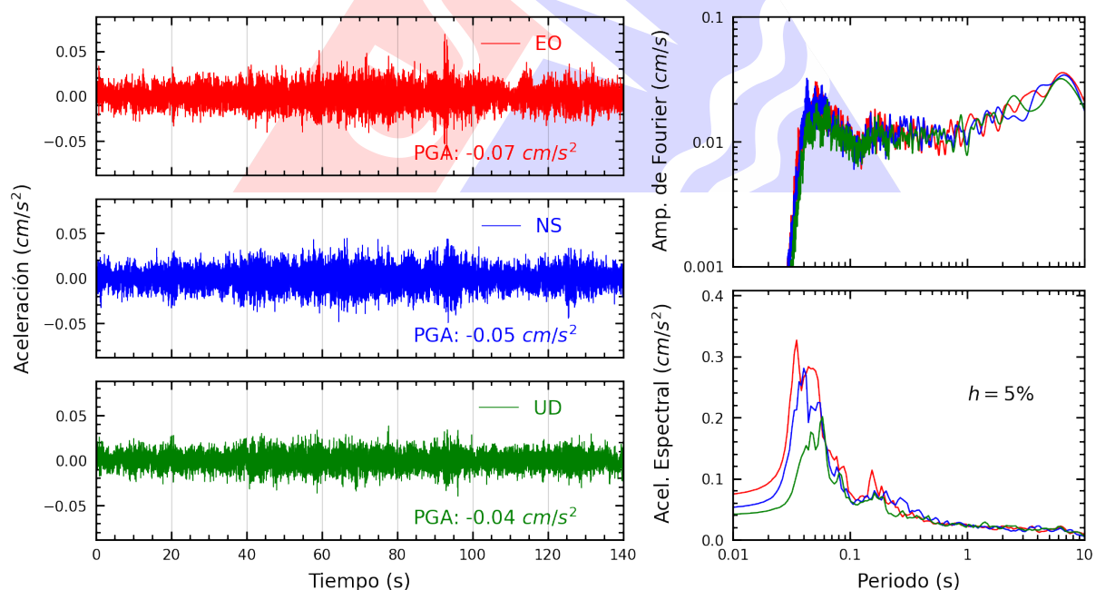
Figura A.24: Registros tiempo-historia, espectros de Fourier y de respuesta en las direcciones EO, NS y vertical de la estación FICPE. Sismo de Antabamba, Antabamba - Apurimac del 2025-07-01, 04:09:30 (Hora local)
