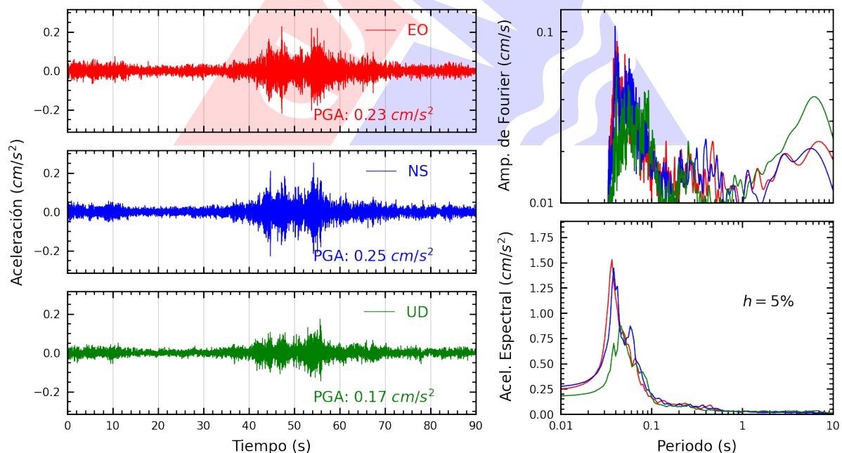
Figura A.4: Registros tiempo-historia, espectros de Fourier y de respuesta en las direcciones EO, NS y vertical de la estación OLIVO. Sismo de Antabamba, Antabamba - Apurimac del 2025-07-01, 04:09:30 (Hora local)
