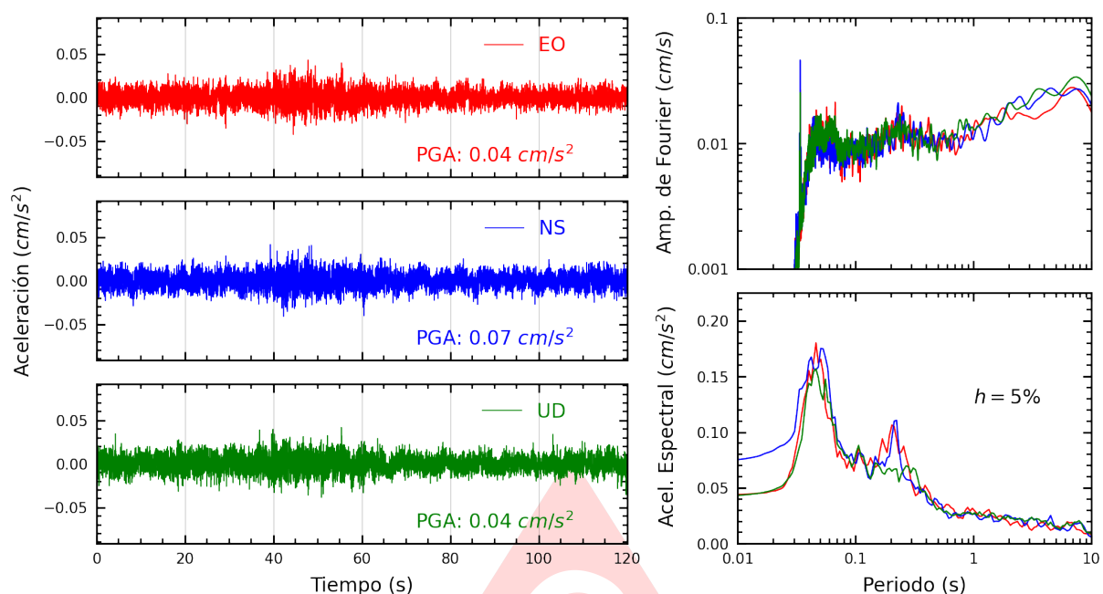
Figura A.23: Registros tiempo-historia, espectros de Fourier y de respuesta en las direcciones EO, NS y vertical de la estación USMP. Sismo de Antabamba, Antabamba - Apurimac del 2025-07-01, 04:09:30 (Hora local)
