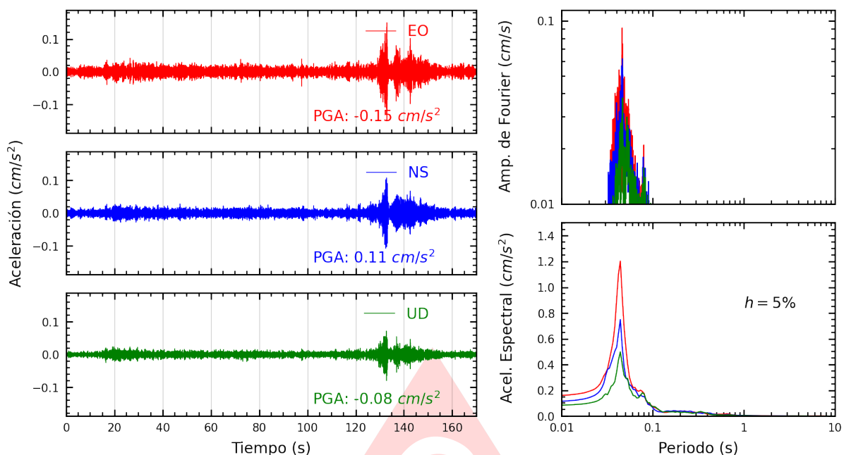
Figura A.11: Registros tiempo-historia, espectros de Fourier y de respuesta en las direcciones EO, NS y vertical de la estación BORJA. Sismo de Antabamba, Antabamba - Apurímac del 2025-07-01, 04:09:30 (Hora local)
