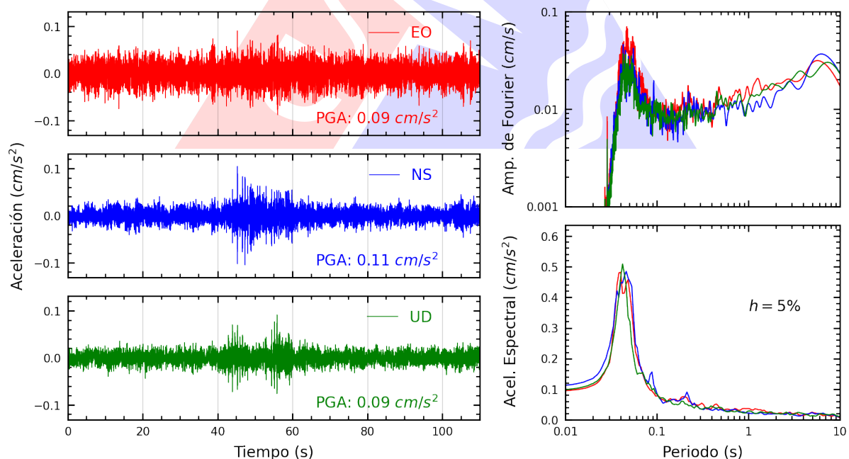
Figura A.18: Registros tiempo-historia, espectros de Fourier y de respuesta en las direcciones EO, NS y vertical de la estación INICT. Sismo de Antabamba, Antabamba - Apurimac del 2025-07-01, 04:09:30 (Hora local)
