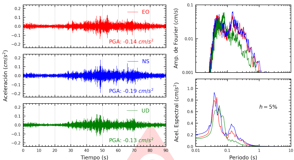
Figura A.9: Registros tiempo-historia, espectros de Fourier y de respuesta en las direcciones EO, NS y vertical de la estación CARAB. Sismo de Antabamba, Antabamba - Apurimac del 2025-07-01, 04:09:30 (Hora local)
