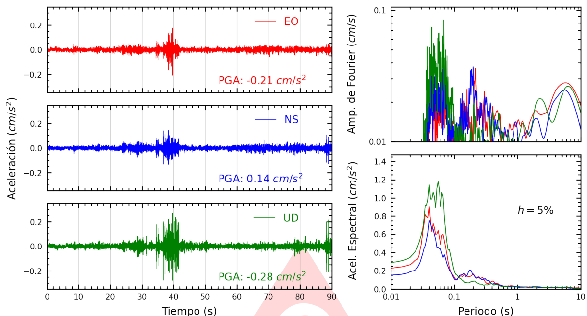
Figura A.3: Registros tiempo-historia, espectros de Fourier y de respuesta en las direcciones EO, NS y vertical de la estación SOCHO. Sismo de Antabamba, Antabamba - Apurimac del 2025-07-01, 04:09:30 (Hora local)
