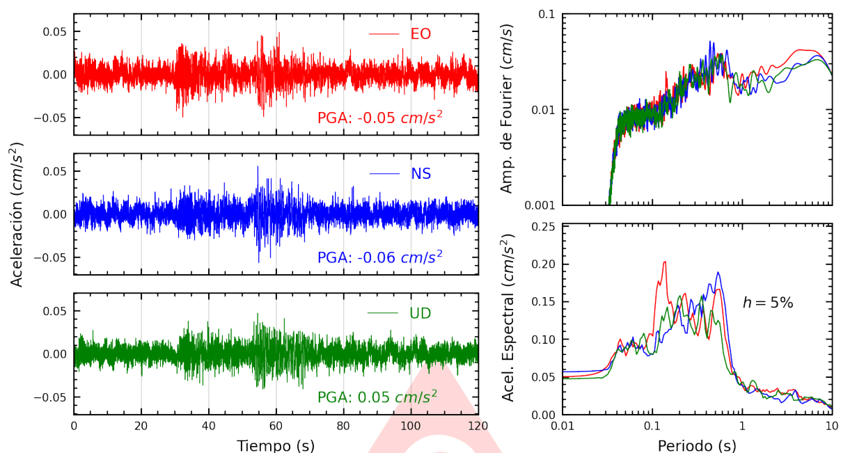
Figura A.29: Registros tiempo-historia, espectros de Fourier y de respuesta en las direcciones EO, NS y vertical de la estación UNSCH. Sismo de Antabamba, Antabamba - Apurímac del 2025-07-01, 04:09:30 (Hora local)
