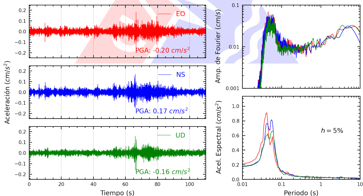
Figura A.8: Registros tiempo-historia, espectros de Fourier y de respuesta en las direcciones EO, NS y vertical de la estación JOSEO. Sismo de Antabamba, Antabamba - Apurímac del 2025-07-01, 04:09:30 (Hora local)
