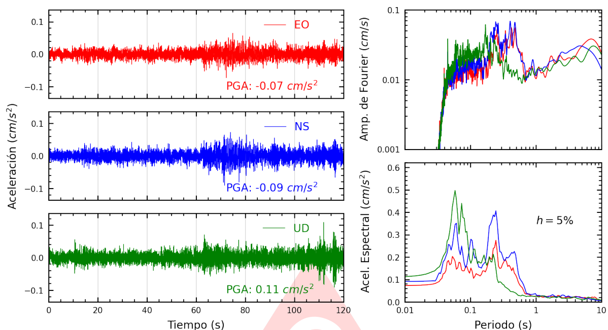
Figura A.17: Registros tiempo-historia, espectros de Fourier y de respuesta en las direcciones EO, NS y vertical de la estación MDPP. Sismo de Antabamba, Antabamba - Apurimac del 2025-07-01, 04:09:30 (Hora local)
