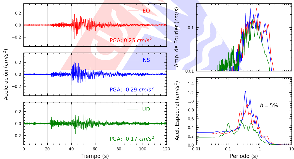
Figura A.2: Registros tiempo-historia, espectros de Fourier y de respuesta en las direcciones EO, NS y vertical de la estación SCCUS. Sismo de Antabamba, Antabamba - Apurímac del 2025-07-01, 04:09:30 (Hora local)
