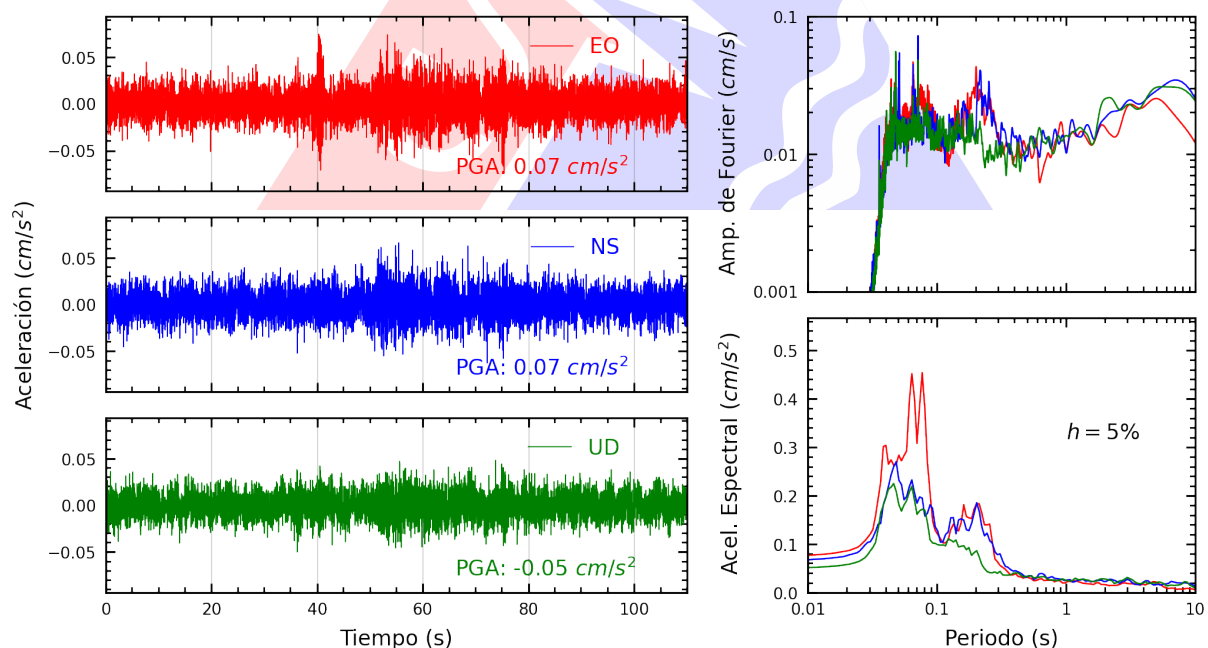
Figura A.22: Registros tiempo-historia, espectros de Fourier y de respuesta en las direcciones EO, NS y vertical de la estación INDEP. Sismo de Antabamba, Antabamba - Apurímac del 2025-07-01, 04:09:30 (Hora local)
