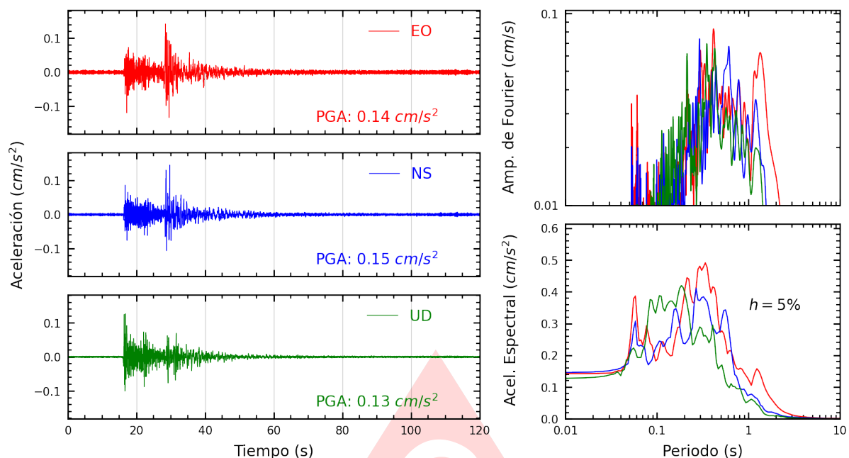
Figura A.13: Registros tiempo-historia, espectros de Fourier y de respuesta en las direcciones EO, NS y vertical de la estación UNMBA. Sismo de Antabamba, Antabamba - Apurímac del 2025-07-01, 04:09:30 (Hora local)
