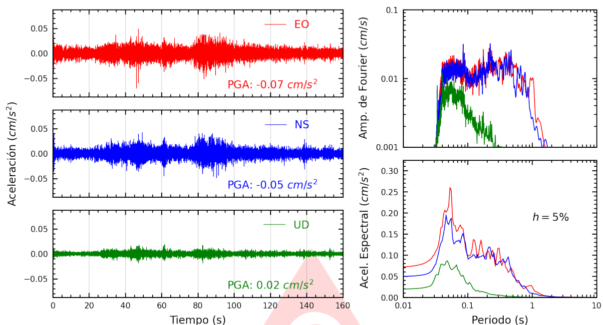
Figura A.25: Registros tiempo-historia, espectros de Fourier y de respuesta en las direcciones EO, NS y vertical de la estación UCVAT. Sismo de Antabamba, Antabamba - Apurímac del 2025-07-01, 04:09:30 (Hora local)
