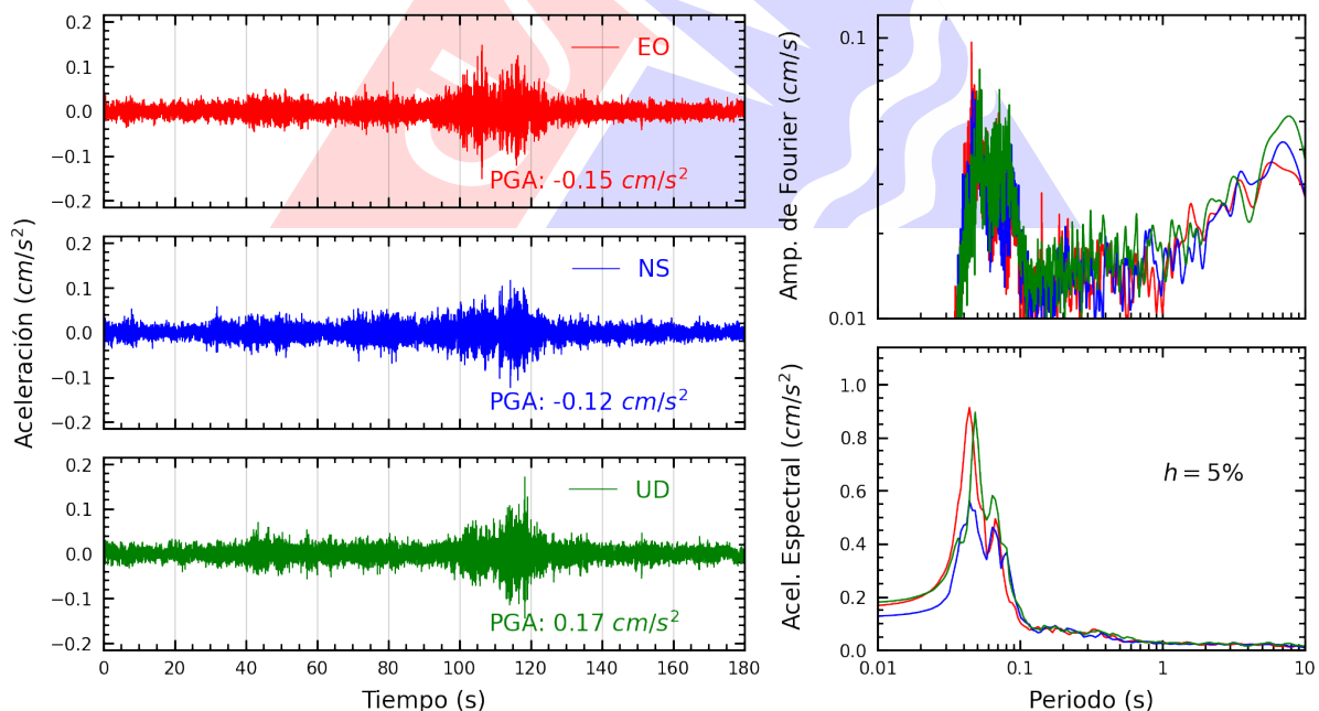
Figura A.10: Registros tiempo-historia, espectros de Fourier y de respuesta en las direcciones EO, NS y vertical de la estación IMCA. Sismo de Antabamba, Antabamba - Apurimac del 2025-07-01, 04:09:30 (Hora local)
