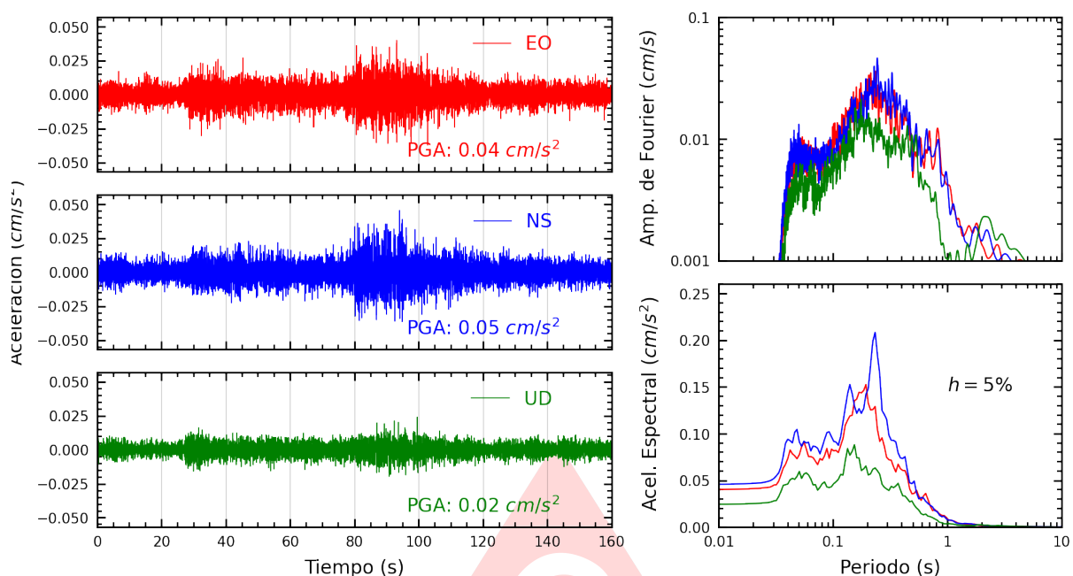
Figura A.31: Registros tiempo-historia, espectros de Fourier y de respuesta en las direcciones EO, NS y vertical de la estación BRIS2. Sismo de Antabamba, Antabamba - Apurimac del 2025-07-01, 04:09:30 (Hora local)
