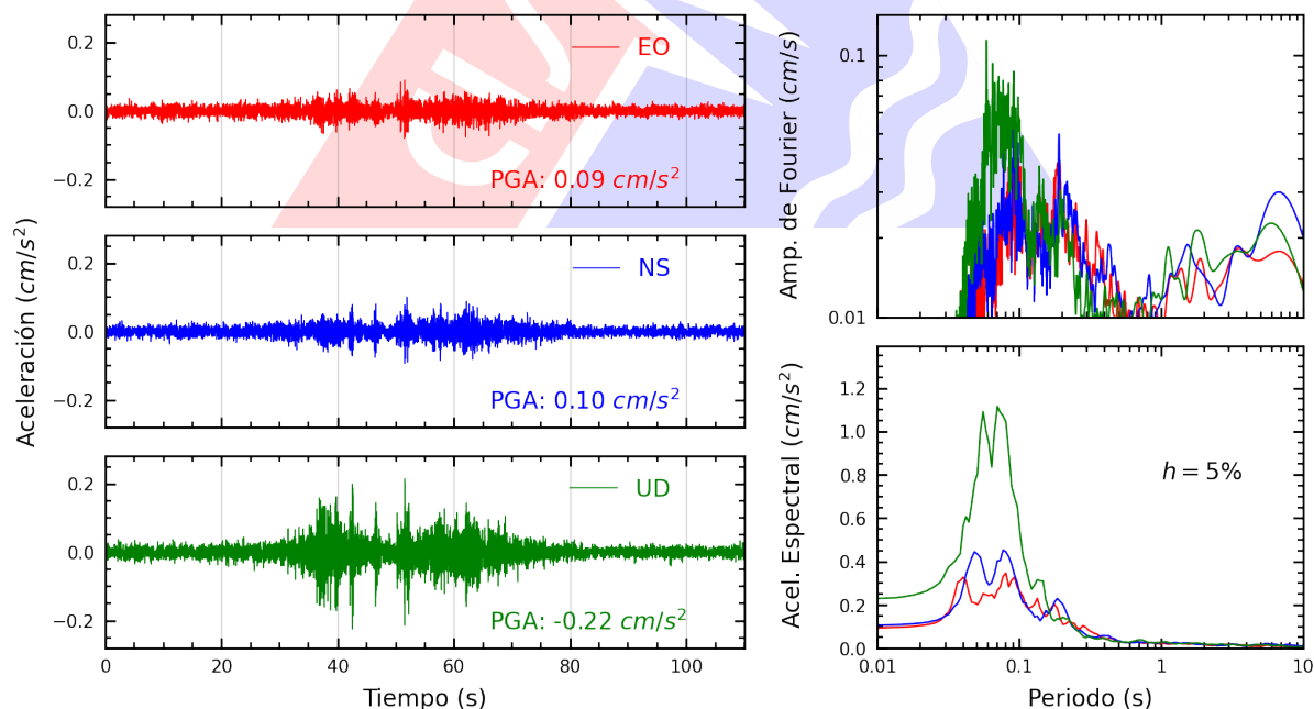
Figura A.6: Registros tiempo-historia, espectros de Fourier y de respuesta en las direcciones EO, NS y vertical de la estación RAMON. Sismo de Antabamba, Antabamba - Apurímac del 2025-07-01, 04:09:30 (Hora local)
