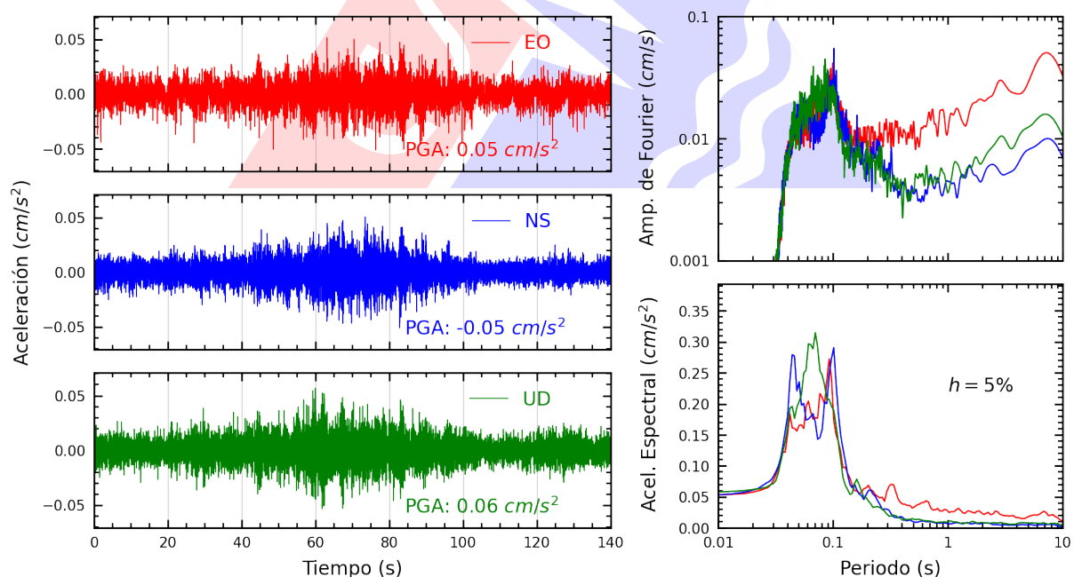
Figura A.28: Registros tiempo-historia, espectros de Fourier y de respuesta en las direcciones EO, NS y vertical de la estación UJBG3. Sismo de Antabamba, Antabamba - Apurímac del 2025-07-01, 04:09:30 (Hora local)
