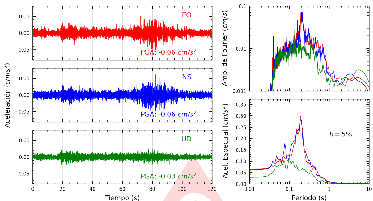
Figura A.27: Registros tiempo-historia, espectros de Fourier y de respuesta en las direcciones EO, NS y vertical de la estación SCCHO. Sismo de Antabamba, Antabamba - Apurímac del 2025-07-01, 04:09:30 (Hora local)
