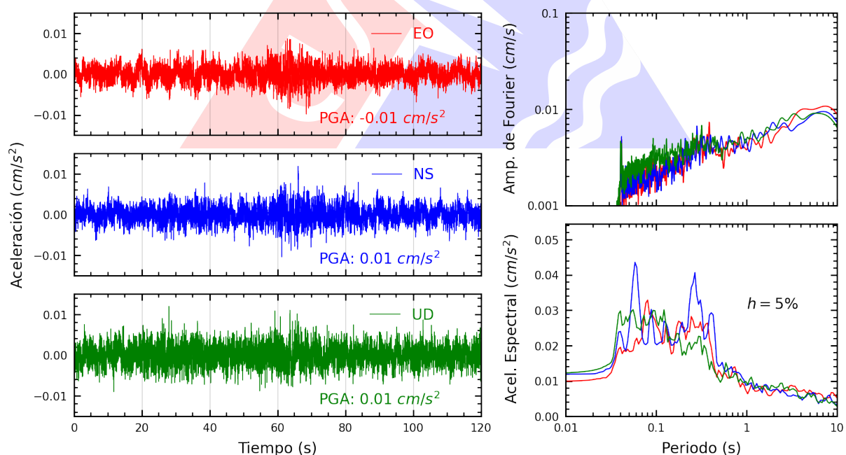
Figura A.8: Registros tiempo-historia, espectros de Fourier y de respuesta en las direcciones EO, NS y vertical de la estación UNJ. Sismo de San Pedro De Lloc, Pacasmayo - La Libertad del 2025-07-01, 04:24:32 (Hora local)
