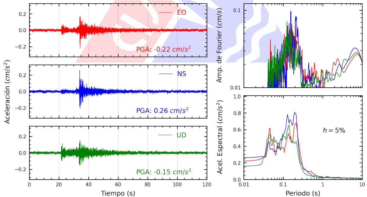
Figura A.4: Registros tiempo-historia, espectros de Fourier y de respuesta en las direcciones EO, NS y vertical de la estación UPAOT. Sismo de San Pedro De Lloc, Pacasmayo - La Libertad del 2025-07-01, 04:24:32 (Hora local)
