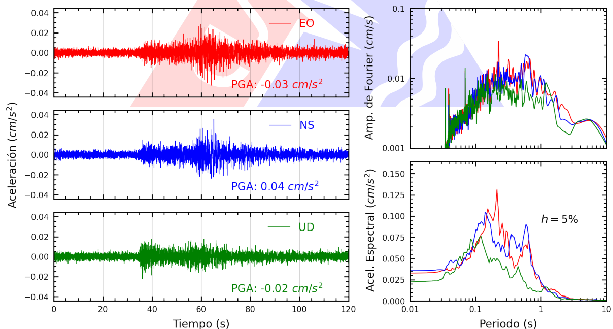
Figura A.6: Registros tiempo-historia, espectros de Fourier y de respuesta en las direcciones EO, NS y vertical de la estación UNC. Sismo de San Pedro De Lloc, Pacasmayo - La Libertad del 2025-07-01, 04:24:32 (Hora local)
