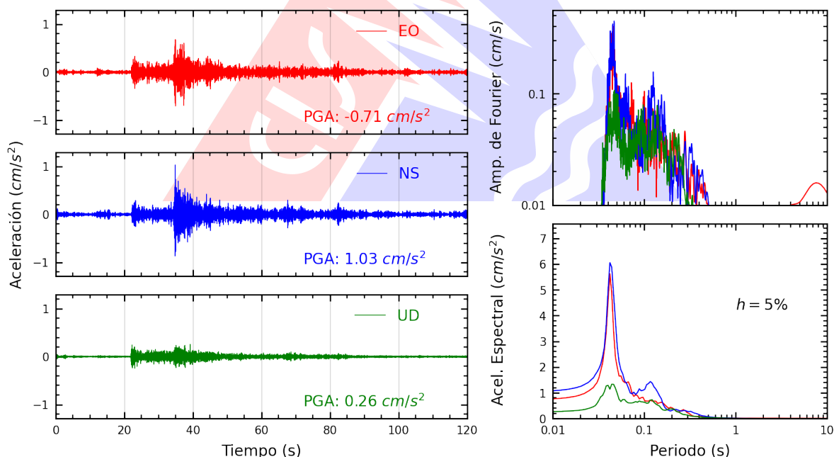
Figura A.2: Registros tiempo-historia, espectros de Fourier y de respuesta en las direcciones EO, NS y vertical de la estación SCTRU. Sismo de San Pedro De Lloc, Pacasmayo - La Libertad del 2025-07-01, 04:24:32 (Hora local)
