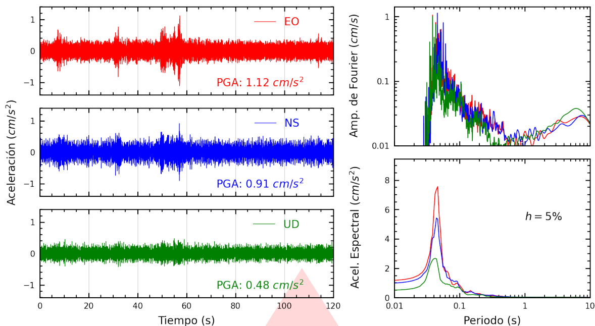
Figura A.1: Registros tiempo-historia, espectros de Fourier y de respuesta en las direcciones EO, NS y vertical de la estación USP. Sismo de San Pedro De Lloc, Pacasmayo - La Libertad del 2025-07-01, 04:24:32 (Hora local)
