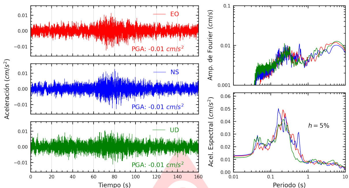
Figura A.7: Registros tiempo-historia, espectros de Fourier y de respuesta en las direcciones EO, NS y vertical de la estación CARAL. Sismo de San Pedro De Lloc, Pacasmayo - La Libertad del 2025-07-01, 04:24:32 (Hora local)
