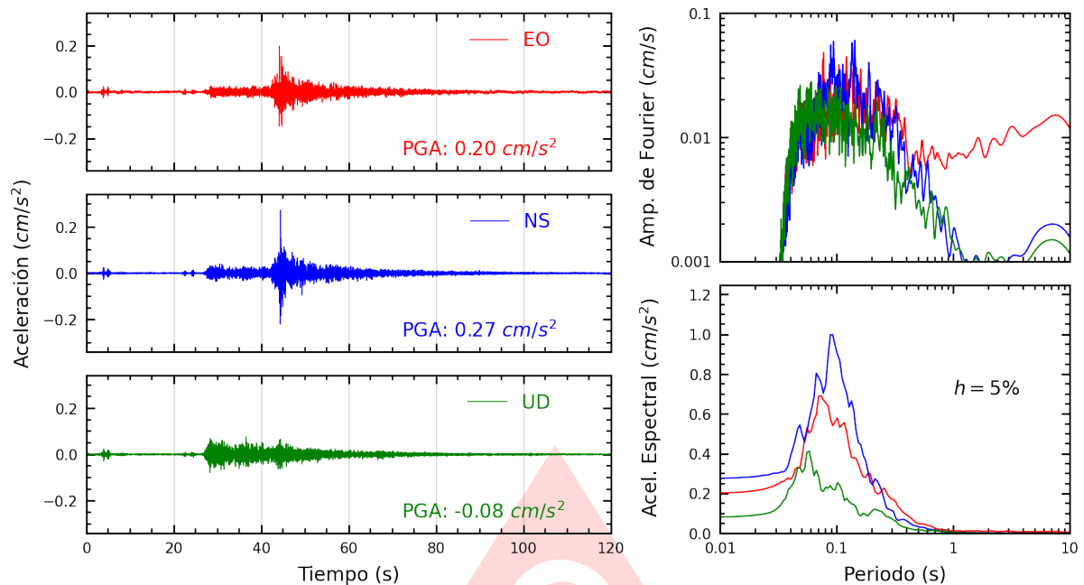
Figura A.3: Registros tiempo-historia, espectros de Fourier y de respuesta en las direcciones EO, NS y vertical de la estación SCCHI. Sismo de San Pedro De Lloc, Pacasmayo - La Libertad del 2025-07-01, 04:24:32 (Hora local)
