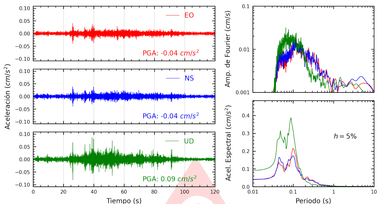
Figura A.5: Registros tiempo-historia, espectros de Fourier y de respuesta en las direcciones EO, NS y vertical de la estación UNP. Sismo de San Pedro De Lloc, Pacasmayo - La Libertad del 2025-07-01, 04:24:32 (Hora local)
