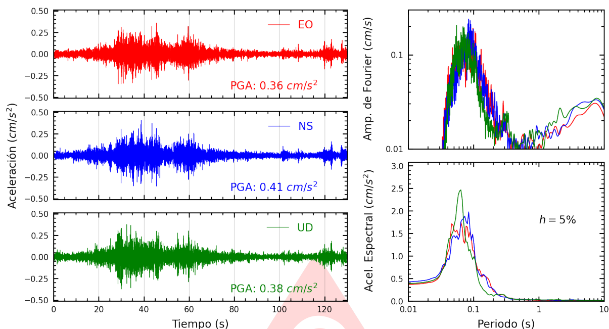
Figura A.5: Registros tiempo-historia, espectros de Fourier y de respuesta en las direcciones EO, NS y vertical de la estación SJLSV. Sismo de Huasichanca, Huancayo - Junin del 2025-07-02, 23:57:57 (Hora local)
