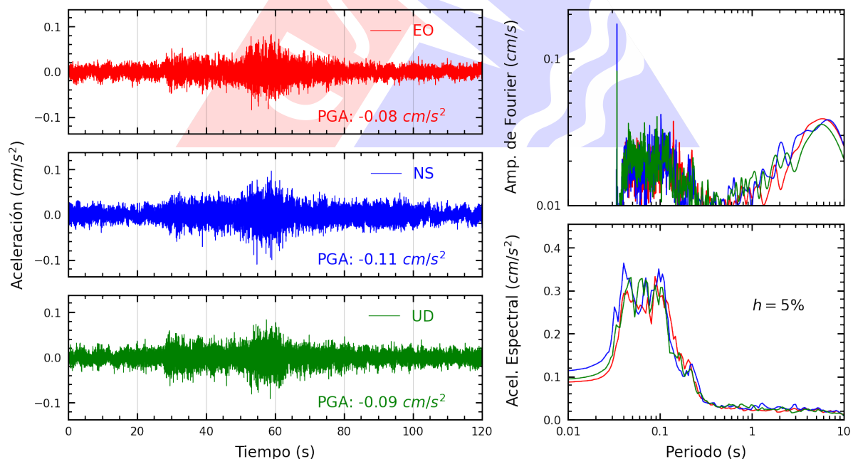
Figura A.22: Registros tiempo-historia, espectros de Fourier y de respuesta en las direcciones EO, NS y vertical de la estación USMP. Sismo de Huasichanca, Huancayo - Junin del 2025-07-02, 23:57:57 (Hora local)
