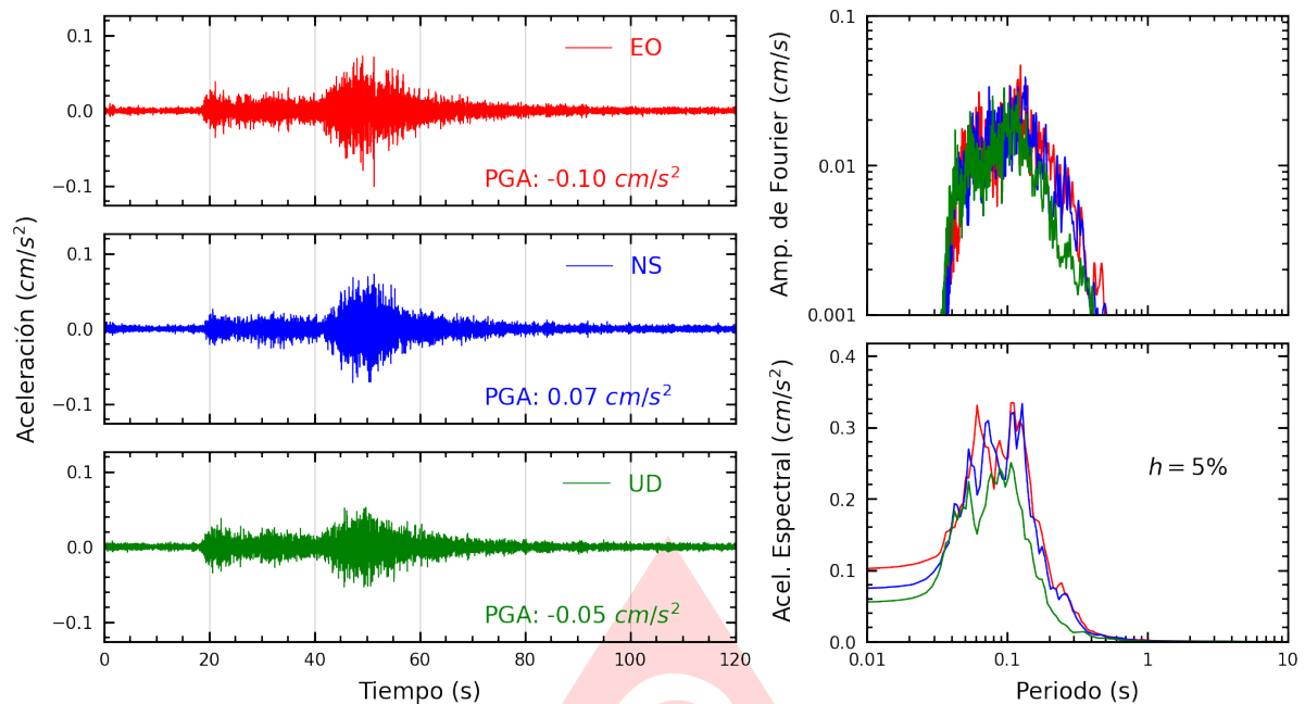
Figura A.29: Registros tiempo-historia, espectros de Fourier y de respuesta en las direcciones EO, NS y vertical de la estación JALV2. Sismo de Huasicancha, Huancayo - Junin del 2025-07-02, 23:57:57 (Hora local)
