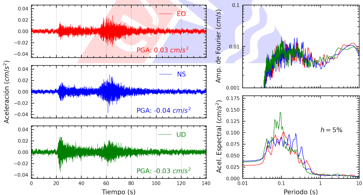
Figura A.38: Registros tiempo-historia, espectros de Fourier y de respuesta en las direcciones EO, NS y vertical de la estación CARAL. Sismo de Huasicancha, Huancayo - Junin del 2025-07-02, 23:57:57 (Hora local)
