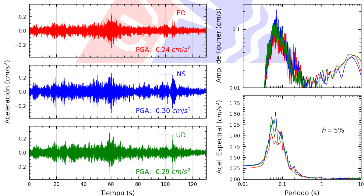
Figura A.8: Registros tiempo-historia, espectros de Fourier y de respuesta en las direcciones EO, NS y vertical de la estación SJLSC. Sismo de Huasicancha, Huancayo - Junin del 2025-07-02, 23:57:57 (Hora local)
