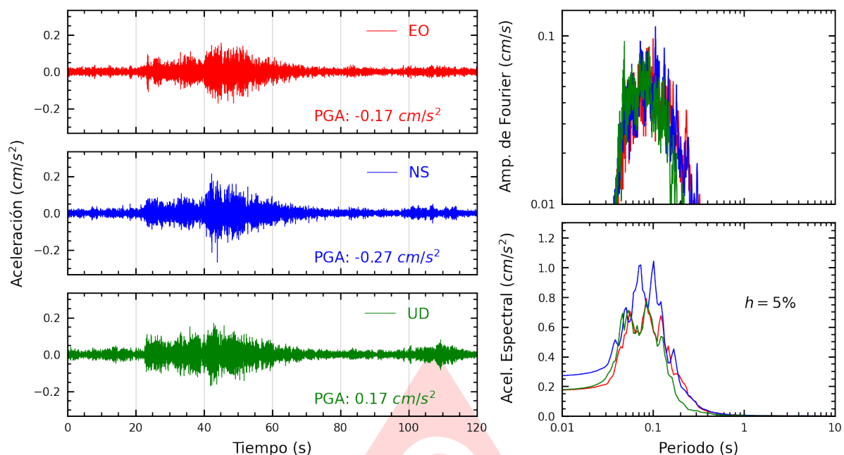
Figura A.9: Registros tiempo-historia, espectros de Fourier y de respuesta en las direcciones EO, NS y vertical de la estación ASIA. Sismo de Huasicancha, Huancayo - Junin del 2025-07-02, 23:57:57 (Hora local)
