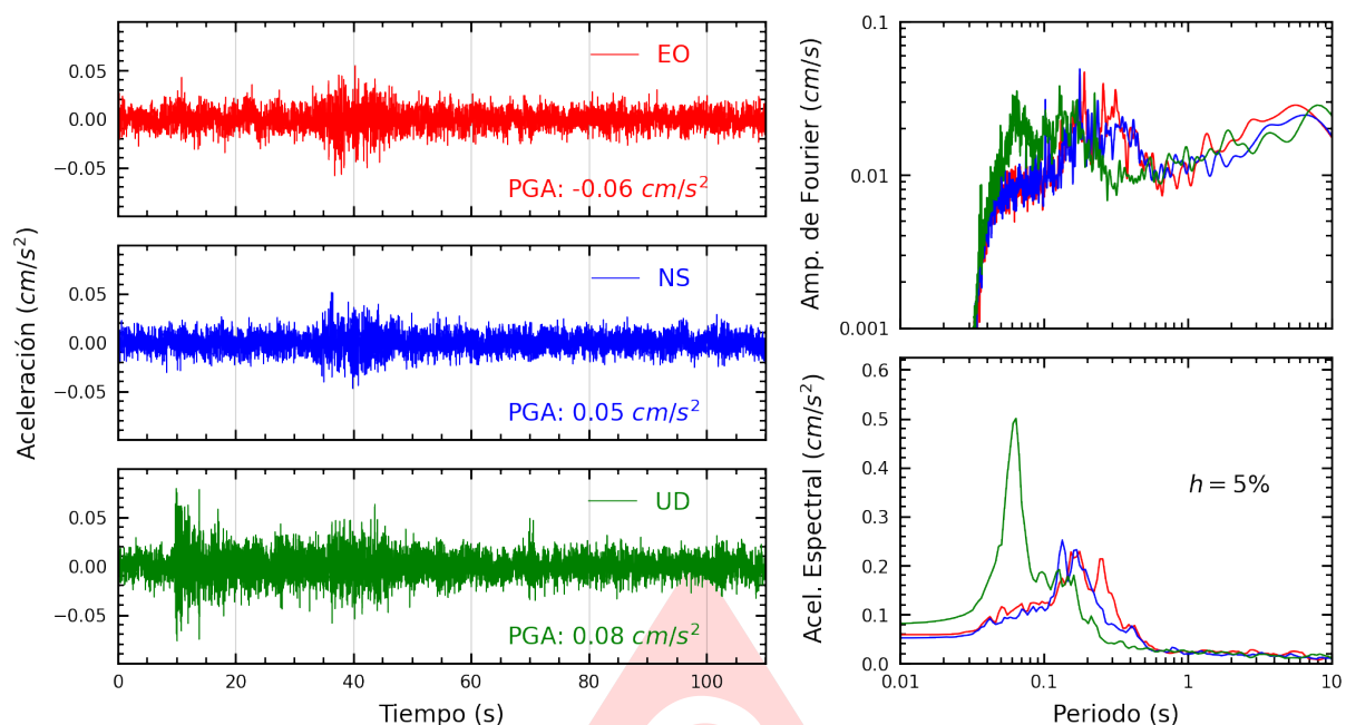
Figura A.35: Registros tiempo-historia, espectros de Fourier y de respuesta en las direcciones EO, NS y vertical de la estación ACAPU. Sismo de Huasichanca, Huancayo - Junin del 2025-07-02, 23:57:57 (Hora local)
