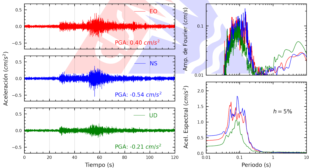
Figura A.2: Registros tiempo-historia, espectros de Fourier y de respuesta en las direcciones EO, NS y vertical de la estación USILM. Sismo de Huasichanca, Huancayo - Junin del 2025-07-02, 23:57:57 (Hora local)
