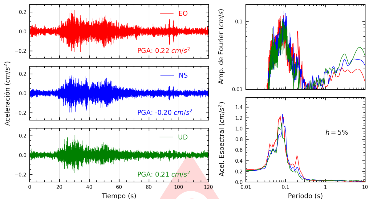
Figura A.13: Registros tiempo-historia, espectros de Fourier y de respuesta en las direcciones EO, NS y vertical de la estación INDEP. Sismo de Huasicancha, Huancayo - Junin del 2025-07-02, 23:57:57 (Hora local)
