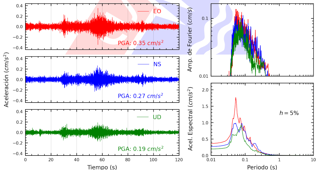
Figura A.6: Registros tiempo-historia, espectros de Fourier y de respuesta en las direcciones EO, NS y vertical de la estación UNTEL. Sismo de Huasichanca, Huancayo - Junin del 2025-07-02, 23:57:57 (Hora local)
