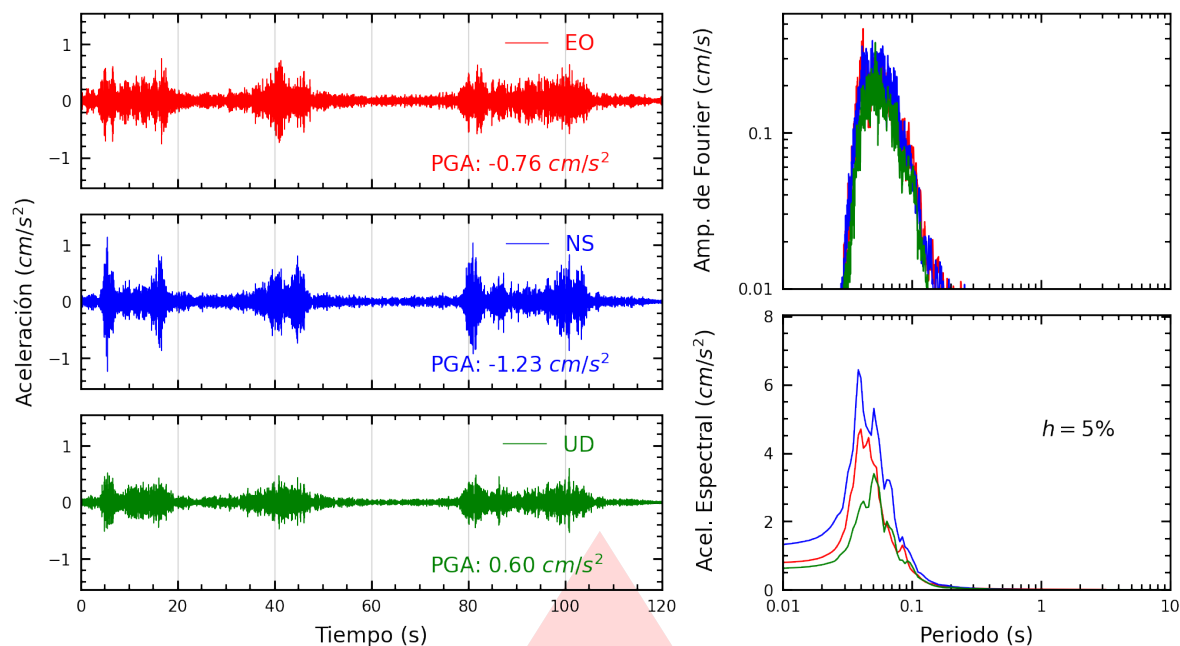
Figura A.1: Registros tiempo-historia, espectros de Fourier y de respuesta en las direcciones EO, NS y vertical de la estación PACHA. Sismo de Huasichanca, Huancayo - Junin del 2025-07-02, 23:57:57 (Hora local)
