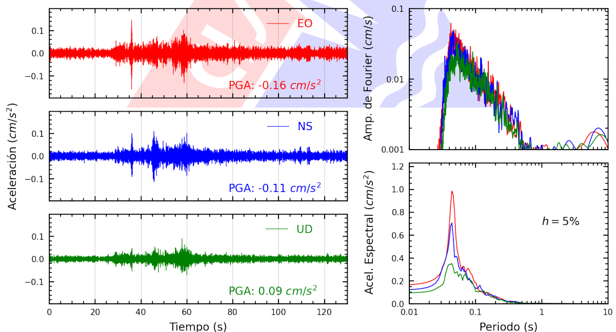
Figura A.16: Registros tiempo-historia, espectros de Fourier y de respuesta en las direcciones EO, NS y vertical de la estación BORJA. Sismo de Huasicancha, Huancayo - Junin del 2025-07-02, 23:57:57 (Hora local)
