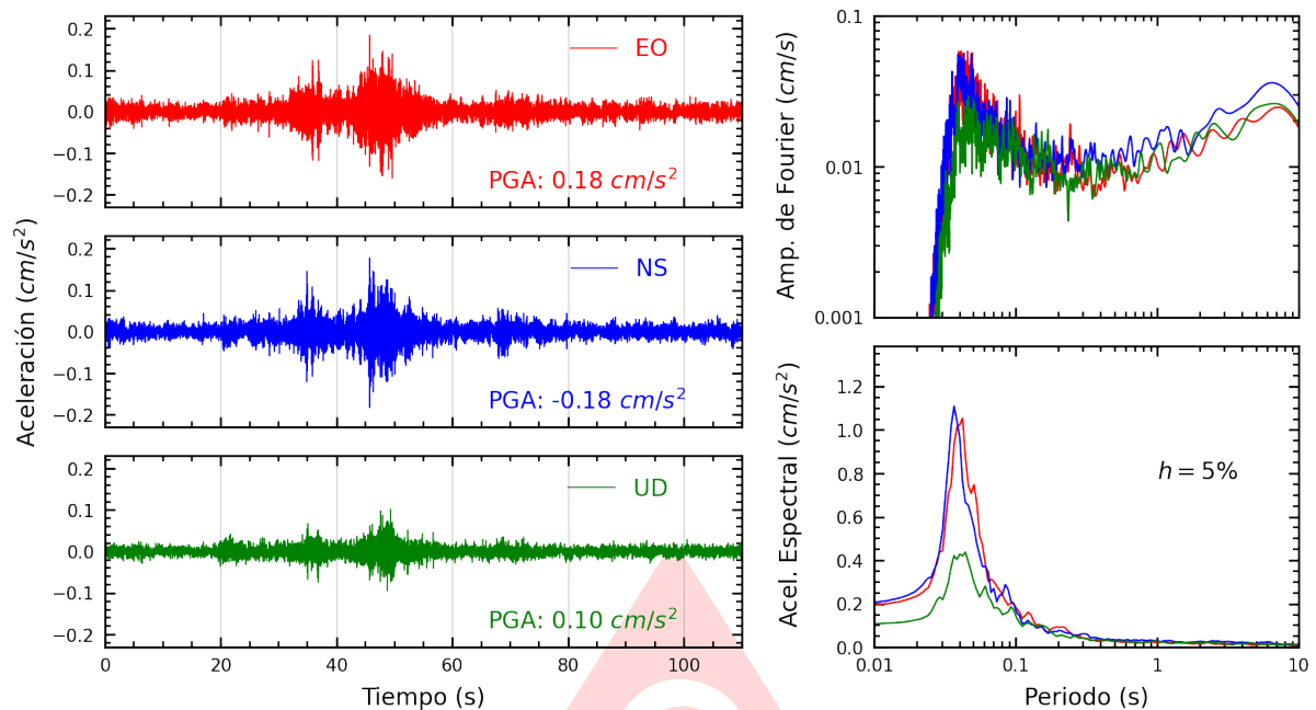
Figura A.15: Registros tiempo-historia, espectros de Fourier y de respuesta en las direcciones EO, NS y vertical de la estación CEPRE. Sismo de Huasicancha, Huancayo - Junin del 2025-07-02, 23:57:57 (Hora local)
