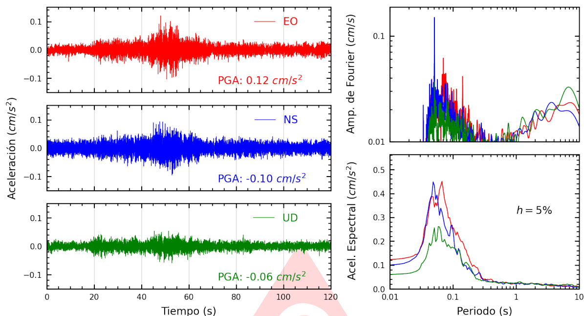
Figura A.19: Registros tiempo-historia, espectros de Fourier y de respuesta en las direcciones EO, NS y vertical de la estación FICPE. Sismo de Huasichanca, Huancayo - Junin del 2025-07-02, 23:57:57 (Hora local)
