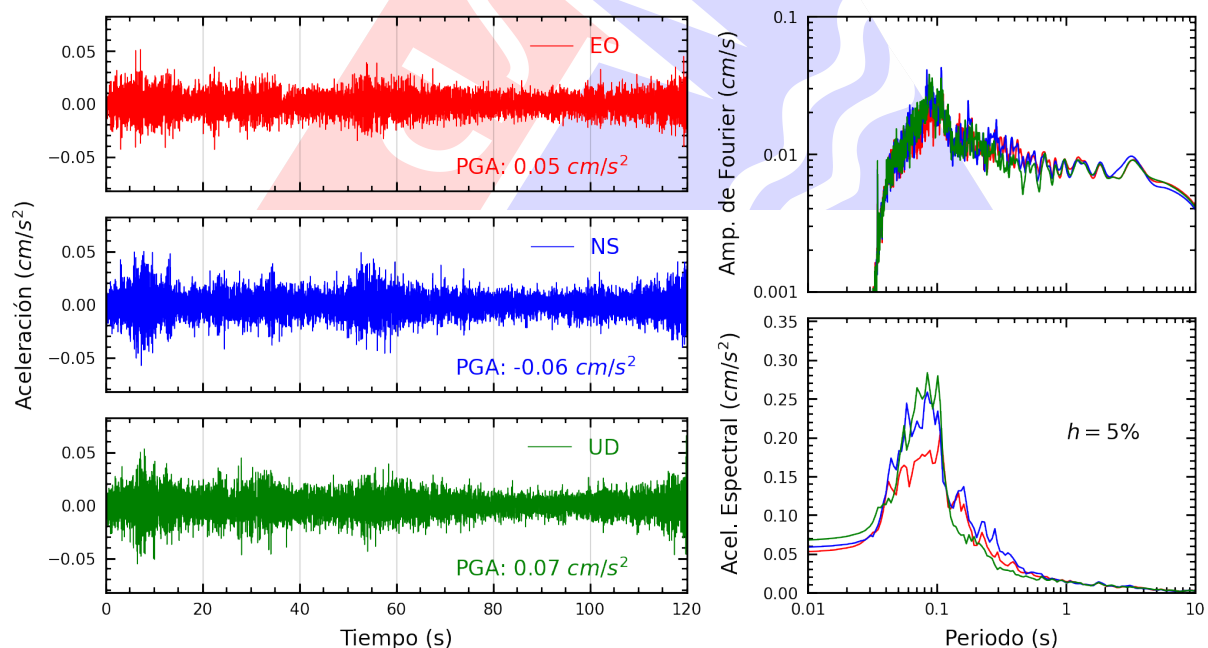
Figura A.36: Registros tiempo-historia, espectros de Fourier y de respuesta en las direcciones EO, NS y vertical de la estación UNICA. Sismo de Huasichanca, Huancayo - Junin del 2025-07-02, 23:57:57 (Hora local)
