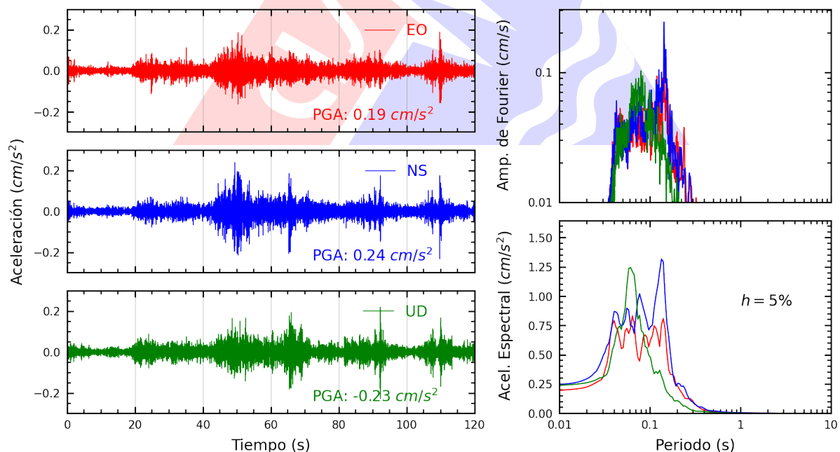
Figura A.12: Registros tiempo-historia, espectros de Fourier y de respuesta en las direcciones EO, NS y vertical de la estación CARAB. Sismo de Huasicancha, Huancayo - Junin del 2025-07-02, 23:57:57 (Hora local)
