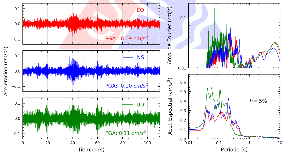
Figura A.26: Registros tiempo-historia, espectros de Fourier y de respuesta en las direcciones EO, NS y vertical de la estación MDPP. Sismo de Huasichanca, Huancayo - Junin del 2025-07-02, 23:57:57 (Hora local)
