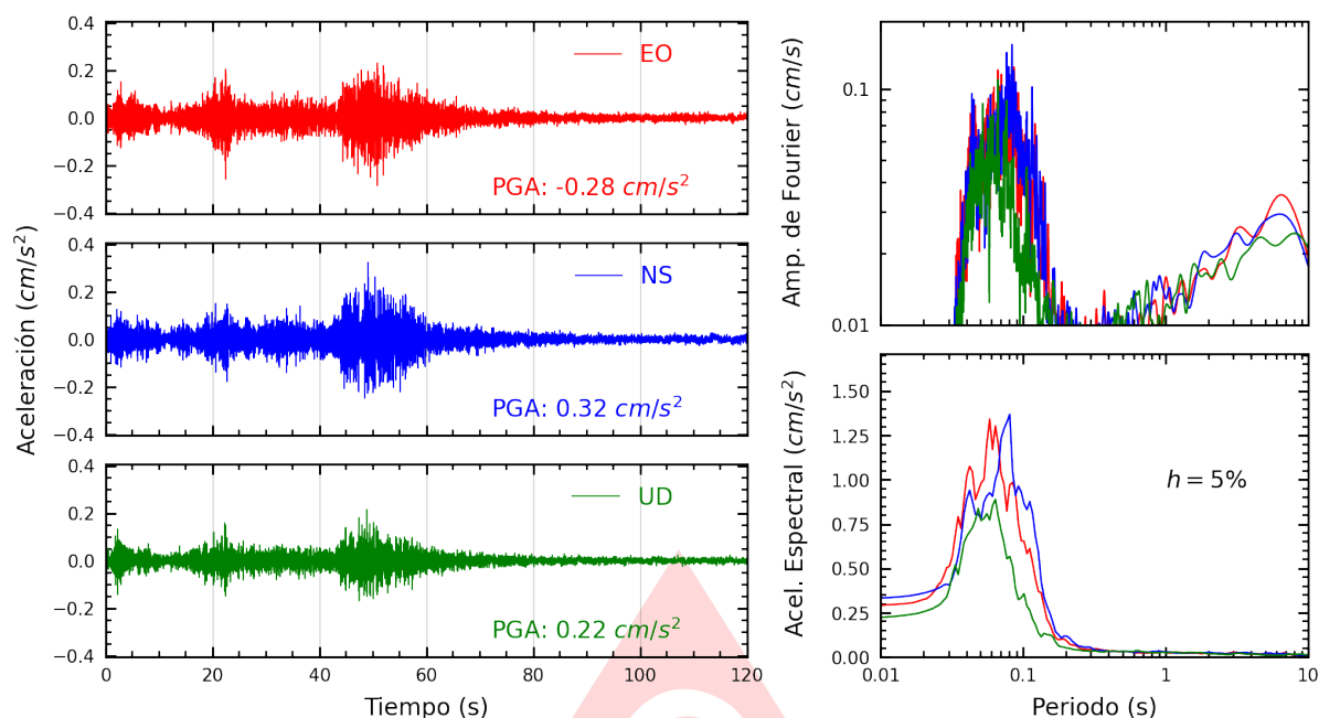
Figura A.7: Registros tiempo-historia, espectros de Fourier y de respuesta en las direcciones EO, NS y vertical de la estación JOSEO. Sismo de Huasicancha, Huancayo - Junin del 2025-07-02, 23:57:57 (Hora local)
