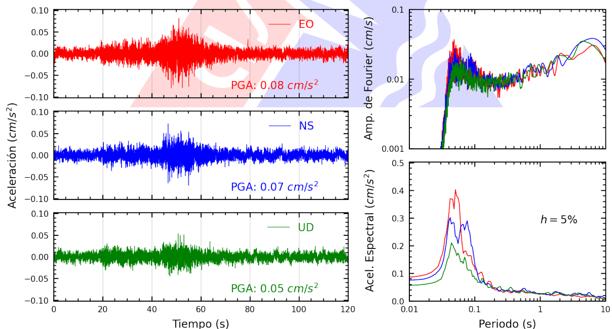
Figura A.34: Registros tiempo-historia, espectros de Fourier y de respuesta en las direcciones EO, NS y vertical de la estación UCSS. Sismo de Huasichanca, Huancayo - Junin del 2025-07-02, 23:57:57 (Hora local)
