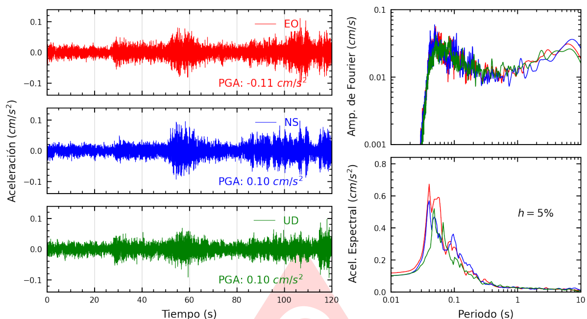
Figura A.21: Registros tiempo-historia, espectros de Fourier y de respuesta en las direcciones EO, NS y vertical de la estación IMCA. Sismo de Huasichanca, Huancayo - Junin del 2025-07-02, 23:57:57 (Hora local)
