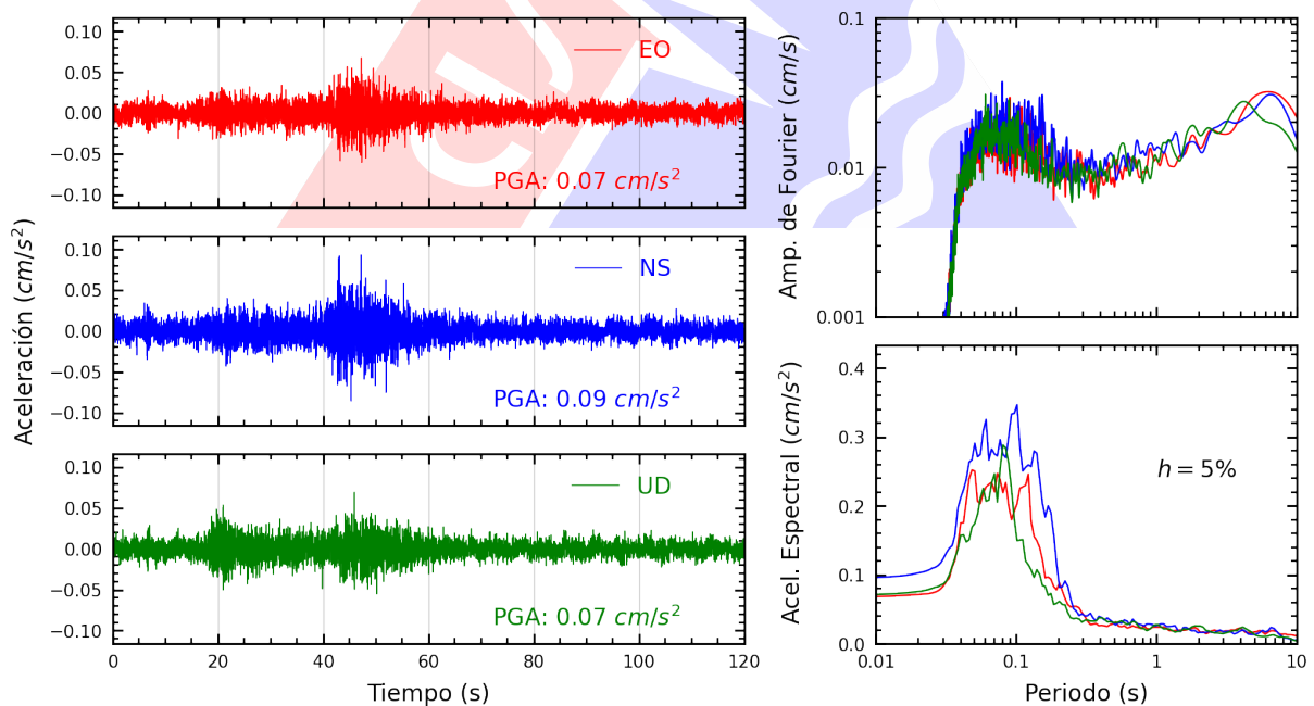
Figura A.30: Registros tiempo-historia, espectros de Fourier y de respuesta en las direcciones EO, NS y vertical de la estación SERVI. Sismo de Huasicancha, Huancayo - Junin del 2025-07-02, 23:57:57 (Hora local)
