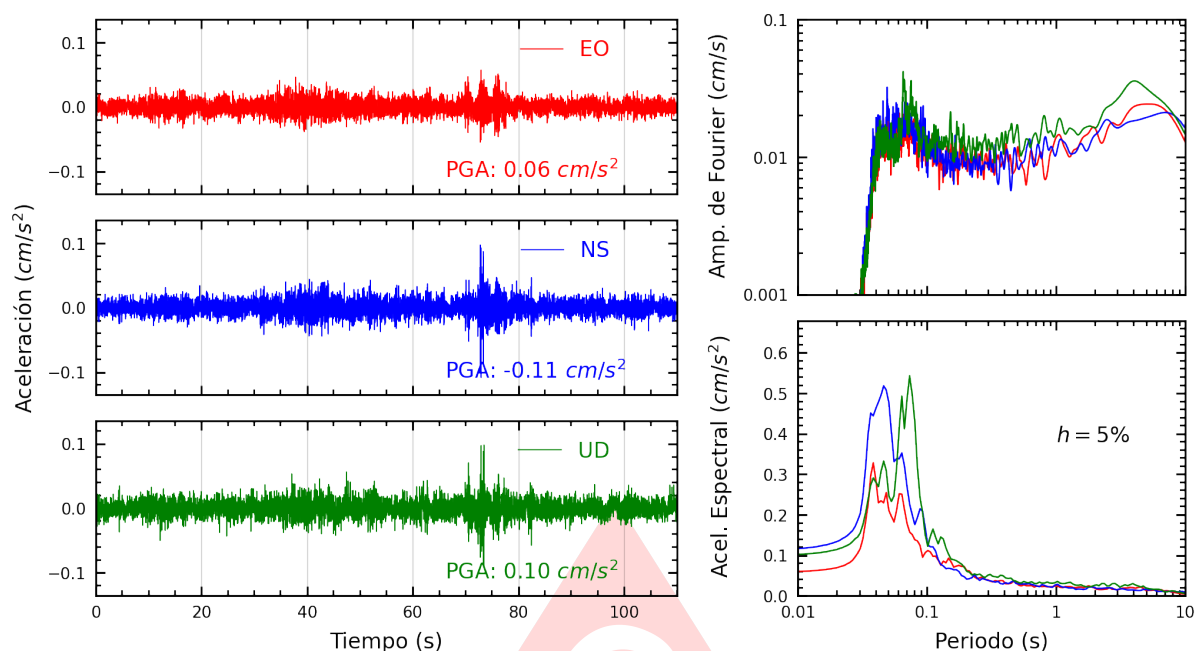
Figura A.25: Registros tiempo-historia, espectros de Fourier y de respuesta en las direcciones EO, NS y vertical de la estación UNFV. Sismo de Huasichanca, Huancayo - Junin del 2025-07-02, 23:57:57 (Hora local)
