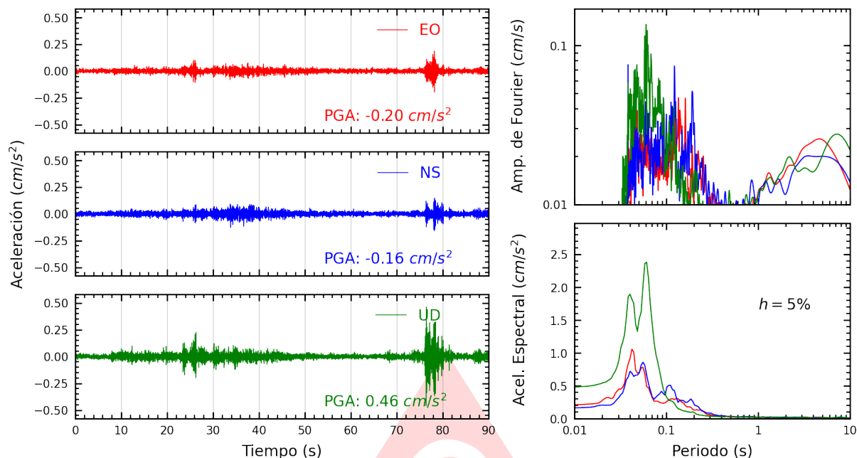
Figura A.3: Registros tiempo-historia, espectros de Fourier y de respuesta en las direcciones EO, NS y vertical de la estación SOCHO. Sismo de Huasichanca, Huancayo - Junin del 2025-07-02, 23:57:57 (Hora local)
