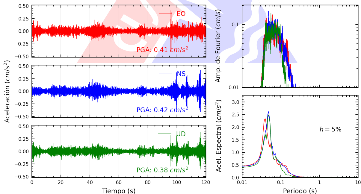
Figura A.4: Registros tiempo-historia, espectros de Fourier y de respuesta en las direcciones EO, NS y vertical de la estación SROSA. Sismo de Huasichanca, Huancayo - Junin del 2025-07-02, 23:57:57 (Hora local)
