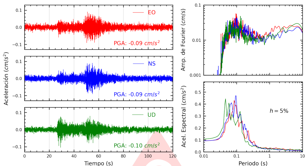
Figura A.27: Registros tiempo-historia, espectros de Fourier y de respuesta en las direcciones EO, NS y vertical de la estación USILP. Sismo de Huasichanca, Huancayo - Junin del 2025-07-02, 23:57:57 (Hora local)
