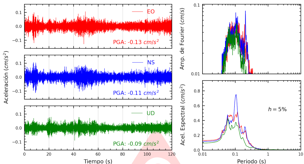
Figura A.17: Registros tiempo-historia, espectros de Fourier y de respuesta en las direcciones EO, NS y vertical de la estación SCCHO. Sismo de Huasicancha, Huancayo - Junin del 2025-07-02, 23:57:57 (Hora local)
