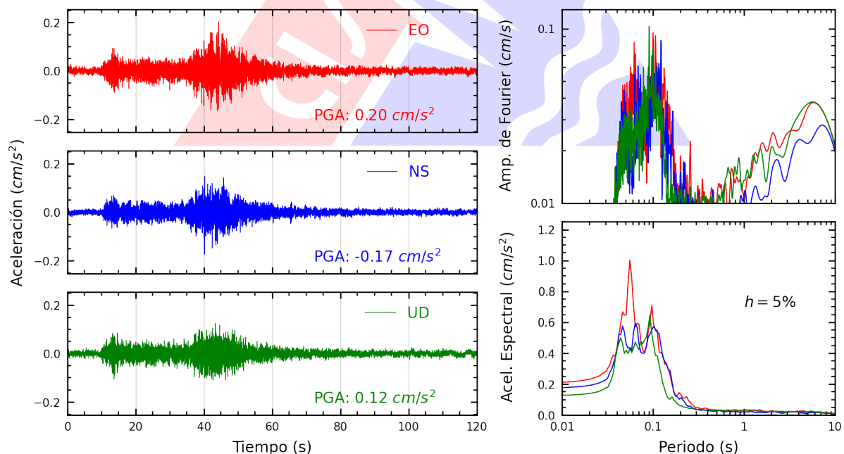
Figura A.14: Registros tiempo-historia, espectros de Fourier y de respuesta en las direcciones EO, NS y vertical de la estación AMORE. Sismo de Huasicancha, Huancayo - Junin del 2025-07-02, 23:57:57 (Hora local)
