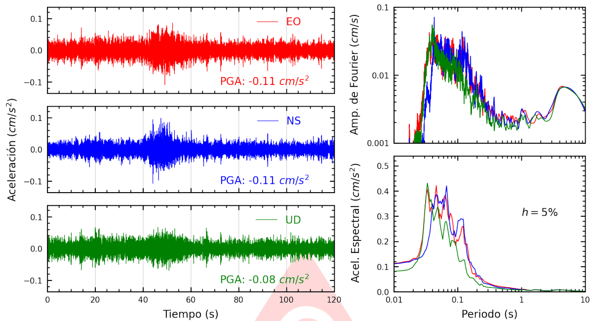
Figura A.23: Registros tiempo-historia, espectros de Fourier y de respuesta en las direcciones EO, NS y vertical de la estación ATARJ. Sismo de Huasichanca, Huancayo - Junin del 2025-07-02, 23:57:57 (Hora local)
