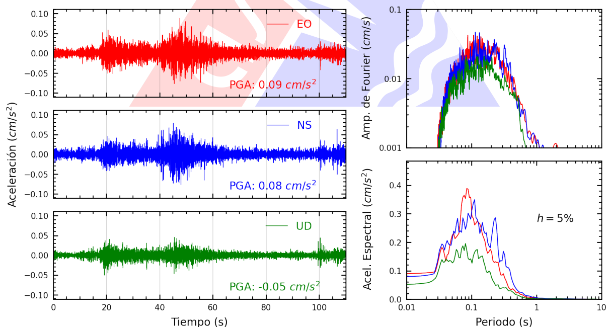
Figura A.32: Registros tiempo-historia, espectros de Fourier y de respuesta en las direcciones EO, NS y vertical de la estación BRIS2. Sismo de Huasicancha, Huancayo - Junin del 2025-07-02, 23:57:57 (Hora local)
