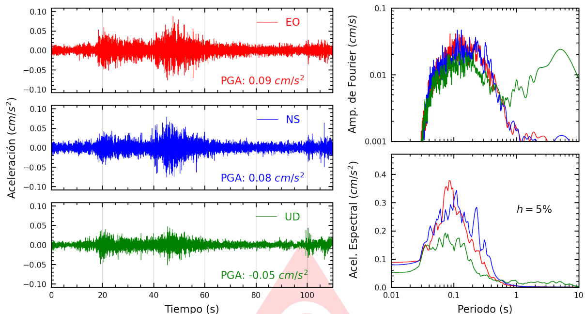
Figura A.33: Registros tiempo-historia, espectros de Fourier y de respuesta en las direcciones EO, NS y vertical de la estación BRISA. Sismo de Huasichanca, Huancayo - Junin del 2025-07-02, 23:57:57 (Hora local)
