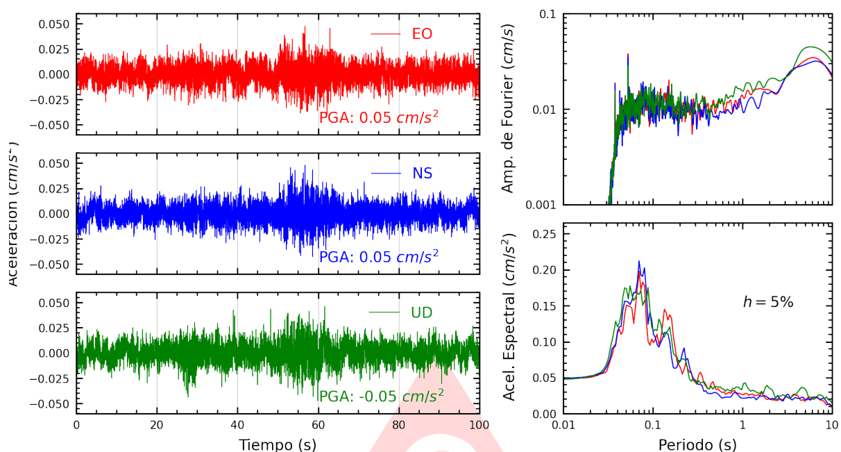
Figura A.37: Registros tiempo-historia, espectros de Fourier y de respuesta en las direcciones EO, NS y vertical de la estación UNMSM. Sismo de Huasicancha, Huancayo - Junin del 2025-07-02, 23:57:57 (Hora local)
