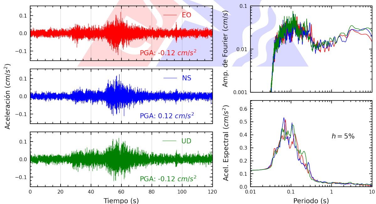
Figura A.18: Registros tiempo-historia, espectros de Fourier y de respuesta en las direcciones EO, NS y vertical de la estación SOVES. Sismo de Huasicancha, Huancayo - Junin del 2025-07-02, 23:57:57 (Hora local)
