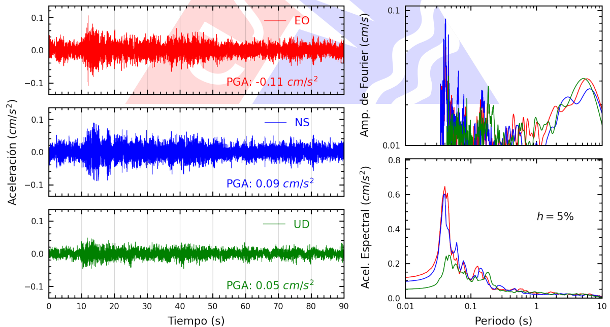
Figura A.24: Registros tiempo-historia, espectros de Fourier y de respuesta en las direcciones EO, NS y vertical de la estación DHNPE. Sismo de Huasichanca, Huancayo - Junin del 2025-07-02, 23:57:57 (Hora local)
