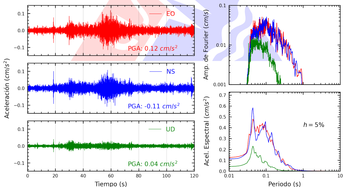
Figura A.20: Registros tiempo-historia, espectros de Fourier y de respuesta en las direcciones EO, NS y vertical de la estación UCVAT. Sismo de Huasichanca, Huancayo - Junin del 2025-07-02, 23:57:57 (Hora local)
