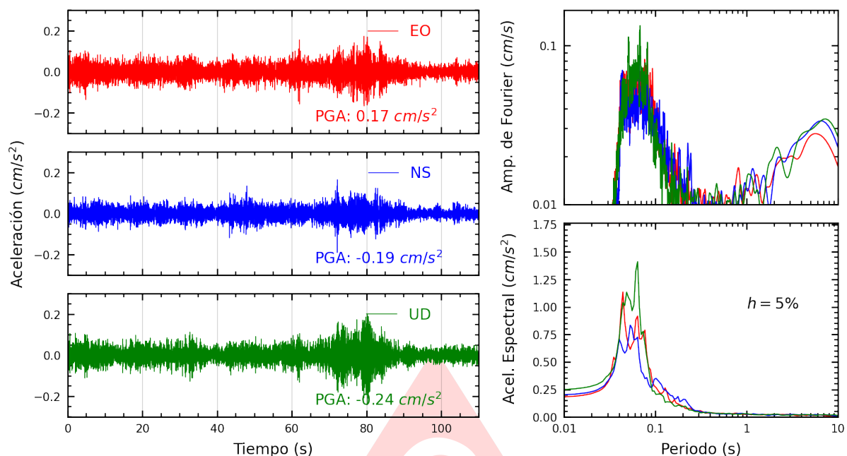
Figura A.11: Registros tiempo-historia, espectros de Fourier y de respuesta en las direcciones EO, NS y vertical de la estación URPE. Sismo de Huasicancha, Huancayo - Junin del 2025-07-02, 23:57:57 (Hora local)
