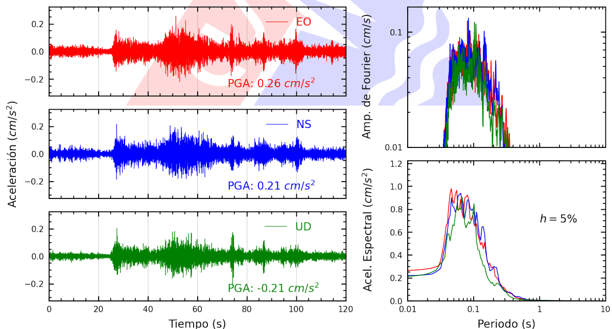
Figura A.10: Registros tiempo-historia, espectros de Fourier y de respuesta en las direcciones EO, NS y vertical de la estación PHERM. Sismo de Huasicancha, Huancayo - Junin del 2025-07-02, 23:57:57 (Hora local)
