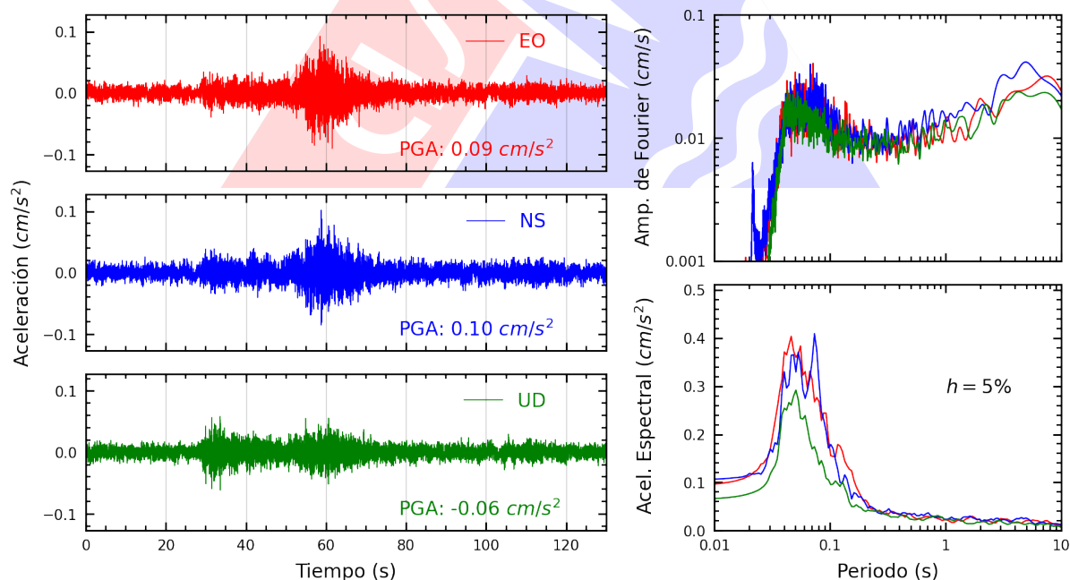
Figura A.28: Registros tiempo-historia, espectros de Fourier y de respuesta en las direcciones EO, NS y vertical de la estación SJLCE. Sismo de Huasichanca, Huancayo - Junin del 2025-07-02, 23:57:57 (Hora local)
