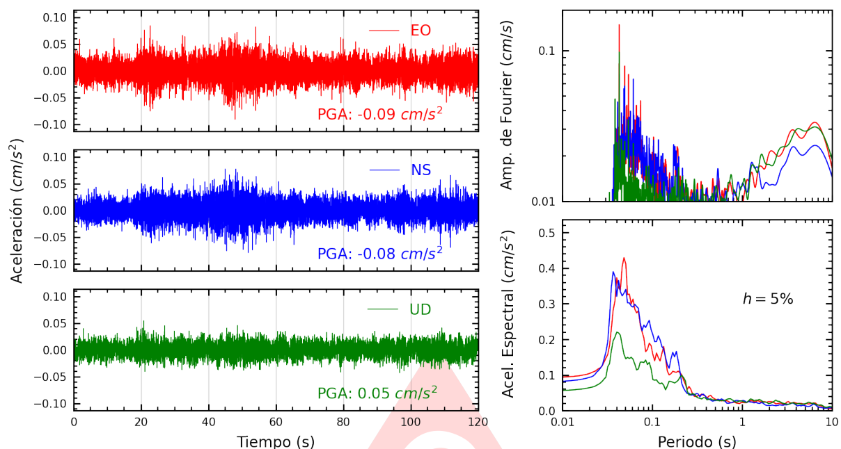
Figura A.31: Registros tiempo-historia, espectros de Fourier y de respuesta en las direcciones EO, NS y vertical de la estación UPCVI. Sismo de Huasicancha, Huancayo - Junin del 2025-07-02, 23:57:57 (Hora local)
