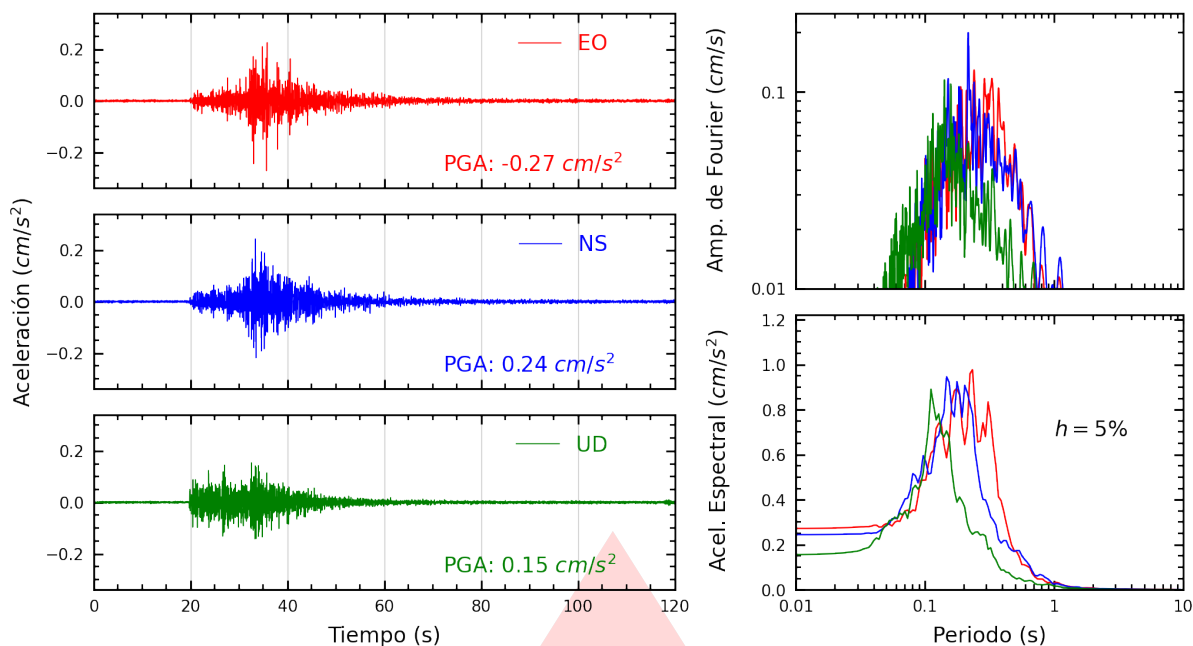
Figura A.1: Registros tiempo-historia, espectros de Fourier y de respuesta en las direcciones EO, NS y vertical de la estación UNP. Sismo de Sechura, Sechura - Piura del 2025-07-03, 01:52:34 (Hora local)
