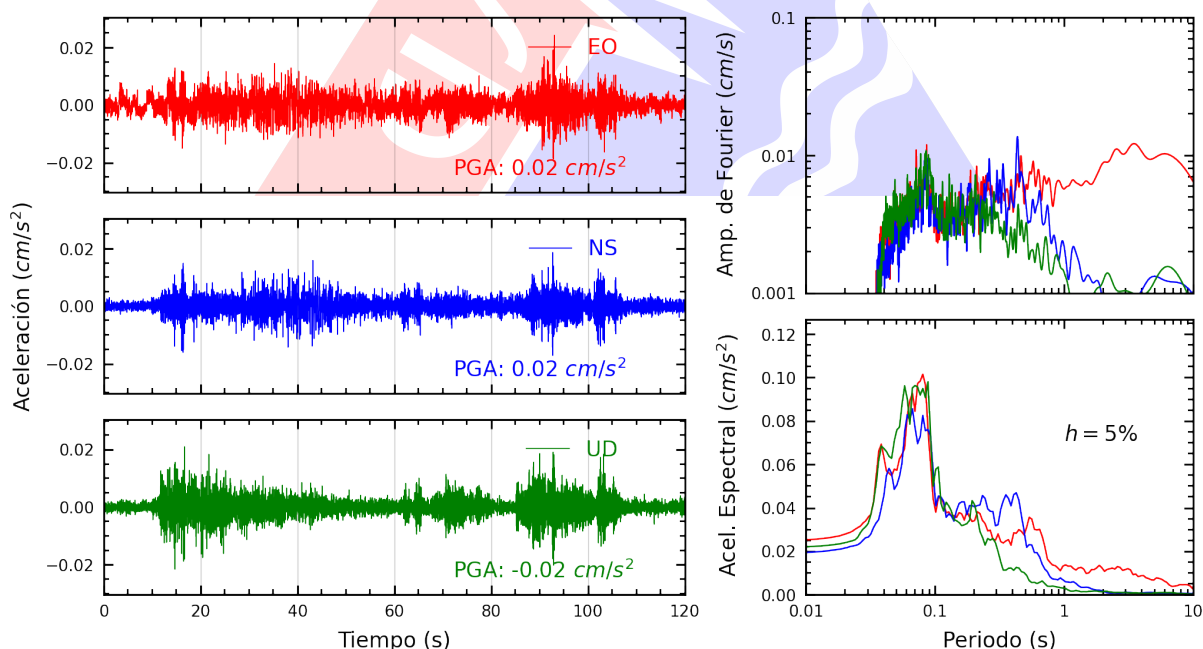
Figura A.4: Registros tiempo-historia, espectros de Fourier y de respuesta en las direcciones EO, NS y vertical de la estación SCCHI. Sismo de Sechura, Sechura - Piura del 2025-07-03, 01:52:34 (Hora local)
