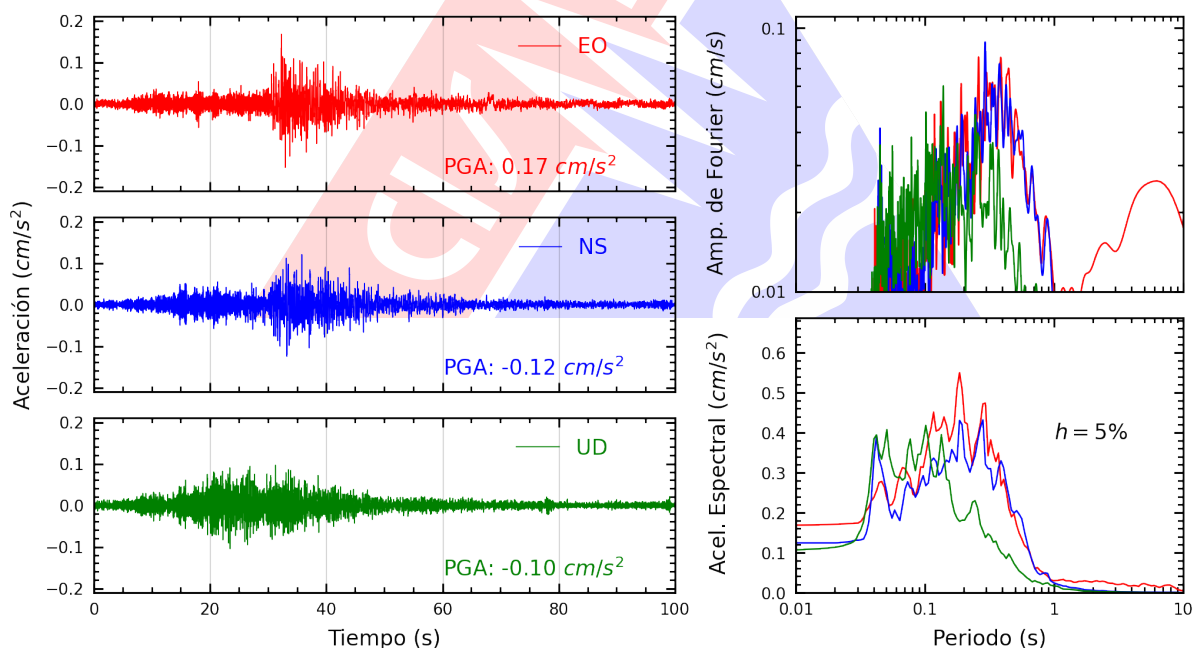
Figura A.2: Registros tiempo-historia, espectros de Fourier y de respuesta en las direcciones EO, NS y vertical de la estación SCPIU. Sismo de Sechura, Sechura - Piura del 2025-07-03, 01:52:34 (Hora local)
