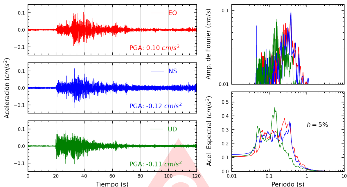
Figura A.3: Registros tiempo-historia, espectros de Fourier y de respuesta en las direcciones EO, NS y vertical de la estación UPAOP. Sismo de Sechura, Sechura - Piura del 2025-07-03, 01:52:34 (Hora local)
