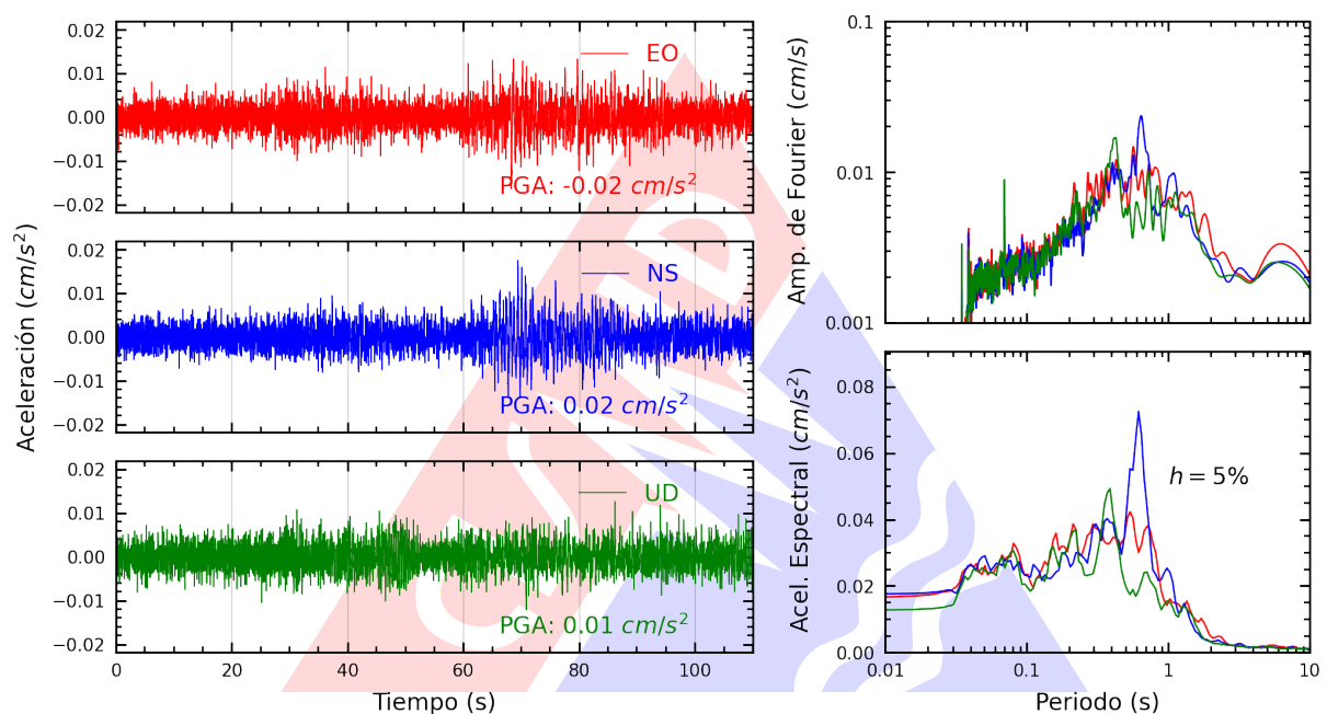
Figura A.5: Registros tiempo-historia, espectros de Fourier y de respuesta en las direcciones EO, NS y vertical de la estación UNC. Sismo de Sechura, Sechura - Piura del 2025-07-03, 01:52:34 (Hora local)
