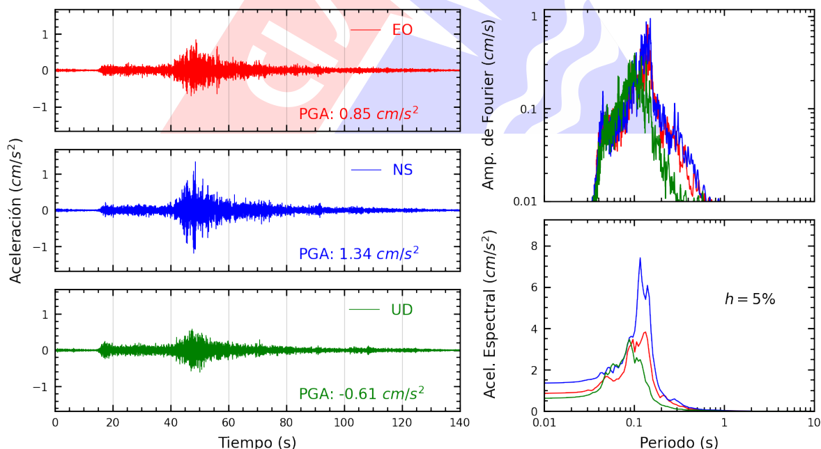
Figura A.6: Registros tiempo-historia, espectros de Fourier y de respuesta en las direcciones EO, NS y vertical de la estación CARAB. Sismo de Huancano, Pisco - Ica del 2025-07-03, 04:50:10 (Hora local)
