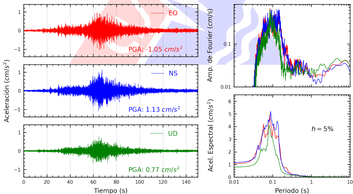
Figura A.10: Registros tiempo-historia, espectros de Fourier y de respuesta en las direcciones EO, NS y vertical de la estación USILM. Sismo de Huancano, Pisco - Ica del 2025-07-03, 04:50:10 (Hora local)
