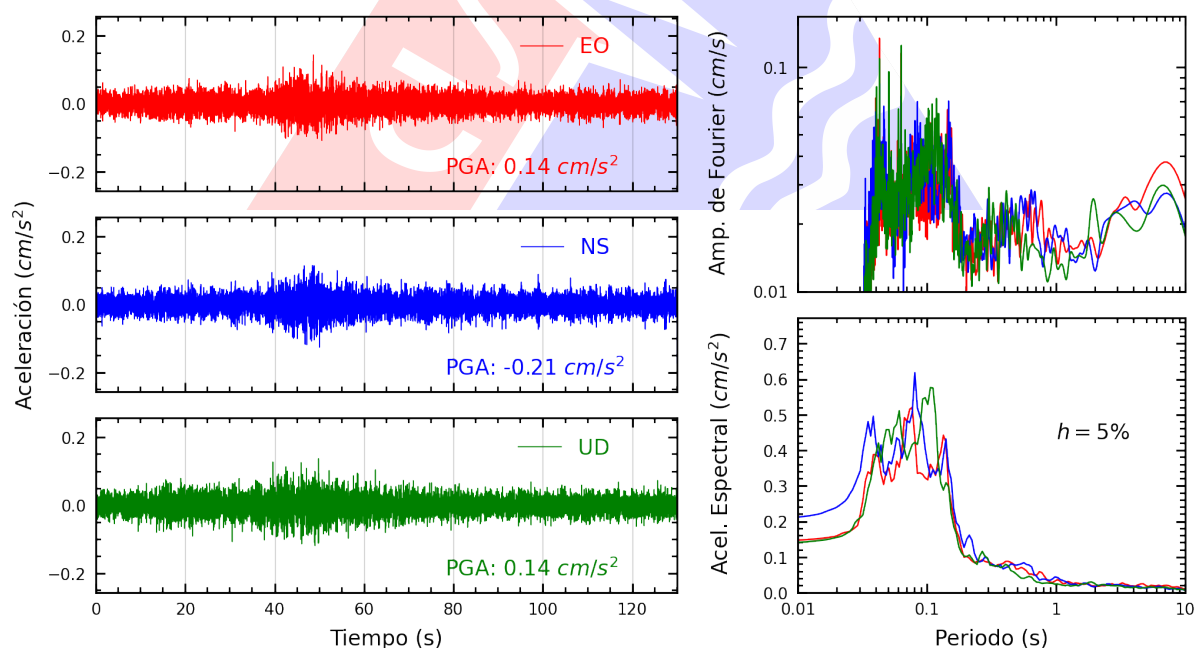
Figura A.42: Registros tiempo-historia, espectros de Fourier y de respuesta en las direcciones EO, NS y vertical de la estación BONDY. Sismo de Huancano, Pisco - Ica del 2025-07-03, 04:50:10 (Hora local)
