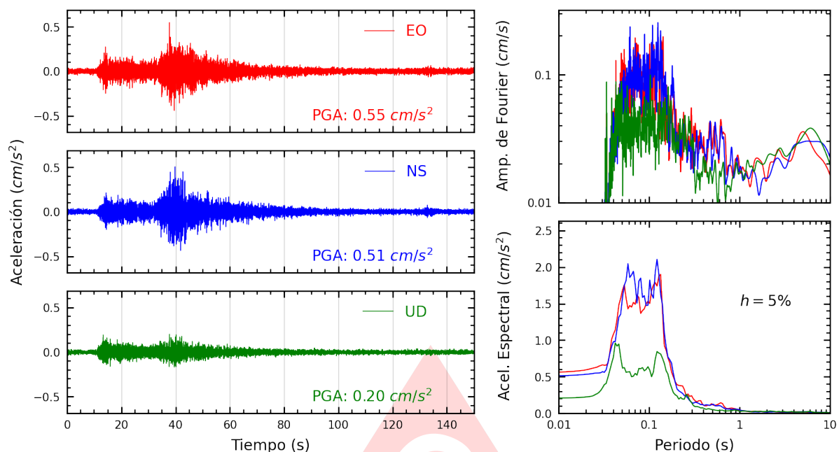
Figura A.21: Registros tiempo-historia, espectros de Fourier y de respuesta en las direcciones EO, NS y vertical de la estación UPCVI. Sismo de Huancano, Pisco - Ica del 2025-07-03, 04:50:10 (Hora local)
