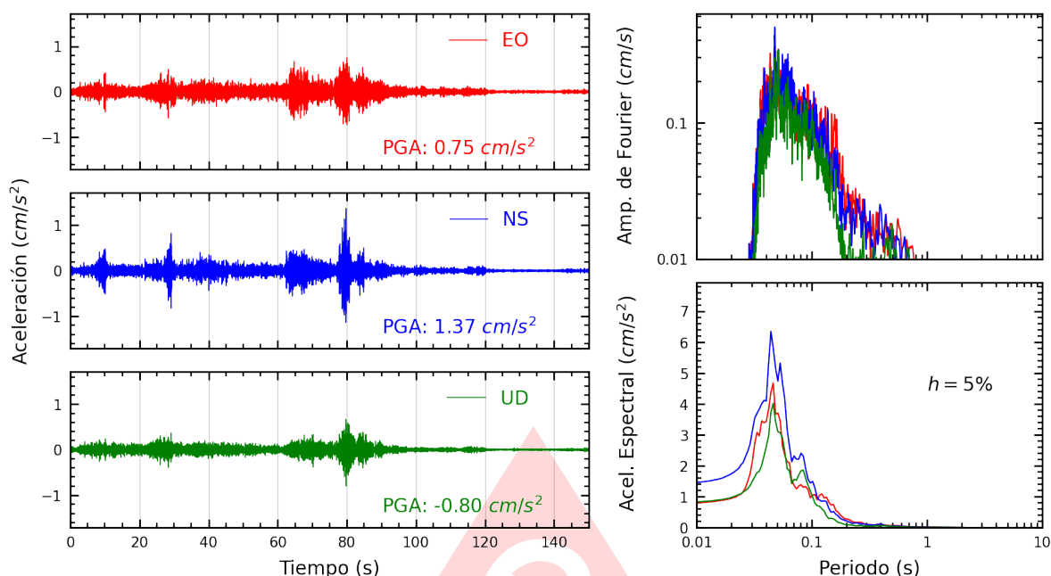
Figura A.5: Registros tiempo-historia, espectros de Fourier y de respuesta en las direcciones EO, NS y vertical de la estación PACHA. Sismo de Huancano, Pisco - Ica del 2025-07-03, 04:50:10 (Hora local)
