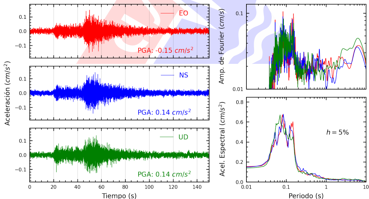
Figura A.48: Registros tiempo-historia, espectros de Fourier y de respuesta en las direcciones EO, NS y vertical de la estación UNMSM. Sismo de Huancano, Pisco - Ica del 2025-07-03, 04:50:10 (Hora local)
