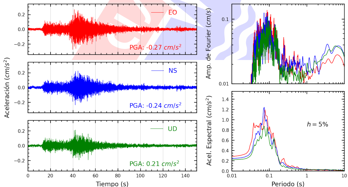
Figura A.40: Registros tiempo-historia, espectros de Fourier y de respuesta en las direcciones EO, NS y vertical de la estación CEPRE. Sismo de Huancano, Pisco - Ica del 2025-07-03, 04:50:10 (Hora local)
