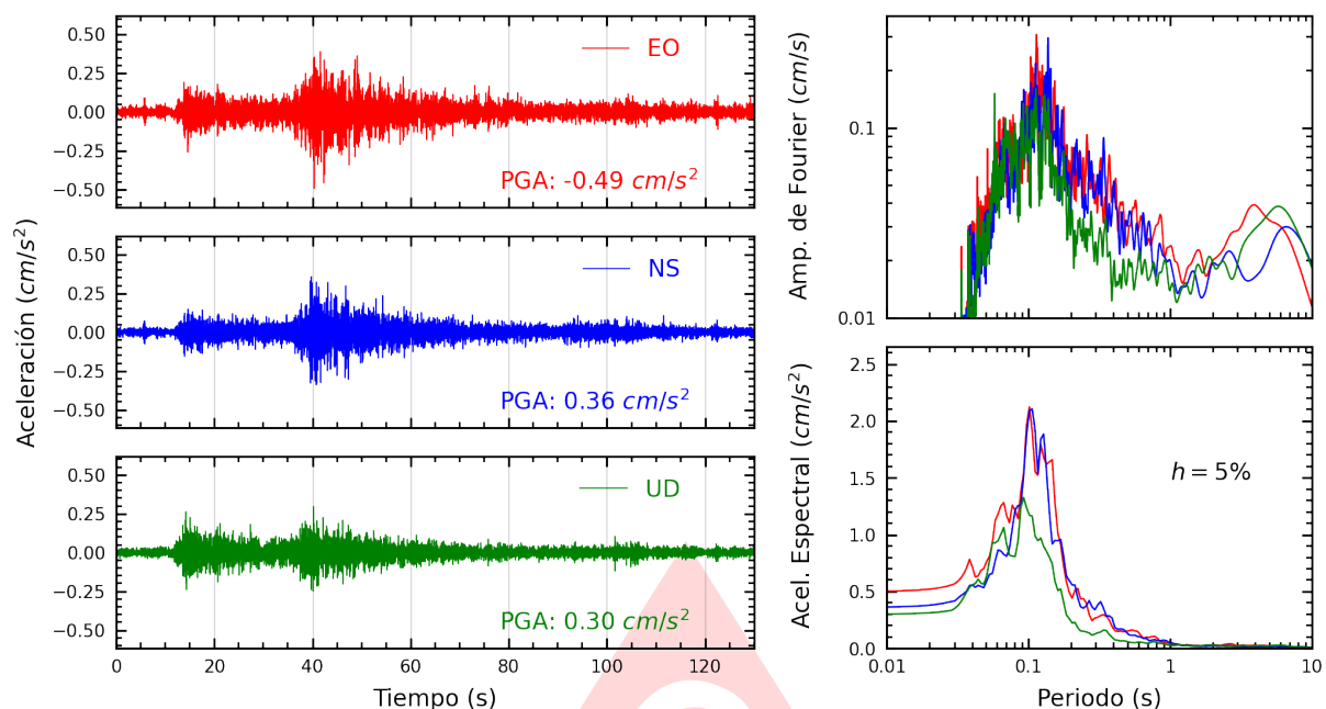
Figura A.25: Registros tiempo-historia, espectros de Fourier y de respuesta en las direcciones EO, NS y vertical de la estación SOBAR. Sismo de Huancano, Pisco - Ica del 2025-07-03, 04:50:10 (Hora local)
