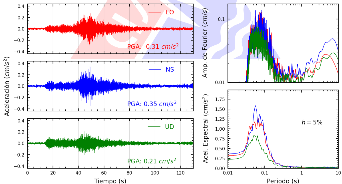
Figura A.32: Registros tiempo-historia, espectros de Fourier y de respuesta en las direcciones EO, NS y vertical de la estación SJLCE. Sismo de Huancano, Pisco - Ica del 2025-07-03, 04:50:10 (Hora local)
