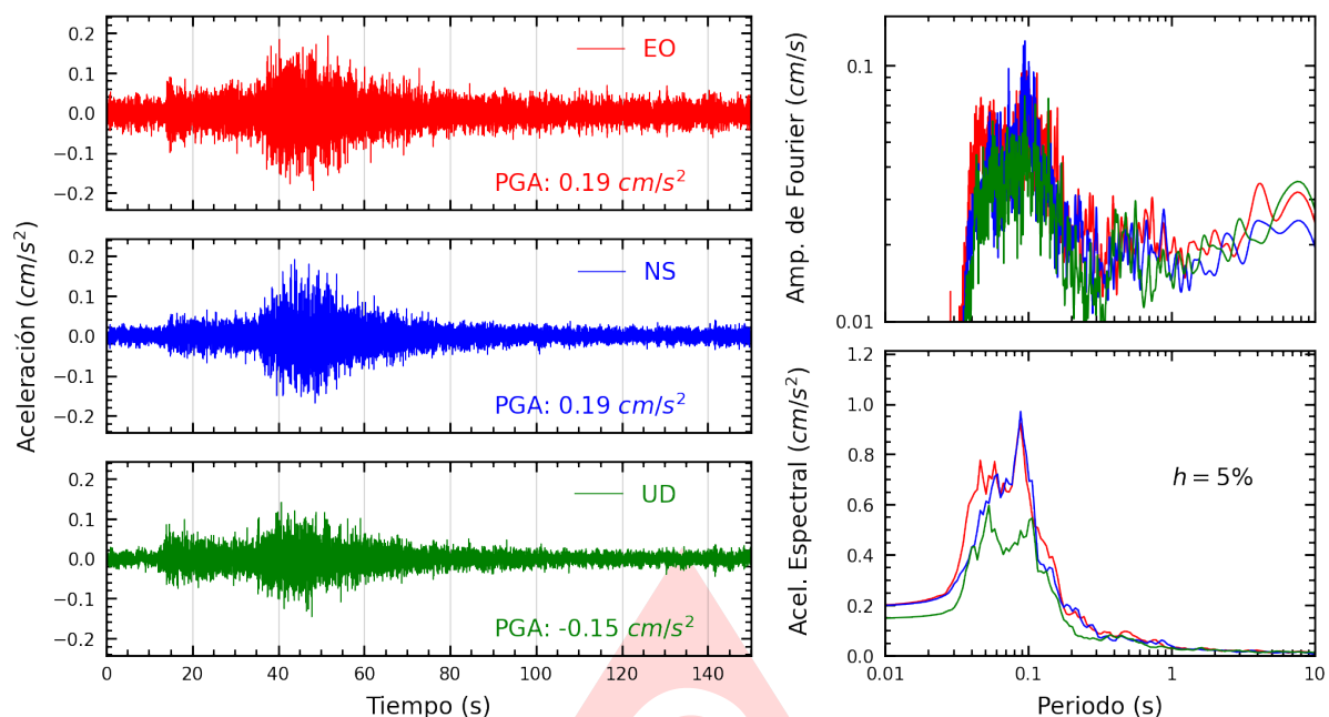
Figura A.43: Registros tiempo-historia, espectros de Fourier y de respuesta en las direcciones EO, NS y vertical de la estación INICT. Sismo de Huancano, Pisco - Ica del 2025-07-03, 04:50:10 (Hora local)
