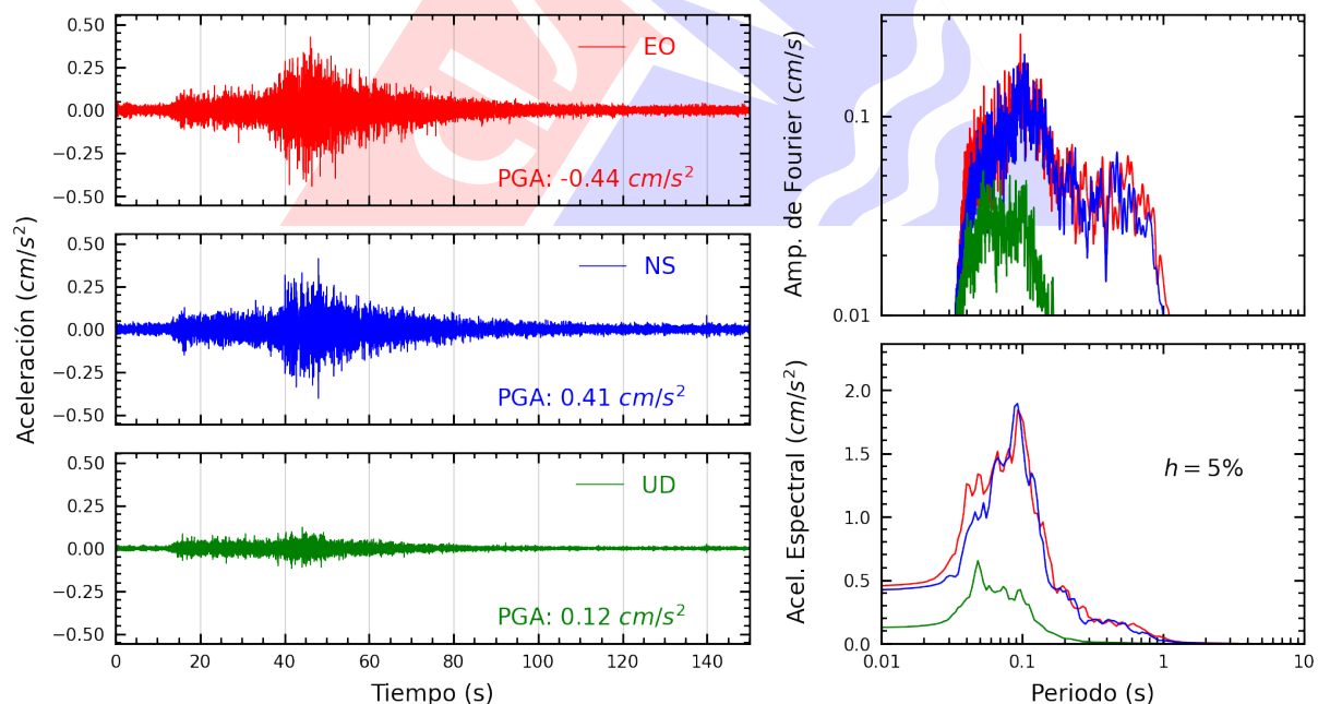
Figura A.26: Registros tiempo-historia, espectros de Fourier y de respuesta en las direcciones EO, NS y vertical de la estación UCVAT. Sismo de Huancano, Pisco - Ica del 2025-07-03, 04:50:10 (Hora local)
