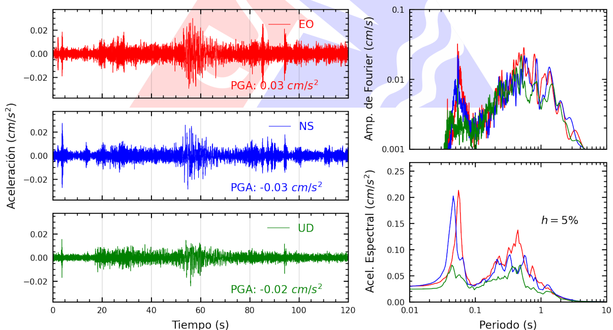
Figura A.50: Registros tiempo-historia, espectros de Fourier y de respuesta en las direcciones EO, NS y vertical de la estación UNMBA. Sismo de Huancano, Pisco - Ica del 2025-07-03, 04:50:10 (Hora local)
