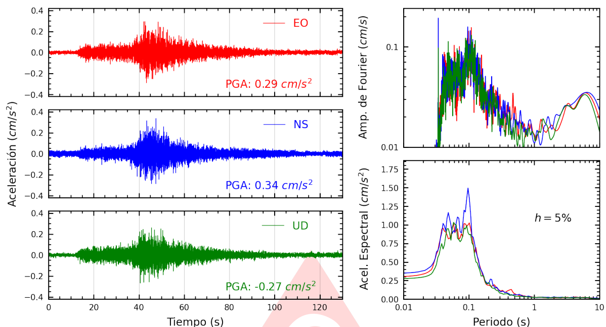
Figura A.33: Registros tiempo-historia, espectros de Fourier y de respuesta en las direcciones EO, NS y vertical de la estación USMP. Sismo de Huancano, Pisco - Ica del 2025-07-03, 04:50:10 (Hora local)
