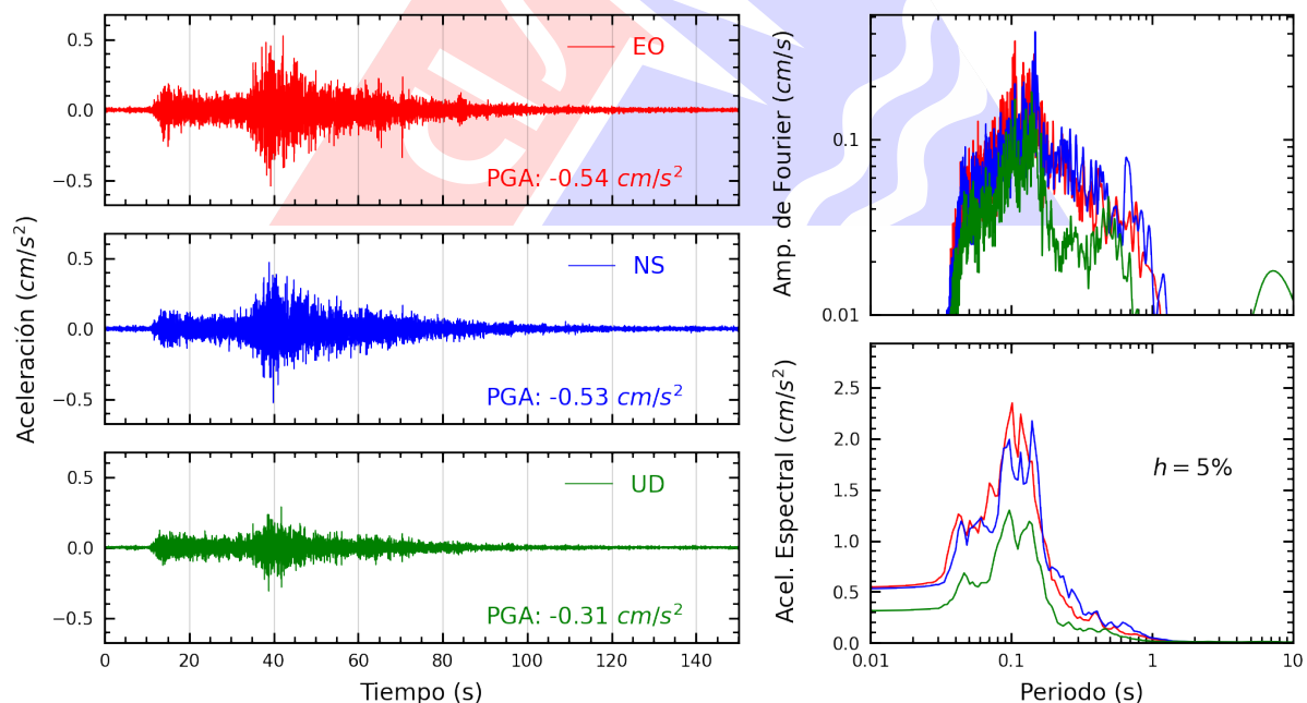
Figura A.22: Registros tiempo-historia, espectros de Fourier y de respuesta en las direcciones EO, NS y vertical de la estación BRISA. Sismo de Huancano, Pisco - Ica del 2025-07-03, 04:50:10 (Hora local)
