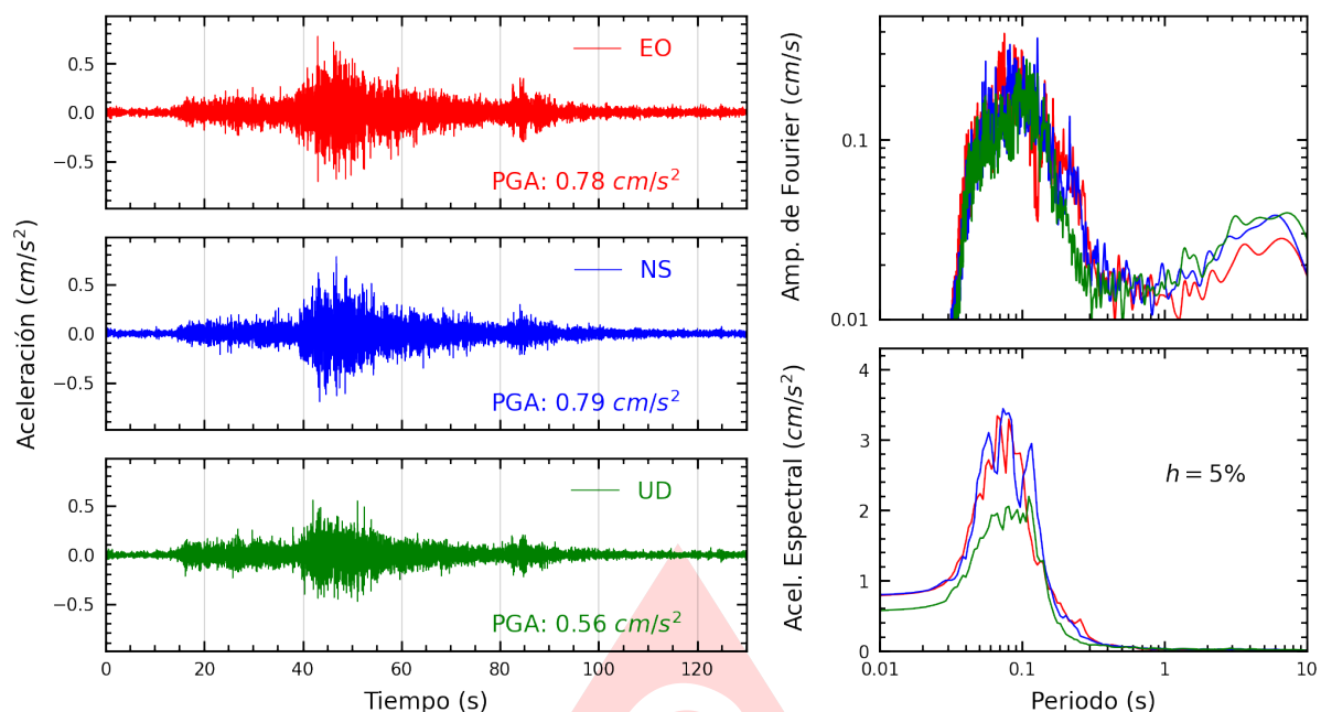
Figura A.15: Registros tiempo-historia, espectros de Fourier y de respuesta en las direcciones EO, NS y vertical de la estación INDEP. Sismo de Huancano, Pisco - Ica del 2025-07-03, 04:50:10 (Hora local)
