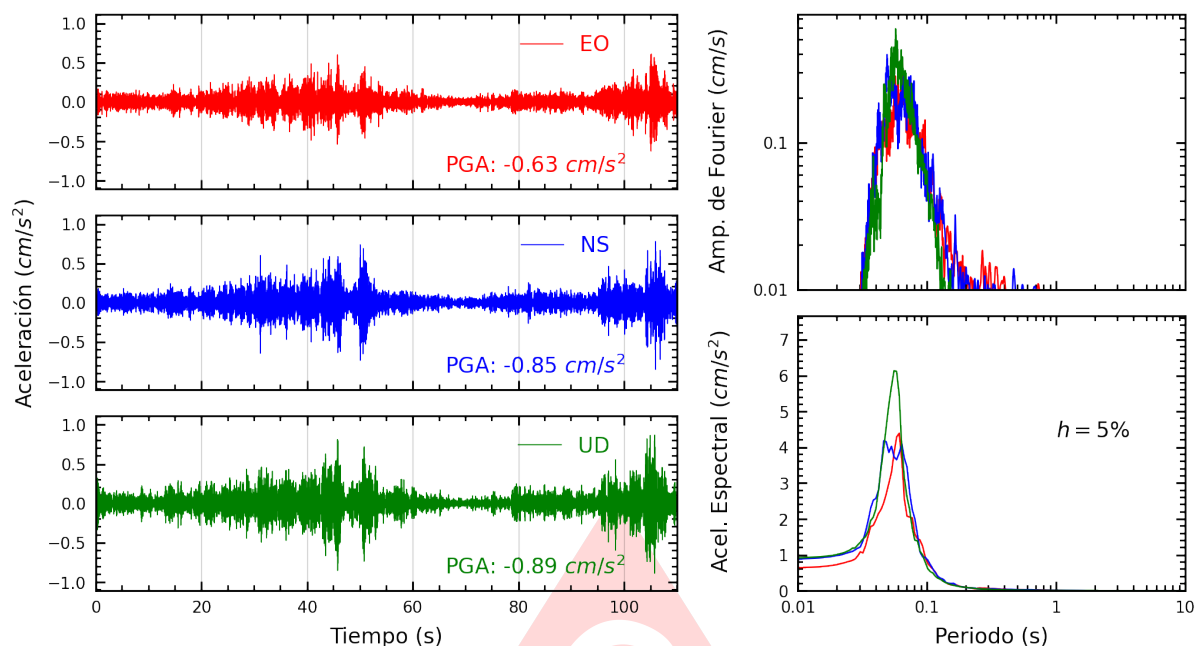
Figura A.13: Registros tiempo-historia, espectros de Fourier y de respuesta en las direcciones EO, NS y vertical de la estación SCAR2. Sismo de Huancano, Pisco - Ica del 2025-07-03, 04:50:10 (Hora local)
