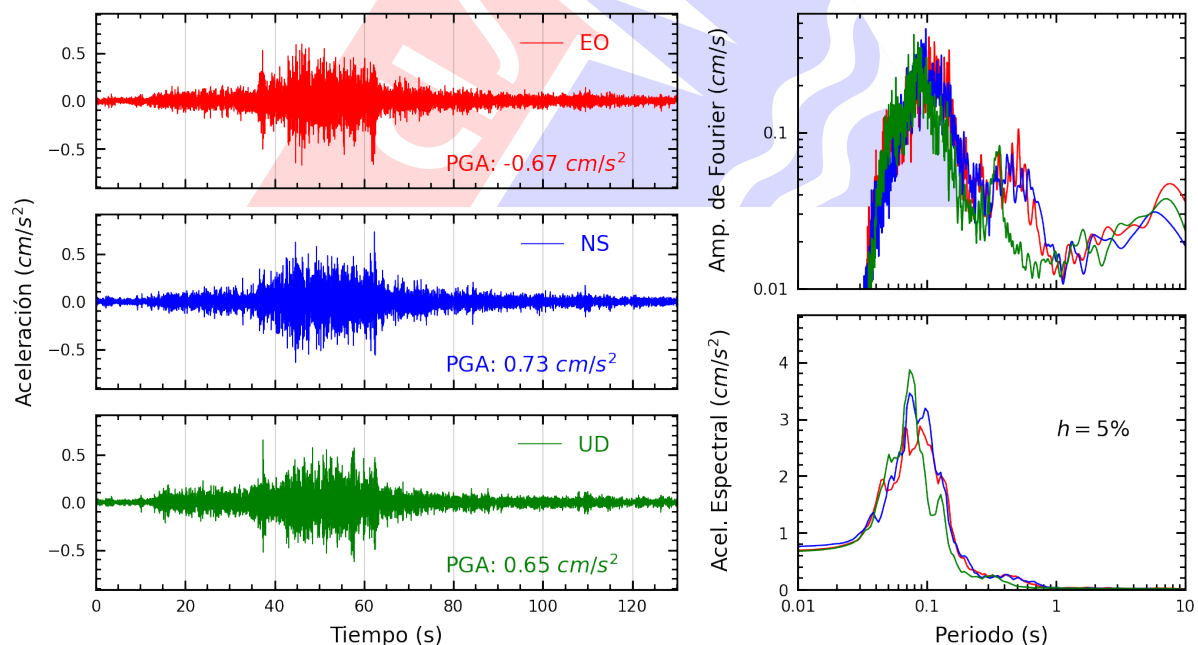
Figura A.16: Registros tiempo-historia, espectros de Fourier y de respuesta en las direcciones EO, NS y vertical de la estación SJLSV. Sismo de Huancano, Pisco - Ica del 2025-07-03, 04:50:10 (Hora local)
