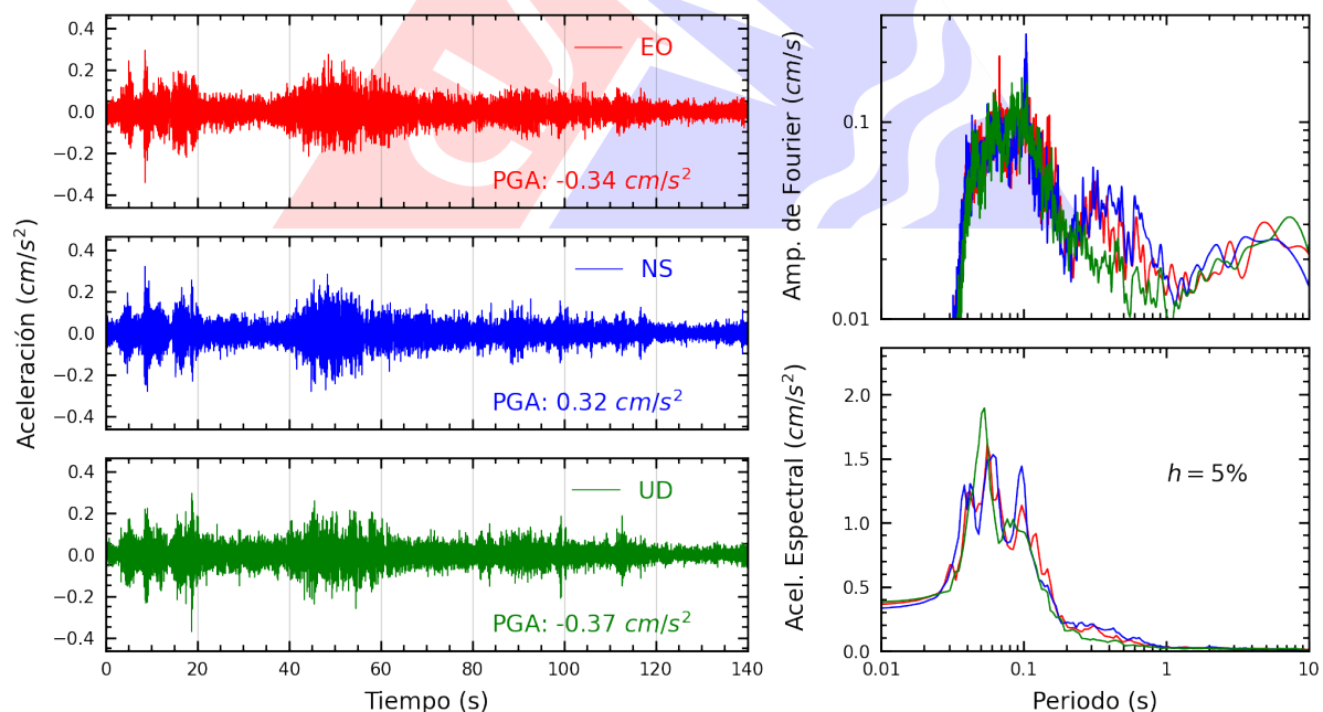
Figura A.30: Registros tiempo-historia, espectros de Fourier y de respuesta en las direcciones EO, NS y vertical de la estación MADRE. Sismo de Huancano, Pisco - Ica del 2025-07-03, 04:50:10 (Hora local)
