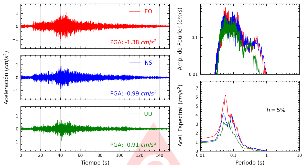
Figura A.3: Registros tiempo-historia, espectros de Fourier y de respuesta en las direcciones EO, NS y vertical de la estación UNTEL. Sismo de Huancano, Pisco - Ica del 2025-07-03, 04:50:10 (Hora local)
