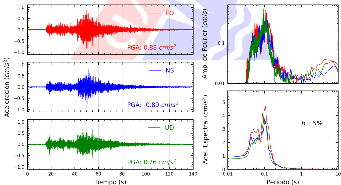
Figura A.14: Registros tiempo-historia, espectros de Fourier y de respuesta en las direcciones EO, NS y vertical de la estación AMORE. Sismo de Huancano, Pisco - Ica del 2025-07-03, 04:50:10 (Hora local)
