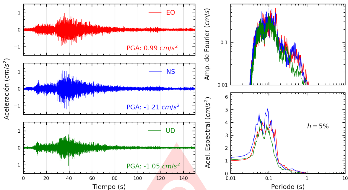
Figura A.9: Registros tiempo-historia, espectros de Fourier y de respuesta en las direcciones EO, NS y vertical de la estación PHERM. Sismo de Huancano, Pisco - Ica del 2025-07-03, 04:50:10 (Hora local)
