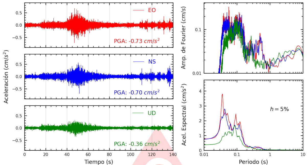
Figura A.17: Registros tiempo-historia, espectros de Fourier y de respuesta en las direcciones EO, NS y vertical de la estación OLIVO. Sismo de Huancano, Pisco - Ica del 2025-07-03, 04:50:10 (Hora local)
