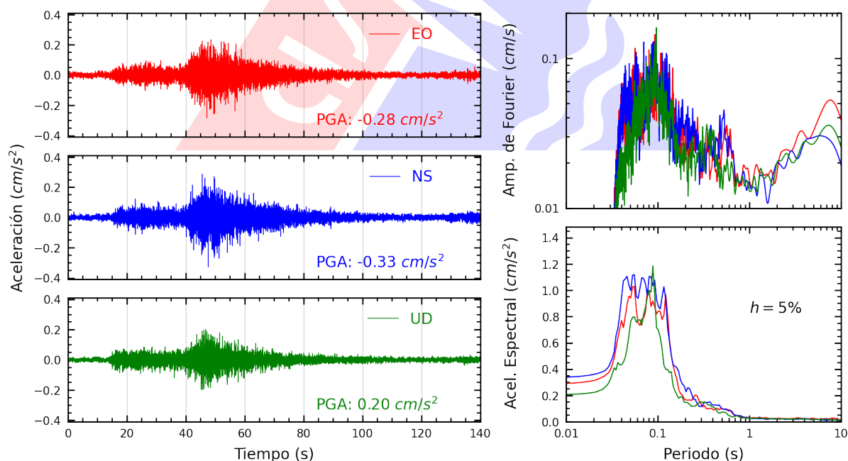
Figura A.36: Registros tiempo-historia, espectros de Fourier y de respuesta en las direcciones EO, NS y vertical de la estación COMAS. Sismo de Huancano, Pisco - Ica del 2025-07-03, 04:50:10 (Hora local)
