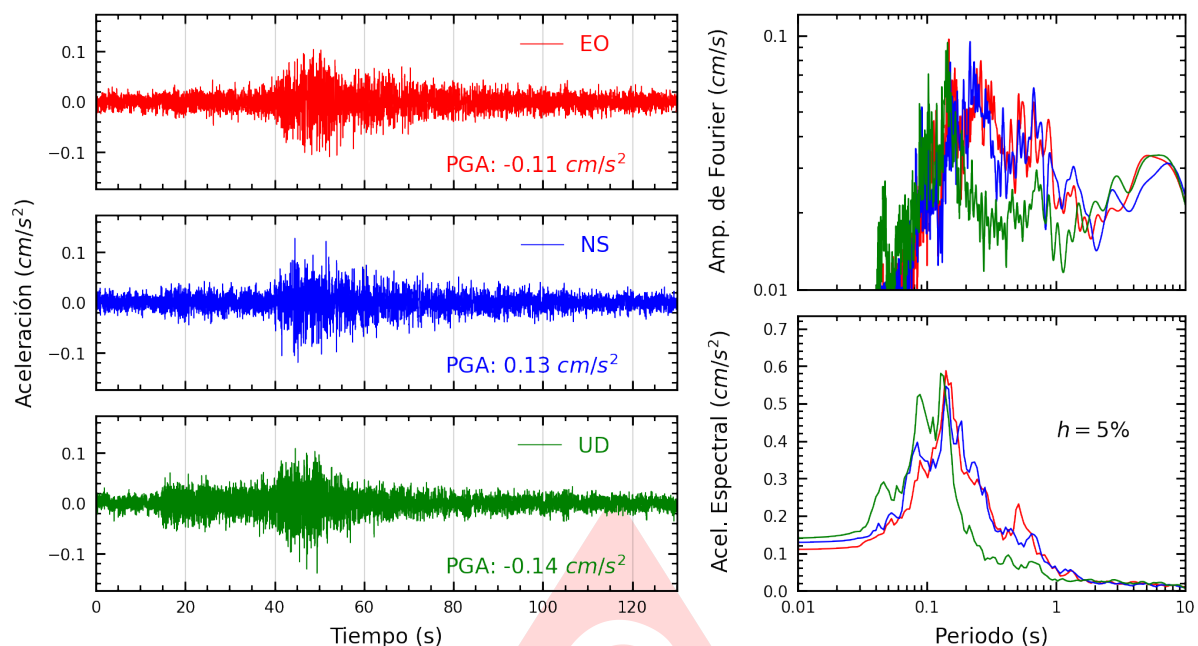
Figura A.49: Registros tiempo-historia, espectros de Fourier y de respuesta en las direcciones EO, NS y vertical de la estación DSML. Sismo de Huancano, Pisco - Ica del 2025-07-03, 04:50:10 (Hora local)
