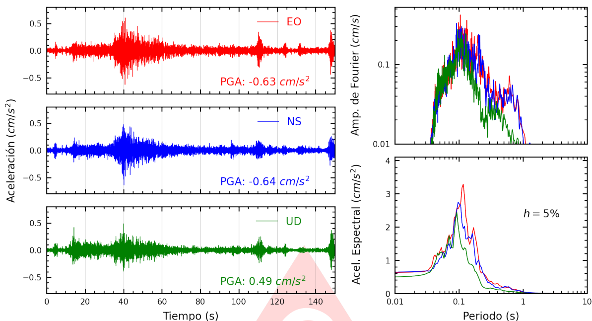
Figura A.19: Registros tiempo-historia, espectros de Fourier y de respuesta en las direcciones EO, NS y vertical de la estación SCCHO. Sismo de Huancano, Pisco - Ica del 2025-07-03, 04:50:10 (Hora local)
