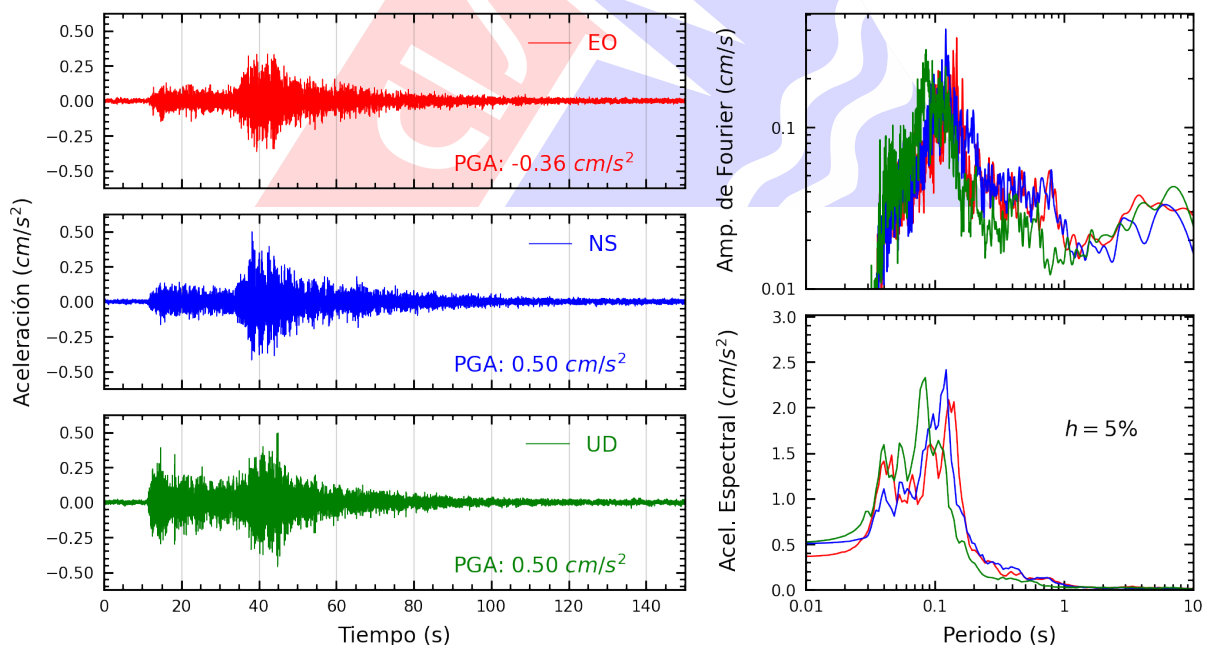
Figura A.24: Registros tiempo-historia, espectros de Fourier y de respuesta en las direcciones EO, NS y vertical de la estación SOCHO. Sismo de Huancano, Pisco - Ica del 2025-07-03, 04:50:10 (Hora local)
