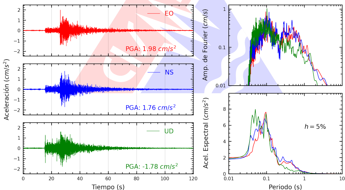
Figura A.2: Registros tiempo-historia, espectros de Fourier y de respuesta en las direcciones EO, NS y vertical de la estación UNICA. Sismo de Huancano, Pisco - Ica del 2025-07-03, 04:50:10 (Hora local)
