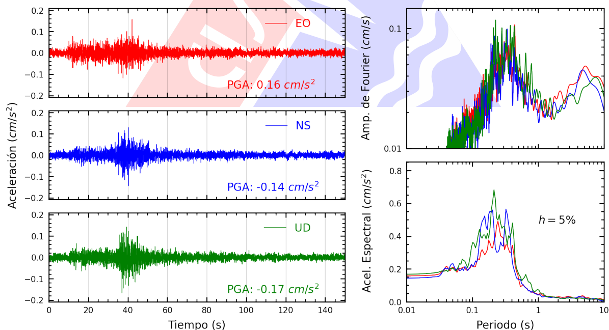
Figura A.46: Registros tiempo-historia, espectros de Fourier y de respuesta en las direcciones EO, NS y vertical de la estación UNSCH. Sismo de Huancano, Pisco - Ica del 2025-07-03, 04:50:10 (Hora local)
