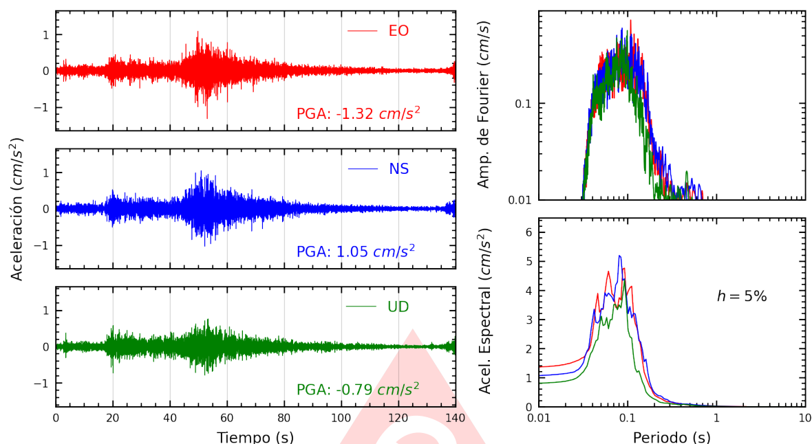
Figura A.7: Registros tiempo-historia, espectros de Fourier y de respuesta en las direcciones EO, NS y vertical de la estación SROSA. Sismo de Huancano, Pisco - Ica del 2025-07-03, 04:50:10 (Hora local)
