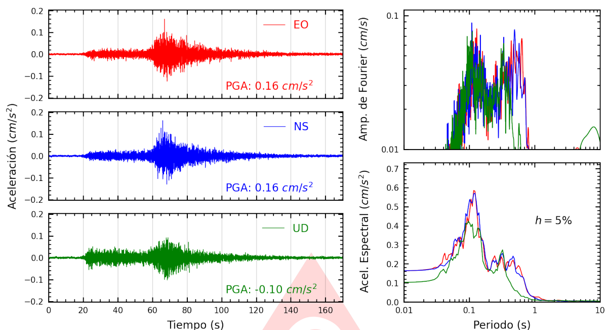
Figura A.47: Registros tiempo-historia, espectros de Fourier y de respuesta en las direcciones EO, NS y vertical de la estación CARAL. Sismo de Huancano, Pisco - Ica del 2025-07-03, 04:50:10 (Hora local)
