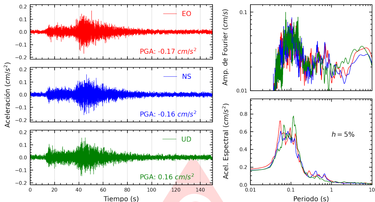
Figura A.45: Registros tiempo-historia, espectros de Fourier y de respuesta en las direcciones EO, NS y vertical de la estación UNFV. Sismo de Huancano, Pisco - Ica del 2025-07-03, 04:50:10 (Hora local)
