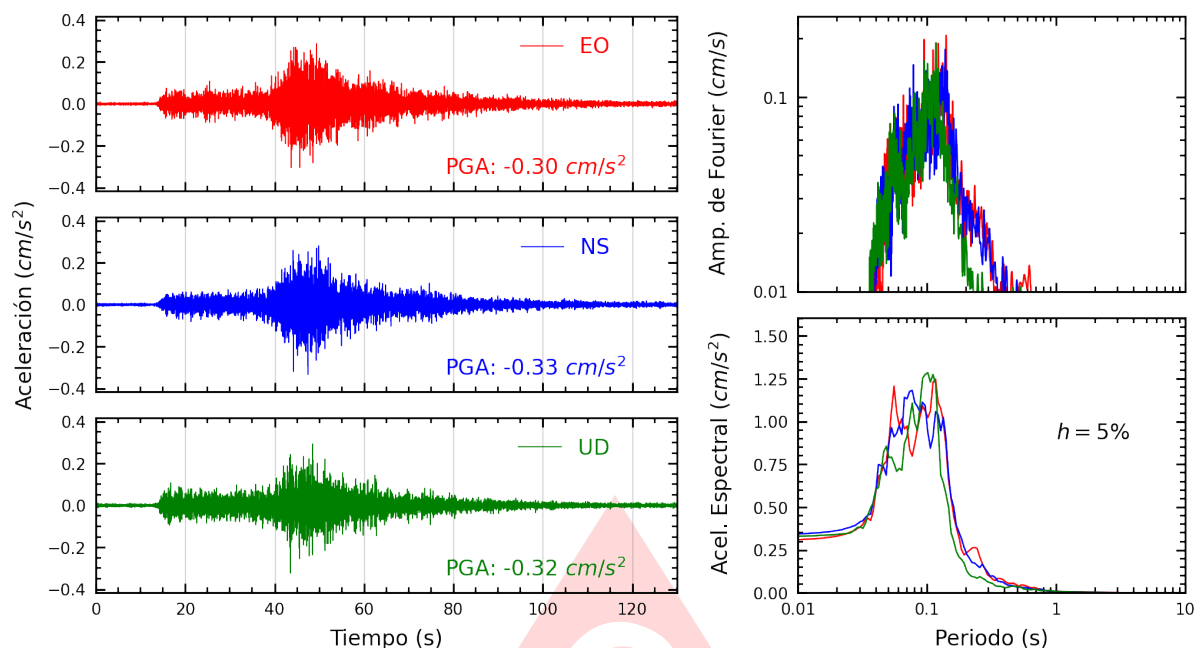
Figura A.35: Registros tiempo-historia, espectros de Fourier y de respuesta en las direcciones EO, NS y vertical de la estación JALV2. Sismo de Huancano, Pisco - Ica del 2025-07-03, 04:50:10 (Hora local)
