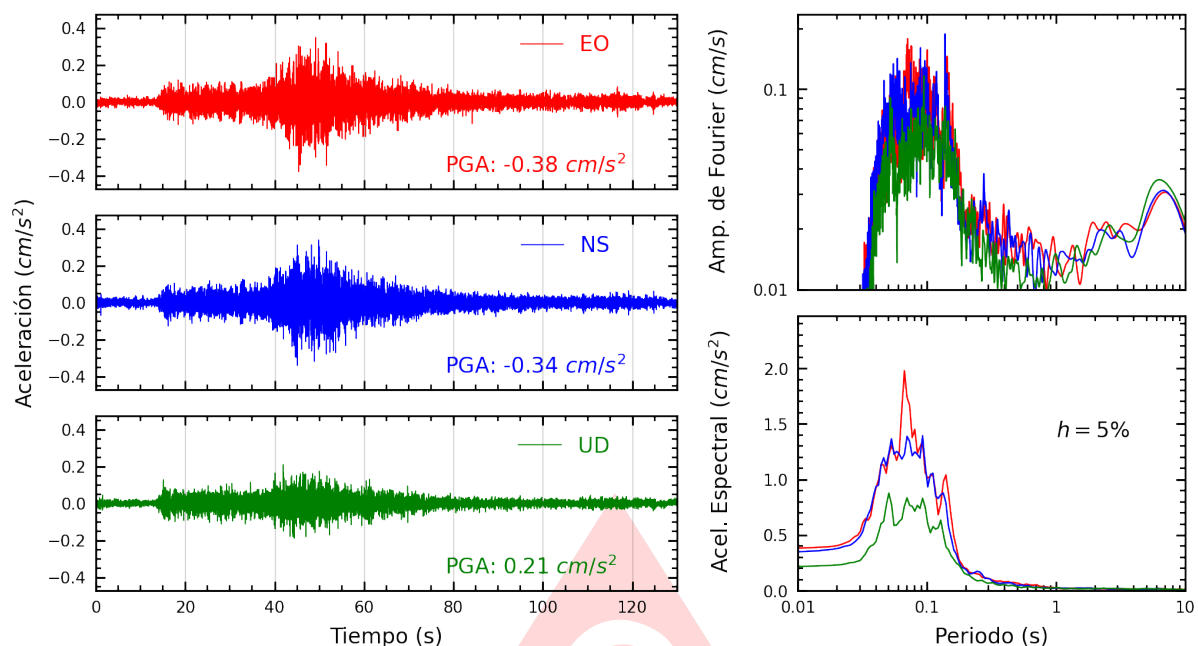
Figura A.29: Registros tiempo-historia, espectros de Fourier y de respuesta en las direcciones EO, NS y vertical de la estación FICPE. Sismo de Huancano, Pisco - Ica del 2025-07-03, 04:50:10 (Hora local)
