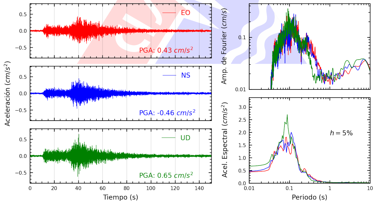
Figura A.18: Registros tiempo-historia, espectros de Fourier y de respuesta en las direcciones EO, NS y vertical de la estación SOVES. Sismo de Huancano, Pisco - Ica del 2025-07-03, 04:50:10 (Hora local)
