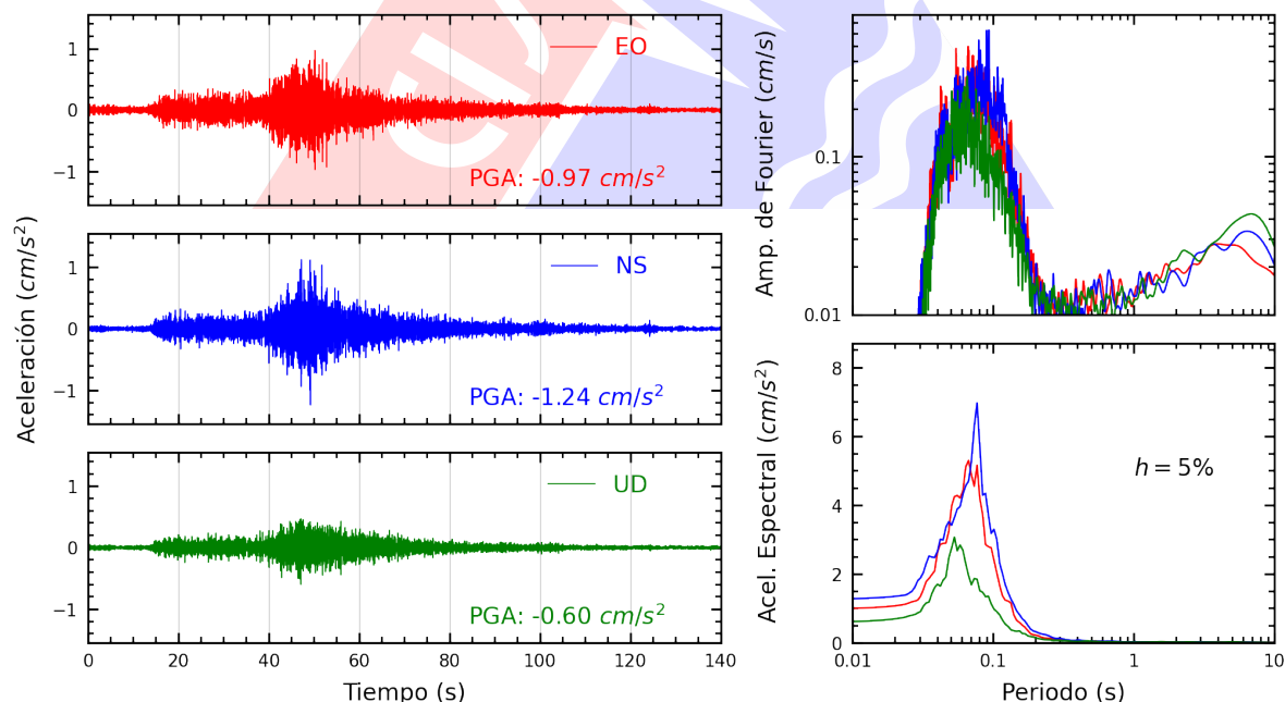
Figura A.8: Registros tiempo-historia, espectros de Fourier y de respuesta en las direcciones EO, NS y vertical de la estación JOSEO. Sismo de Huancano, Pisco - Ica del 2025-07-03, 04:50:10 (Hora local)
