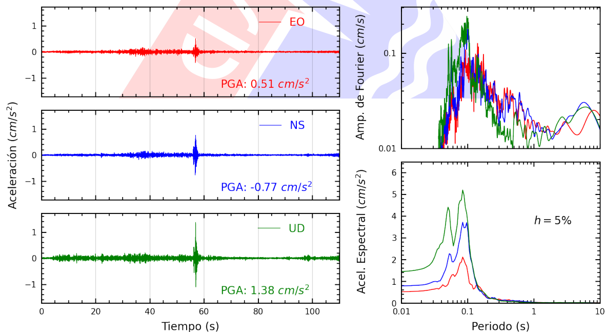
Figura A.4: Registros tiempo-historia, espectros de Fourier y de respuesta en las direcciones EO, NS y vertical de la estación RAMON. Sismo de Huancano, Pisco - Ica del 2025-07-03, 04:50:10 (Hora local)
