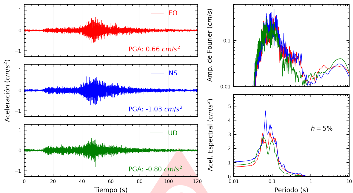
Figura A.11: Registros tiempo-historia, espectros de Fourier y de respuesta en las direcciones EO, NS y vertical de la estación SJLSC. Sismo de Huancano, Pisco - Ica del 2025-07-03, 04:50:10 (Hora local)
