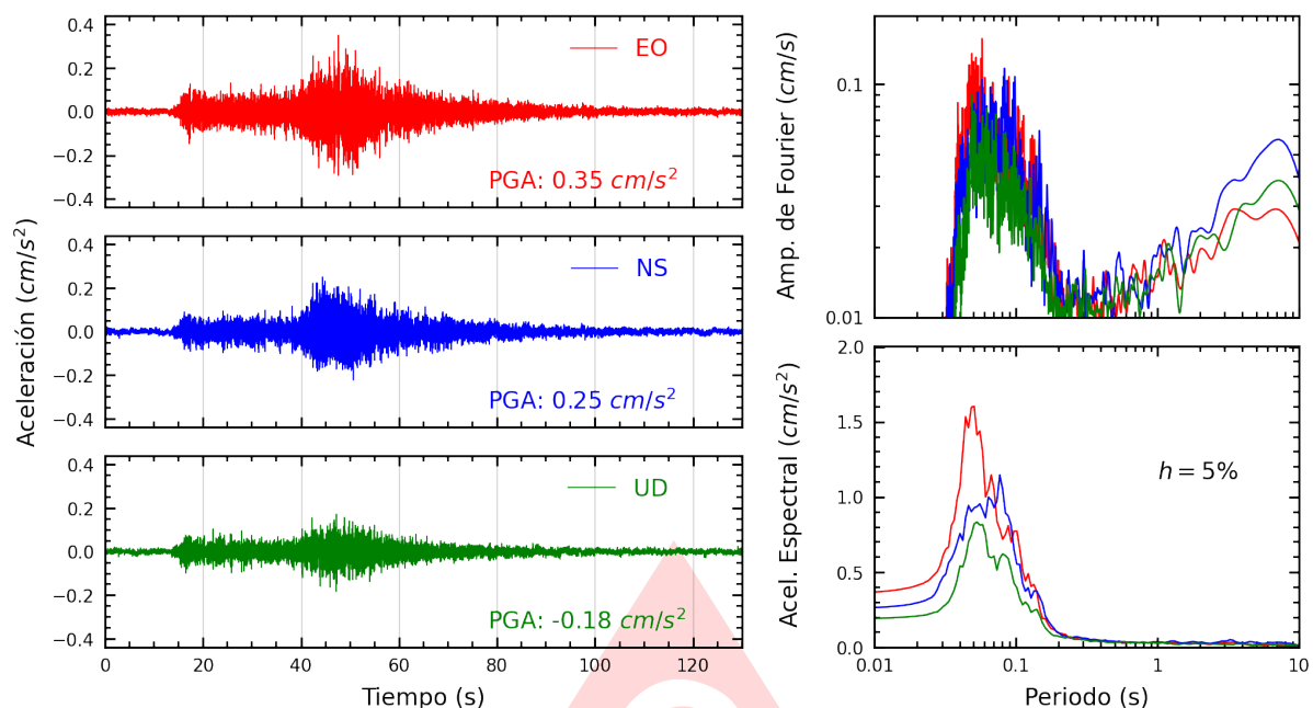
Figura A.31: Registros tiempo-historia, espectros de Fourier y de respuesta en las direcciones EO, NS y vertical de la estación UCSS. Sismo de Huancano, Pisco - Ica del 2025-07-03, 04:50:10 (Hora local)
