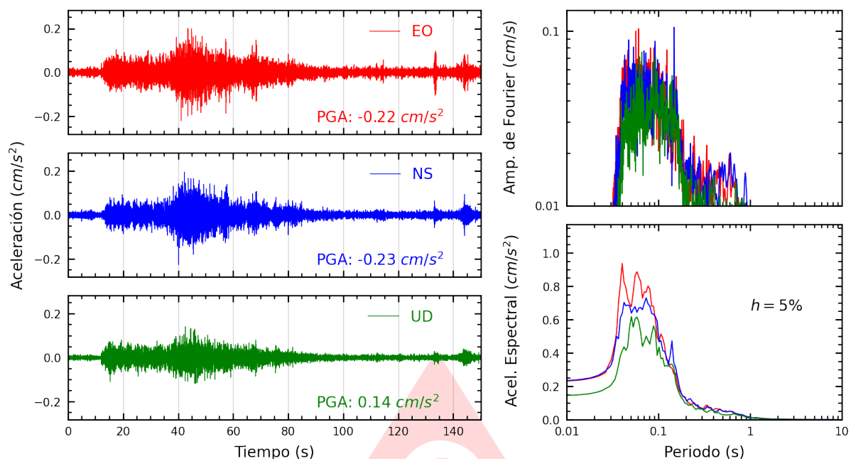
Figura A.41: Registros tiempo-historia, espectros de Fourier y de respuesta en las direcciones EO, NS y vertical de la estación BORJA. Sismo de Huancano, Pisco - Ica del 2025-07-03, 04:50:10 (Hora local)
