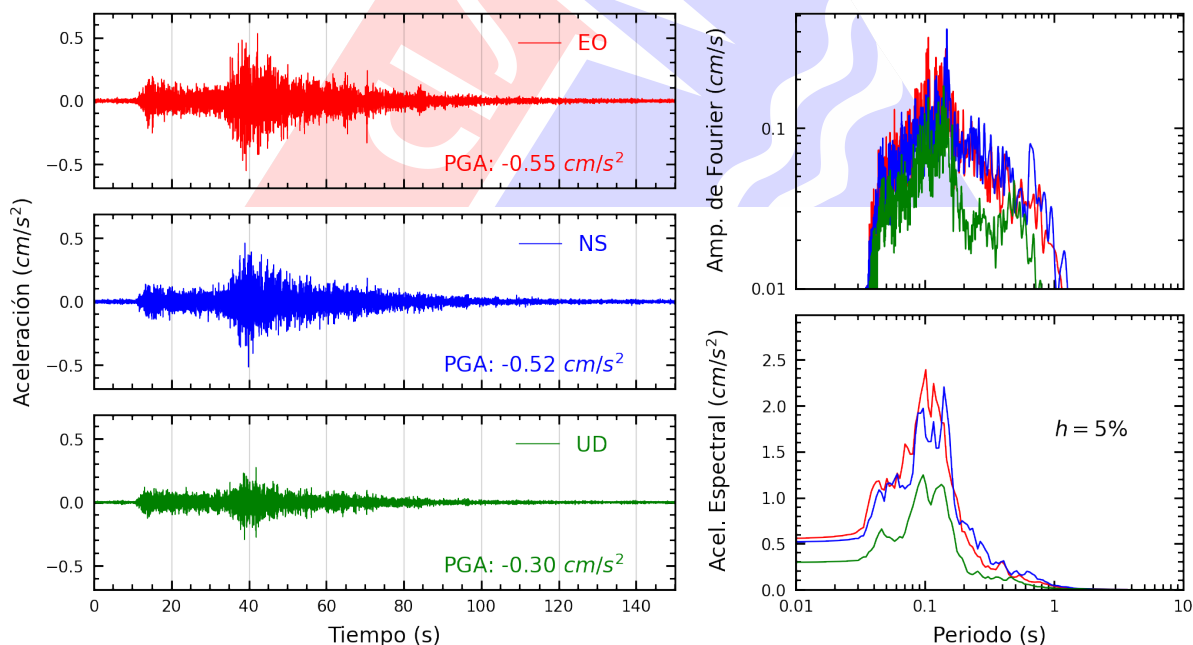
Figura A.20: Registros tiempo-historia, espectros de Fourier y de respuesta en las direcciones EO, NS y vertical de la estación BRIS2. Sismo de Huancano, Pisco - Ica del 2025-07-03, 04:50:10 (Hora local)
