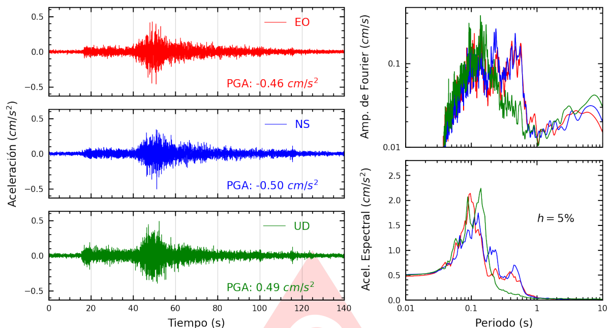
Figura A.23: Registros tiempo-historia, espectros de Fourier y de respuesta en las direcciones EO, NS y vertical de la estación MDPP. Sismo de Huancano, Pisco - Ica del 2025-07-03, 04:50:10 (Hora local)
