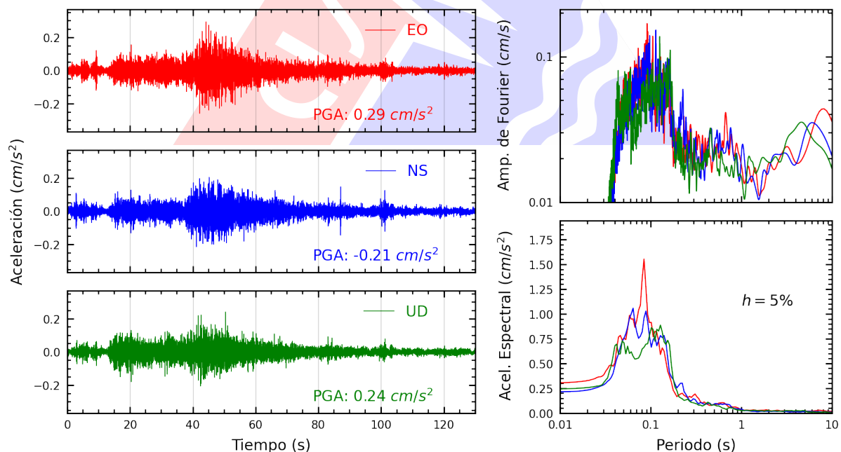
Figura A.38: Registros tiempo-historia, espectros de Fourier y de respuesta en las direcciones EO, NS y vertical de la estación UPCSM. Sismo de Huancano, Pisco - Ica del 2025-07-03, 04:50:10 (Hora local)
