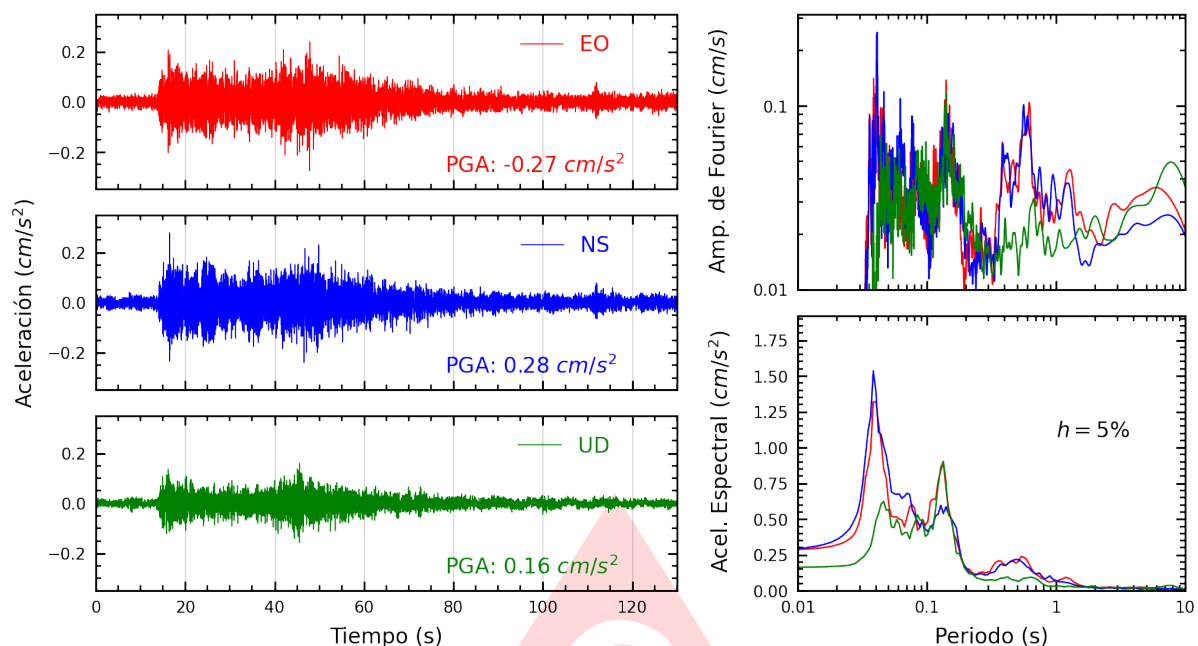
Figura A.39: Registros tiempo-historia, espectros de Fourier y de respuesta en las direcciones EO, NS y vertical de la estación DHNPE. Sismo de Huancano, Pisco - Ica del 2025-07-03, 04:50:10 (Hora local)
