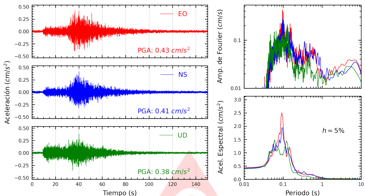
Figura A.27: Registros tiempo-historia, espectros de Fourier y de respuesta en las direcciones EO, NS y vertical de la estación USILP. Sismo de Huancano, Pisco - Ica del 2025-07-03, 04:50:10 (Hora local)
