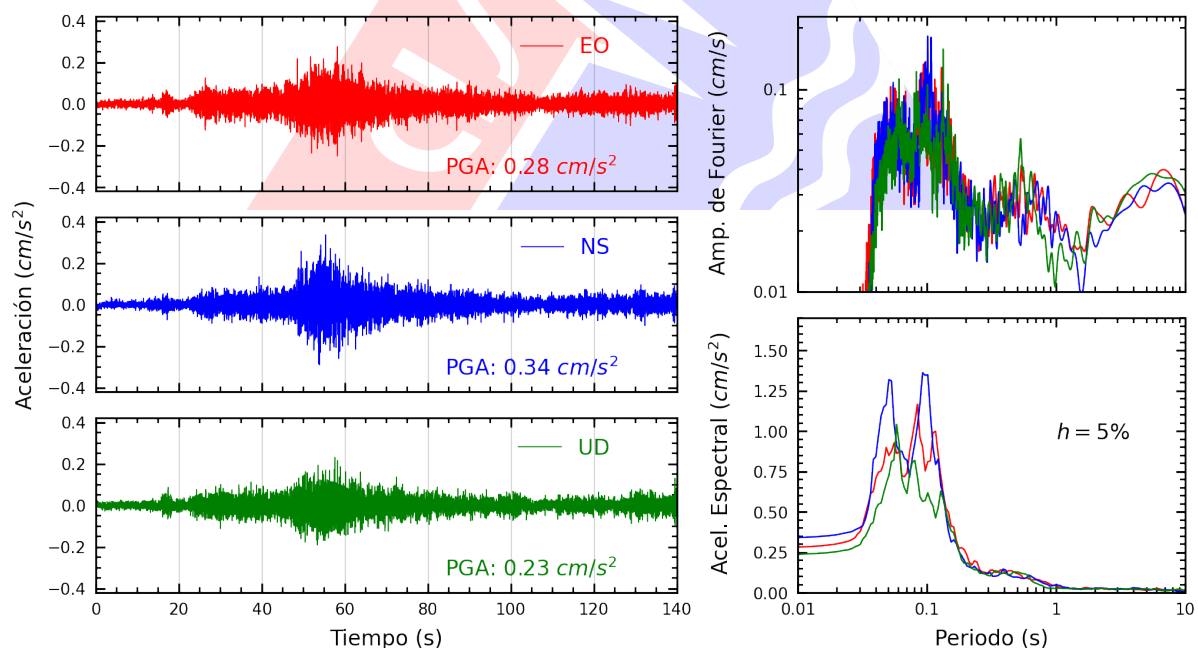
Figura A.34: Registros tiempo-historia, espectros de Fourier y de respuesta en las direcciones EO, NS y vertical de la estación IMCA. Sismo de Huancano, Pisco - Ica del 2025-07-03, 04:50:10 (Hora local)
