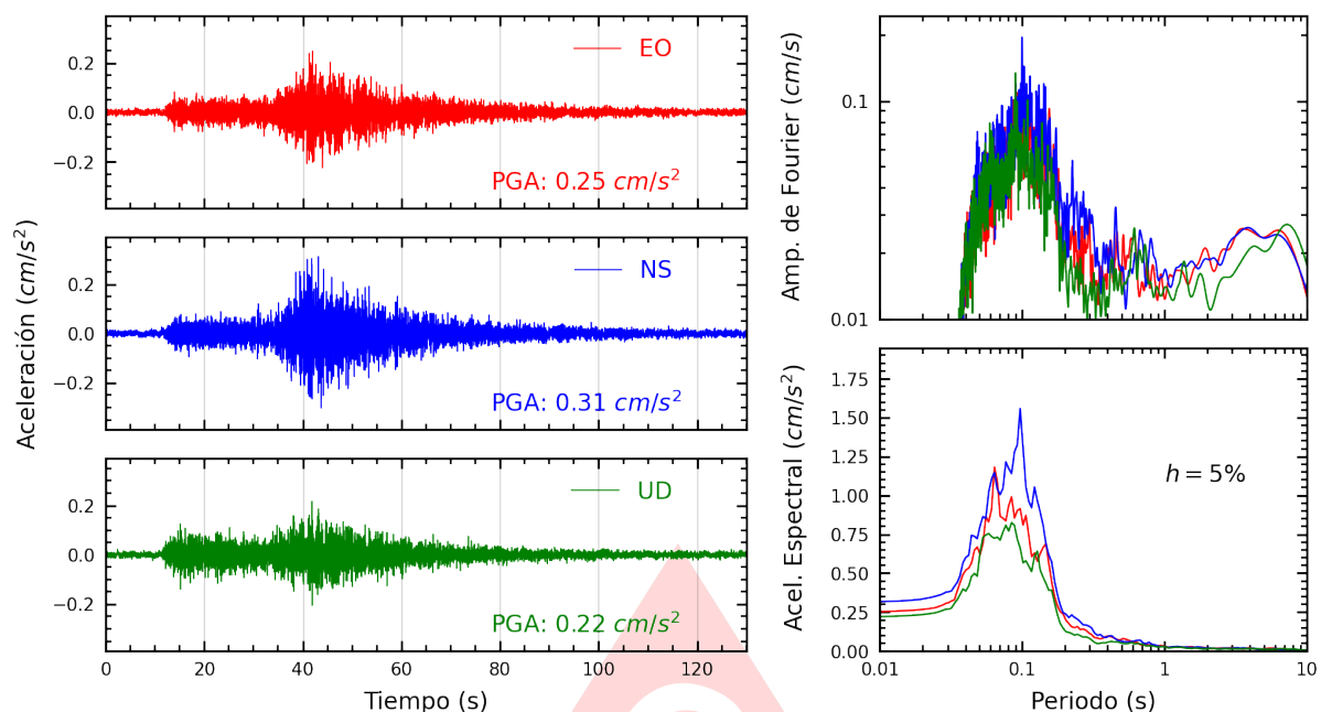
Figura A.37: Registros tiempo-historia, espectros de Fourier y de respuesta en las direcciones EO, NS y vertical de la estación SERVI. Sismo de Huancano, Pisco - Ica del 2025-07-03, 04:50:10 (Hora local)
