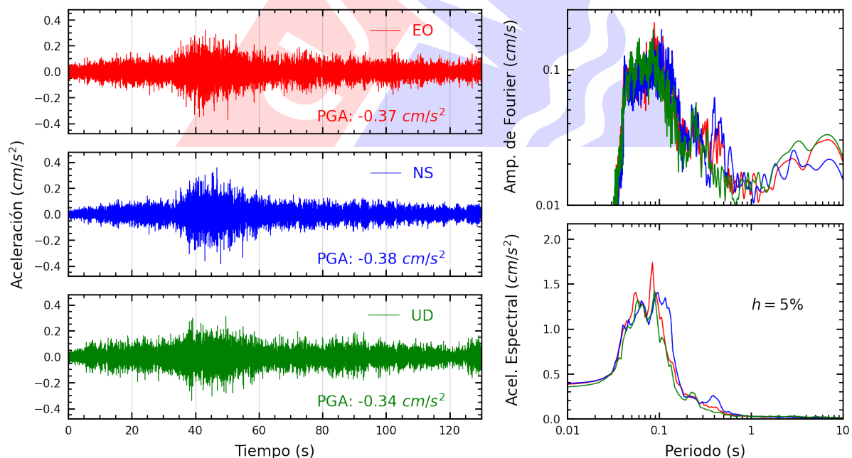
Figura A.28: Registros tiempo-historia, espectros de Fourier y de respuesta en las direcciones EO, NS y vertical de la estación URPPE. Sismo de Huancano, Pisco - Ica del 2025-07-03, 04:50:10 (Hora local)
