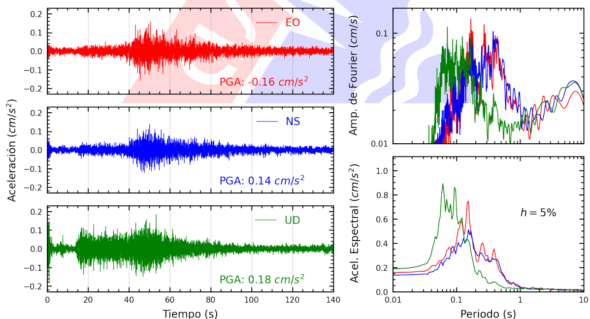
Figura A.44: Registros tiempo-historia, espectros de Fourier y de respuesta en las direcciones EO, NS y vertical de la estación ACAPU. Sismo de Huancano, Pisco - Ica del 2025-07-03, 04:50:10 (Hora local)
