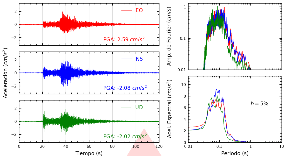
Figura A.1: Registros tiempo-historia, espectros de Fourier y de respuesta en las direcciones EO, NS y vertical de la estación ASIA. Sismo de Huancano, Pisco - Ica del 2025-07-03, 04:50:10 (Hora local)
