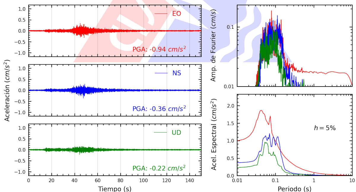
Figura A.12: Registros tiempo-historia, espectros de Fourier y de respuesta en las direcciones EO, NS y vertical de la estación ATARJ. Sismo de Huancano, Pisco - Ica del 2025-07-03, 04:50:10 (Hora local)
