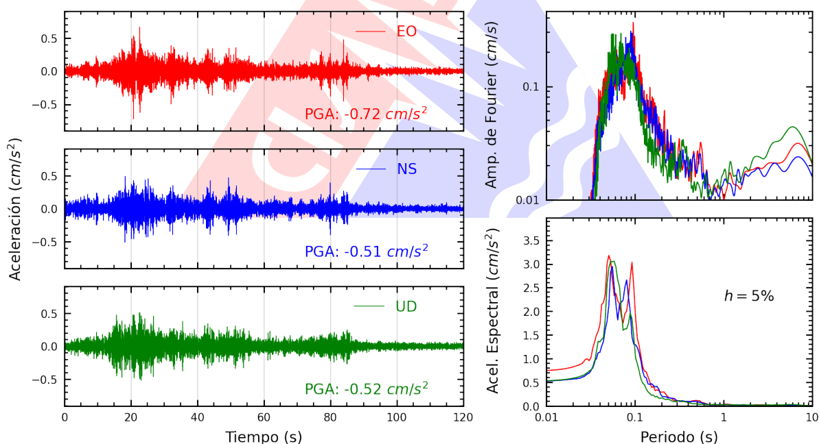
Figura A.2: Registros tiempo-historia, espectros de Fourier y de respuesta en las direcciones EO, NS y vertical de la estación SJLSV. Sismo de Huarmey, Huarmey - Ancash del 2025-07-03, 10:13:23 (Hora local)
