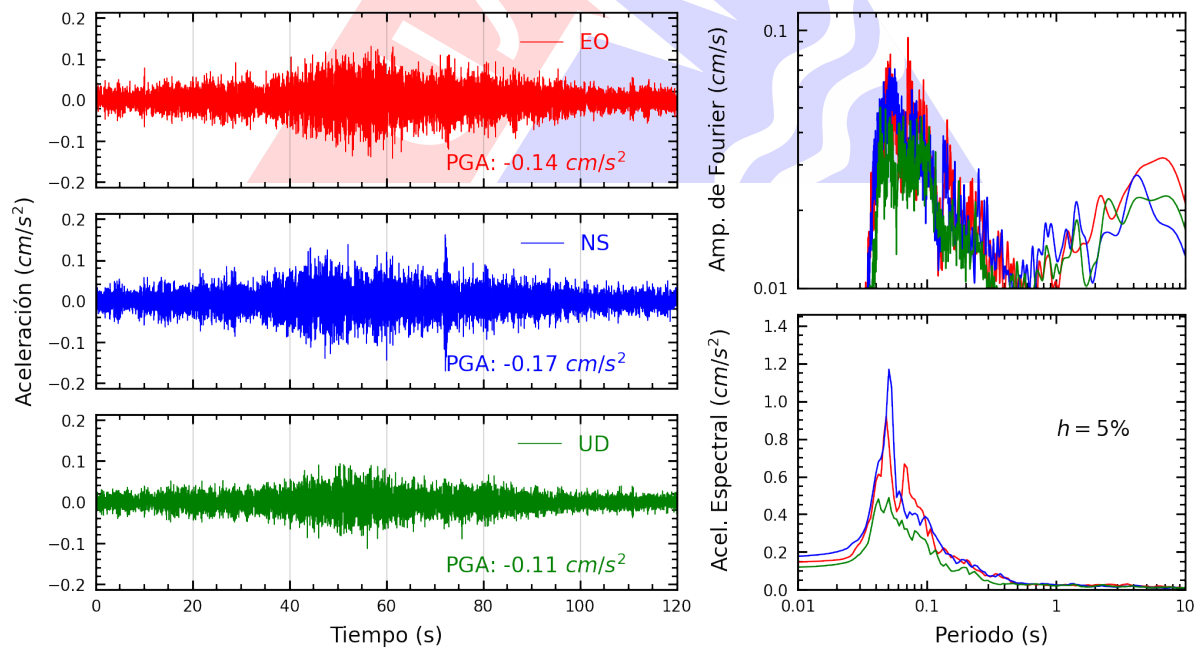
Figura A.6: Registros tiempo-historia, espectros de Fourier y de respuesta en las direcciones EO, NS y vertical de la estación FICPE. Sismo de Huarney, Huarney - Ancash del 2025-07-03, 10:13:23 (Hora local)
