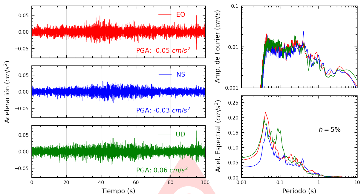
Figura A.19: Registros tiempo-historia, espectros de Fourier y de respuesta en las direcciones EO, NS y vertical de la estación UNC. Sismo de Huarney, Huarney - Ancash del 2025-07-03, 10:13:23 (Hora local)
