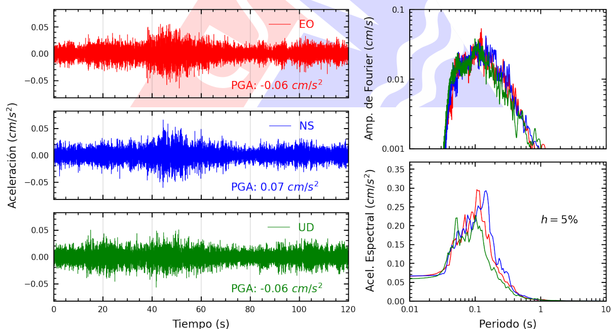
Figura A.18: Registros tiempo-historia, espectros de Fourier y de respuesta en las direcciones EO, NS y vertical de la estación JALV2. Sismo de Huarney, Huarney - Ancash del 2025-07-03, 10:13:23 (Hora local)
