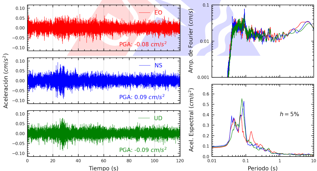
Figura A.12: Registros tiempo-historia, espectros de Fourier y de respuesta en las direcciones EO, NS y vertical de la estación IMCA. Sismo de Huarney, Huarney - Ancash del 2025-07-03, 10:13:23 (Hora local)
