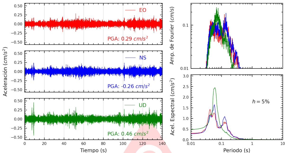
Figura A.3: Registros tiempo-historia, espectros de Fourier y de respuesta en las direcciones EO, NS y vertical de la estación CARAB. Sismo de Huarney, Huarney - Ancash del 2025-07-03, 10:13:23 (Hora local)
