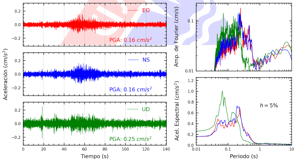
Figura A.4: Registros tiempo-historia, espectros de Fourier y de respuesta en las direcciones EO, NS y vertical de la estación MDPP. Sismo de Huarney, Huarney - Ancash del 2025-07-03, 10:13:23 (Hora local)
