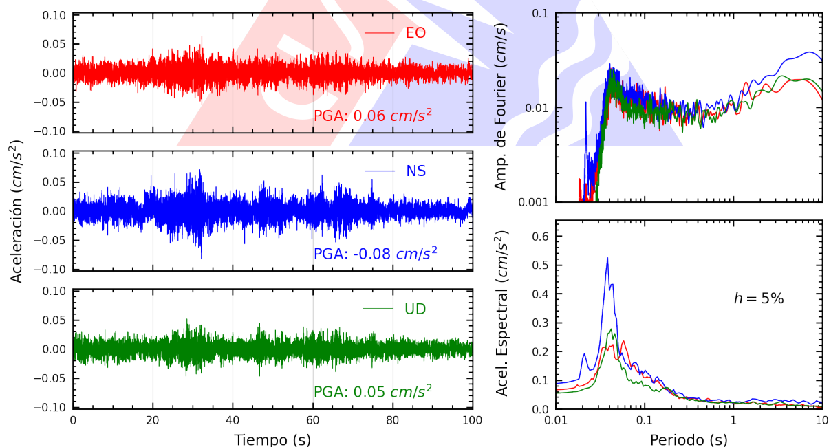
Figura A.14: Registros tiempo-historia, espectros de Fourier y de respuesta en las direcciones EO, NS y vertical de la estación SJLCE. Sismo de Huarney, Huarney - Ancash del 2025-07-03, 10:13:23 (Hora local)
