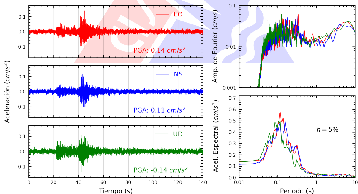
Figura A.10: Registros tiempo-historia, espectros de Fourier y de respuesta en las direcciones EO, NS y vertical de la estación UNASA. Sismo de Huarney, Huarney - Ancash del 2025-07-03, 10:13:23 (Hora local)
