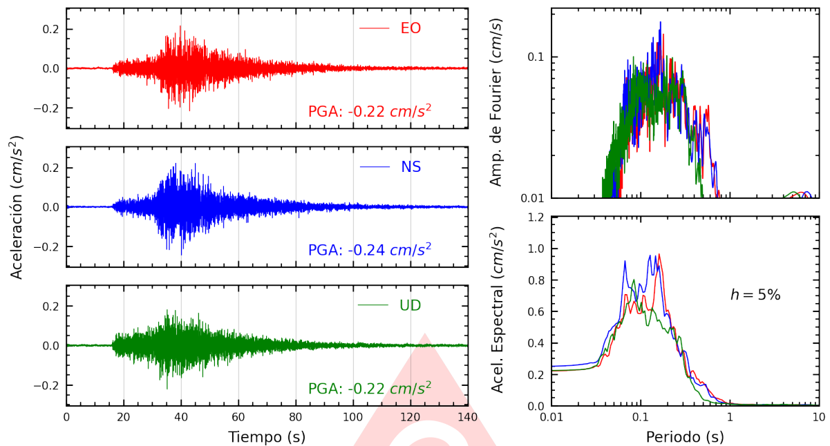
Figura A.5: Registros tiempo-historia, espectros de Fourier y de respuesta en las direcciones EO, NS y vertical de la estación CARAL. Sismo de Huarney, Huarney - Ancash del 2025-07-03, 10:13:23 (Hora local)
