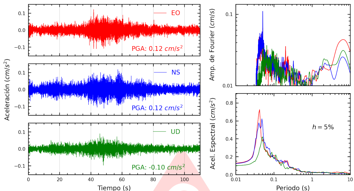
Figura A.11: Registros tiempo-historia, espectros de Fourier y de respuesta en las direcciones EO, NS y vertical de la estación COMAS. Sismo de Huarney, Huarney - Ancash del 2025-07-03, 10:13:23 (Hora local)
