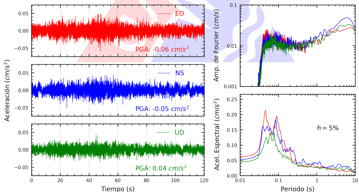
Figura A.20: Registros tiempo-historia, espectros de Fourier y de respuesta en las direcciones EO, NS y vertical de la estación UCSS. Sismo de Huarney, Huarney - Ancash del 2025-07-03, 10:13:23 (Hora local)
