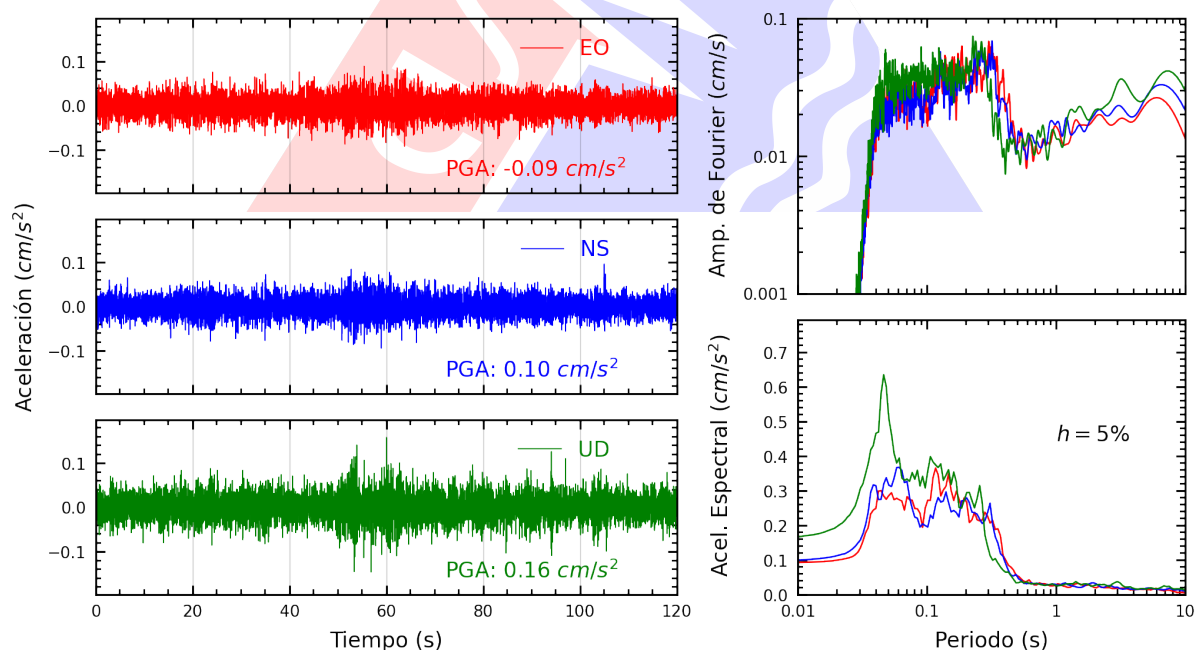
Figura A.8: Registros tiempo-historia, espectros de Fourier y de respuesta en las direcciones EO, NS y vertical de la estación SOVES. Sismo de Huarney, Huarney - Ancash del 2025-07-03, 10:13:23 (Hora local)
