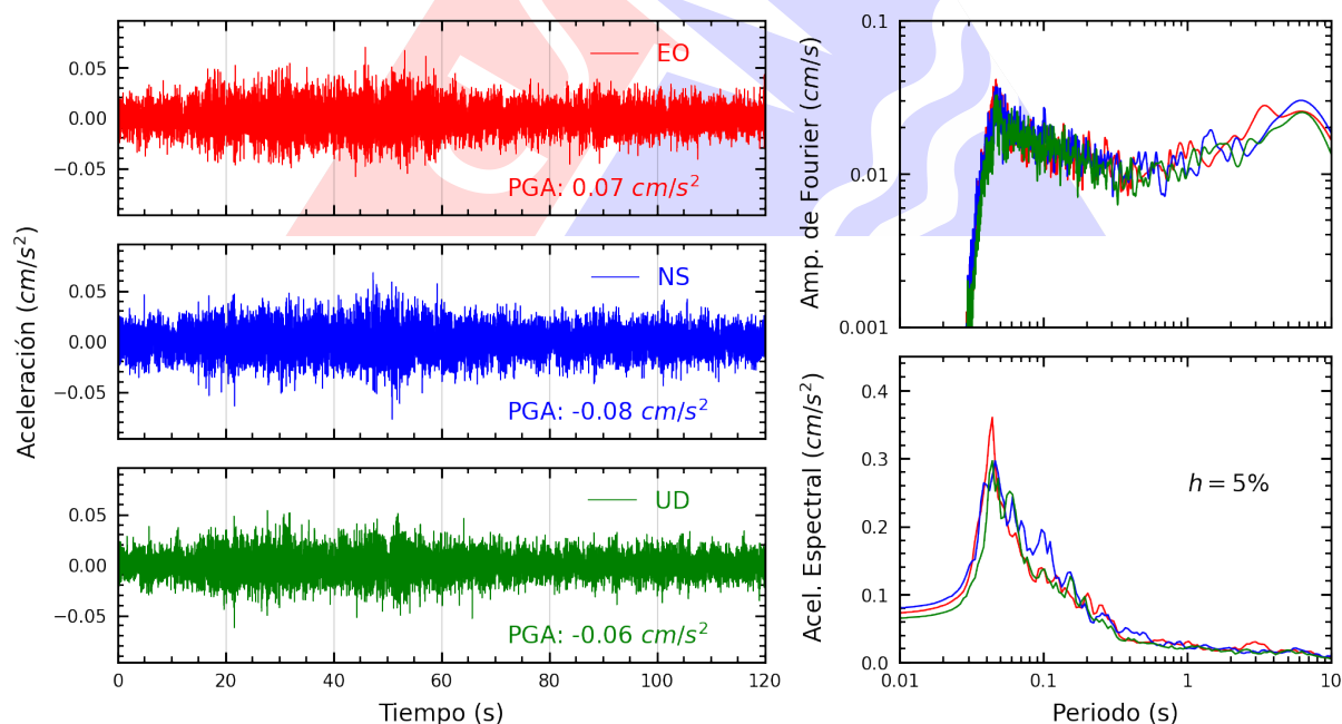
Figura A.16: Registros tiempo-historia, espectros de Fourier y de respuesta en las direcciones EO, NS y vertical de la estación SERVI. Sismo de Huarney, Huarney - Ancash del 2025-07-03, 10:13:23 (Hora local)
