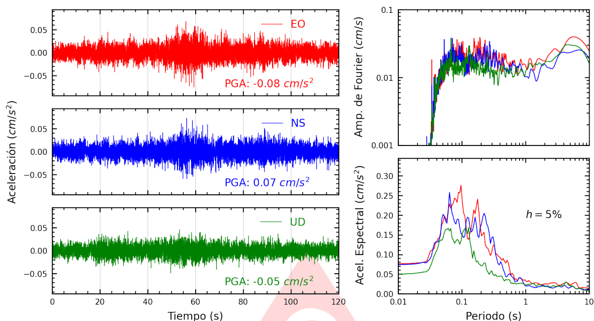
Figura A.17: Registros tiempo-historia, espectros de Fourier y de respuesta en las direcciones EO, NS y vertical de la estación USILP. Sismo de Huarney, Huarney - Ancash del 2025-07-03, 10:13:23 (Hora local)
