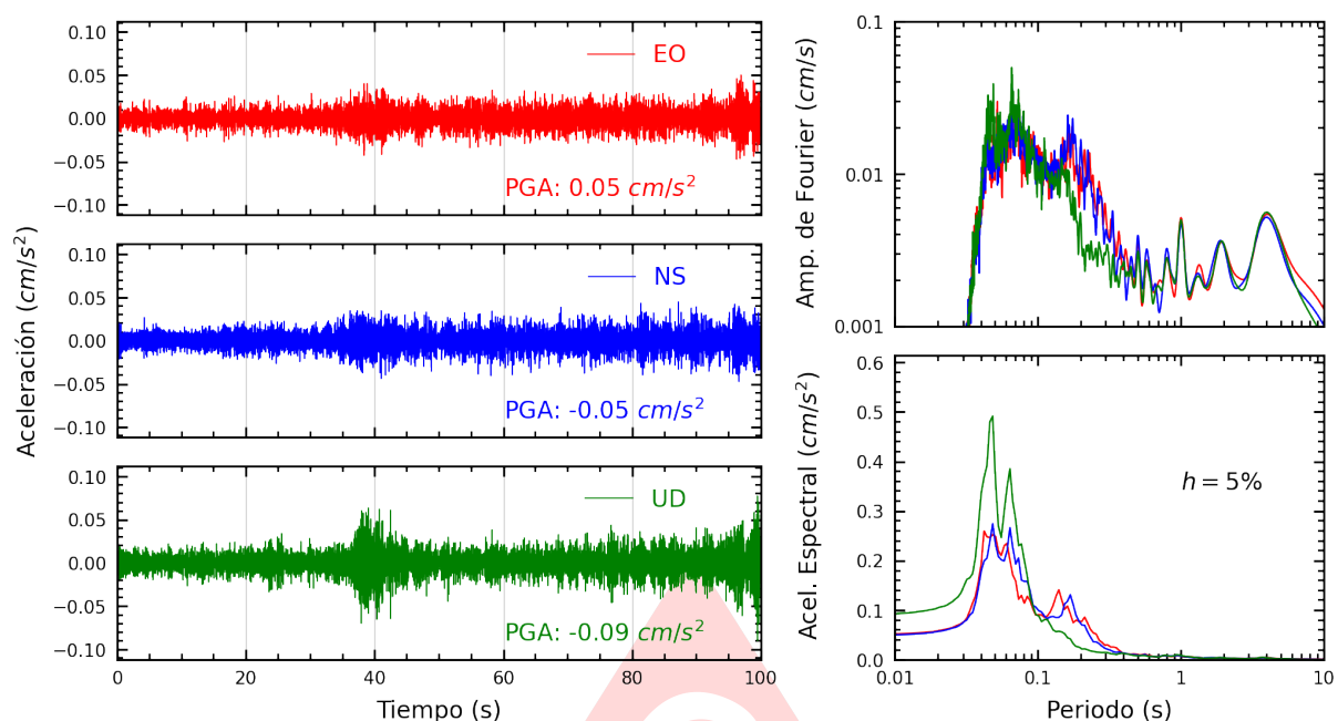
Figura A.13: Registros tiempo-historia, espectros de Fourier y de respuesta en las direcciones EO, NS y vertical de la estación ASIA. Sismo de Huarney, Huarney - Ancash del 2025-07-03, 10:13:23 (Hora local)
