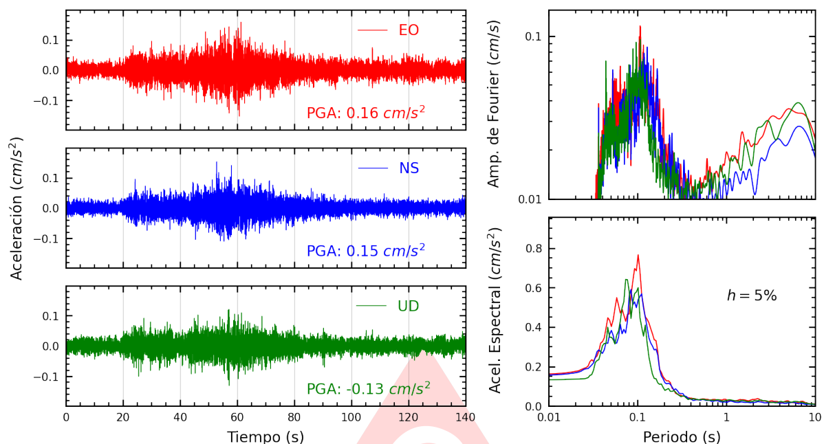
Figura A.7: Registros tiempo-historia, espectros de Fourier y de respuesta en las direcciones EO, NS y vertical de la estación AMORE. Sismo de Huarney, Huarney - Ancash del 2025-07-03, 10:13:23 (Hora local)
