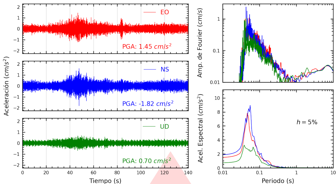
Figura A.1: Registros tiempo-historia, espectros de Fourier y de respuesta en las direcciones EO, NS y vertical de la estación USP. Sismo de Huarmey, Huarmey - Ancash del 2025-07-03, 10:13:23 (Hora local)
