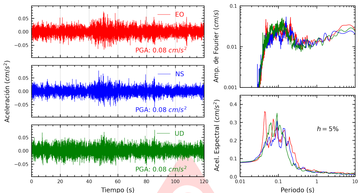
Figura A.15: Registros tiempo-historia, espectros de Fourier y de respuesta en las direcciones EO, NS y vertical de la estación UPAOT. Sismo de Huarney, Huarney - Ancash del 2025-07-03, 10:13:23 (Hora local)
