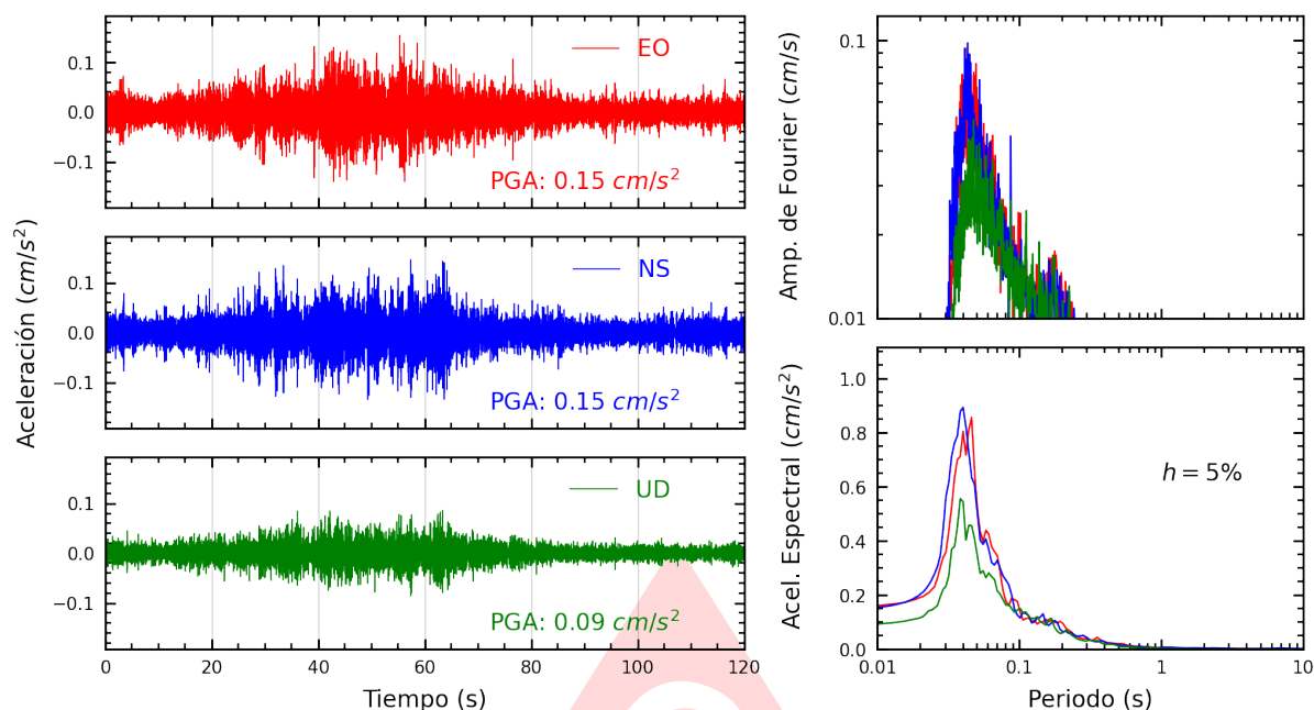
Figura A.9: Registros tiempo-historia, espectros de Fourier y de respuesta en las direcciones EO, NS y vertical de la estación BORJA. Sismo de Huarney, Huarney - Ancash del 2025-07-03, 10:13:23 (Hora local)
