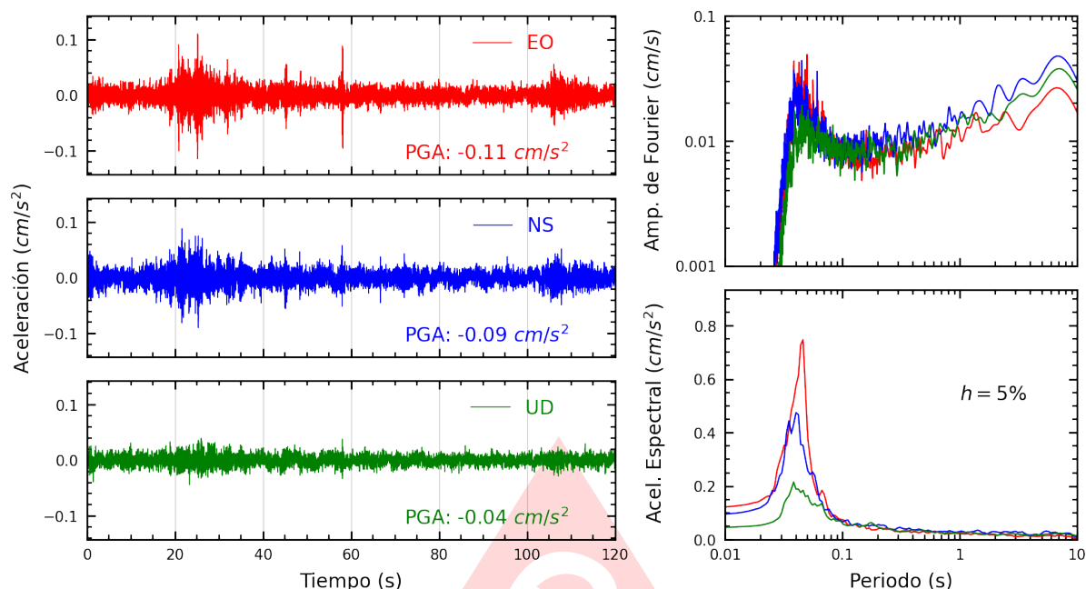
Figura A.9: Registros tiempo-historia, espectros de Fourier y de respuesta en las direcciones EO, NS y vertical de la estación CEPRE. Sismo de Ica, Ica - Ica del 2025-07-04, 01:11:12 (Hora local)
