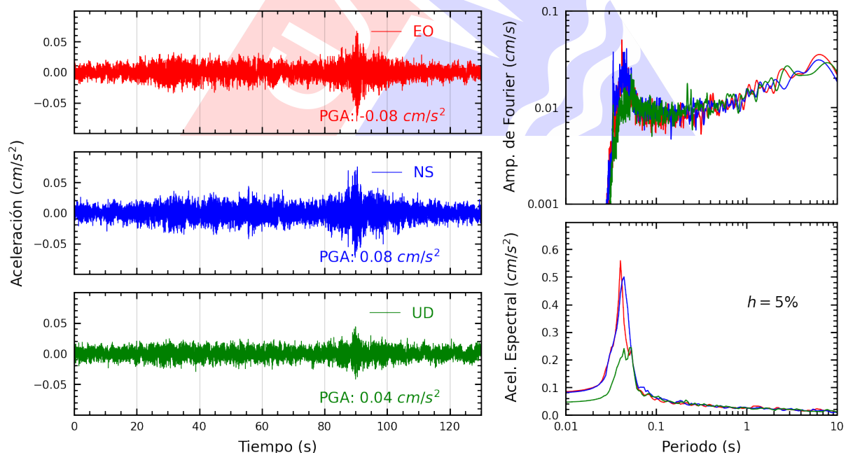
Figura A.12: Registros tiempo-historia, espectros de Fourier y de respuesta en las direcciones EO, NS y vertical de la estación COMAS. Sismo de Ica, Ica - Ica del 2025-07-04, 01:11:12 (Hora local)
