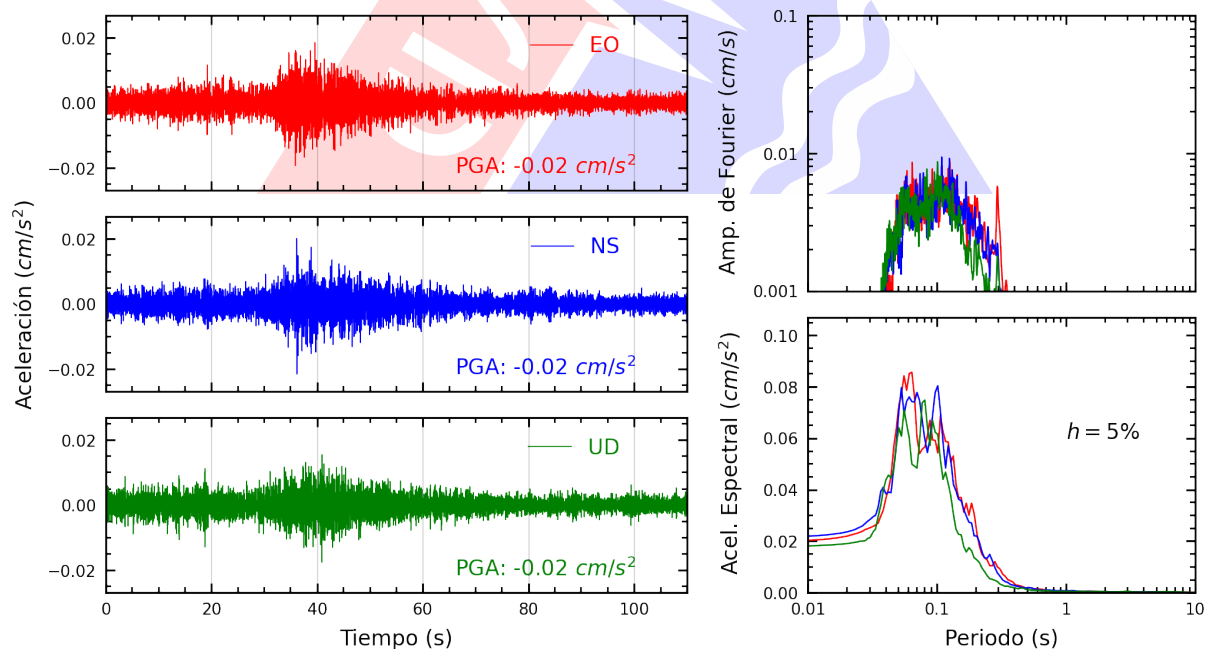
Figura A.16: Registros tiempo-historia, espectros de Fourier y de respuesta en las direcciones EO, NS y vertical de la estación JALV2. Sismo de Ica, Ica - Ica del 2025-07-04, 01:11:12 (Hora local)
