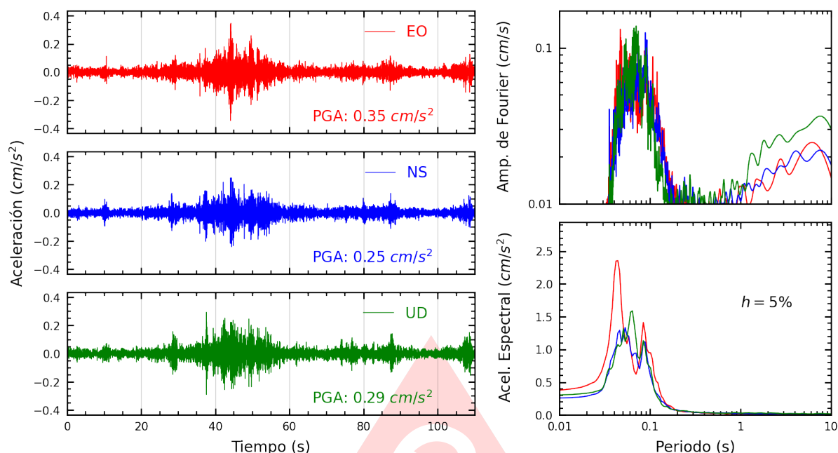
Figura A.3: Registros tiempo-historia, espectros de Fourier y de respuesta en las direcciones EO, NS y vertical de la estación SJLSV. Sismo de Ica, Ica - Ica del 2025-07-04, 01:11:12 (Hora local)
