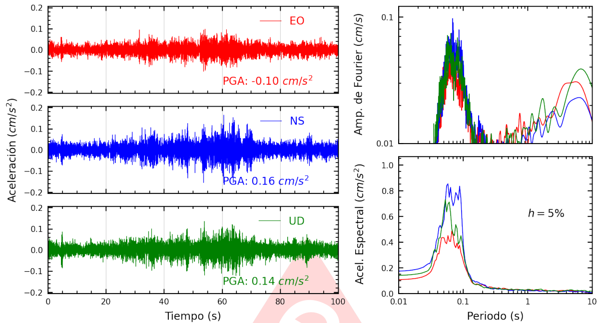
Figura A.7: Registros tiempo-historia, espectros de Fourier y de respuesta en las direcciones EO, NS y vertical de la estación SJLSC. Sismo de Ica, Ica - Ica del 2025-07-04, 01:11:12 (Hora local)
