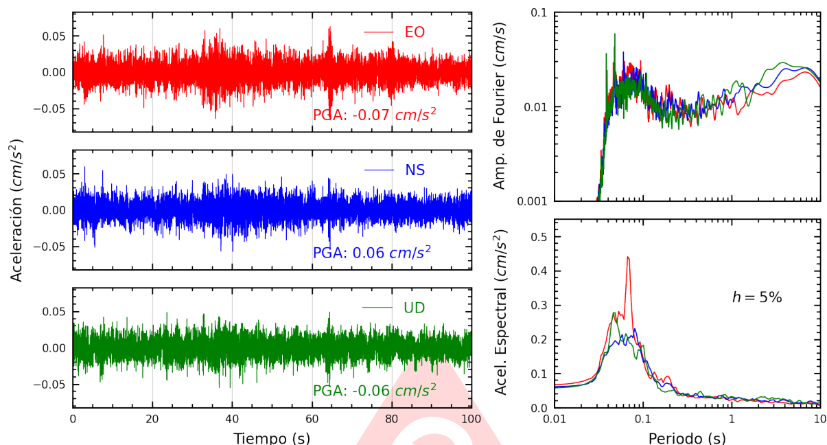
Figura A.13: Registros tiempo-historia, espectros de Fourier y de respuesta en las direcciones EO, NS y vertical de la estación INDEP. Sismo de Ica, Ica - Ica del 2025-07-04, 01:11:12 (Hora local)
