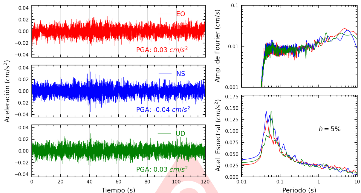
Figura A.15: Registros tiempo-historia, espectros de Fourier y de respuesta en las direcciones EO, NS y vertical de la estación SERVI. Sismo de Ica, Ica - Ica del 2025-07-04, 01:11:12 (Hora local)
