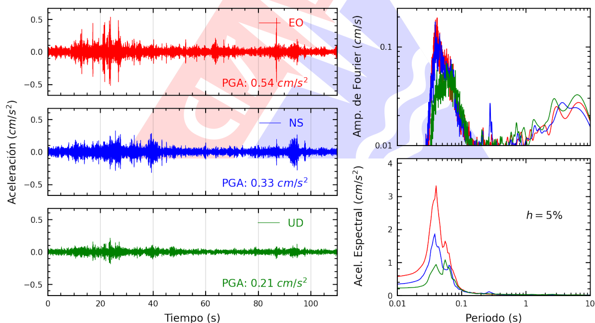
Figura A.2: Registros tiempo-historia, espectros de Fourier y de respuesta en las direcciones EO, NS y vertical de la estación OLIVO. Sismo de Ica, Ica - Ica del 2025-07-04, 01:11:12 (Hora local)
