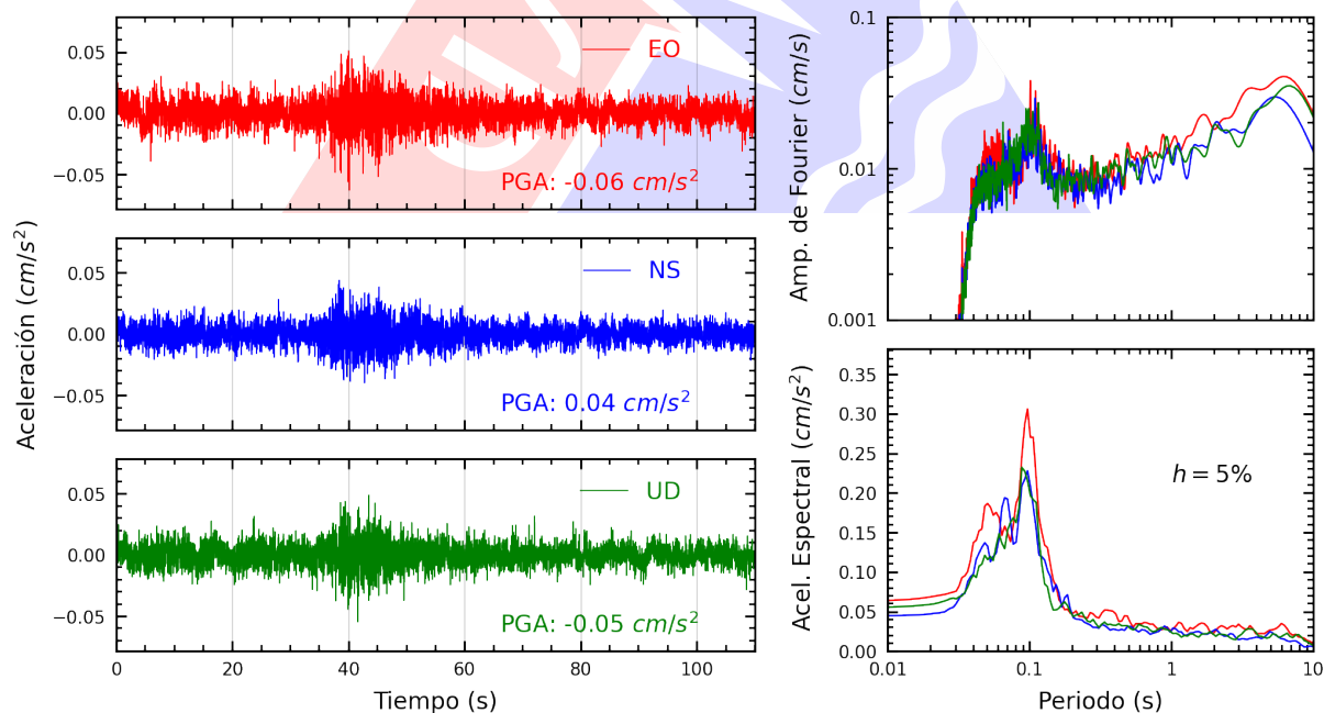
Figura A.14: Registros tiempo-historia, espectros de Fourier y de respuesta en las direcciones EO, NS y vertical de la estación AMORE. Sismo de Ica, Ica - Ica del 2025-07-04, 01:11:12 (Hora local)
