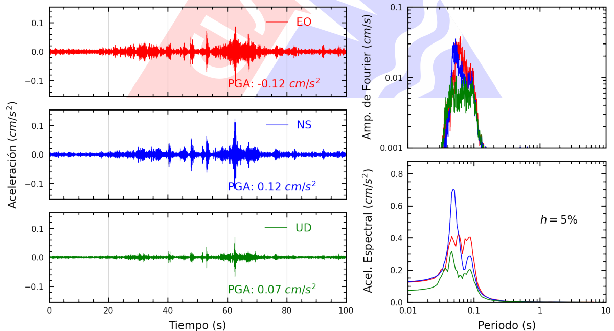
Figura A.8: Registros tiempo-historia, espectros de Fourier y de respuesta en las direcciones EO, NS y vertical de la estación UNMBA. Sismo de Ica, Ica - Ica del 2025-07-04, 01:11:12 (Hora local)
