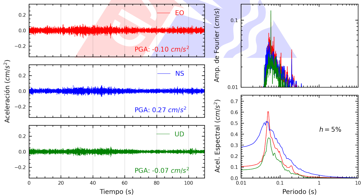
Figura A.6: Registros tiempo-historia, espectros de Fourier y de respuesta en las direcciones EO, NS y vertical de la estación UNTEL. Sismo de Ica, Ica - Ica del 2025-07-04, 01:11:12 (Hora local)
