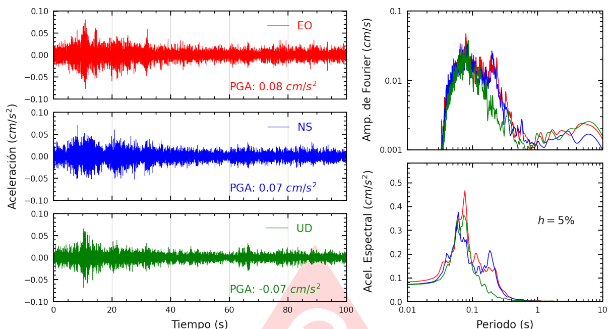
Figura A.11: Registros tiempo-historia, espectros de Fourier y de respuesta en las direcciones EO, NS y vertical de la estación SCCHO. Sismo de Ica, Ica - Ica del 2025-07-04, 01:11:12 (Hora local)
