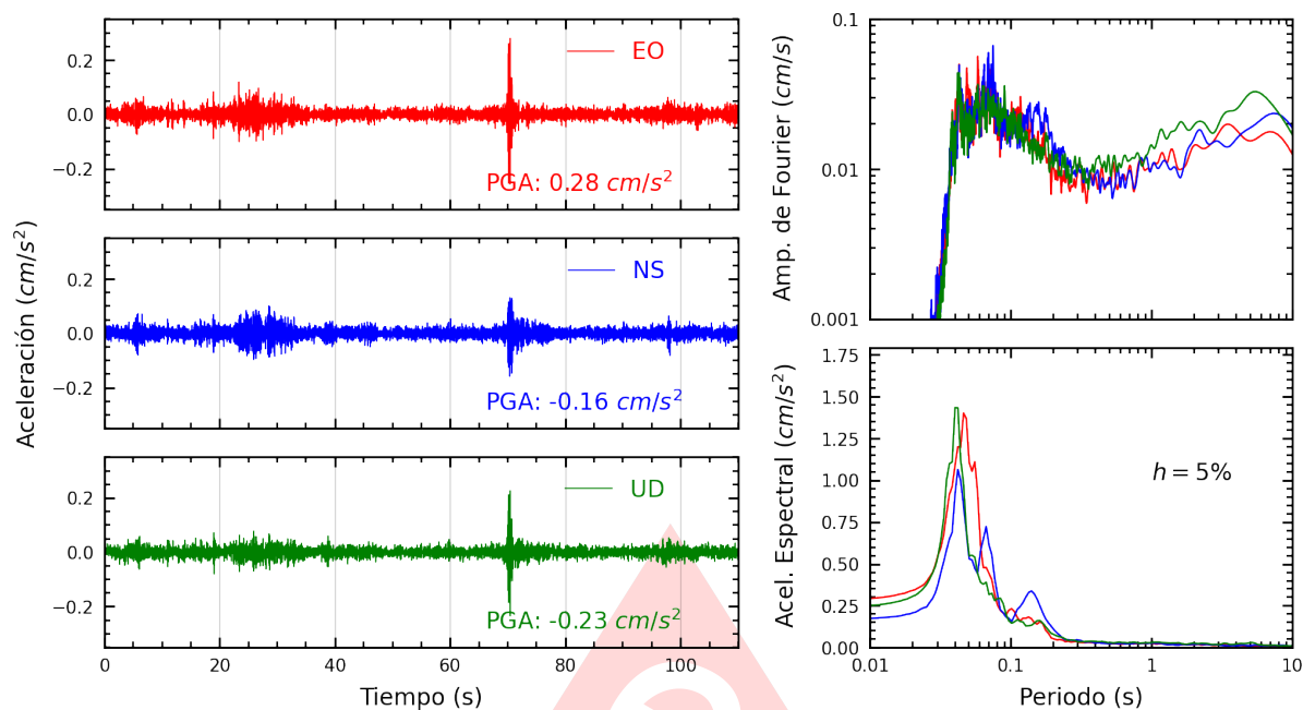
Figura A.5: Registros tiempo-historia, espectros de Fourier y de respuesta en las direcciones EO, NS y vertical de la estación PRADO. Sismo de Ica, Ica - Ica del 2025-07-04, 01:11:12 (Hora local)
