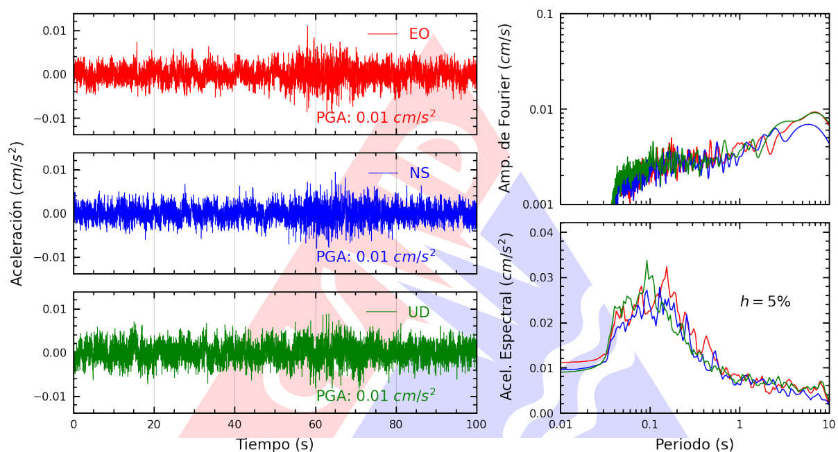
Figura A.17: Registros tiempo-historia, espectros de Fourier y de respuesta en las direcciones EO, NS y vertical de la estación CARAL. Sismo de Ica, Ica - Ica del 2025-07-04, 01:11:12 (Hora local)
