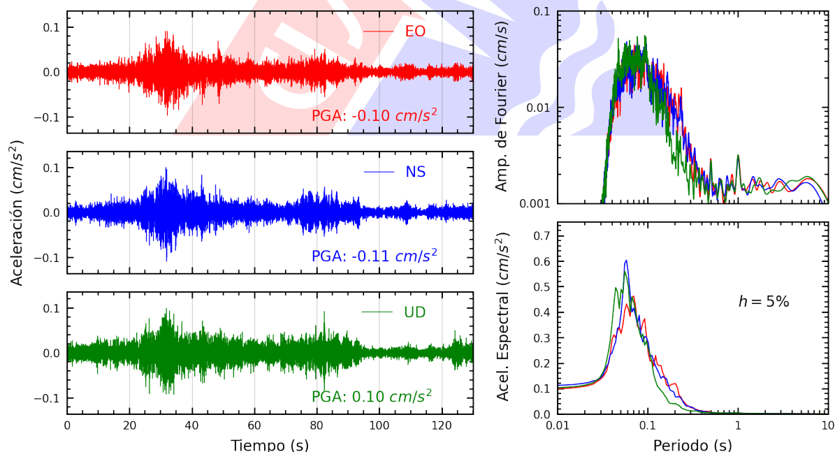
Figura A.10: Registros tiempo-historia, espectros de Fourier y de respuesta en las direcciones EO, NS y vertical de la estación ASIA. Sismo de Ica, Ica - Ica del 2025-07-04, 01:11:12 (Hora local)
