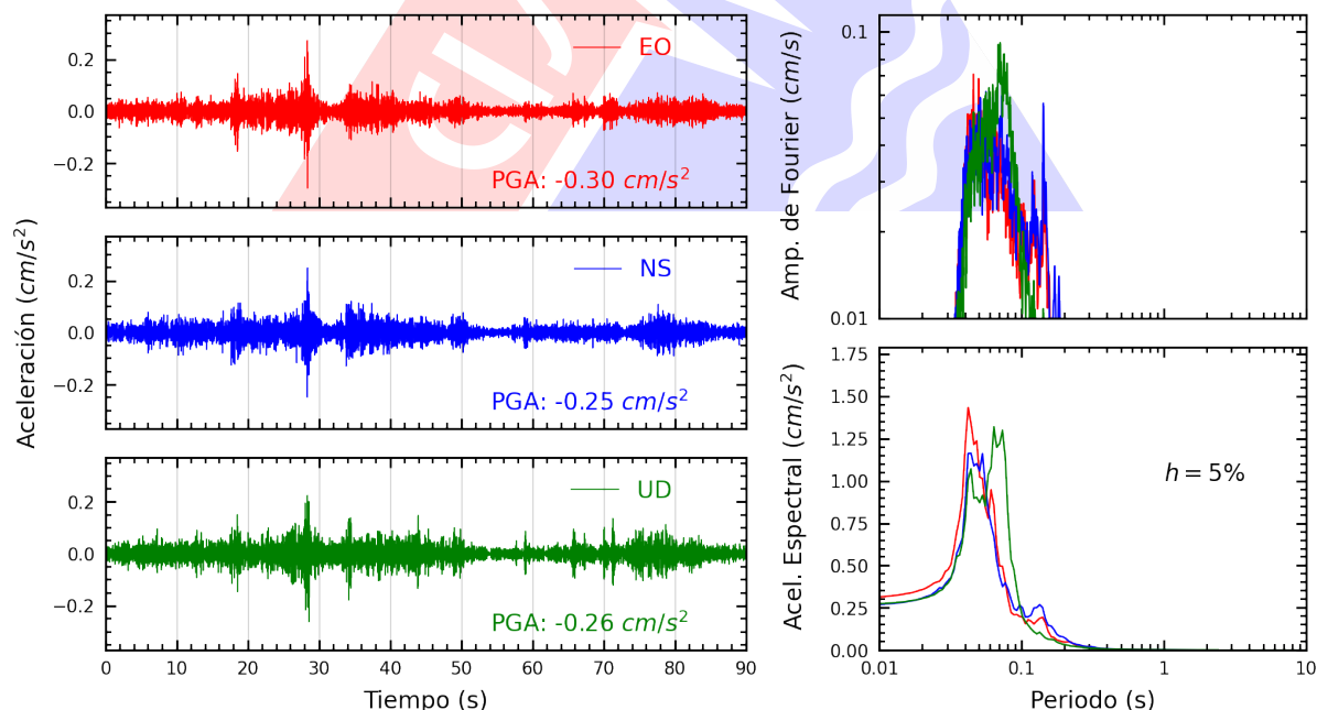
Figura A.4: Registros tiempo-historia, espectros de Fourier y de respuesta en las direcciones EO, NS y vertical de la estación CARAB. Sismo de Ica, Ica - Ica del 2025-07-04, 01:11:12 (Hora local)
