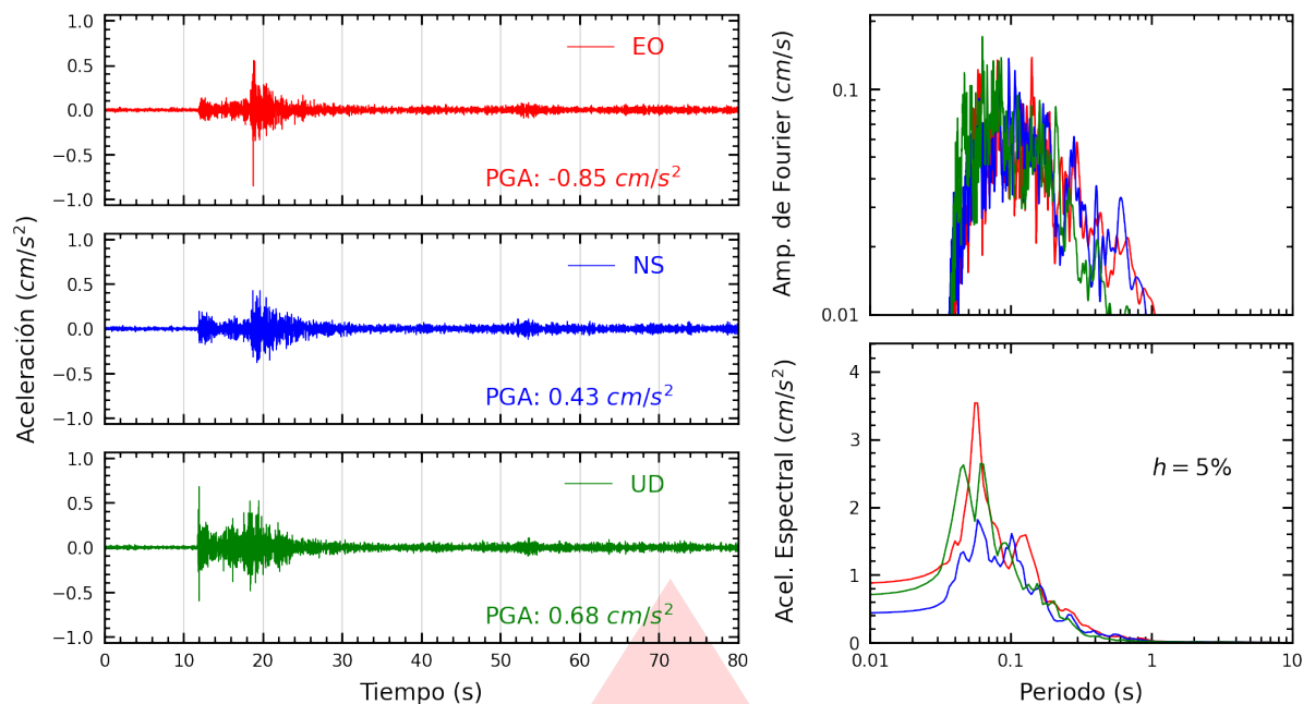
Figura A.1: Registros tiempo-historia, espectros de Fourier y de respuesta en las direcciones EO, NS y vertical de la estación UNICA. Sismo de Ica, Ica - Ica del 2025-07-04, 01:11:12 (Hora local)
