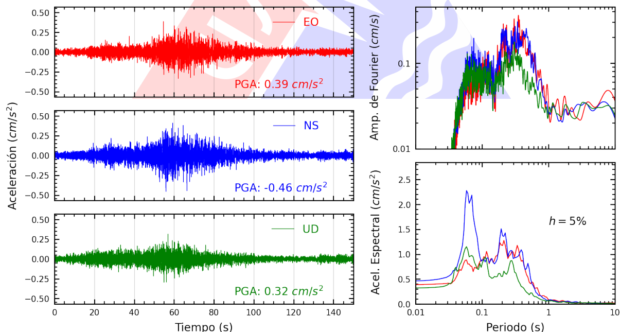
Figura A.18: Registros tiempo-historia, espectros de Fourier y de respuesta en las direcciones EO, NS y vertical de la estación SJLSC. Sismo de Ica, Ica - Ica del 2025-07-04, 03:55:11 (Hora local)
