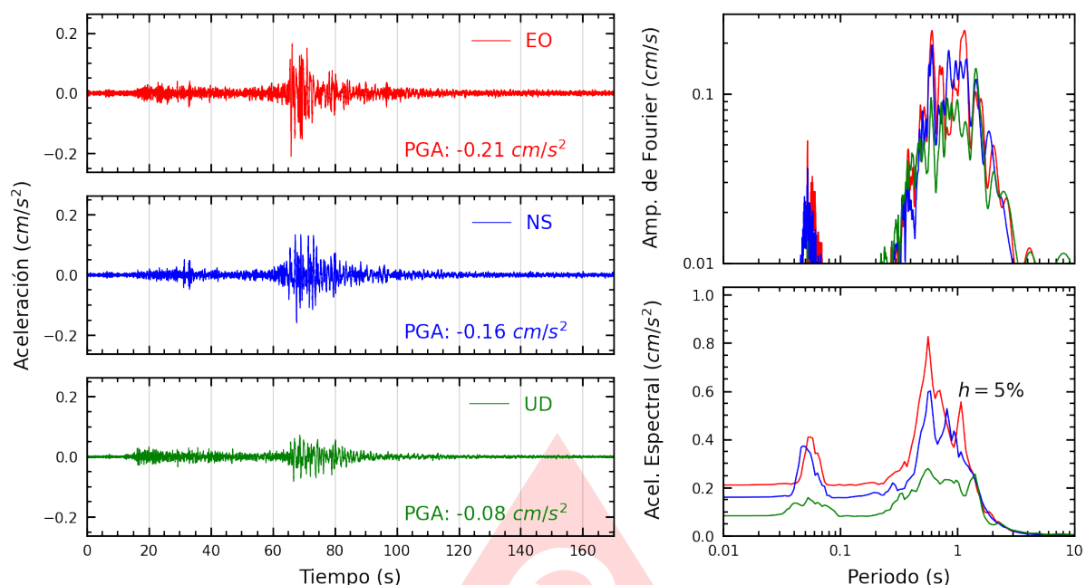
Figura A.39: Registros tiempo-historia, espectros de Fourier y de respuesta en las direcciones EO, NS y vertical de la estación UNMBA. Sismo de Ica, Ica - Ica del 2025-07-04, 03:55:11 (Hora local)
