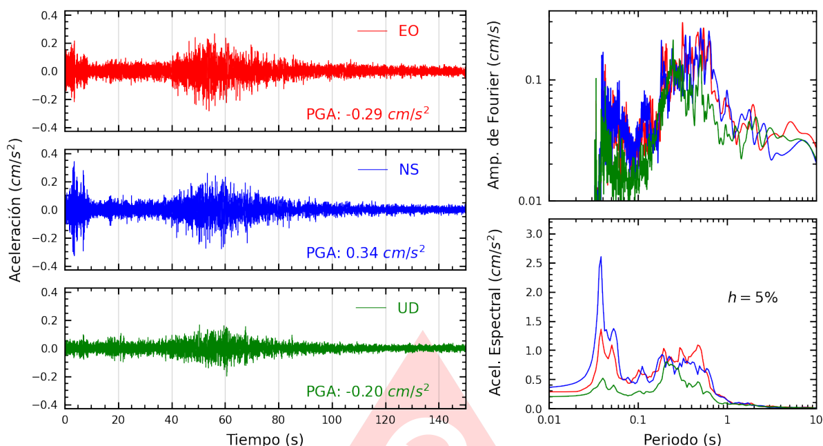
Figura A.25: Registros tiempo-historia, espectros de Fourier y de respuesta en las direcciones EO, NS y vertical de la estación UPCVI. Sismo de Ica, Ica - Ica del 2025-07-04, 03:55:11 (Hora local)
