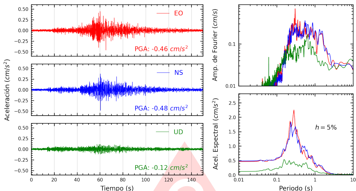
Figura A.15: Registros tiempo-historia, espectros de Fourier y de respuesta en las direcciones EO, NS y vertical de la estación DSML. Sismo de Ica, Ica - Ica del 2025-07-04, 03:55:11 (Hora local)
