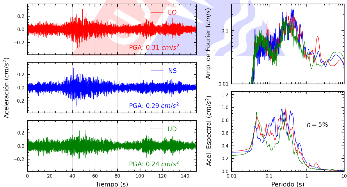
Figura A.26: Registros tiempo-historia, espectros de Fourier y de respuesta en las direcciones EO, NS y vertical de la estación URPE. Sismo de Ica, Ica - Ica del 2025-07-04, 03:55:11 (Hora local)
