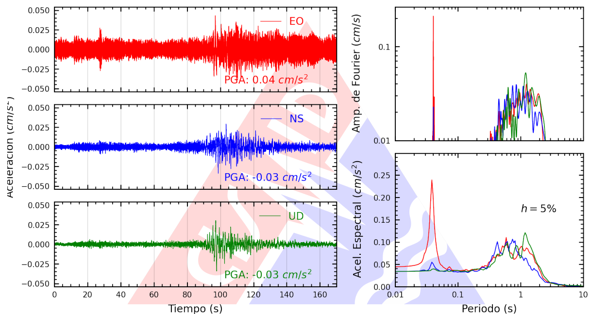
Figura A.49: Registros tiempo-historia, espectros de Fourier y de respuesta en las direcciones EO, NS y vertical de la estación UNAM. Sismo de Ica, Ica - Ica del 2025-07-04, 03:55:11 (Hora local)
