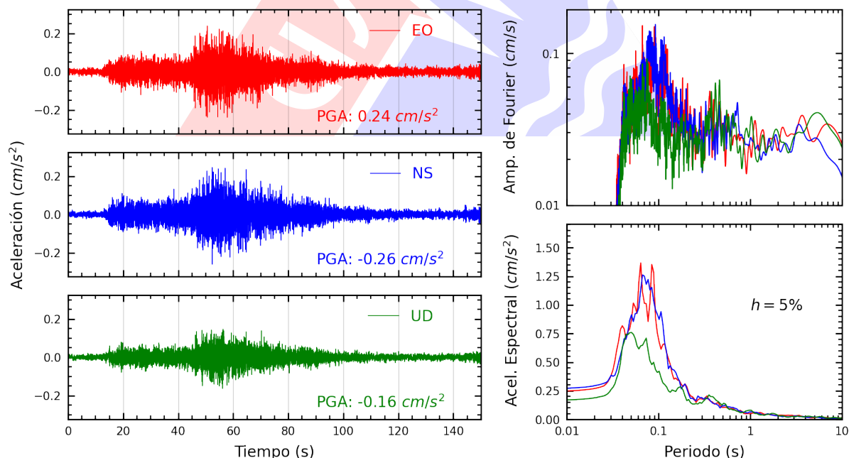
Figura A.34: Registros tiempo-historia, espectros de Fourier y de respuesta en las direcciones EO, NS y vertical de la estación JOSEO. Sismo de Ica, Ica - Ica del 2025-07-04, 03:55:11 (Hora local)
