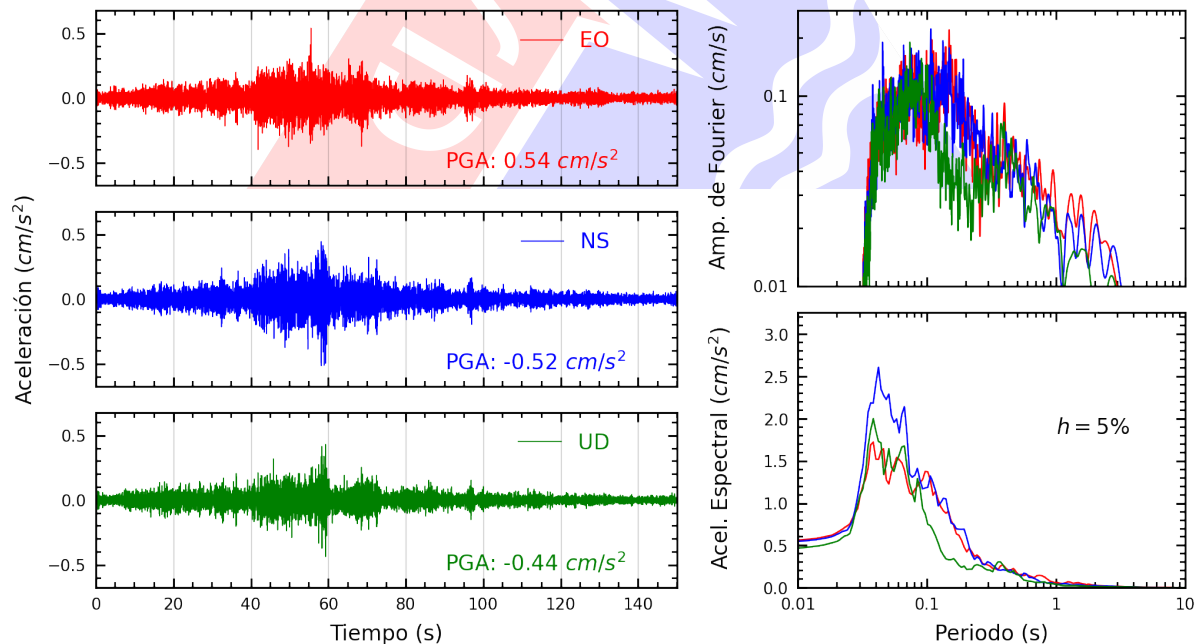
Figura A.14: Registros tiempo-historia, espectros de Fourier y de respuesta en las direcciones EO, NS y vertical de la estación SROSA. Sismo de Ica, Ica - Ica del 2025-07-04, 03:55:11 (Hora local)
