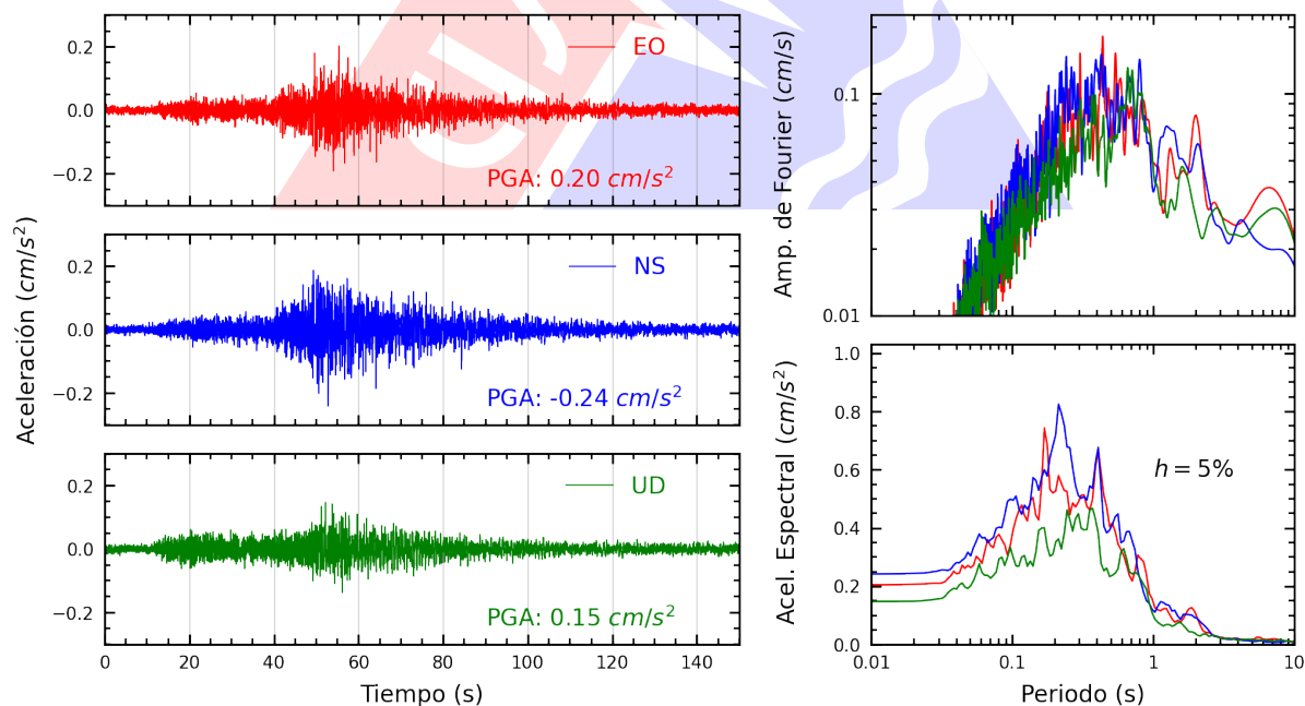
Figura A.36: Registros tiempo-historia, espectros de Fourier y de respuesta en las direcciones EO, NS y vertical de la estación SERVI. Sismo de Ica, Ica - Ica del 2025-07-04, 03:55:11 (Hora local)
