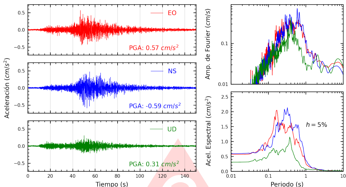
Figura A.11: Registros tiempo-historia, espectros de Fourier y de respuesta en las direcciones EO, NS y vertical de la estación USILP. Sismo de Ica, Ica - Ica del 2025-07-04, 03:55:11 (Hora local)
