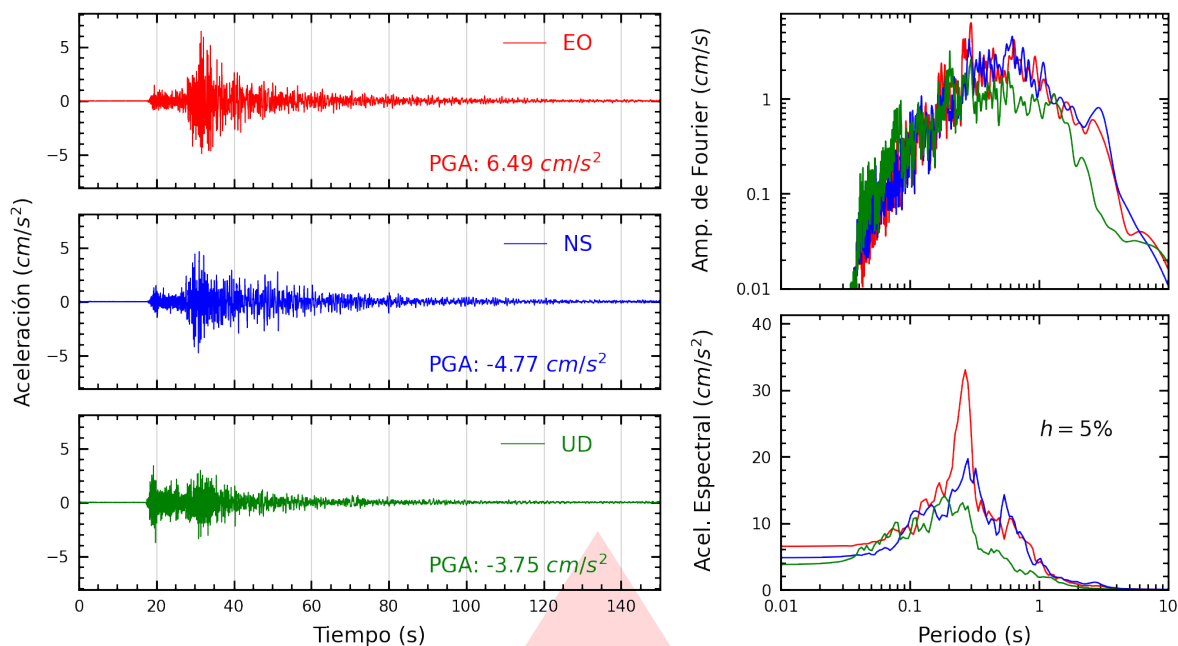
Figura A.1: Registros tiempo-historia, espectros de Fourier y de respuesta en las direcciones EO, NS y vertical de la estación UNICA. Sismo de Ica, Ica - Ica del 2025-07-04, 03:55:11 (Hora local)
