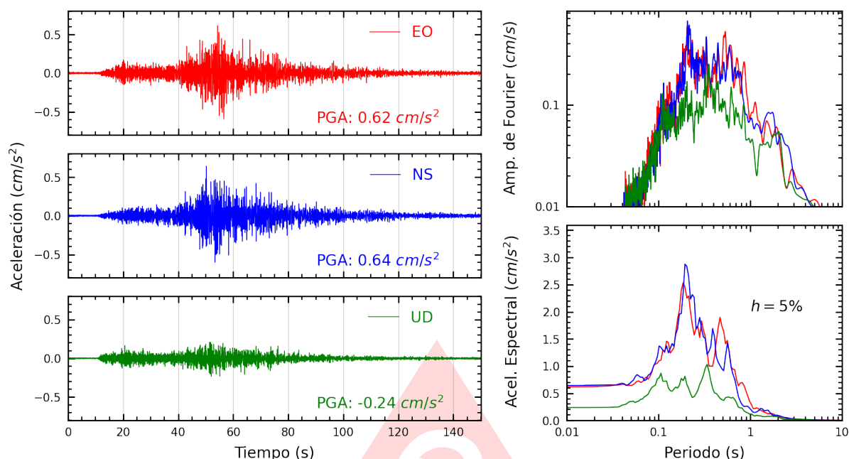
Figura A.7: Registros tiempo-historia, espectros de Fourier y de respuesta en las direcciones EO, NS y vertical de la estación SCCHO. Sismo de Ica, Ica - Ica del 2025-07-04, 03:55:11 (Hora local)
