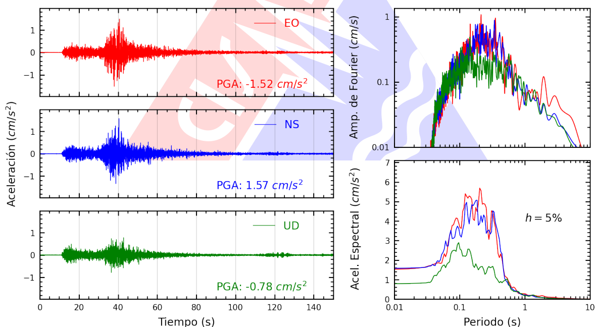
Figura A.2: Registros tiempo-historia, espectros de Fourier y de respuesta en las direcciones EO, NS y vertical de la estación ASIA. Sismo de Ica, Ica - Ica del 2025-07-04, 03:55:11 (Hora local)
