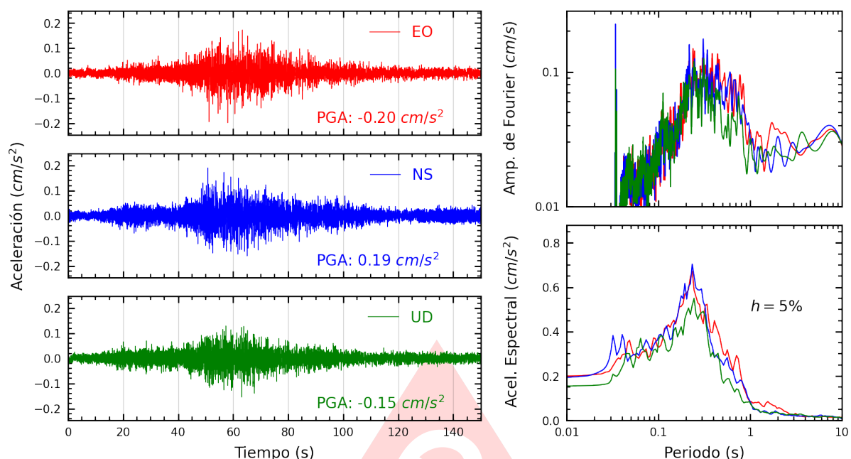
Figura A.43: Registros tiempo-historia, espectros de Fourier y de respuesta en las direcciones EO, NS y vertical de la estación USMP. Sismo de Ica, Ica - Ica del 2025-07-04, 03:55:11 (Hora local)
