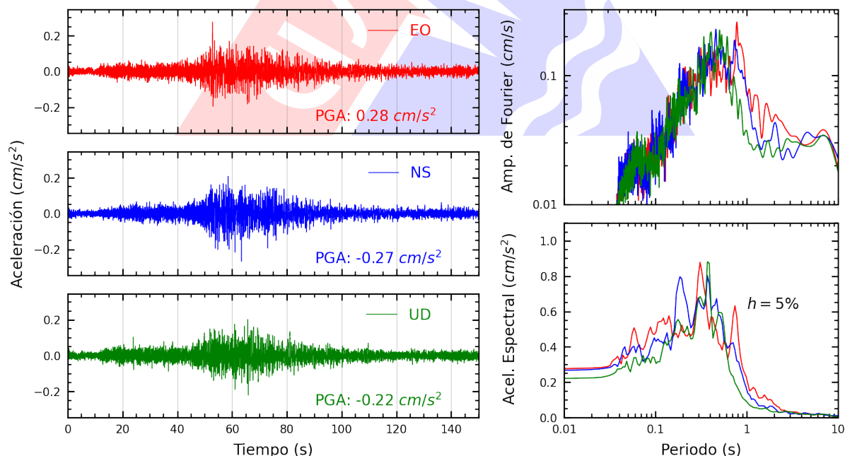
Figura A.32: Registros tiempo-historia, espectros de Fourier y de respuesta en las direcciones EO, NS y vertical de la estación IMCA. Sismo de Ica, Ica - Ica del 2025-07-04, 03:55:11 (Hora local)
