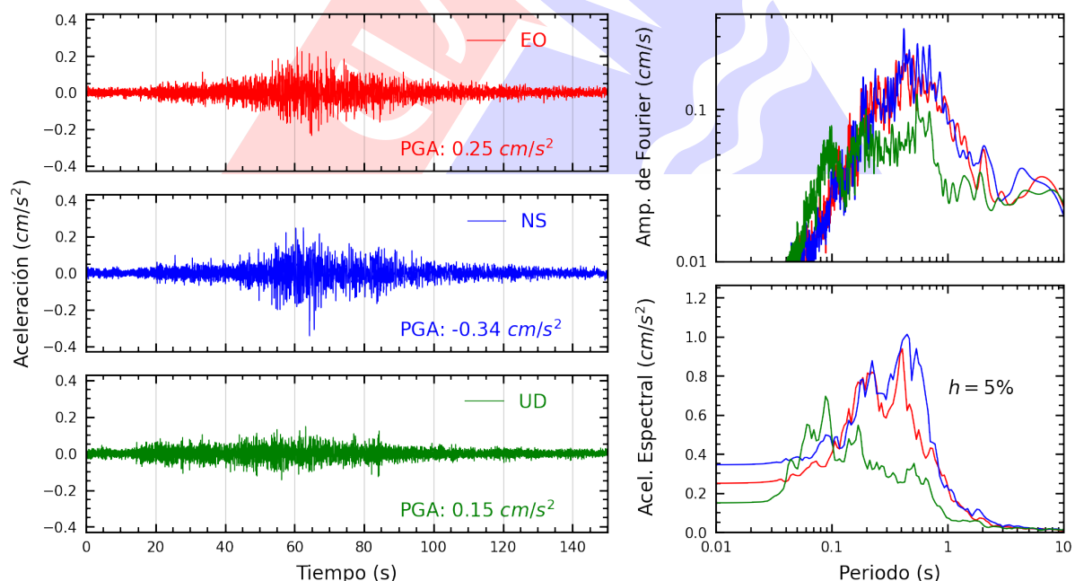
Figura A.24: Registros tiempo-historia, espectros de Fourier y de respuesta en las direcciones EO, NS y vertical de la estación RAMON. Sismo de Ica, Ica - Ica del 2025-07-04, 03:55:11 (Hora local)
