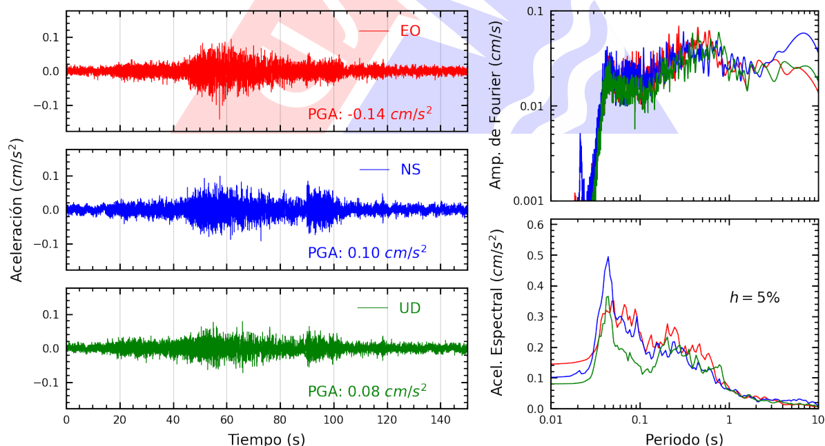
Figura A.46: Registros tiempo-historia, espectros de Fourier y de respuesta en las direcciones EO, NS y vertical de la estación SJLCE. Sismo de Ica, Ica - Ica del 2025-07-04, 03:55:11 (Hora local)
