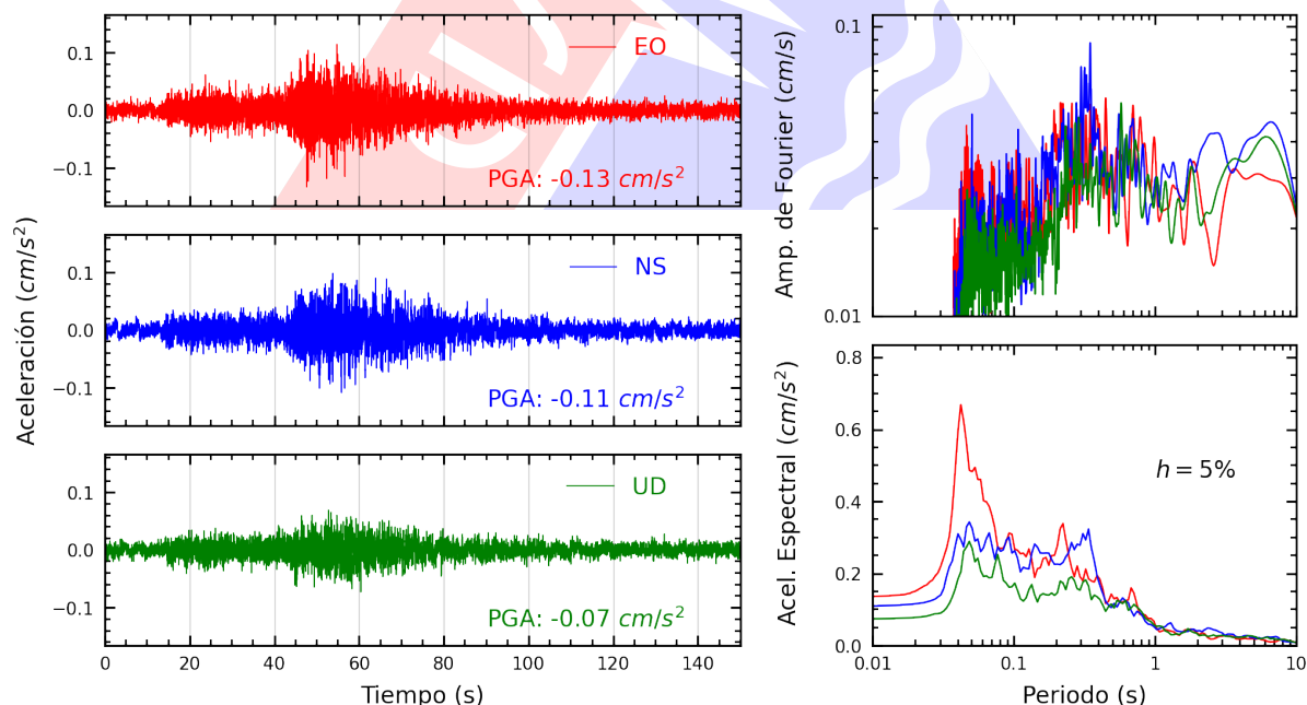
Figura A.48: Registros tiempo-historia, espectros de Fourier y de respuesta en las direcciones EO, NS y vertical de la estación UCSS. Sismo de Ica, Ica - Ica del 2025-07-04, 03:55:11 (Hora local)
