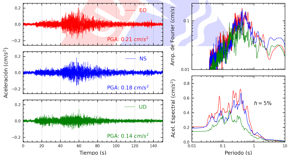
Figura A.40: Registros tiempo-historia, espectros de Fourier y de respuesta en las direcciones EO, NS y vertical de la estación CEPRE. Sismo de Ica, Ica - Ica del 2025-07-04, 03:55:11 (Hora local)
