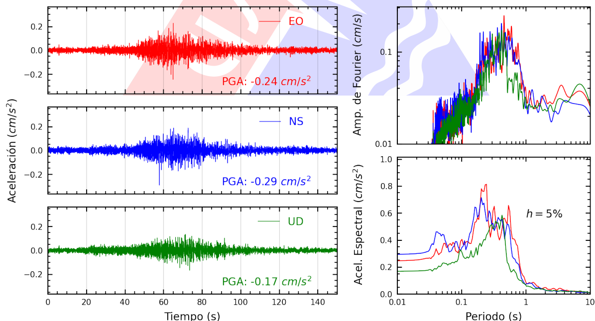
Figura A.28: Registros tiempo-historia, espectros de Fourier y de respuesta en las direcciones EO, NS y vertical de la estación COMAS. Sismo de Ica, Ica - Ica del 2025-07-04, 03:55:11 (Hora local)
