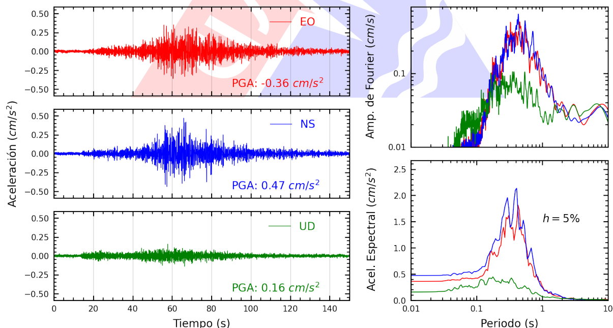
Figura A.16: Registros tiempo-historia, espectros de Fourier y de respuesta en las direcciones EO, NS y vertical de la estación ACAPU. Sismo de Ica, Ica - Ica del 2025-07-04, 03:55:11 (Hora local)
