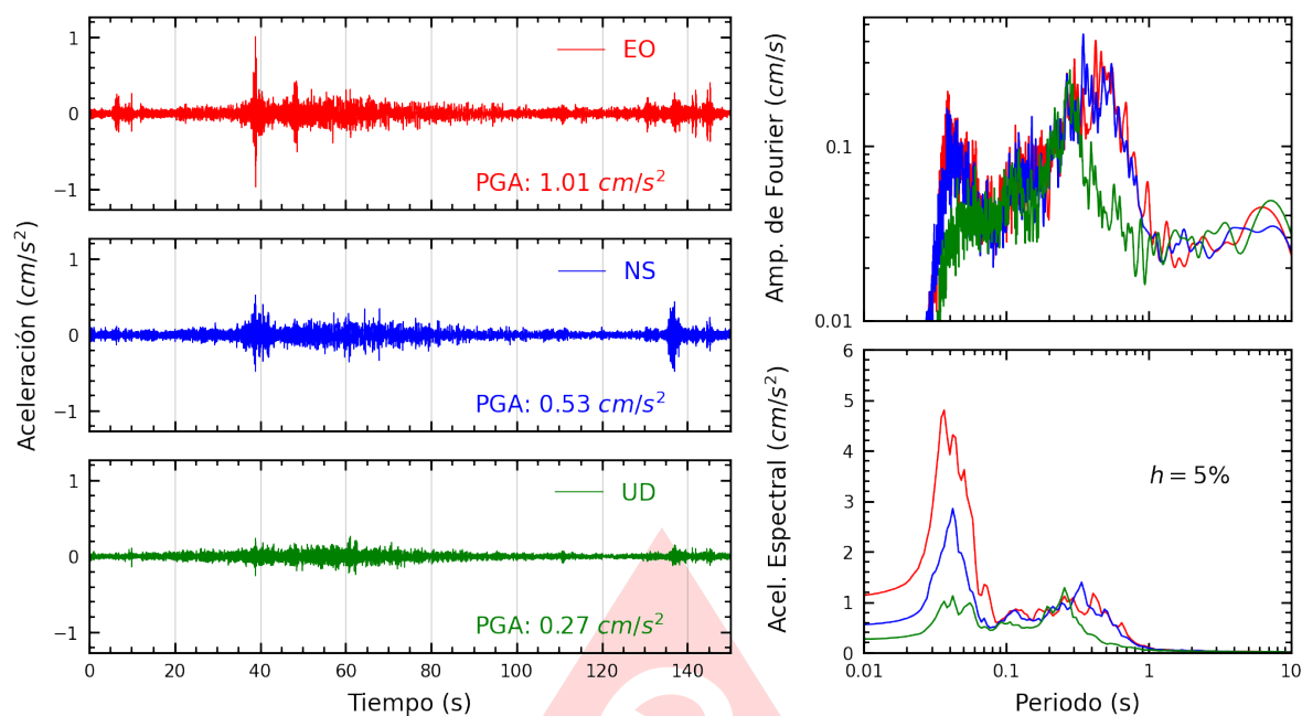
Figura A.3: Registros tiempo-historia, espectros de Fourier y de respuesta en las direcciones EO, NS y vertical de la estación OLIVO. Sismo de Ica, Ica - Ica del 2025-07-04, 03:55:11 (Hora local)
