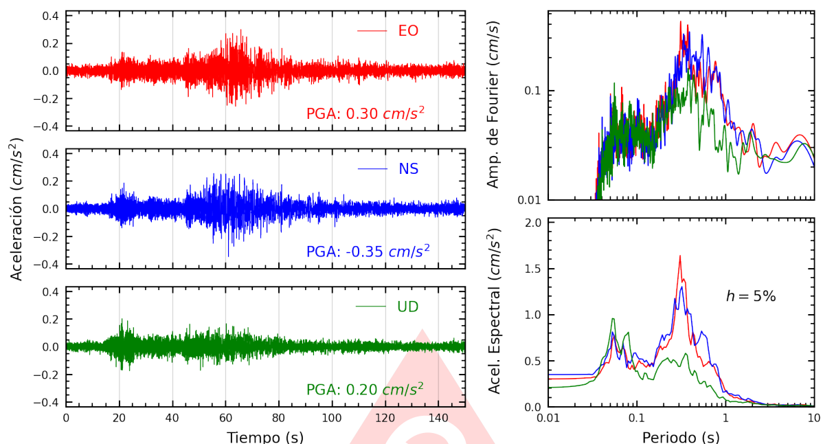
Figura A.23: Registros tiempo-historia, espectros de Fourier y de respuesta en las direcciones EO, NS y vertical de la estación MADRE. Sismo de Ica, Ica - Ica del 2025-07-04, 03:55:11 (Hora local)
