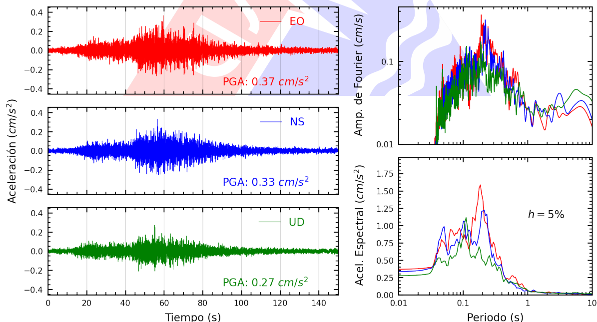
Figura A.22: Registros tiempo-historia, espectros de Fourier y de respuesta en las direcciones EO, NS y vertical de la estación INDEP. Sismo de Ica, Ica - Ica del 2025-07-04, 03:55:11 (Hora local)
