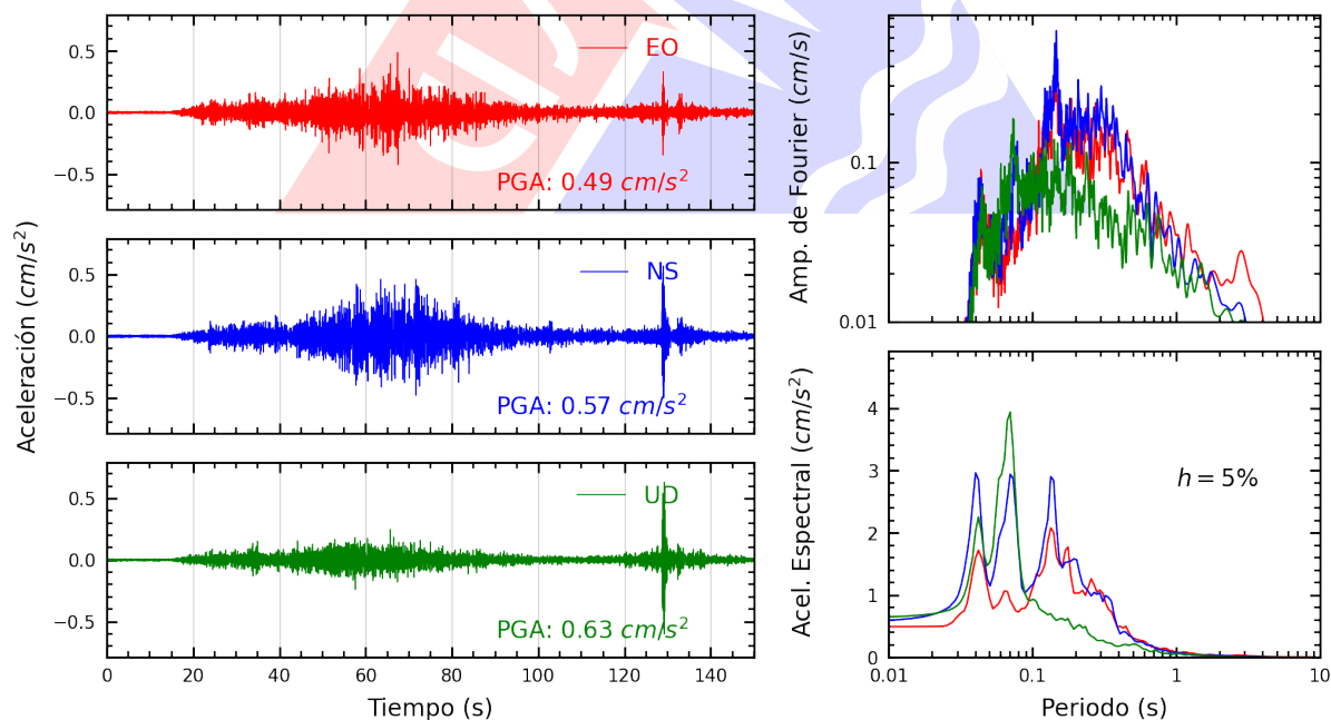
Figura A.8: Registros tiempo-historia, espectros de Fourier y de respuesta en las direcciones EO, NS y vertical de la estación CARAB. Sismo de Ica, Ica - Ica del 2025-07-04, 03:55:11 (Hora local)
