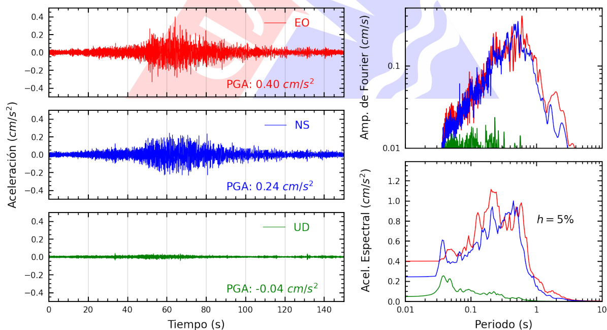
Figura A.20: Registros tiempo-historia, espectros de Fourier y de respuesta en las direcciones EO, NS y vertical de la estación UCVAT. Sismo de Ica, Ica - Ica del 2025-07-04, 03:55:11 (Hora local)
