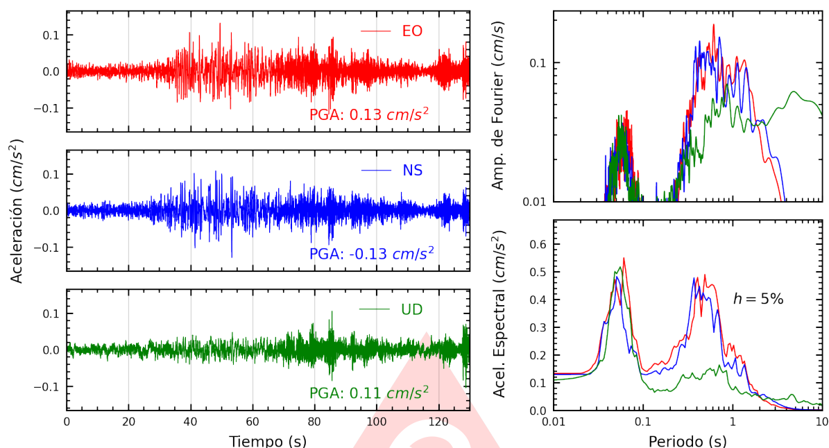
Figura A.47: Registros tiempo-historia, espectros de Fourier y de respuesta en las direcciones EO, NS y vertical de la estación SCARQ. Sismo de Ica, Ica - Ica del 2025-07-04, 03:55:11 (Hora local)
