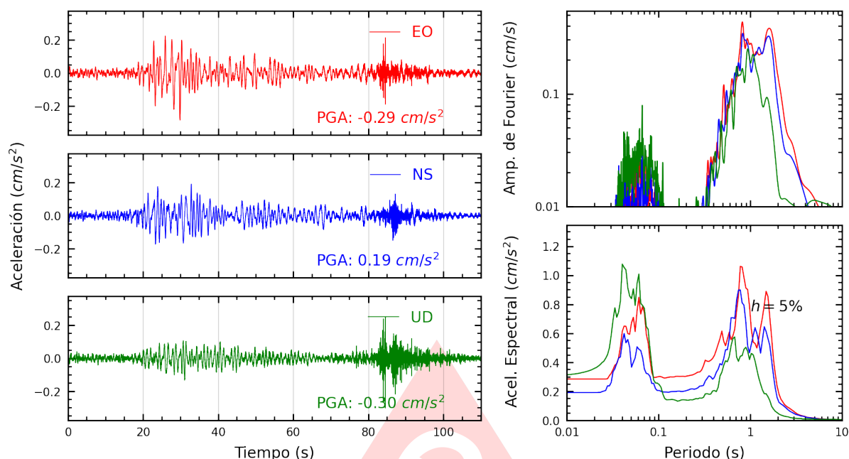
Figura A.27: Registros tiempo-historia, espectros de Fourier y de respuesta en las direcciones EO, NS y vertical de la estación SCCUS. Sismo de Ica, Ica - Ica del 2025-07-04, 03:55:11 (Hora local)
