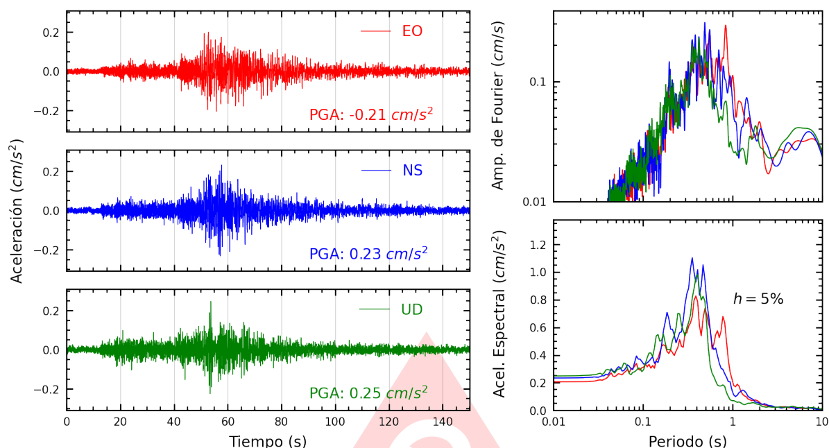
Figura A.35: Registros tiempo-historia, espectros de Fourier y de respuesta en las direcciones EO, NS y vertical de la estación UNFV. Sismo de Ica, Ica - Ica del 2025-07-04, 03:55:11 (Hora local)
