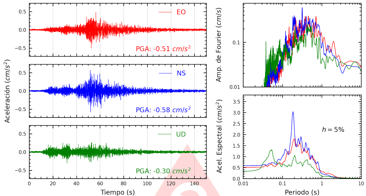
Figura A.13: Registros tiempo-historia, espectros de Fourier y de respuesta en las direcciones EO, NS y vertical de la estación SOCHO. Sismo de Ica, Ica - Ica del 2025-07-04, 03:55:11 (Hora local)
