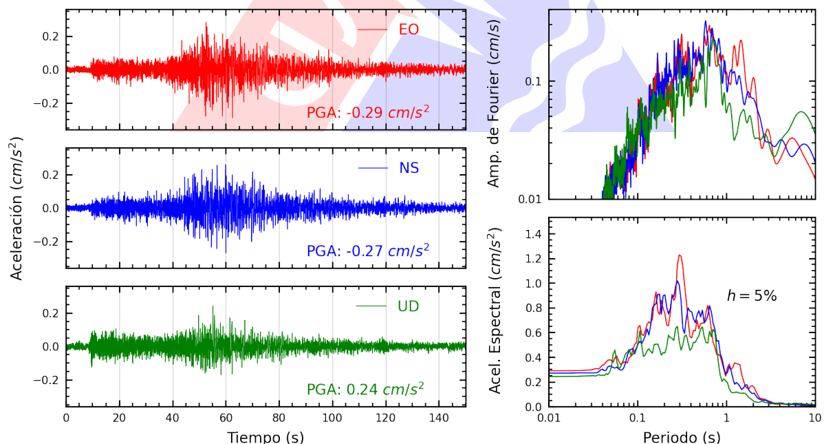
Figura A.30: Registros tiempo-historia, espectros de Fourier y de respuesta en las direcciones EO, NS y vertical de la estación PRADO. Sismo de Ica, Ica - Ica del 2025-07-04, 03:55:11 (Hora local)
