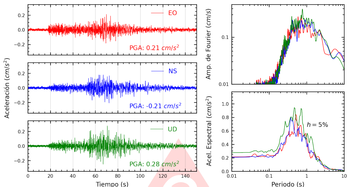
Figura A.31: Registros tiempo-historia, espectros de Fourier y de respuesta en las direcciones EO, NS y vertical de la estación UNSCH. Sismo de Ica, Ica - Ica del 2025-07-04, 03:55:11 (Hora local)
