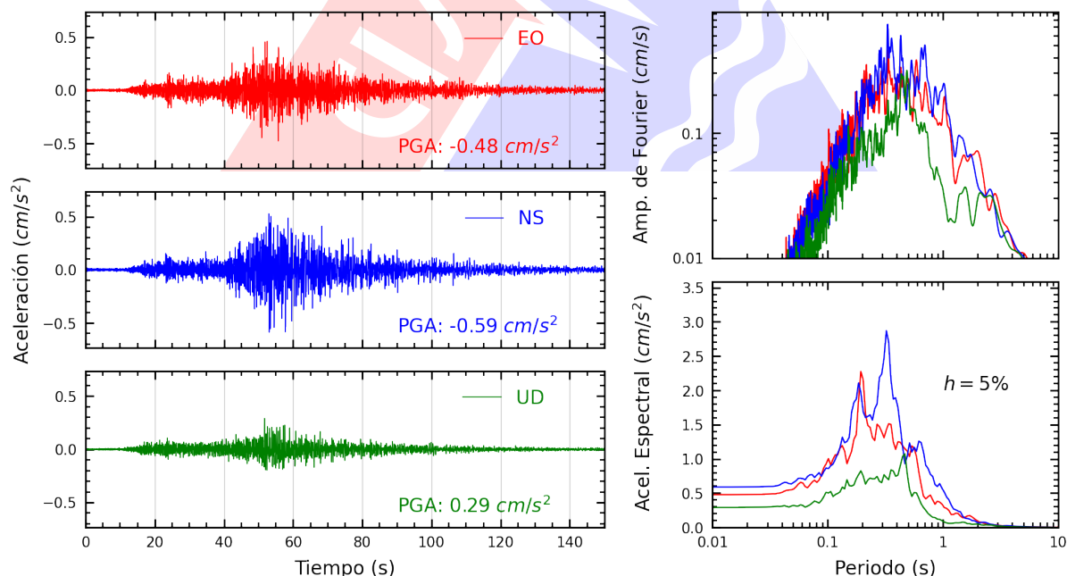
Figura A.12: Registros tiempo-historia, espectros de Fourier y de respuesta en las direcciones EO, NS y vertical de la estación BRIS2. Sismo de Ica, Ica - Ica del 2025-07-04, 03:55:11 (Hora local)
