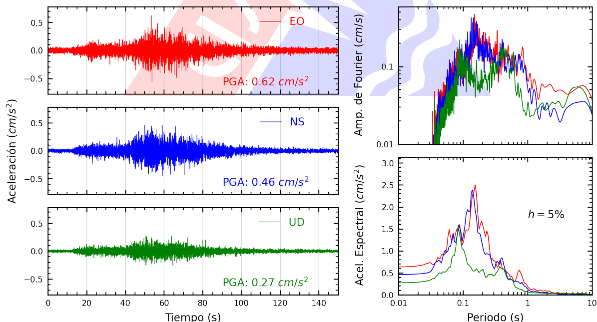
Figura A.10: Registros tiempo-historia, espectros de Fourier y de respuesta en las direcciones EO, NS y vertical de la estación USILM. Sismo de Ica, Ica - Ica del 2025-07-04, 03:55:11 (Hora local)
