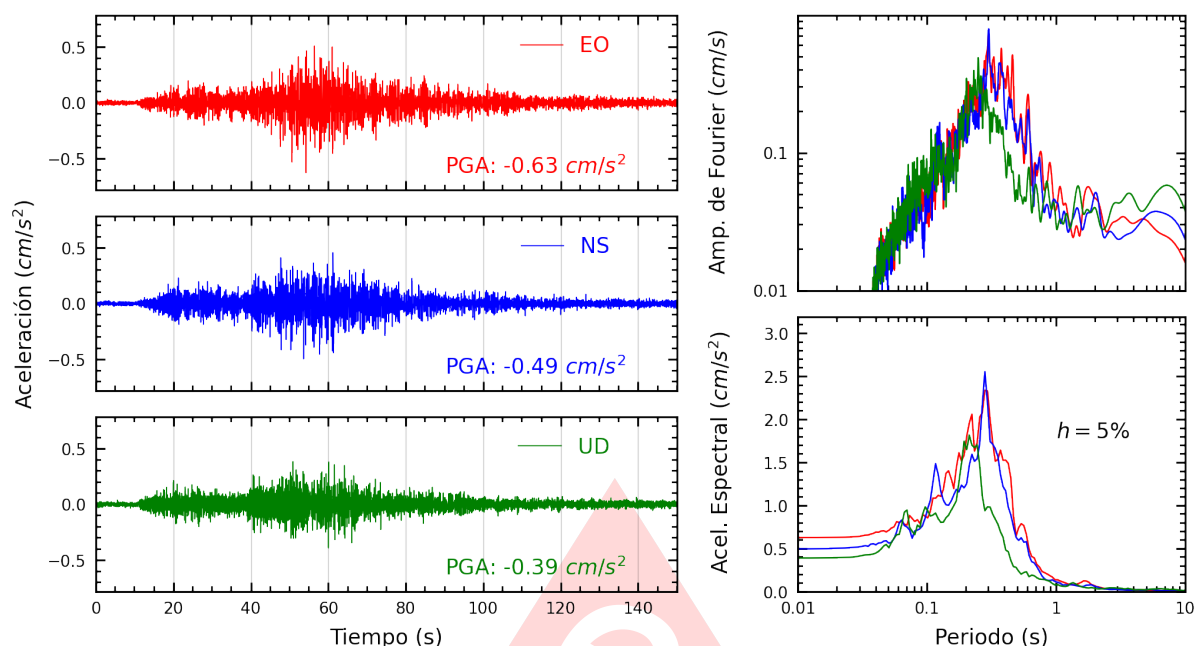
Figura A.9: Registros tiempo-historia, espectros de Fourier y de respuesta en las direcciones EO, NS y vertical de la estación SOVES. Sismo de Ica, Ica - Ica del 2025-07-04, 03:55:11 (Hora local)
