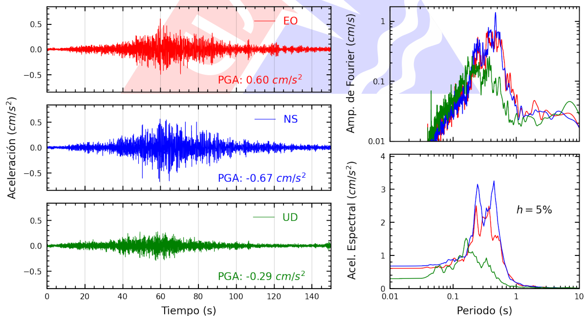
Figura A.6: Registros tiempo-historia, espectros de Fourier y de respuesta en las direcciones EO, NS y vertical de la estación MDPP. Sismo de Ica, Ica - Ica del 2025-07-04, 03:55:11 (Hora local)
