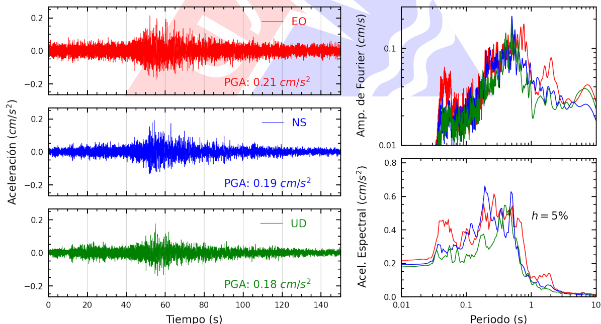
Figura A.38: Registros tiempo-historia, espectros de Fourier y de respuesta en las direcciones EO, NS y vertical de la estación INICT. Sismo de Ica, Ica - Ica del 2025-07-04, 03:55:11 (Hora local)
