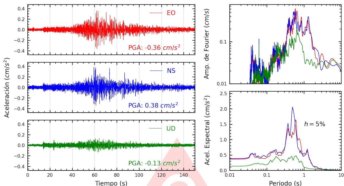
Figura A.21: Registros tiempo-historia, espectros de Fourier y de respuesta en las direcciones EO, NS y vertical de la estación DHNPE. Sismo de Ica, Ica - Ica del 2025-07-04, 03:55:11 (Hora local)
