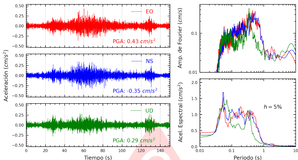
Figura A.19: Registros tiempo-historia, espectros de Fourier y de respuesta en las direcciones EO, NS y vertical de la estación SJLSV. Sismo de Ica, Ica - Ica del 2025-07-04, 03:55:11 (Hora local)
