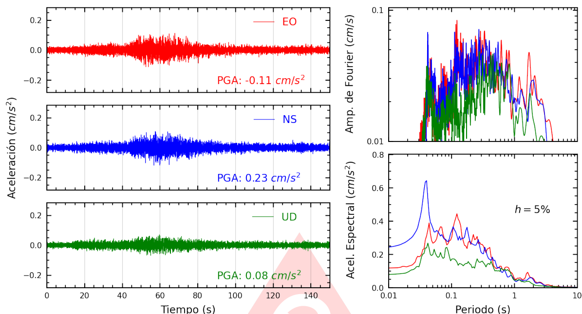
Figura A.37: Registros tiempo-historia, espectros de Fourier y de respuesta en las direcciones EO, NS y vertical de la estación ATARJ. Sismo de Ica, Ica - Ica del 2025-07-04, 03:55:11 (Hora local)
