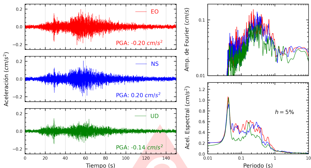
Figura A.41: Registros tiempo-historia, espectros de Fourier y de respuesta en las direcciones EO, NS y vertical de la estación FICPE. Sismo de Ica, Ica - Ica del 2025-07-04, 03:55:11 (Hora local)
