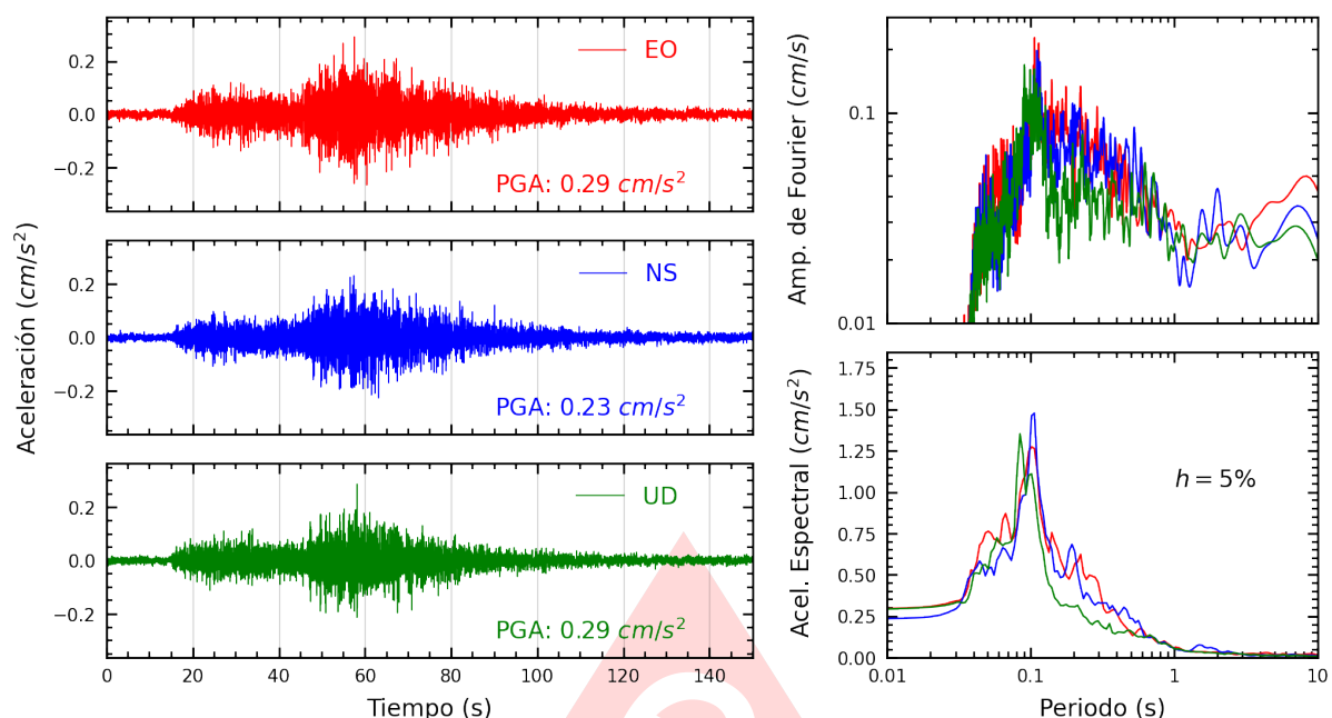
Figura A.29: Registros tiempo-historia, espectros de Fourier y de respuesta en las direcciones EO, NS y vertical de la estación AMORE. Sismo de Ica, Ica - Ica del 2025-07-04, 03:55:11 (Hora local)
