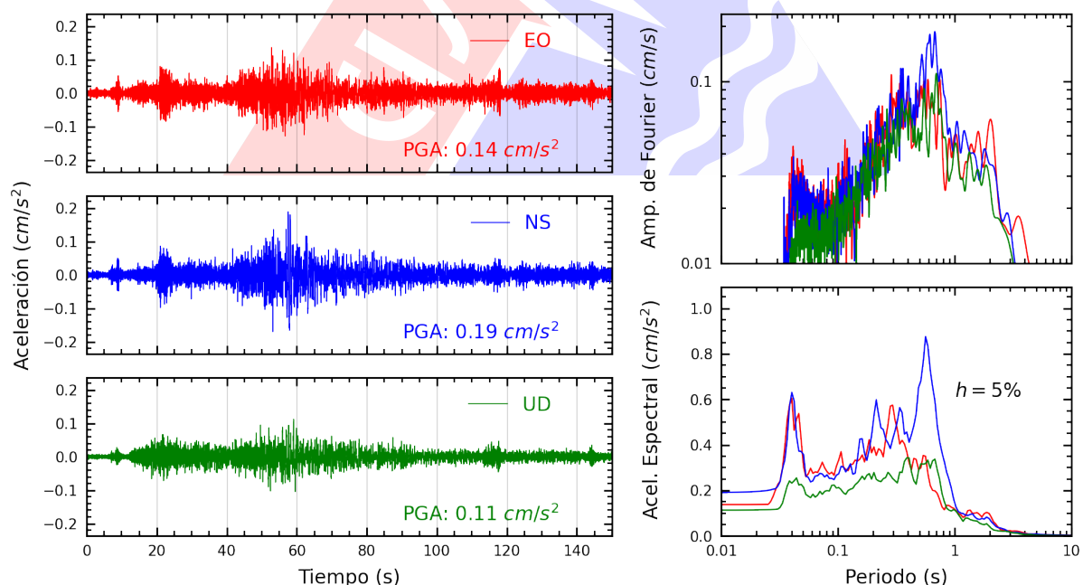
Figura A.44: Registros tiempo-historia, espectros de Fourier y de respuesta en las direcciones EO, NS y vertical de la estación BORJA. Sismo de Ica, Ica - Ica del 2025-07-04, 03:55:11 (Hora local)
