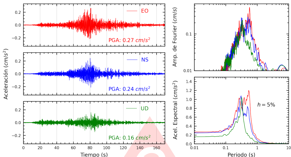
Figura A.33: Registros tiempo-historia, espectros de Fourier y de respuesta en las direcciones EO, NS y vertical de la estación CARAL. Sismo de Ica, Ica - Ica del 2025-07-04, 03:55:11 (Hora local)
