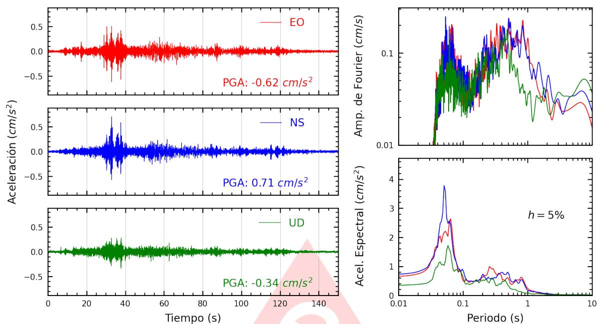
Figura A.5: Registros tiempo-historia, espectros de Fourier y de respuesta en las direcciones EO, NS y vertical de la estación UPCS. Sismo de Ica, Ica - Ica del 2025-07-04, 03:55:11 (Hora local)
