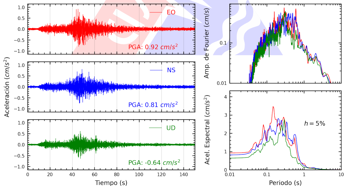
Figura A.4: Registros tiempo-historia, espectros de Fourier y de respuesta en las direcciones EO, NS y vertical de la estación PHERM. Sismo de Ica, Ica - Ica del 2025-07-04, 03:55:11 (Hora local)
