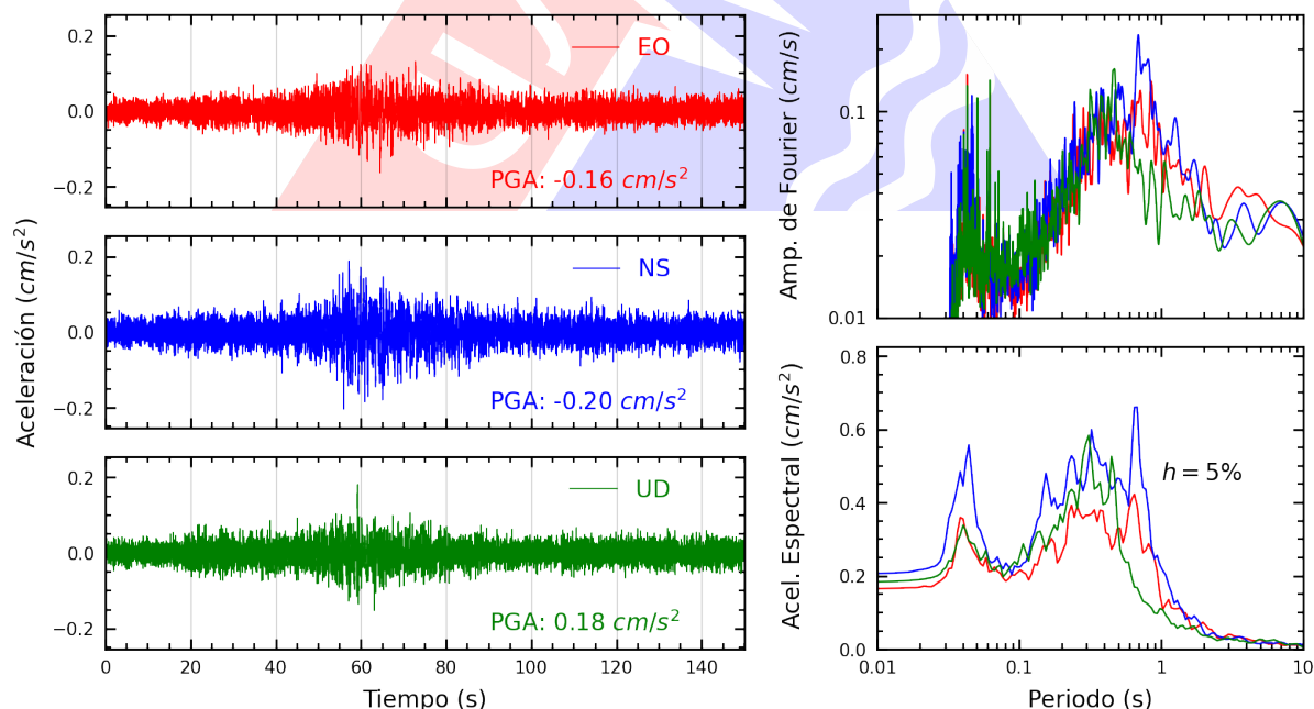
Figura A.42: Registros tiempo-historia, espectros de Fourier y de respuesta en las direcciones EO, NS y vertical de la estación BONDY. Sismo de Ica, Ica - Ica del 2025-07-04, 03:55:11 (Hora local)
