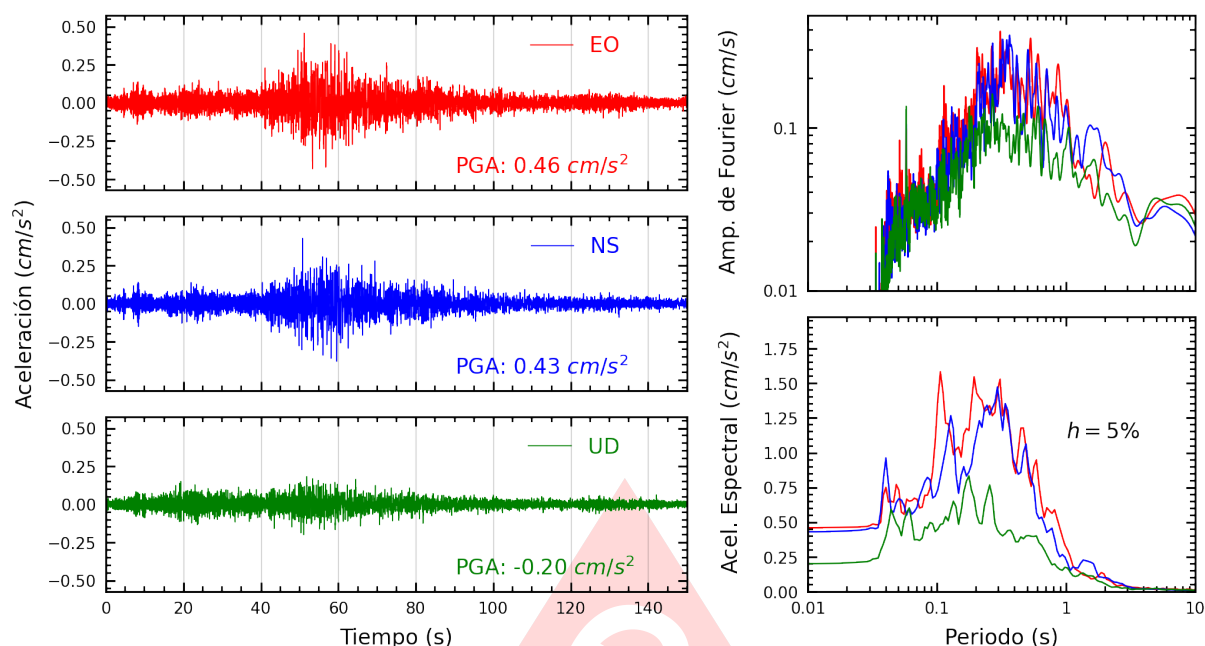
Figura A.17: Registros tiempo-historia, espectros de Fourier y de respuesta en las direcciones EO, NS y vertical de la estación SOBAR. Sismo de Ica, Ica - Ica del 2025-07-04, 03:55:11 (Hora local)
