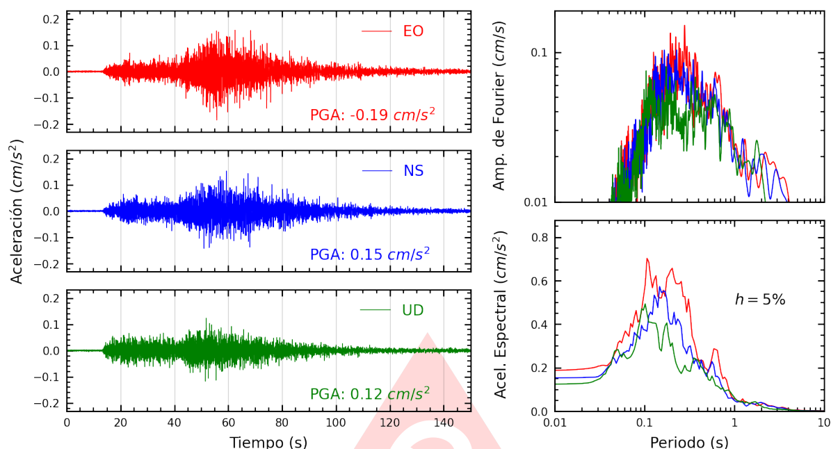
Figura A.45: Registros tiempo-historia, espectros de Fourier y de respuesta en las direcciones EO, NS y vertical de la estación JALV2. Sismo de Ica, Ica - Ica del 2025-07-04, 03:55:11 (Hora local)
