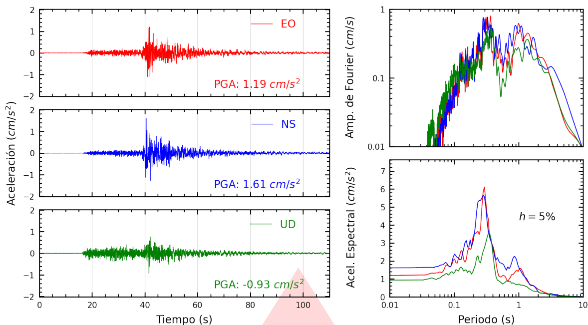
Figura A.1: Registros tiempo-historia, espectros de Fourier y de respuesta en las direcciones EO, NS y vertical de la estación UNJ. Sismo de Nueva Cajamarca, Rioja - San Martín del 2025-07-06, 06:27:45 (Hora local)
