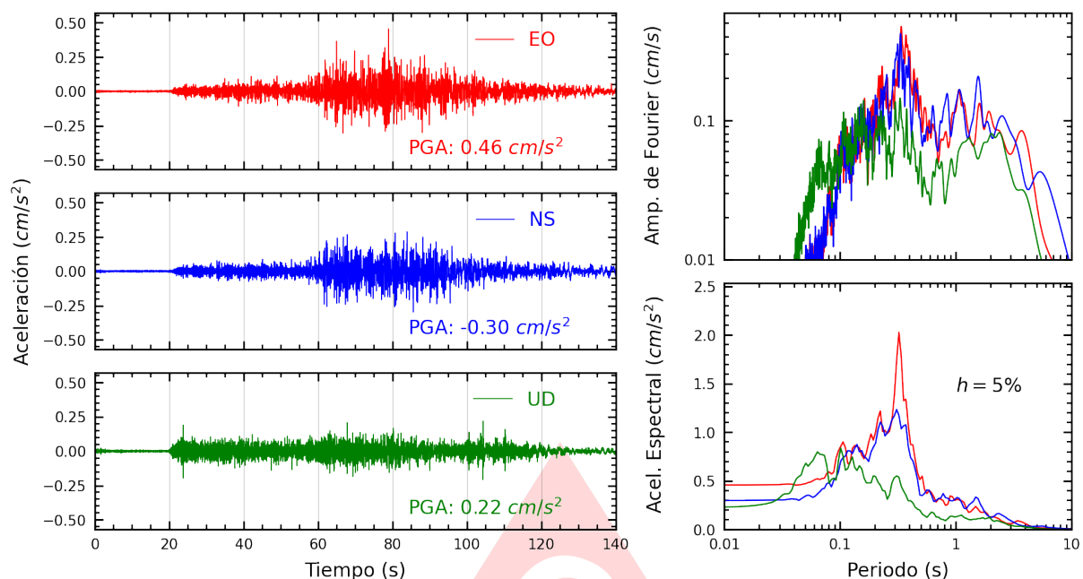
Figura A.3: Registros tiempo-historia, espectros de Fourier y de respuesta en las direcciones EO, NS y vertical de la estación UNP. Sismo de Nueva Cajamarca, Rioja - San Martín del 2025-07-06, 06:27:45 (Hora local)
