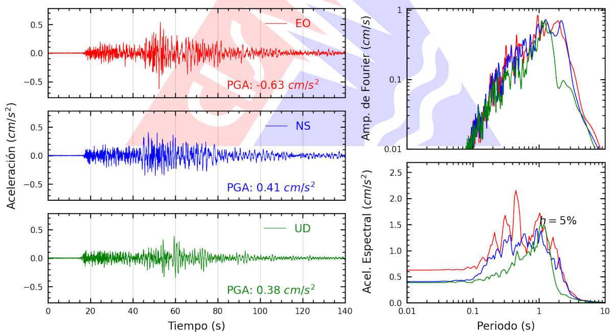
Figura A.2: Registros tiempo-historia, espectros de Fourier y de respuesta en las direcciones EO, NS y vertical de la estación UNC. Sismo de Nueva Cajamarca, Rioja - San Martín del 2025-07-06, 06:27:45 (Hora local)
