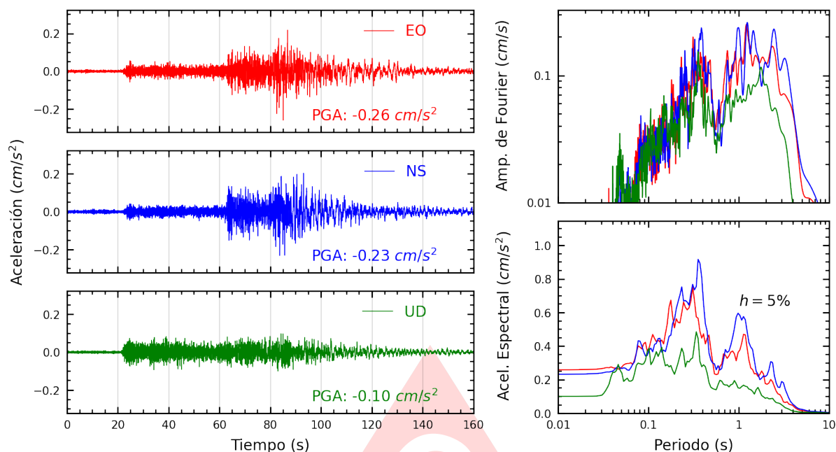
Figura A.5: Registros tiempo-historia, espectros de Fourier y de respuesta en las direcciones EO, NS y vertical de la estación UNF. Sismo de Nueva Cajamarca, Rioja - San Martín del 2025-07-06, 06:27:45 (Hora local)
