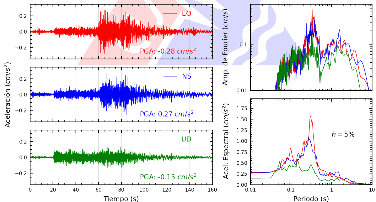
Figura A.4: Registros tiempo-historia, espectros de Fourier y de respuesta en las direcciones EO, NS y vertical de la estación UPAOP. Sismo de Nueva Cajamarca, Rioja - San Martín del 2025-07-06, 06:27:45 (Hora local)
