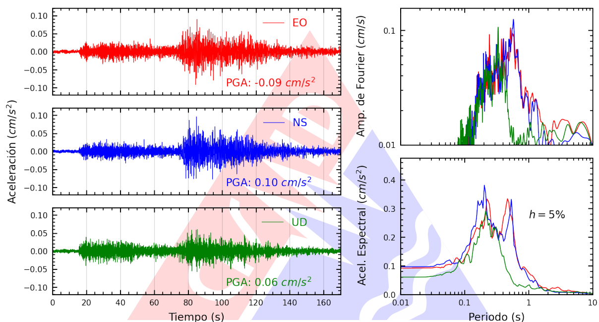
Figura A.7: Registros tiempo-historia, espectros de Fourier y de respuesta en las direcciones EO, NS y vertical de la estación CARAL. Sismo de Nueva Cajamarca, Rioja - San Martín del 2025-07-06, 06:27:45 (Hora local)
