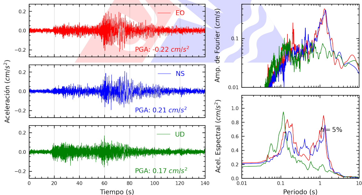
Figura A.6: Registros tiempo-historia, espectros de Fourier y de respuesta en las direcciones EO, NS y vertical de la estación UPAT. Sismo de Nueva Cajamarca, Rioja - San Martín del 2025-07-06, 06:27:45 (Hora local)
