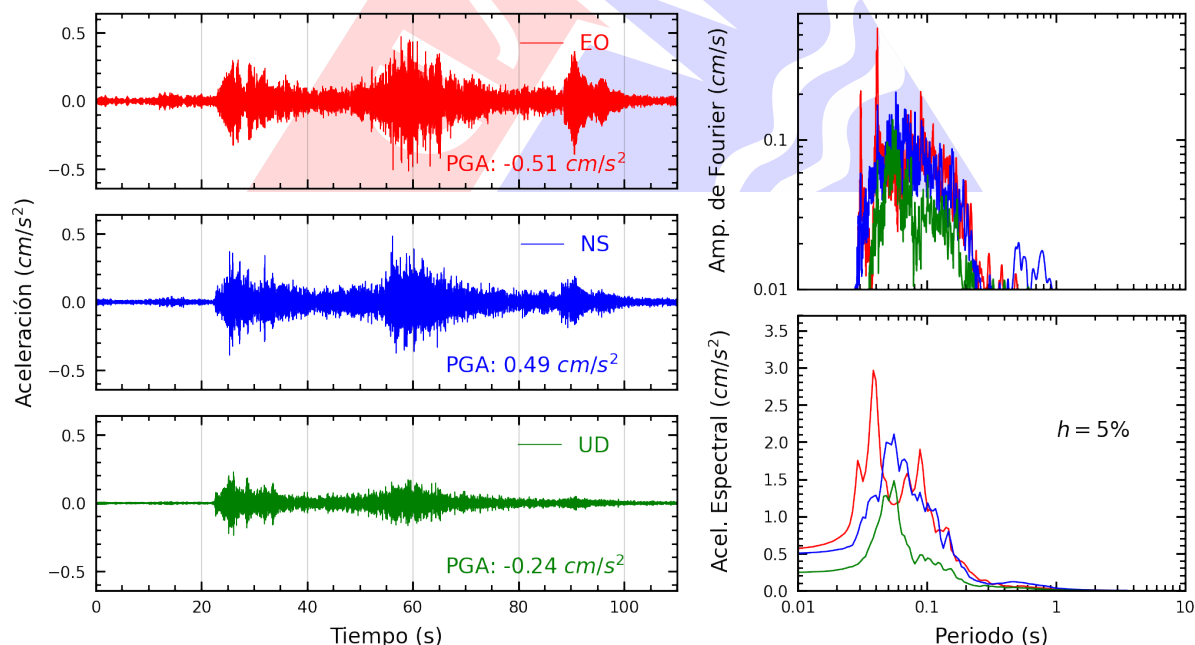
Figura A.4: Registros tiempo-historia, espectros de Fourier y de respuesta en las direcciones EO, NS y vertical de la estación UNAM. Sismo de Ilave, El Collao - Puno del 2025-07-07, 18:30:57 (Hora local)
