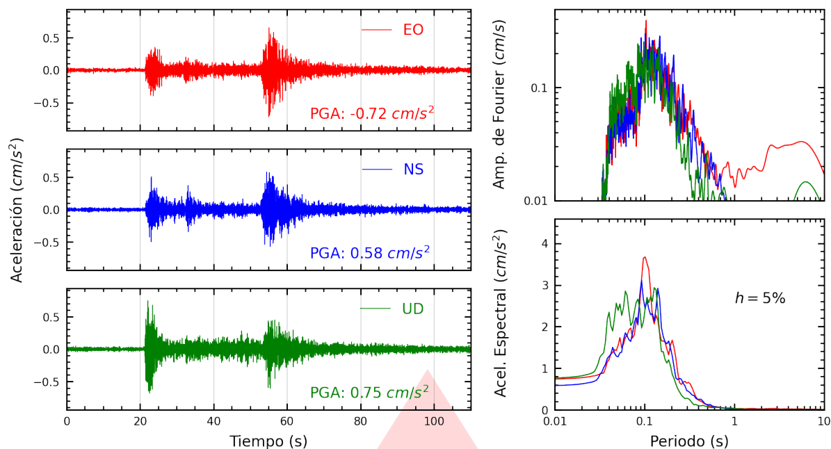
Figura A.1: Registros tiempo-historia, espectros de Fourier y de respuesta en las direcciones EO, NS y vertical de la estación UJBG3. Sismo de Ilave, El Collao - Puno del 2025-07-07, 18:30:57 (Hora local)
