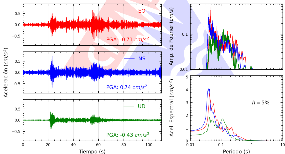
Figura A.2: Registros tiempo-historia, espectros de Fourier y de respuesta en las direcciones EO, NS y vertical de la estación UPTAC. Sismo de Ilave, El Collao - Puno del 2025-07-07, 18:30:57 (Hora local)
