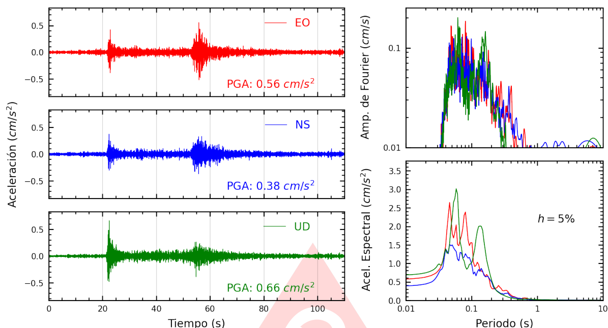
Figura A.3: Registros tiempo-historia, espectros de Fourier y de respuesta en las direcciones EO, NS y vertical de la estación CREY. Sismo de Ilave, El Collao - Puno del 2025-07-07, 18:30:57 (Hora local)
