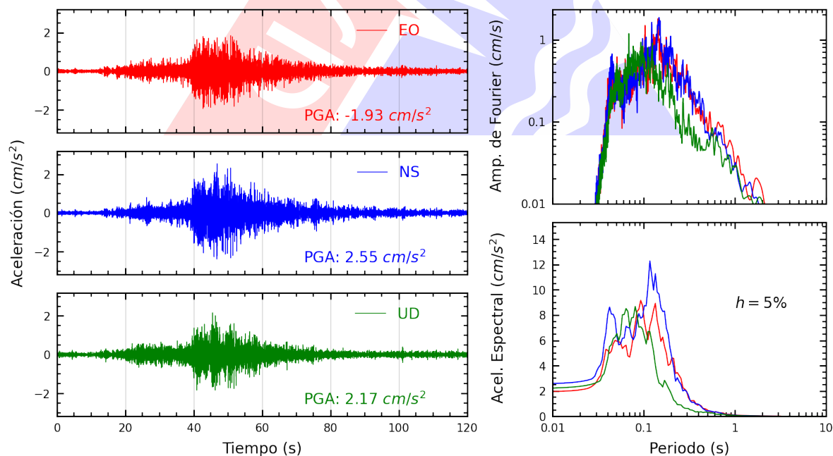
Figura A.18: Registros tiempo-historia, espectros de Fourier y de respuesta en las direcciones EO, NS y vertical de la estación CARAB. Sismo de Pisco, Pisco - Ica del 2025-07-08, 06:40:05 (Hora local)
