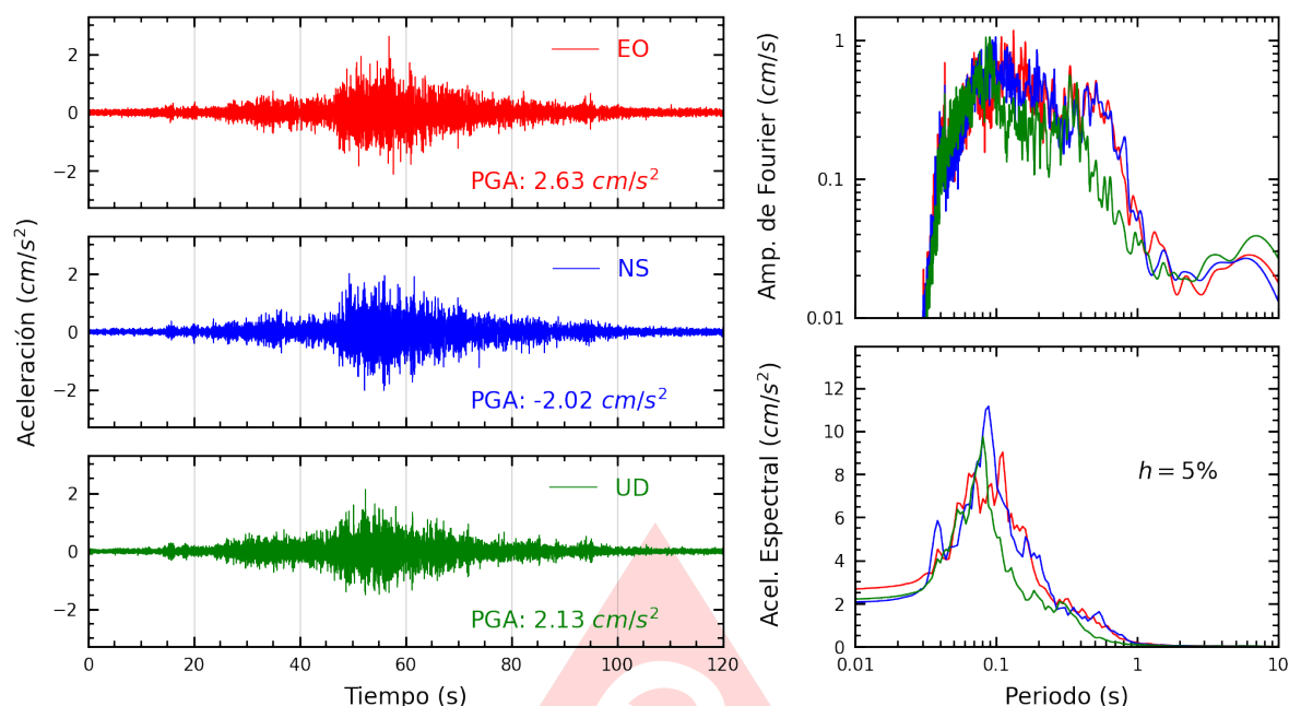
Figura A.17: Registros tiempo-historia, espectros de Fourier y de respuesta en las direcciones EO, NS y vertical de la estación SJLSV. Sismo de Pisco, Pisco - Ica del 2025-07-08, 06:40:05 (Hora local)
