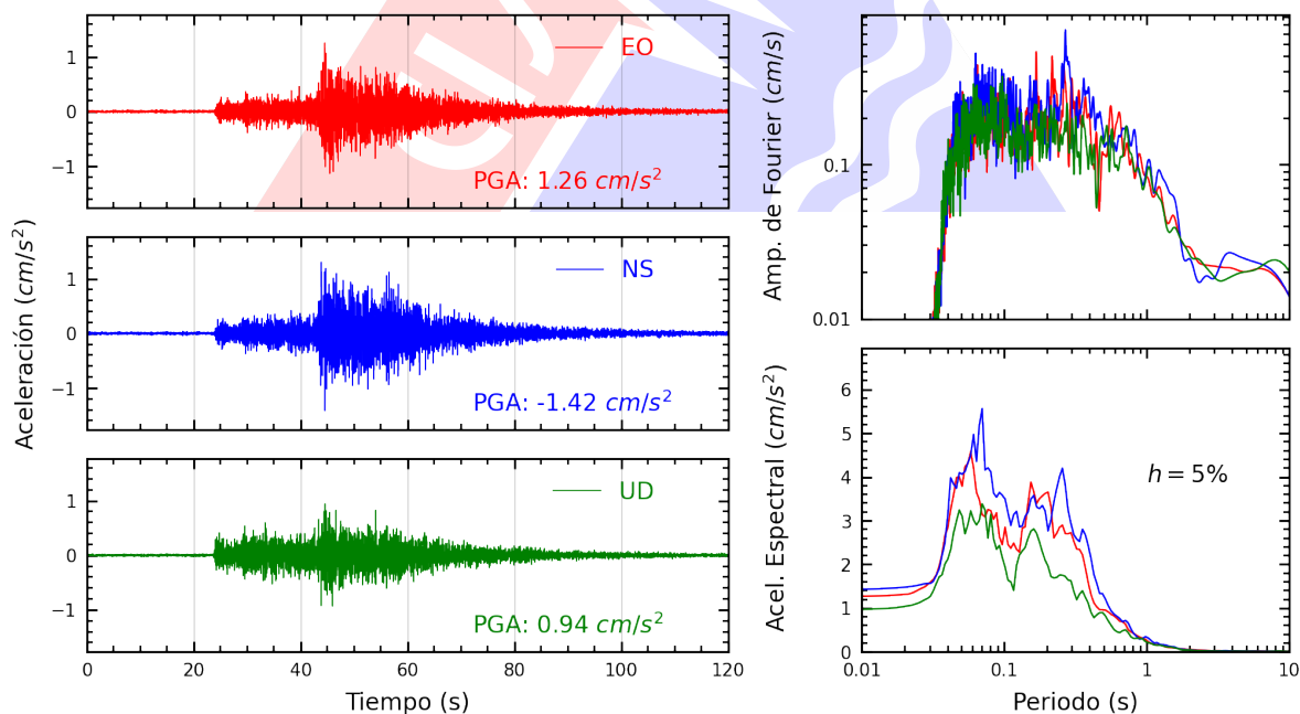
Figura A.30: Registros tiempo-historia, espectros de Fourier y de respuesta en las direcciones EO, NS y vertical de la estación SERVI. Sismo de Pisco, Pisco - Ica del 2025-07-08, 06:40:05 (Hora local)
