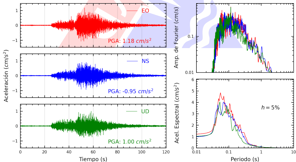
Figura A.40: Registros tiempo-historia, espectros de Fourier y de respuesta en las direcciones EO, NS y vertical de la estación JALV2. Sismo de Pisco, Pisco - Ica del 2025-07-08, 06:40:05 (Hora local)
