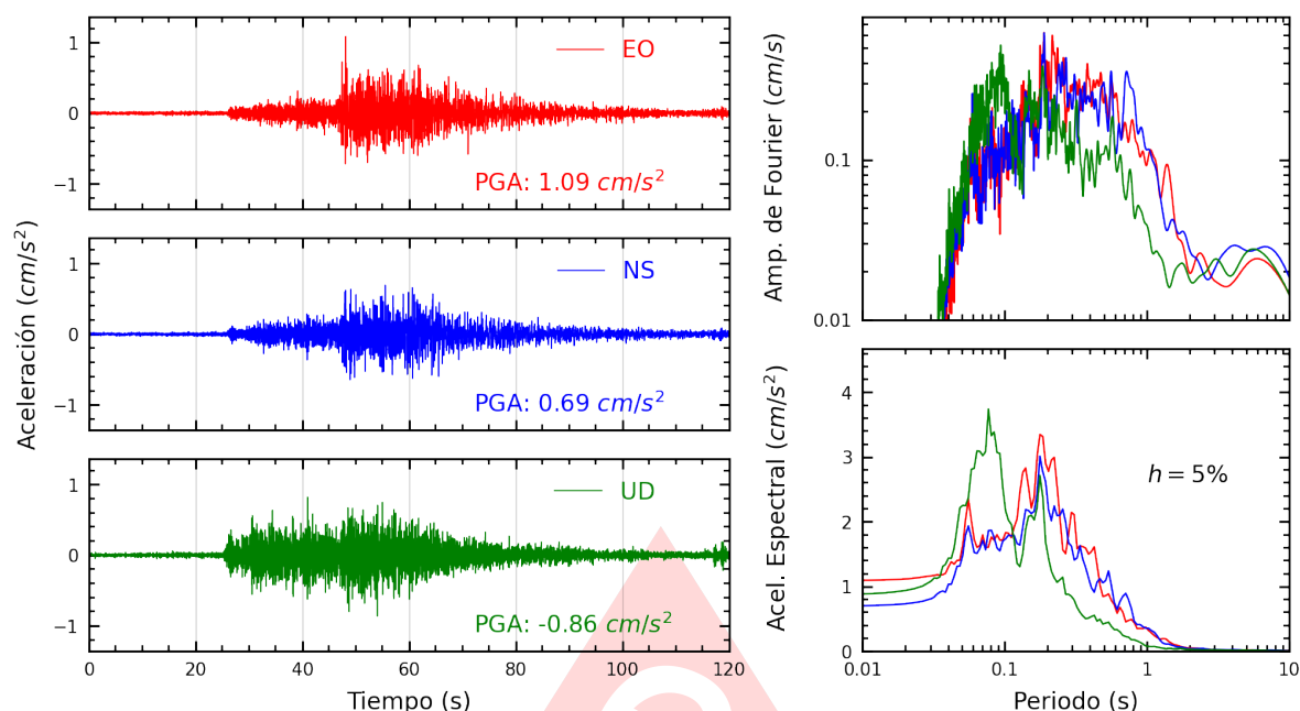
Figura A.41: Registros tiempo-historia, espectros de Fourier y de respuesta en las direcciones EO, NS y vertical de la estación RAMON. Sismo de Pisco, Pisco - Ica del 2025-07-08, 06:40:05 (Hora local)
