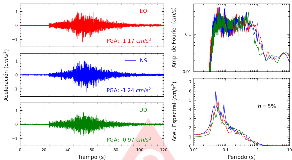
Figura A.39: Registros tiempo-historia, espectros de Fourier y de respuesta en las direcciones EO, NS y vertical de la estación IMCA. Sismo de Pisco, Pisco - Ica del 2025-07-08, 06:40:05 (Hora local)
