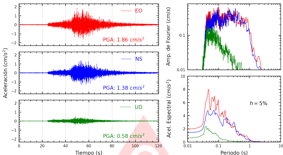
Figura A.23: Registros tiempo-historia, espectros de Fourier y de respuesta en las direcciones EO, NS y vertical de la estación UCVAT. Sismo de Pisco, Pisco - Ica del 2025-07-08, 06:40:05 (Hora local)
