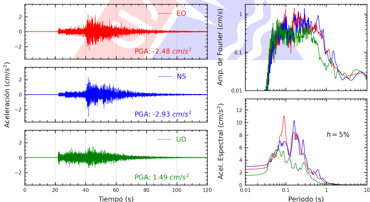
Figura A.12: Registros tiempo-historia, espectros de Fourier y de respuesta en las direcciones EO, NS y vertical de la estación USILP. Sismo de Pisco, Pisco - Ica del 2025-07-08, 06:40:05 (Hora local)
