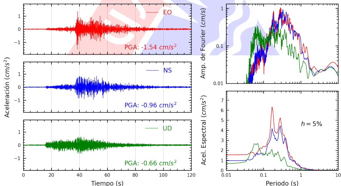
Figura A.28: Registros tiempo-historia, espectros de Fourier y de respuesta en las direcciones EO, NS y vertical de la estación ACAPU. Sismo de Pisco, Pisco - Ica del 2025-07-08, 06:40:05 (Hora local)
