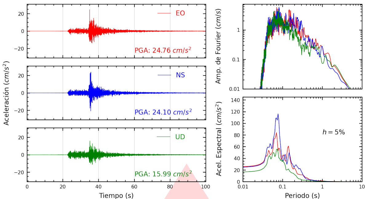
Figura A.1: Registros tiempo-historia, espectros de Fourier y de respuesta en las direcciones EO, NS y vertical de la estación ASIA. Sismo de Pisco, Pisco - Ica del 2025-07-08, 06:40:05 (Hora local)
