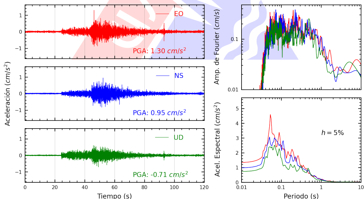
Figura A.36: Registros tiempo-historia, espectros de Fourier y de respuesta en las direcciones EO, NS y vertical de la estación INICT. Sismo de Pisco, Pisco - Ica del 2025-07-08, 06:40:05 (Hora local)
