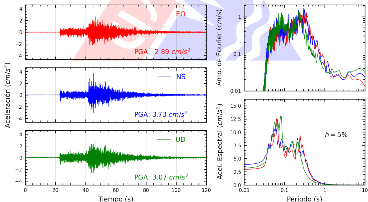
Figura A.8: Registros tiempo-historia, espectros de Fourier y de respuesta en las direcciones EO, NS y vertical de la estación SOVES. Sismo de Pisco, Pisco - Ica del 2025-07-08, 06:40:05 (Hora local)
