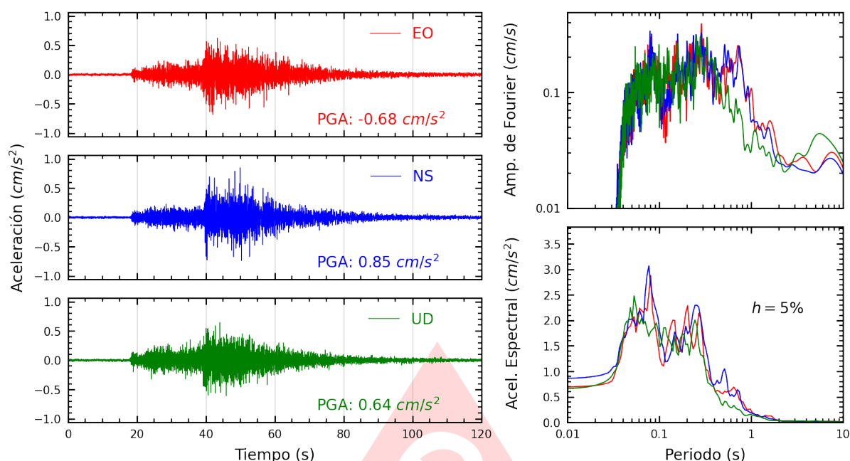
Figura A.45: Registros tiempo-historia, espectros de Fourier y de respuesta en las direcciones EO, NS y vertical de la estación UNMSM. Sismo de Pisco, Pisco - Ica del 2025-07-08, 06:40:05 (Hora local)
