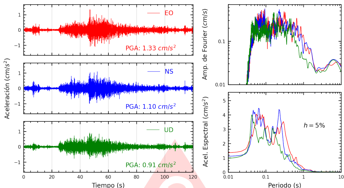
Figura A.35: Registros tiempo-historia, espectros de Fourier y de respuesta en las direcciones EO, NS y vertical de la estación UPCSM. Sismo de Pisco, Pisco - Ica del 2025-07-08, 06:40:05 (Hora local)
