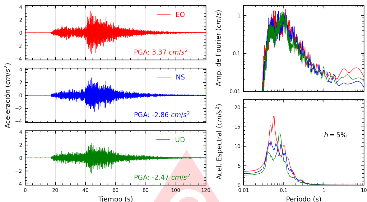
Figura A.9: Registros tiempo-historia, espectros de Fourier y de respuesta en las direcciones EO, NS y vertical de la estación AMORE. Sismo de Pisco, Pisco - Ica del 2025-07-08, 06:40:05 (Hora local)
