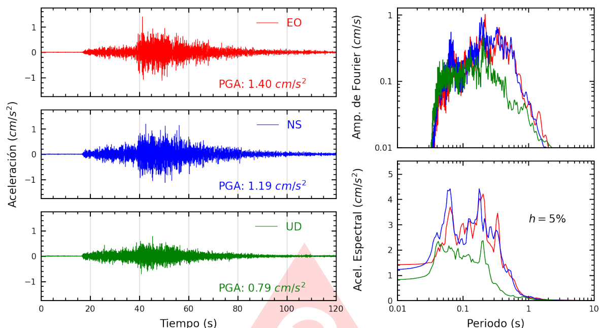
Figura A.31: Registros tiempo-historia, espectros de Fourier y de respuesta en las direcciones EO, NS y vertical de la estación VHAYA. Sismo de Pisco, Pisco - Ica del 2025-07-08, 06:40:05 (Hora local)
