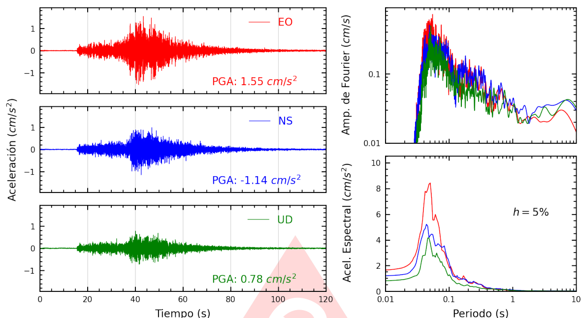
Figura A.27: Registros tiempo-historia, espectros de Fourier y de respuesta en las direcciones EO, NS y vertical de la estación UCSS. Sismo de Pisco, Pisco - Ica del 2025-07-08, 06:40:05 (Hora local)
