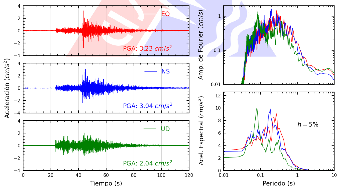
Figura A.10: Registros tiempo-historia, espectros de Fourier y de respuesta en las direcciones EO, NS y vertical de la estación SOCHO. Sismo de Pisco, Pisco - Ica del 2025-07-08, 06:40:05 (Hora local)
