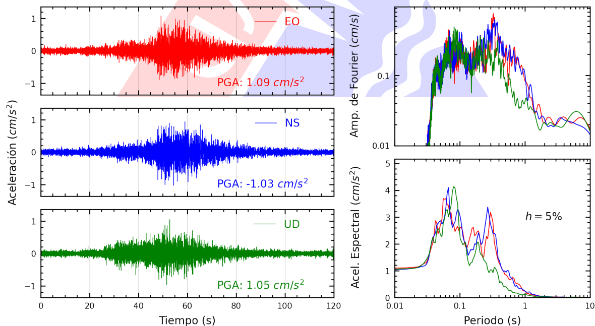
Figura A.42: Registros tiempo-historia, espectros de Fourier y de respuesta en las direcciones EO, NS y vertical de la estación MADRE. Sismo de Pisco, Pisco - Ica del 2025-07-08, 06:40:05 (Hora local)
