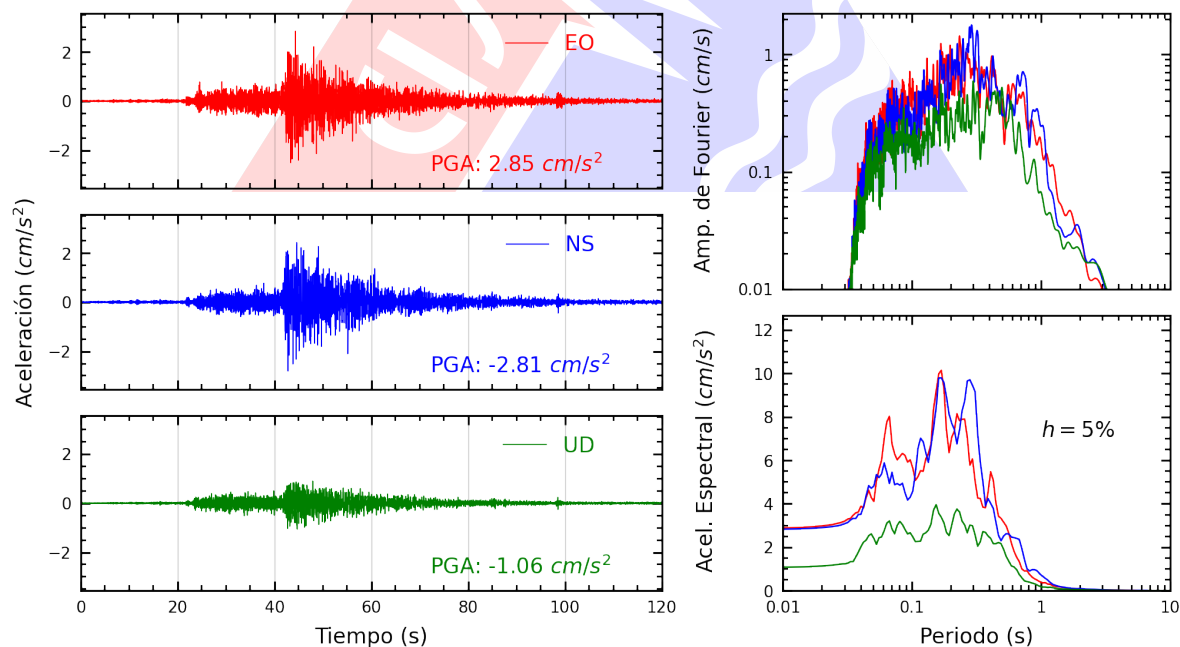
Figura A.14: Registros tiempo-historia, espectros de Fourier y de respuesta en las direcciones EO, NS y vertical de la estación BRIS2. Sismo de Pisco, Pisco - Ica del 2025-07-08, 06:40:05 (Hora local)
