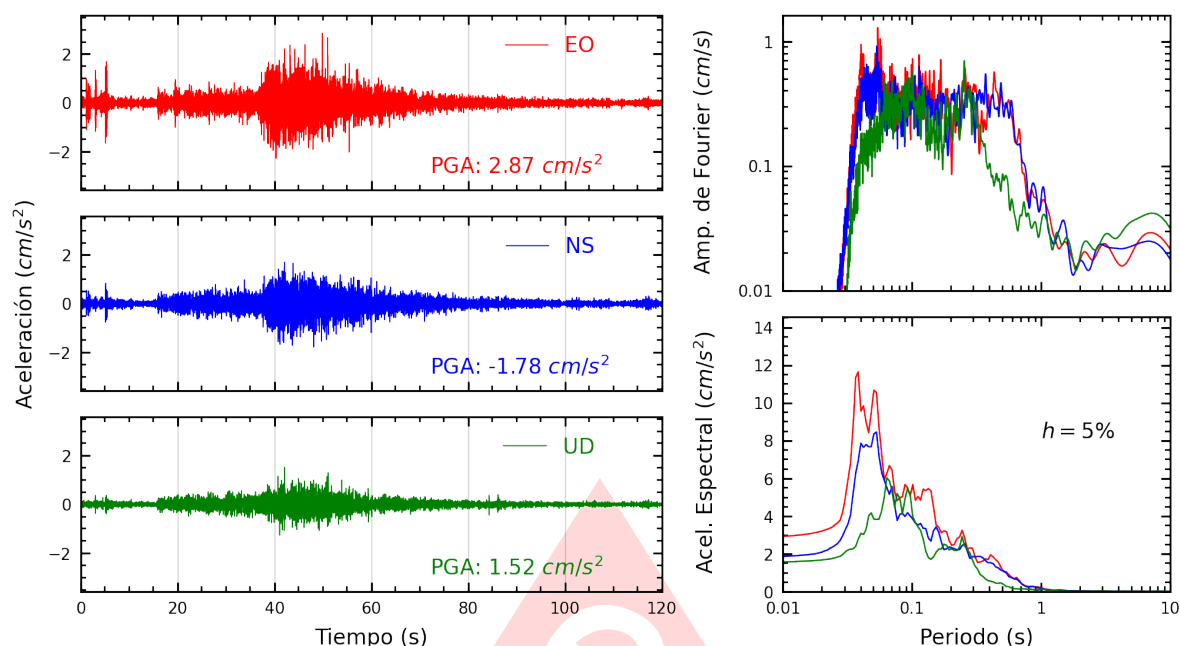
Figura A.13: Registros tiempo-historia, espectros de Fourier y de respuesta en las direcciones EO, NS y vertical de la estación OLIVO. Sismo de Pisco, Pisco - Ica del 2025-07-08, 06:40:05 (Hora local)
