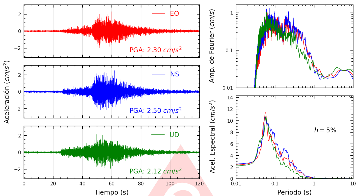
Figura A.19: Registros tiempo-historia, espectros de Fourier y de respuesta en las direcciones EO, NS y vertical de la estación SJLSC. Sismo de Pisco, Pisco - Ica del 2025-07-08, 06:40:05 (Hora local)
