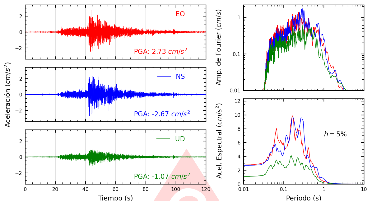
Figura A.15: Registros tiempo-historia, espectros de Fourier y de respuesta en las direcciones EO, NS y vertical de la estación BRISA. Sismo de Pisco, Pisco - Ica del 2025-07-08, 06:40:05 (Hora local)
