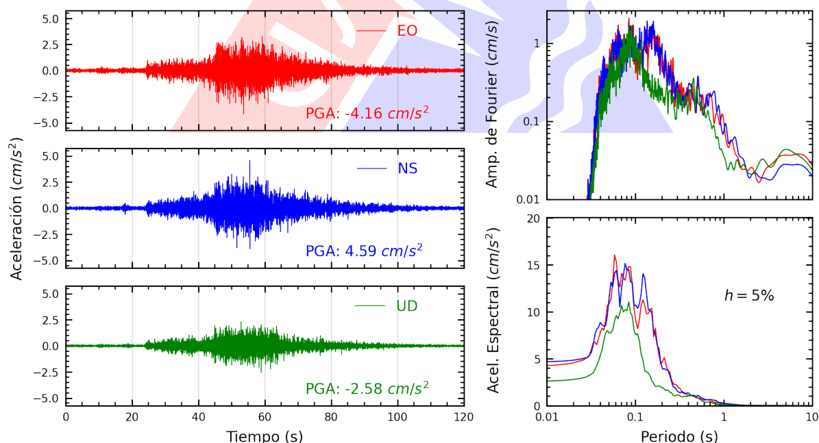
Figura A.6: Registros tiempo-historia, espectros de Fourier y de respuesta en las direcciones EO, NS y vertical de la estación USILM. Sismo de Pisco, Pisco - Ica del 2025-07-08, 06:40:05 (Hora local)
