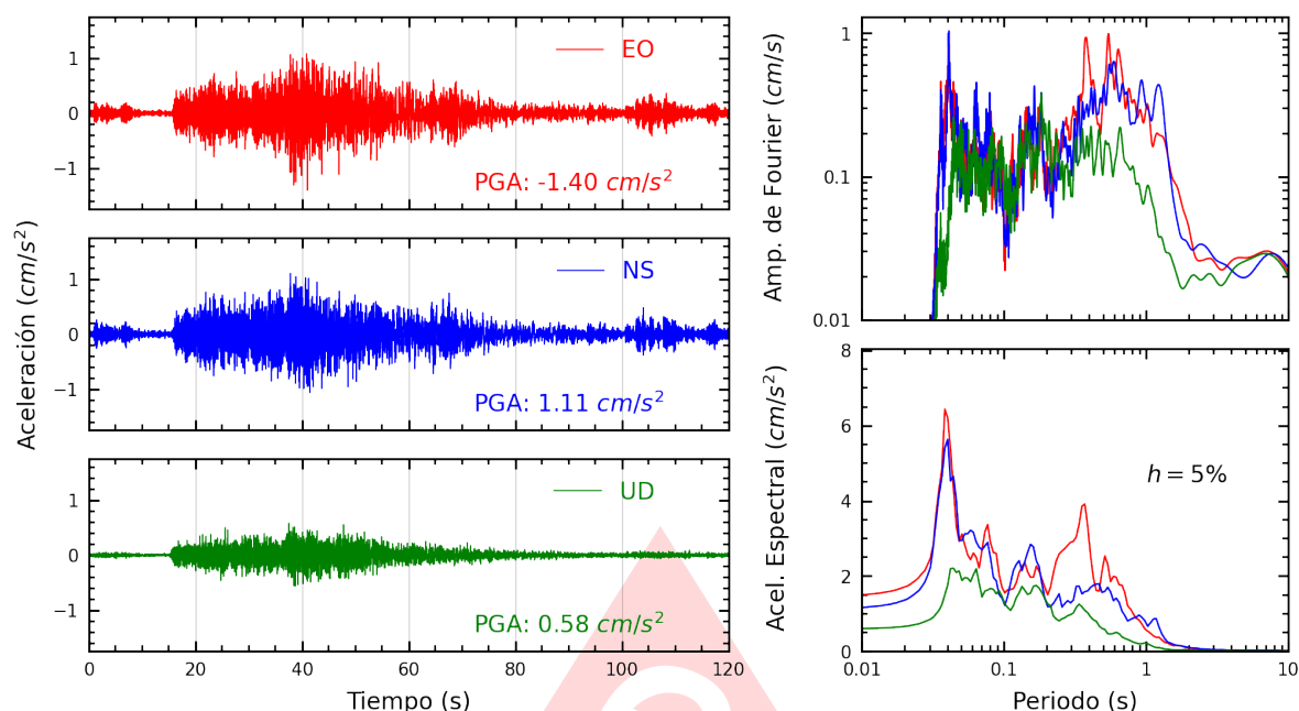
Figura A.33: Registros tiempo-historia, espectros de Fourier y de respuesta en las direcciones EO, NS y vertical de la estación DHNPE. Sismo de Pisco, Pisco - Ica del 2025-07-08, 06:40:05 (Hora local)
