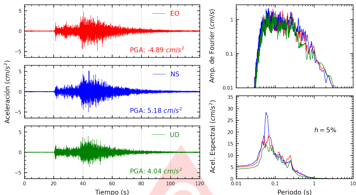
Figura A.5: Registros tiempo-historia, espectros de Fourier y de respuesta en las direcciones EO, NS y vertical de la estación PHERM. Sismo de Pisco, Pisco - Ica del 2025-07-08, 06:40:05 (Hora local)
