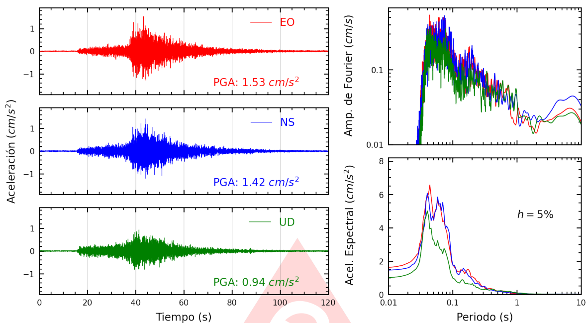
Figura A.29: Registros tiempo-historia, espectros de Fourier y de respuesta en las direcciones EO, NS y vertical de la estación SJLCE. Sismo de Pisco, Pisco - Ica del 2025-07-08, 06:40:05 (Hora local)
