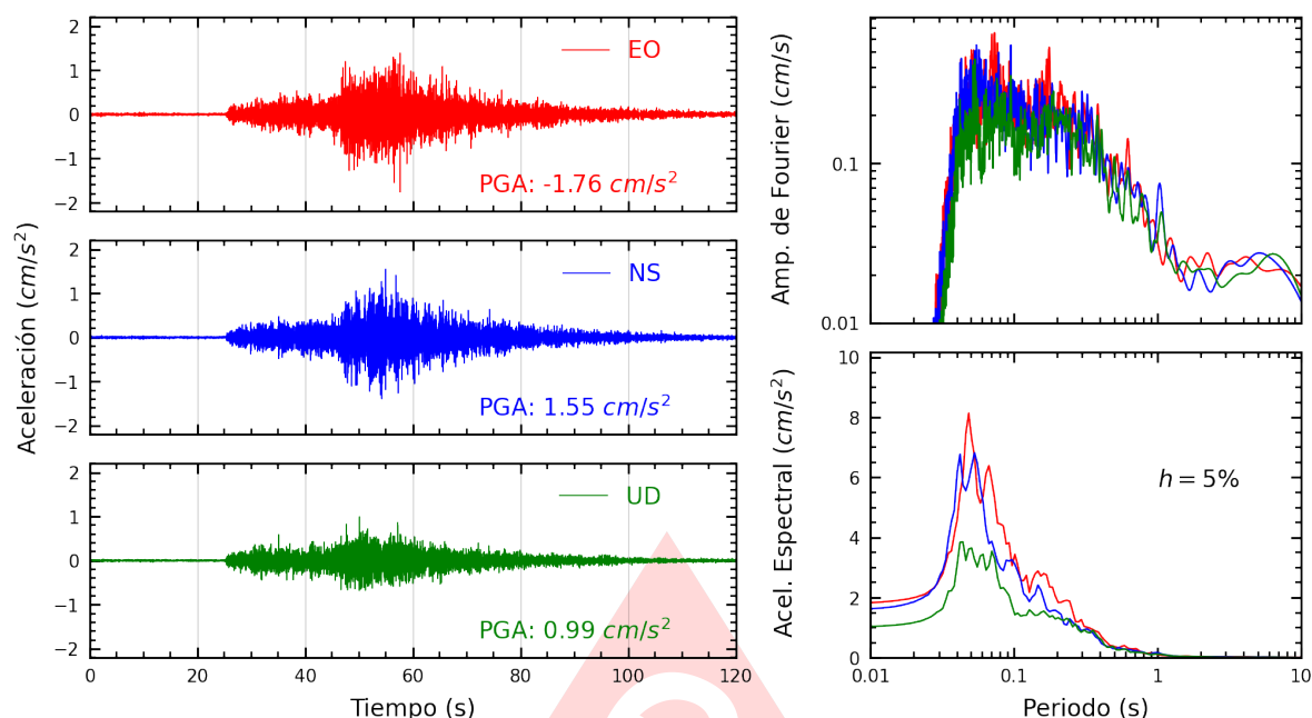
Figura A.25: Registros tiempo-historia, espectros de Fourier y de respuesta en las direcciones EO, NS y vertical de la estación FICPE. Sismo de Pisco, Pisco - Ica del 2025-07-08, 06:40:05 (Hora local)
