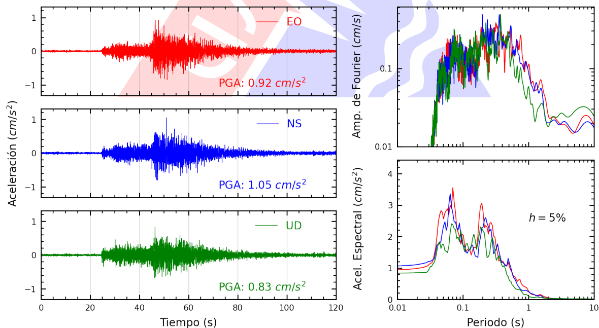
Figura A.44: Registros tiempo-historia, espectros de Fourier y de respuesta en las direcciones EO, NS y vertical de la estación UNFV. Sismo de Pisco, Pisco - Ica del 2025-07-08, 06:40:05 (Hora local)
