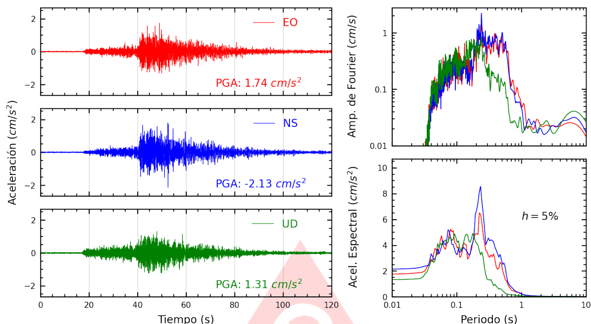
Figura A.21: Registros tiempo-historia, espectros de Fourier y de respuesta en las direcciones EO, NS y vertical de la estación MDPP. Sismo de Pisco, Pisco - Ica del 2025-07-08, 06:40:05 (Hora local)
