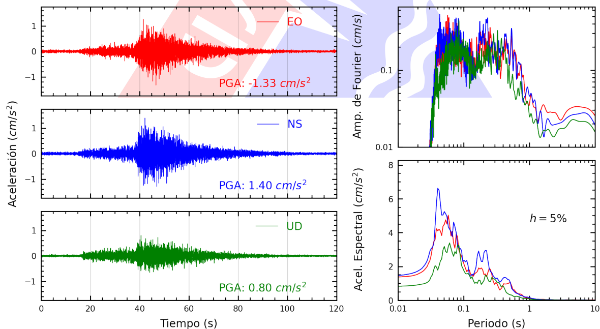
Figura A.32: Registros tiempo-historia, espectros de Fourier y de respuesta en las direcciones EO, NS y vertical de la estación COMAS. Sismo de Pisco, Pisco - Ica del 2025-07-08, 06:40:05 (Hora local)
