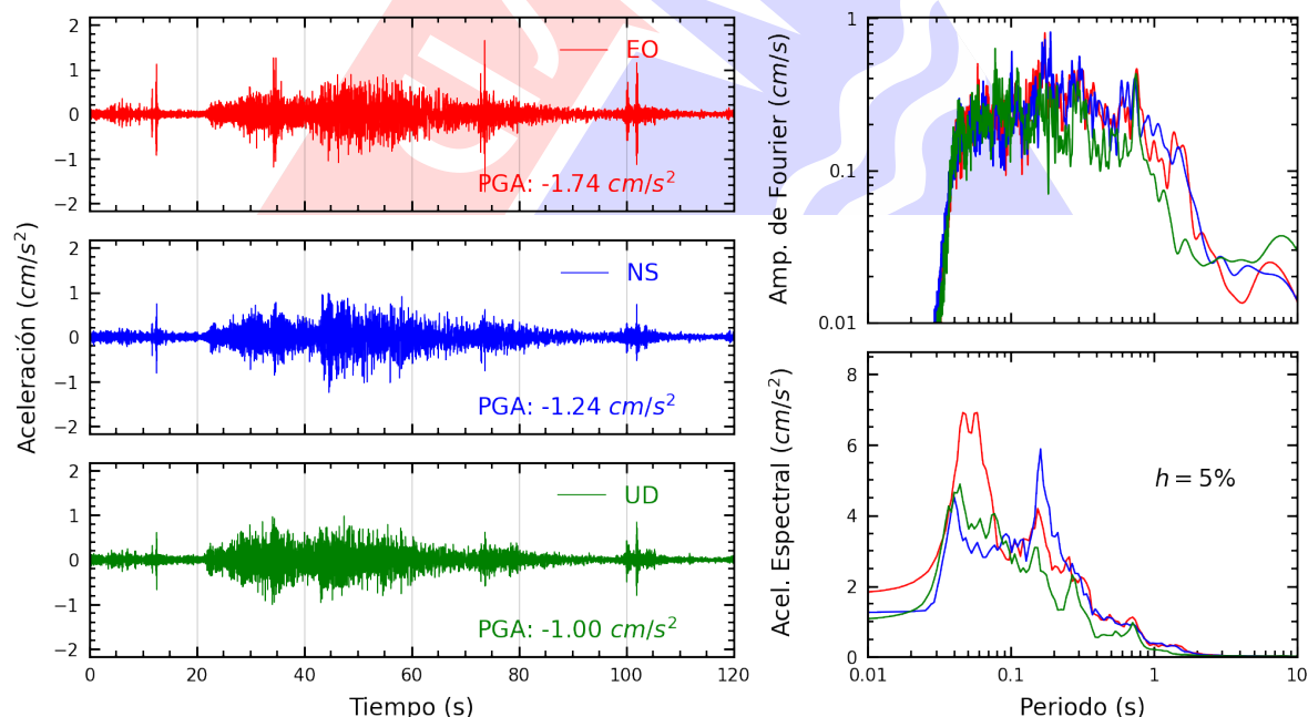
Figura A.26: Registros tiempo-historia, espectros de Fourier y de respuesta en las direcciones EO, NS y vertical de la estación PRADO. Sismo de Pisco, Pisco - Ica del 2025-07-08, 06:40:05 (Hora local)
