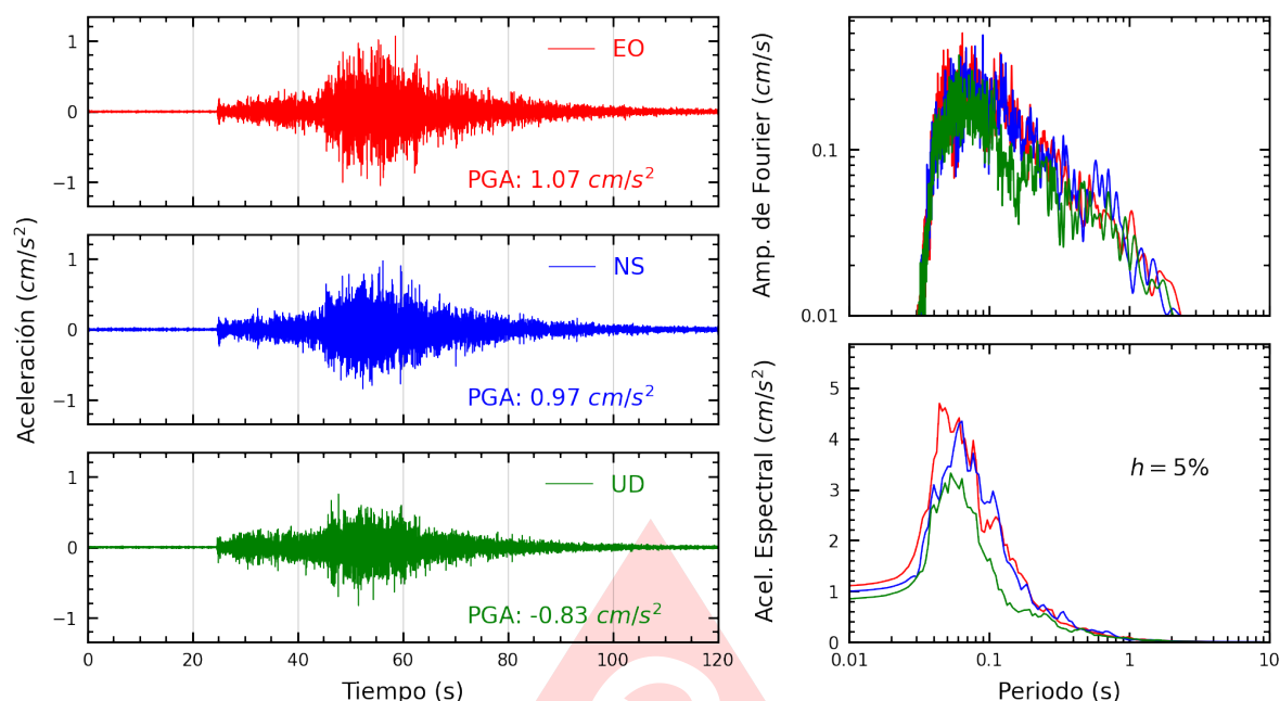
Figura A.43: Registros tiempo-historia, espectros de Fourier y de respuesta en las direcciones EO, NS y vertical de la estación ATARJ. Sismo de Pisco, Pisco - Ica del 2025-07-08, 06:40:05 (Hora local)
