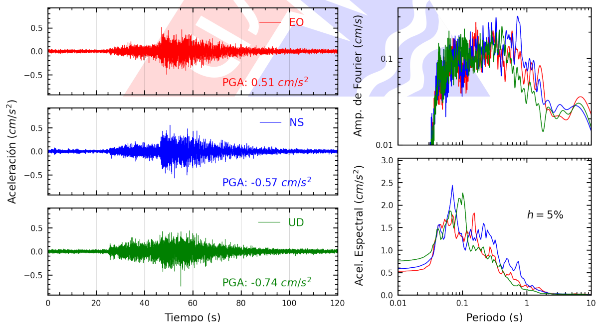
Figura A.46: Registros tiempo-historia, espectros de Fourier y de respuesta en las direcciones EO, NS y vertical de la estación BONDY. Sismo de Pisco, Pisco - Ica del 2025-07-08, 06:40:05 (Hora local)
