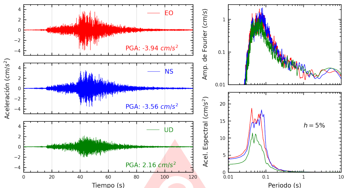
Figura A.7: Registros tiempo-historia, espectros de Fourier y de respuesta en las direcciones EO, NS y vertical de la estación JOSEO. Sismo de Pisco, Pisco - Ica del 2025-07-08, 06:40:05 (Hora local)
