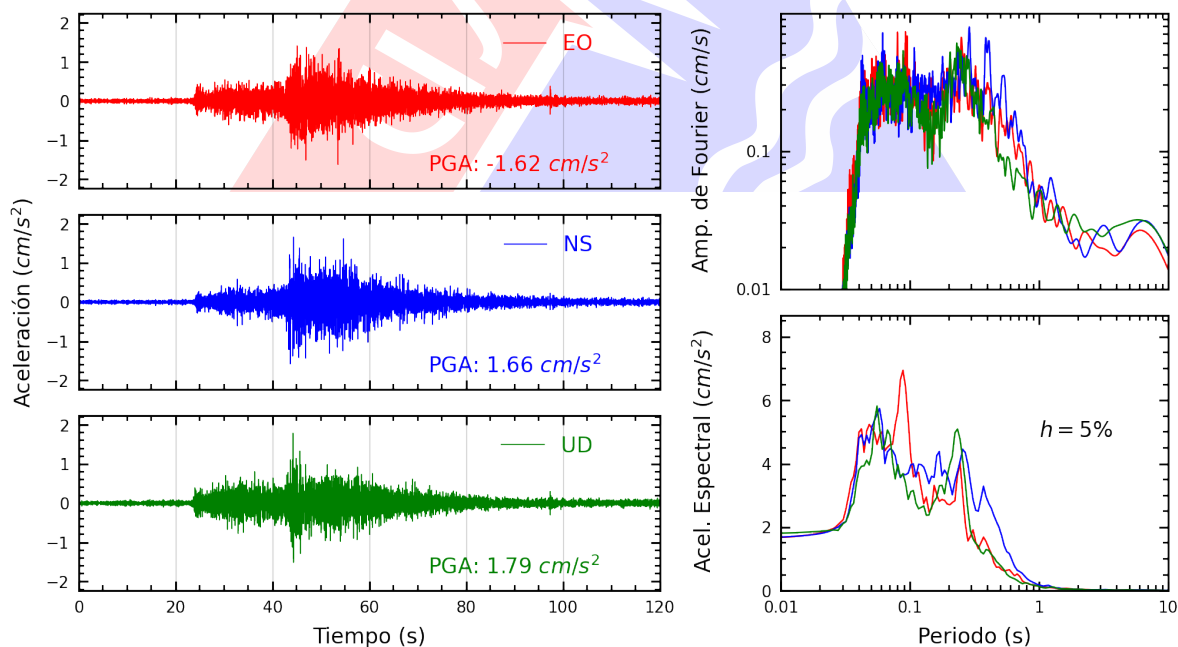
Figura A.24: Registros tiempo-historia, espectros de Fourier y de respuesta en las direcciones EO, NS y vertical de la estación URPPE. Sismo de Pisco, Pisco - Ica del 2025-07-08, 06:40:05 (Hora local)
