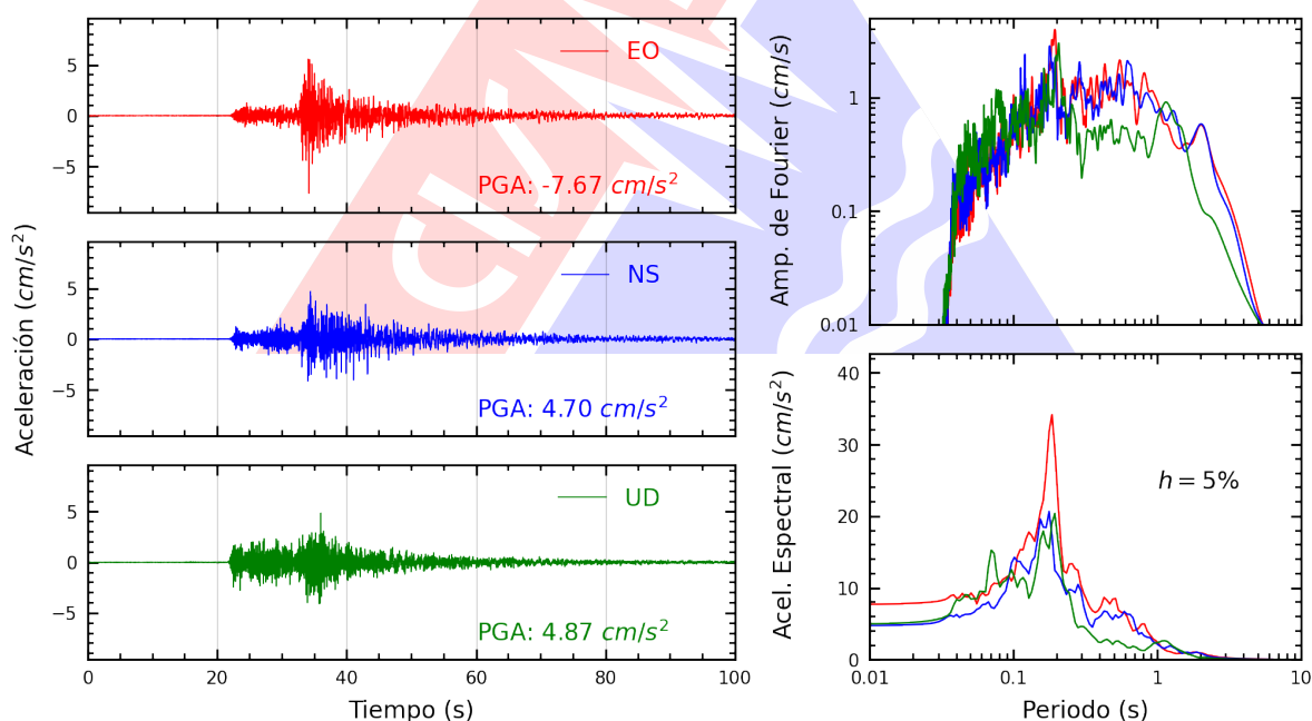
Figura A.2: Registros tiempo-historia, espectros de Fourier y de respuesta en las direcciones EO, NS y vertical de la estación UNICA. Sismo de Pisco, Pisco - Ica del 2025-07-08, 06:40:05 (Hora local)
