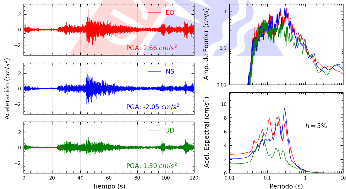
Figura A.16: Registros tiempo-historia, espectros de Fourier y de respuesta en las direcciones EO, NS y vertical de la estación SOBAR. Sismo de Pisco, Pisco - Ica del 2025-07-08, 06:40:05 (Hora local)
