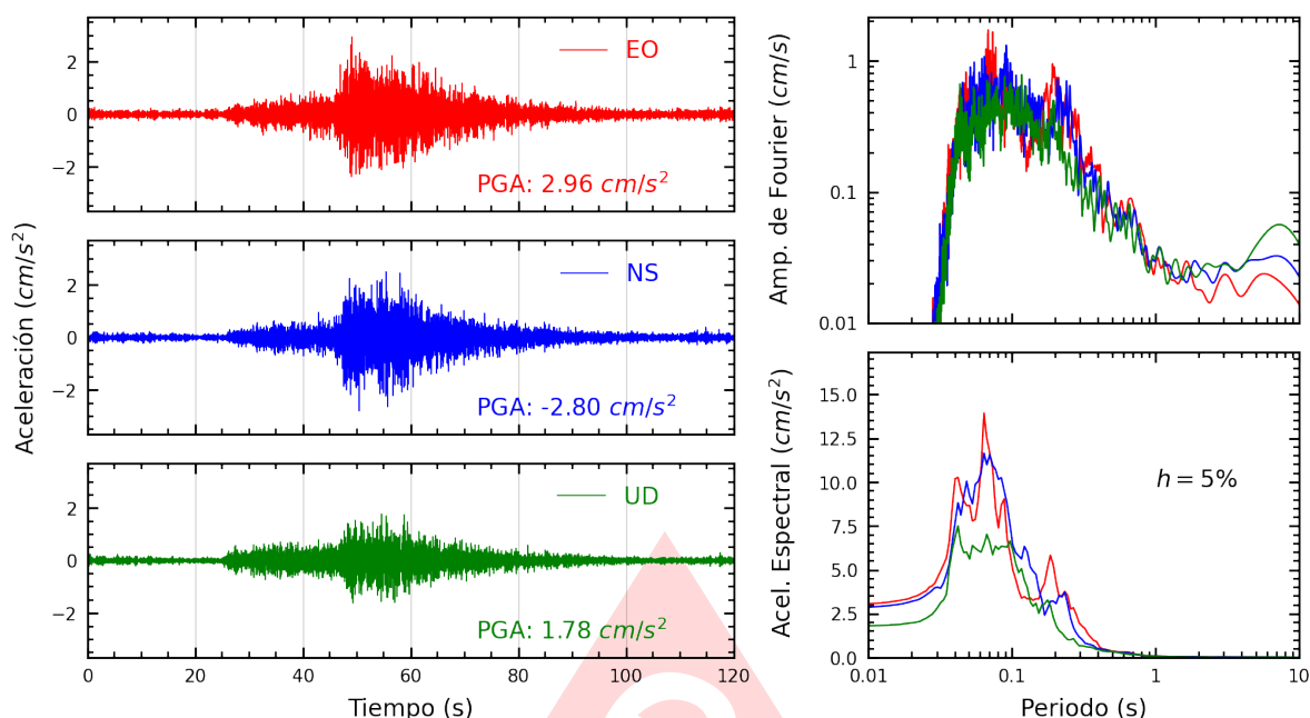
Figura A.11: Registros tiempo-historia, espectros de Fourier y de respuesta en las direcciones EO, NS y vertical de la estación INDEP. Sismo de Pisco, Pisco - Ica del 2025-07-08, 06:40:05 (Hora local)
