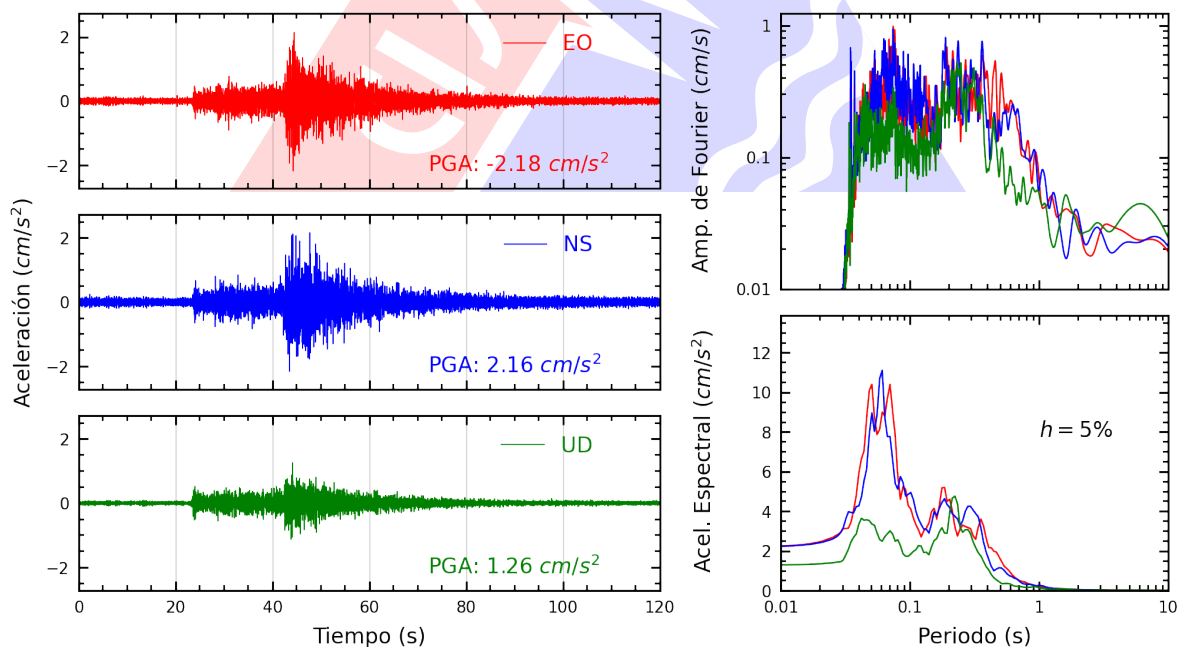
Figura A.20: Registros tiempo-historia, espectros de Fourier y de respuesta en las direcciones EO, NS y vertical de la estación UPCVI. Sismo de Pisco, Pisco - Ica del 2025-07-08, 06:40:05 (Hora local)
