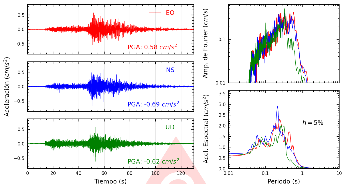
Figura A.47: Registros tiempo-historia, espectros de Fourier y de respuesta en las direcciones EO, NS y vertical de la estación CARAL. Sismo de Pisco, Pisco - Ica del 2025-07-08, 06:40:05 (Hora local)
