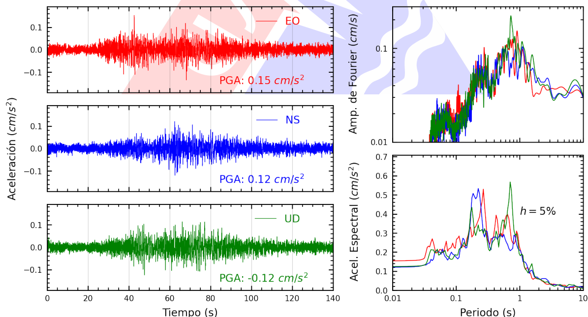
Figura A.48: Registros tiempo-historia, espectros de Fourier y de respuesta en las direcciones EO, NS y vertical de la estación UNSCH. Sismo de Pisco, Pisco - Ica del 2025-07-08, 06:40:05 (Hora local)
