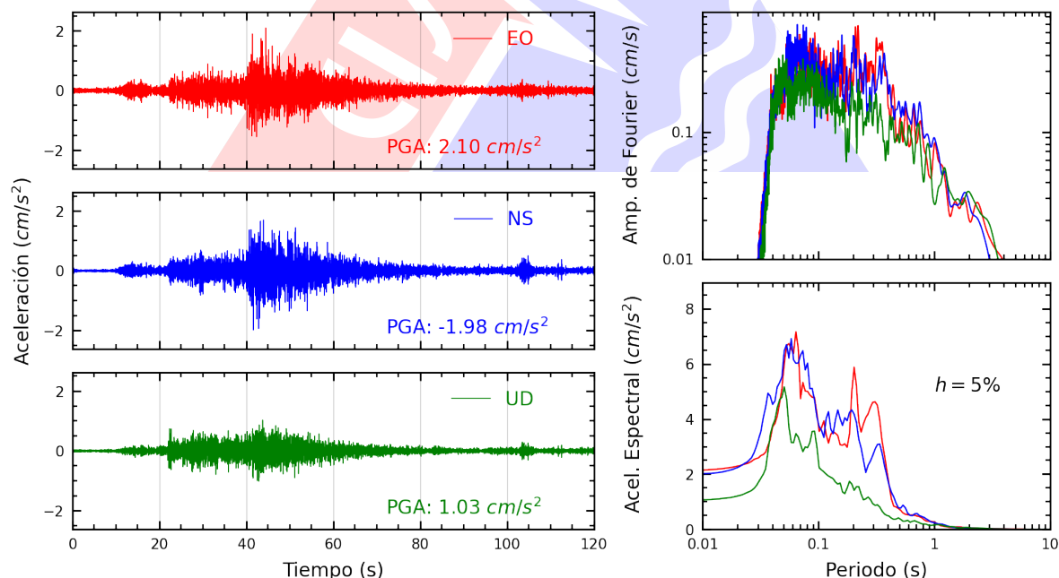
Figura A.22: Registros tiempo-historia, espectros de Fourier y de respuesta en las direcciones EO, NS y vertical de la estación PACHA. Sismo de Pisco, Pisco - Ica del 2025-07-08, 06:40:05 (Hora local)
