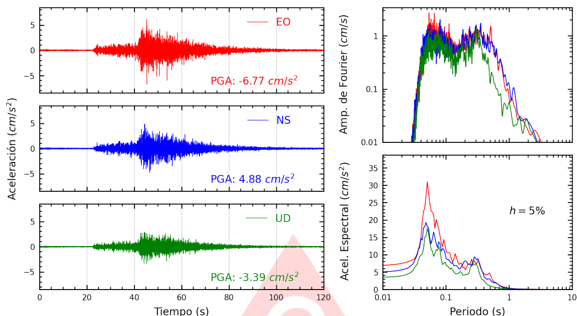
Figura A.3: Registros tiempo-historia, espectros de Fourier y de respuesta en las direcciones EO, NS y vertical de la estación UNTEL. Sismo de Pisco, Pisco - Ica del 2025-07-08, 06:40:05 (Hora local)
