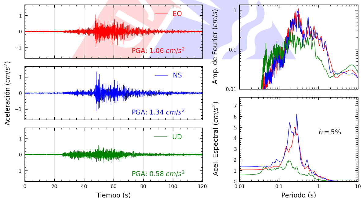
Figura A.34: Registros tiempo-historia, espectros de Fourier y de respuesta en las direcciones EO, NS y vertical de la estación DSMI. Sismo de Pisco, Pisco - Ica del 2025-07-08, 06:40:05 (Hora local)
