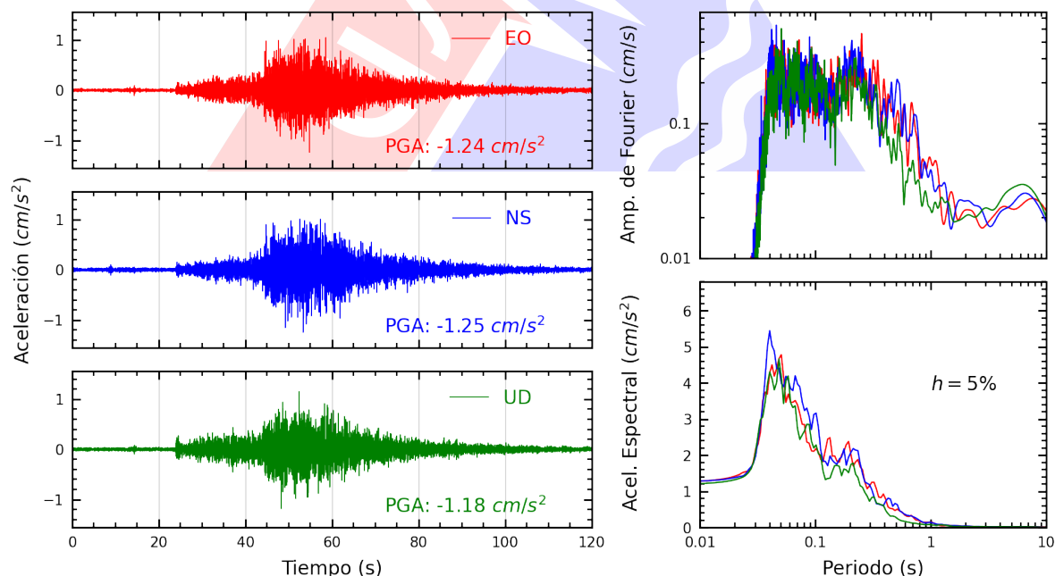
Figura A.38: Registros tiempo-historia, espectros de Fourier y de respuesta en las direcciones EO, NS y vertical de la estación USMP. Sismo de Pisco, Pisco - Ica del 2025-07-08, 06:40:05 (Hora local)
