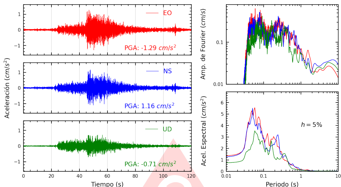
Figura A.37: Registros tiempo-historia, espectros de Fourier y de respuesta en las direcciones EO, NS y vertical de la estación CEPRE. Sismo de Pisco, Pisco - Ica del 2025-07-08, 06:40:05 (Hora local)
