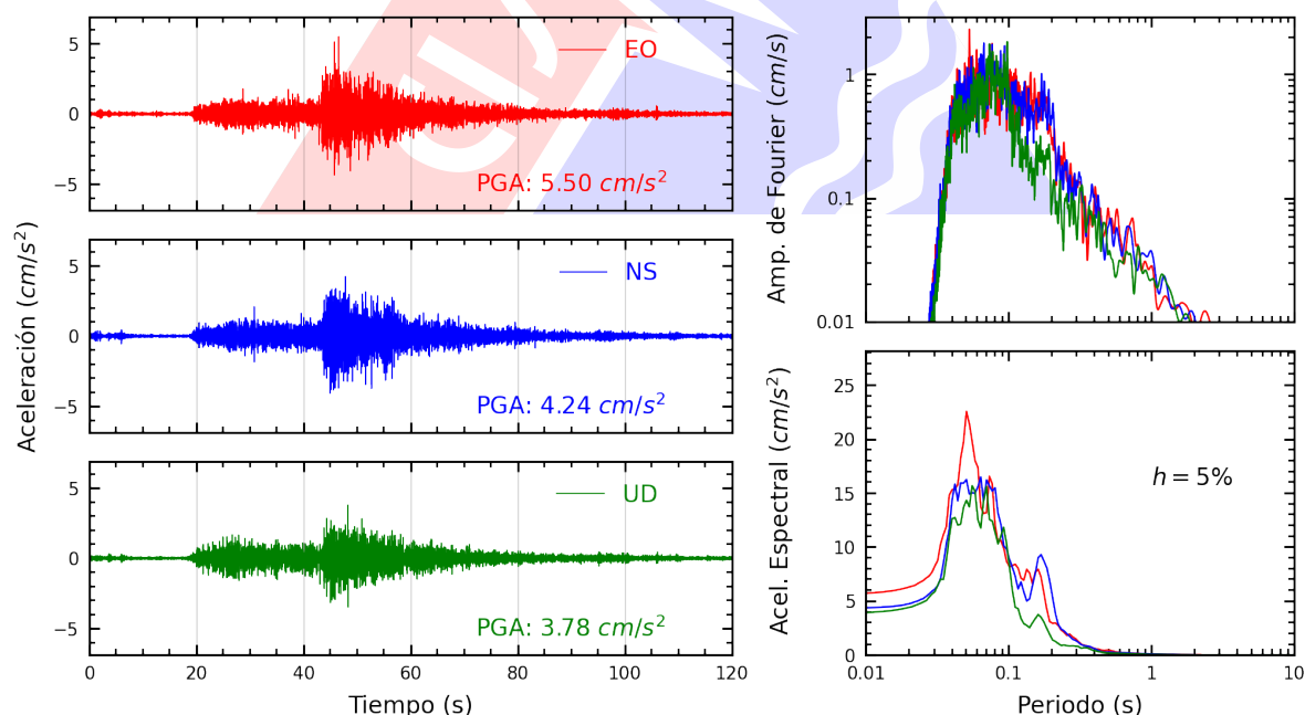
Figura A.4: Registros tiempo-historia, espectros de Fourier y de respuesta en las direcciones EO, NS y vertical de la estación SROSA. Sismo de Pisco, Pisco - Ica del 2025-07-08, 06:40:05 (Hora local)
