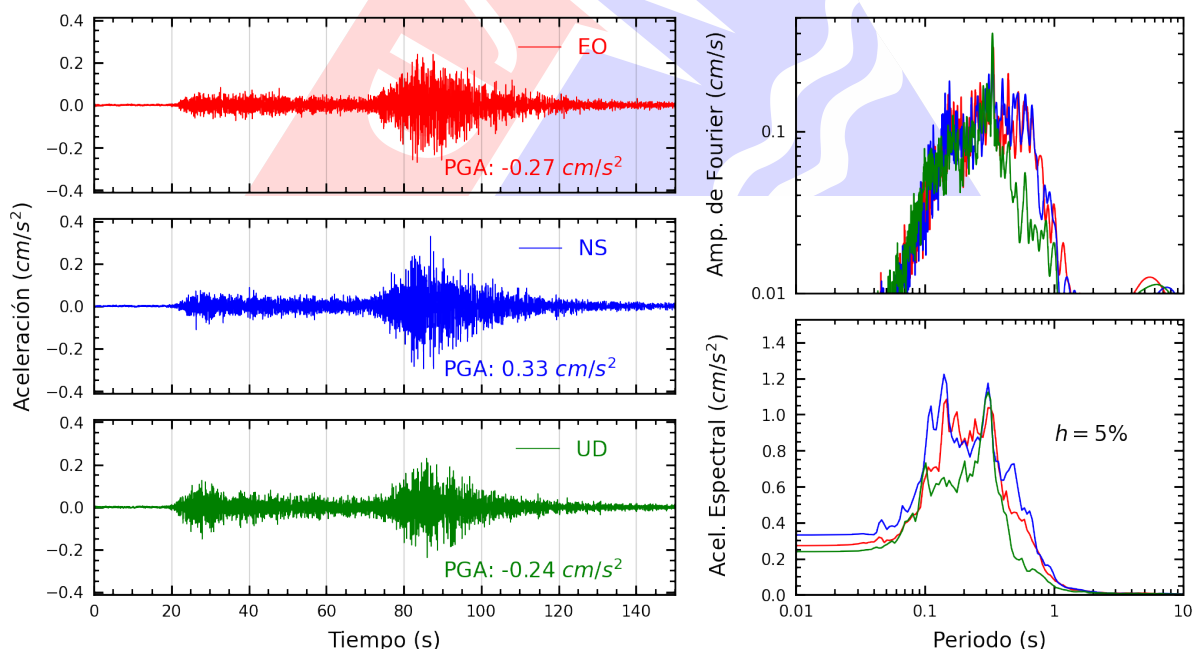
Figura A.30: Registros tiempo-historia, espectros de Fourier y de respuesta en las direcciones EO, NS y vertical de la estación CARAL. Sismo de Palpa, Palpa - Ica del 2025-07-08, 16:32:53 (Hora local)
