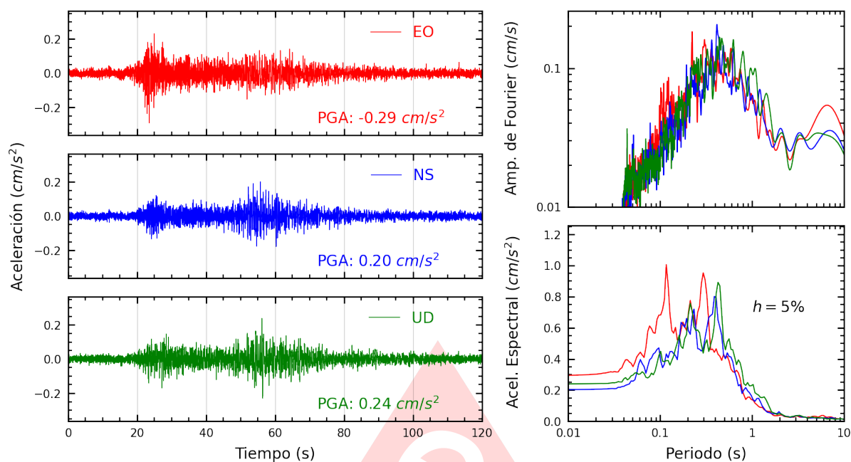
Figura A.33: Registros tiempo-historia, espectros de Fourier y de respuesta en las direcciones EO, NS y vertical de la estación UNSCH. Sismo de Palpa, Palpa - Ica del 2025-07-08, 16:32:53 (Hora local)
