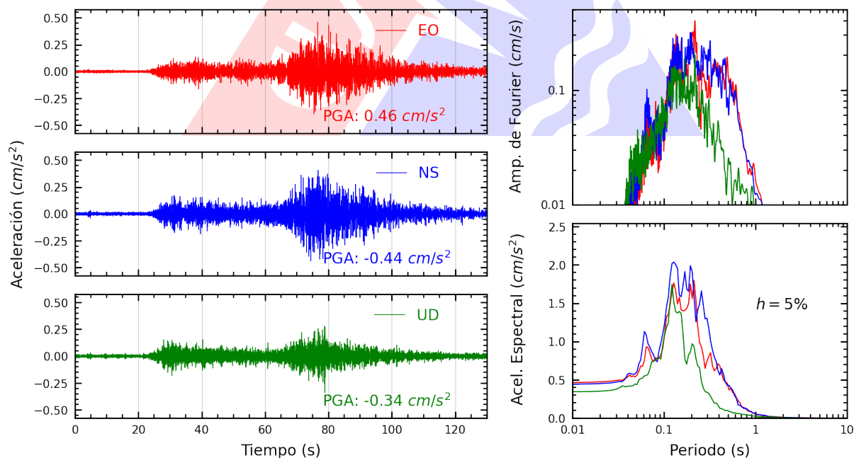
Figura A.24: Registros tiempo-historia, espectros de Fourier y de respuesta en las direcciones EO, NS y vertical de la estación VHAYA. Sismo de Palpa, Palpa - Ica del 2025-07-08, 16:32:53 (Hora local)
