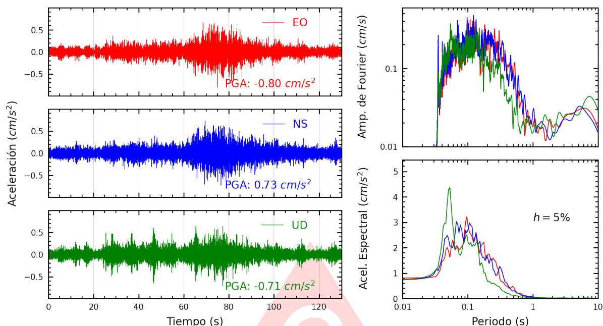
Figura A.15: Registros tiempo-historia, espectros de Fourier y de respuesta en las direcciones EO, NS y vertical de la estación SJLSC. Sismo de Palpa, Palpa - Ica del 2025-07-08, 16:32:53 (Hora local)
