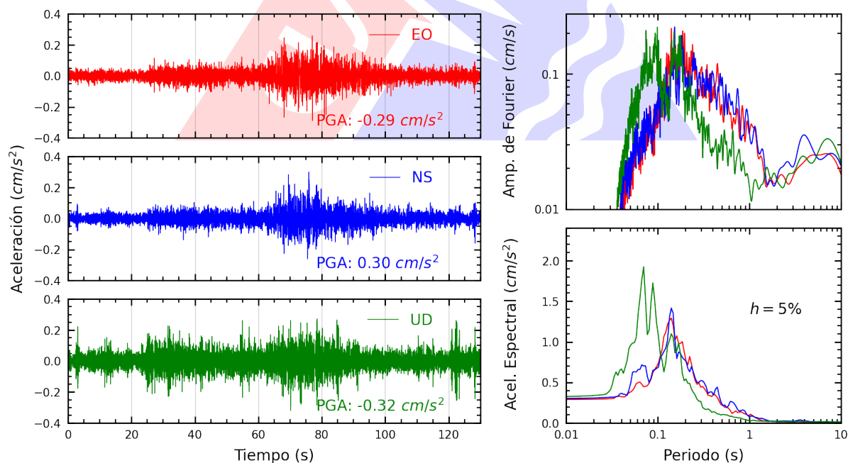
Figura A.32: Registros tiempo-historia, espectros de Fourier y de respuesta en las direcciones EO, NS y vertical de la estación RAMON. Sismo de Palpa, Palpa - Ica del 2025-07-08, 16:32:53 (Hora local)
