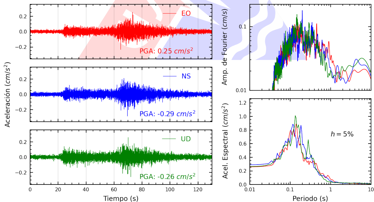
Figura A.34: Registros tiempo-historia, espectros de Fourier y de respuesta en las direcciones EO, NS y vertical de la estación UNFV. Sismo de Palpa, Palpa - Ica del 2025-07-08, 16:32:53 (Hora local)
