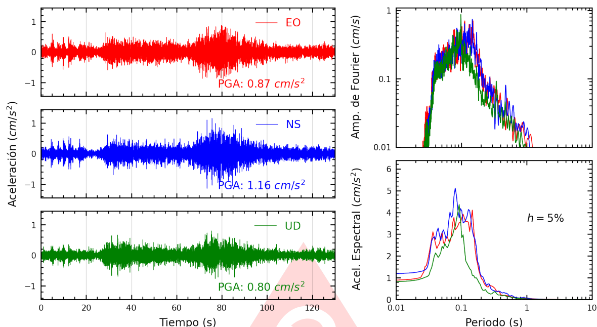
Figura A.7: Registros tiempo-historia, espectros de Fourier y de respuesta en las direcciones EO, NS y vertical de la estación SROSA. Sismo de Palpa, Palpa - Ica del 2025-07-08, 16:32:53 (Hora local)
