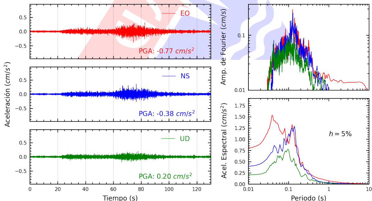
Figura A.16: Registros tiempo-historia, espectros de Fourier y de respuesta en las direcciones EO, NS y vertical de la estación ATARJ. Sismo de Palpa, Palpa - Ica del 2025-07-08, 16:32:53 (Hora local)
