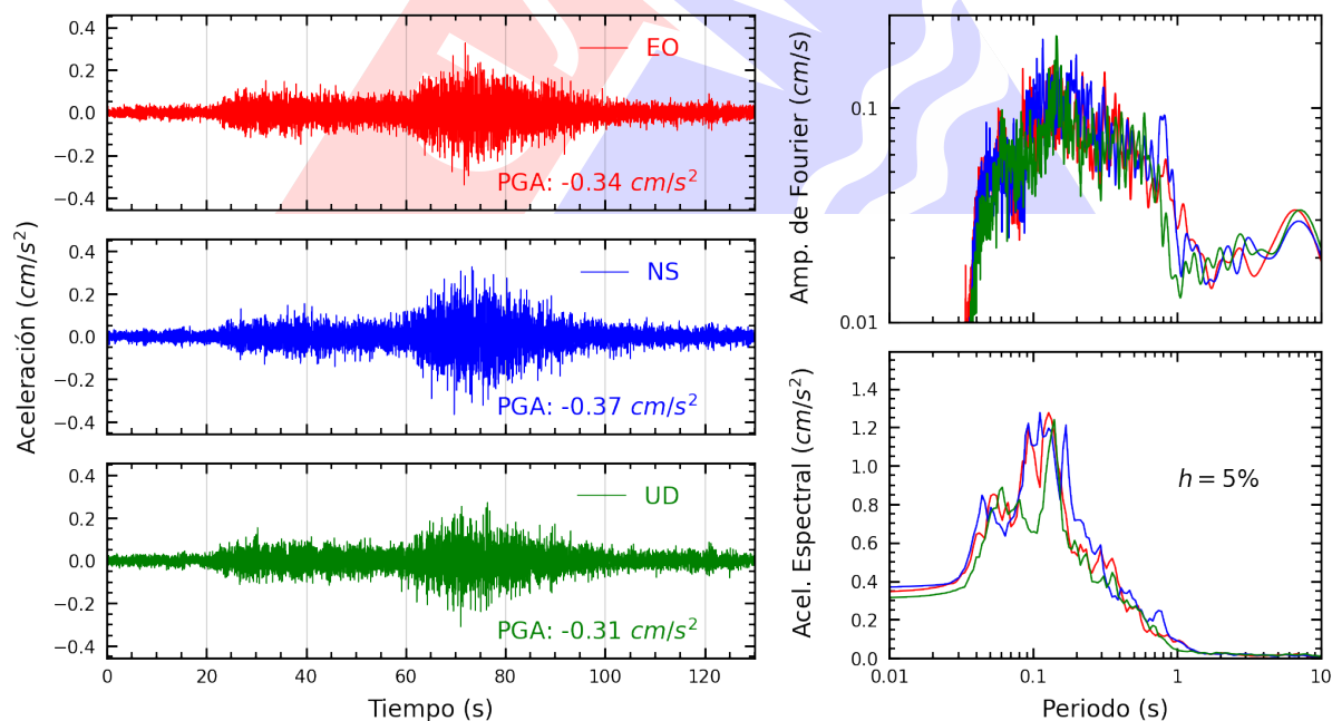
Figura A.28: Registros tiempo-historia, espectros de Fourier y de respuesta en las direcciones EO, NS y vertical de la estación IMCA. Sismo de Palpa, Palpa - Ica del 2025-07-08, 16:32:53 (Hora local)
