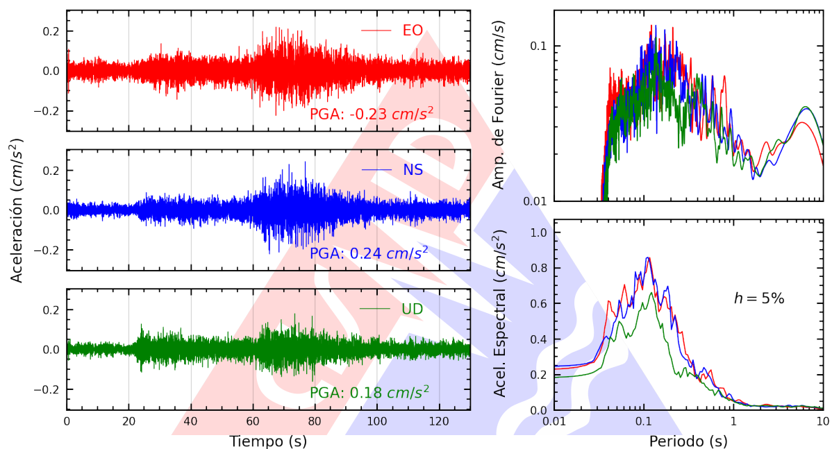
Figura A.39: Registros tiempo-historia, espectros de Fourier y de respuesta en las direcciones EO, NS y vertical de la estación INICT. Sismo de Palpa, Palpa - Ica del 2025-07-08, 16:32:53 (Hora local)
