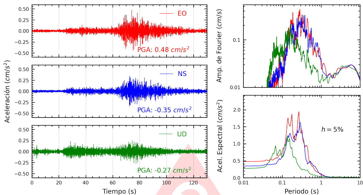
Figura A.21: Registros tiempo-historia, espectros de Fourier y de respuesta en las direcciones EO, NS y vertical de la estación ACAPU. Sismo de Palpa, Palpa - Ica del 2025-07-08, 16:32:53 (Hora local)
