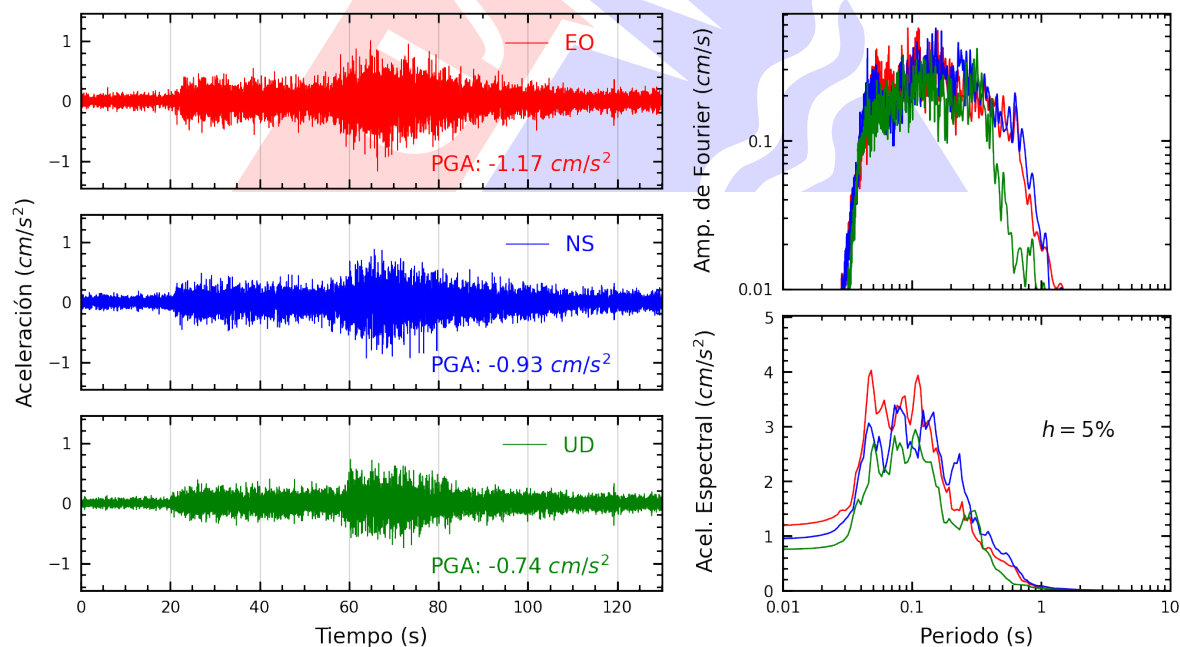
Figura A.6: Registros tiempo-historia, espectros de Fourier y de respuesta en las direcciones EO, NS y vertical de la estación UNTEL. Sismo de Palpa, Palpa - Ica del 2025-07-08, 16:32:53 (Hora local)
