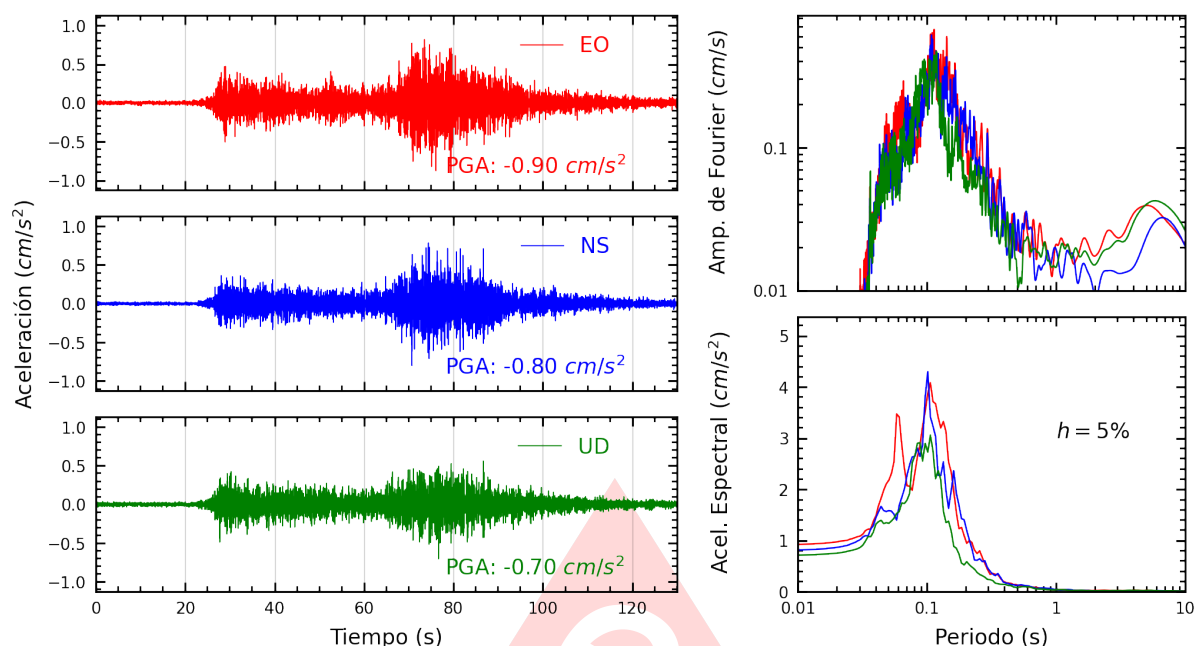
Figura A.11: Registros tiempo-historia, espectros de Fourier y de respuesta en las direcciones EO, NS y vertical de la estación AMORE. Sismo de Palpa, Palpa - Ica del 2025-07-08, 16:32:53 (Hora local)
