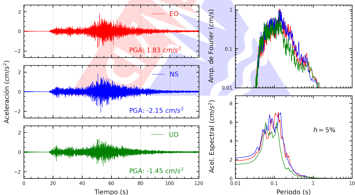
Figura A.2: Registros tiempo-historia, espectros de Fourier y de respuesta en las direcciones EO, NS y vertical de la estación ASIA. Sismo de Palpa, Palpa - Ica del 2025-07-08, 16:32:53 (Hora local)
