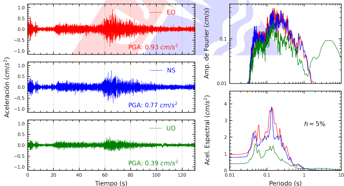
Figura A.10: Registros tiempo-historia, espectros de Fourier y de respuesta en las direcciones EO, NS y vertical de la estación BRISA. Sismo de Palpa, Palpa - Ica del 2025-07-08, 16:32:53 (Hora local)
