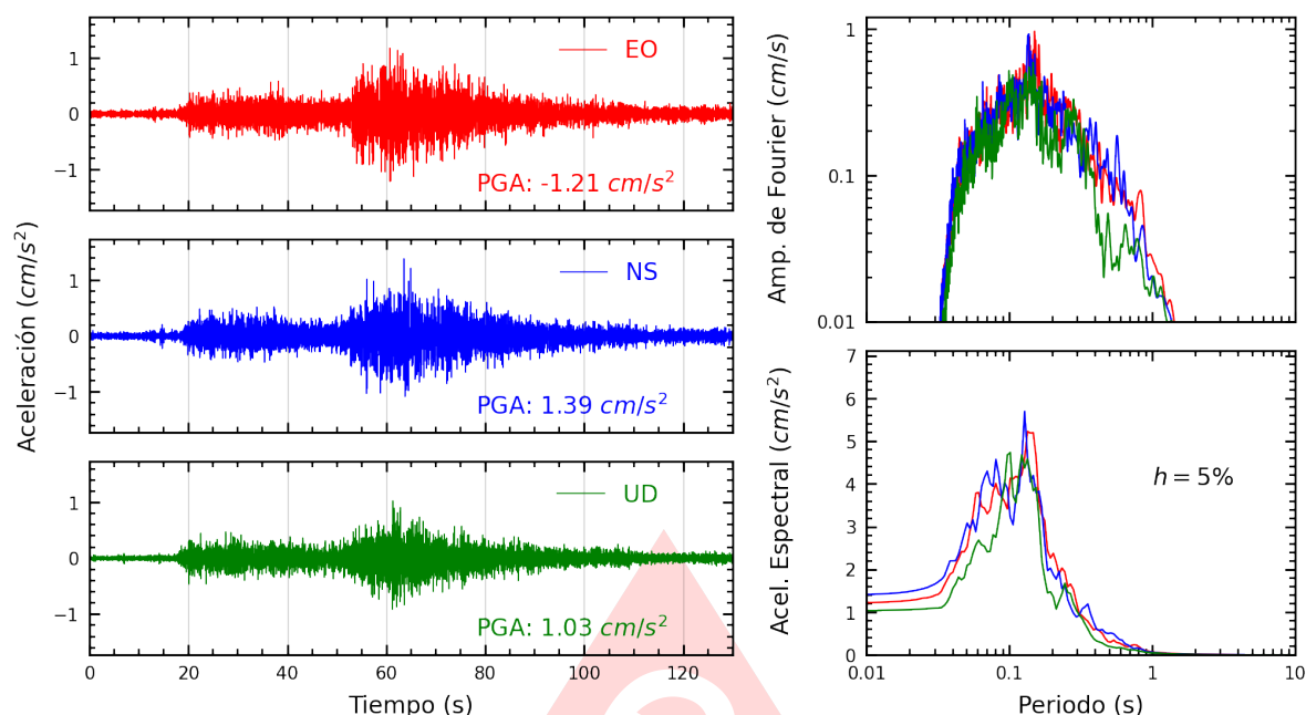
Figura A.5: Registros tiempo-historia, espectros de Fourier y de respuesta en las direcciones EO, NS y vertical de la estación PHERM. Sismo de Palpa, Palpa - Ica del 2025-07-08, 16:32:53 (Hora local)
