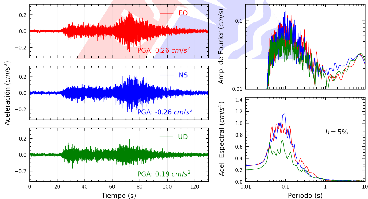
Figura A.36: Registros tiempo-historia, espectros de Fourier y de respuesta en las direcciones EO, NS y vertical de la estación SJLCE. Sismo de Palpa, Palpa - Ica del 2025-07-08, 16:32:53 (Hora local)
