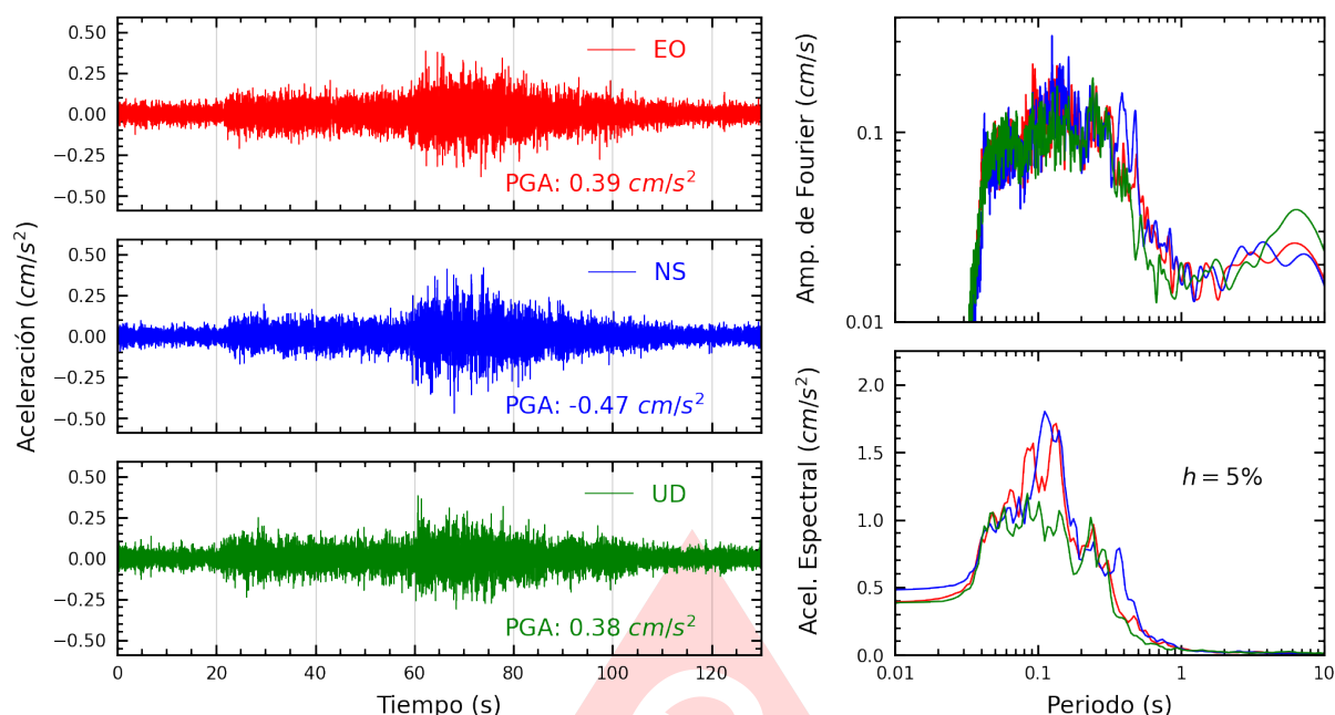
Figura A.23: Registros tiempo-historia, espectros de Fourier y de respuesta en las direcciones EO, NS y vertical de la estación URPE. Sismo de Palpa, Palpa - Ica del 2025-07-08, 16:32:53 (Hora local)
