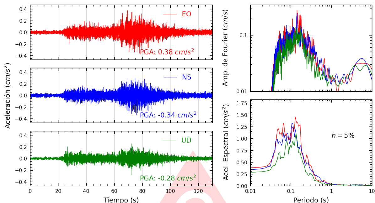
Figura A.27: Registros tiempo-historia, espectros de Fourier y de respuesta en las direcciones EO, NS y vertical de la estación FICPE. Sismo de Palpa, Palpa - Ica del 2025-07-08, 16:32:53 (Hora local)
