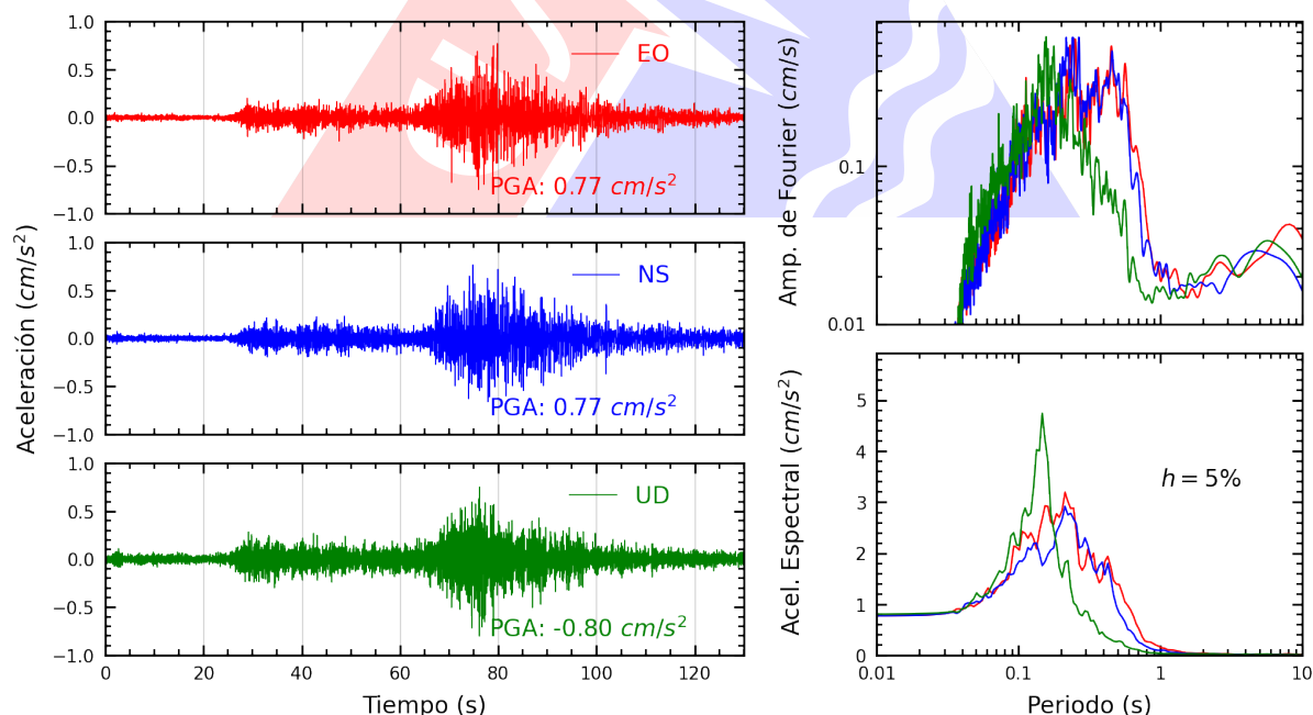
Figura A.14: Registros tiempo-historia, espectros de Fourier y de respuesta en las direcciones EO, NS y vertical de la estación MDPP. Sismo de Palpa, Palpa - Ica del 2025-07-08, 16:32:53 (Hora local)
