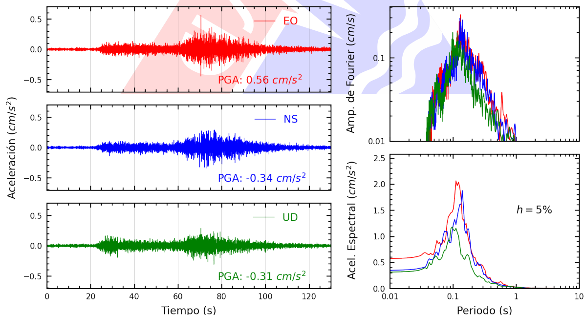
Figura A.20: Registros tiempo-historia, espectros de Fourier y de respuesta en las direcciones EO, NS y vertical de la estación JALV2. Sismo de Palpa, Palpa - Ica del 2025-07-08, 16:32:53 (Hora local)
