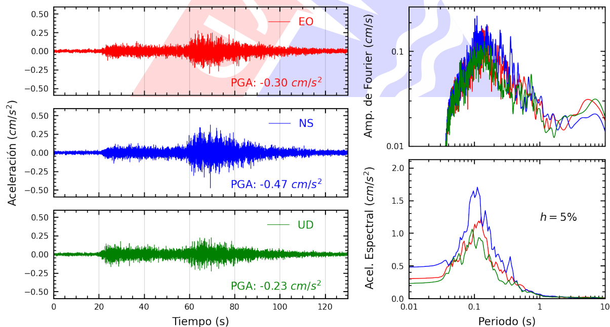
Figura A.22: Registros tiempo-historia, espectros de Fourier y de respuesta en las direcciones EO, NS y vertical de la estación SERVI. Sismo de Palpa, Palpa - Ica del 2025-07-08, 16:32:53 (Hora local)
