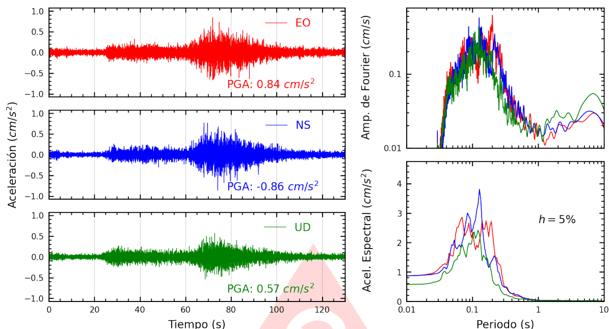
Figura A.13: Registros tiempo-historia, espectros de Fourier y de respuesta en las direcciones EO, NS y vertical de la estación INDEP. Sismo de Palpa, Palpa - Ica del 2025-07-08, 16:32:53 (Hora local)
