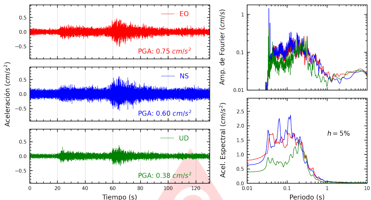
Figura A.17: Registros tiempo-historia, espectros de Fourier y de respuesta en las direcciones EO, NS y vertical de la estación UPCVI. Sismo de Palpa, Palpa - Ica del 2025-07-08, 16:32:53 (Hora local)
