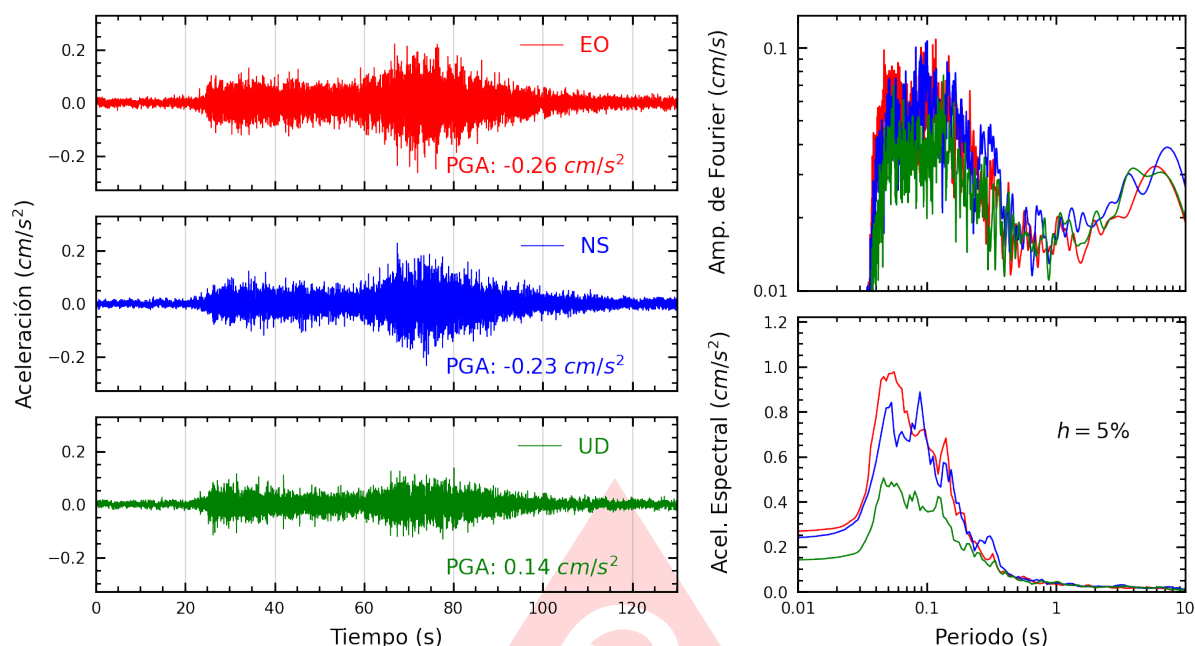
Figura A.37: Registros tiempo-historia, espectros de Fourier y de respuesta en las direcciones EO, NS y vertical de la estación UCSS. Sismo de Palpa, Palpa - Ica del 2025-07-08, 16:32:53 (Hora local)
