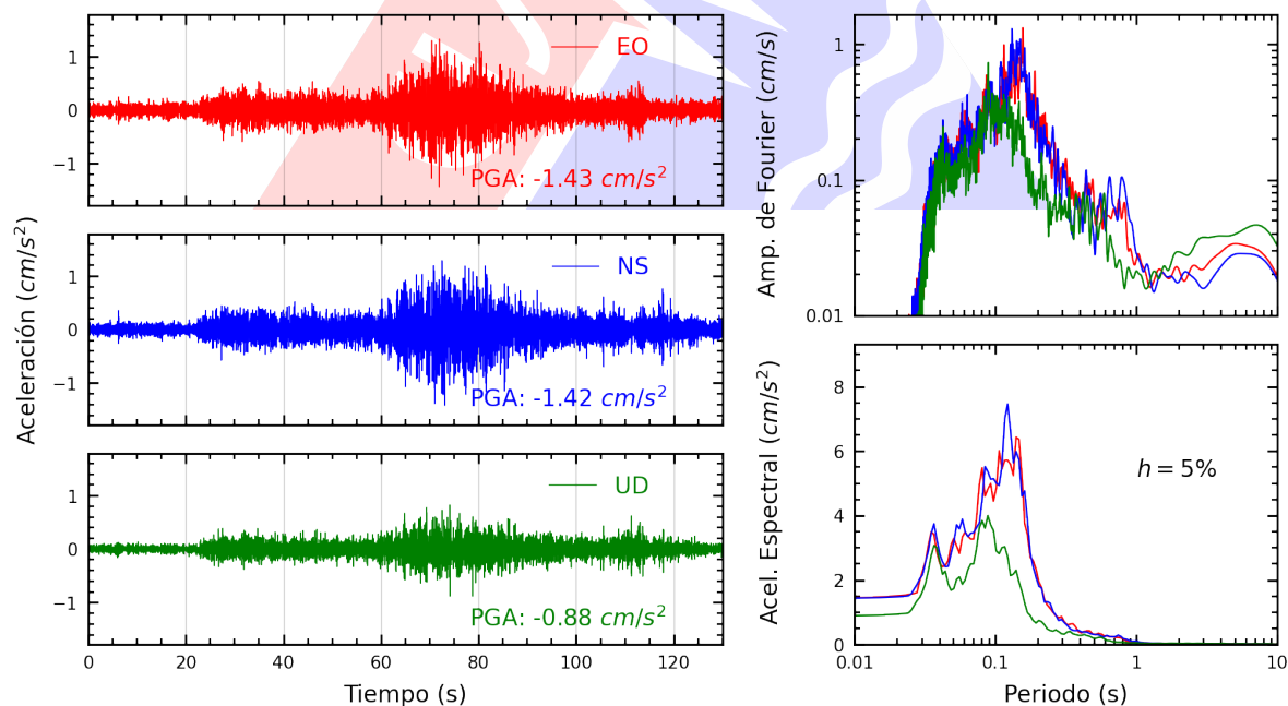
Figura A.4: Registros tiempo-historia, espectros de Fourier y de respuesta en las direcciones EO, NS y vertical de la estación USILM. Sismo de Palpa, Palpa - Ica del 2025-07-08, 16:32:53 (Hora local)
