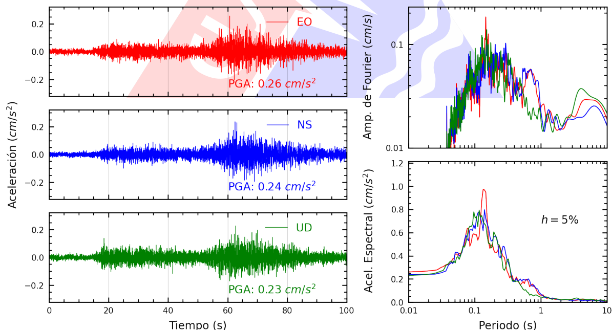
Figura A.38: Registros tiempo-historia, espectros de Fourier y de respuesta en las direcciones EO, NS y vertical de la estación UNMSM. Sismo de Palpa, Palpa - Ica del 2025-07-08, 16:32:53 (Hora local)
