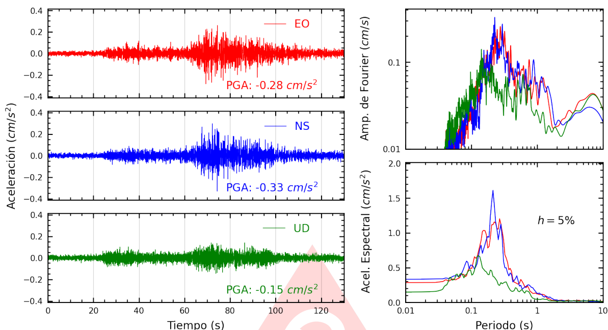
Figura A.29: Registros tiempo-historia, espectros de Fourier y de respuesta en las direcciones EO, NS y vertical de la estación DSML. Sismo de Palpa, Palpa - Ica del 2025-07-08, 16:32:53 (Hora local)
