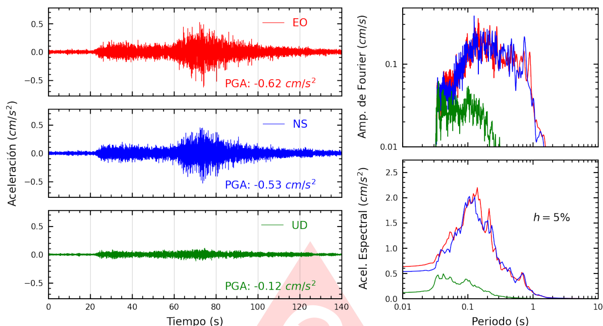
Figura A.19: Registros tiempo-historia, espectros de Fourier y de respuesta en las direcciones EO, NS y vertical de la estación UCVAT. Sismo de Palpa, Palpa - Ica del 2025-07-08, 16:32:53 (Hora local)
