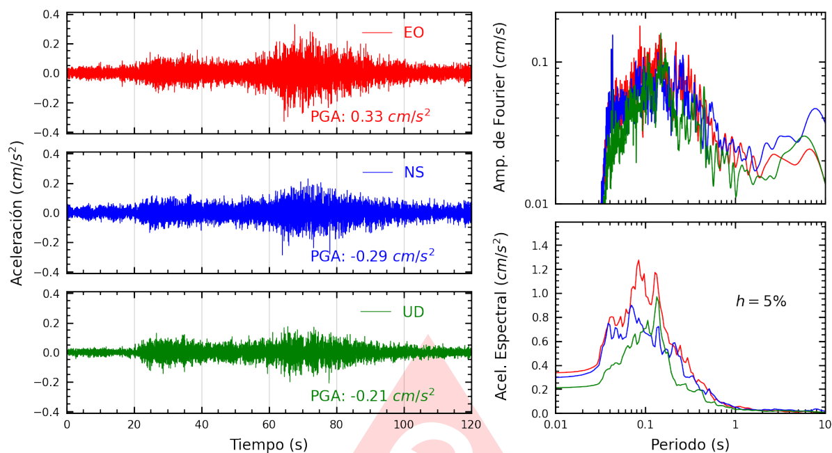
Figura A.31: Registros tiempo-historia, espectros de Fourier y de respuesta en las direcciones EO, NS y vertical de la estación CEPRE. Sismo de Palpa, Palpa - Ica del 2025-07-08, 16:32:53 (Hora local)
