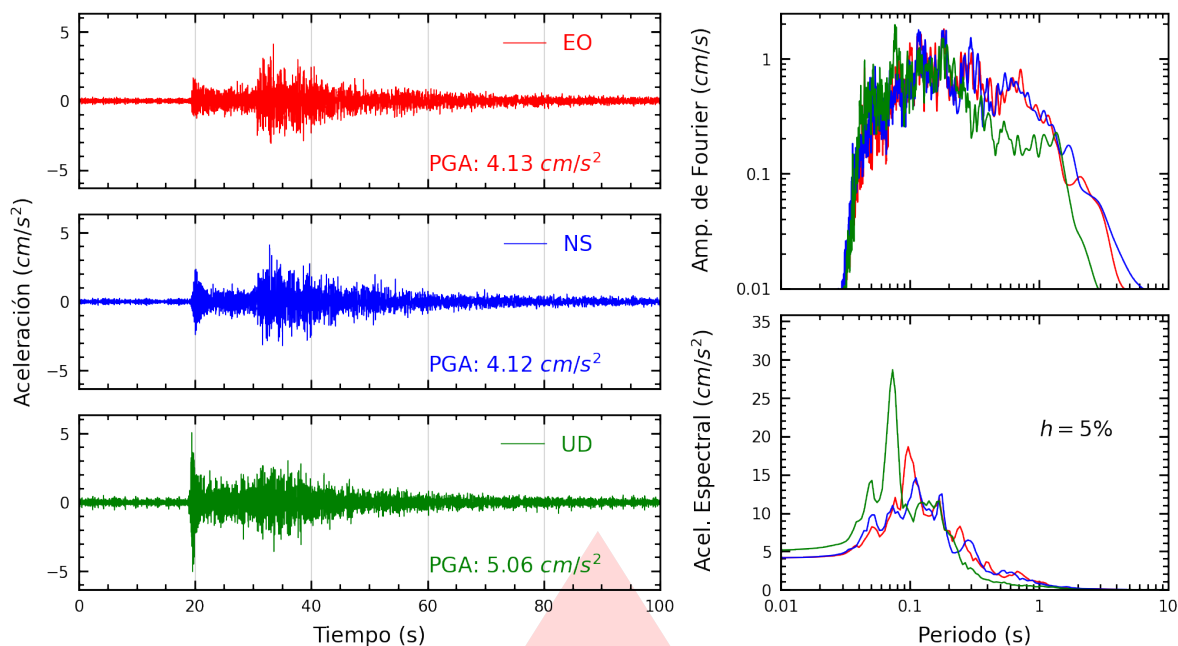
Figura A.1: Registros tiempo-historia, espectros de Fourier y de respuesta en las direcciones EO, NS y vertical de la estación UNICA. Sismo de Palpa, Palpa - Ica del 2025-07-08, 16:32:53 (Hora local)
