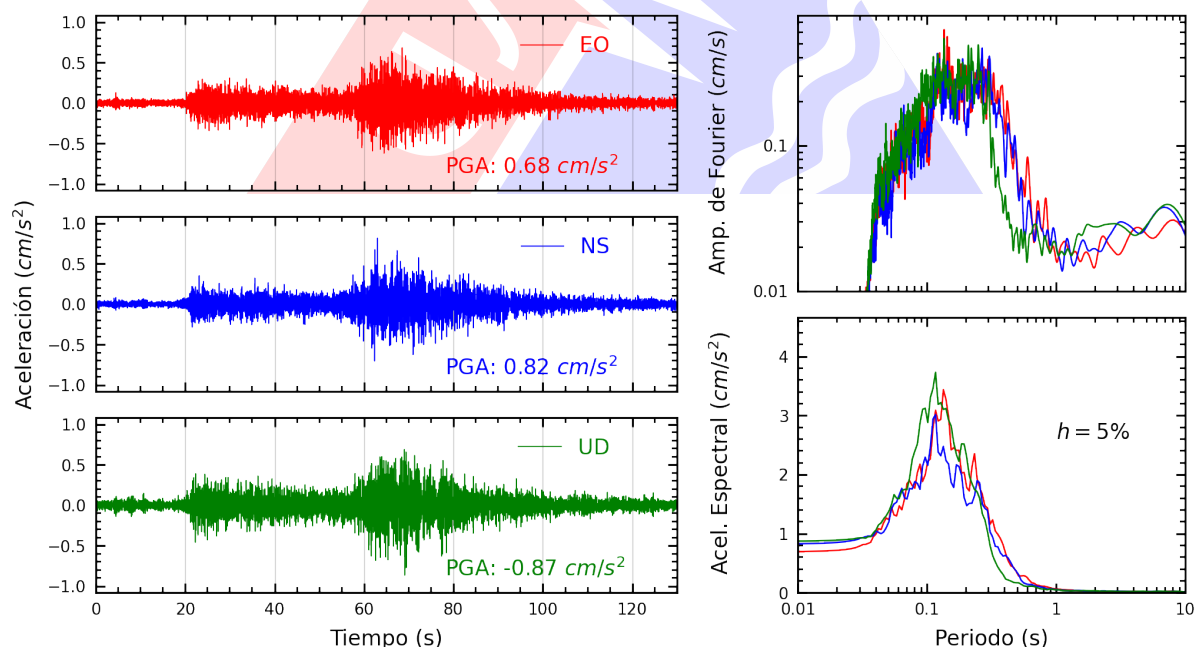
Figura A.12: Registros tiempo-historia, espectros de Fourier y de respuesta en las direcciones EO, NS y vertical de la estación SOVES. Sismo de Palpa, Palpa - Ica del 2025-07-08, 16:32:53 (Hora local)
