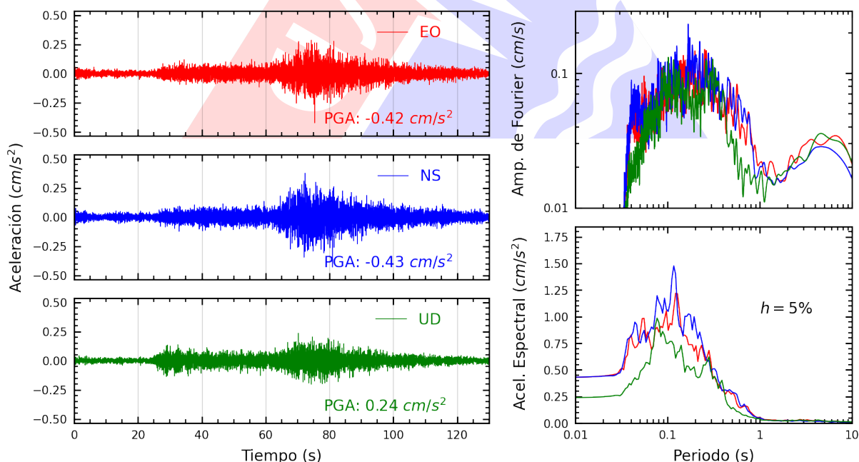
Figura A.26: Registros tiempo-historia, espectros de Fourier y de respuesta en las direcciones EO, NS y vertical de la estación COMAS. Sismo de Palpa, Palpa - Ica del 2025-07-08, 16:32:53 (Hora local)
