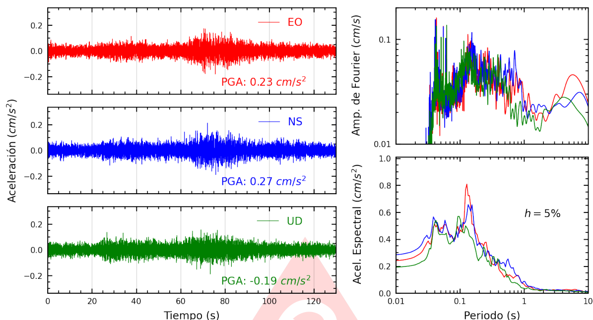
Figura A.35: Registros tiempo-historia, espectros de Fourier y de respuesta en las direcciones EO, NS y vertical de la estación BONDY. Sismo de Palpa, Palpa - Ica del 2025-07-08, 16:32:53 (Hora local)
