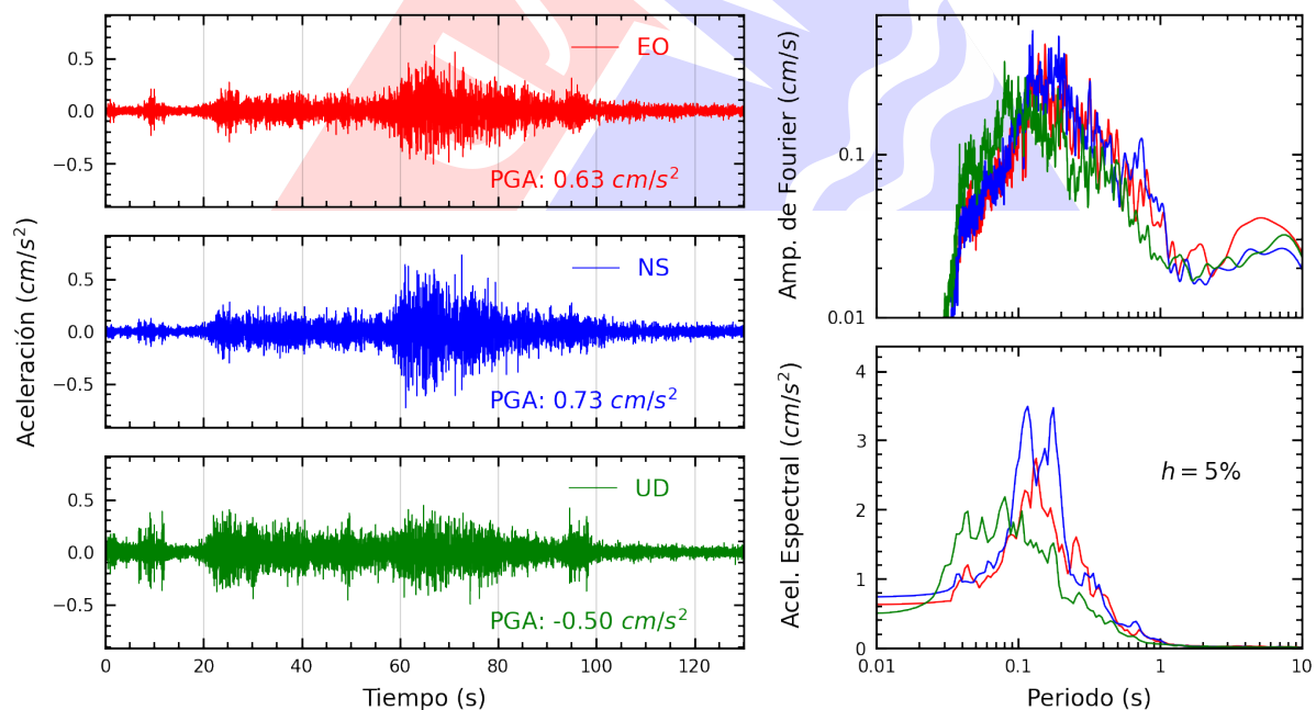
Figura A.18: Registros tiempo-historia, espectros de Fourier y de respuesta en las direcciones EO, NS y vertical de la estación SOCHO. Sismo de Palpa, Palpa - Ica del 2025-07-08, 16:32:53 (Hora local)
