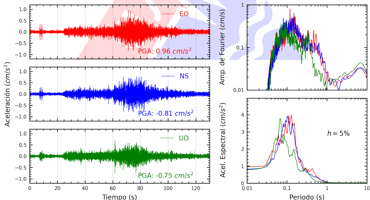
Figura A.8: Registros tiempo-historia, espectros de Fourier y de respuesta en las direcciones EO, NS y vertical de la estación SJLSV. Sismo de Palpa, Palpa - Ica del 2025-07-08, 16:32:53 (Hora local)
