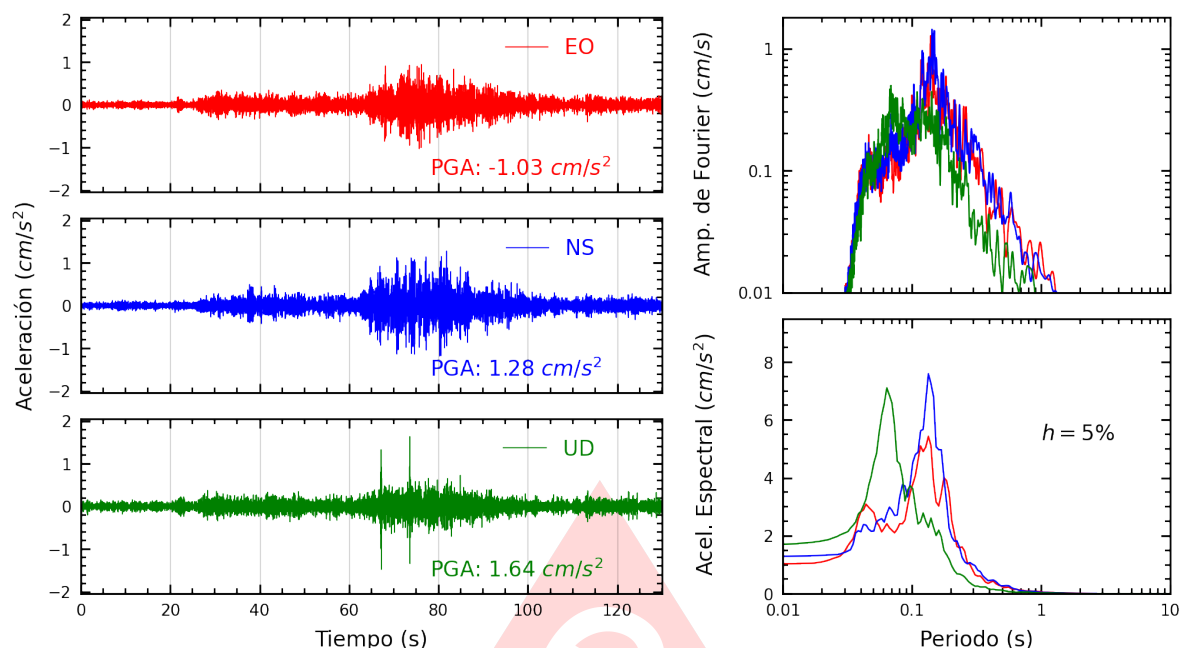
Figura A.3: Registros tiempo-historia, espectros de Fourier y de respuesta en las direcciones EO, NS y vertical de la estación CARAB. Sismo de Palpa, Palpa - Ica del 2025-07-08, 16:32:53 (Hora local)
