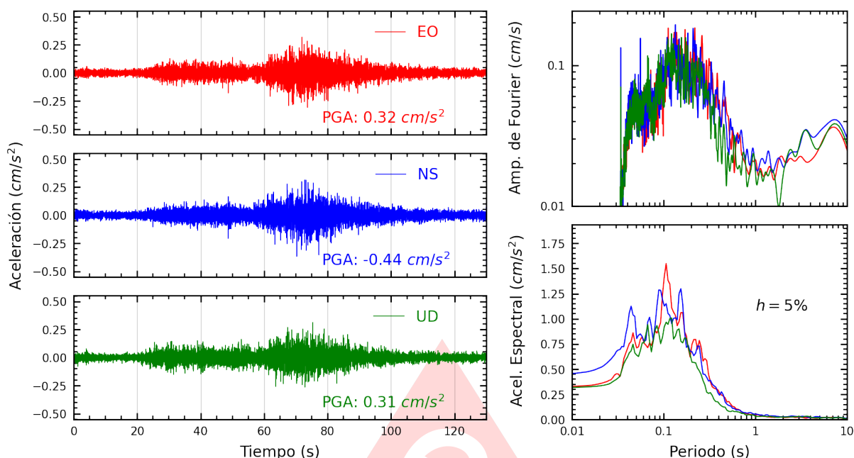
Figura A.25: Registros tiempo-historia, espectros de Fourier y de respuesta en las direcciones EO, NS y vertical de la estación USMP. Sismo de Palpa, Palpa - Ica del 2025-07-08, 16:32:53 (Hora local)
