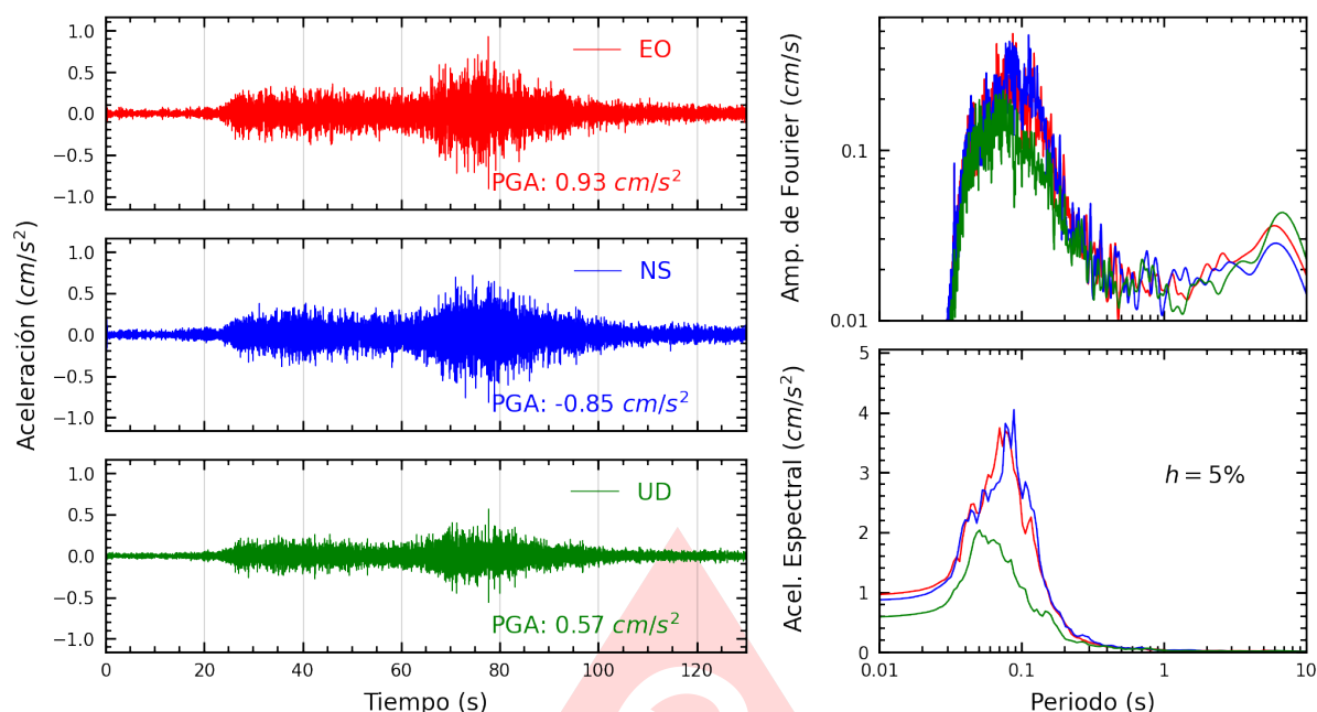
Figura A.9: Registros tiempo-historia, espectros de Fourier y de respuesta en las direcciones EO, NS y vertical de la estación JOSEO. Sismo de Palpa, Palpa - Ica del 2025-07-08, 16:32:53 (Hora local)
