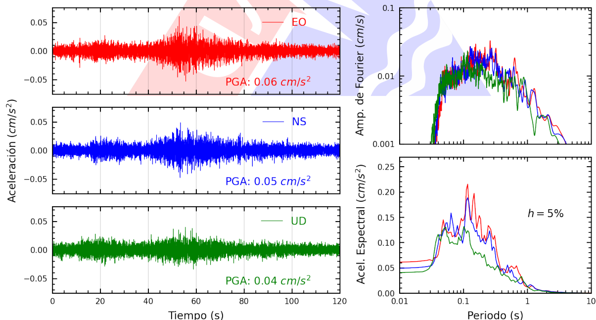
Figura A.10: Registros tiempo-historia, espectros de Fourier y de respuesta en las direcciones EO, NS y vertical de la estación JALV2. Sismo de Ica, Ica - Ica del 2025-07-09, 22:58:21 (Hora local)
