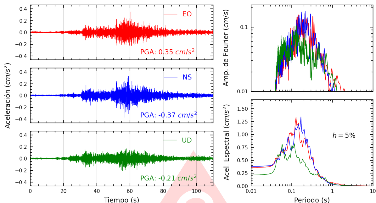
Figura A.3: Registros tiempo-historia, espectros de Fourier y de respuesta en las direcciones EO, NS y vertical de la estación ASIA. Sismo de Ica, Ica - Ica del 2025-07-09, 22:58:21 (Hora local)
