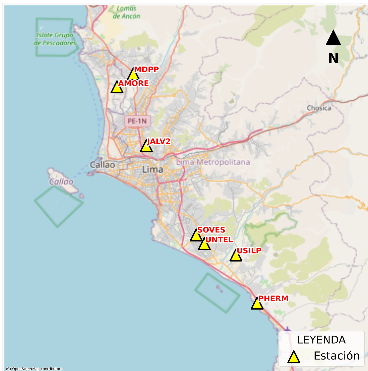
Figura 3: Mapa de ubicación de la(s) estación(es) acelerográfica(s) en Lima Metropolitana correspondiente(s) al Sismo de Ica, Ica - Ica del 09 de julio de 2025 a las 22:58:21 (hora local)
