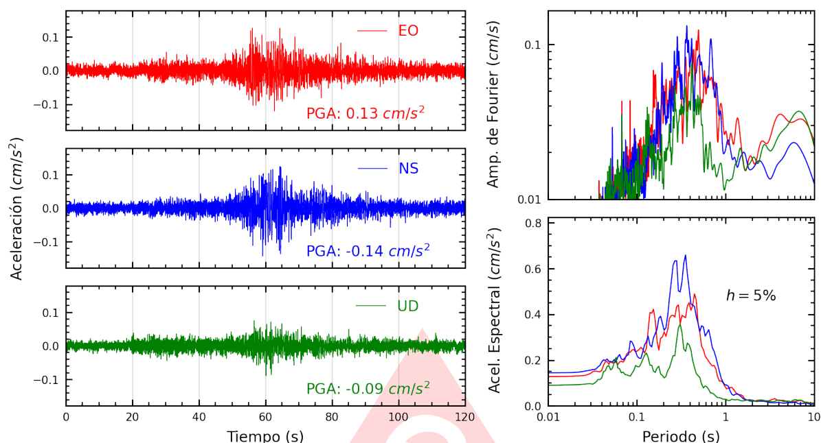
Figura A.7: Registros tiempo-historia, espectros de Fourier y de respuesta en las direcciones EO, NS y vertical de la estación USILP. Sismo de Ica, Ica - Ica del 2025-07-09, 22:58:21 (Hora local)
