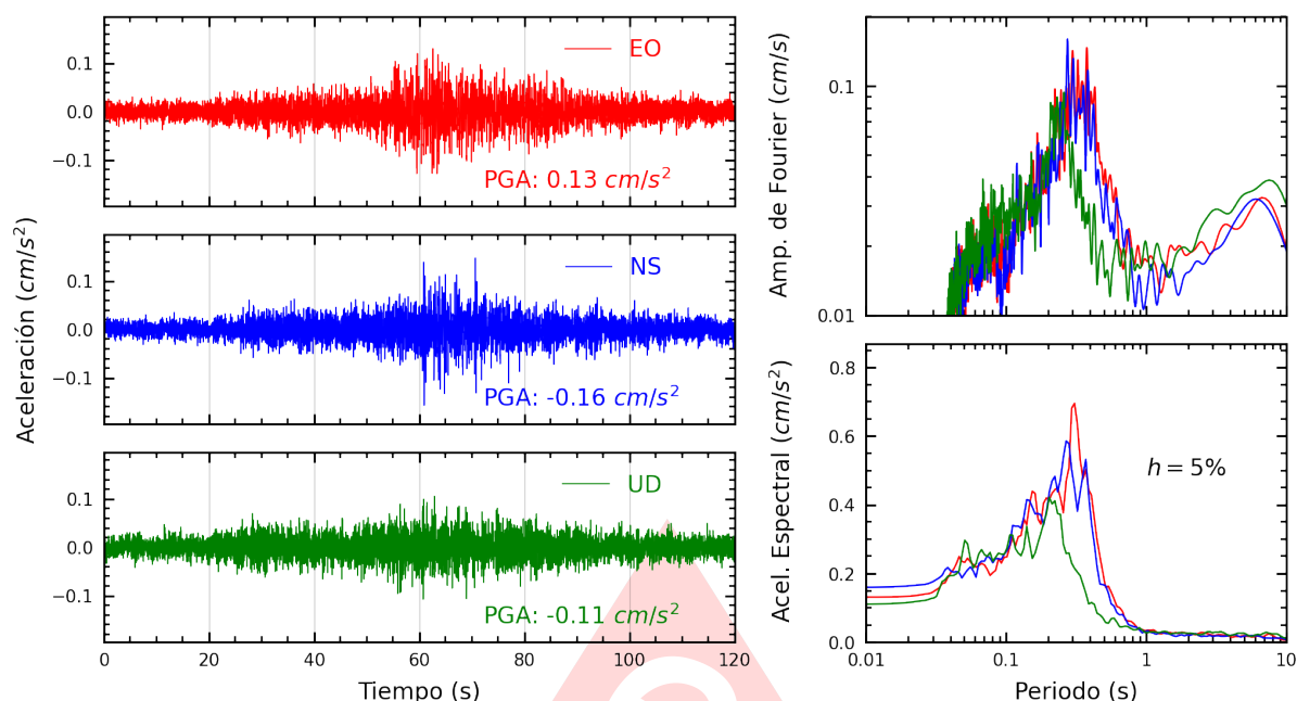
Figura A.5: Registros tiempo-historia, espectros de Fourier y de respuesta en las direcciones EO, NS y vertical de la estación SOVES. Sismo de Ica, Ica - Ica del 2025-07-09, 22:58:21 (Hora local)
