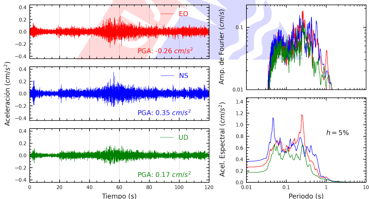
Figura A.4: Registros tiempo-historia, espectros de Fourier y de respuesta en las direcciones EO, NS y vertical de la estación PHERM. Sismo de Ica, Ica - Ica del 2025-07-09, 22:58:21 (Hora local)
