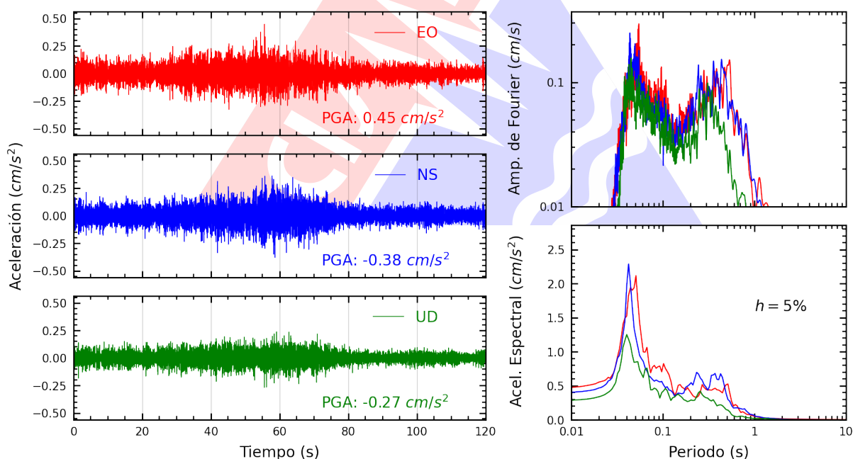
Figura A.2: Registros tiempo-historia, espectros de Fourier y de respuesta en las direcciones EO, NS y vertical de la estación UNTEL. Sismo de Ica, Ica - Ica del 2025-07-09, 22:58:21 (Hora local)
