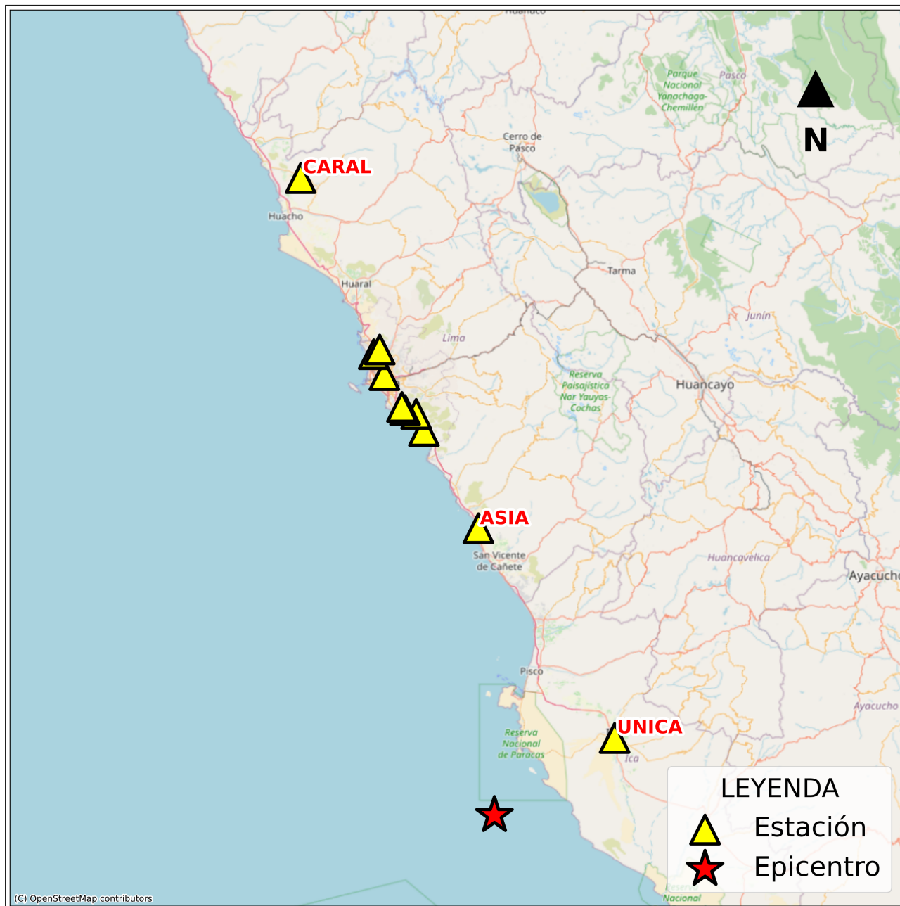
Figura 2: Mapa de ubicación de la(s) estación(es) acelerográfica(s) a nivel nacional correspondiente(s) al Sismo de Ica, Ica - Ica del 09 de julio de 2025 a las 22:58:21 (hora local)
