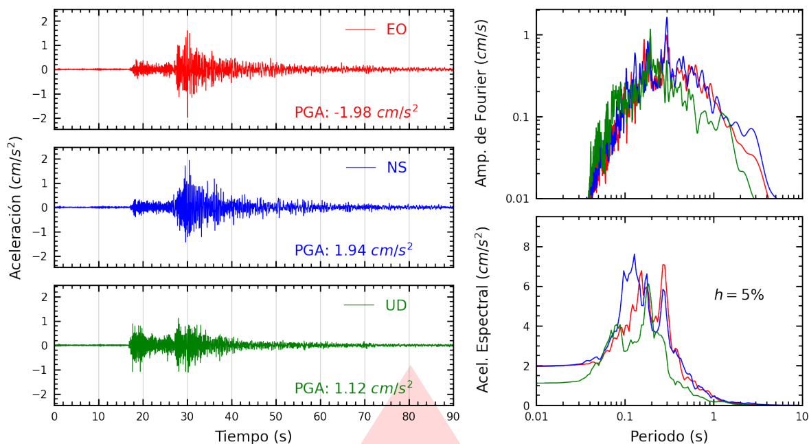
Figura A.1: Registros tiempo-historia, espectros de Fourier y de respuesta en las direcciones EO, NS y vertical de la estación UNICA. Sismo de Ica, Ica - Ica del 2025-07-09, 22:58:21 (Hora local)
