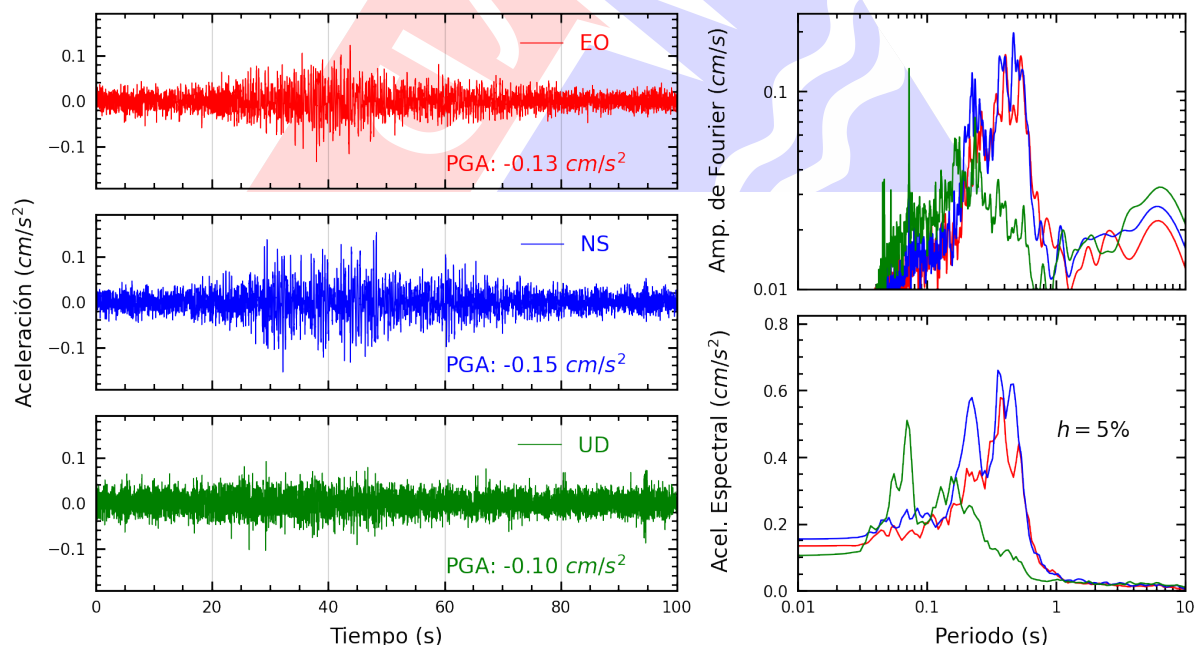
Figura A.6: Registros tiempo-historia, espectros de Fourier y de respuesta en las direcciones EO, NS y vertical de la estación MDPP. Sismo de Ica, Ica - Ica del 2025-07-09, 22:58:21 (Hora local)
