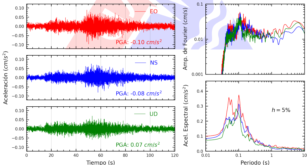
Figura A.8: Registros tiempo-historia, espectros de Fourier y de respuesta en las direcciones EO, NS y vertical de la estación AMORE. Sismo de Ica, Ica - Ica del 2025-07-09, 22:58:21 (Hora local)
