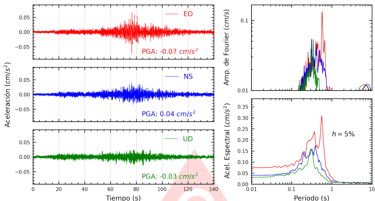
Figura A.9: Registros tiempo-historia, espectros de Fourier y de respuesta en las direcciones EO, NS y vertical de la estación CARAL. Sismo de Ica, Ica - Ica del 2025-07-09, 22:58:21 (Hora local)
