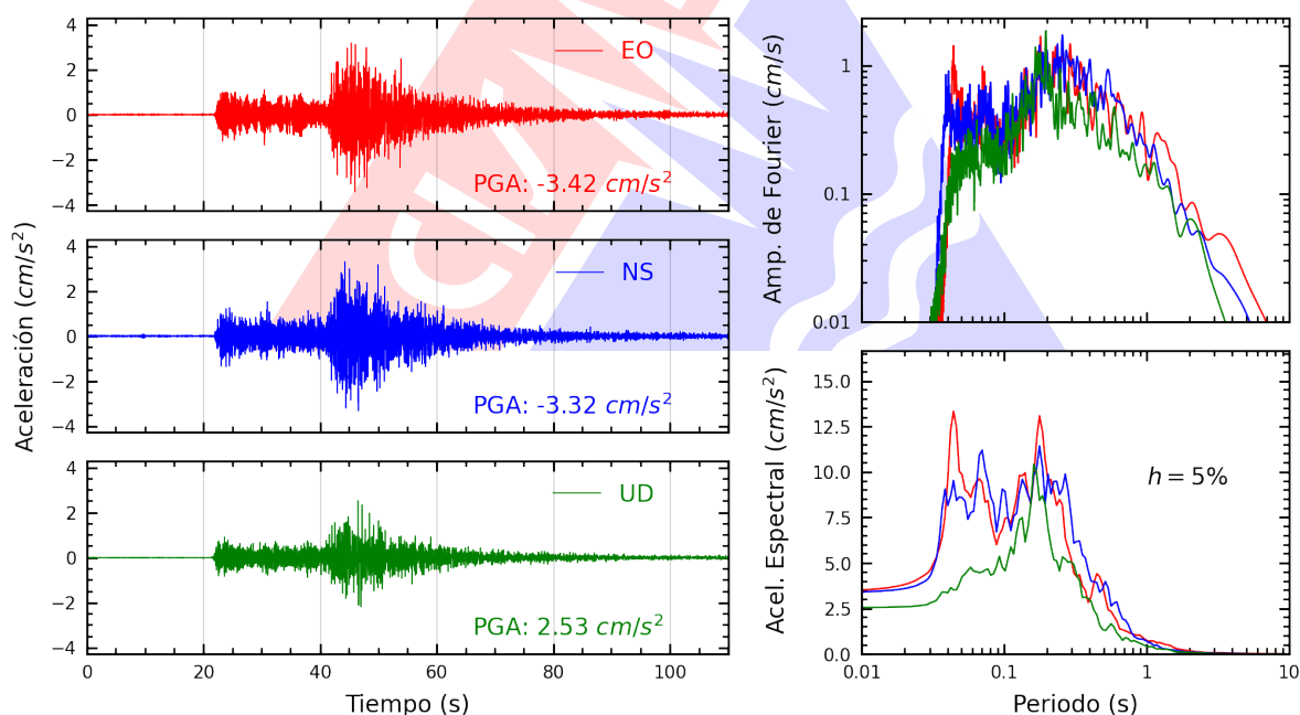
Figura A.2: Registros tiempo-historia, espectros de Fourier y de respuesta en las direcciones EO, NS y vertical de la estación UPTAC. Sismo de Calana, Tacna - Tacna del 2025-07-10, 04:26:05 (Hora local)
