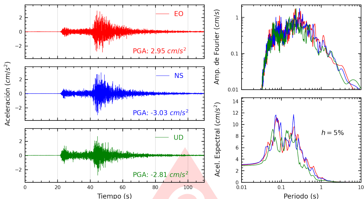
Figura A.3: Registros tiempo-historia, espectros de Fourier y de respuesta en las direcciones EO, NS y vertical de la estación CREY. Sismo de Calana, Tacna - Tacna del 2025-07-10, 04:26:05 (Hora local)
