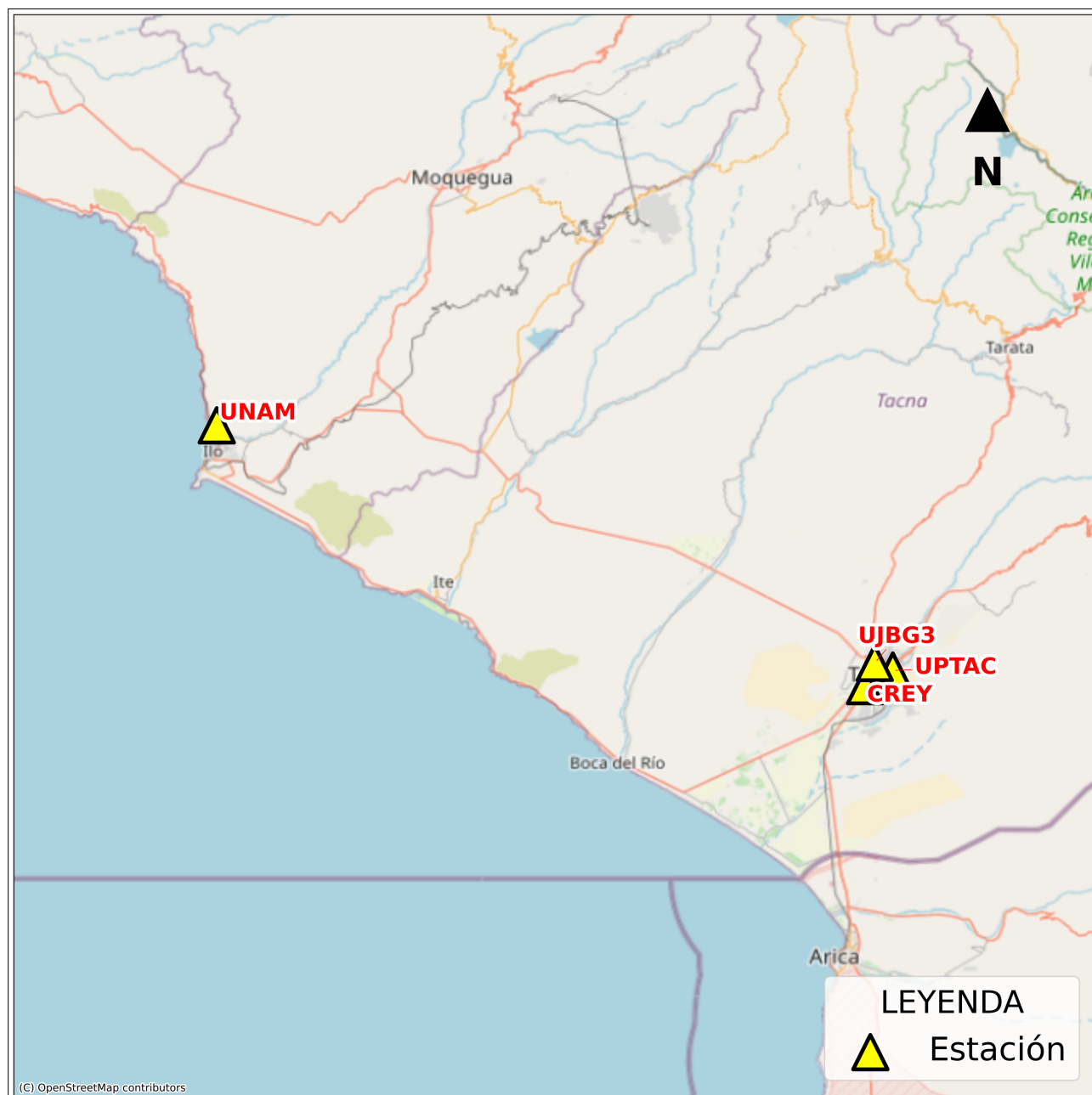
Figura 2: Mapa de ubicación de la(s) estación(es) acelerográfica(s) correspondiente(s) al Sismo de Calana, Tacna - Tacna del 10 de julio de 2025 a las 04:26:05 (hora local)
