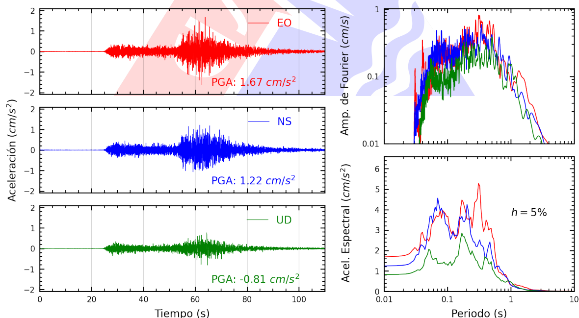
Figura A.4: Registros tiempo-historia, espectros de Fourier y de respuesta en las direcciones EO, NS y vertical de la estación UNAM. Sismo de Calana, Tacna - Tacna del 2025-07-10, 04:26:05 (Hora local)
