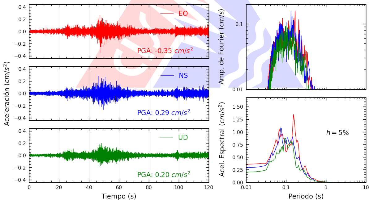
Figura A.2: Registros tiempo-historia, espectros de Fourier y de respuesta en las direcciones EO, NS y vertical de la estación PHERM. Sismo de Huancavelica, Huancavelica - Huancavelica del 2025-07-13, 05:07:36 (Hora local)
