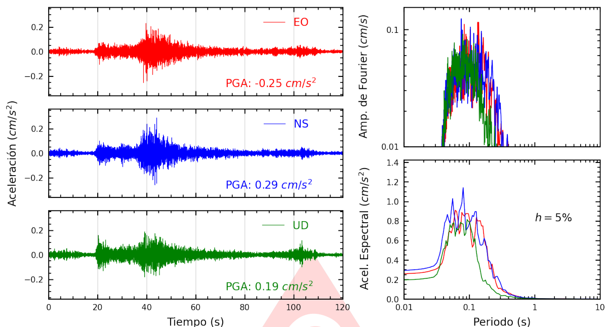
Figura A.3: Registros tiempo-historia, espectros de Fourier y de respuesta en las direcciones EO, NS y vertical de la estación ASIA. Sismo de Huancavelica, Huancavelica - Huancavelica del 2025-07-13, 05:07:36 (Hora local)
