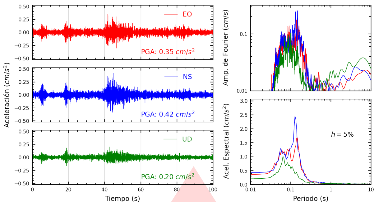
Figura A.1: Registros tiempo-historia, espectros de Fourier y de respuesta en las direcciones EO, NS y vertical de la estación USILM. Sismo de Huancavelica, Huancavelica - Huancavelica del 2025-07-13, 05:07:36 (Hora local)
