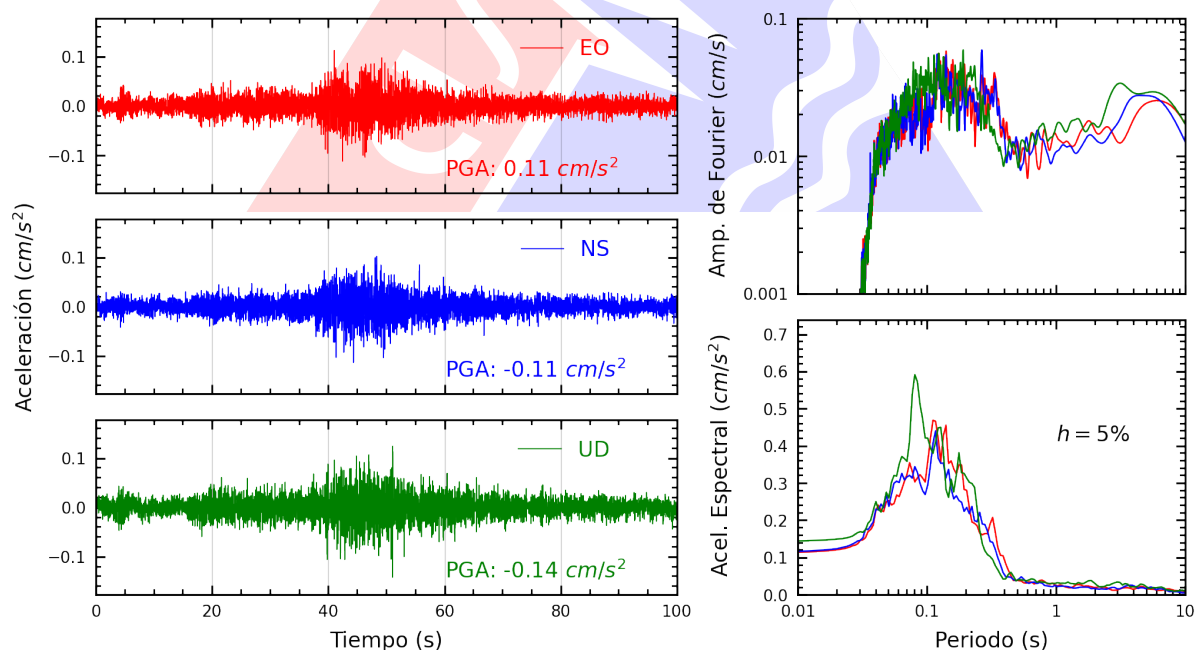
Figura A.4: Registros tiempo-historia, espectros de Fourier y de respuesta en las direcciones EO, NS y vertical de la estación SOVES. Sismo de Huancavelica, Huancavelica - Huancavelica del 2025-07-13, 05:07:36 (Hora local)
