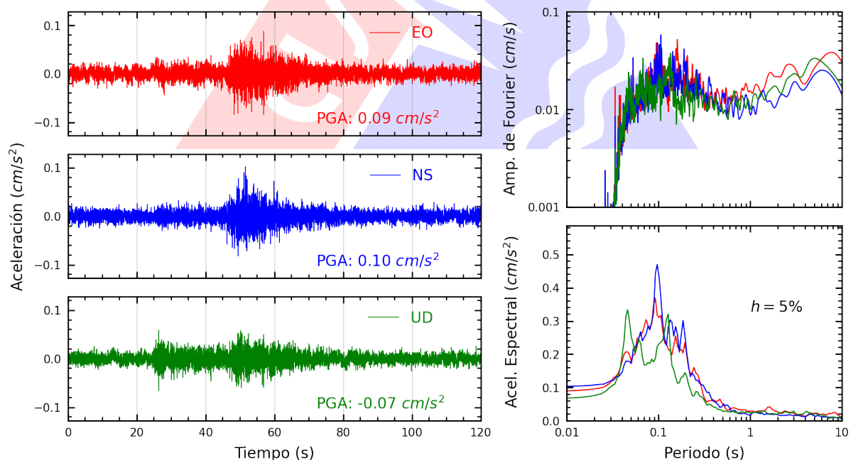
Figura A.6: Registros tiempo-historia, espectros de Fourier y de respuesta en las direcciones EO, NS y vertical de la estación USILP. Sismo de Huancavelica, Huancavelica - Huancavelica del 2025-07-13, 05:07:36 (Hora local)
