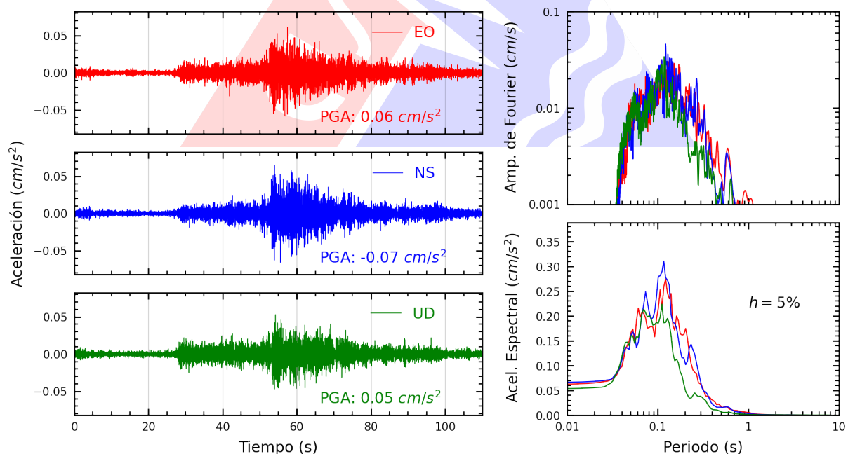
Figura A.8: Registros tiempo-historia, espectros de Fourier y de respuesta en las direcciones EO, NS y vertical de la estación JALV2. Sismo de Huancavelica, Huancavelica - Huancavelica del 2025-07-13, 05:07:36 (Hora local)
