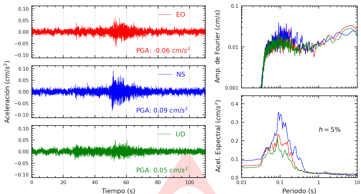
Figura A.7: Registros tiempo-historia, espectros de Fourier y de respuesta en las direcciones EO, NS y vertical de la estación SERVI. Sismo de Huancavelica, Huancavelica - Huancavelica del 2025-07-13, 05:07:36 (Hora local)
