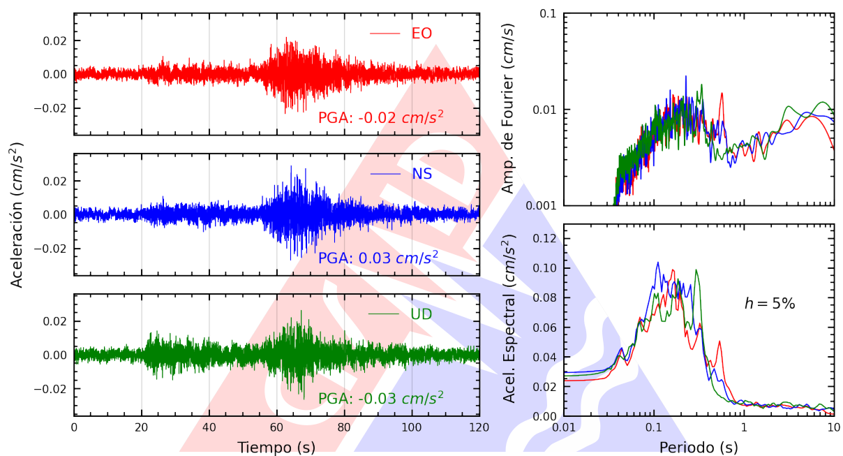
Figura A.9: Registros tiempo-historia, espectros de Fourier y de respuesta en las direcciones EO, NS y vertical de la estación CARAL. Sismo de Huancavelica, Huancavelica - Huancavelica del 2025-07-13, 05:07:36 (Hora local)
