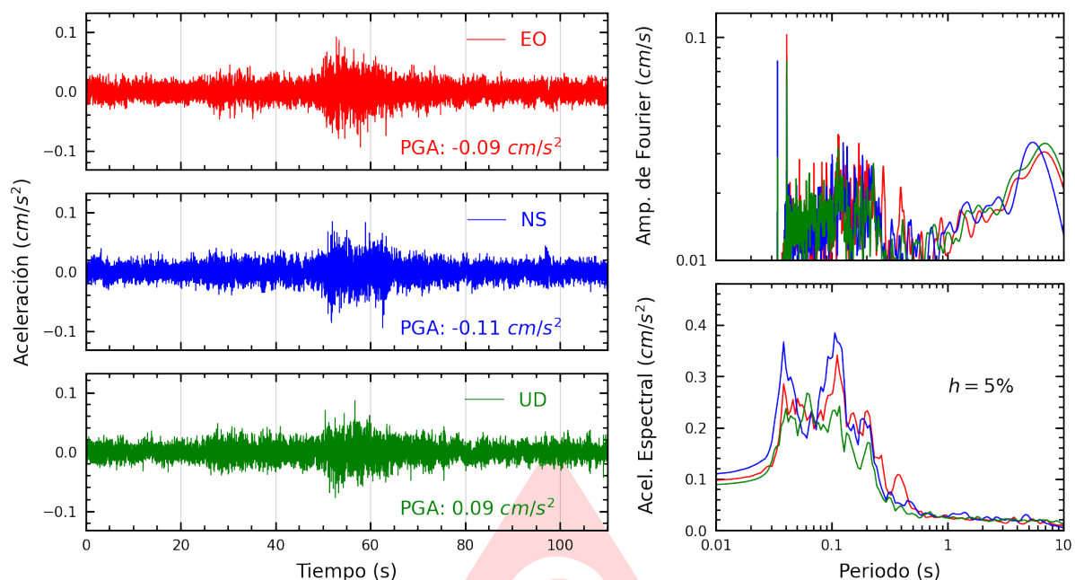
Figura A.5: Registros tiempo-historia, espectros de Fourier y de respuesta en las direcciones EO, NS y vertical de la estación USMP. Sismo de Huancavelica, Huancavelica - Huancavelica del 2025-07-13, 05:07:36 (Hora local)
