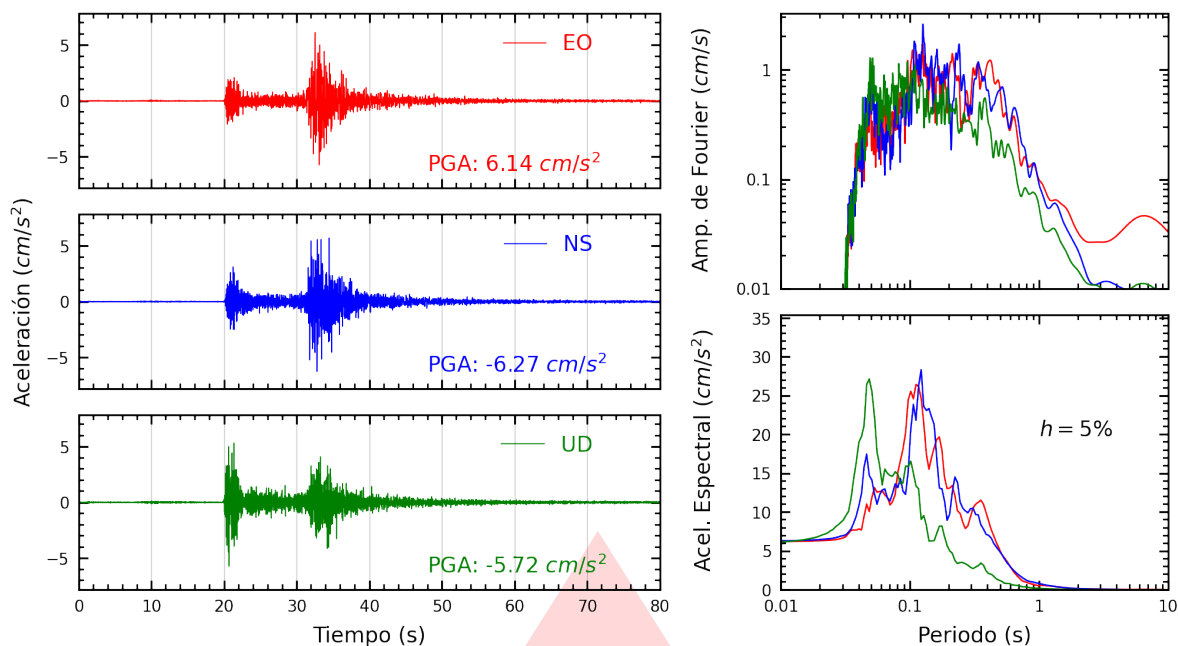
Figura A.1: Registros tiempo-historia, espectros de Fourier y de respuesta en las direcciones EO, NS y vertical de la estación UJBG3. Sismo de Calana, Tacna - Tacna del 2025-07-14, 14:37:05 (Hora local)
