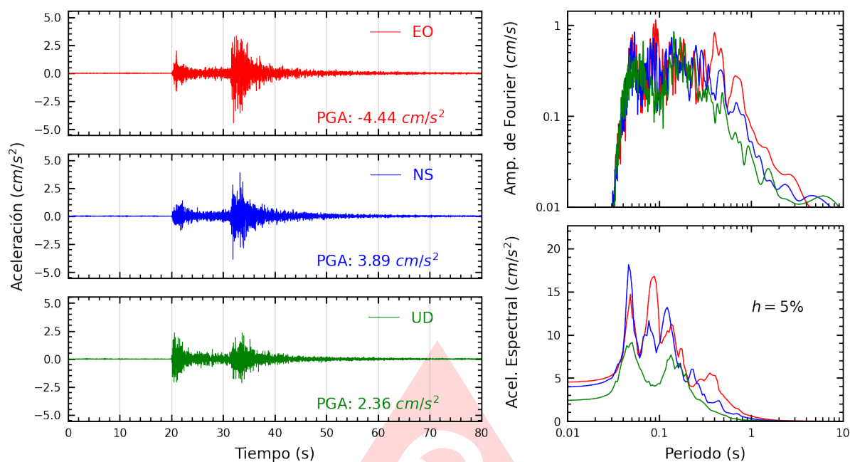
Figura A.3: Registros tiempo-historia, espectros de Fourier y de respuesta en las direcciones EO, NS y vertical de la estación CREY. Sismo de Calana, Tacna - Tacna del 2025-07-14, 14:37:05 (Hora local)
