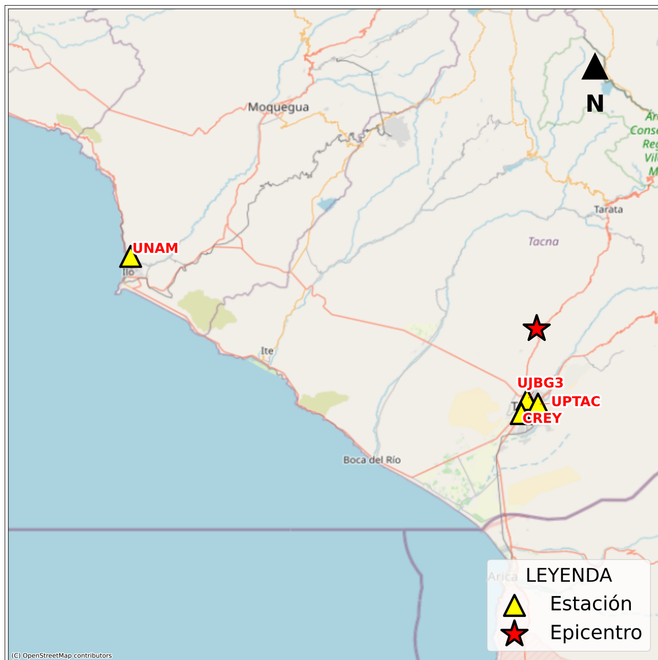
Figura 2: Mapa de ubicación de la(s) estación(es) acelerográfica(s) correspondiente(s) al Sismo de Calana, Tacna - Tacna del 14 de julio de 2025 a las 14:37:05 (hora local)
