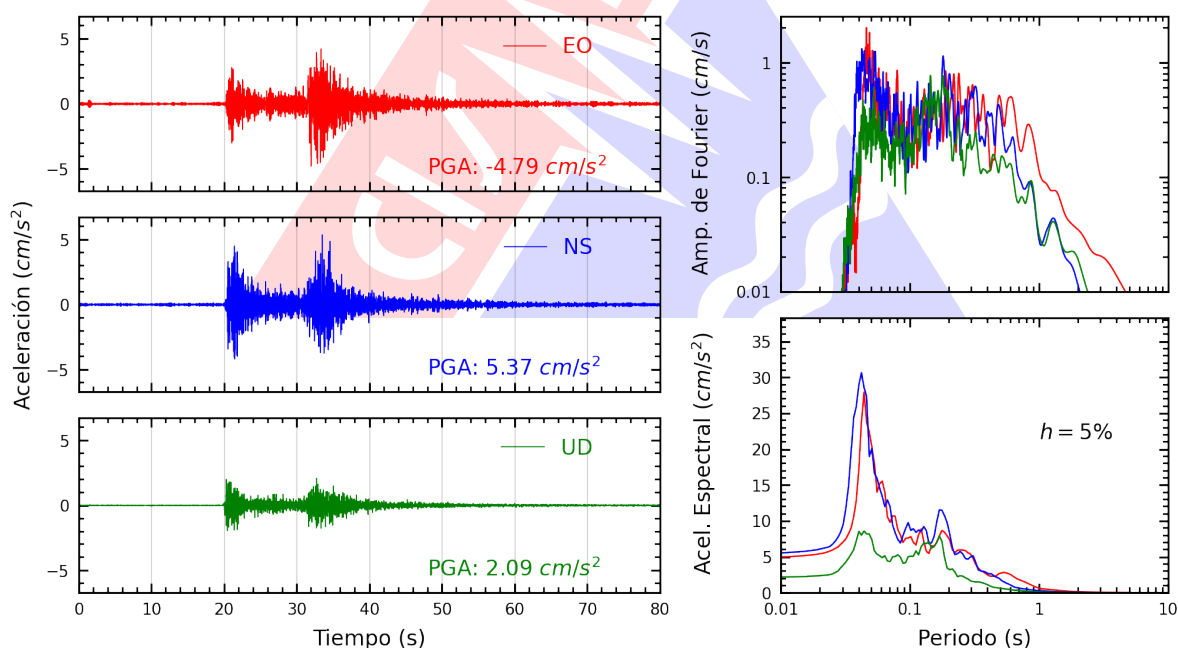
Figura A.2: Registros tiempo-historia, espectros de Fourier y de respuesta en las direcciones EO, NS y vertical de la estación UPTAC. Sismo de Calana, Tacna - Tacna del 2025-07-14, 14:37:05 (Hora local)
