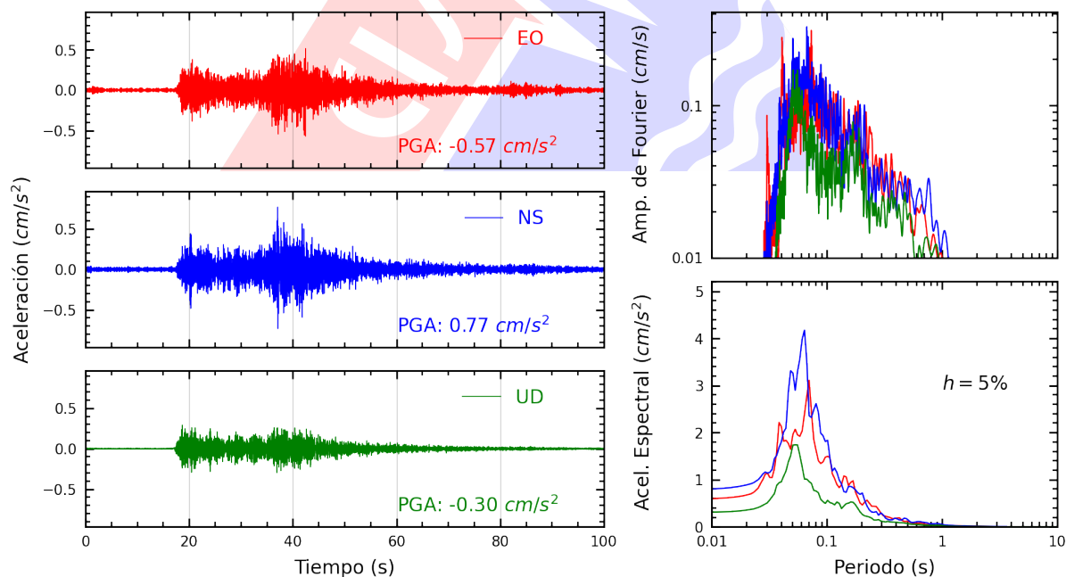
Figura A.4: Registros tiempo-historia, espectros de Fourier y de respuesta en las direcciones EO, NS y vertical de la estación UNAM. Sismo de Calana, Tacna - Tacna del 2025-07-14, 14:37:05 (Hora local)
