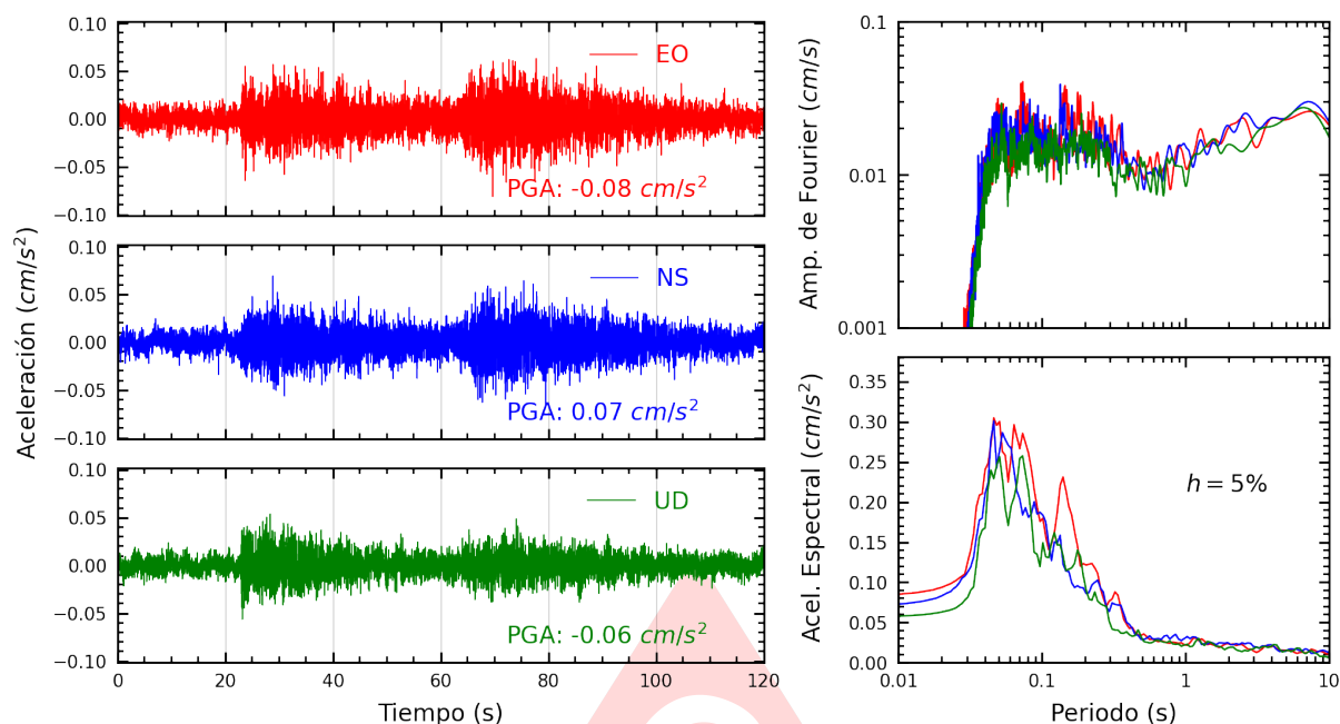
Figura A.9: Registros tiempo-historia, espectros de Fourier y de respuesta en las direcciones EO, NS y vertical de la estación FICPE. Sismo de Salaverry, Trujillo - La Libertad del 2025-07-15, 01:46:13 (Hora local)
