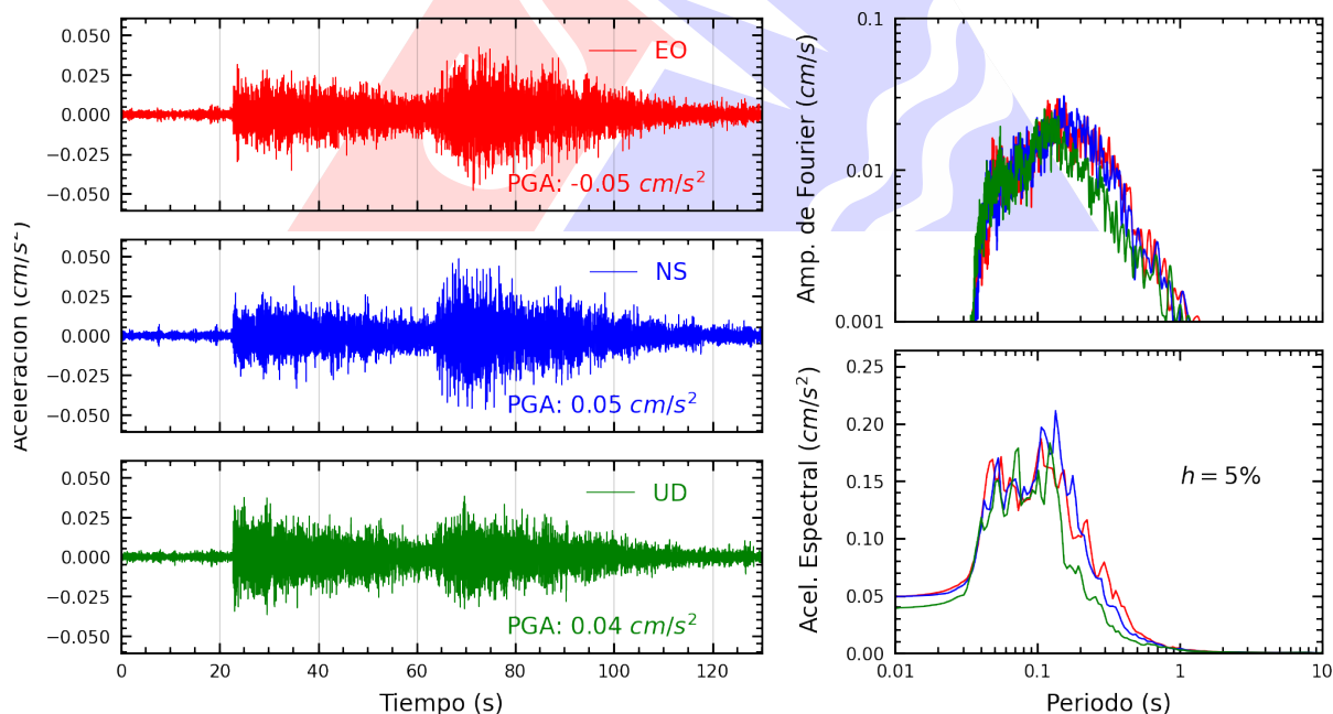
Figura A.10: Registros tiempo-historia, espectros de Fourier y de respuesta en las direcciones EO, NS y vertical de la estación JALV2. Sismo de Salaverry, Trujillo - La Libertad del 2025-07-15, 01:46:13 (Hora local)
