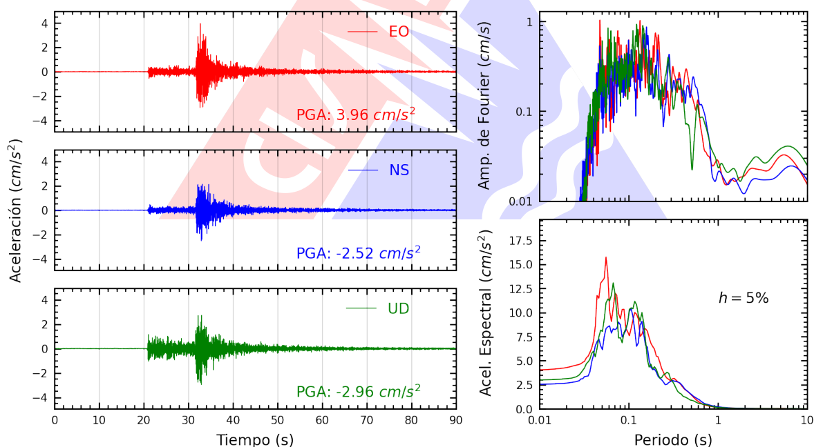
Figura A.2: Registros tiempo-historia, espectros de Fourier y de respuesta en las direcciones EO, NS y vertical de la estación UPAOT. Sismo de Salaverry, Trujillo - La Libertad del 2025-07-15, 01:46:13 (Hora local)
