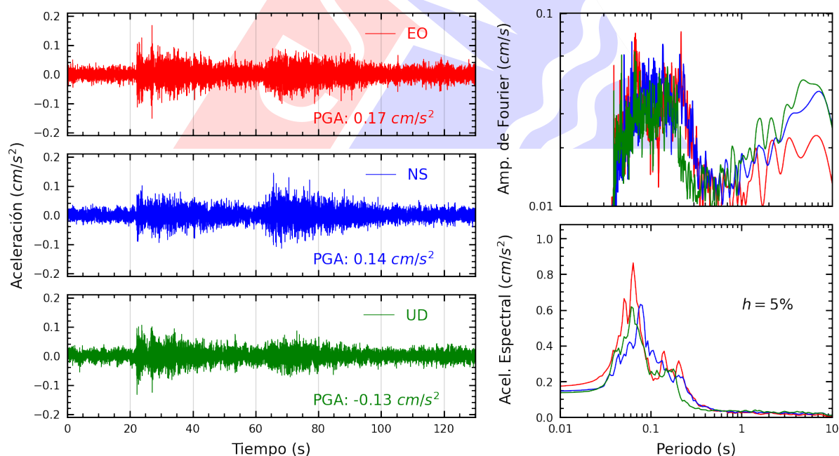
Figura A.4: Registros tiempo-historia, espectros de Fourier y de respuesta en las direcciones EO, NS y vertical de la estación INDEP. Sismo de Salaverry, Trujillo - La Libertad del 2025-07-15, 01:46:13 (Hora local)
