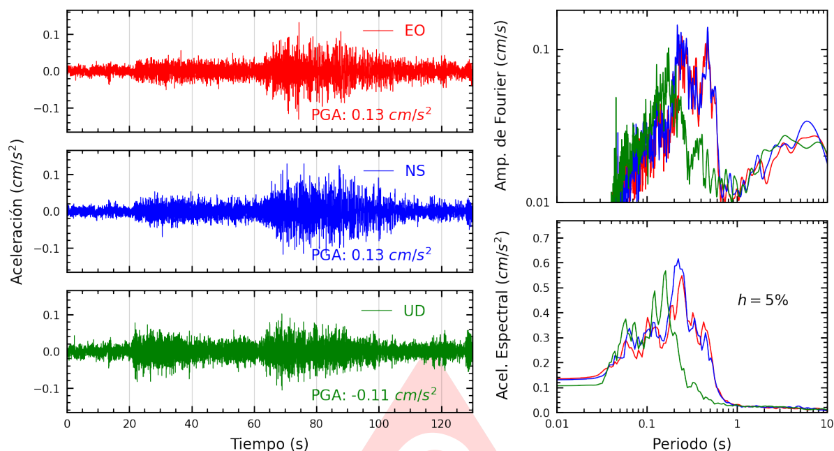
Figura A.7: Registros tiempo-historia, espectros de Fourier y de respuesta en las direcciones EO, NS y vertical de la estación MDPP. Sismo de Salaverry, Trujillo - La Libertad del 2025-07-15, 01:46:13 (Hora local)
