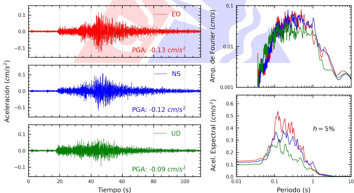
Figura A.8: Registros tiempo-historia, espectros de Fourier y de respuesta en las direcciones EO, NS y vertical de la estación UNC. Sismo de Salaverry, Trujillo - La Libertad del 2025-07-15, 01:46:13 (Hora local)
