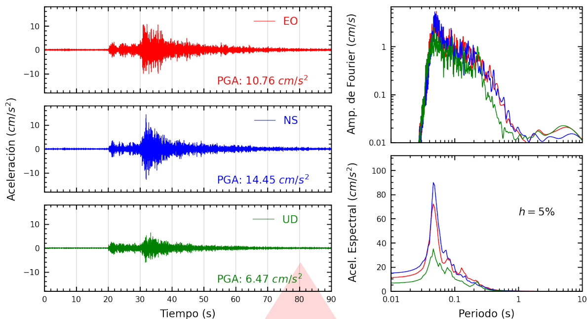
Figura A.1: Registros tiempo-historia, espectros de Fourier y de respuesta en las direcciones EO, NS y vertical de la estación USP. Sismo de Salaverry, Trujillo - La Libertad del 2025-07-15, 01:46:13 (Hora local)
