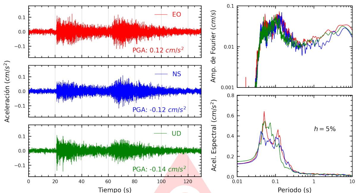
Figura A.5: Registros tiempo-historia, espectros de Fourier y de respuesta en las direcciones EO, NS y vertical de la estación AMORE. Sismo de Salaverry, Trujillo - La Libertad del 2025-07-15, 01:46:13 (Hora local)
