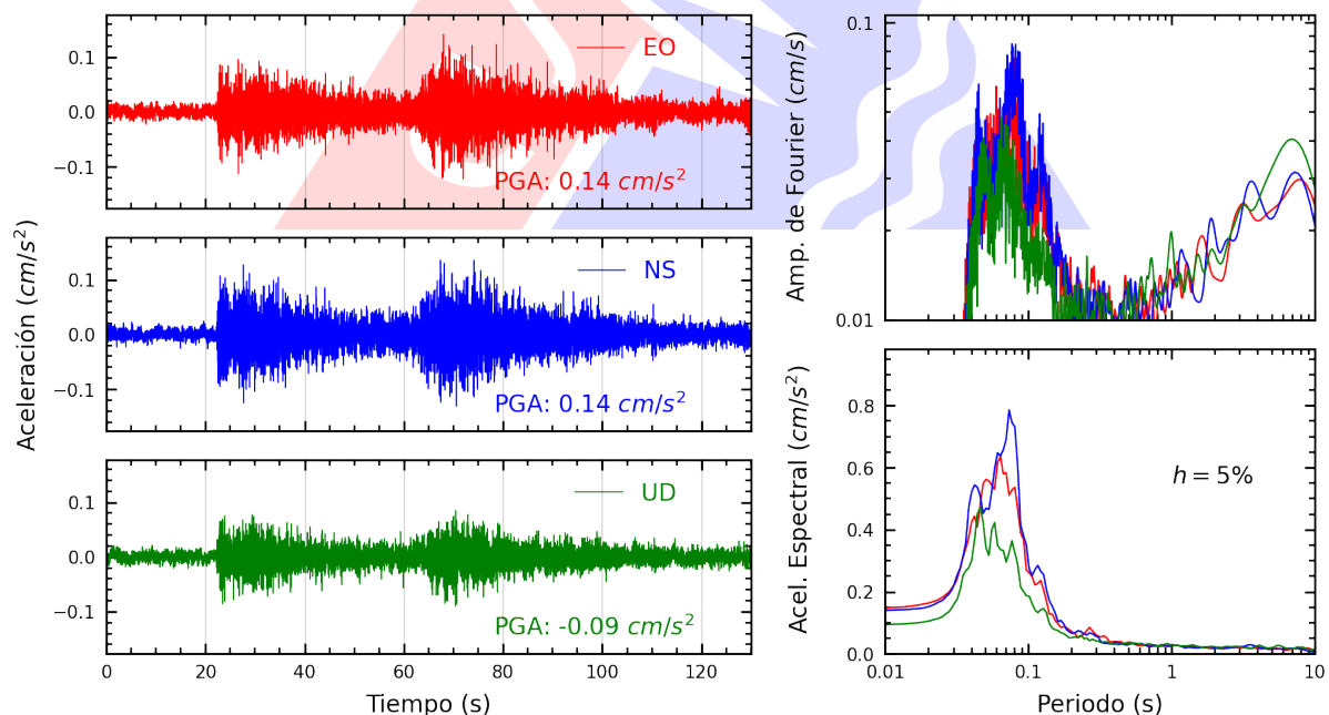
Figura A.6: Registros tiempo-historia, espectros de Fourier y de respuesta en las direcciones EO, NS y vertical de la estación JOSEO. Sismo de Salaverry, Trujillo - La Libertad del 2025-07-15, 01:46:13 (Hora local)
