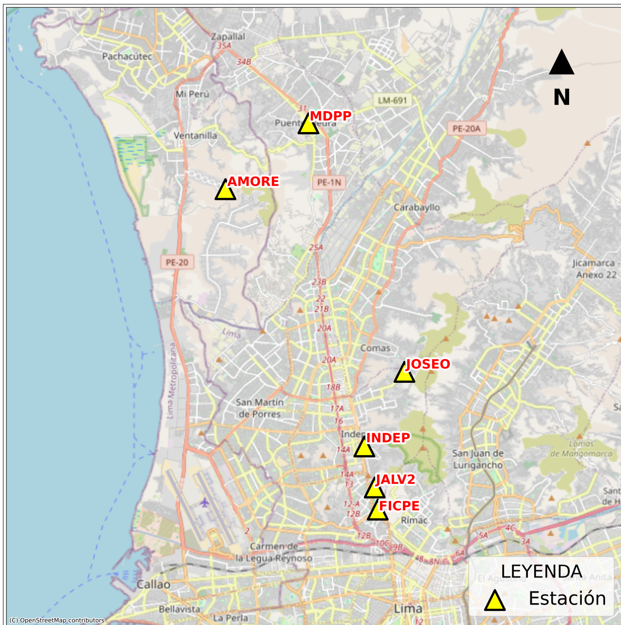
Figura 3: Mapa de ubicación de la(s) estación(es) acelerográfica(s) en Lima Metropolitana correspondiente(s) al Sismo de Salaverry, Trujillo - La Libertad del 15 de julio de 2025 a las 01:46:13 (hora local)
