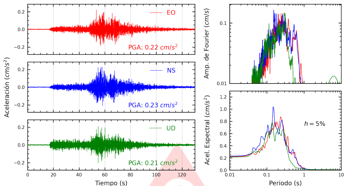
Figura A.3: Registros tiempo-historia, espectros de Fourier y de respuesta en las direcciones EO, NS y vertical de la estación CARAL. Sismo de Salaverry, Trujillo - La Libertad del 2025-07-15, 01:46:13 (Hora local)
