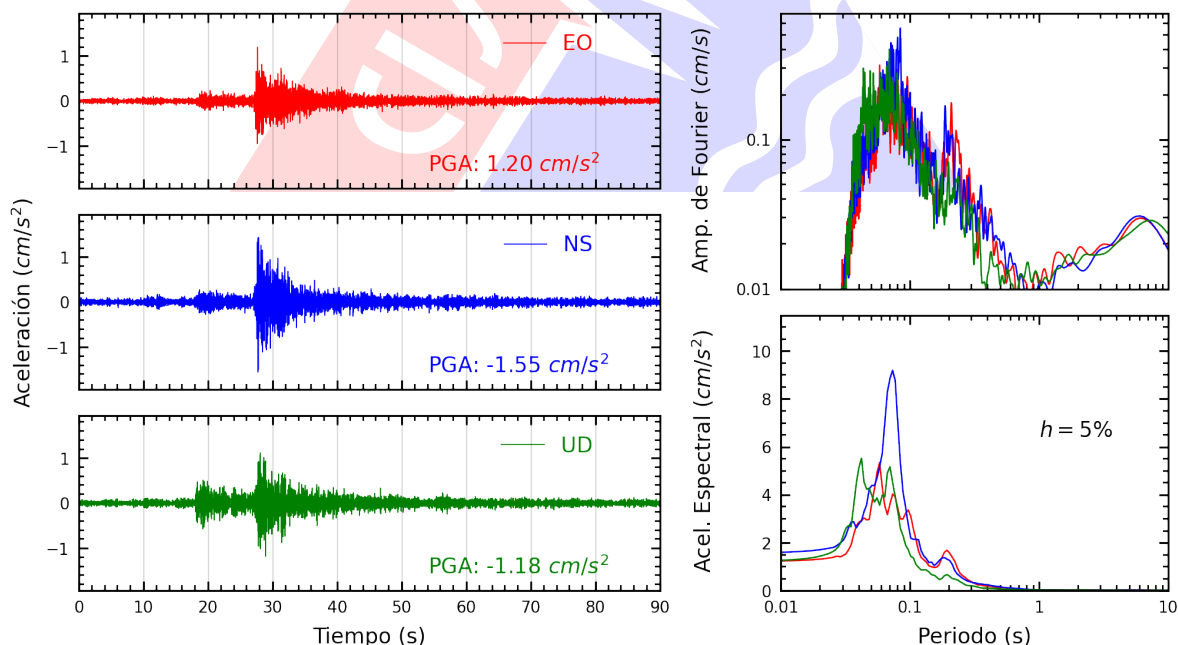
Figura A.6: Registros tiempo-historia, espectros de Fourier y de respuesta en las direcciones EO, NS y vertical de la estación SJLSC. Sismo de Chilca, Cañete - Lima del 2025-07-18, 07:13:55 (Hora local)
