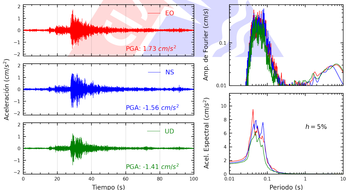
Figura A.4: Registros tiempo-historia, espectros de Fourier y de respuesta en las direcciones EO, NS y vertical de la estación JOSEO. Sismo de Chilca, Cañete - Lima del 2025-07-18, 07:13:55 (Hora local)
