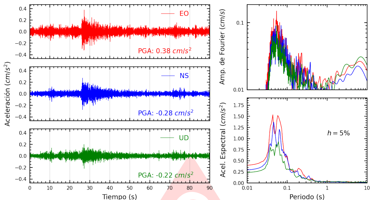
Figura A.31: Registros tiempo-historia, espectros de Fourier y de respuesta en las direcciones EO, NS y vertical de la estación INICT. Sismo de Chilca, Cañete - Lima del 2025-07-18, 07:13:55 (Hora local)
