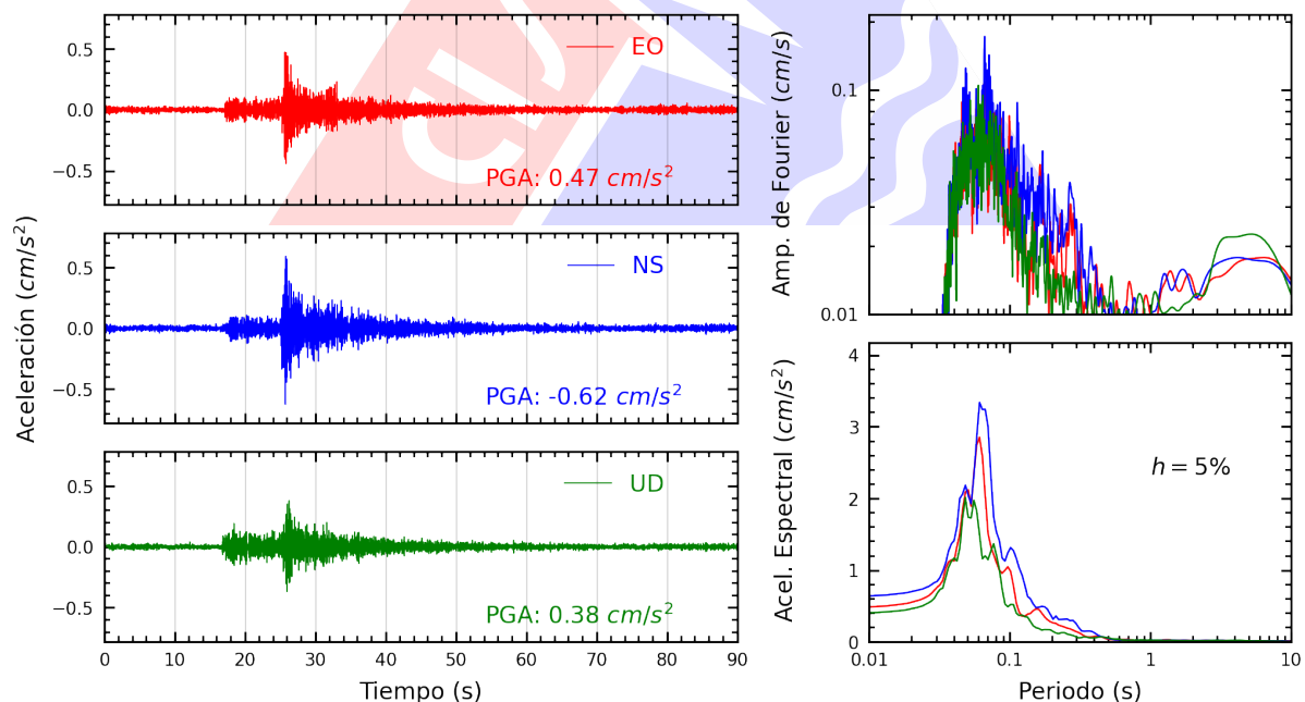
Figura A.24: Registros tiempo-historia, espectros de Fourier y de respuesta en las direcciones EO, NS y vertical de la estación SERVI. Sismo de Chilca, Cañete - Lima del 2025-07-18, 07:13:55 (Hora local)
