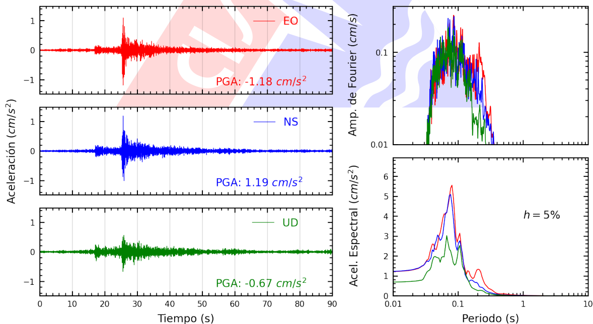
Figura A.10: Registros tiempo-historia, espectros de Fourier y de respuesta en las direcciones EO, NS y vertical de la estación ASIA. Sismo de Chilca, Cañete - Lima del 2025-07-18, 07:13:55 (Hora local)
