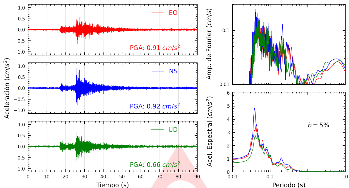
Figura A.13: Registros tiempo-historia, espectros de Fourier y de respuesta en las direcciones EO, NS y vertical de la estación USMP. Sismo de Chilca, Cañete - Lima del 2025-07-18, 07:13:55 (Hora local)
