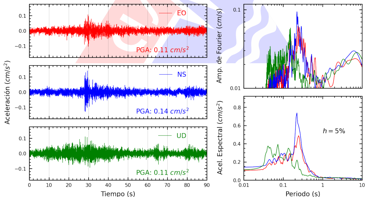
Figura A.34: Registros tiempo-historia, espectros de Fourier y de respuesta en las direcciones EO, NS y vertical de la estación DSMI. Sismo de Chilca, Cañete - Lima del 2025-07-18, 07:13:55 (Hora local)
