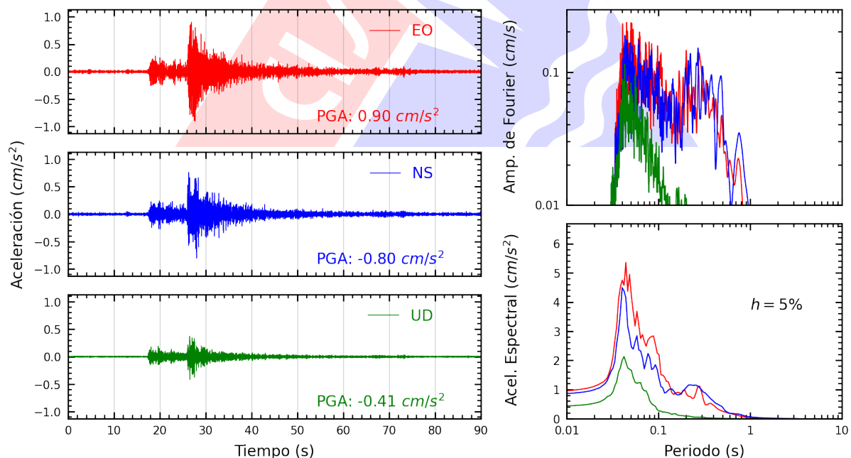
Figura A.14: Registros tiempo-historia, espectros de Fourier y de respuesta en las direcciones EO, NS y vertical de la estación UCVAT. Sismo de Chilca, Cañete - Lima del 2025-07-18, 07:13:55 (Hora local)
