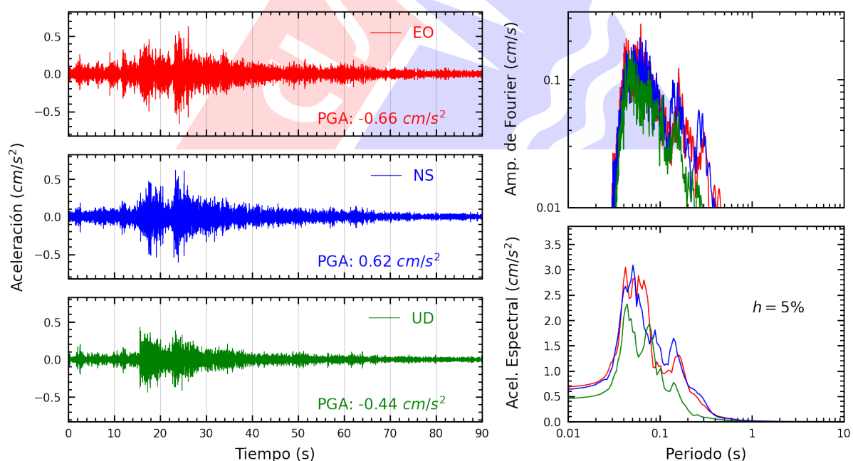
Figura A.20: Registros tiempo-historia, espectros de Fourier y de respuesta en las direcciones EO, NS y vertical de la estación PACHA. Sismo de Chilca, Cañete - Lima del 2025-07-18, 07:13:55 (Hora local)
