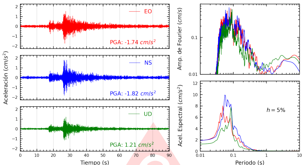
Figura A.3: Registros tiempo-historia, espectros de Fourier y de respuesta en las direcciones EO, NS y vertical de la estación USILM. Sismo de Chilca, Cañete - Lima del 2025-07-18, 07:13:55 (Hora local)
