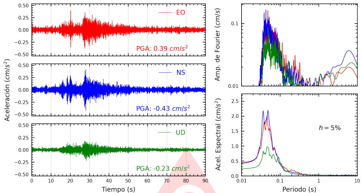
Figura A.29: Registros tiempo-historia, espectros de Fourier y de respuesta en las direcciones EO, NS y vertical de la estación CEPRE. Sismo de Chilca, Cañete - Lima del 2025-07-18, 07:13:55 (Hora local)
