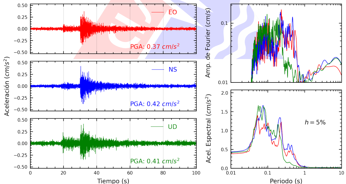
Figura A.30: Registros tiempo-historia, espectros de Fourier y de respuesta en las direcciones EO, NS y vertical de la estación MDPP. Sismo de Chilca, Cañete - Lima del 2025-07-18, 07:13:55 (Hora local)
