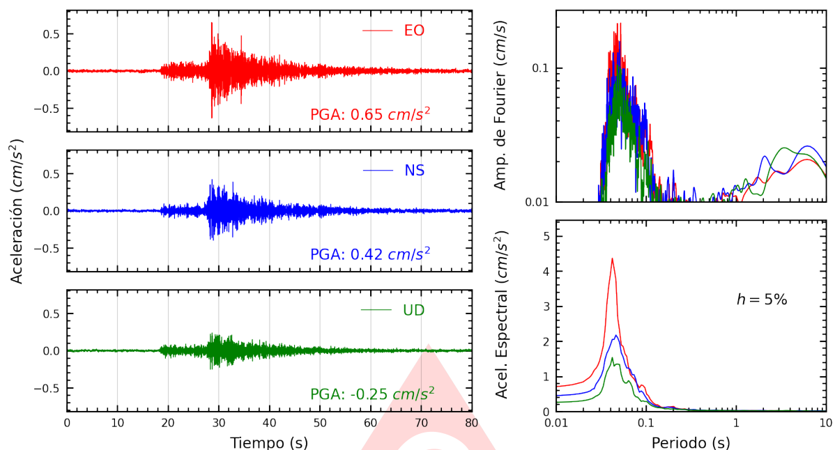
Figura A.21: Registros tiempo-historia, espectros de Fourier y de respuesta en las direcciones EO, NS y vertical de la estación UCSS. Sismo de Chilca, Cañete - Lima del 2025-07-18, 07:13:55 (Hora local)
