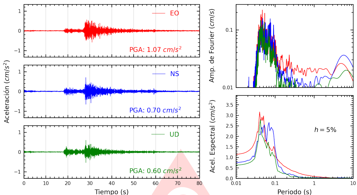
Figura A.11: Registros tiempo-historia, espectros de Fourier y de respuesta en las direcciones EO, NS y vertical de la estación SJLCE. Sismo de Chilca, Cañete - Lima del 2025-07-18, 07:13:55 (Hora local)
