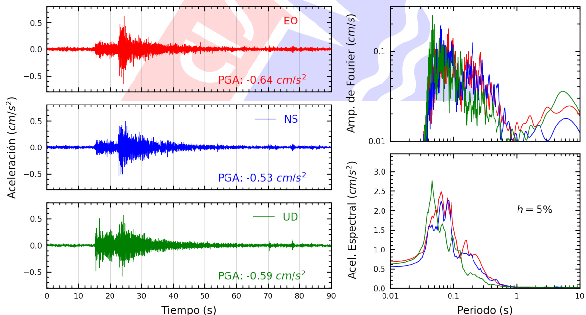
Figura A.22: Registros tiempo-historia, espectros de Fourier y de respuesta en las direcciones EO, NS y vertical de la estación USILP. Sismo de Chilca, Cañete - Lima del 2025-07-18, 07:13:55 (Hora local)
