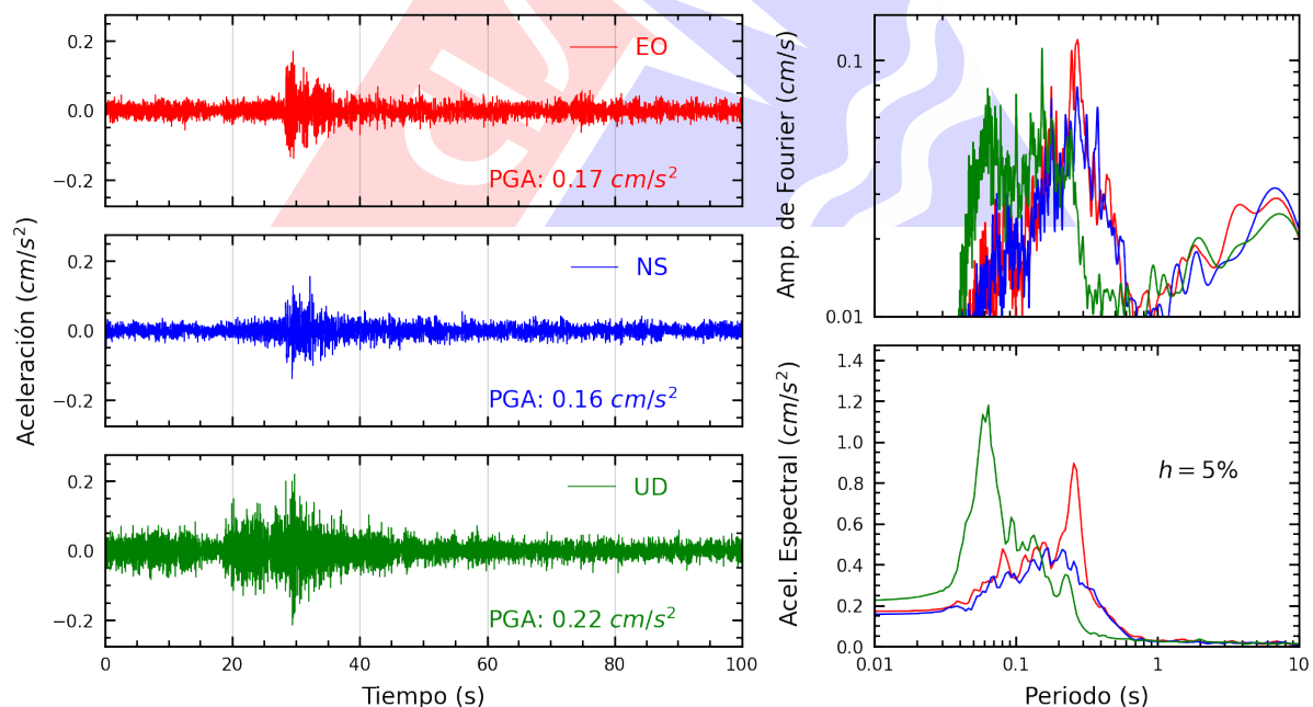
Figura A.32: Registros tiempo-historia, espectros de Fourier y de respuesta en las direcciones EO, NS y vertical de la estación ACAPU. Sismo de Chilca, Cañete - Lima del 2025-07-18, 07:13:55 (Hora local)
