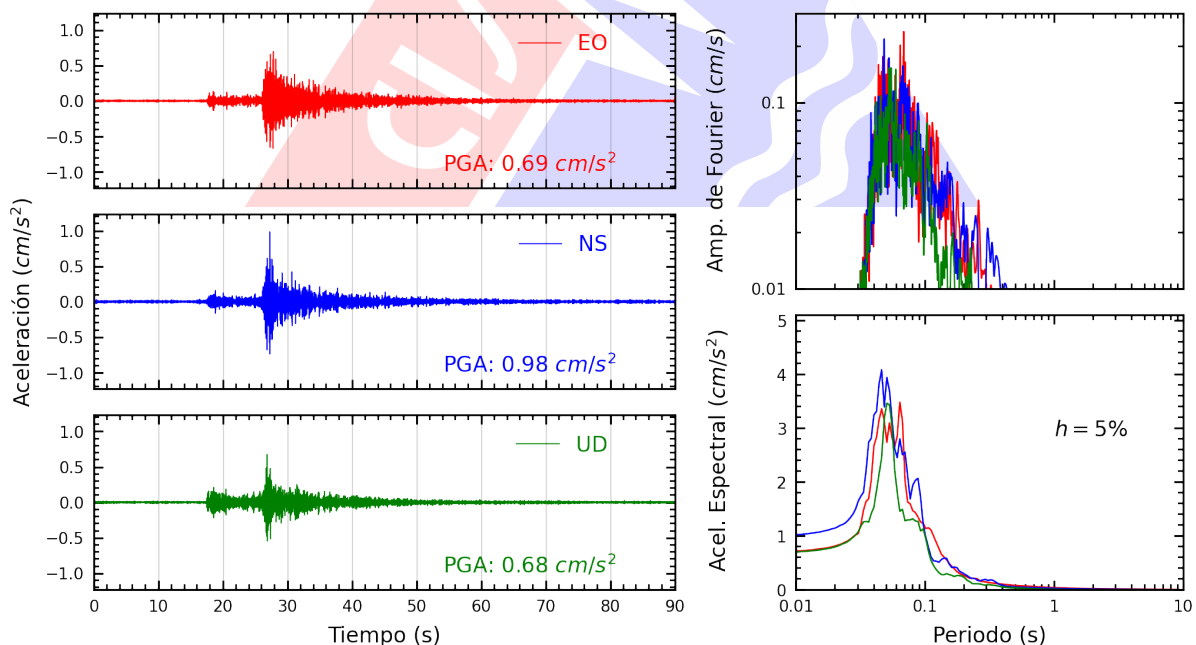
Figura A.12: Registros tiempo-historia, espectros de Fourier y de respuesta en las direcciones EO, NS y vertical de la estación ATARJ. Sismo de Chilca, Cañete - Lima del 2025-07-18, 07:13:55 (Hora local)
