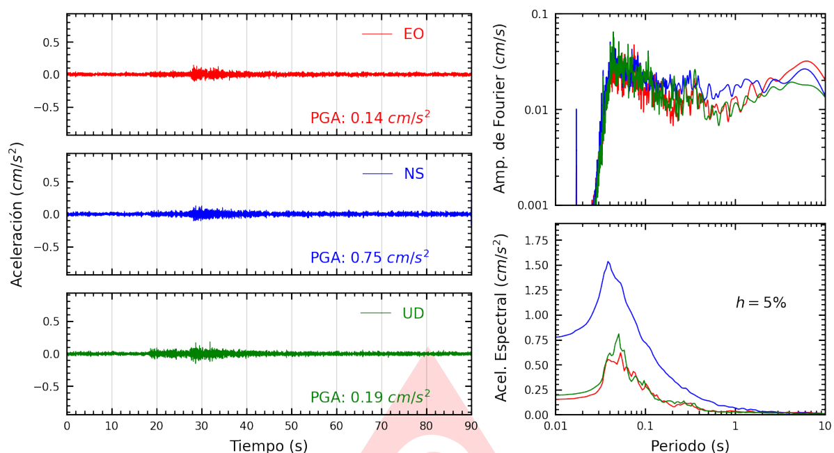
Figura A.17: Registros tiempo-historia, espectros de Fourier y de respuesta en las direcciones EO, NS y vertical de la estación BONDY. Sismo de Chilca, Cañete - Lima del 2025-07-18, 07:13:55 (Hora local)
