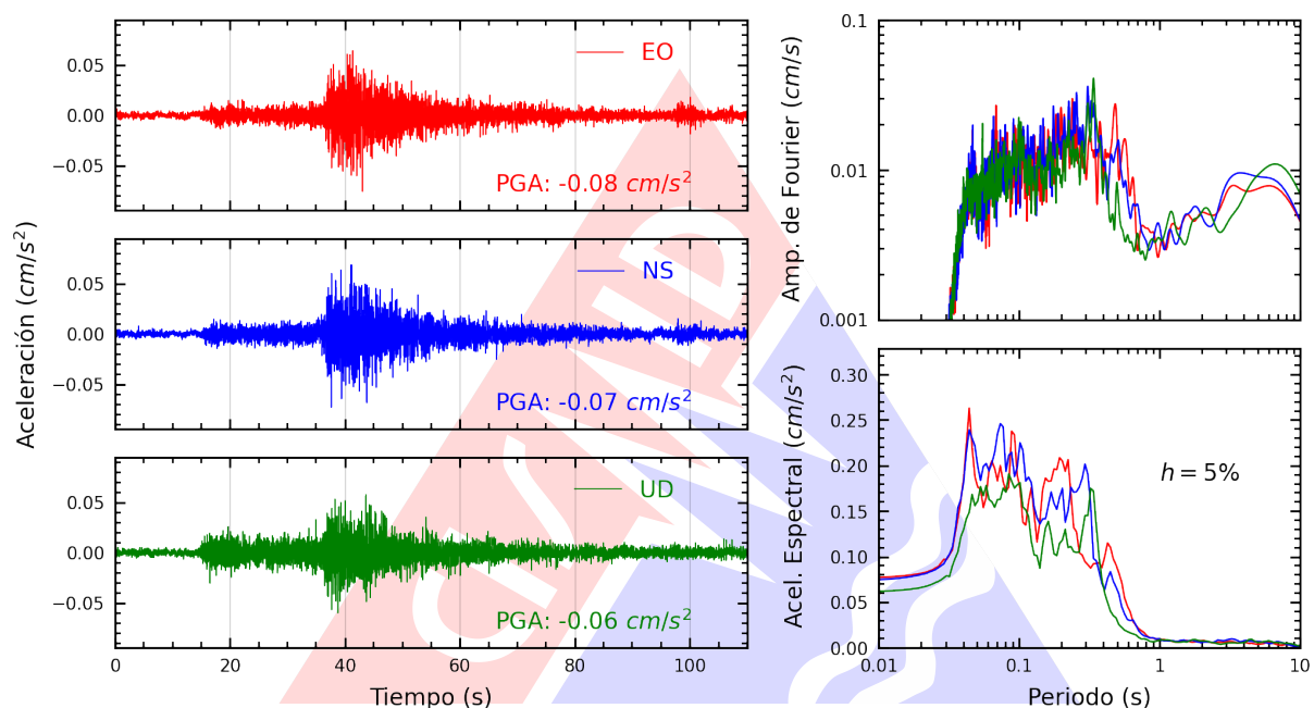
Figura A.35: Registros tiempo-historia, espectros de Fourier y de respuesta en las direcciones EO, NS y vertical de la estación CARAL. Sismo de Chilca, Cañete - Lima del 2025-07-18, 07:13:55 (Hora local)
