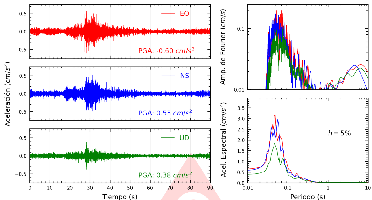
Figura A.25: Registros tiempo-historia, espectros de Fourier y de respuesta en las direcciones EO, NS y vertical de la estación FICPE. Sismo de Chilca, Cañete - Lima del 2025-07-18, 07:13:55 (Hora local)
