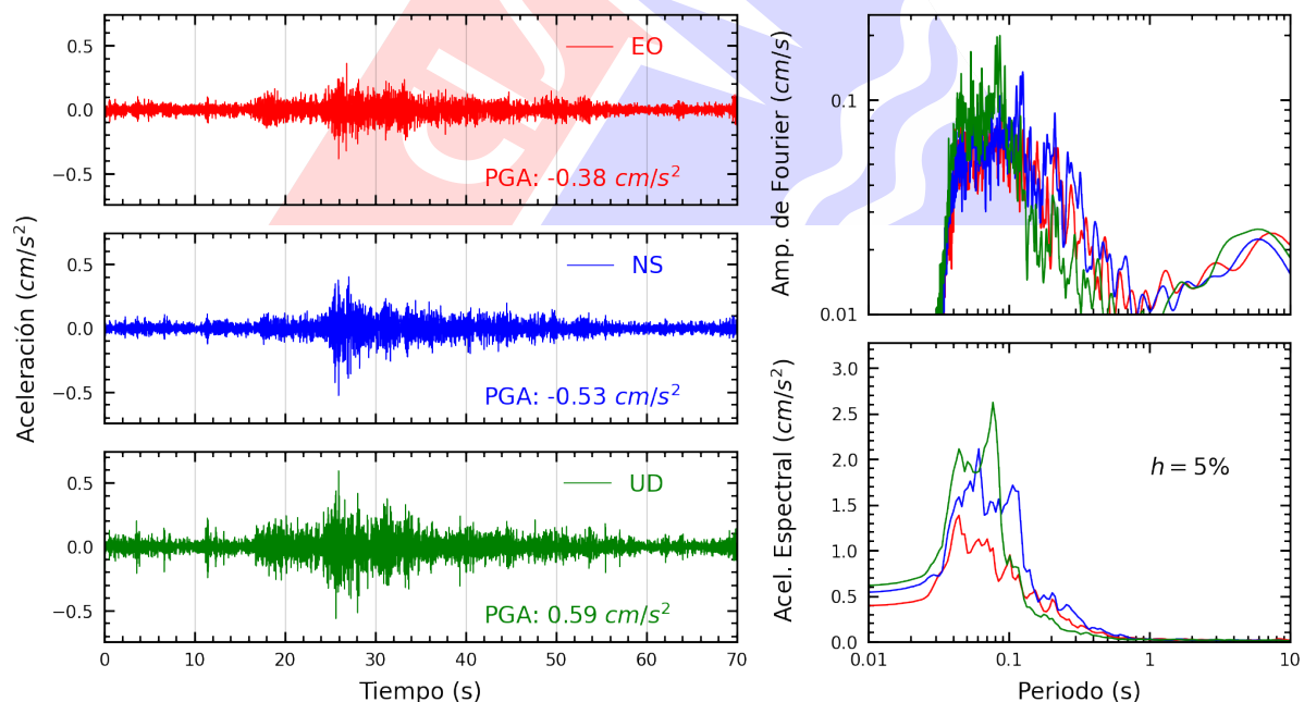
Figura A.26: Registros tiempo-historia, espectros de Fourier y de respuesta en las direcciones EO, NS y vertical de la estación SOCHO. Sismo de Chilca, Cañete - Lima del 2025-07-18, 07:13:55 (Hora local)
