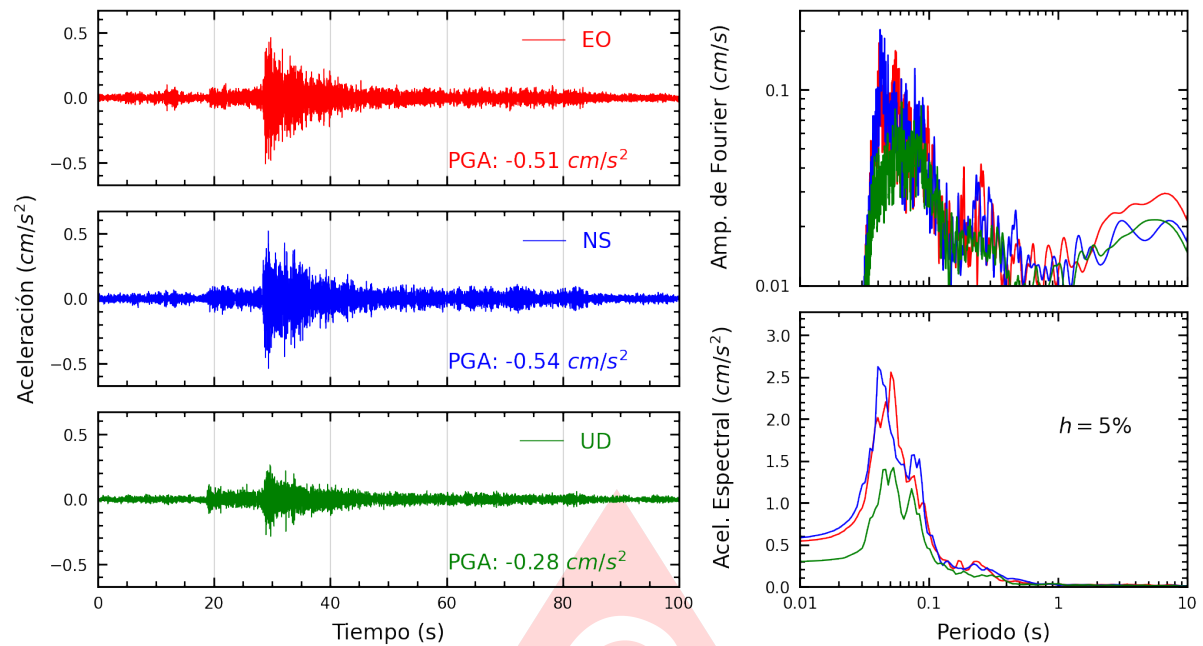
Figura A.27: Registros tiempo-historia, espectros de Fourier y de respuesta en las direcciones EO, NS y vertical de la estación COMAS. Sismo de Chilca, Cañete - Lima del 2025-07-18, 07:13:55 (Hora local)
