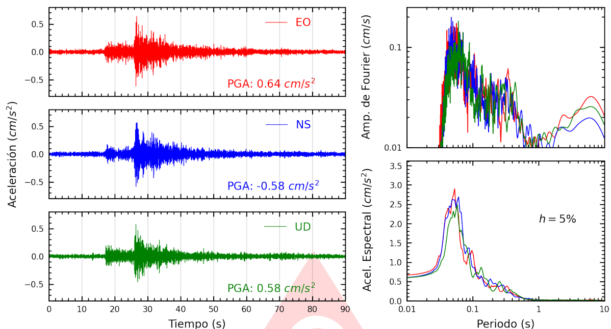
Figura A.23: Registros tiempo-historia, espectros de Fourier y de respuesta en las direcciones EO, NS y vertical de la estación IMCA. Sismo de Chilca, Cañete - Lima del 2025-07-18, 07:13:55 (Hora local)
