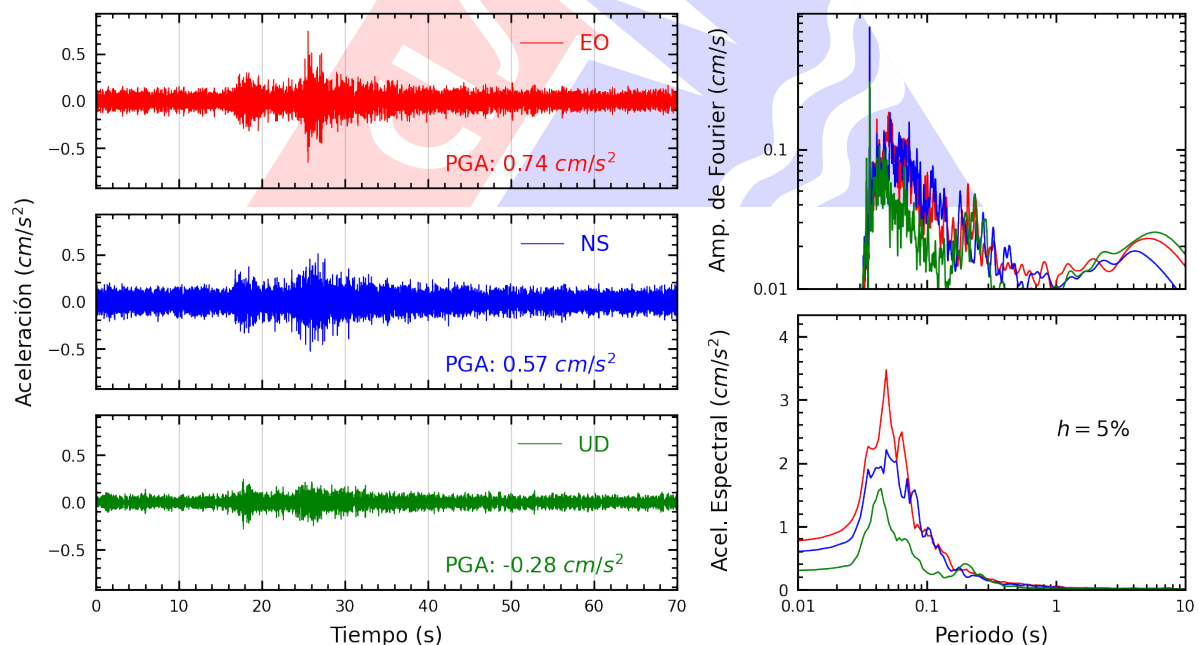
Figura A.18: Registros tiempo-historia, espectros de Fourier y de respuesta en las direcciones EO, NS y vertical de la estación UPCVI. Sismo de Chilca, Cañete - Lima del 2025-07-18, 07:13:55 (Hora local)
