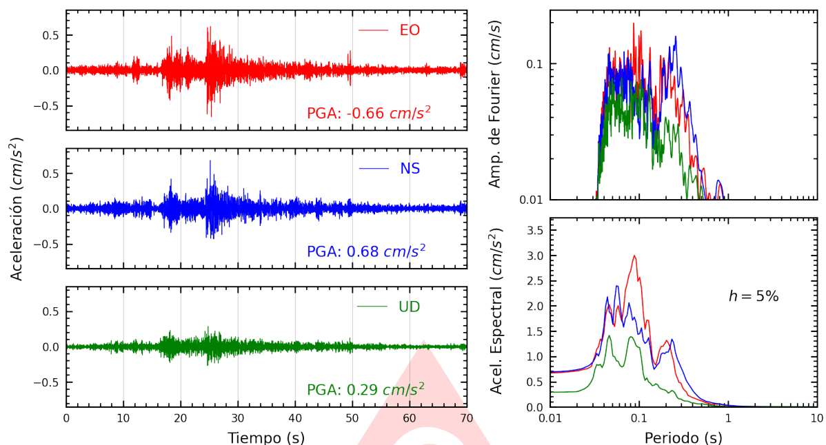
Figura A.19: Registros tiempo-historia, espectros de Fourier y de respuesta en las direcciones EO, NS y vertical de la estación BRISA. Sismo de Chilca, Cañete - Lima del 2025-07-18, 07:13:55 (Hora local)
