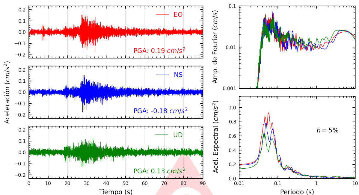
Figura A.33: Registros tiempo-historia, espectros de Fourier y de respuesta en las direcciones EO, NS y vertical de la estación UNFV. Sismo de Chilca, Cañete - Lima del 2025-07-18, 07:13:55 (Hora local)
