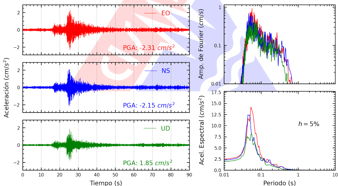
Figura A.2: Registros tiempo-historia, espectros de Fourier y de respuesta en las direcciones EO, NS y vertical de la estación UNTEL. Sismo de Chilca, Cañete - Lima del 2025-07-18, 07:13:55 (Hora local)
