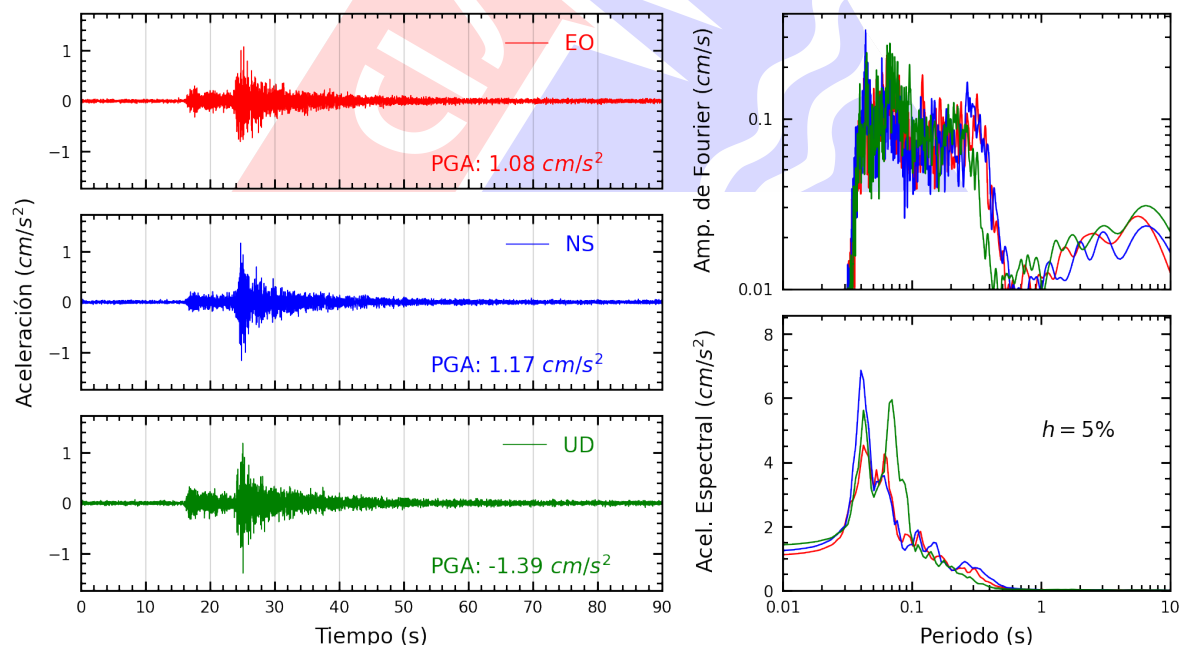
Figura A.8: Registros tiempo-historia, espectros de Fourier y de respuesta en las direcciones EO, NS y vertical de la estación SOVES. Sismo de Chilca, Cañete - Lima del 2025-07-18, 07:13:55 (Hora local)
