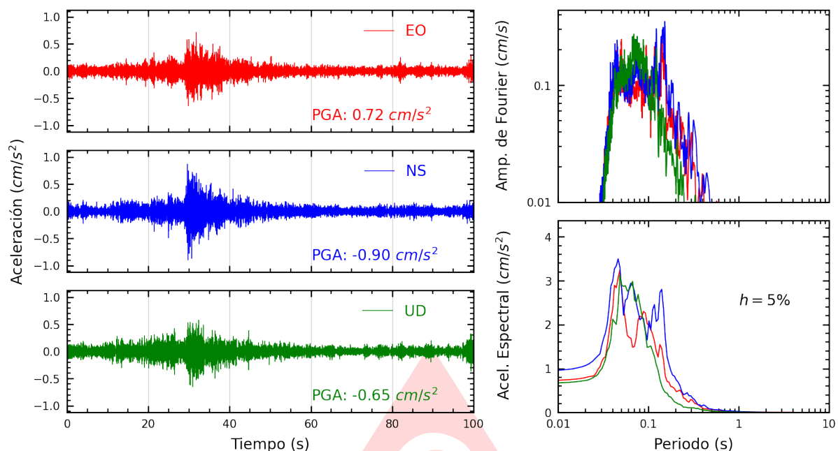
Figura A.15: Registros tiempo-historia, espectros de Fourier y de respuesta en las direcciones EO, NS y vertical de la estación CARAB. Sismo de Chilca, Cañete - Lima del 2025-07-18, 07:13:55 (Hora local)
