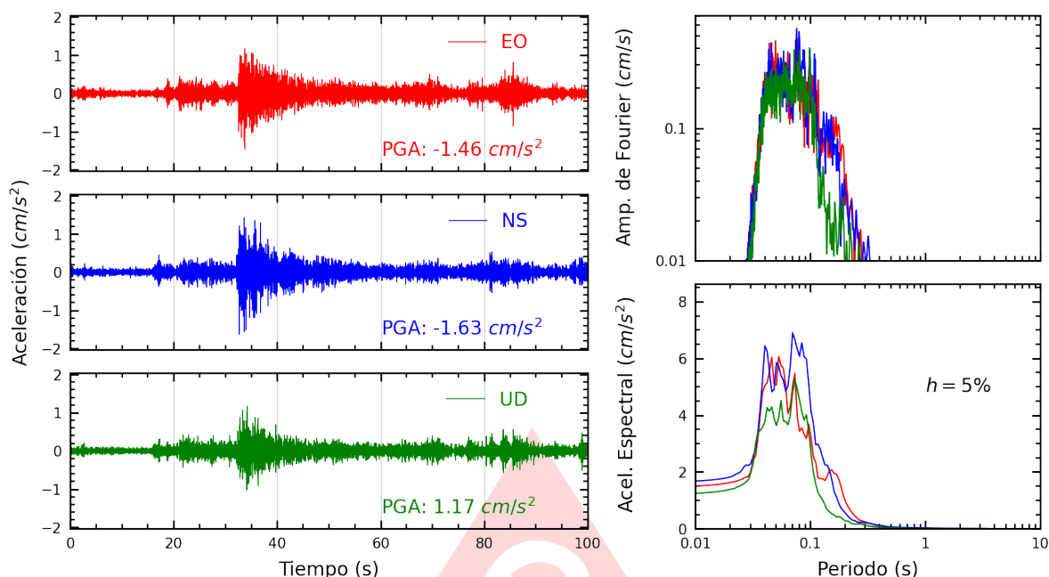
Figura A.5: Registros tiempo-historia, espectros de Fourier y de respuesta en las direcciones EO, NS y vertical de la estación SROSA. Sismo de Chilca, Cañete - Lima del 2025-07-18, 07:13:55 (Hora local)
