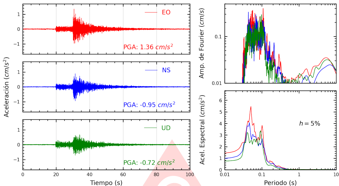
Figura A.9: Registros tiempo-historia, espectros de Fourier y de respuesta en las direcciones EO, NS y vertical de la estación AMORE. Sismo de Chilca, Cañete - Lima del 2025-07-18, 07:13:55 (Hora local)
