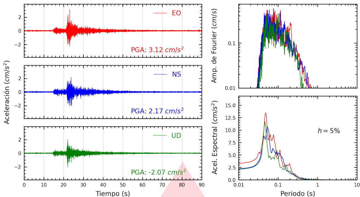
Figura A.1: Registros tiempo-historia, espectros de Fourier y de respuesta en las direcciones EO, NS y vertical de la estación PHERM. Sismo de Chilca, Cañete - Lima del 2025-07-18, 07:13:55 (Hora local)
