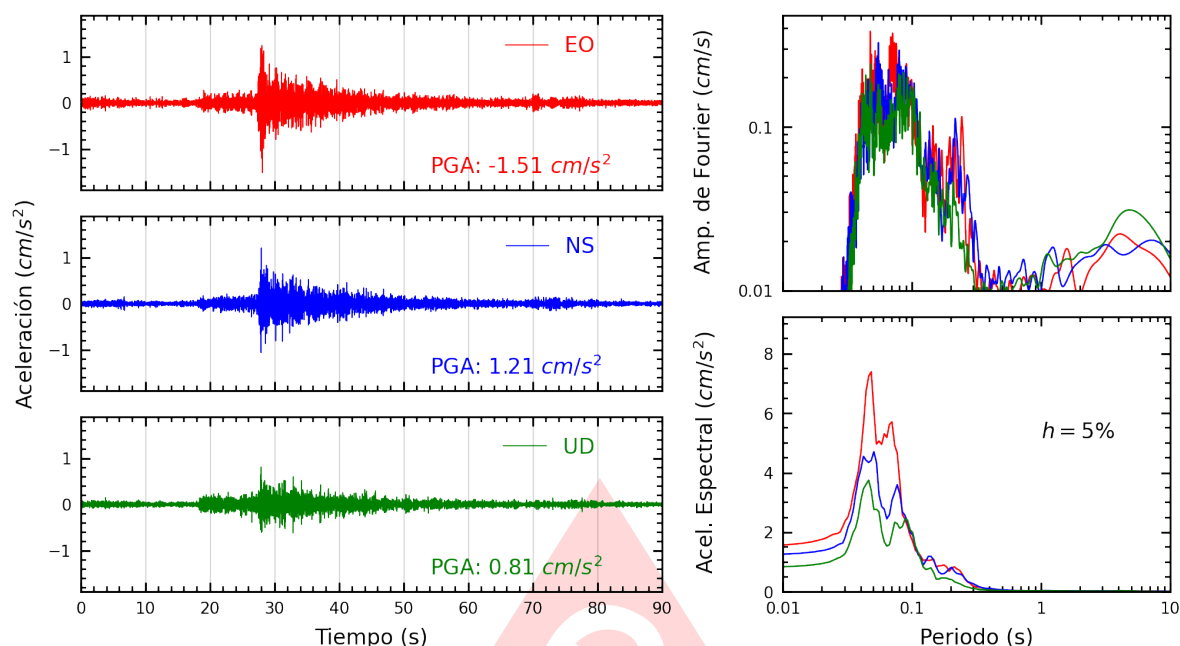
Figura A.7: Registros tiempo-historia, espectros de Fourier y de respuesta en las direcciones EO, NS y vertical de la estación INDEP. Sismo de Chilca, Cañete - Lima del 2025-07-18, 07:13:55 (Hora local)
