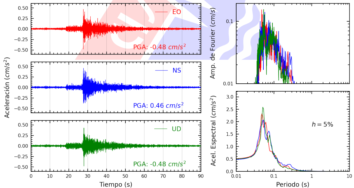
Figura A.28: Registros tiempo-historia, espectros de Fourier y de respuesta en las direcciones EO, NS y vertical de la estación JALV2. Sismo de Chilca, Cañete - Lima del 2025-07-18, 07:13:55 (Hora local)
