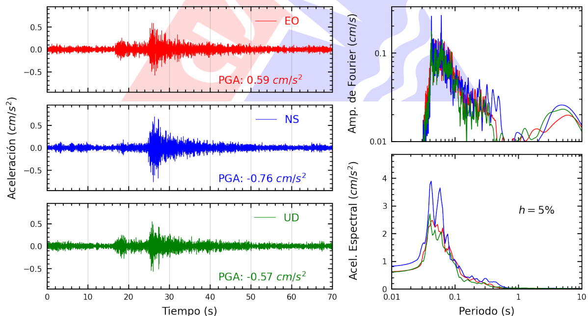
Figura A.16: Registros tiempo-historia, espectros de Fourier y de respuesta en las direcciones EO, NS y vertical de la estación URPPE. Sismo de Chilca, Cañete - Lima del 2025-07-18, 07:13:55 (Hora local)
