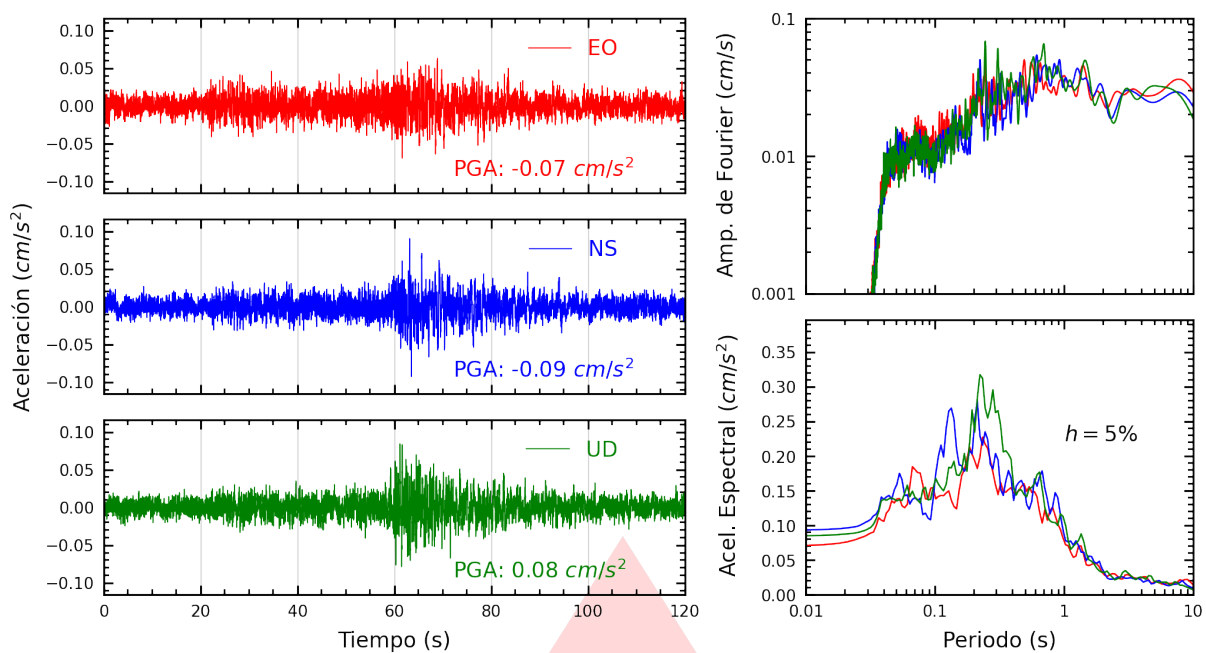
Figura A.1: Registros tiempo-historia, espectros de Fourier y de respuesta en las direcciones EO, NS y vertical de la estación UNSCH. Sismo de Atalaya, Atalaya - Ucayali del 2025-07-18, 19:30:00 (Hora local)
