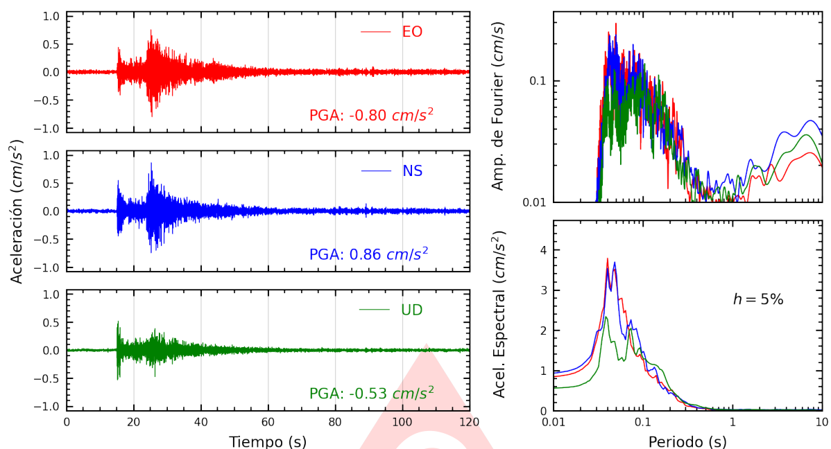
Figura A.29: Registros tiempo-historia, espectros de Fourier y de respuesta en las direcciones EO, NS y vertical de la estación CEPRE. Sismo de Provincia Constitucional del Callao , Callao - Lima del 2025-07-24, 22:18:22 (Hora local)
