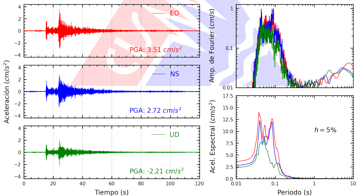
Figura A.2: Registros tiempo-historia, espectros de Fourier y de respuesta en las direcciones EO, NS y vertical de la estación JOSEO. Sismo de Provincia Constitucional del Callao , Callao - Lima del 2025-07-24, 22:18:22 (Hora local)
