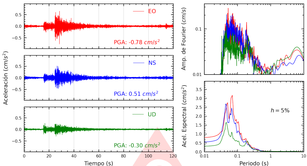
Figura A.31: Registros tiempo-historia, espectros de Fourier y de respuesta en las direcciones EO, NS y vertical de la estación UPCVI. Sismo de Provincia Constitucional del Callao , Callao - Lima del 2025-07-24, 22:18:22 (Hora local)
