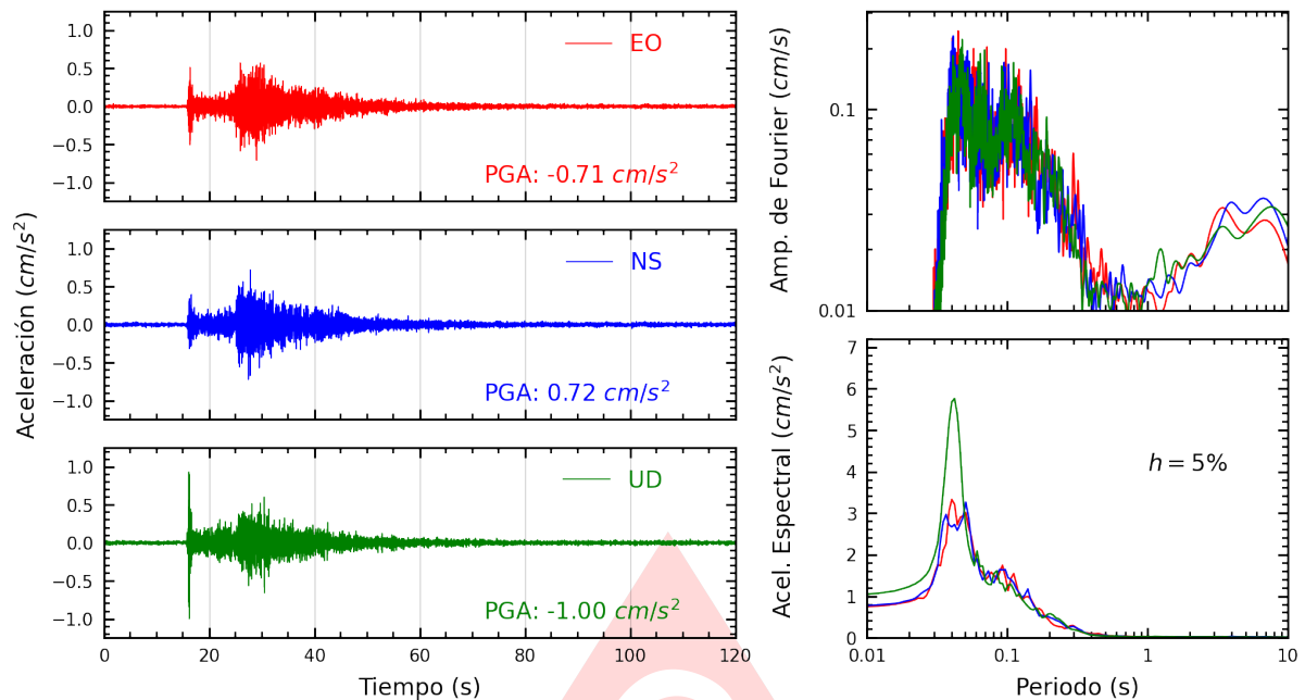
Figura A.27: Registros tiempo-historia, espectros de Fourier y de respuesta en las direcciones EO, NS y vertical de la estación USMP. Sismo de Provincia Constitucional del Callao , Callao - Lima del 2025-07-24, 22:18:22 (Hora local)
