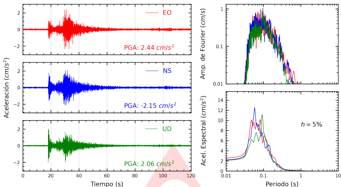
Figura A.7: Registros tiempo-historia, espectros de Fourier y de respuesta en las direcciones EO, NS y vertical de la estación PHERM. Sismo de Provincia Constitucional del Callao , Callao - Lima del 2025-07-24, 22:18:22 (Hora local)
