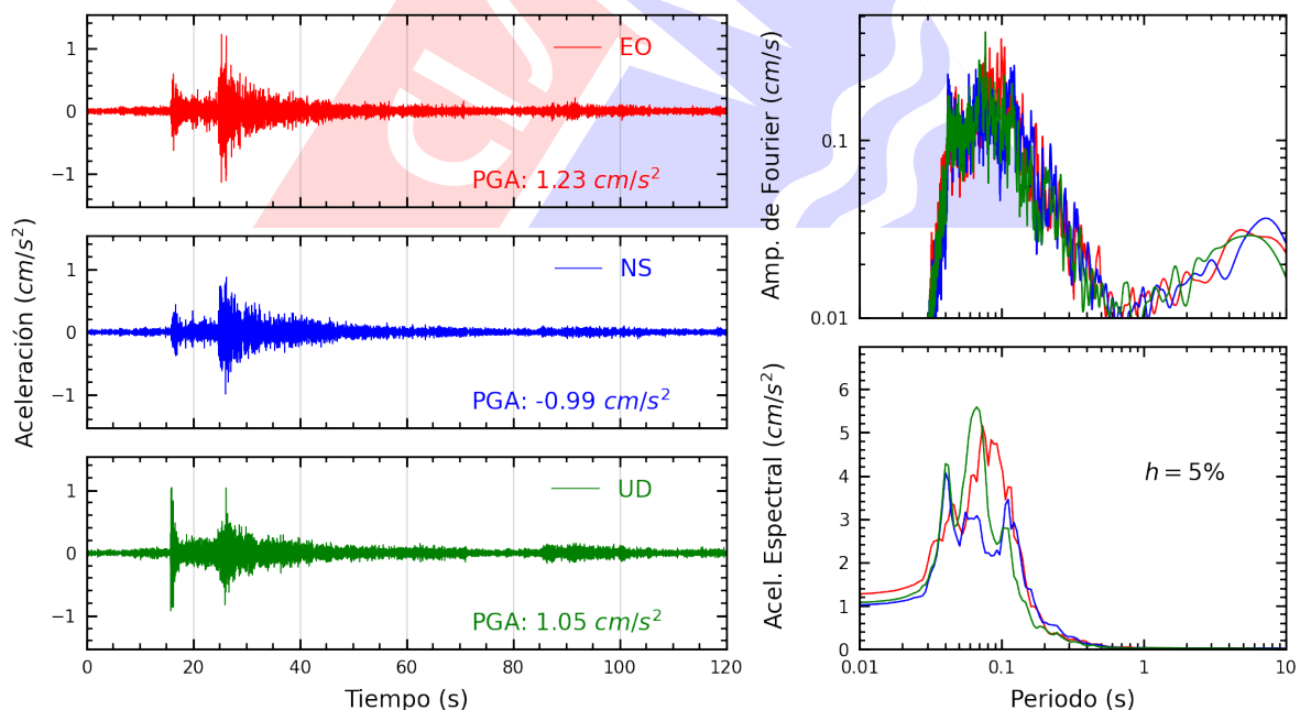
Figura A.24: Registros tiempo-historia, espectros de Fourier y de respuesta en las direcciones EO, NS y vertical de la estación URPE. Sismo de Provincia Constitucional del Callao, Callao - Lima del 2025-07-24, 22:18:22 (Hora local)
