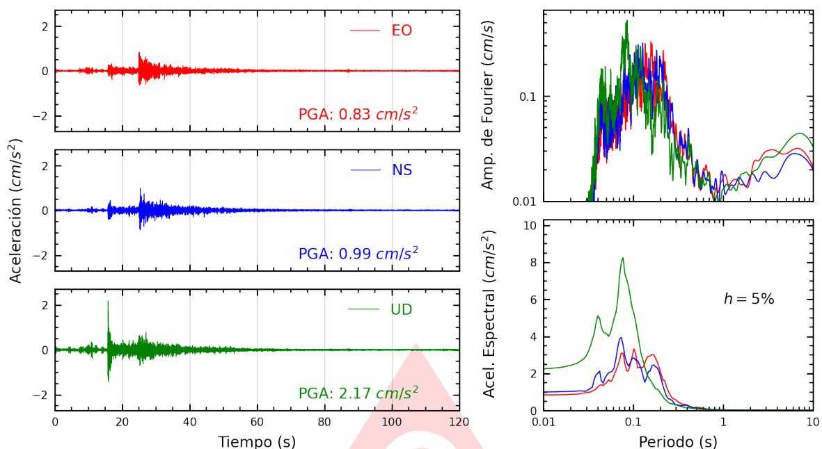
Figura A.9: Registros tiempo-historia, espectros de Fourier y de respuesta en las direcciones EO, NS y vertical de la estación SOCHO. Sismo de Provincia Constitucional del Callao , Callao - Lima del 2025-07-24, 22:18:22 (Hora local)
