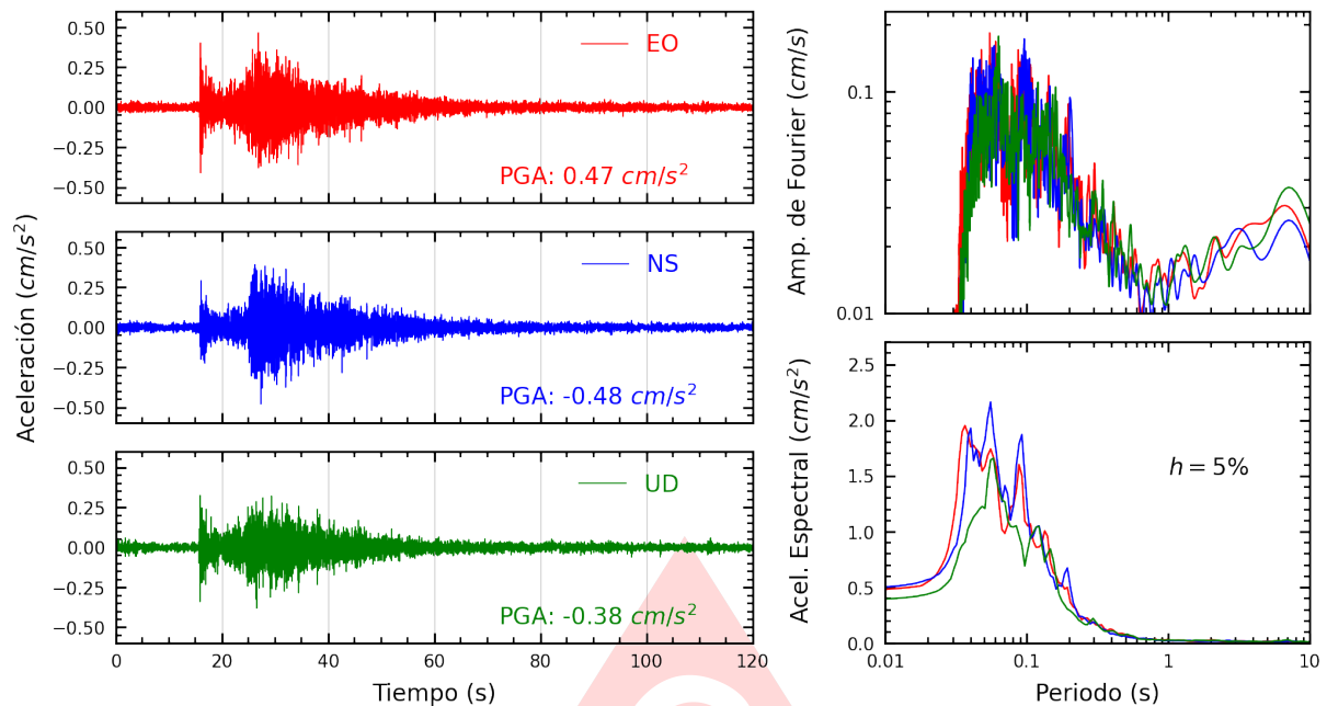
Figura A.37: Registros tiempo-historia, espectros de Fourier y de respuesta en las direcciones EO, NS y vertical de la estación IMCA. Sismo de Provincia Constitucional del Callao , Callao - Lima del 2025-07-24, 22:18:22 (Hora local)
