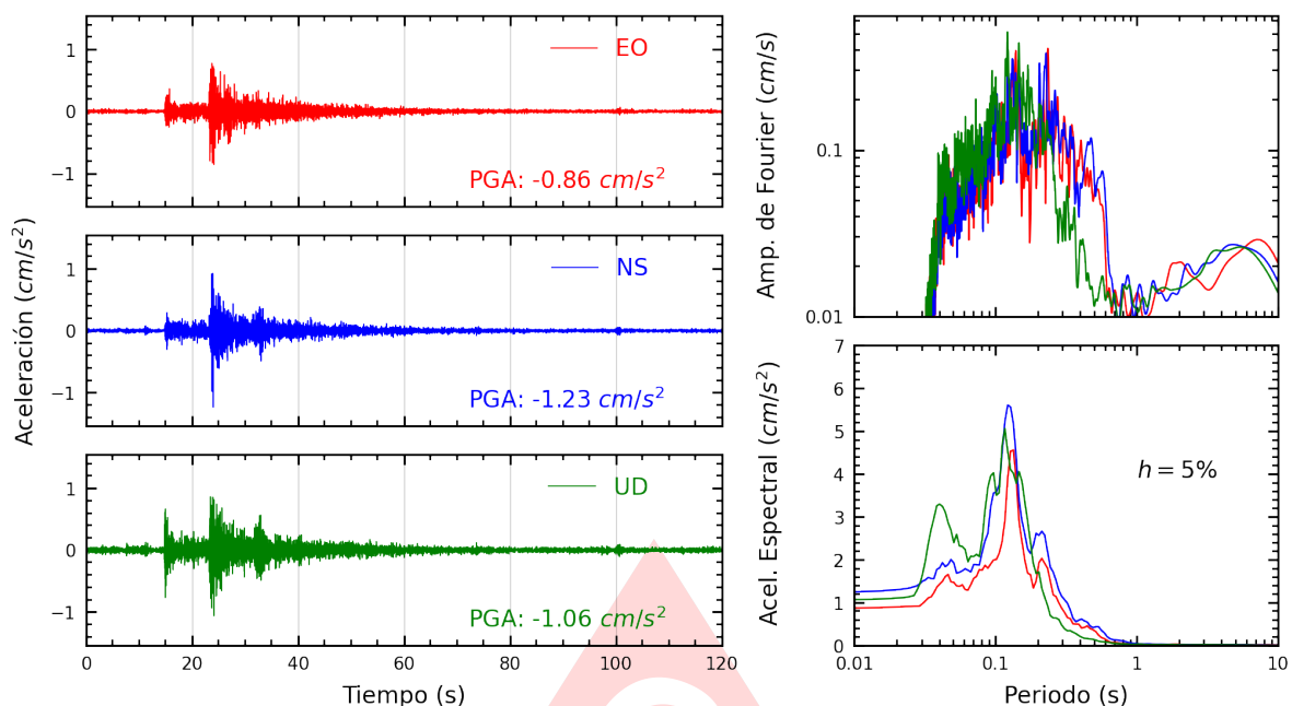
Figura A.23: Registros tiempo-historia, espectros de Fourier y de respuesta en las direcciones EO, NS y vertical de la estación MDP. Sismo de Provincia Constitucional del Callao, Callao - Lima del 2025-07-24, 22:18:22 (Hora local)
