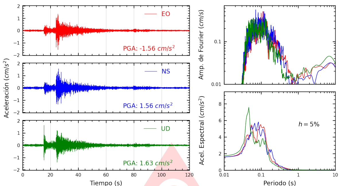
Figura A.17: Registros tiempo-historia, espectros de Fourier y de respuesta en las direcciones EO, NS y vertical de la estación SJLSC. Sismo de Provincia Constitucional del Callao , Callao - Lima del 2025-07-24, 22:18:22 (Hora local)
