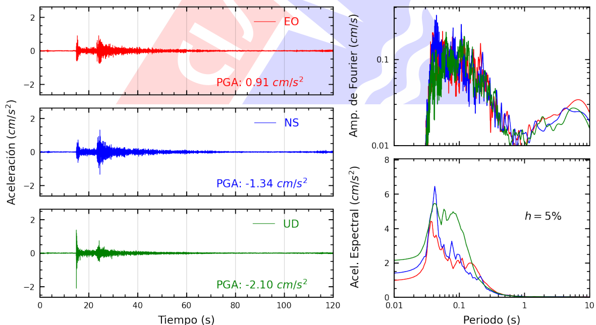
Figura A.10: Registros tiempo-historia, espectros de Fourier y de respuesta en las direcciones EO, NS y vertical de la estación COMAS. Sismo de Provincia Constitucional del Callao , Callao - Lima del 2025-07-24, 22:18:22 (Hora local)
