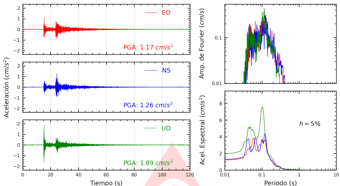
Figura A.13: Registros tiempo-historia, espectros de Fourier y de respuesta en las direcciones EO, NS y vertical de la estación JALV2. Sismo de Provincia Constitucional del Callao , Callao - Lima del 2025-07-24, 22:18:22 (Hora local)
