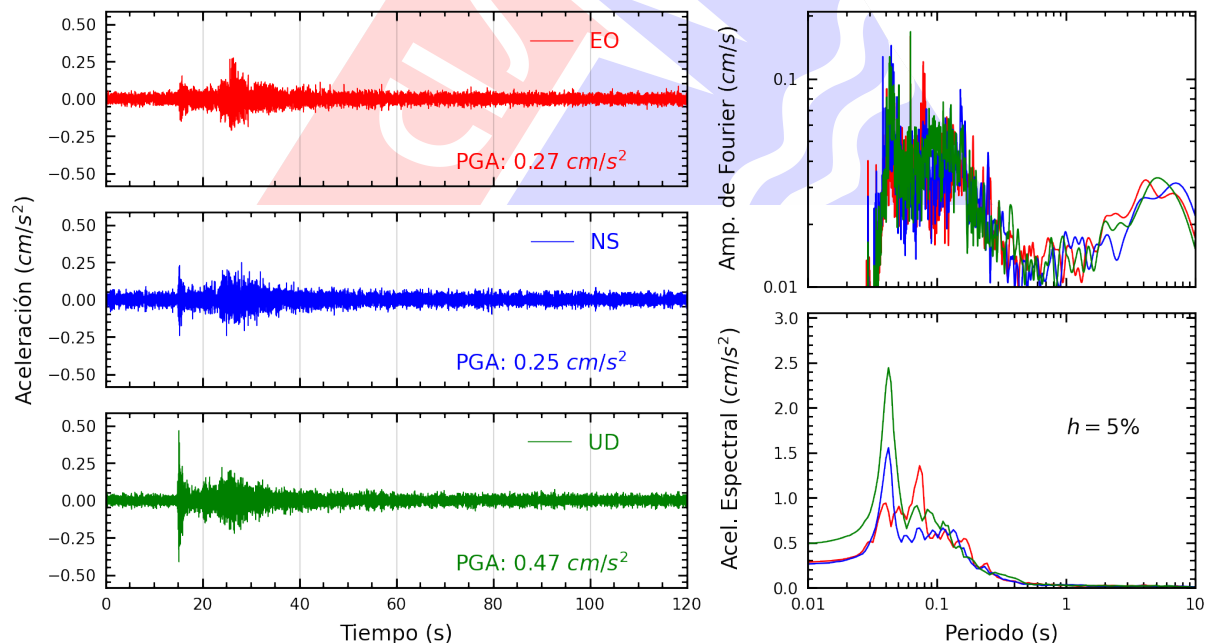
Figura A.38: Registros tiempo-historia, espectros de Fourier y de respuesta en las direcciones EO, NS y vertical de la estación BONDY. Sismo de Provincia Constitucional del Callao , Callao - Lima del 2025-07-24, 22:18:22 (Hora local)
