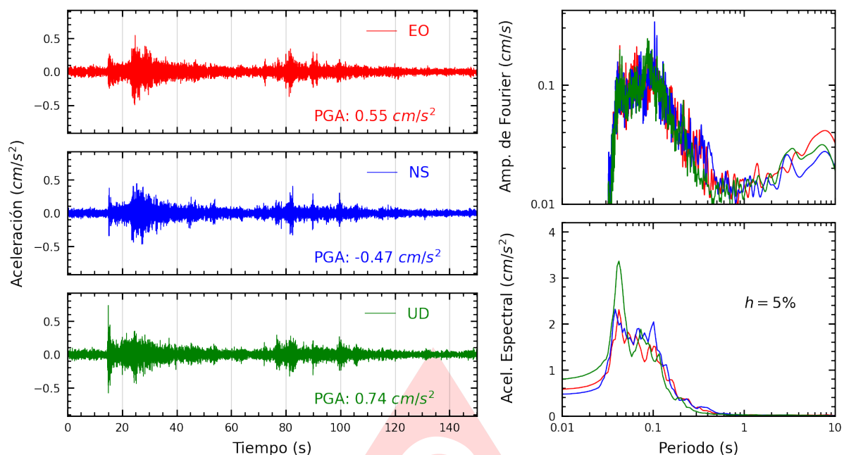
Figura A.33: Registros tiempo-historia, espectros de Fourier y de respuesta en las direcciones EO, NS y vertical de la estación MADRE. Sismo de Provincia Constitucional del Callao , Callao - Lima del 2025-07-24, 22:18:22 (Hora local)
