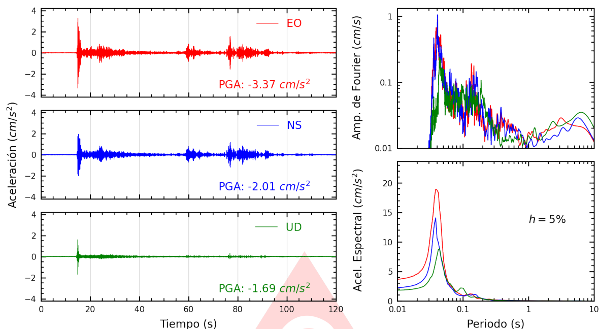
Figura A.3: Registros tiempo-historia, espectros de Fourier y de respuesta en las direcciones EO, NS y vertical de la estación DHNPE. Sismo de Provincia Constitucional del Callao , Callao - Lima del 2025-07-24, 22:18:22 (Hora local)
