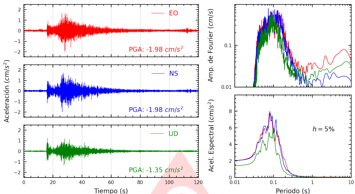
Figura A.11: Registros tiempo-historia, espectros de Fourier y de respuesta en las direcciones EO, NS y vertical de la estación USILM. Sismo de Provincia Constitucional del Callao , Callao - Lima del 2025-07-24, 22:18:22 (Hora local)
