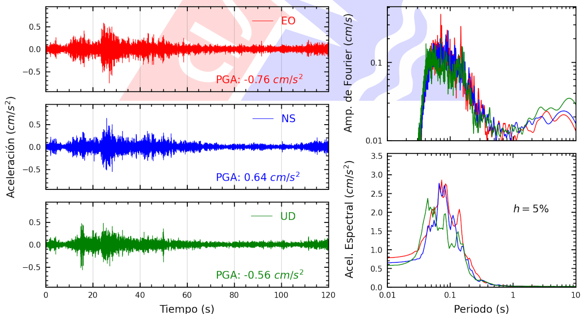
Figura A.32: Registros tiempo-historia, espectros de Fourier y de respuesta en las direcciones EO, NS y vertical de la estación UPCSM. Sismo de Provincia Constitucional del Callao , Callao - Lima del 2025-07-24, 22:18:22 (Hora local)
