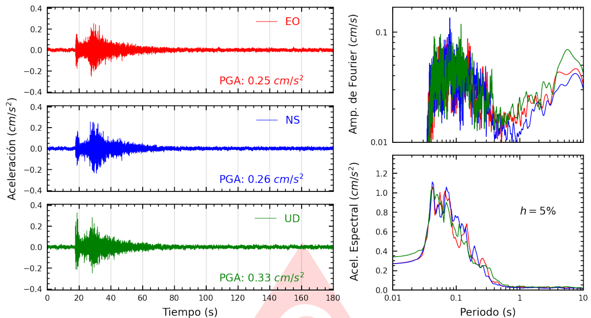
Figura A.41: Registros tiempo-historia, espectros de Fourier y de respuesta en las direcciones EO, NS y vertical de la estación UNMSM. Sismo de Provincia Constitucional del Callao , Callao - Lima del 2025-07-24, 22:18:22 (Hora local)
