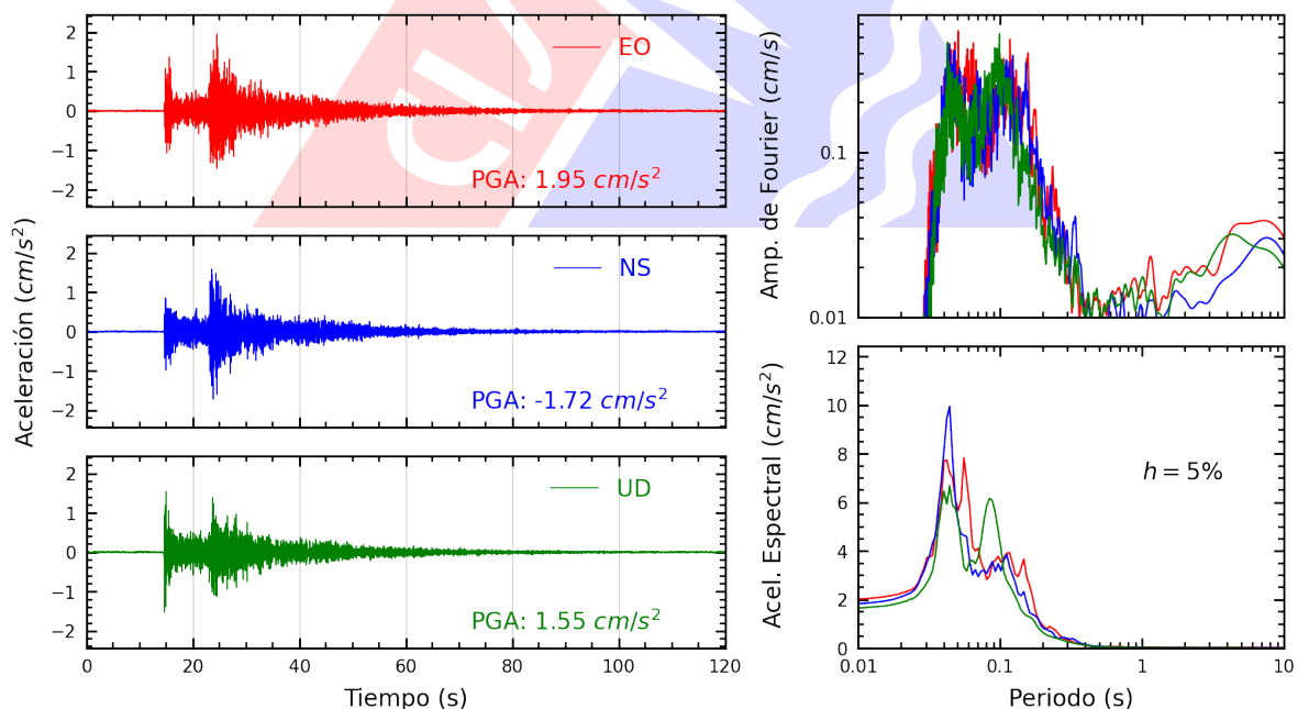
Figura A.12: Registros tiempo-historia, espectros de Fourier y de respuesta en las direcciones EO, NS y vertical de la estación AMORE. Sismo de Provincia Constitucional del Callao , Callao - Lima del 2025-07-24, 22:18:22 (Hora local)
