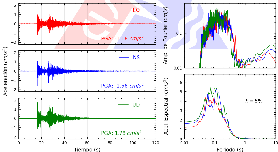
Figura A.16: Registros tiempo-historia, espectros de Fourier y de respuesta en las direcciones EO, NS y vertical de la estación SOVES. Sismo de Provincia Constitucional del Callao , Callao - Lima del 2025-07-24, 22:18:22 (Hora local)
