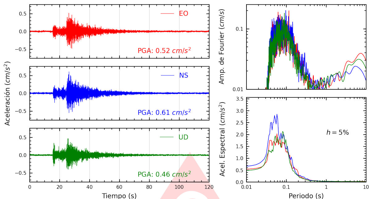
Figura A.35: Registros tiempo-historia, espectros de Fourier y de respuesta en las direcciones EO, NS y vertical de la estación SERVI. Sismo de Provincia Constitucional del Callao , Callao - Lima del 2025-07-24, 22:18:22 (Hora local)
