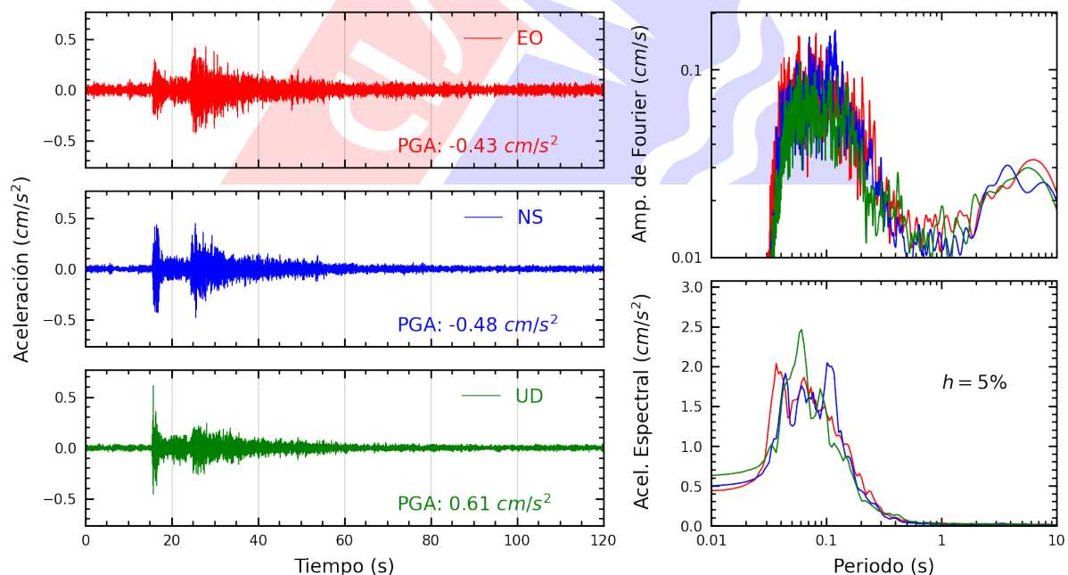
Figura A.34: Registros tiempo-historia, espectros de Fourier y de respuesta en las direcciones EO, NS y vertical de la estación INICT. Sismo de Provincia Constitucional del Callao , Callao - Lima del 2025-07-24, 22:18:22 (Hora local)
