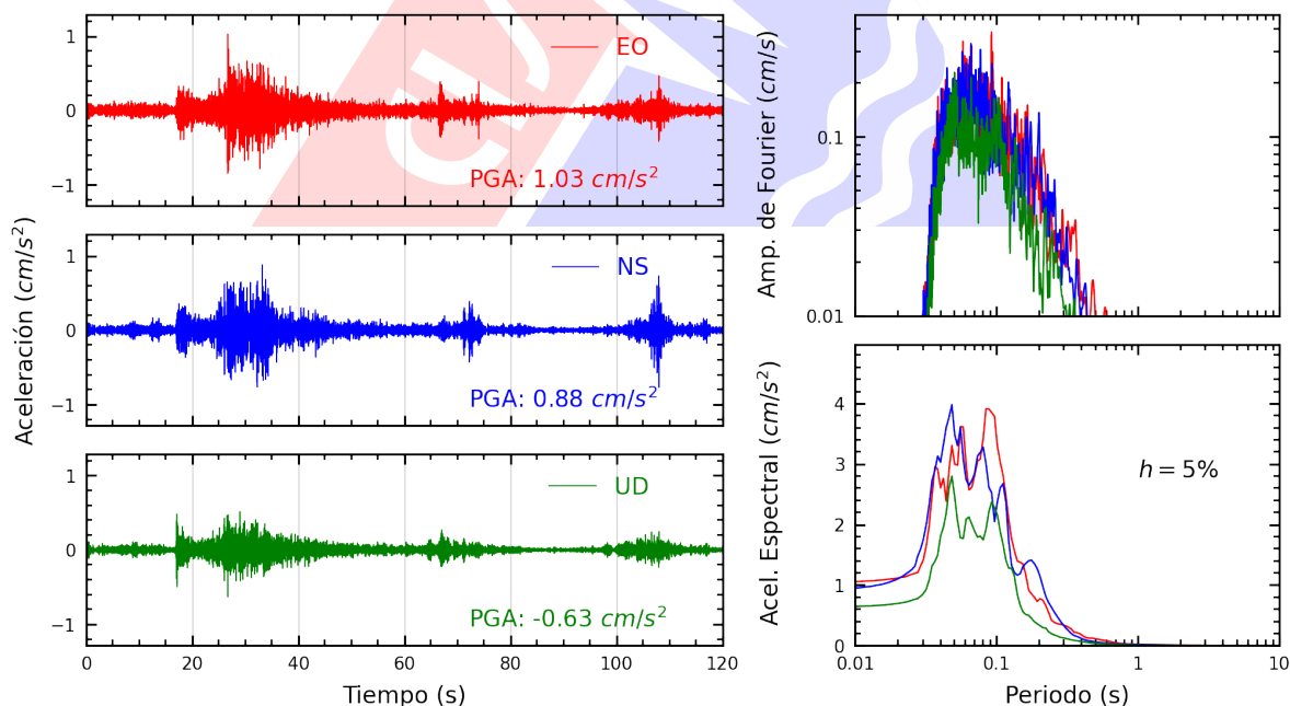
Figura A.26: Registros tiempo-historia, espectros de Fourier y de respuesta en las direcciones EO, NS y vertical de la estación PACHA. Sismo de Provincia Constitucional del Callao, Callao - Lima del 2025-07-24, 22:18:22 (Hora local)
