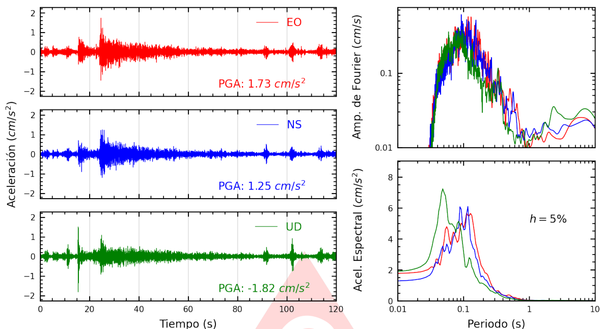
Figura A.15: Registros tiempo-historia, espectros de Fourier y de respuesta en las direcciones EO, NS y vertical de la estación SJLSV. Sismo de Provincia Constitucional del Callao , Callao - Lima del 2025-07-24, 22:18:22 (Hora local)
