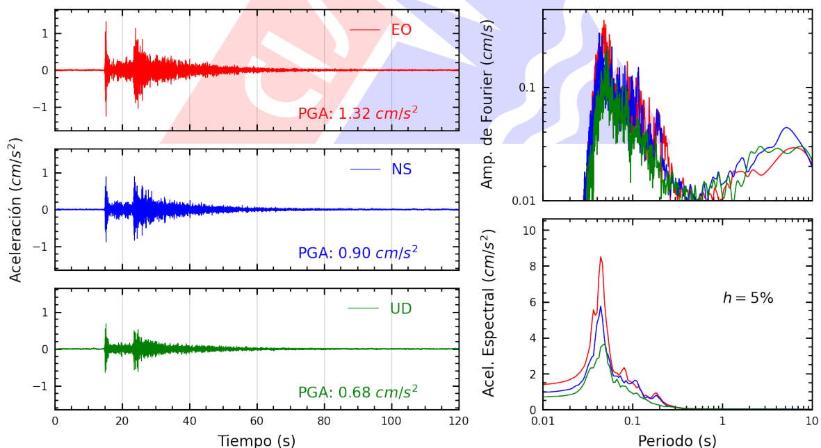
Figura A.22: Registros tiempo-historia, espectros de Fourier y de respuesta en las direcciones EO, NS y vertical de la estación UCSS. Sismo de Provincia Constitucional del Callao , Callao - Lima del 2025-07-24, 22:18:22 (Hora local)
