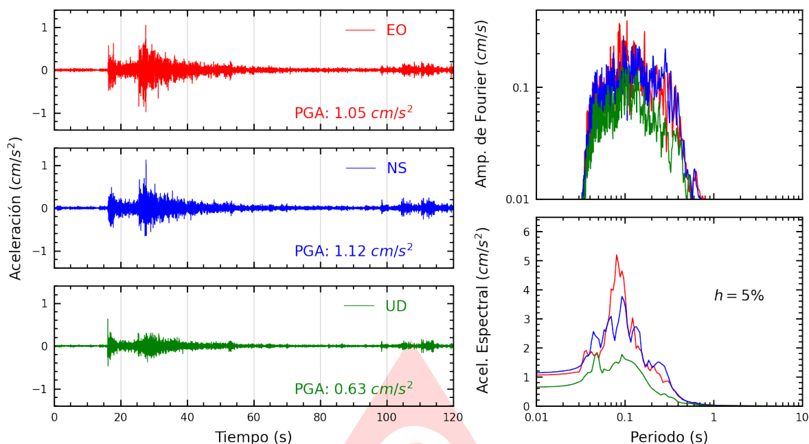
Figura A.25: Registros tiempo-historia, espectros de Fourier y de respuesta en las direcciones EO, NS y vertical de la estación BRISA. Sismo de Provincia Constitucional del Callao, Callao - Lima del 2025-07-24, 22:18:22 (Hora local)
