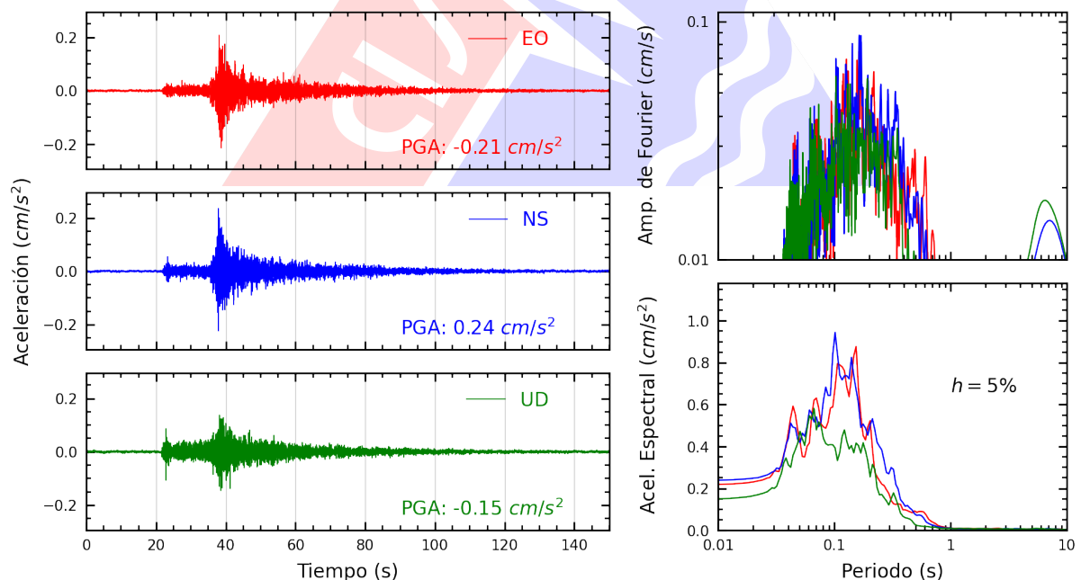
Figura A.42: Registros tiempo-historia, espectros de Fourier y de respuesta en las direcciones EO, NS y vertical de la estación CARAL. Sismo de Provincia Constitucional del Callao , Callao - Lima del 2025-07-24, 22:18:22 (Hora local)
