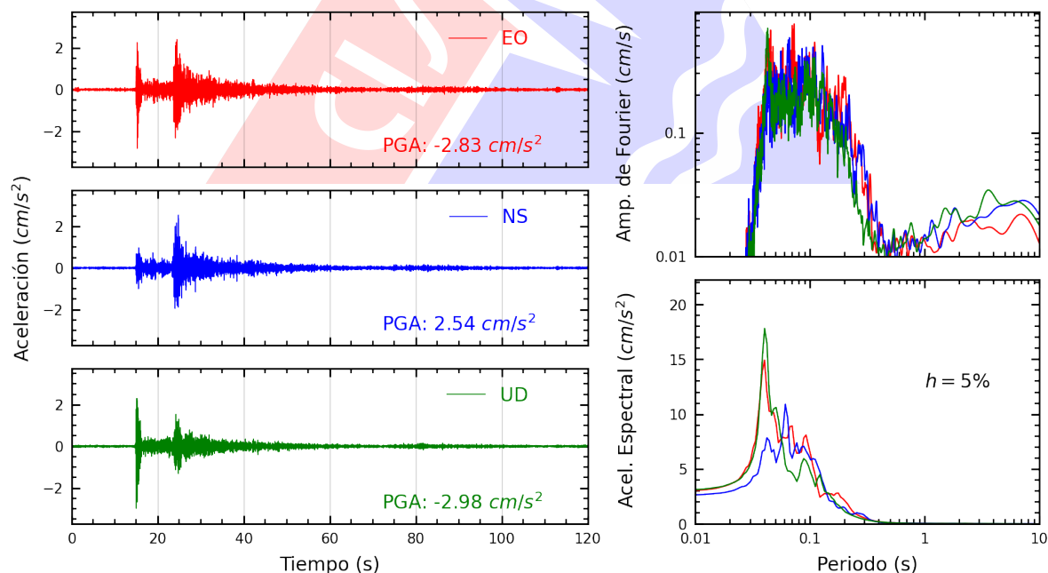
Figura A.4: Registros tiempo-historia, espectros de Fourier y de respuesta en las direcciones EO, NS y vertical de la estación INDEP. Sismo de Provincia Constitucional del Callao , Callao - Lima del 2025-07-24, 22:18:22 (Hora local)
