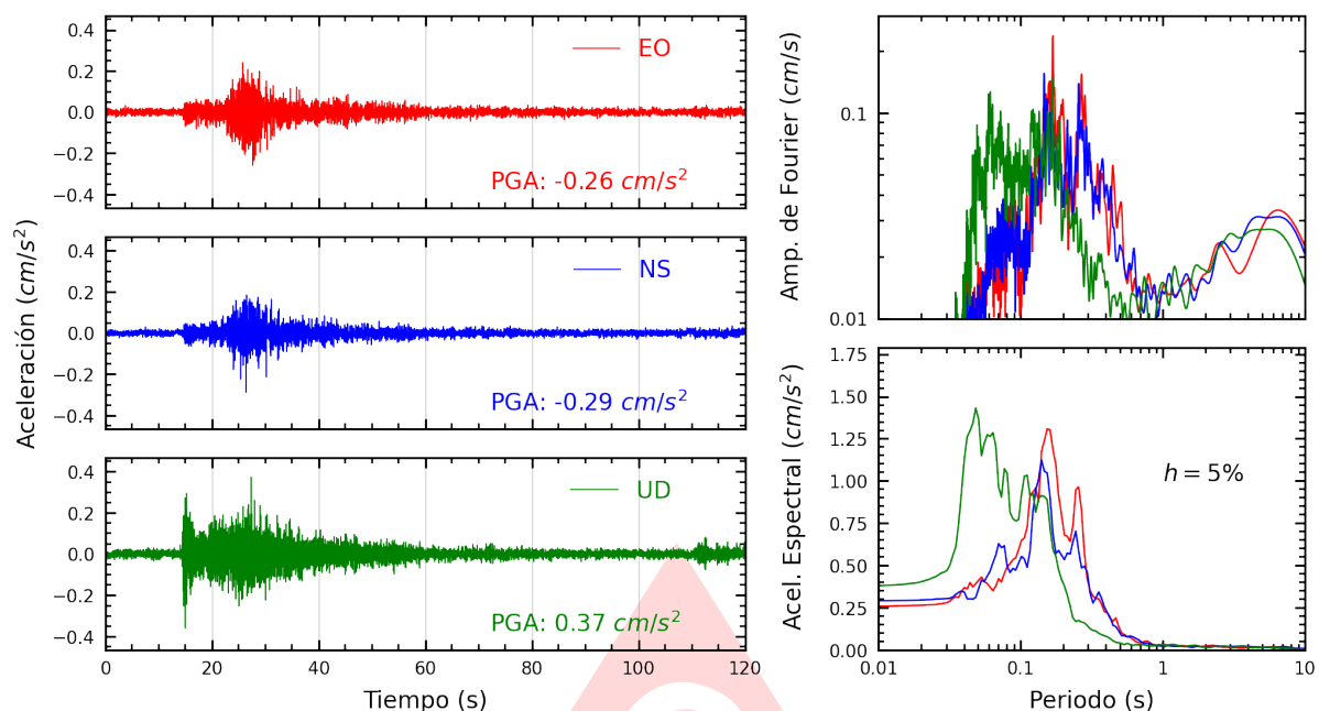
Figura A.39: Registros tiempo-historia, espectros de Fourier y de respuesta en las direcciones EO, NS y vertical de la estación ACAPU. Sismo de Provincia Constitucional del Callao , Callao - Lima del 2025-07-24, 22:18:22 (Hora local)
