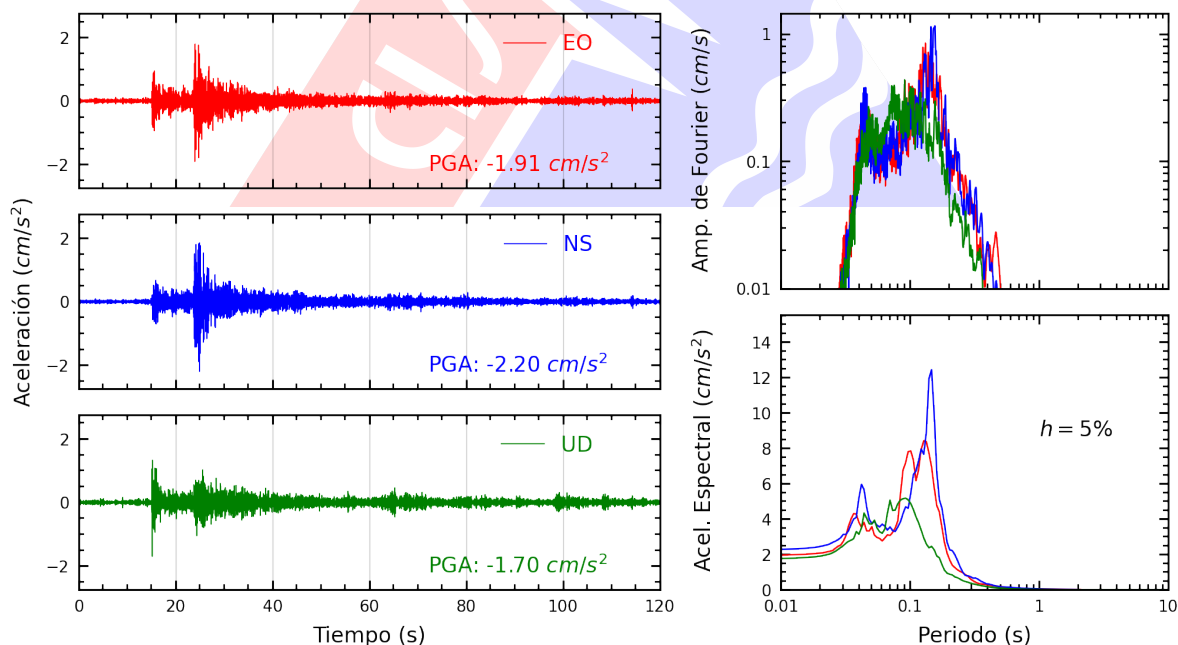
Figura A.8: Registros tiempo-historia, espectros de Fourier y de respuesta en las direcciones EO, NS y vertical de la estación CARAB. Sismo de Provincia Constitucional del Callao , Callao - Lima del 2025-07-24, 22:18:22 (Hora local)
