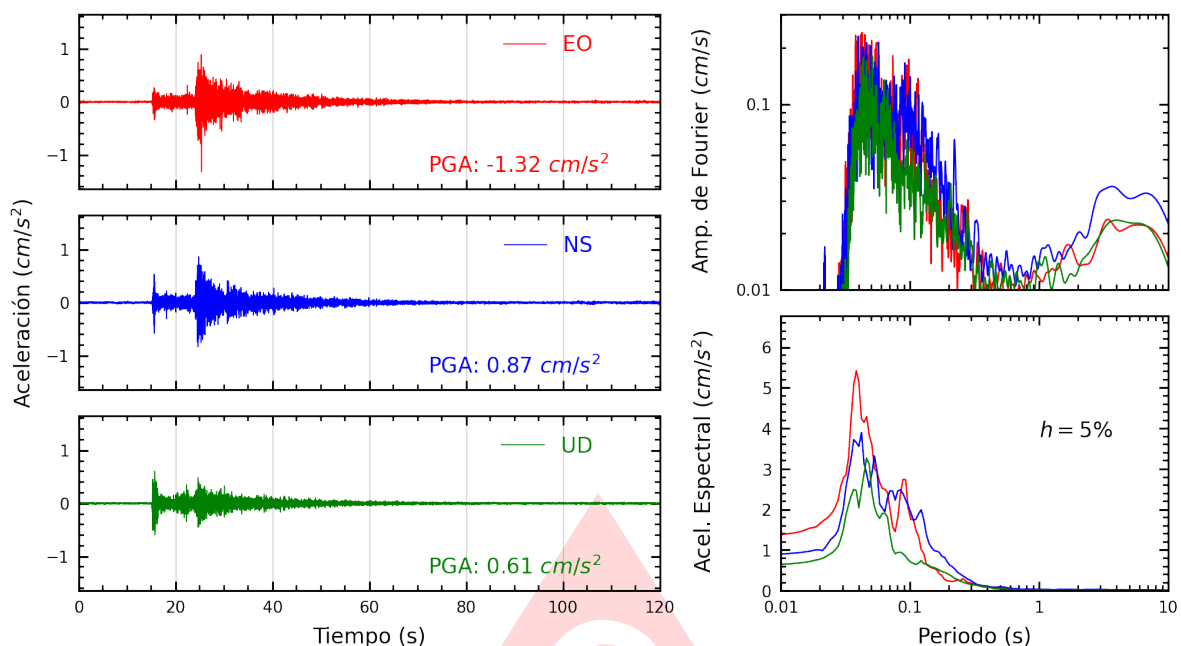
Figura A.21: Registros tiempo-historia, espectros de Fourier y de respuesta en las direcciones EO, NS y vertical de la estación SJLCE. Sismo de Provincia Constitucional del Callao , Callao - Lima del 2025-07-24, 22:18:22 (Hora local)
