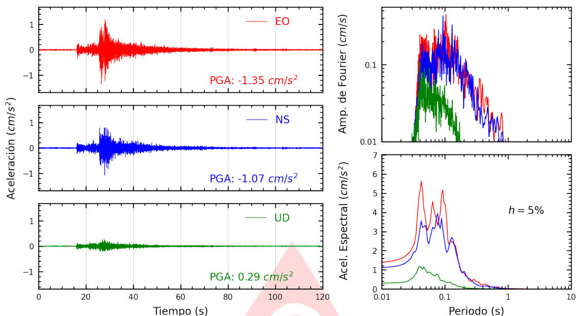
Figura A.19: Registros tiempo-historia, espectros de Fourier y de respuesta en las direcciones EO, NS y vertical de la estación UCVAT. Sismo de Provincia Constitucional del Callao, Callao - Lima del 2025-07-24, 22:18:22 (Hora local)
