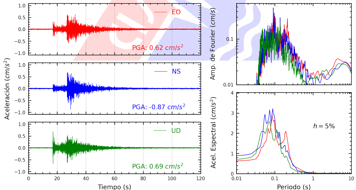
Figura A.28: Registros tiempo-historia, espectros de Fourier y de respuesta en las direcciones EO, NS y vertical de la estación USILP. Sismo de Provincia Constitucional del Callao , Callao - Lima del 2025-07-24, 22:18:22 (Hora local)
