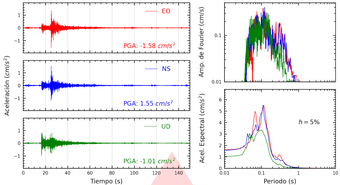
Figura A.1: Registros tiempo-historia, espectros de Fourier y de respuesta en las direcciones EO, NS y vertical de la estación UPAOP. Sismo de Chulucanas, Morropon - Piura del 2025-07-24, 23:31:14 (Hora local)
