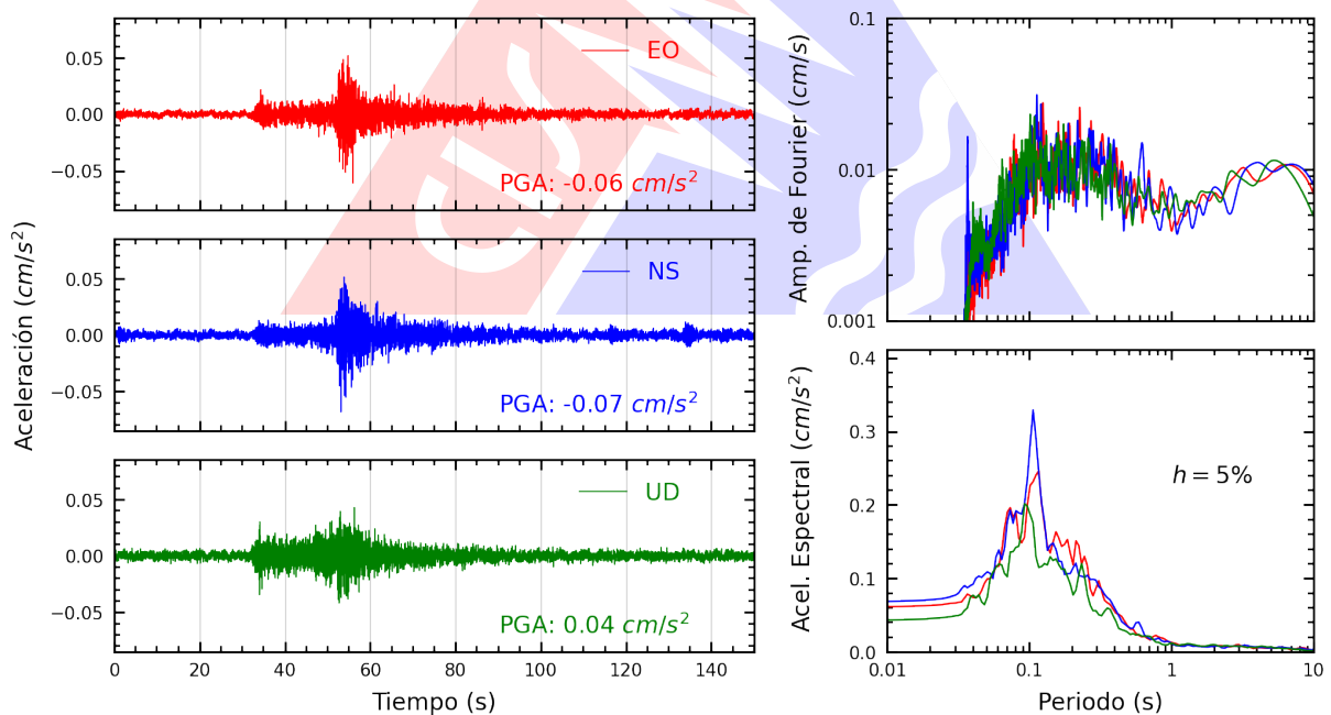
Figura A.2: Registros tiempo-historia, espectros de Fourier y de respuesta en las direcciones EO, NS y vertical de la estación UNJ. Sismo de Chulucanas, Morropon - Piura del 2025-07-24, 23:31:14 (Hora local)
