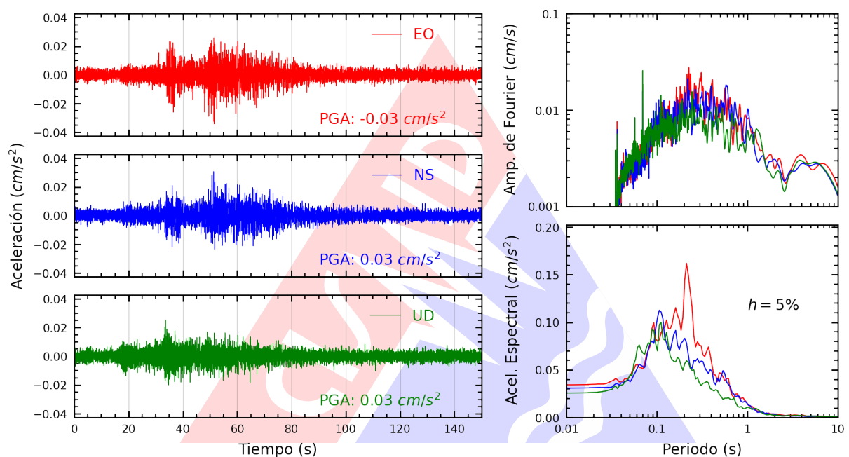
Figura A.3: Registros tiempo-historia, espectros de Fourier y de respuesta en las direcciones EO, NS y vertical de la estación UNC. Sismo de Chulucanas, Morropon - Piura del 2025-07-24, 23:31:14 (Hora local)
