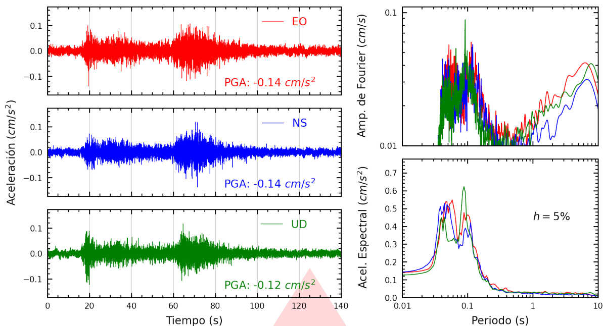
Figura A.1: Registros tiempo-historia, espectros de Fourier y de respuesta en las direcciones EO, NS y vertical de la estación AMORE. Sismo de Puerto Inca, Puerto Inca - Huanuco del 2025-07-27, 05:20:17 (Hora local)
