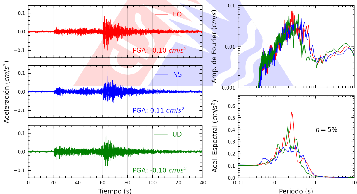
Figura A.2: Registros tiempo-historia, espectros de Fourier y de respuesta en las direcciones EO, NS y vertical de la estación CARAL. Sismo de Puerto Inca, Puerto Inca - Huanuco del 2025-07-27, 05:20:17 (Hora local)
