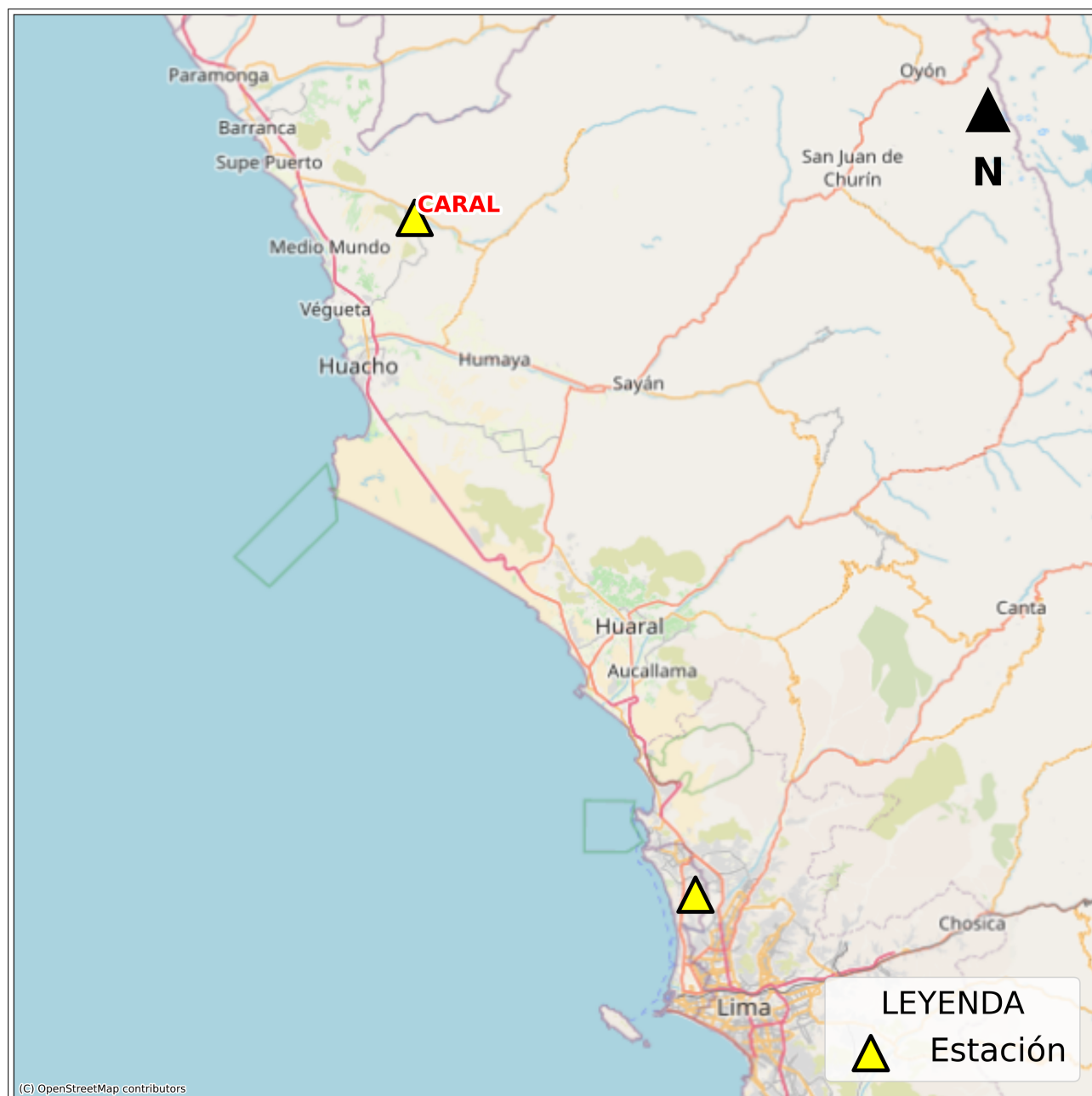
Figura 2: Mapa de ubicación de la(s) estación(es) acelerográfica(s) a nivel nacional correspondiente(s) al Sismo de Puerto Inca, Puerto Inca - Huanuco del 27 de julio de 2025 a las 05:20:17 (hora local)
