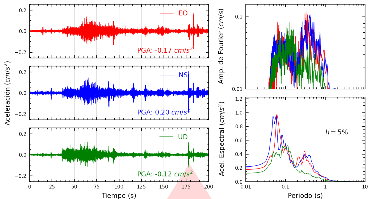
Figura A.1: Registros tiempo-historia, espectros de Fourier y de respuesta en las direcciones EO, NS y vertical de la estación UPAOP. Sismo de Zarumilla, Zarumilla - Tumbes del 2025-07-28, 07:33:57 (Hora local)
