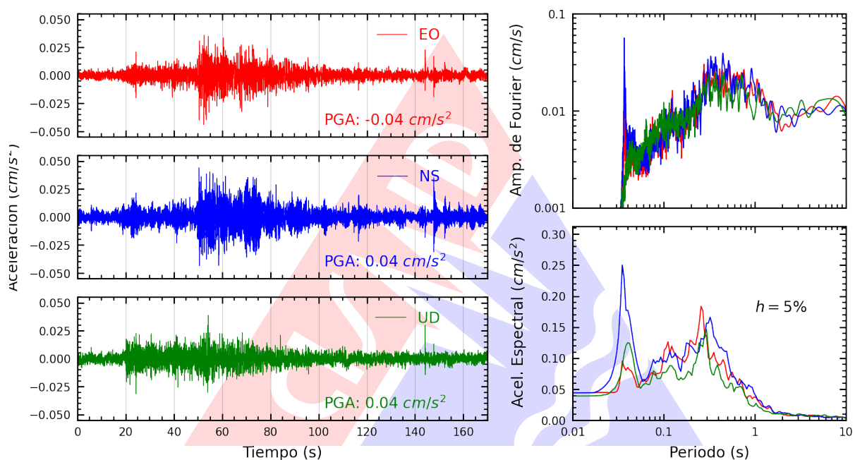
Figura A.3: Registros tiempo-historia, espectros de Fourier y de respuesta en las direcciones EO, NS y vertical de la estación UNJ. Sismo de Zarumilla, Zarumilla - Tumbes del 2025-07-28, 07:33:57 (Hora local)
