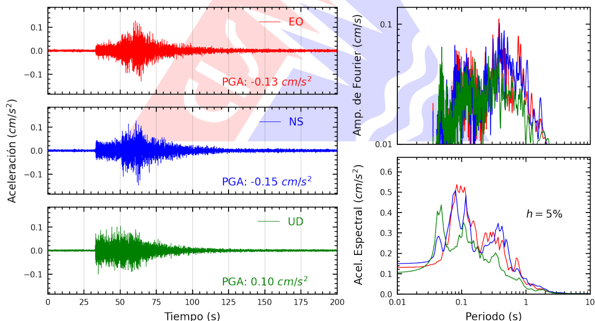
Figura A.2: Registros tiempo-historia, espectros de Fourier y de respuesta en las direcciones EO, NS y vertical de la estación UNF. Sismo de Zarumilla, Zarumilla - Tumbes del 2025-07-28, 07:33:57 (Hora local)
