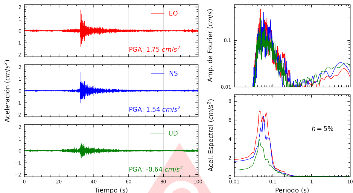
Figura A.3: Registros tiempo-historia, espectros de Fourier y de respuesta en las direcciones EO, NS y vertical de la estación INDEP. Sismo de Chilca, Cañete - Lima del 2025-07-29, 14:13:27 (Hora local)
