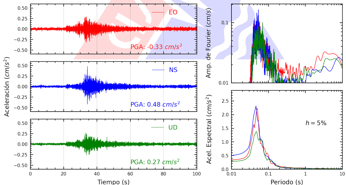
Figura A.22: Registros tiempo-historia, espectros de Fourier y de respuesta en las direcciones EO, NS y vertical de la estación IMCA. Sismo de Chilca, Cañete - Lima del 2025-07-29, 14:13:27 (Hora local)
