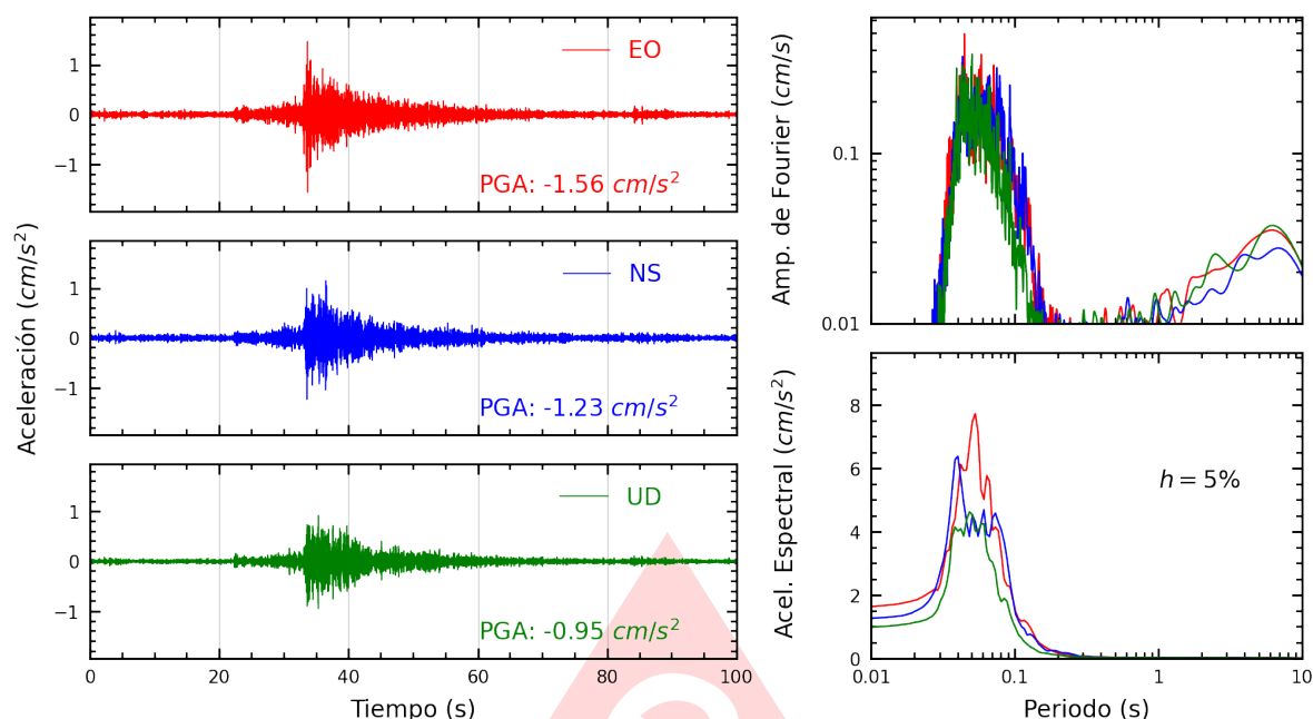
Figura A.5: Registros tiempo-historia, espectros de Fourier y de respuesta en las direcciones EO, NS y vertical de la estación JOSEO. Sismo de Chilca, Cañete - Lima del 2025-07-29, 14:13:27 (Hora local)
