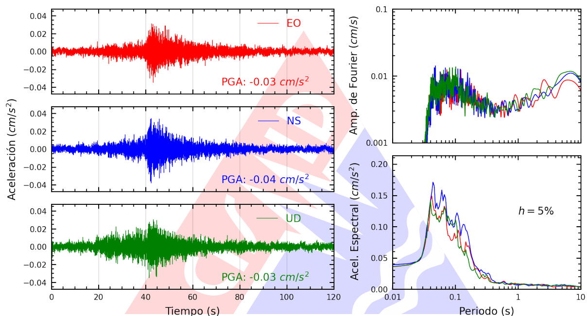
Figura A.35: Registros tiempo-historia, espectros de Fourier y de respuesta en las direcciones EO, NS y vertical de la estación CARAL. Sismo de Chilca, Cañete - Lima del 2025-07-29, 14:13:27 (Hora local)
