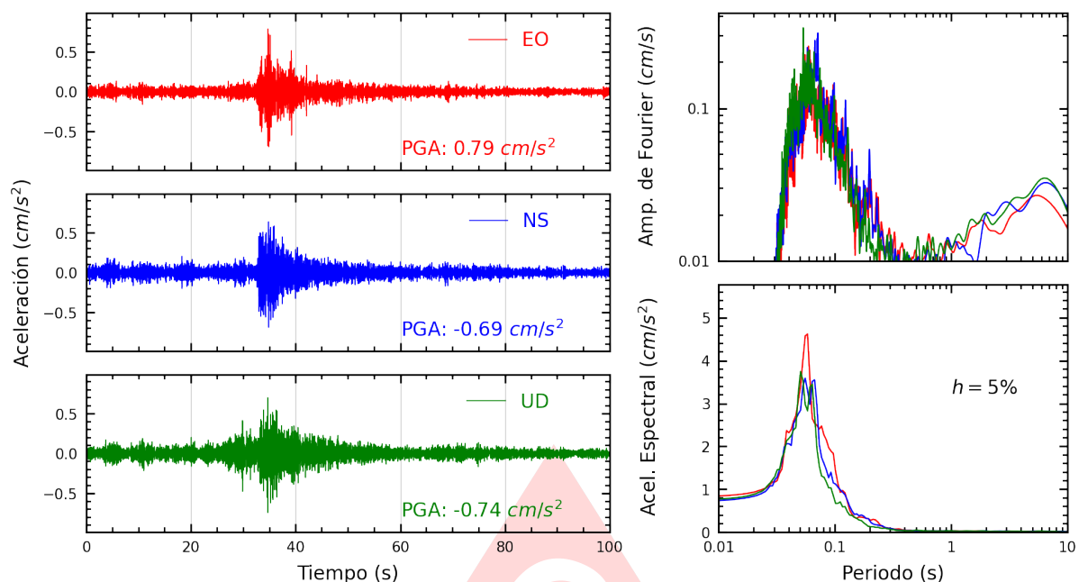
Figura A.13: Registros tiempo-historia, espectros de Fourier y de respuesta en las direcciones EO, NS y vertical de la estación SJLSC. Sismo de Chilca, Cañete - Lima del 2025-07-29, 14:13:27 (Hora local)
