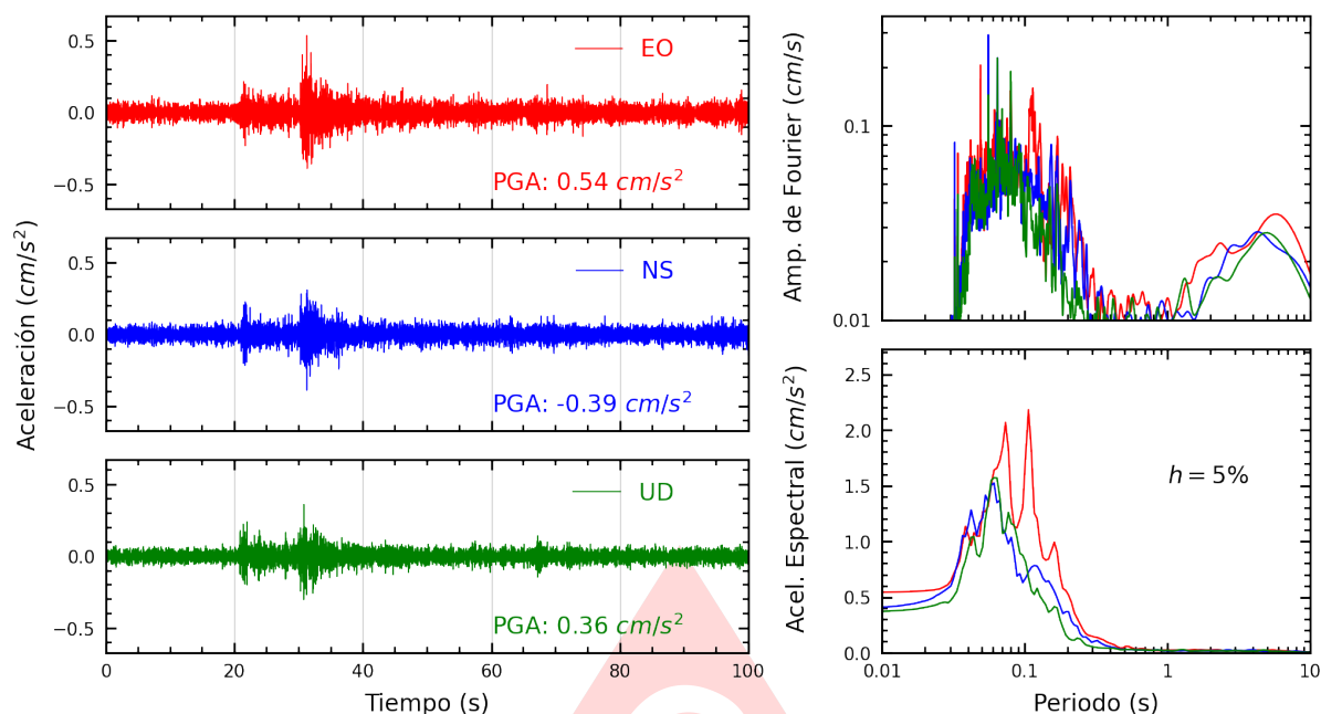
Figura A.17: Registros tiempo-historia, espectros de Fourier y de respuesta en las direcciones EO, NS y vertical de la estación SOBAR. Sismo de Chilca, Cañete - Lima del 2025-07-29, 14:13:27 (Hora local)
