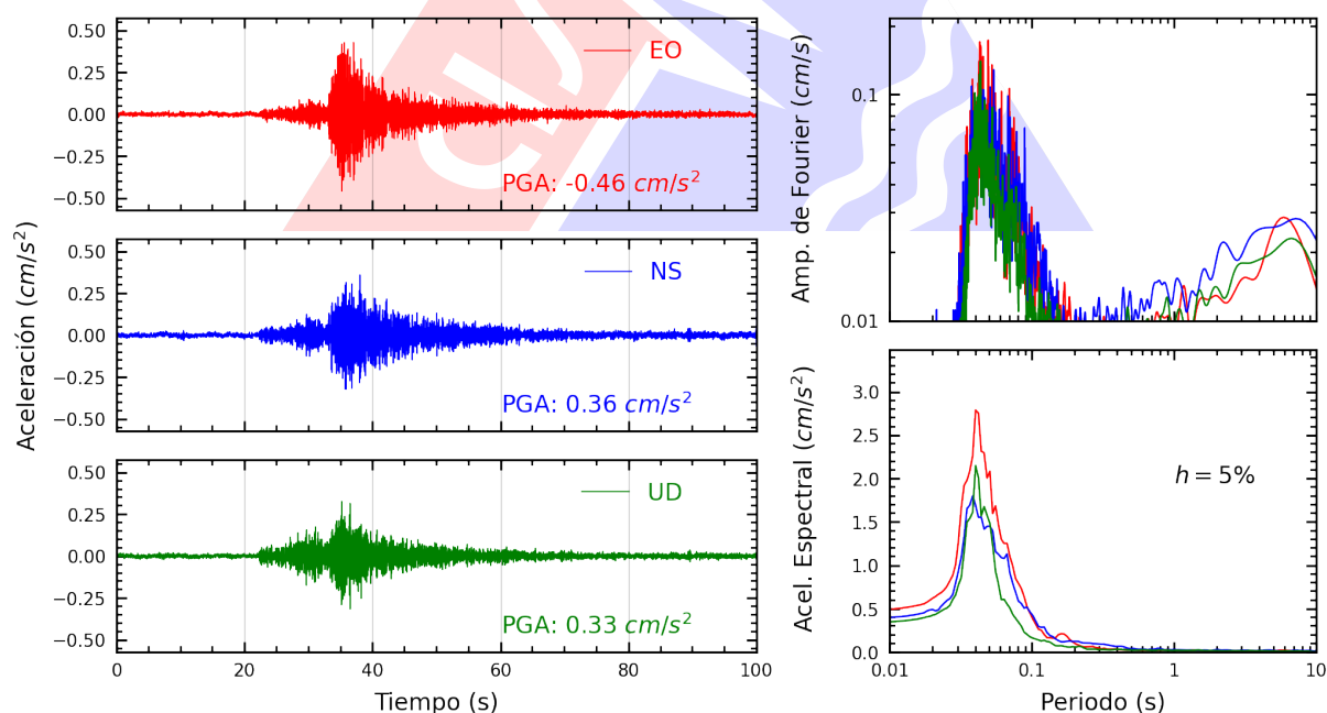
Figura A.24: Registros tiempo-historia, espectros de Fourier y de respuesta en las direcciones EO, NS y vertical de la estación SJLCE. Sismo de Chilca, Cañete - Lima del 2025-07-29, 14:13:27 (Hora local)
