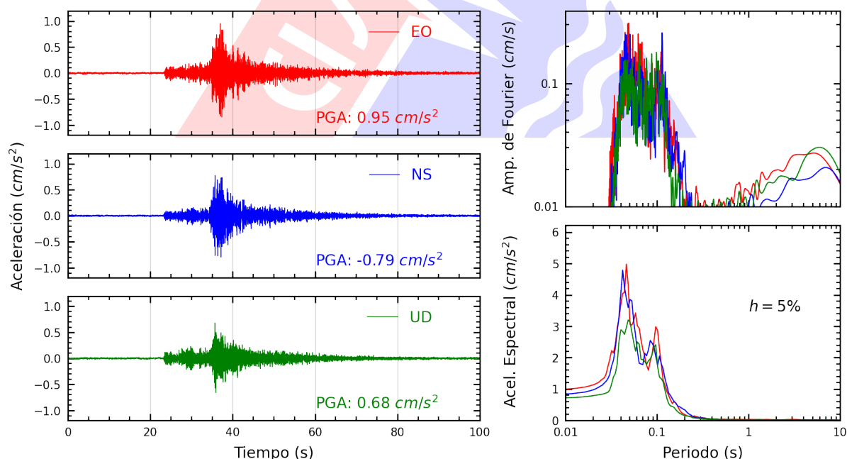
Figura A.8: Registros tiempo-historia, espectros de Fourier y de respuesta en las direcciones EO, NS y vertical de la estación AMORE. Sismo de Chilca, Cañete - Lima del 2025-07-29, 14:13:27 (Hora local)
