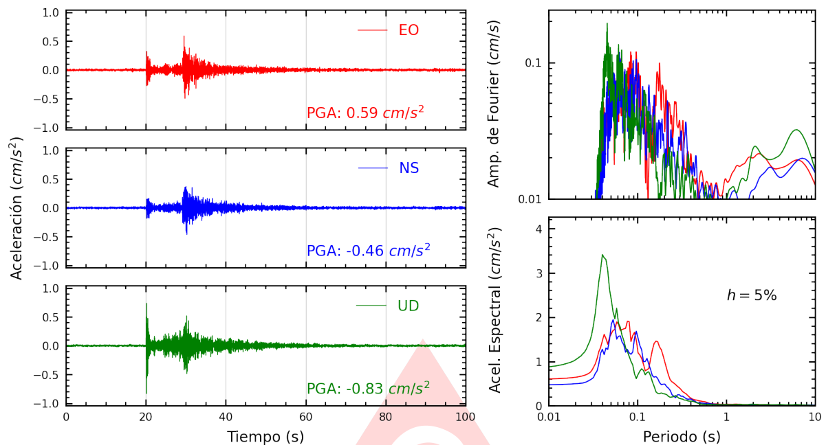
Figura A.11: Registros tiempo-historia, espectros de Fourier y de respuesta en las direcciones EO, NS y vertical de la estación USILP. Sismo de Chilca, Cañete - Lima del 2025-07-29, 14:13:27 (Hora local)
