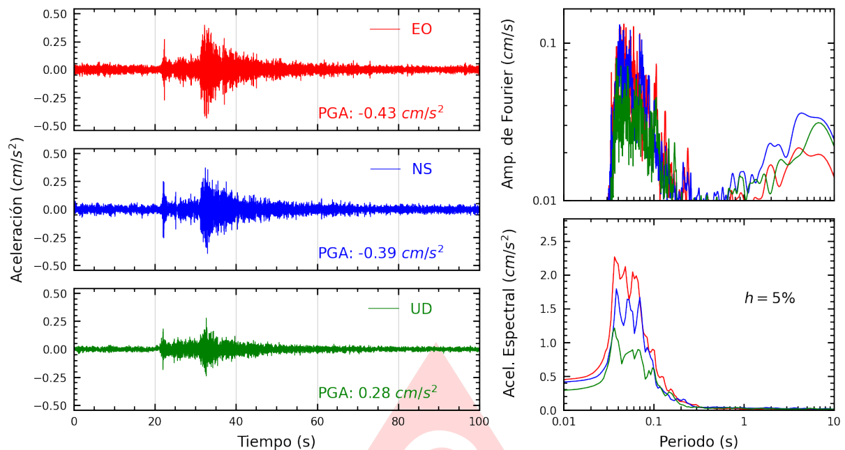
Figura A.25: Registros tiempo-historia, espectros de Fourier y de respuesta en las direcciones EO, NS y vertical de la estación CEPRE. Sismo de Chilca, Cañete - Lima del 2025-07-29, 14:13:27 (Hora local)
