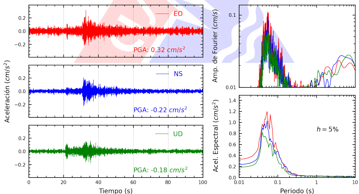
Figura A.30: Registros tiempo-historia, espectros de Fourier y de respuesta en las direcciones EO, NS y vertical de la estación INICT. Sismo de Chilca, Cañete - Lima del 2025-07-29, 14:13:27 (Hora local)
