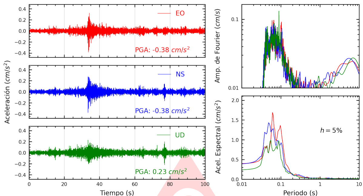
Figura A.29: Registros tiempo-historia, espectros de Fourier y de respuesta en las direcciones EO, NS y vertical de la estación MADRE. Sismo de Chilca, Cañete - Lima del 2025-07-29, 14:13:27 (Hora local)
