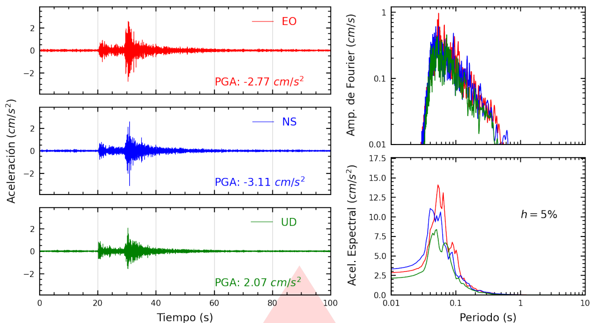
Figura A.1: Registros tiempo-historia, espectros de Fourier y de respuesta en las direcciones EO, NS y vertical de la estación UNTEL. Sismo de Chilca, Cañete - Lima del 2025-07-29, 14:13:27 (Hora local)
