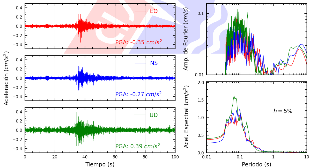
Figura A.28: Registros tiempo-historia, espectros de Fourier y de respuesta en las direcciones EO, NS y vertical de la estación MDPP. Sismo de Chilca, Cañete - Lima del 2025-07-29, 14:13:27 (Hora local)
