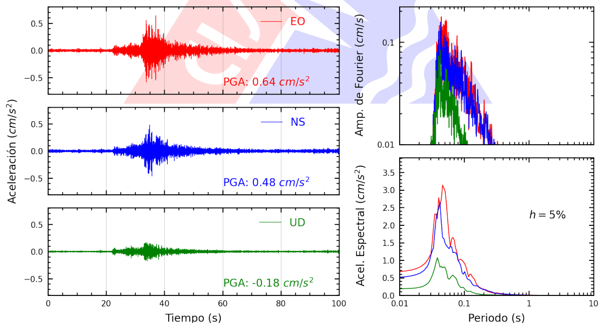
Figura A.16: Registros tiempo-historia, espectros de Fourier y de respuesta en las direcciones EO, NS y vertical de la estación UCVAT. Sismo de Chilca, Cañete - Lima del 2025-07-29, 14:13:27 (Hora local)
