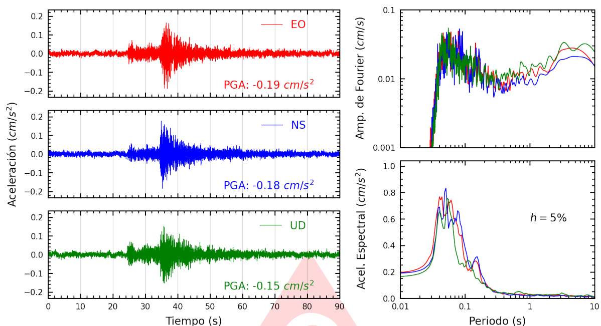
Figura A.33: Registros tiempo-historia, espectros de Fourier y de respuesta en las direcciones EO, NS y vertical de la estación UNMSM. Sismo de Chilca, Cañete - Lima del 2025-07-29, 14:13:27 (Hora local)
