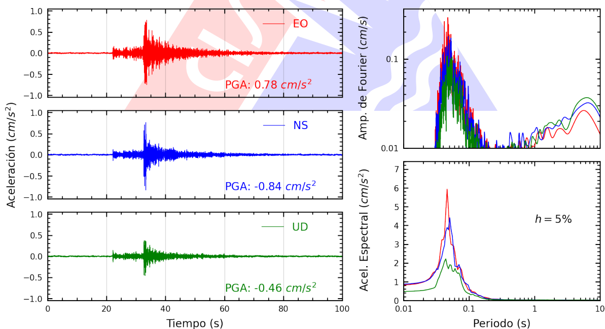
Figura A.10: Registros tiempo-historia, espectros de Fourier y de respuesta en las direcciones EO, NS y vertical de la estación UCSS. Sismo de Chilca, Cañete - Lima del 2025-07-29, 14:13:27 (Hora local)
