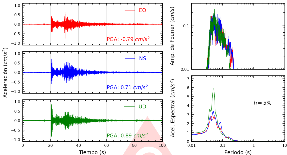
Figura A.9: Registros tiempo-historia, espectros de Fourier y de respuesta en las direcciones EO, NS y vertical de la estación ASIA. Sismo de Chilca, Cañete - Lima del 2025-07-29, 14:13:27 (Hora local)
