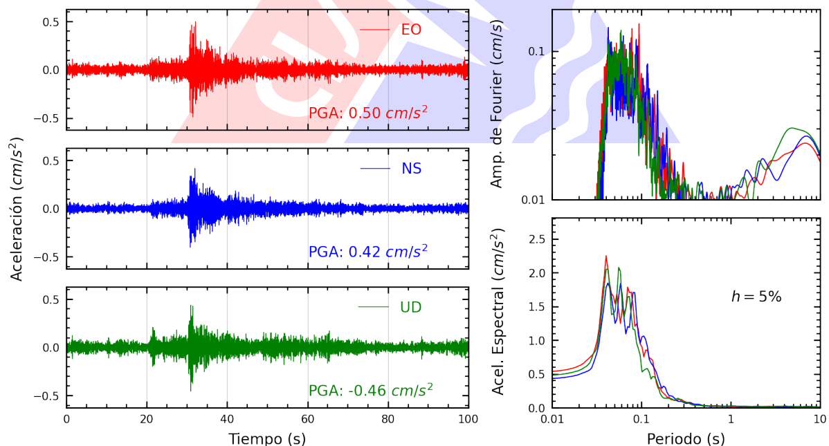
Figura A.20: Registros tiempo-historia, espectros de Fourier y de respuesta en las direcciones EO, NS y vertical de la estación URPPE. Sismo de Chilca, Cañete - Lima del 2025-07-29, 14:13:27 (Hora local)
