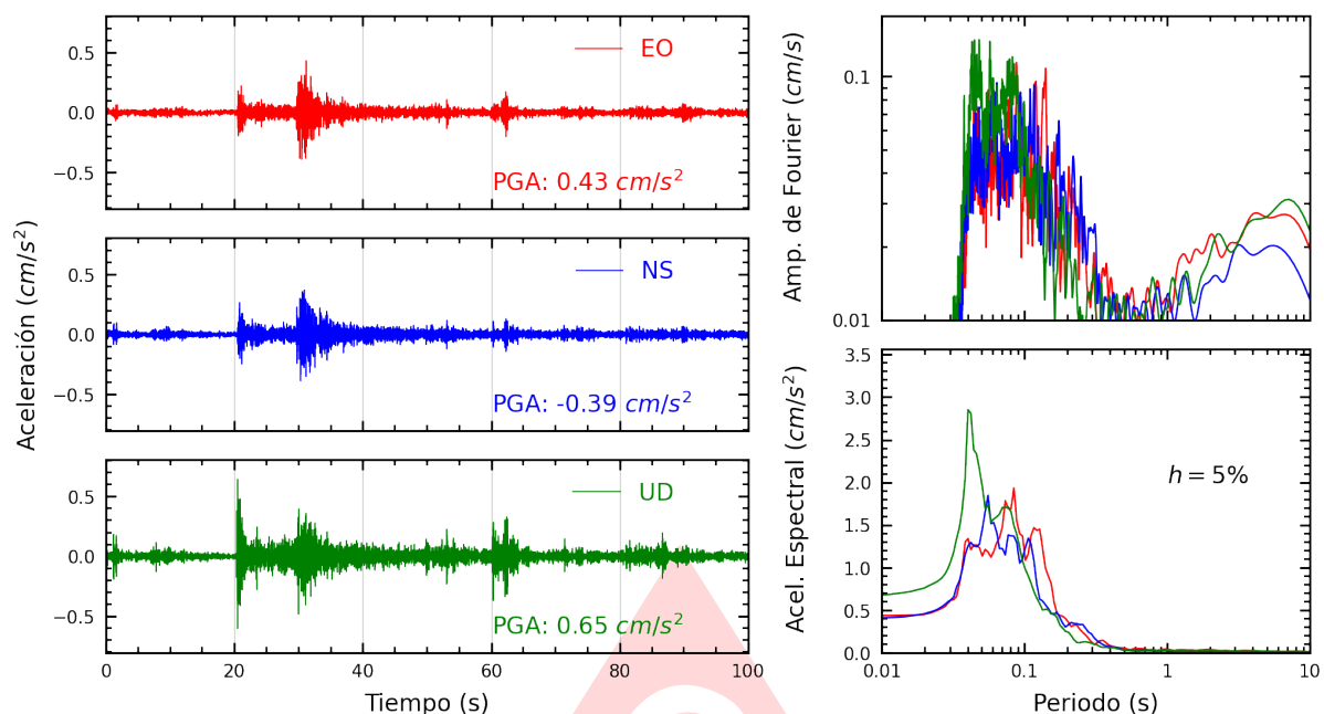
Figura A.15: Registros tiempo-historia, espectros de Fourier y de respuesta en las direcciones EO, NS y vertical de la estación SOCHO. Sismo de Chilca, Cañete - Lima del 2025-07-29, 14:13:27 (Hora local)
