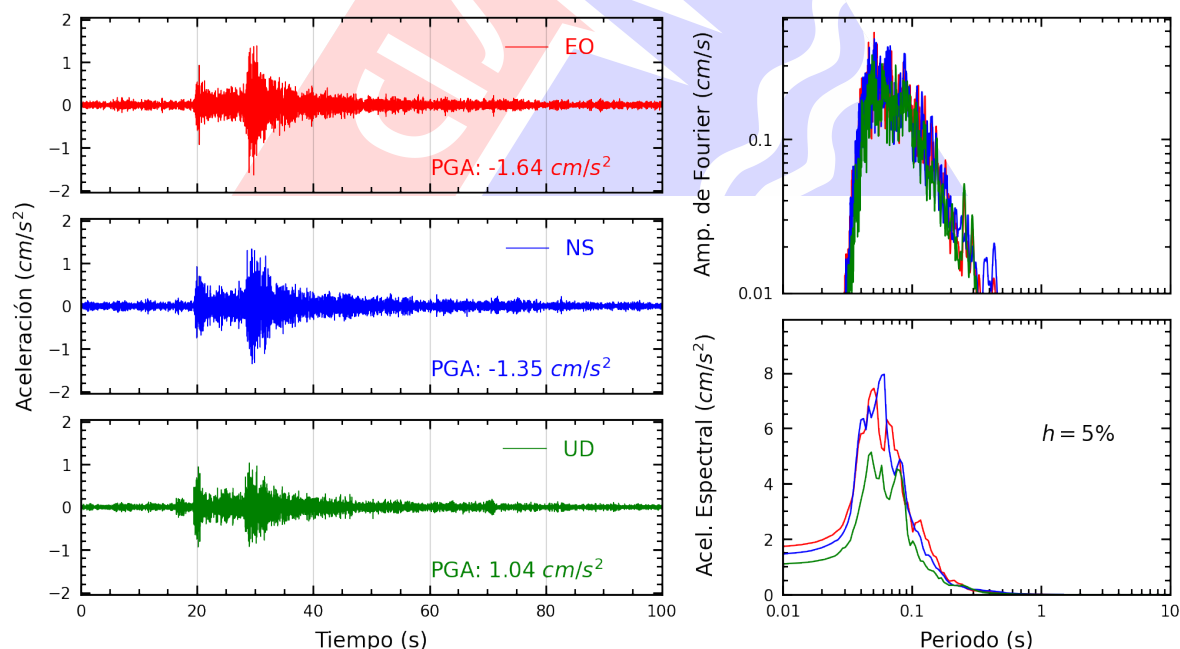
Figura A.4: Registros tiempo-historia, espectros de Fourier y de respuesta en las direcciones EO, NS y vertical de la estación PHERM. Sismo de Chilca, Cañete - Lima del 2025-07-29, 14:13:27 (Hora local)
