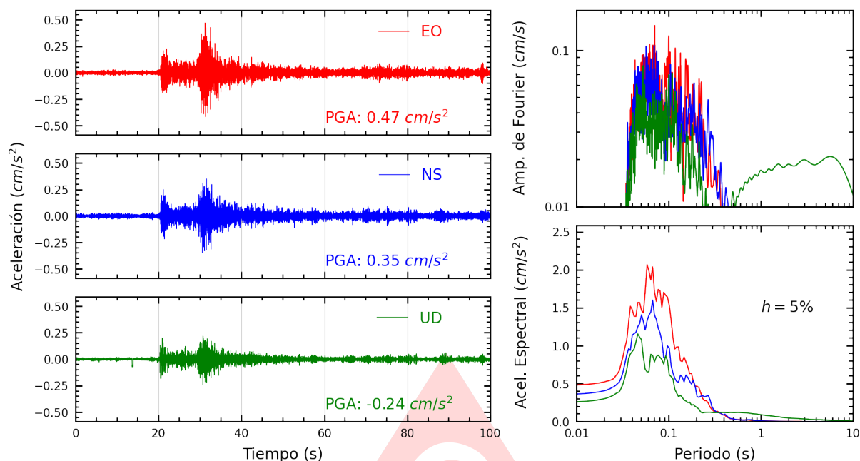
Figura A.23: Registros tiempo-historia, espectros de Fourier y de respuesta en las direcciones EO, NS y vertical de la estación BRISA. Sismo de Chilca, Cañete - Lima del 2025-07-29, 14:13:27 (Hora local)
