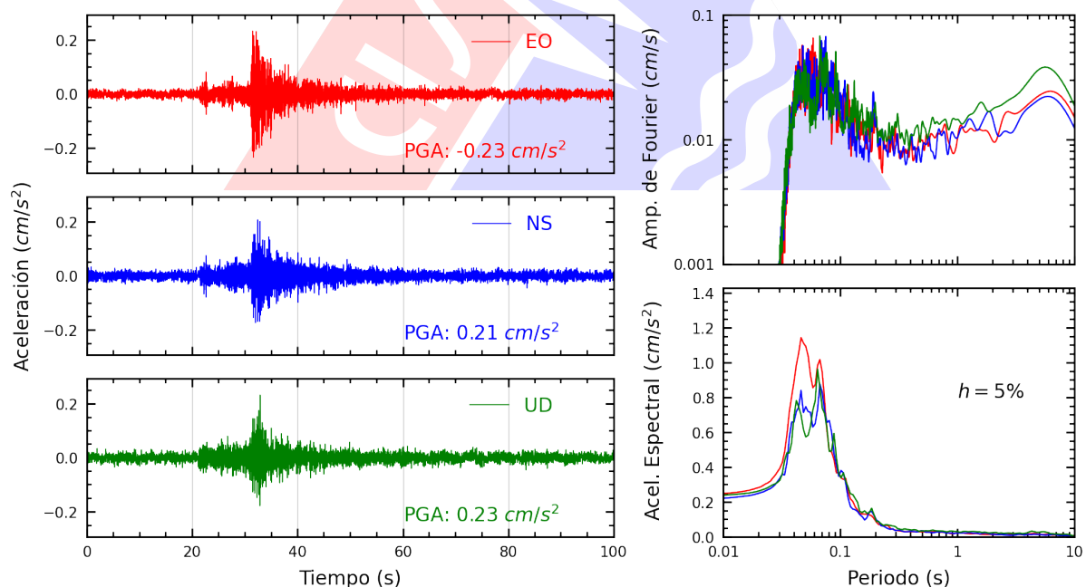
Figura A.32: Registros tiempo-historia, espectros de Fourier y de respuesta en las direcciones EO, NS y vertical de la estación UNFV. Sismo de Chilca, Cañete - Lima del 2025-07-29, 14:13:27 (Hora local)
