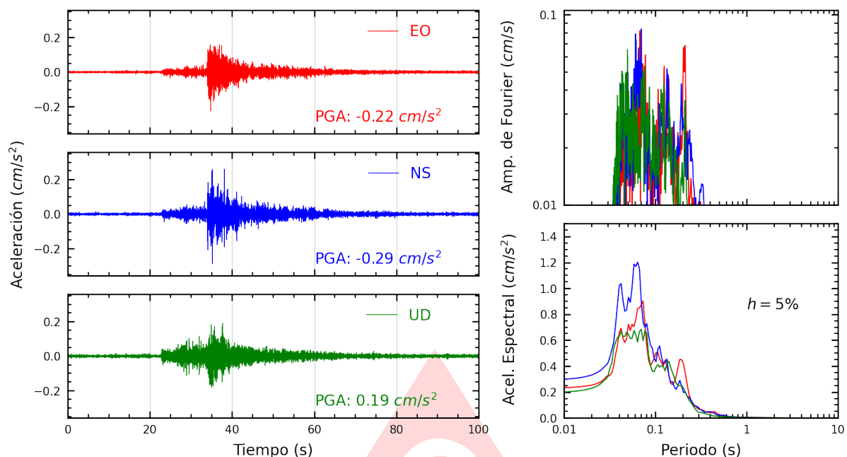
Figura A.31: Registros tiempo-historia, espectros de Fourier y de respuesta en las direcciones EO, NS y vertical de la estación VHAYA. Sismo de Chilca, Cañete - Lima del 2025-07-29, 14:13:27 (Hora local)
