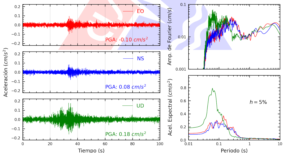
Figura A.34: Registros tiempo-historia, espectros de Fourier y de respuesta en las direcciones EO, NS y vertical de la estación ACAPU. Sismo de Chilca, Cañete - Lima del 2025-07-29, 14:13:27 (Hora local)
