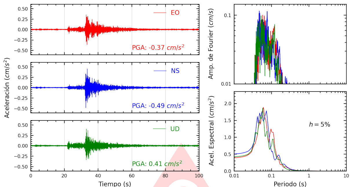
Figura A.21: Registros tiempo-historia, espectros de Fourier y de respuesta en las direcciones EO, NS y vertical de la estación JALV2. Sismo de Chilca, Cañete - Lima del 2025-07-29, 14:13:27 (Hora local)
