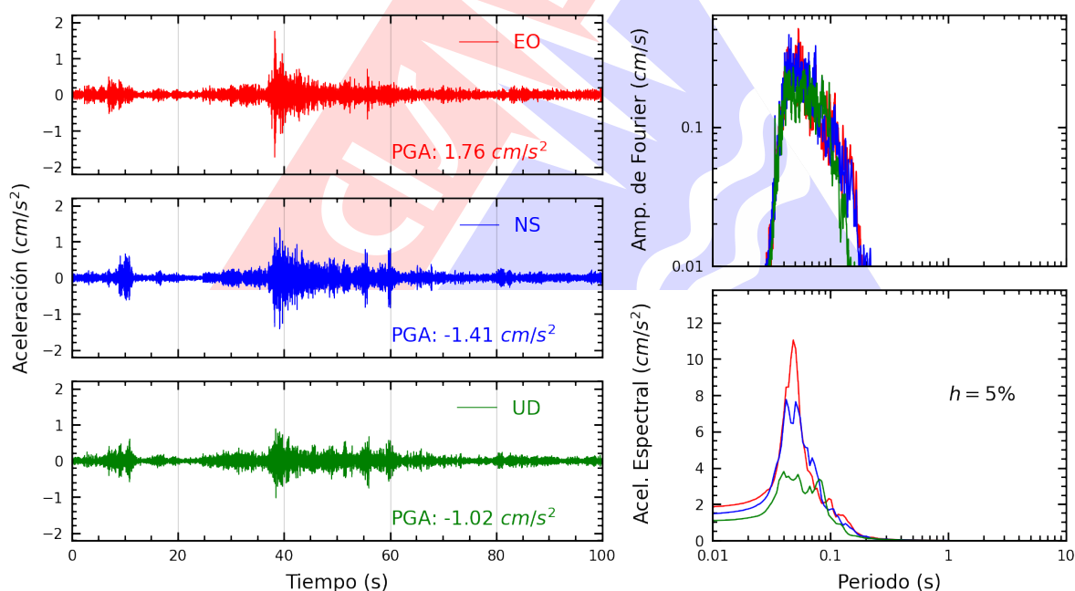
Figura A.2: Registros tiempo-historia, espectros de Fourier y de respuesta en las direcciones EO, NS y vertical de la estación SROSA. Sismo de Chilca, Cañete - Lima del 2025-07-29, 14:13:27 (Hora local)
