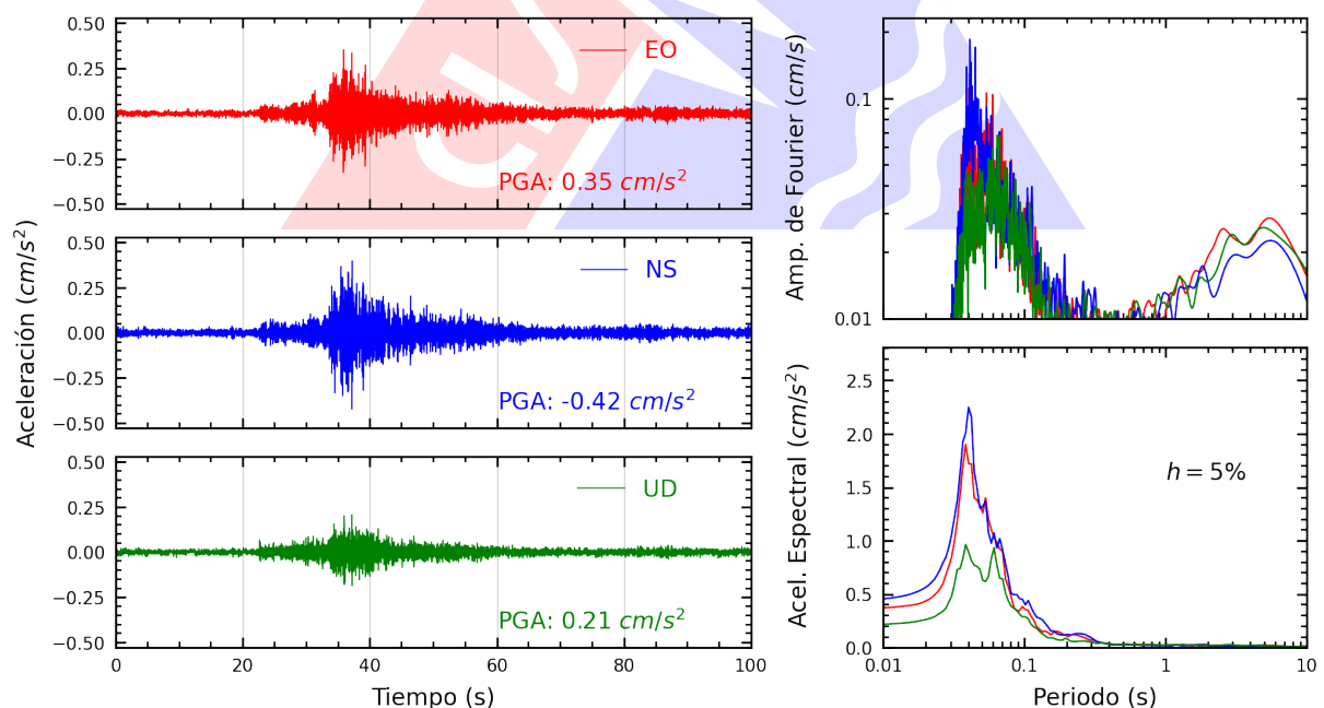
Figura A.26: Registros tiempo-historia, espectros de Fourier y de respuesta en las direcciones EO, NS y vertical de la estación COMAS. Sismo de Chilca, Cañete - Lima del 2025-07-29, 14:13:27 (Hora local)
