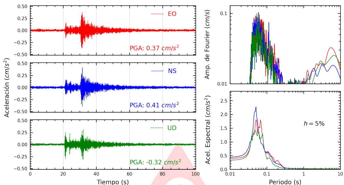
Figura A.27: Registros tiempo-historia, espectros de Fourier y de respuesta en las direcciones EO, NS y vertical de la estación SERVI. Sismo de Chilca, Cañete - Lima del 2025-07-29, 14:13:27 (Hora local)
