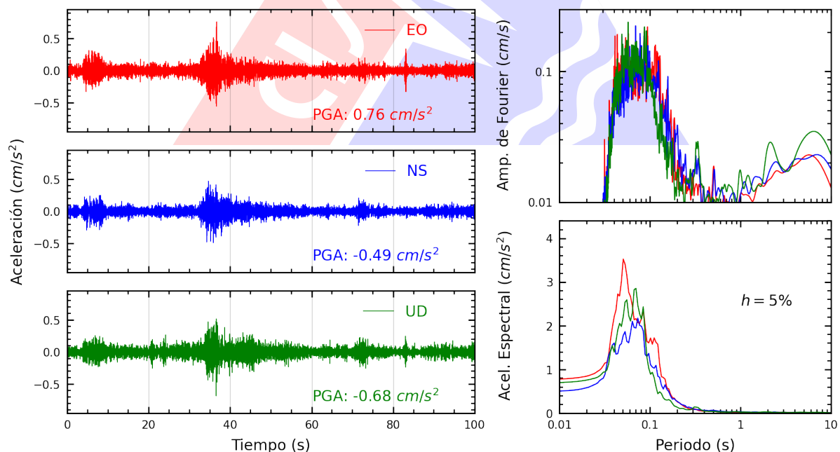
Figura A.14: Registros tiempo-historia, espectros de Fourier y de respuesta en las direcciones EO, NS y vertical de la estación SJLSV. Sismo de Chilca, Cañete - Lima del 2025-07-29, 14:13:27 (Hora local)
