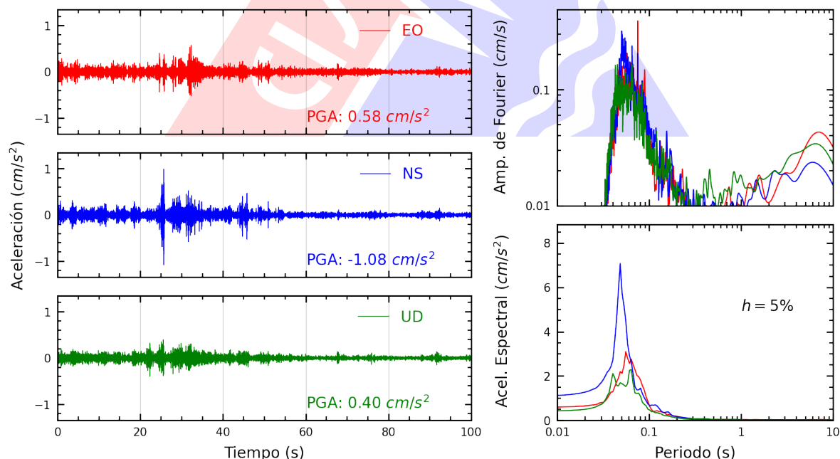
Figura A.6: Registros tiempo-historia, espectros de Fourier y de respuesta en las direcciones EO, NS y vertical de la estación UPCSM. Sismo de Chilca, Cañete - Lima del 2025-07-29, 14:13:27 (Hora local)
