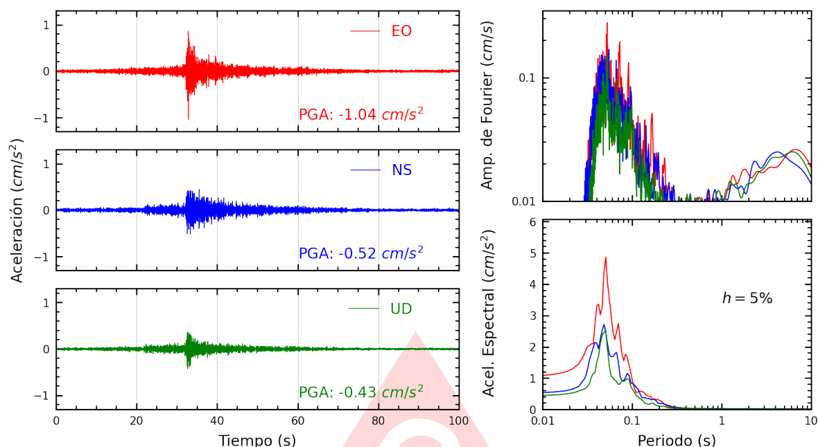
Figura A.7: Registros tiempo-historia, espectros de Fourier y de respuesta en las direcciones EO, NS y vertical de la estación FICPE. Sismo de Chilca, Cañete - Lima del 2025-07-29, 14:13:27 (Hora local)
