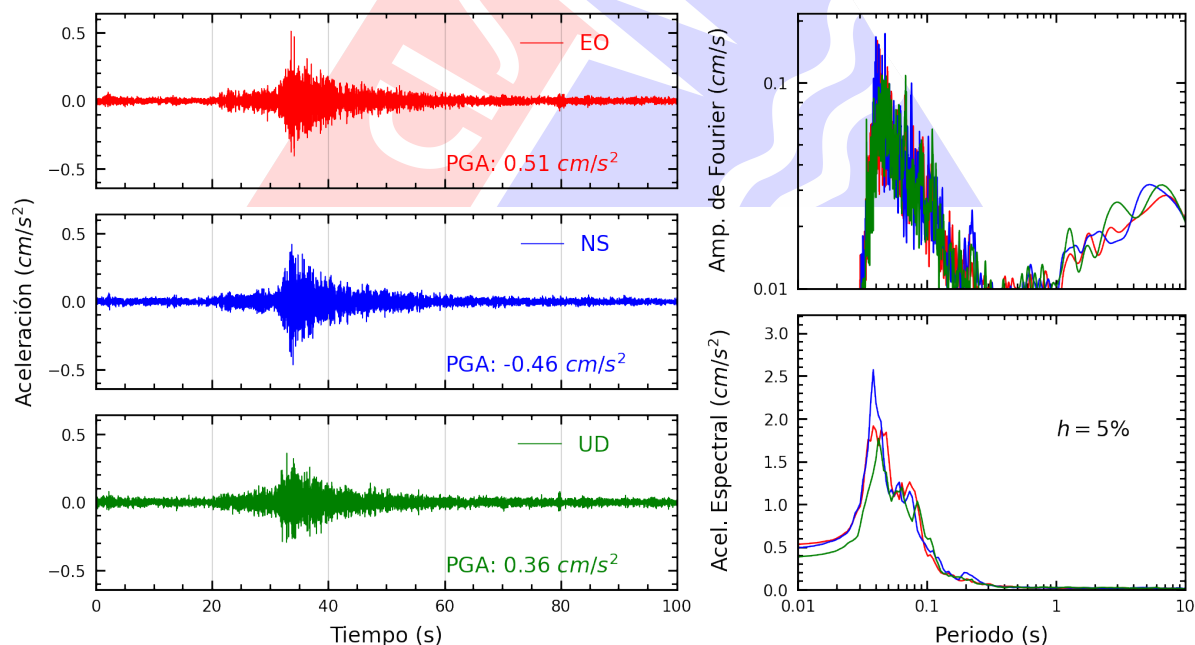
Figura A.18: Registros tiempo-historia, espectros de Fourier y de respuesta en las direcciones EO, NS y vertical de la estación USMP. Sismo de Chilca, Cañete - Lima del 2025-07-29, 14:13:27 (Hora local)
