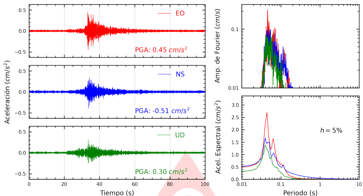
Figura A.19: Registros tiempo-historia, espectros de Fourier y de respuesta en las direcciones EO, NS y vertical de la estación ATARJ. Sismo de Chilca, Cañete - Lima del 2025-07-29, 14:13:27 (Hora local)
