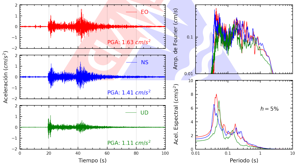
Figura A.2: Registros tiempo-historia, espectros de Fourier y de respuesta en las direcciones EO, NS y vertical de la estación UPTAC. Sismo de Tarata, Tarata - Tacna del 2025-07-29, 22:49:12 (Hora local)
