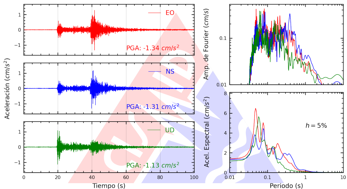
Figura A.3: Registros tiempo-historia, espectros de Fourier y de respuesta en las direcciones EO, NS y vertical de la estación CREY. Sismo de Tarata, Tarata - Tacna del 2025-07-29, 22:49:12 (Hora local)
