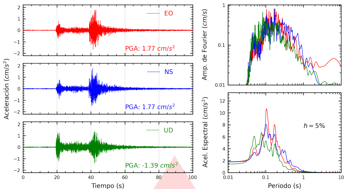
Figura A.1: Registros tiempo-historia, espectros de Fourier y de respuesta en las direcciones EO, NS y vertical de la estación UJBG3. Sismo de Tarata, Tarata - Tacna del 2025-07-29, 22:49:12 (Hora local)
