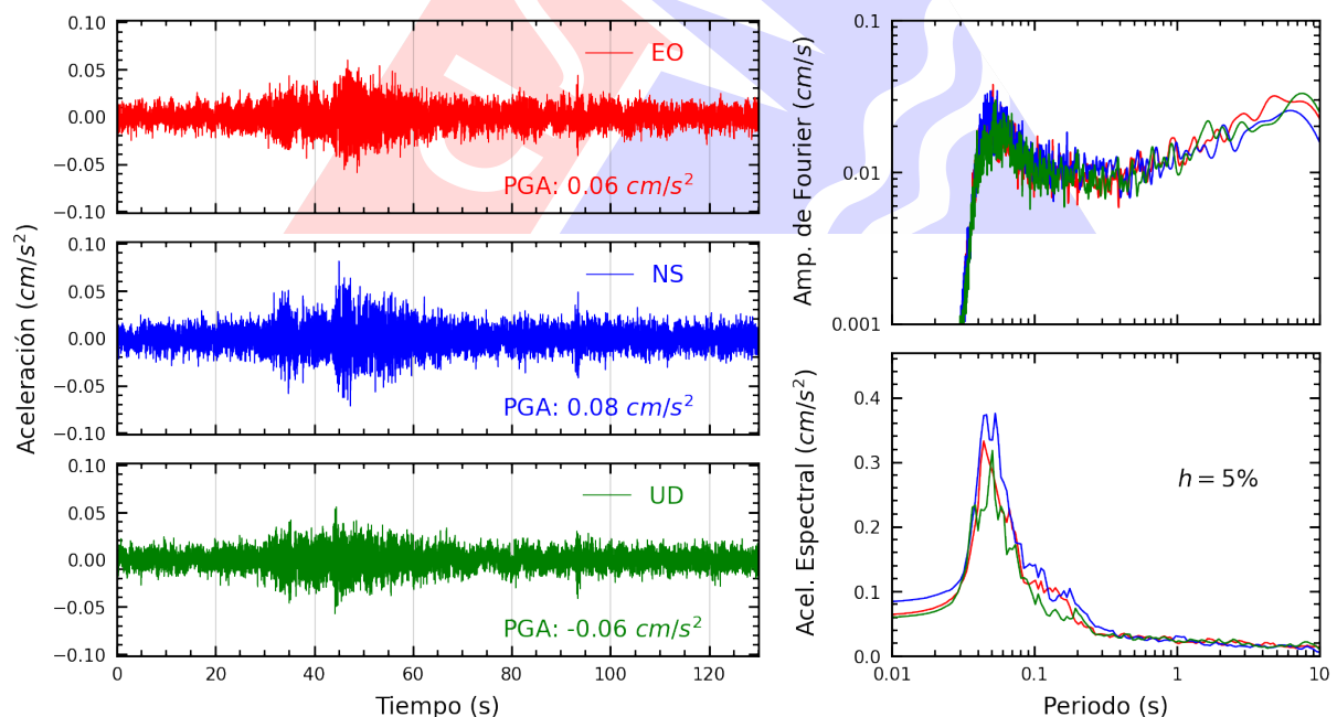
Figura A.10: Registros tiempo-historia, espectros de Fourier y de respuesta en las direcciones EO, NS y vertical de la estación SERVI. Sismo de San Vicente De Cañete, Cañete - Lima del 2025-08-01, 22:53:09 (Hora local)
