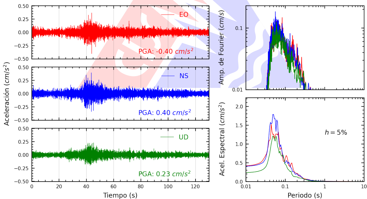
Figura A.2: Registros tiempo-historia, espectros de Fourier y de respuesta en las direcciones EO, NS y vertical de la estación PHERM. Sismo de San Vicente De Cañete, Cañete - Lima del 2025-08-01, 22:53:09 (Hora local)
