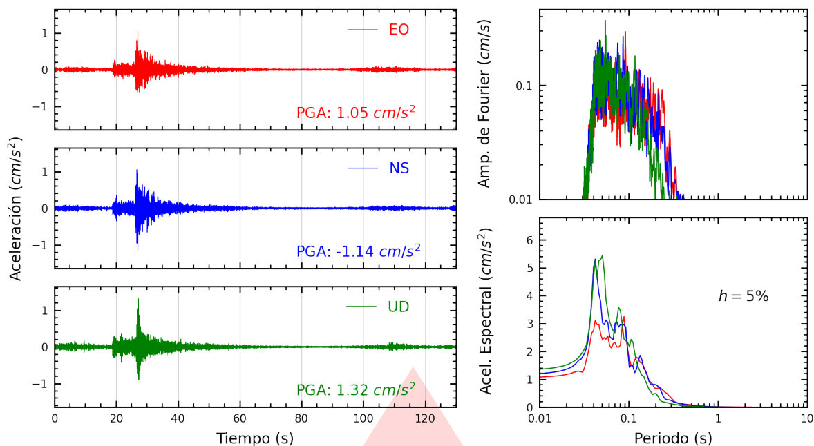
Figura A.1: Registros tiempo-historia, espectros de Fourier y de respuesta en las direcciones EO, NS y vertical de la estación ASIA. Sismo de San Vicente De Cañete, Cañete - Lima del 2025-08-01, 22:53:09 (Hora local)
