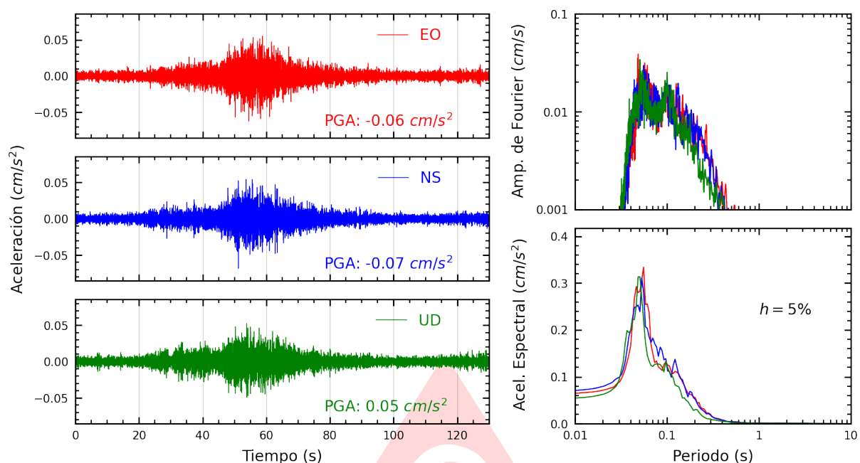
Figura A.11: Registros tiempo-historia, espectros de Fourier y de respuesta en las direcciones EO, NS y vertical de la estación JALV2. Sismo de San Vicente De Cañete, Cañete - Lima del 2025-08-01, 22:53:09 (Hora local)
