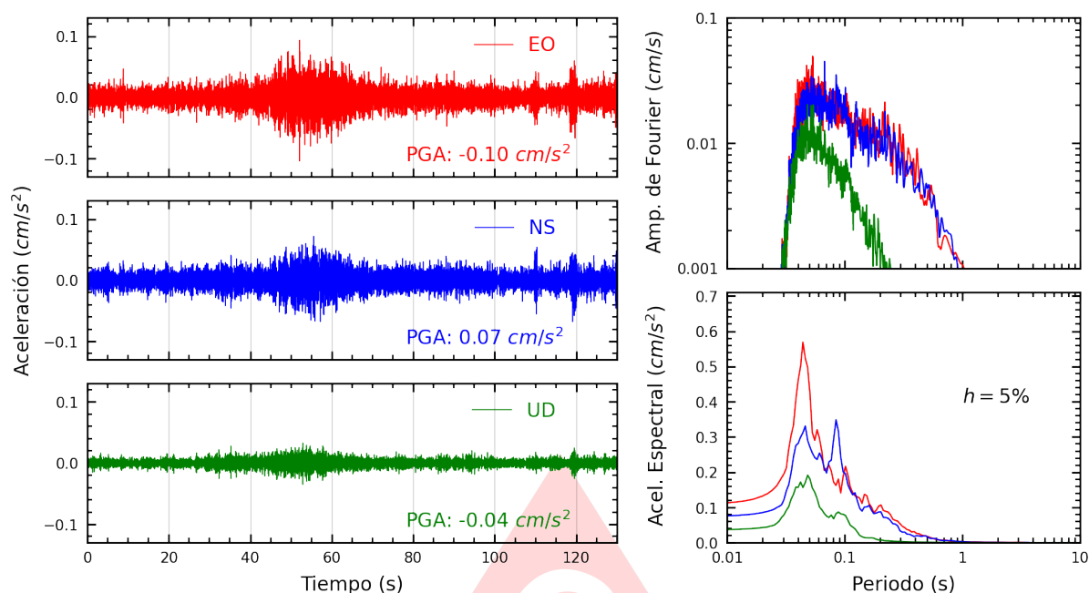
Figura A.7: Registros tiempo-historia, espectros de Fourier y de respuesta en las direcciones EO, NS y vertical de la estación UCVAT. Sismo de San Vicente De Cañete, Cañete - Lima del 2025-08-01, 22:53:09 (Hora local)
