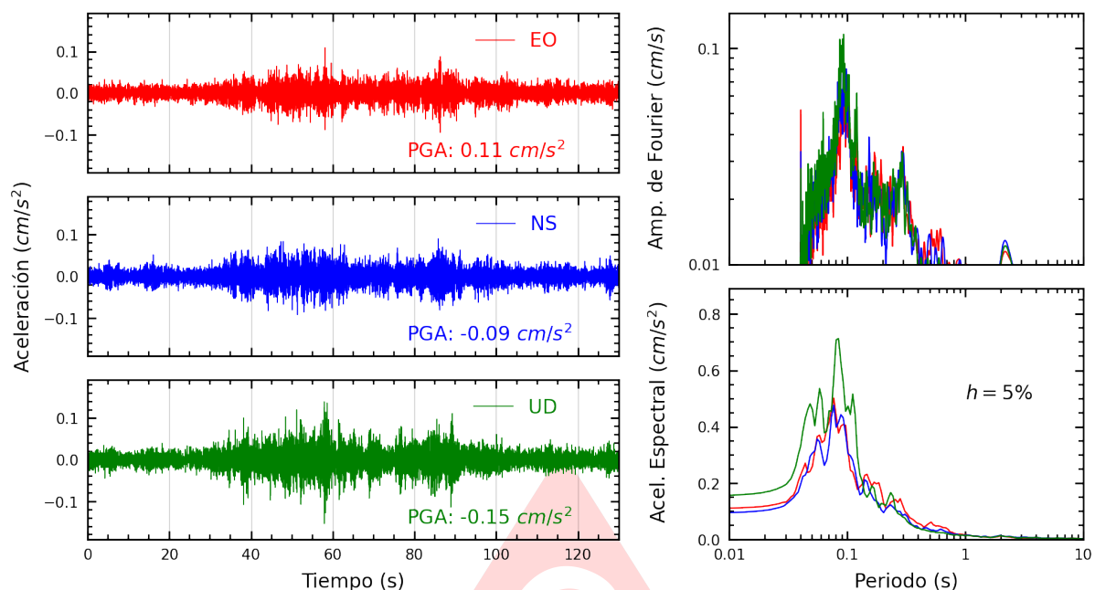
Figura A.5: Registros tiempo-historia, espectros de Fourier y de respuesta en las direcciones EO, NS y vertical de la estación UNICA. Sismo de San Vicente De Cañete, Cañete - Lima del 2025-08-01, 22:53:09 (Hora local)
