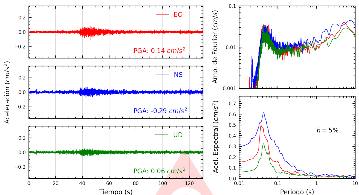
Figura A.3: Registros tiempo-historia, espectros de Fourier y de respuesta en las direcciones EO, NS y vertical de la estación SJLCE. Sismo de San Vicente De Cañete, Cañete - Lima del 2025-08-01, 22:53:09 (Hora local)
