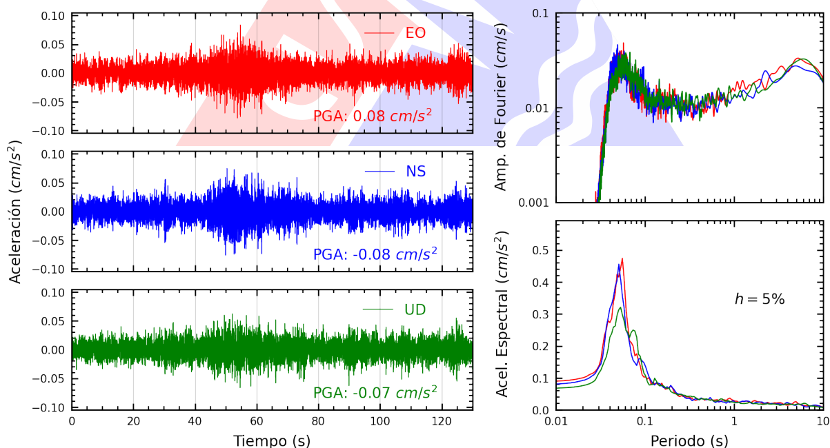
Figura A.8: Registros tiempo-historia, espectros de Fourier y de respuesta en las direcciones EO, NS y vertical de la estación IMCA. Sismo de San Vicente De Cañete, Cañete - Lima del 2025-08-01, 22:53:09 (Hora local)
