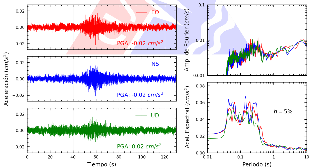
Figura A.12: Registros tiempo-historia, espectros de Fourier y de respuesta en las direcciones EO, NS y vertical de la estación CARAL. Sismo de San Vicente De Cañete, Cañete - Lima del 2025-08-01, 22:53:09 (Hora local)
