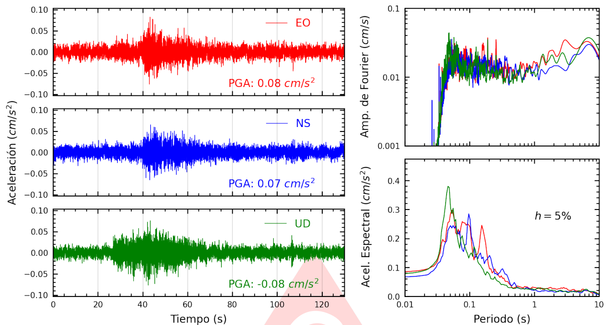
Figura A.9: Registros tiempo-historia, espectros de Fourier y de respuesta en las direcciones EO, NS y vertical de la estación USILP. Sismo de San Vicente De Cañete, Cañete - Lima del 2025-08-01, 22:53:09 (Hora local)
