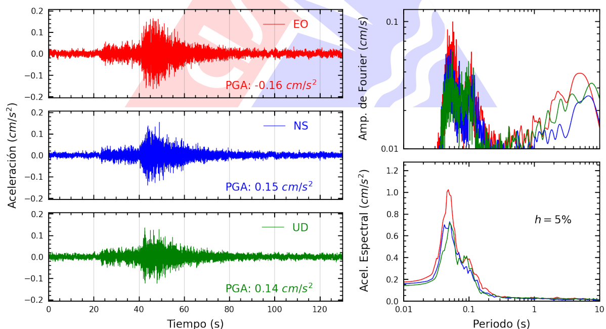
Figura A.4: Registros tiempo-historia, espectros de Fourier y de respuesta en las direcciones EO, NS y vertical de la estación AMORE. Sismo de San Vicente De Cañete, Cañete - Lima del 2025-08-01, 22:53:09 (Hora local)
