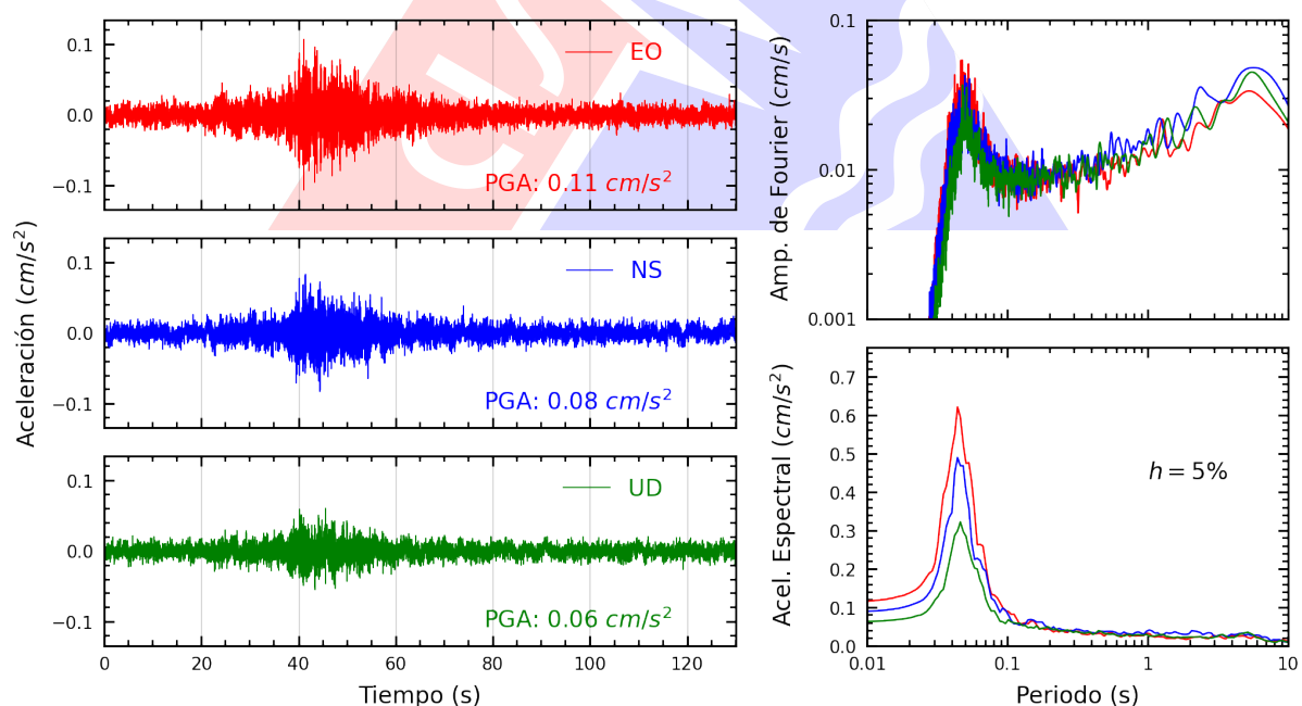
Figura A.6: Registros tiempo-historia, espectros de Fourier y de respuesta en las direcciones EO, NS y vertical de la estación UCSS. Sismo de San Vicente De Cañete, Cañete - Lima del 2025-08-01, 22:53:09 (Hora local)
