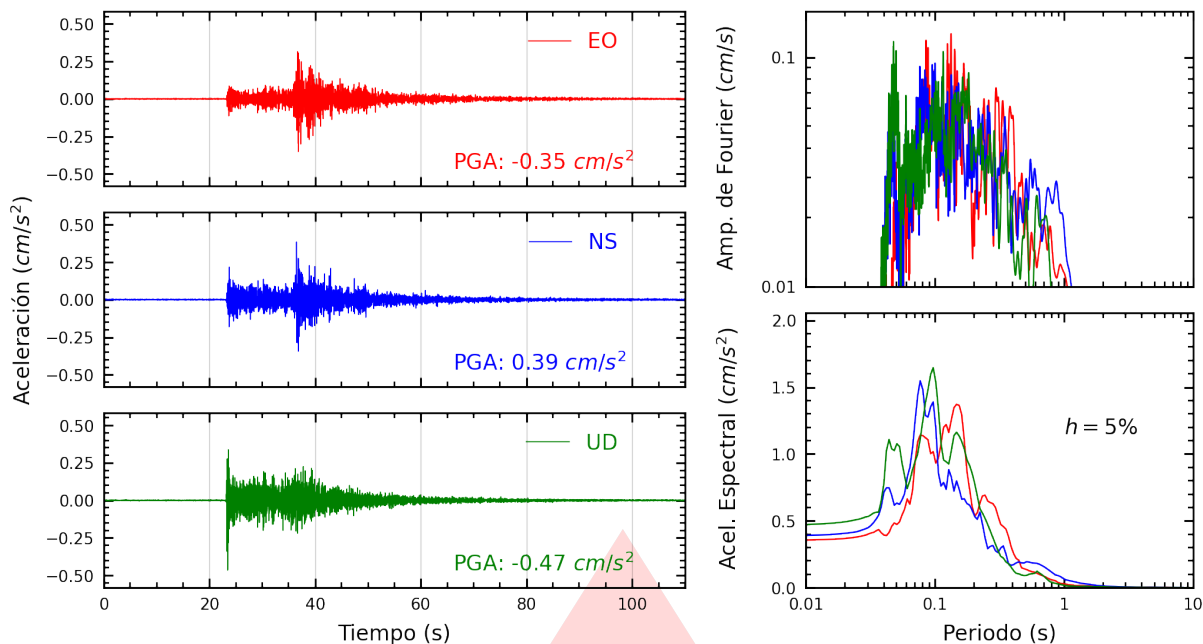
Figura A.1: Registros tiempo-historia, espectros de Fourier y de respuesta en las direcciones EO, NS y vertical de la estación UNF. Sismo de Zorritos, Contralmirante Villar - Tumbes del 2025-08-03, 22:06:15 (Hora local)
