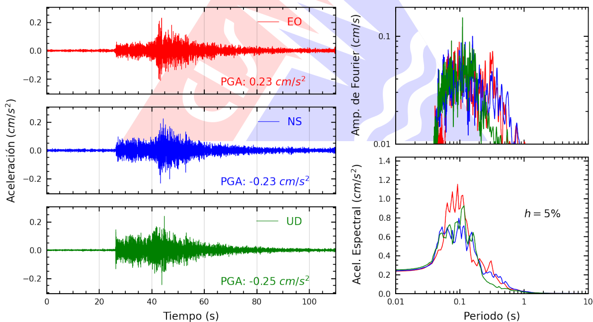
Figura A.2: Registros tiempo-historia, espectros de Fourier y de respuesta en las direcciones EO, NS y vertical de la estación UPAOP. Sismo de Zorritos, Contralmirante Villar - Tumbes del 2025-08-03, 22:06:15 (Hora local)
