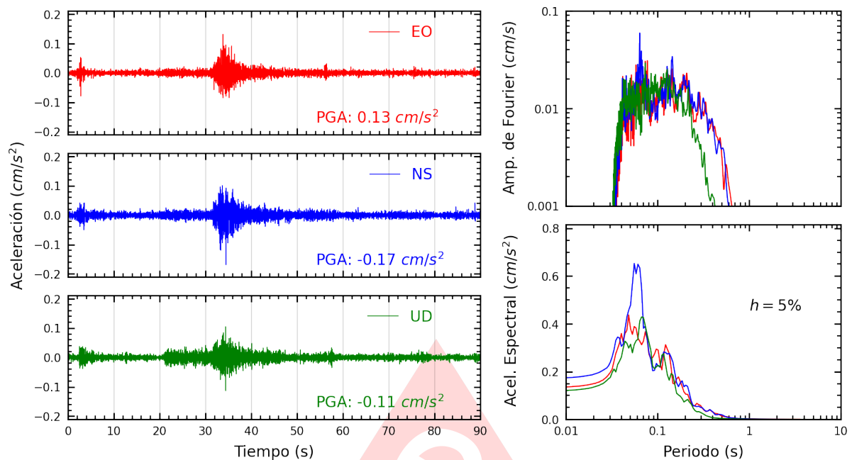
Figura A.3: Registros tiempo-historia, espectros de Fourier y de respuesta en las direcciones EO, NS y vertical de la estación VHAYA. Sismo de Chilca, Cañete - Lima del 2025-08-04, 07:38:26 (Hora local)
