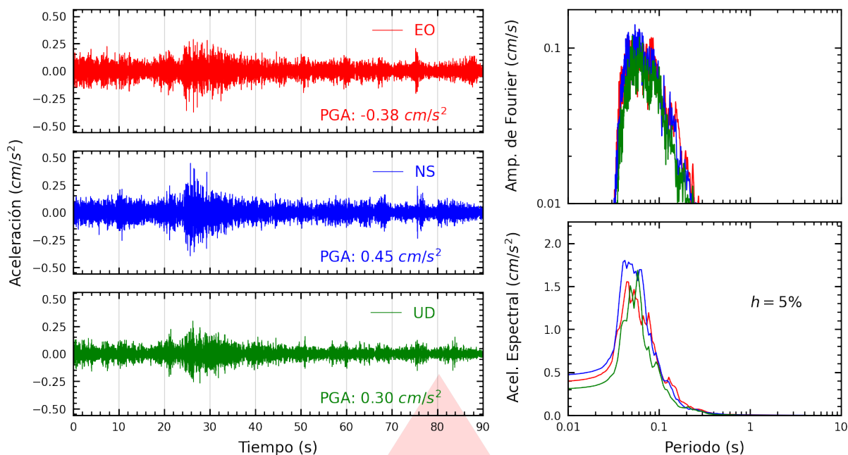
Figura A.1: Registros tiempo-historia, espectros de Fourier y de respuesta en las direcciones EO, NS y vertical de la estación PHERM. Sismo de Chilca, Cañete - Lima del 2025-08-04, 07:38:26 (Hora local)
