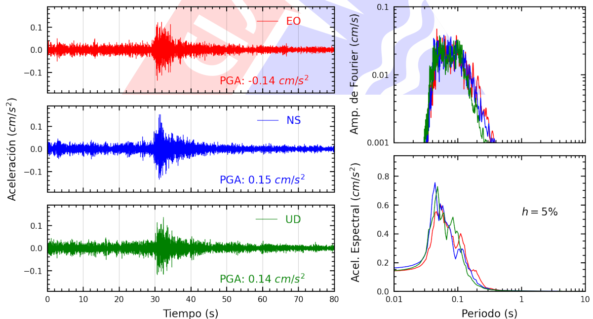
Figura A.4: Registros tiempo-historia, espectros de Fourier y de respuesta en las direcciones EO, NS y vertical de la estación JALV2. Sismo de Chilca, Cañete - Lima del 2025-08-04, 07:38:26 (Hora local)
