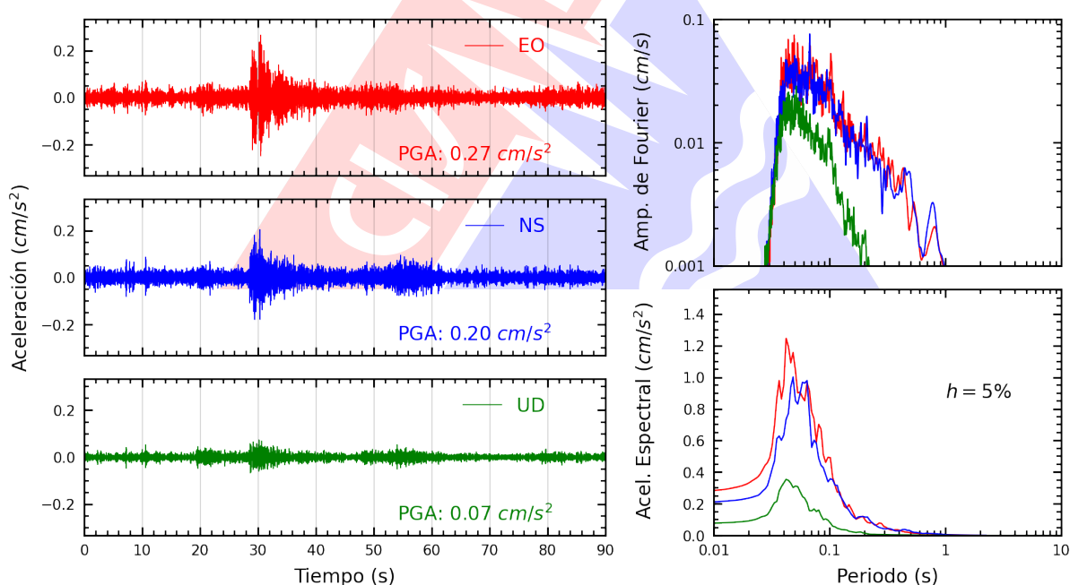
Figura A.2: Registros tiempo-historia, espectros de Fourier y de respuesta en las direcciones EO, NS y vertical de la estación UCVAT. Sismo de Chilca, Cañete - Lima del 2025-08-04, 07:38:26 (Hora local)
