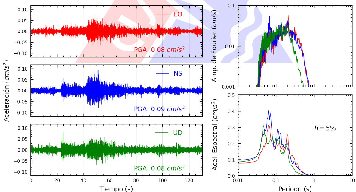
Figura A.10: Registros tiempo-historia, espectros de Fourier y de respuesta en las direcciones EO, NS y vertical de la estación VHAYA. Sismo de Tambo De Mora, Chincha - Ica del 2025-08-06, 13:24:45 (Hora local)
