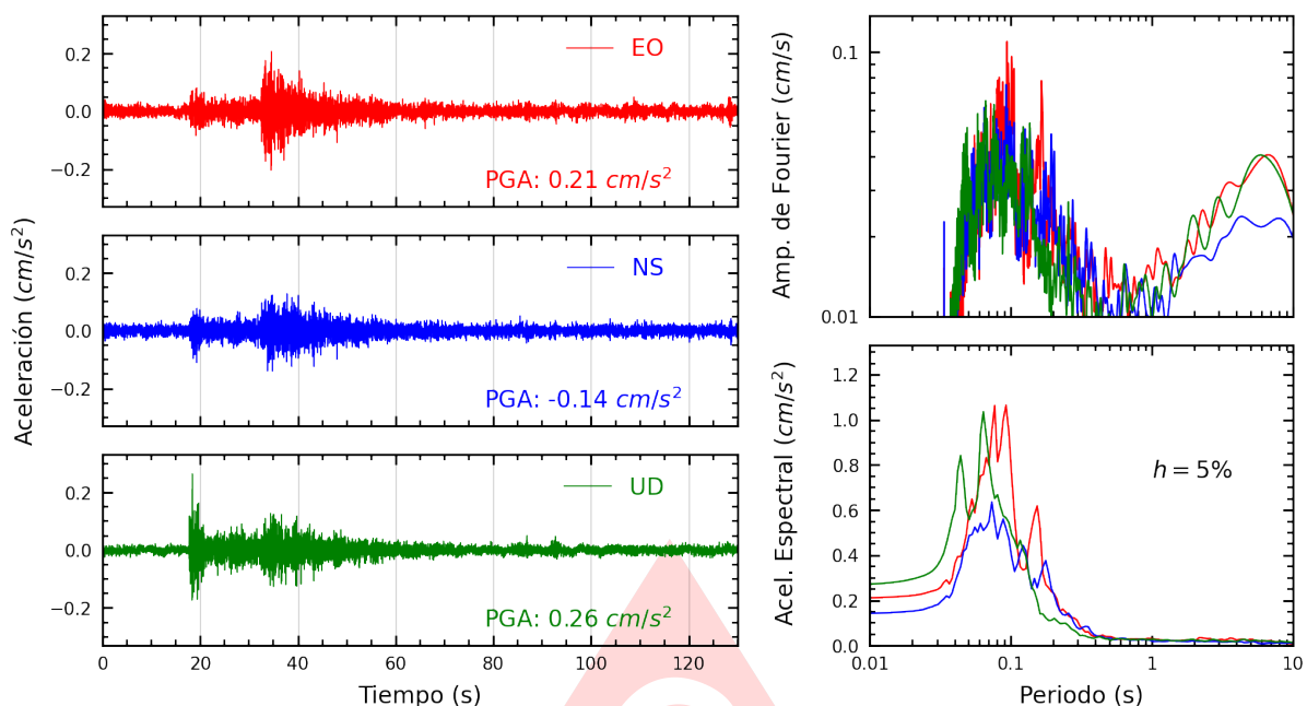
Figura A.5: Registros tiempo-historia, espectros de Fourier y de respuesta en las direcciones EO, NS y vertical de la estación USILP. Sismo de Tambo De Mora, Chincha - Ica del 2025-08-06, 13:24:45 (Hora local)
