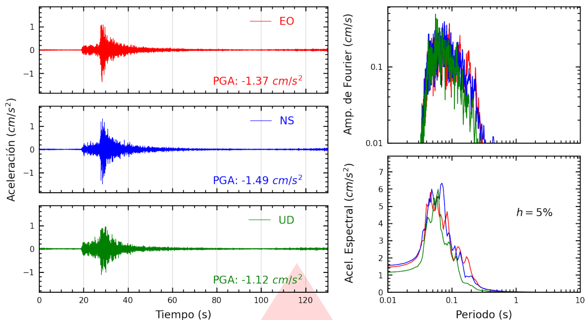
Figura A.1: Registros tiempo-historia, espectros de Fourier y de respuesta en las direcciones EO, NS y vertical de la estación ASIA. Sismo de Tambo De Mora, Chincha - Ica del 2025-08-06, 13:24:45 (Hora local)
