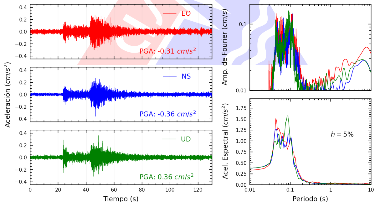
Figura A.4: Registros tiempo-historia, espectros de Fourier y de respuesta en las direcciones EO, NS y vertical de la estación AMORE. Sismo de Tambo De Mora, Chíncha - Ica del 2025-08-06, 13:24:45 (Hora local)
