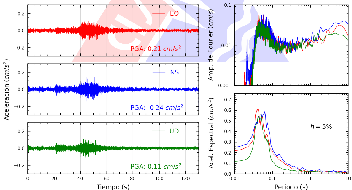
Figura A.6: Registros tiempo-historia, espectros de Fourier y de respuesta en las direcciones EO, NS y vertical de la estación SJLCE. Sismo de Tambo De Mora, Chincha - Ica del 2025-08-06, 13:24:45 (Hora local)
