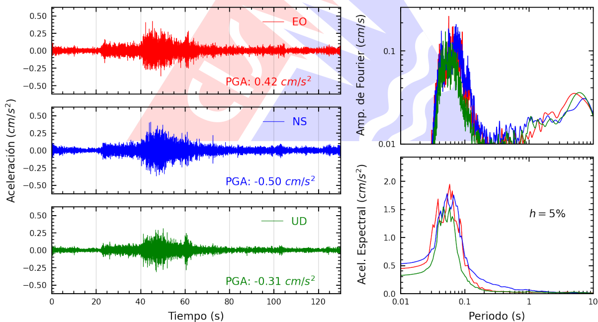
Figura A.2: Registros tiempo-historia, espectros de Fourier y de respuesta en las direcciones EO, NS y vertical de la estación JOSEO. Sismo de Tambo De Mora, Chincha - Ica del 2025-08-06, 13:24:45 (Hora local)
