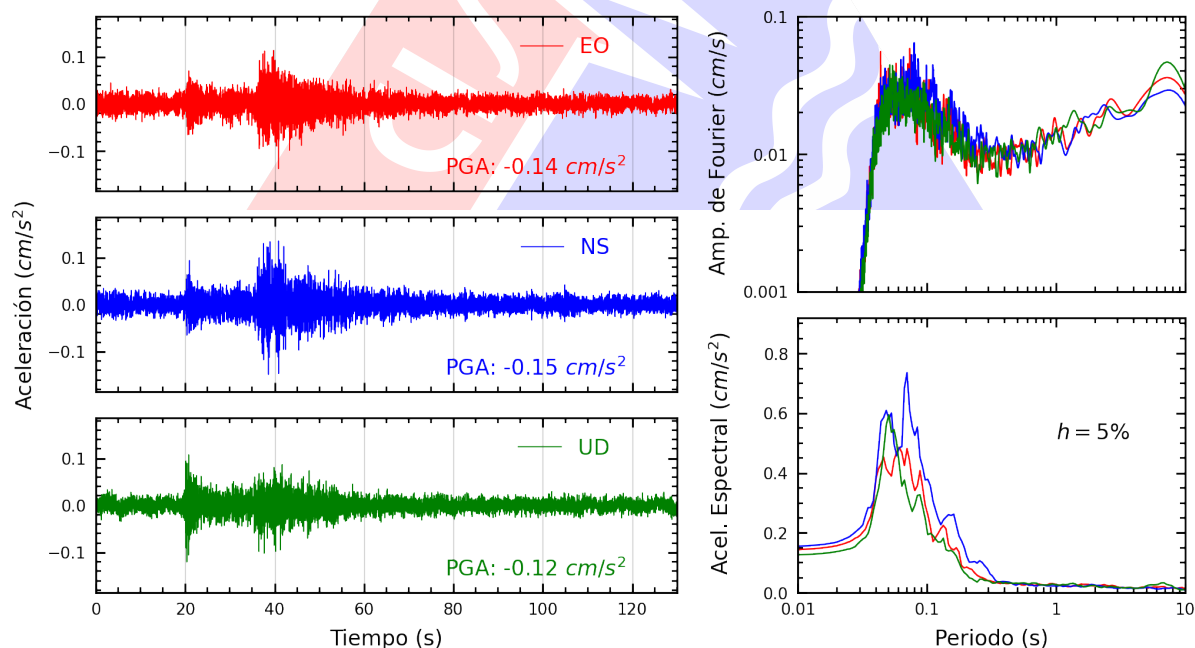
Figura A.8: Registros tiempo-historia, espectros de Fourier y de respuesta en las direcciones EO, NS y vertical de la estación SERVI. Sismo de Tambo De Mora, Chíncha - Ica del 2025-08-06, 13:24:45 (Hora local)
