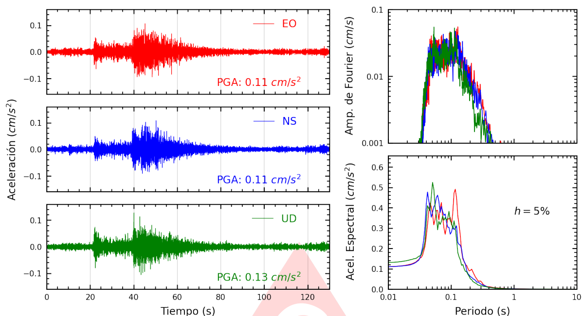
Figura A.9: Registros tiempo-historia, espectros de Fourier y de respuesta en las direcciones EO, NS y vertical de la estación JALV2. Sismo de Tambo De Mora, Chincha - Ica del 2025-08-06, 13:24:45 (Hora local)
