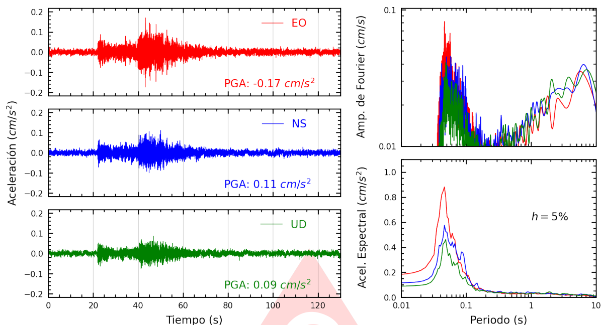
Figura A.7: Registros tiempo-historia, espectros de Fourier y de respuesta en las direcciones EO, NS y vertical de la estación UCSS. Sismo de Tambo De Mora, Chíncha - Ica del 2025-08-06, 13:24:45 (Hora local)
