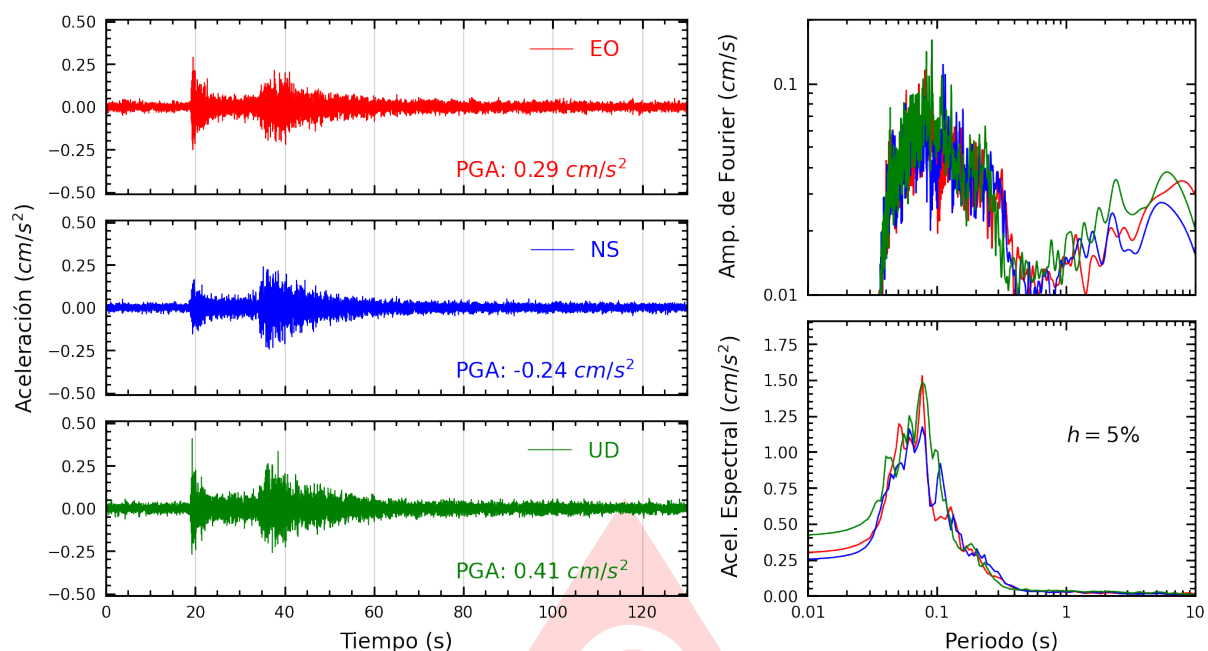
Figura A.3: Registros tiempo-historia, espectros de Fourier y de respuesta en las direcciones EO, NS y vertical de la estación SOVES. Sismo de Tambo De Mora, Chíncha - Ica del 2025-08-06, 13:24:45 (Hora local)
