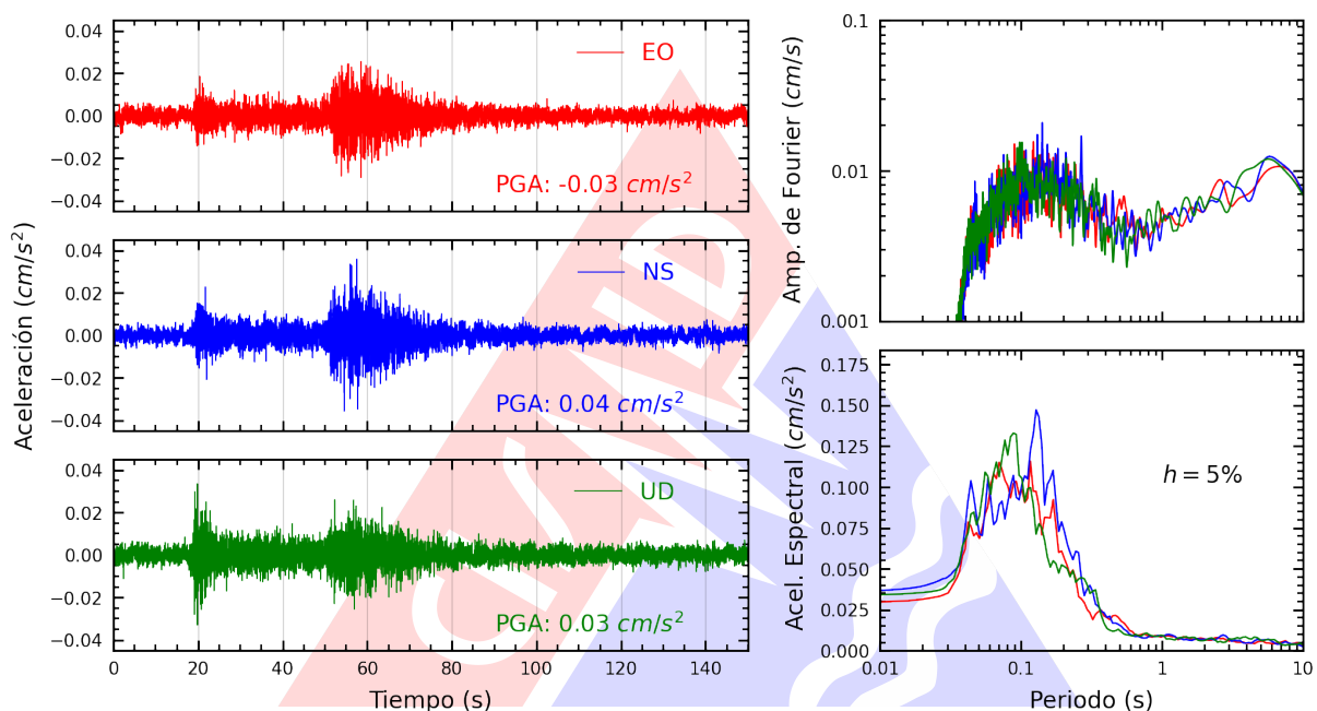
Figura A.11: Registros tiempo-historia, espectros de Fourier y de respuesta en las direcciones EO, NS y vertical de la estación CARAL. Sismo de Tambo De Mora, Chíncha - Ica del 2025-08-06, 13:24:45 (Hora local)
