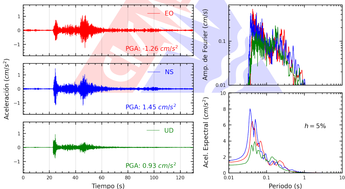
Figura A.2: Registros tiempo-historia, espectros de Fourier y de respuesta en las direcciones EO, NS y vertical de la estación UPTAC. Sismo de Capaso, El Collao - Puno del 2025-08-09, 04:34:44 (Hora local)
