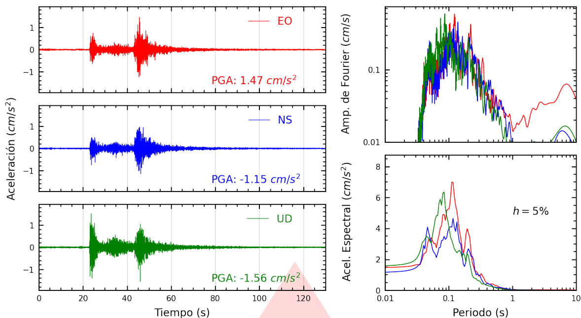
Figura A.1: Registros tiempo-historia, espectros de Fourier y de respuesta en las direcciones EO, NS y vertical de la estación UJBG3. Sismo de Capaso, El Collao - Puno del 2025-08-09, 04:34:44 (Hora local)
